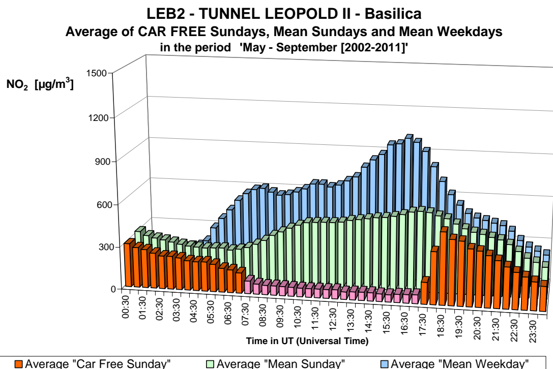
Fig. 28.b : NO 2 in de Leopold II tunnel, richting Basiliek – Gemiddelde Dagprofiel van de tien autoluwe zondagen en van alle zondagen en werkdagen in de periodes ‘mei – september 2002-2011’
