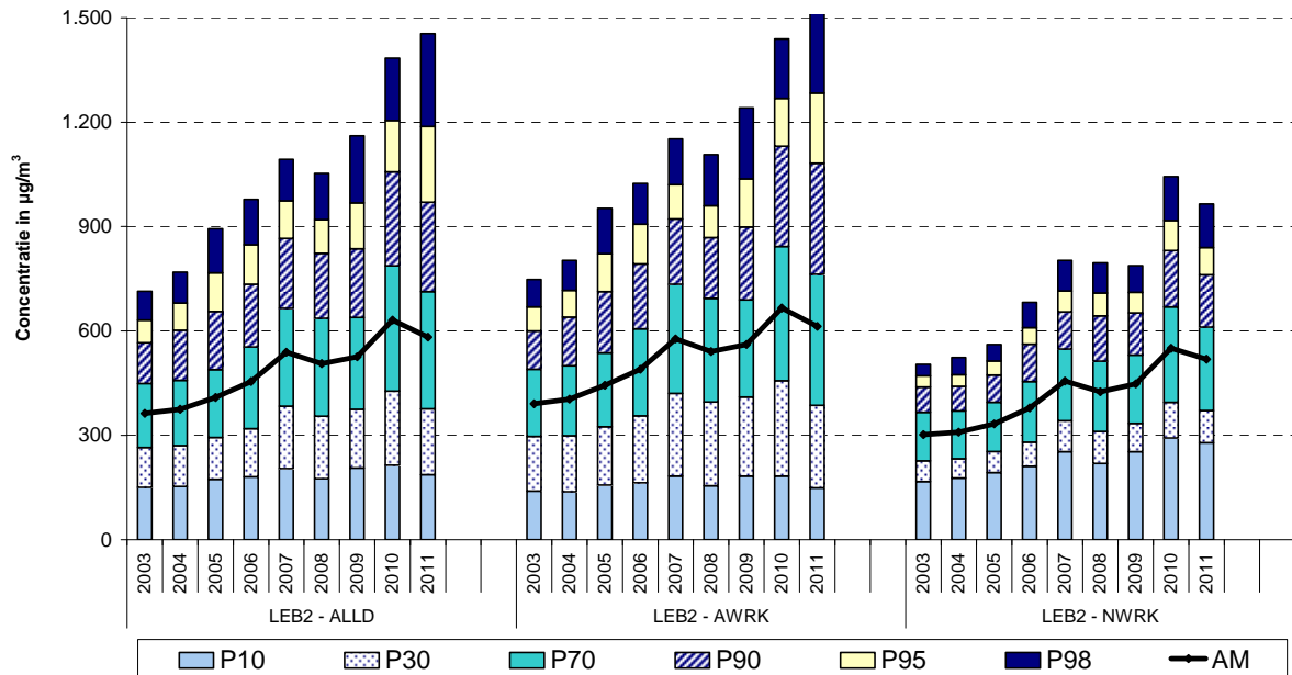
Fig. 5 : NO 2 - Cumulatieve Frequentieverdeling Uurwaarden in beide meetposten van de Leopold II tunnel. Selectie alle dagen , alle werkdagen en alle niet-werkdagen Jaarperiodes 2003 t/m 2011
