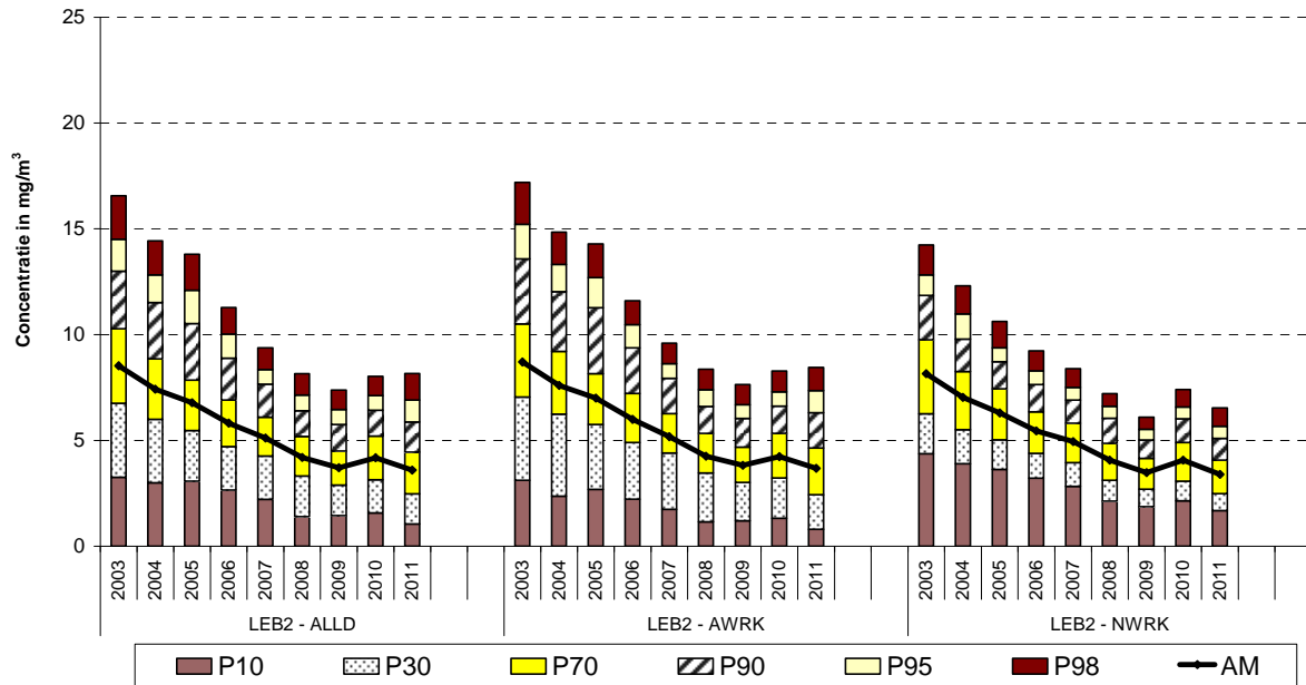
Fig. 6 : CO - Cumulatieve Frequentieverdeling Uurwaarden in beide meetposten van de Leopold II tunnel. Selectie alle dagen , alle werkdagen en alle niet-werkdagen Jaarperiodes 2003 t/m 2011
