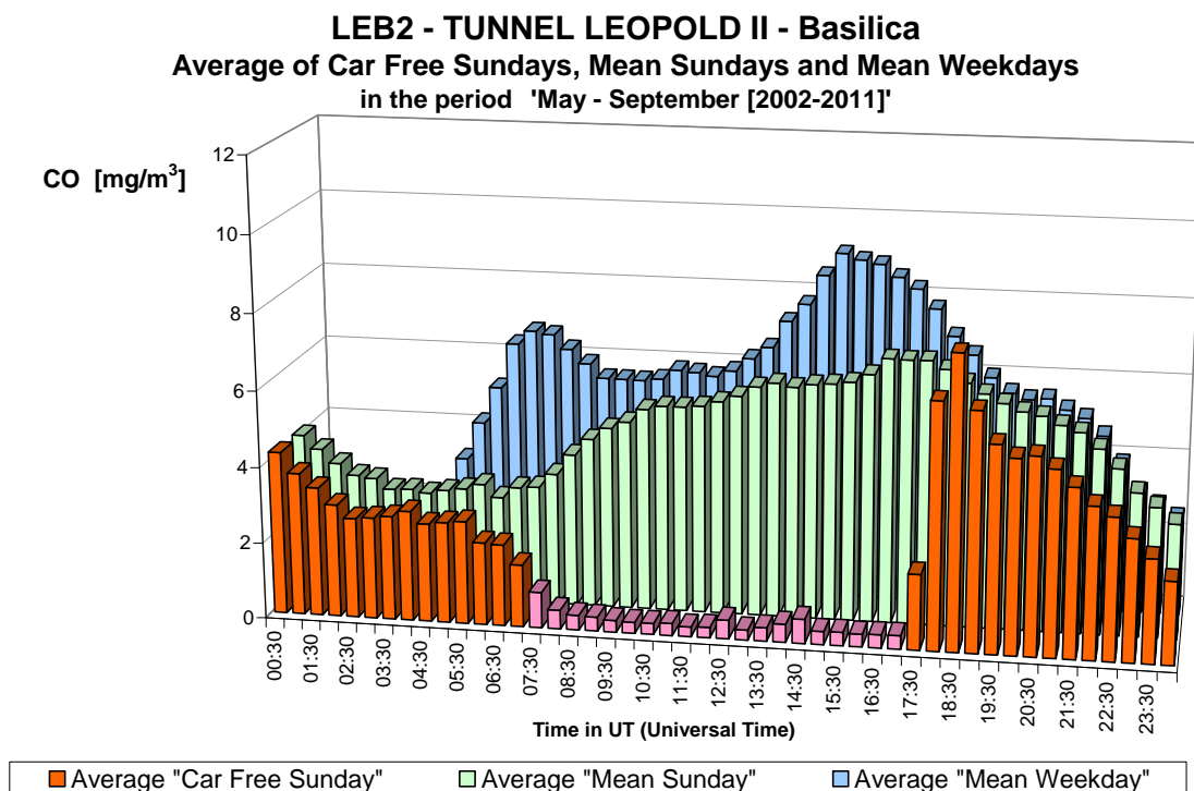
Fig. 32.b : CO in de Leopold II tunnel, richting Basiliek – Gemiddelde Dagprofiel van de tien autoluwe zondagen en van alle zondagen en werkdagen in de periodes 'mei – september 2002-2011'
