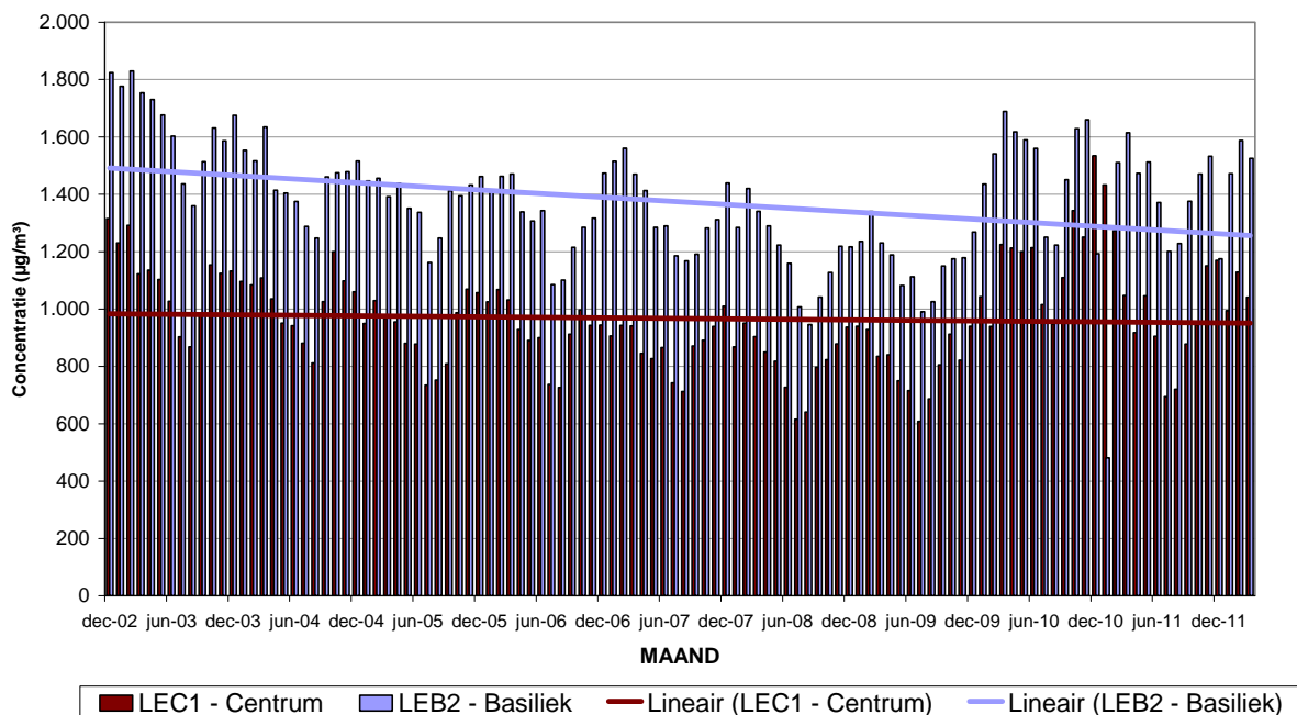
Fig. 9 : NO 2 en NO - Evolutie maandgemiddelde concentratie in beide meetposten van de Leopold II tunnel. Periode "December 2002 – Maart 2012"
