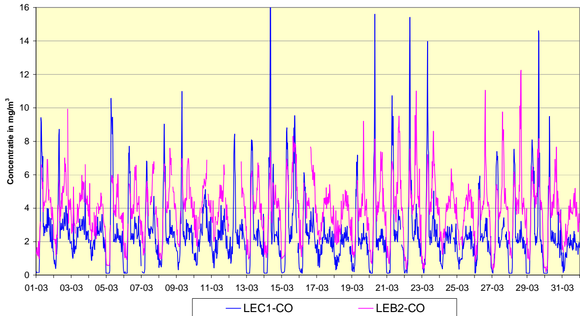
Fig. 3: CO - Evolutie van de uurwaarden en de halfuurwaarden tijdens de maand maart 2012 Meetplaats 41LEC1, richting Centrum - Meetplaats 41LEB2, richting Basiliek
