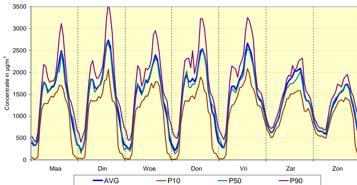
Fig. 26 : Meetpost 41LEB2 (basiliek) - Gemiddeld weekverloop voor NO Vergelijking winterperiode 2011 - 2012 en zomerperiode 2011
