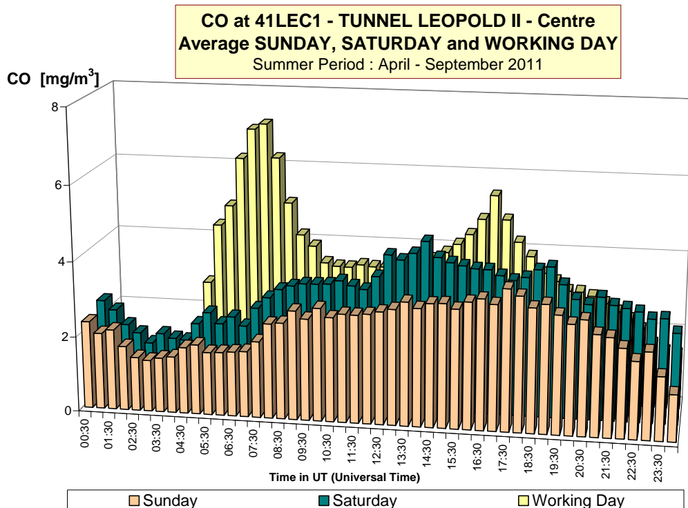
Fig. 19 : CO-dagverloop in de meetpost 41LEC1 (richting centrum) Vergelijking voor een gemiddelde zondag, zaterdag en werkdag Winterperiode 2011-2012 en zomerperiode 2011
