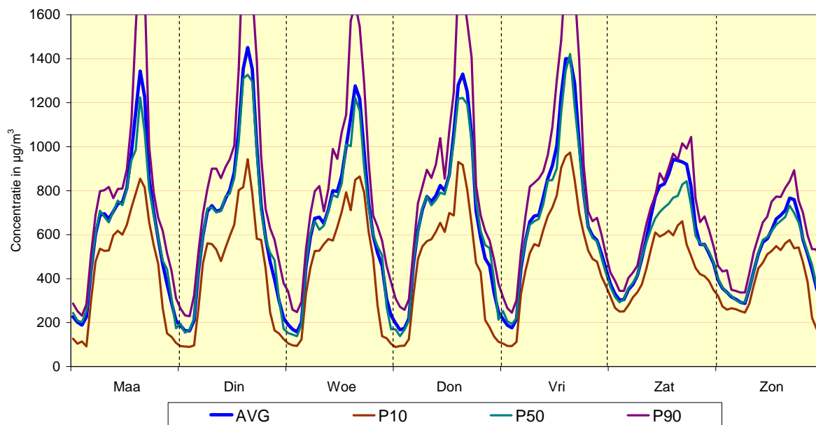
Fig. 22 : Meetpost 41LEB2 (basiliek) - Gemiddeld weekverloop voor NO 2 Vergelijking winterperiode 2011 - 2012 en zomerperiode 2011
