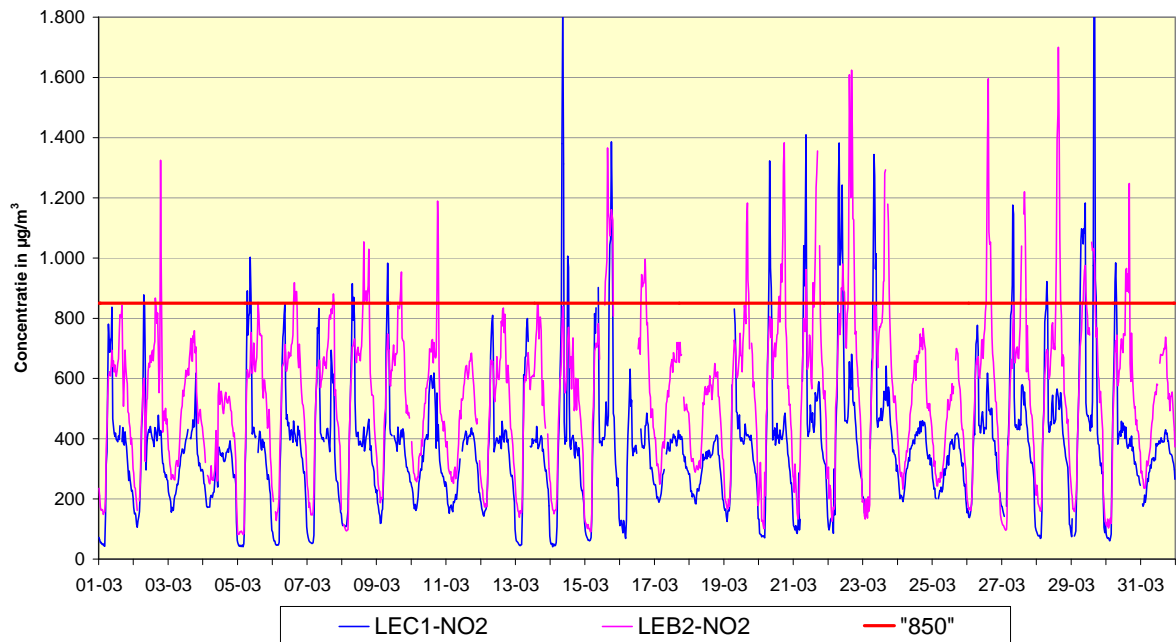
Fig. 1: NO 2 - Evolutie van de uurwaarden en de halfuurwaarden tijdens de maand maart 2012 Meetplaats 41LEC1, richting Centrum - Meetplaats 41LEB2, richting Basiliek
