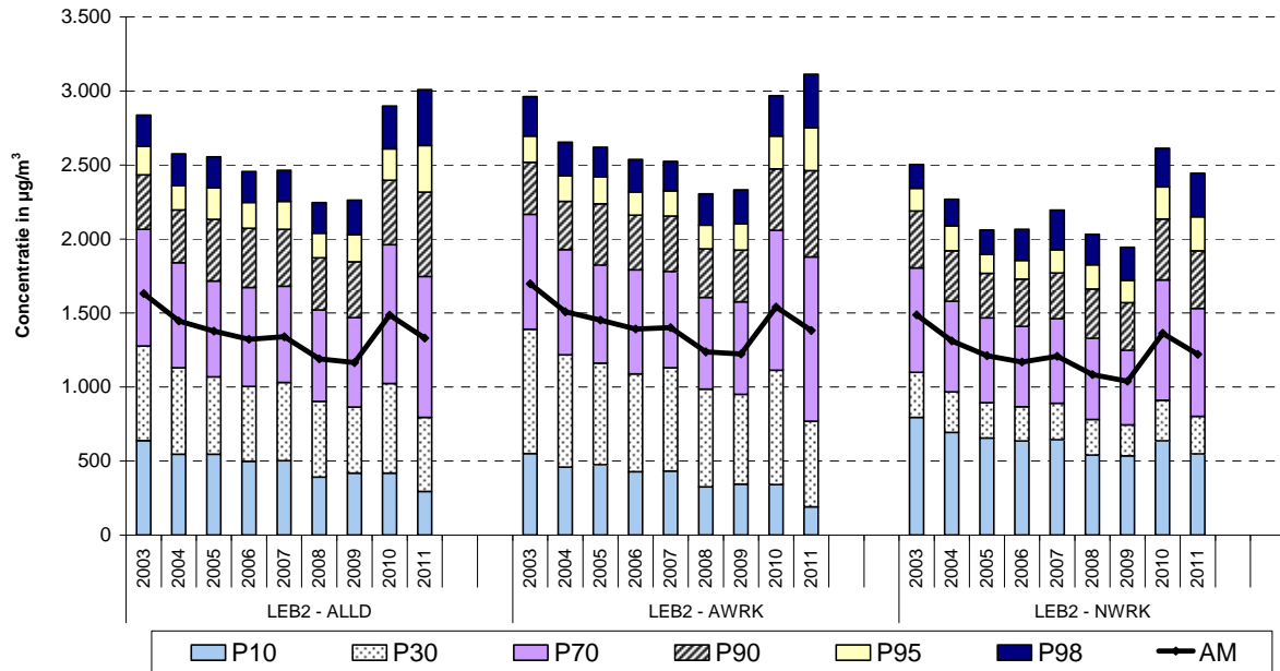
Fig. 7 : NO - Cumulatieve Frequentieverdeling Uurwaarden in beide meetposten van de Leopold II tunnel. Selectie alle dagen , alle werkdagen en alle niet-werkdagen Jaarperiodes 2003 t/m 2011
