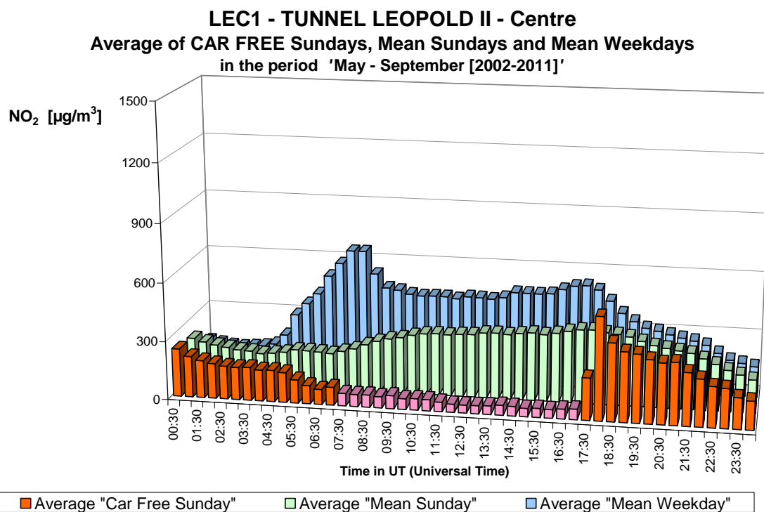
Fig. 27.b : NO 2 in de Leopold II tunnel, richting Centrum – Gemiddelde Dagprofiel van de tien autoluwte zondagen en van alle zondagen en werkdagen in de periodes ‘mei – september 2002-2011’
