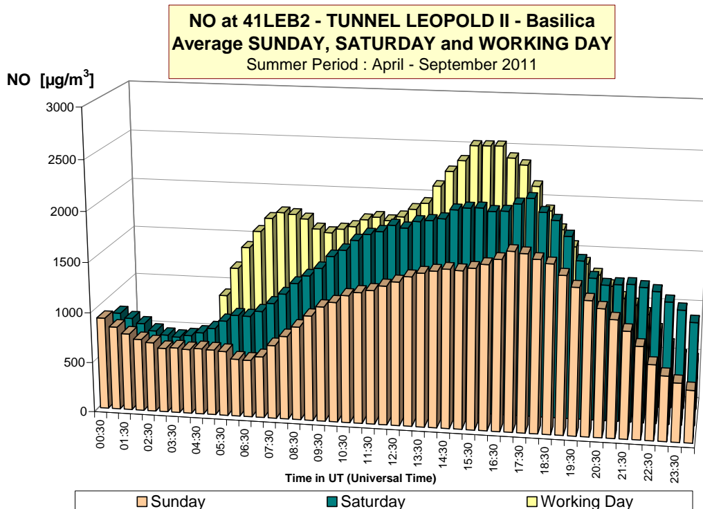
Fig. 18 : NO-dagverloop in de meetpost 41LEB2 (richting basiliek) Vergelijking voor een gemiddelde zondag, zaterdag en werkdag Winterperiode 2011-2012 en zomerperiode 2011
