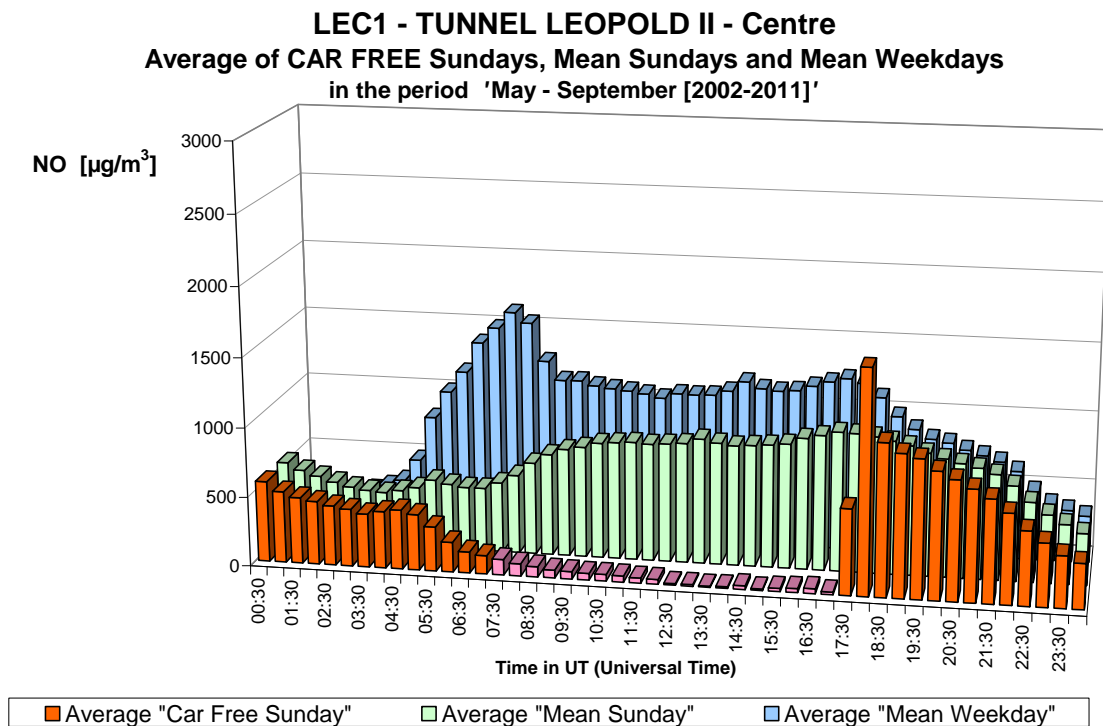
Fig. 29.b : NO in de Leopold II tunnel, richting Centrum – Gemiddelde Dagprofiel van de tien autoluwe zondagen en van alle zondagen en werkdagen in de periodes ‘mei – september 2002-2011’
