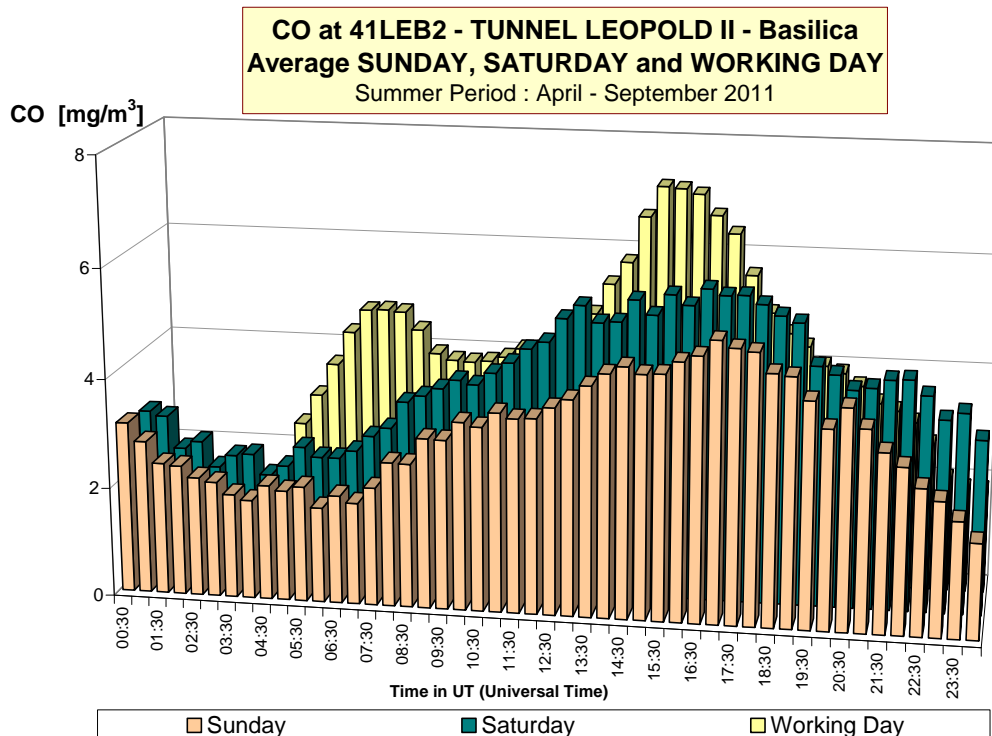
Fig. 20 : CO-dagverloop in de meetpost 41LEB2 (richting basiliek) Vergelijking voor een gemiddelde zondag, zaterdag en werkdag Winterperiode 2011-2012 en zomerperiode 2011
