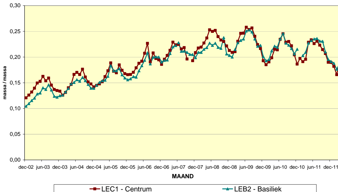
Fig. 11 : Evolutie van de verhouding NO 2 /NO x in beide meetposten van de Leopold II tunnel. Periode "December 2002 – Maart 2012"
