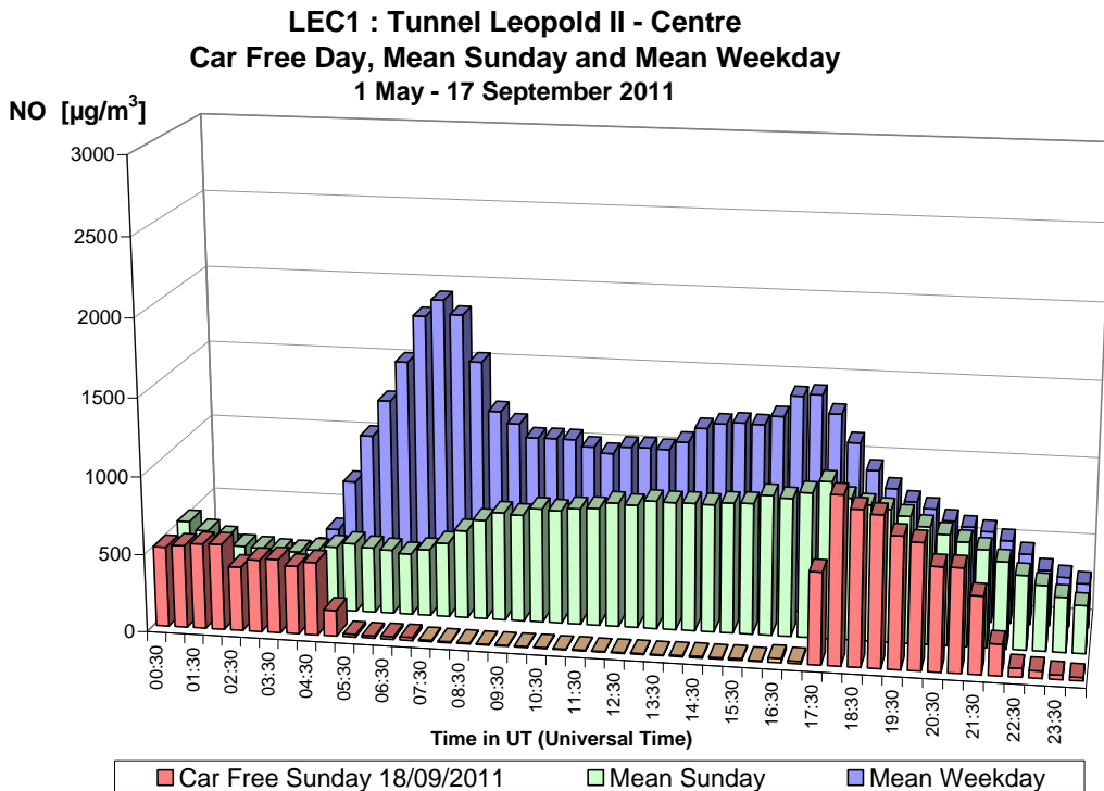
Fig. 29.a : NO in de Leopold II tunnel, richting Centrum – Dagprofiel autoluwe zondag 18-09-2011, gemiddelde zondag en gemiddelde werkdag in de periode ‘mei – september 2011’
