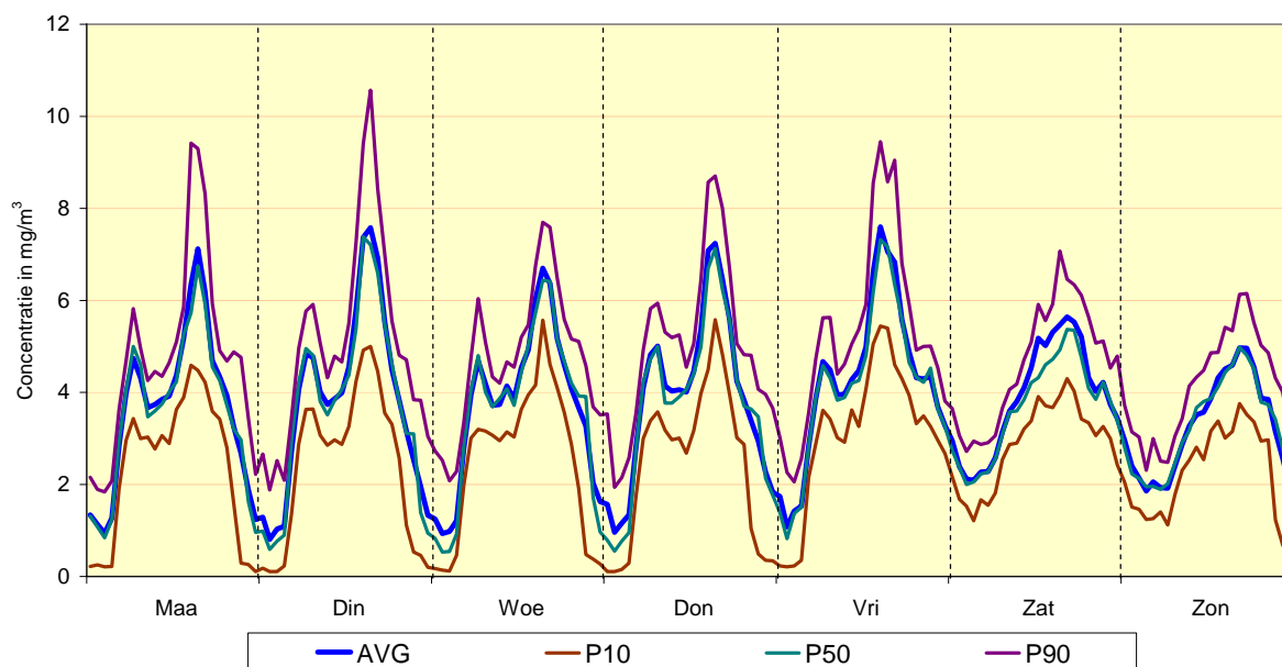
Fig. 24 : Meetpost 41LEB2 (basiliek) - Gemiddeld weekverloop voor CO Vergelijking winterperiode 2011 - 2012 en zomerperiode 2011
