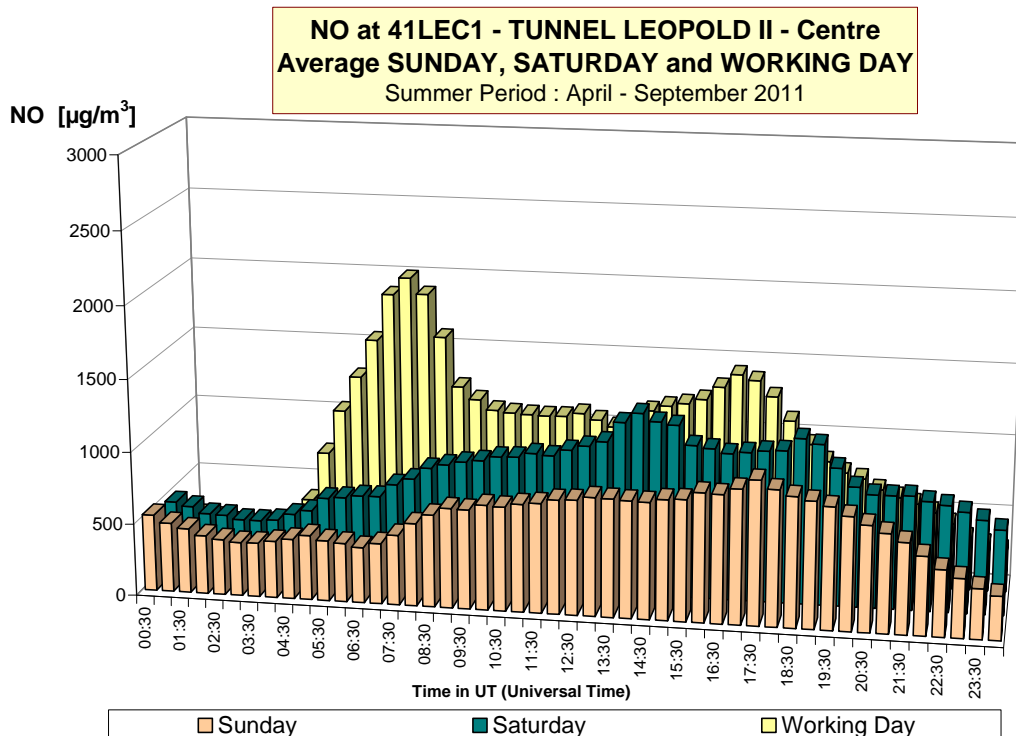
Fig. 17 : NO-dagverloop in de meetpost 41LEC1 (richting centrum) Vergelijking voor een gemiddelde zondag, zaterdag en werkdag Winterperiode 2011-2012 en zomerperiode 2011
