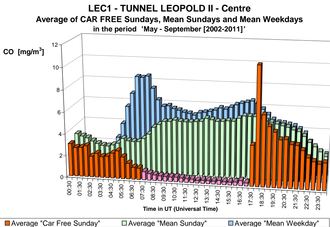
Fig. 31.b : CO in de Leopold II tunnel, richting Centrum – Gemiddelde Dagprofiel van de tien autoluwe zondagen en van alle zondagen en werkdagen in de periodes ‘mei – september 2002-2011’
