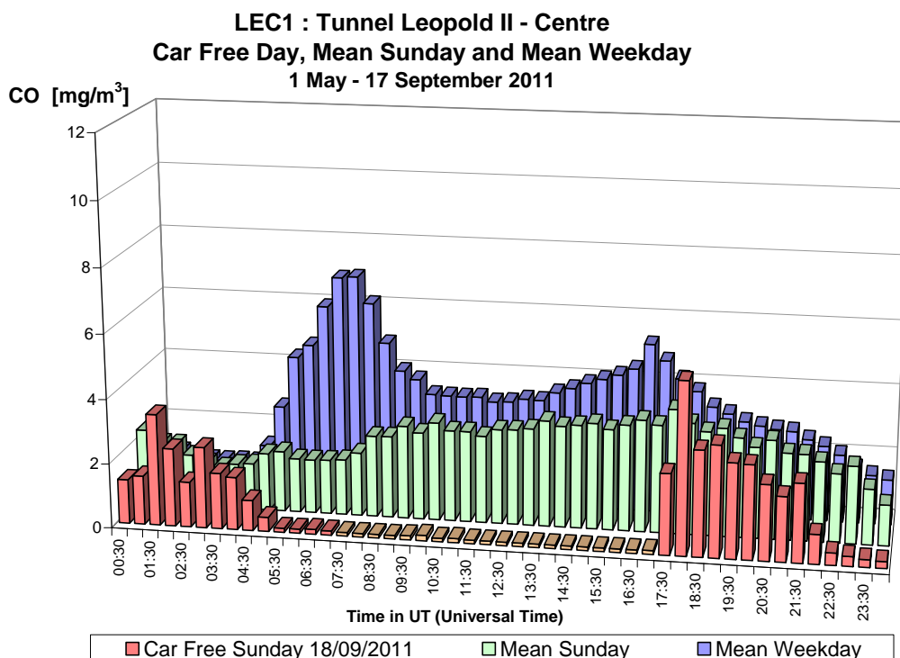
Fig. 31.a : CO in de Leopold II tunnel, richting Centrum – Dagprofiel autoluwe zondag 18-09-2011, gemiddelde zondag en gemiddelde werkdag in de periode ‘mei – september 2011’
