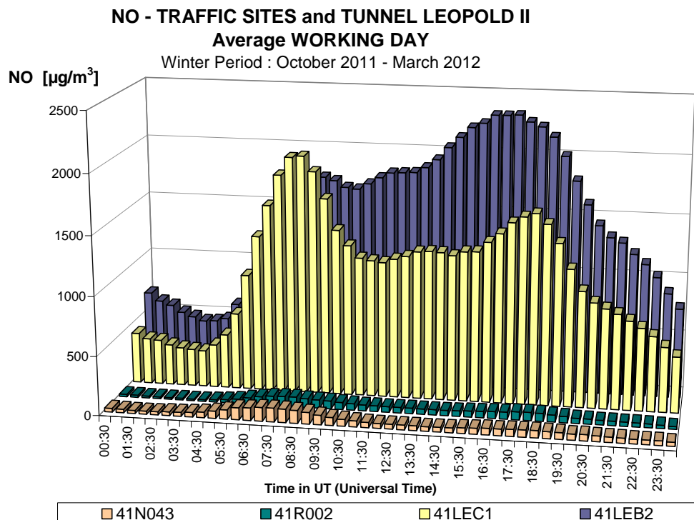
Fig. 34 : Dagverloop NO 2 en NO voor een gemiddelde werkdag tijdens de winter 2011-2012 Meetposten verkeer in de omgevingslucht – Voorhaven (N043) en Kroonlaan (R002) Meetposten in de tunnel Leopold II – LEC1 (centrum) en LEC2 (basiliek)
