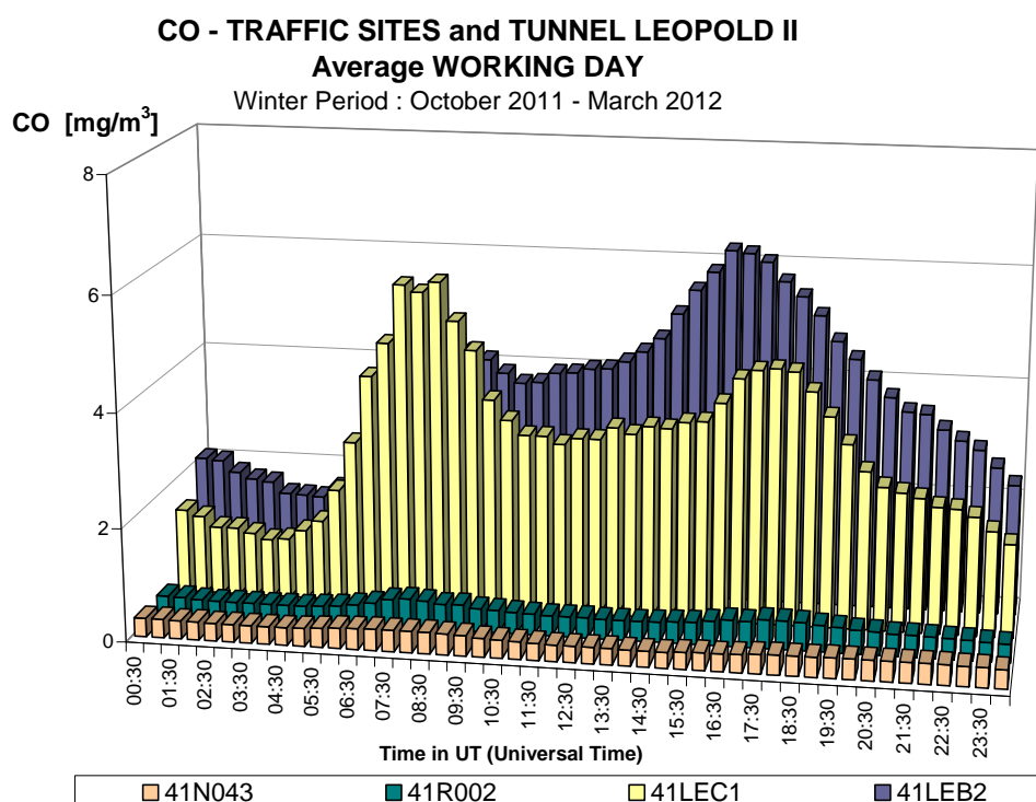
Fig. 33 : CO-dagverloop voor een gemiddelde werkdag tijdens de winter 2011-2012 Meetposten verkeer in de omgevingslucht – Voorhaven (N043) en Kroonlaan (R002) Meetposten in de tunnel Leopold II – LEC1 (centrum) en LEC2 (basiliek)
