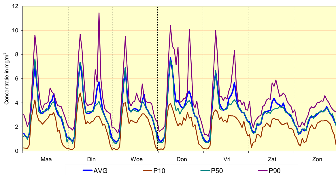
Fig. 23 : Meetpost 41LEC1 (centrum) - Gemiddeld weekverloop voor CO Vergelijking winterperiode 2011 - 2012 en zomerperiode 2011
