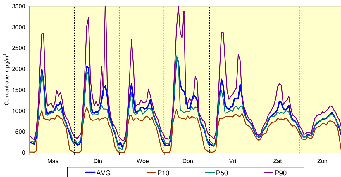
Fig. 25 : Meetpost 41LEC1 (centrum) - Gemiddeld weekverloop voor NO Vergelijking winterperiode 2011 - 2012 en zomerperiode 2011
