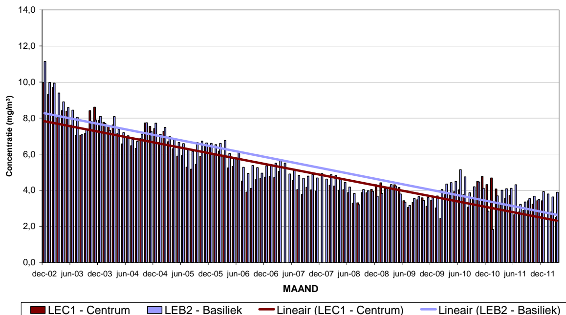
Fig. 10 : NO x en CO - Evolutie maandgemiddelde concentratie in beide meetposten van de Leopold II tunnel. Periode "December 2002 – Maart 2012"
