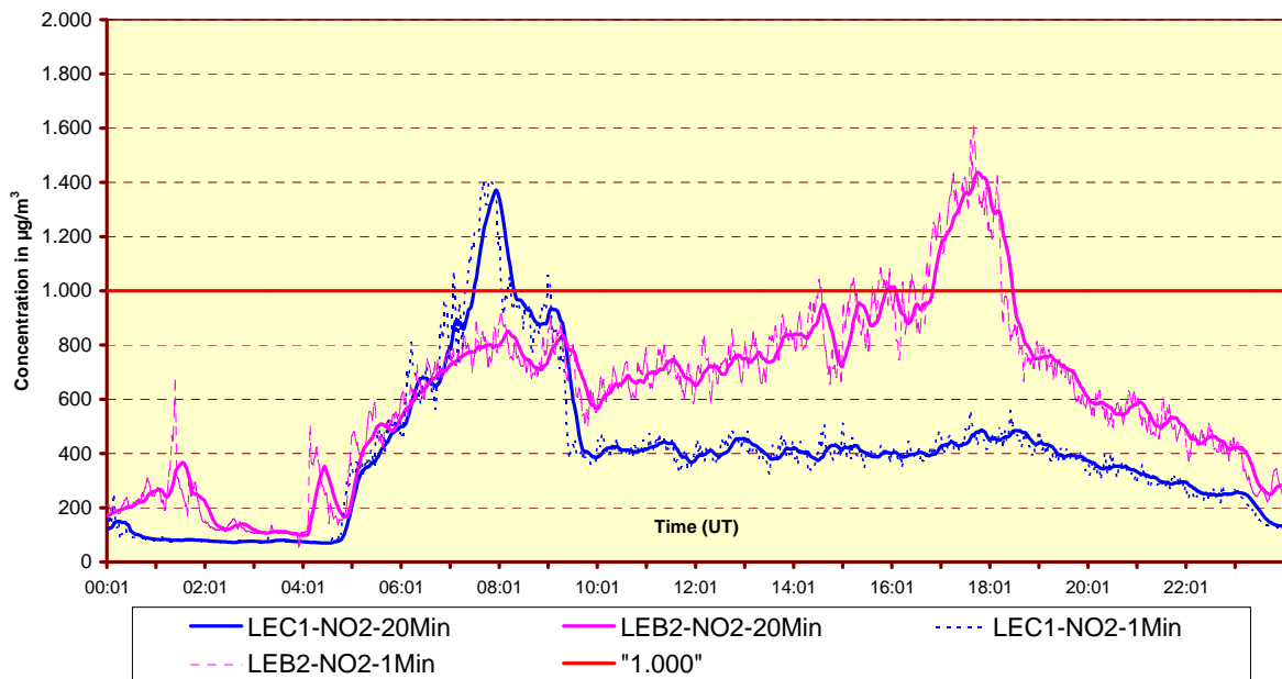
Fig. 4: NO 2 - evolutie minuutwaarden en voortschrijdend 20-minuutsgemiddelde in beide meetposten van de Leopold II tunnel Dinsdag 14 februari 2012 en dinsdag 20 maart 2012
