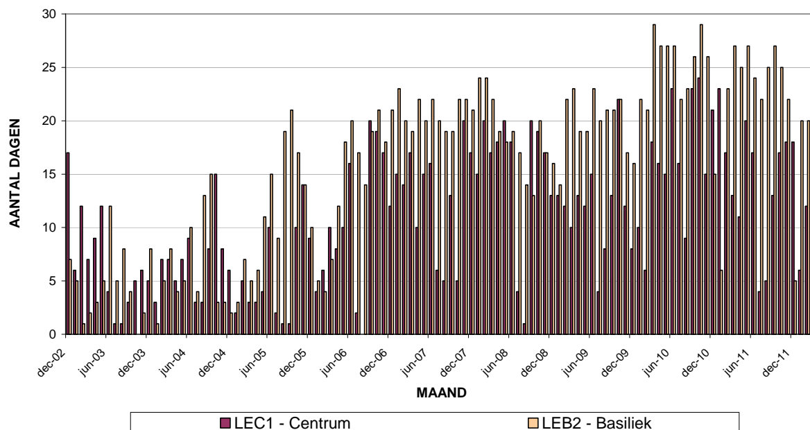
Fig. 13 : NO 2 – Halfuurswaarden > 850 µg/m 3 . Totaal aantal overschrijdingen per maand en aantal dagen per maand met overschrijding (december 2002 – maart 2012)
