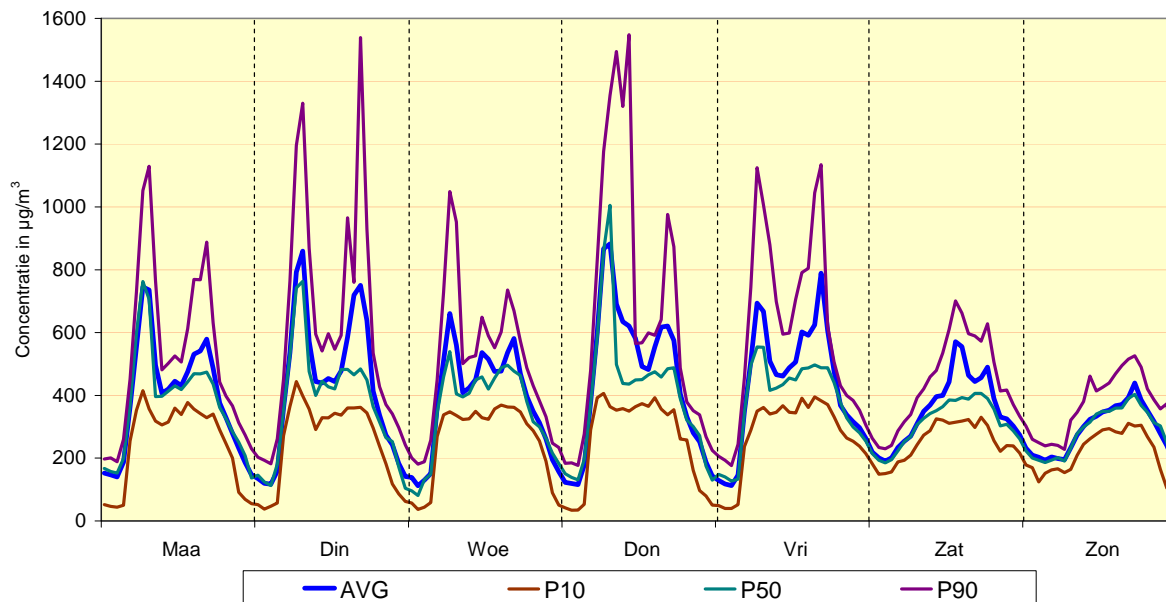
Fig. 21 : Meetpost 41LEC1 (centrum) - Gemiddeld weekverloop voor NO 2 Vergelijking winterperiode 2011 - 2012 en zomerperiode 2011
