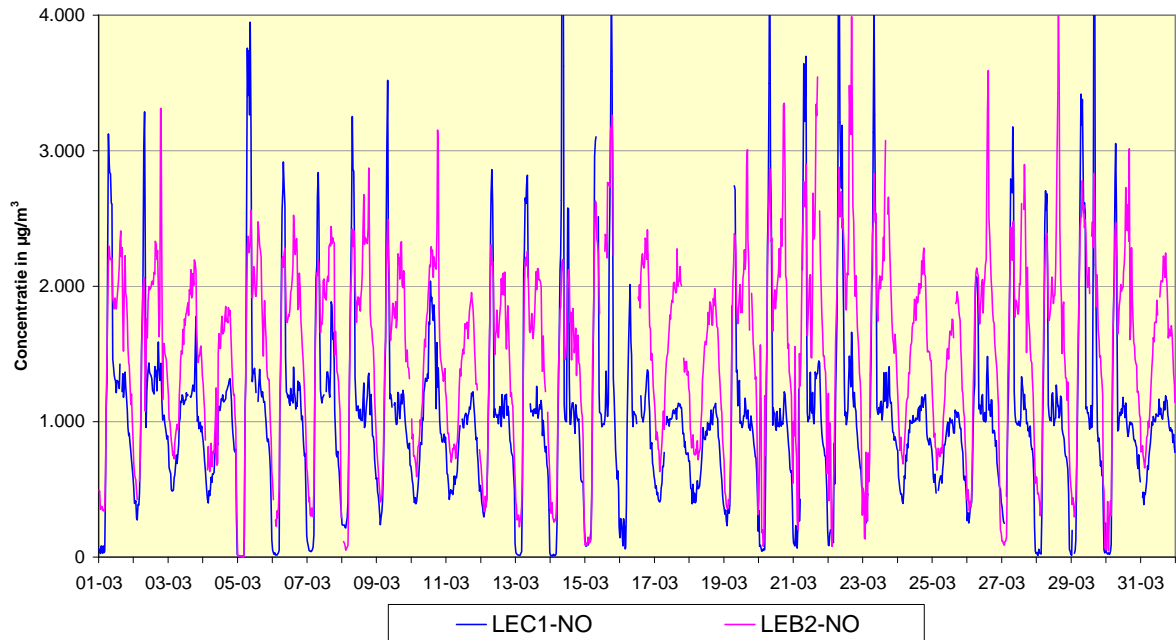
Fig. 2: NO - Evolutie van de uurwaarden en de halfuurwaarden tijdens de maand maart 2012 Meetplaats 41LEC1, richting Centrum - Meetplaats 41LEB2, richting Basiliek
