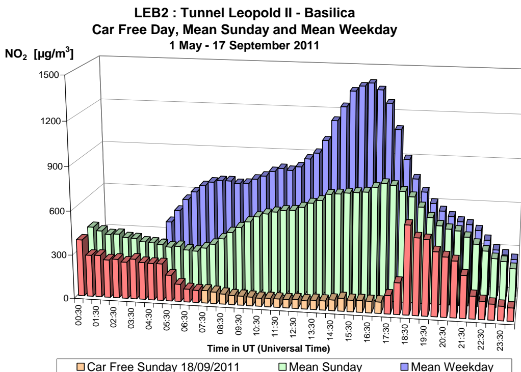
Fig. 28.a : NO 2 in de Leopold II tunnel, richting Basiliek – Dagprofiel autoluwe zondag 18-09-2011, gemiddelde zondag en een gemiddelde werkdag in de periode ‘mei – september 2011’
