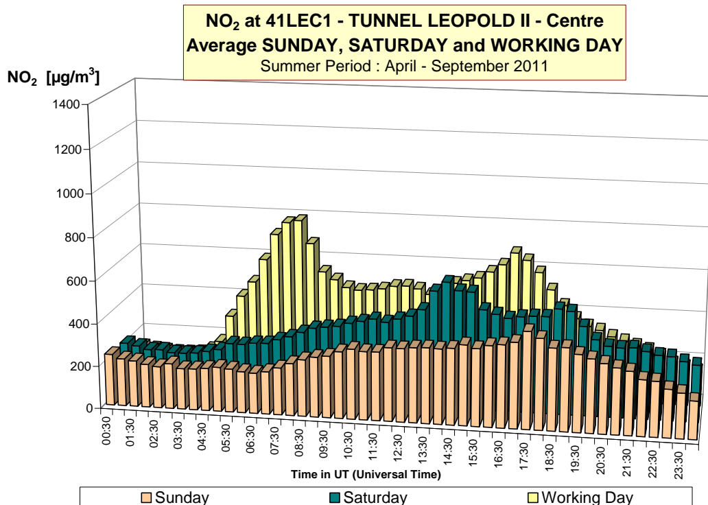
Fig. 15 : NO 2 -dagverloop in de meetpost 41LEC1 (richting centrum) Vergelijking voor een gemiddelde zondag, zaterdag en werkdag Winterperiode 2011-2012 en zomerperiode 2011
