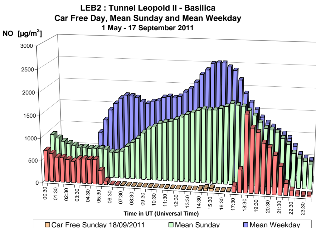
Fig. 30.a : NO in de Leopold II tunnel, richting Basiliek – Dagprofiel autoluwe zondag 18-09-2011, gemiddelde zondag en een gemiddelde werkdag in de periode 'mei – september 2011'
