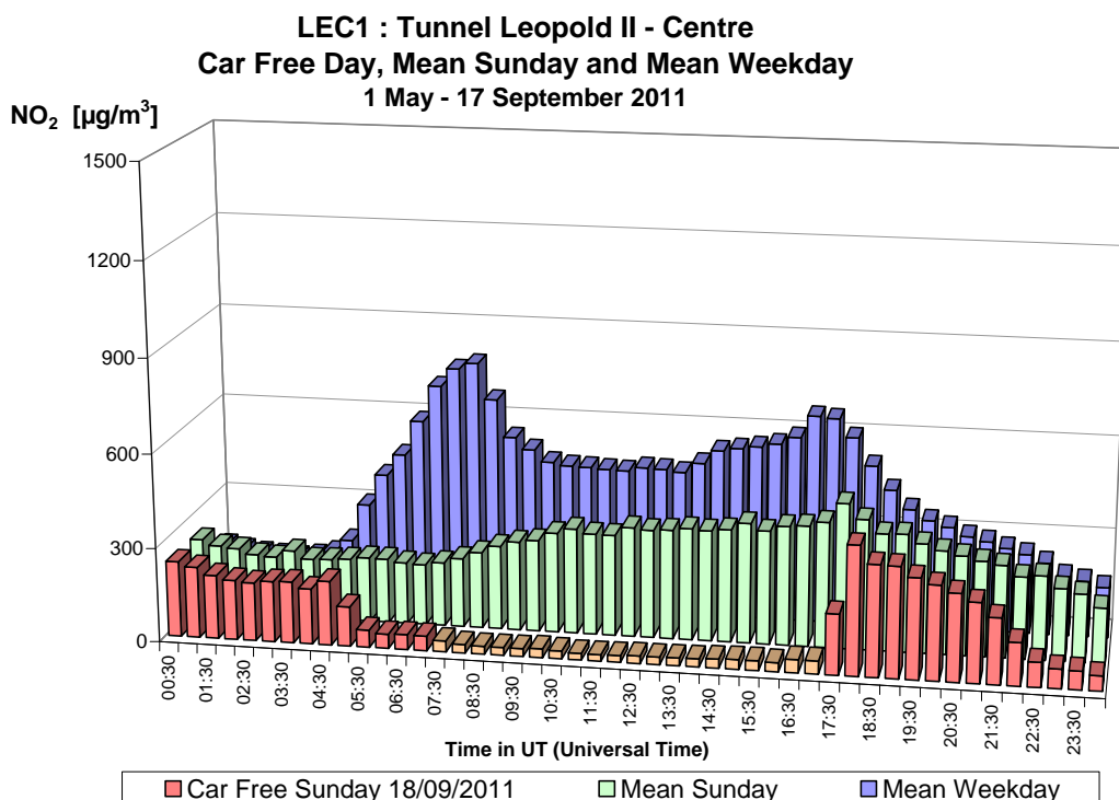
Fig. 27.a : NO 2 in de Leopold II tunnel, richting Centrum – Dagprofiel autoluwte zondag 18-09-2011, gemiddelde zondag en gemiddelde werkdag in de periode ‘mei – september 2011’
