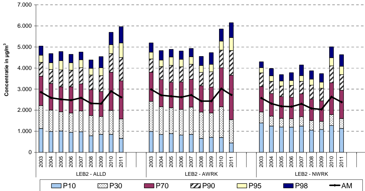
Fig. 8 : NO x - Cumulatieve Frequentieverdeling Uurwaarden in beide meetposten van de Leopold II tunnel. Selectie alle dagen , alle werkdagen en alle niet-werkdagen Jaarperiodes 2003 t/m 2011
