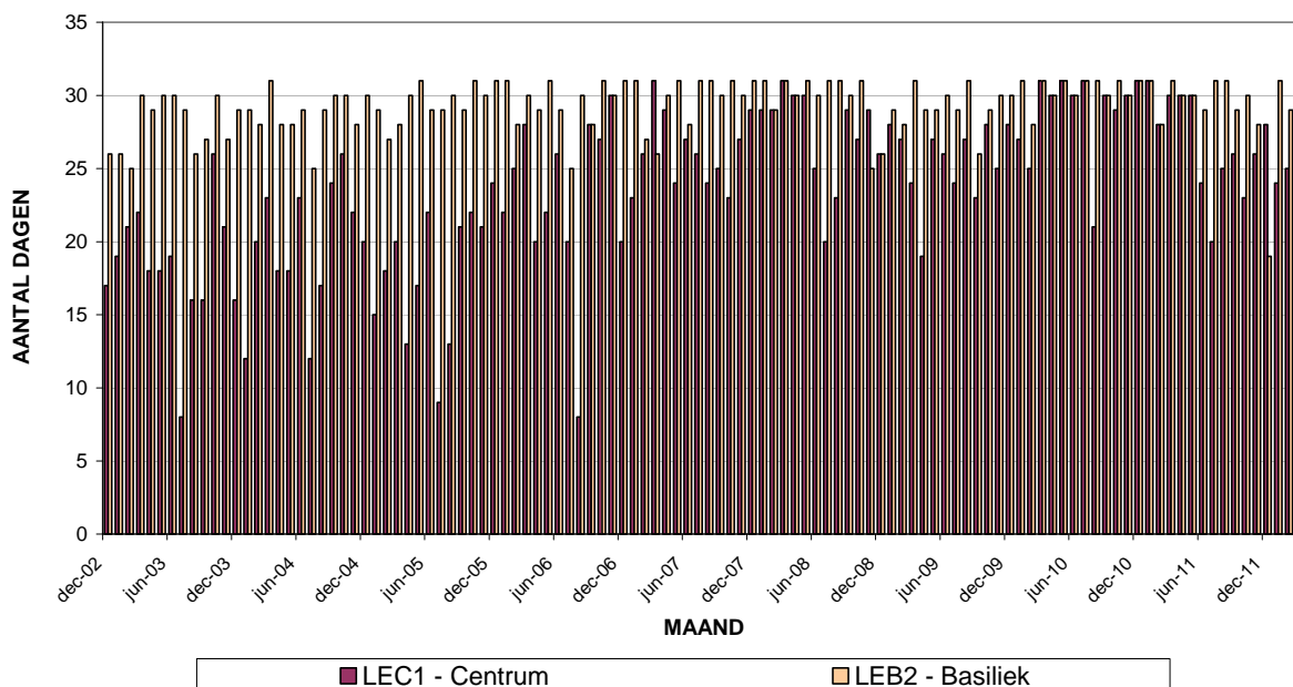
Fig. 14 : NO 2 -Uurwaarden > 400 µg/m 3 . Totaal aantal overschrijdingen per maand en aantal dagen per maand met overschrijding (december 2002 – maart 2012)
