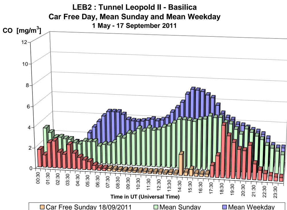
Fig. 32.a : CO in de Leopold II tunnel, richting Basiliek – Dagprofiel autoluwe zondag 18-09-2011, gemiddelde zondag en een gemiddelde werkdag in de periode 'mei – september 2011'
