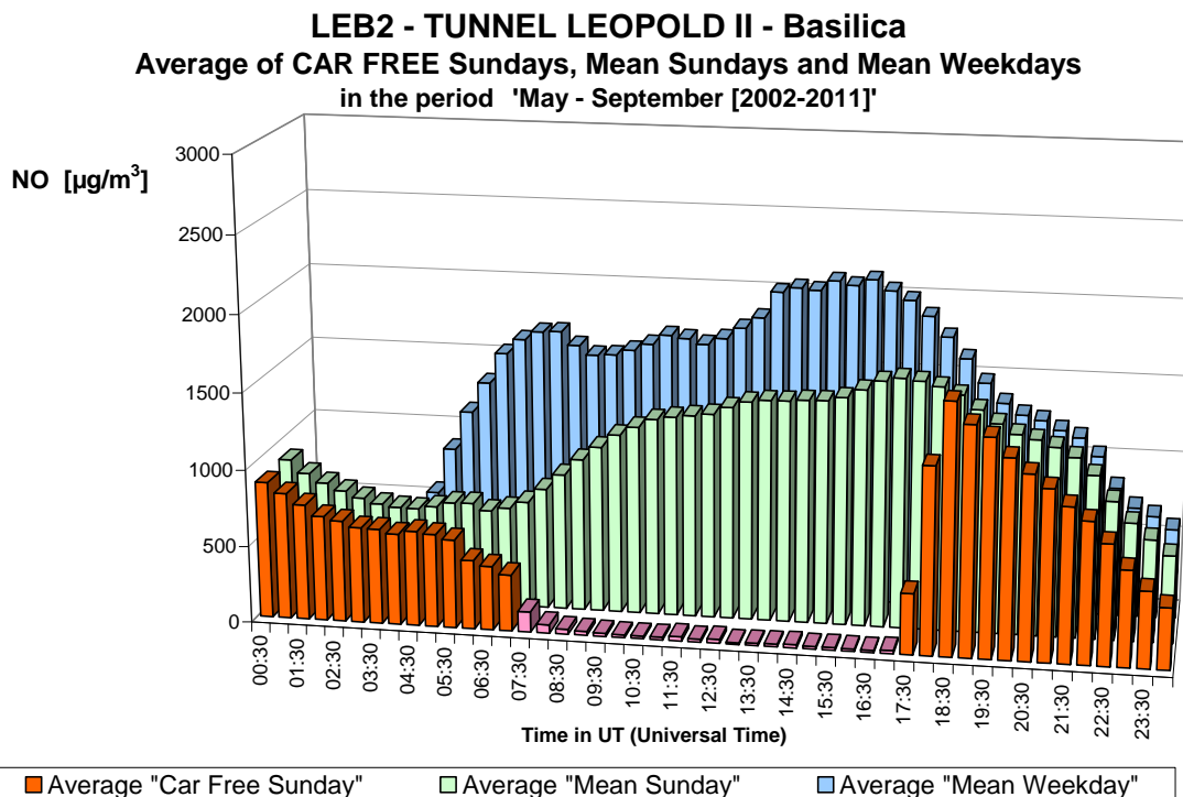
Fig. 30.b : NO in de Leopold II tunnel, richting Basiliek – Gemiddelde Dagprofiel van de tien autoluwe zondagen en van alle zondagen en werkdagen in de periodes 'mei – september 2002-2011'
