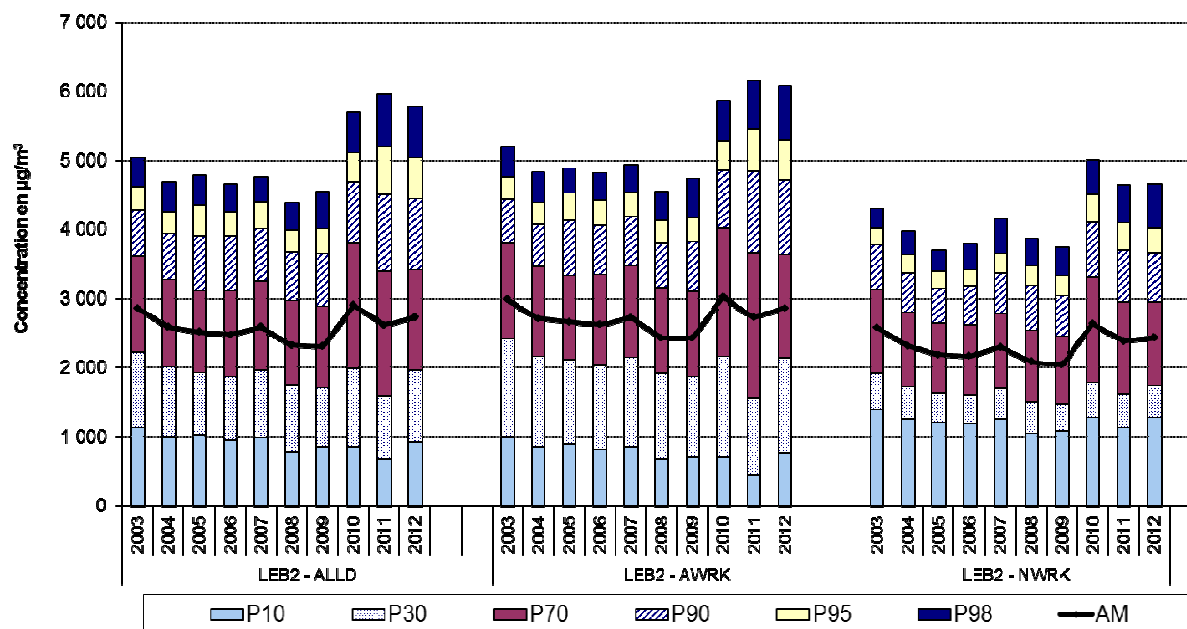
Fig. 8 : NO x - Distribution de Fréquences Cumulées des Valeurs Horaires dans les deux postes de mesure du tunnel Léopold II. Sélection tous les jours , les jours ouvrables et non ouvrables . Périodes annuelles de 2003 à 2012
