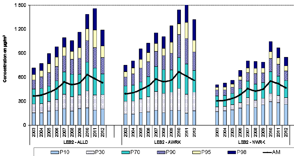
Fig. 5 : NO 2 - Distribution de Fréquences Cumulées des Valeurs Horaires dans les deux postes de mesure du tunnel Léopold II. Sélection tous les jours , les jours ouvrables et non ouvrables . Périodes annuelles de 2003 à 2012
