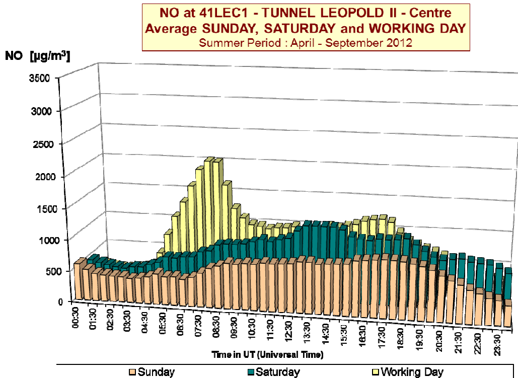
Fig. 17 : NO – évolution journalière moyenne au poste de mesure 41LEC1 (centre) Comparaison entre un dimanche, un samedi et un jour ouvrable moyen Période hivernale 2012-2013 et période estivale 2012
