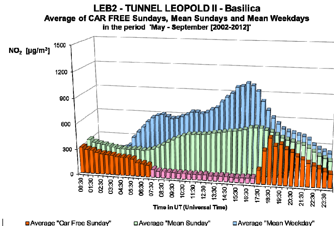
Fig. 28.b : NO 2 dans le tunnel Léopold II, direction Basilique – Profil journalier sur les onze dimanches sans voiture et sur tous les dimanches et jours ouvrables des périodes 'mai – septembre 2002-2012'.
