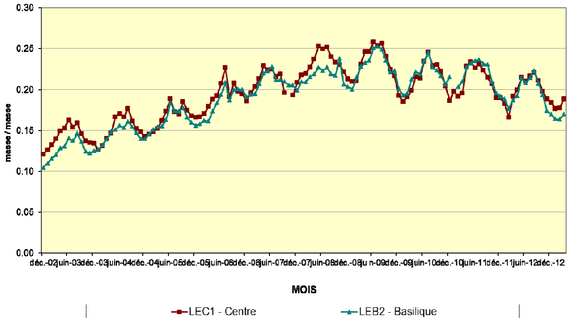
Fig. 11 : Évolution du rapport NO 2 /NO x dans les deux postes de mesure du tunnel Léopold II. Période – « Décembre 2002 – Mars 2013 »
