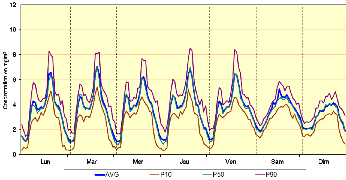
Fig. 24 : Poste de Mesure 41LEB2 (basilique) – Évolution hebdomadaire moyenne pour le CO Période hivernale 2012 - 2013 et période estivale 2012
