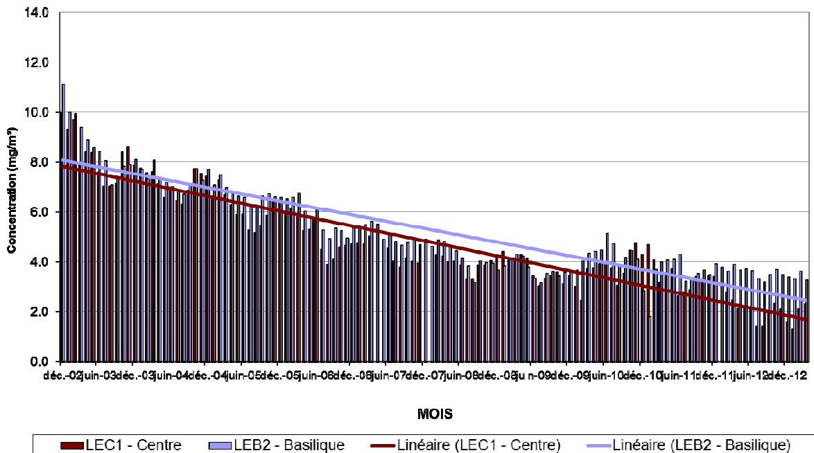
Fig. 10 : NO x et CO – Évolution des concentrations moyennes mensuelles dans les deux postes de mesure du tunnel Léopold II. Période – « Décembre 2002 – Mars 2013 »
