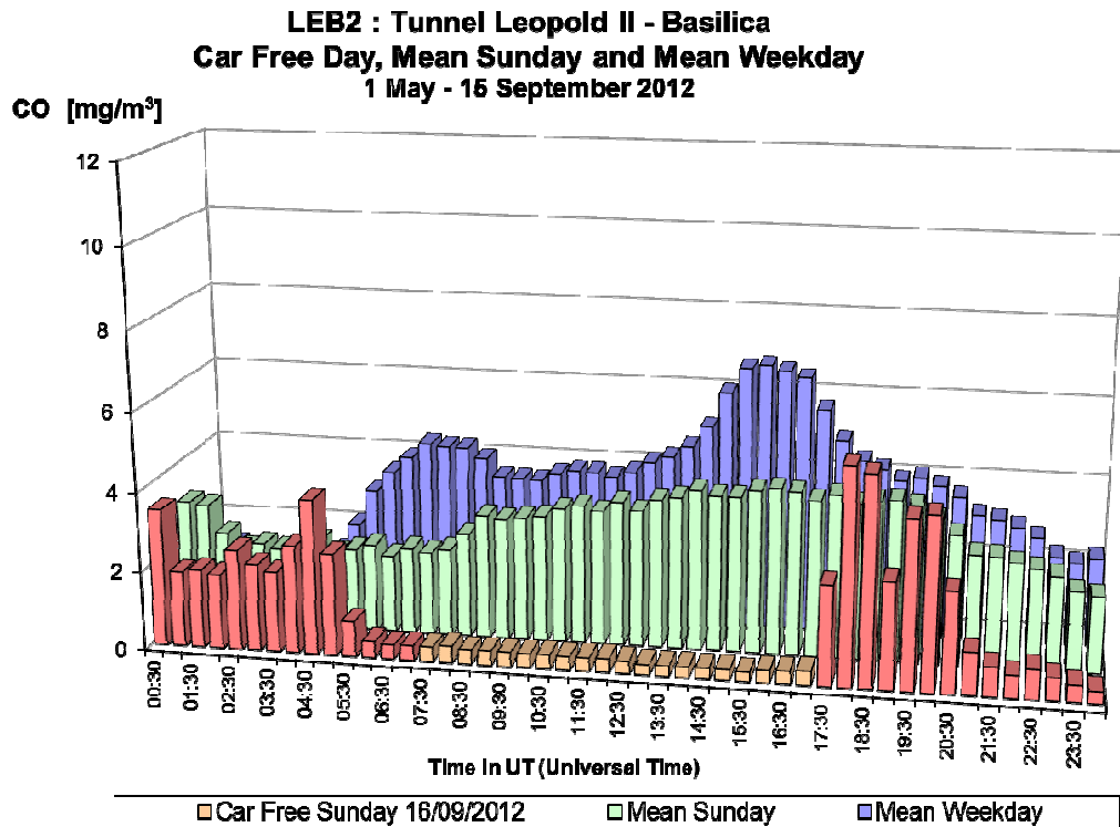
Fig. 32.a : CO dans le tunnel Léopold II, direction Basilique – Profil journalier du dimanche sans voiture, d'un dimanche moyen et d'un jour ouvrable moyen de la période 'mai – septembre 2012'.
