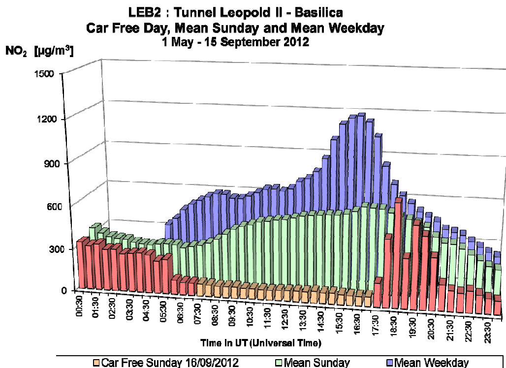
Fig. 28.a : NO 2 dans le tunnel Léopold II, direction Basilique – Profil journalier du dimanche sans voiture, d'un dimanche moyen et d'un jour ouvrable moyen de la période 'mai – septembre 2012'.
