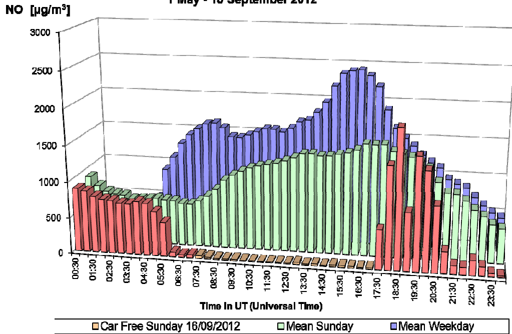
Fig. 30.a : NO dans le tunnel Léopold II, direction Basilique – Profil journalier du dimanche sans voiture, d'un dimanche moyen et d'un jour ouvrable moyen de la période 'mai – septembre 2012'.
