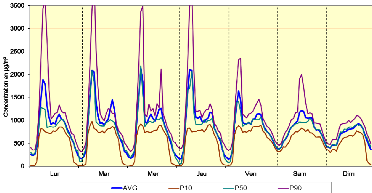
Fig. 25 : Poste de Mesure 41LEC1 (centre) – Évolution hebdomadaire moyenne pour le NO Période hivernale 2012 - 2013 et période estivale 2012
