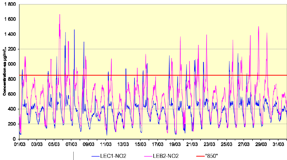
Fig. 1: NO 2 - Évolution des valeurs horaires et semi horaires en mars 2013 Poste de mesure 41LEC1, direction Centre – Poste de mesure 41LEB2, direction Basilique
