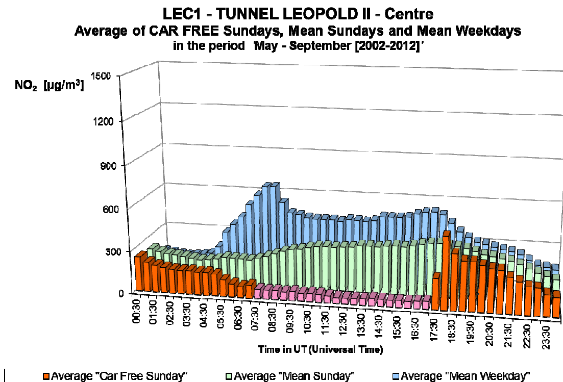
Fig. 27.b : NO 2 dans le tunnel Léopold II, direction Centre – Profil journalier sur les onze dimanches sans voiture et sur tous les dimanches et jours ouvrables des périodes 'mai – septembre 2002-2012'.
