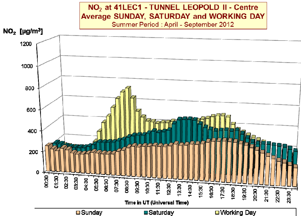
Fig. 15 : NO 2 – évolution journalière moyenne au poste de mesure 41LEC1 (centre) Comparaison entre un dimanche, un samedi et un jour ouvrable moyen Période hivernale 2012-2013 et période estivale 2012
