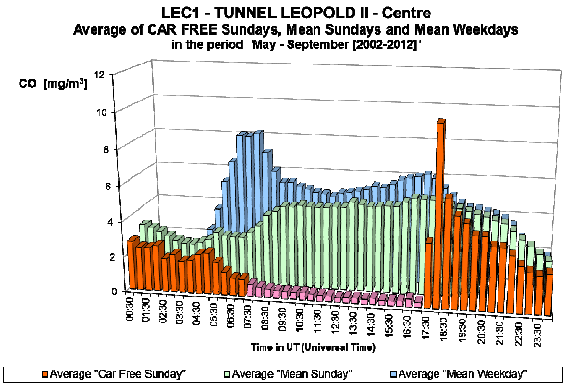
Fig. 31.b : CO dans le tunnel Léopold II, direction Centre – Profil journalier sur les onze dimanches sans voiture et sur tous les dimanches et jours ouvrables des périodes 'mai – septembre 2002-2012'.
