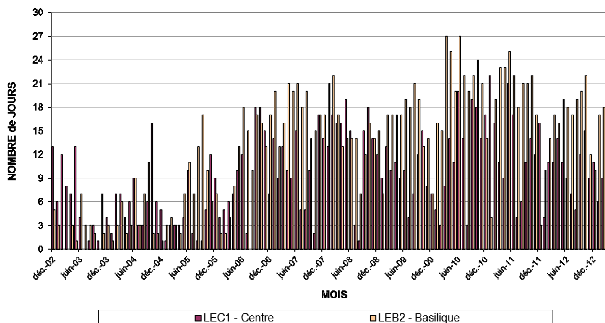
Fig. 12 : NO 2 –Moyennes glissantes sur 20 minutes > 1.000 µg/m 3 . Nombre de dépassements par mois et nombre de jours par mois avec dépassements (décembre 2002 – mars 2013)
