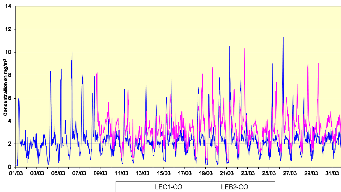
Fig. 3: CO - Évolution des valeurs horaires et semi horaires en mars 2013 Poste de mesure 41LEC1, direction Centre – Poste de mesure 41LEB2, direction Basilique
