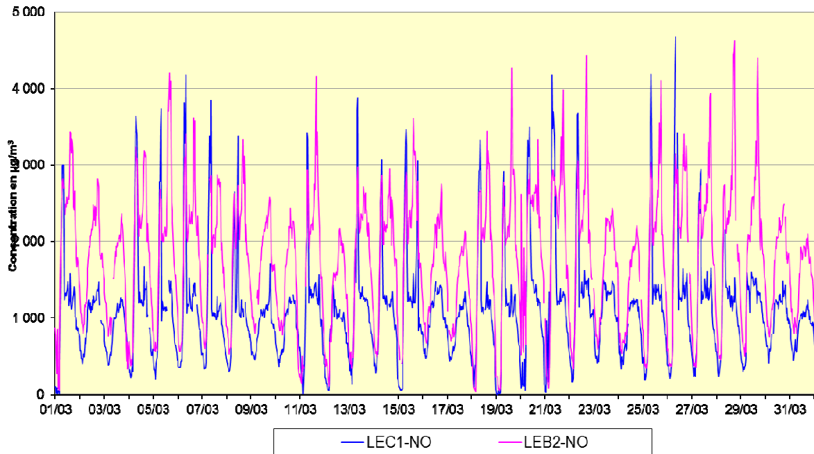
Fig. 2: NO - Évolution des valeurs horaires et semi horaires en mars 2013 Poste de mesure 41LEC1, direction Centre – Poste de mesure 41LEB2, direction Basilique
