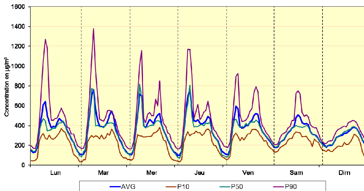
Fig. 21 : Poste de Mesure 41LEC1 (centre) – Évolution hebdomadaire moyenne pour le NO 2 Période hivernale 2012 - 2013 et période estivale 2012
