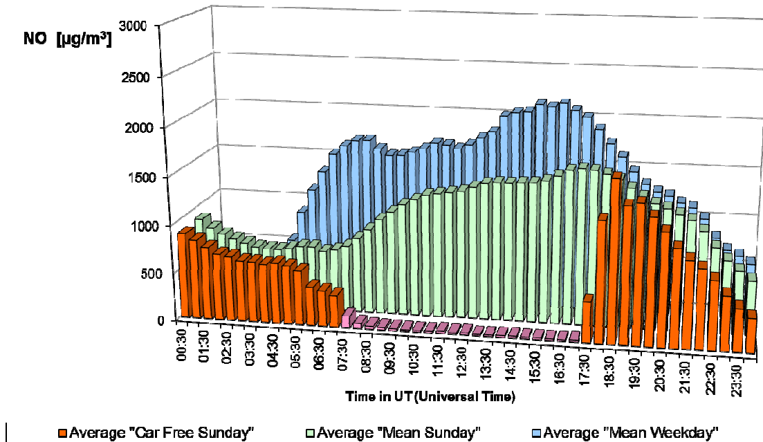
Fig. 30.b : NO dans le tunnel Léopold II, direction Basilique – Profil journalier sur les onze dimanches sans voiture et sur tous les dimanches et jours ouvrables des périodes 'mai – septembre 2002-2012'.
