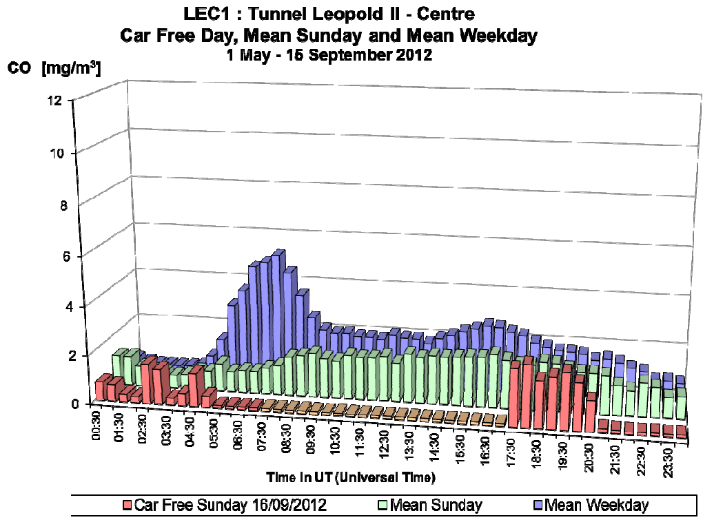
Fig. 31.a : CO dans le tunnel Léopold II, direction Centre – Profil journalier du dimanche sans voiture 16-09-2012, d'un dimanche moyen et d'un jour ouvrable moyen de la période 'mai – septembre 2012'.
