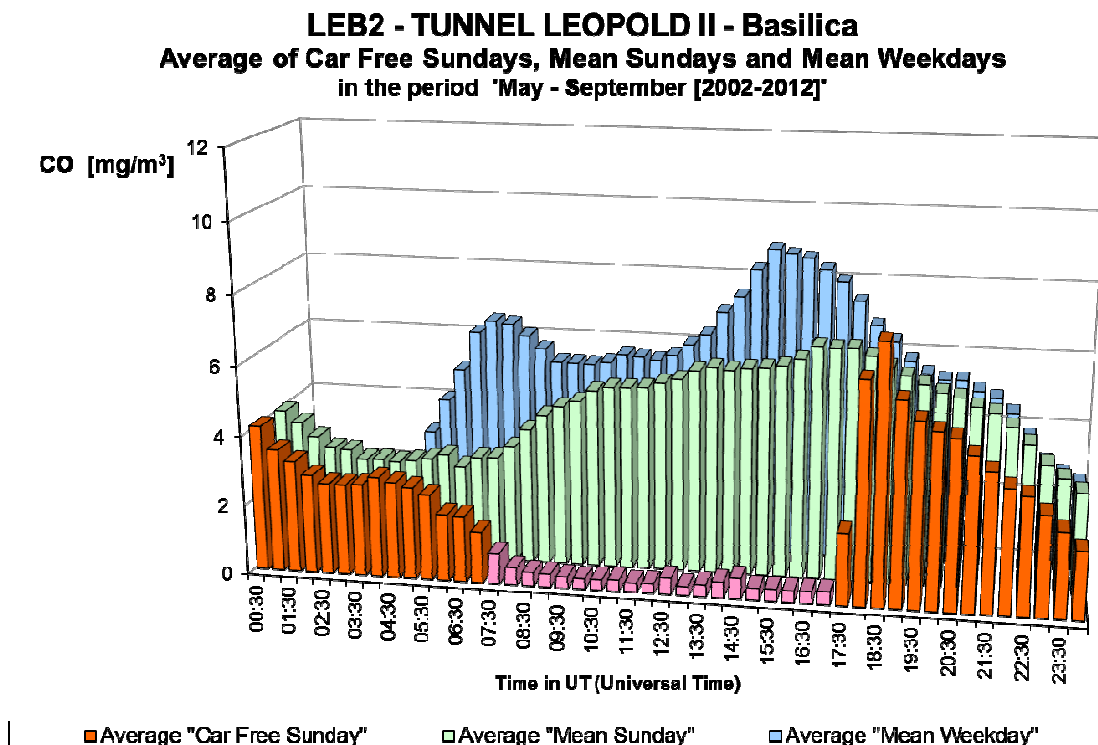
Fig. 32.b : CO dans le tunnel Léopold II, direction Basilique – Profil journalier sur les onze dimanches sans voiture et sur tous les dimanches et jours ouvrables des périodes 'mai – septembre 2002-2012'.
