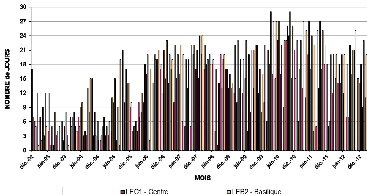
Fig. 13 : NO 2 – Valeurs Semi horaires > 850 µg/m 3 . Nombre de dépassements par mois et nombre de jours par mois avec dépassements (décembre 2002 – mars 2013)
