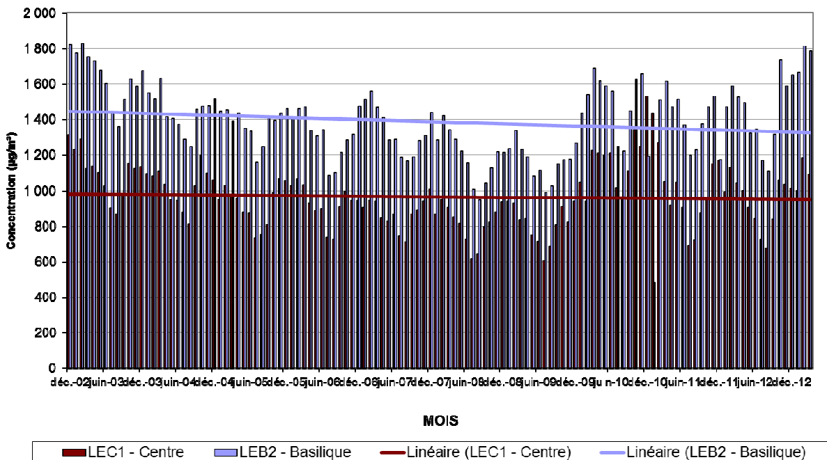
Fig. 9 : NO 2 et NO – Évolution des concentrations moyennes mensuelles dans les deux postes de mesure du tunnel Léopold II. Période – « Décembre 2002 – Mars 2013 »
