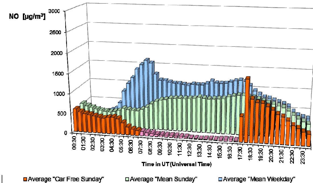
Fig. 29.b : NO dans le tunnel Léopold II, direction Centre – Profil journalier sur les onze dimanches sans voiture et sur tous les dimanches et jours ouvrables des périodes 'mai – septembre 2002-2012'.
