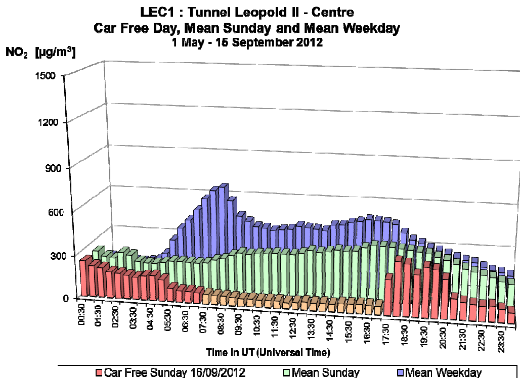
Fig. 27.a : NO 2 dans le tunnel Léopold II, direction Centre – Profil journalier du dimanche sans voiture 16-09-2012, d'un dimanche moyen et d'un jour ouvrable moyen de la période 'mai – septembre 2012'.
