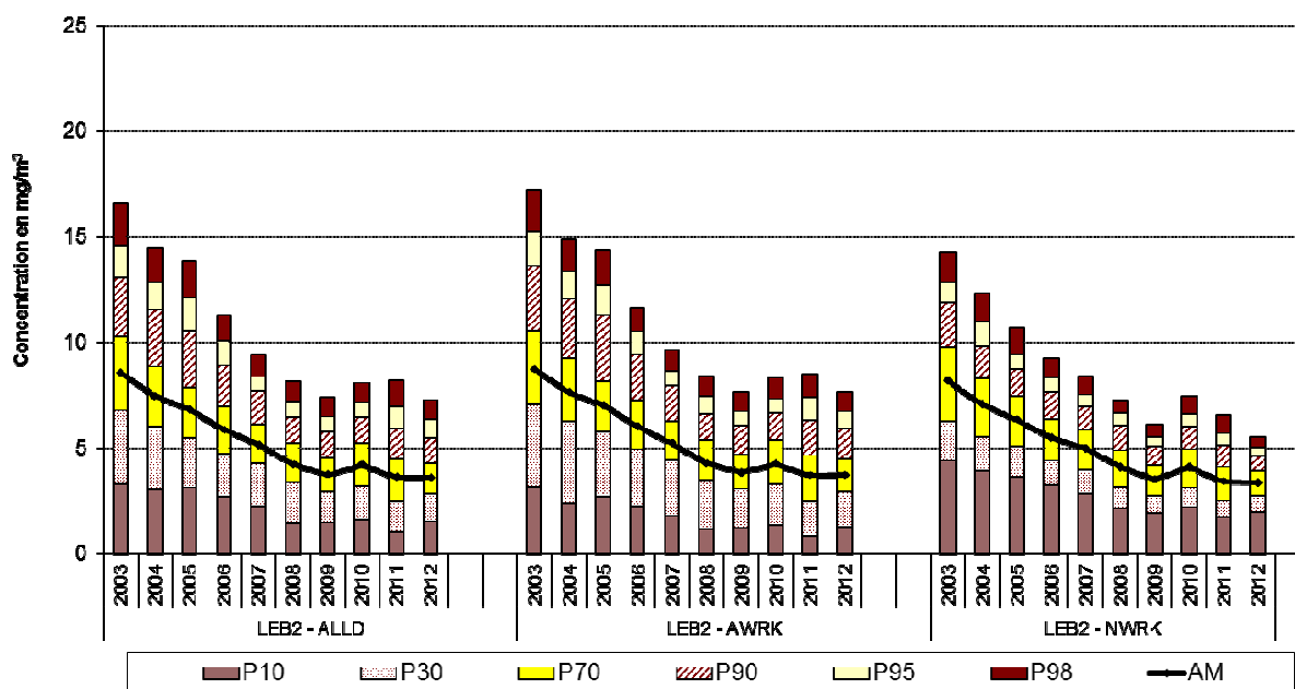
Fig. 6 : CO - Distribution de Fréquences Cumulées des Valeurs Horaires dans les deux postes de mesure du tunnel Léopold II. Sélection tous les jours , les jours ouvrables et non ouvrables . Périodes annuelles de 2003 à 2012
