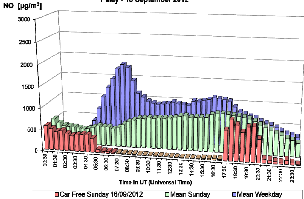
Fig. 29.a : NO dans le tunnel Léopold II, direction Centre – Profil journalier du dimanche sans voiture 16-09-2012, d'un dimanche moyen et d'un jour ouvrable moyen de la période 'mai – septembre 2012'.
