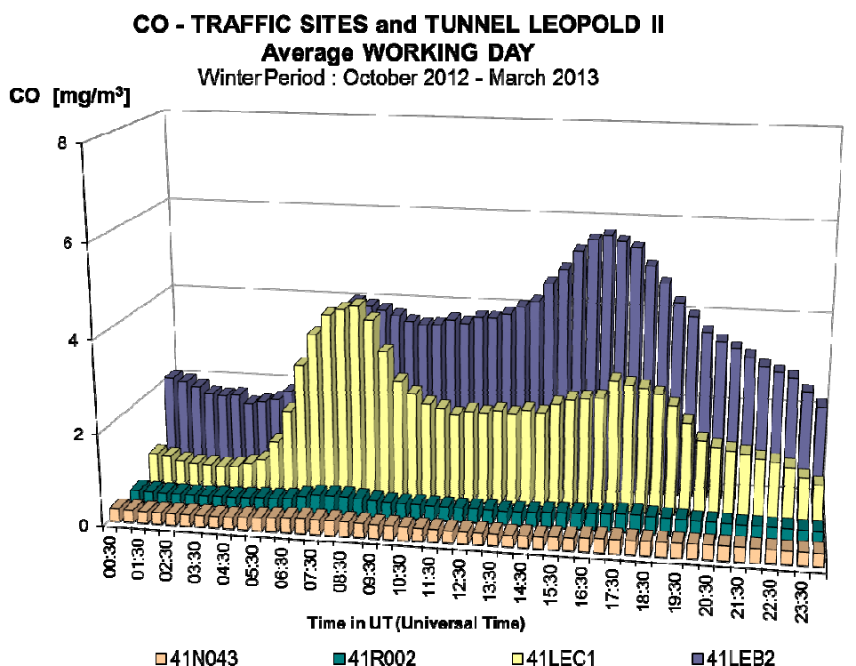
Fig. 33 : CO - Évolution journalière moyenne d'un jour ouvrable moyen ( hiver 2012-2013 ) Postes de mesure trafic à l'air ambiant – Avant Port (N043) et Av. de la Couronne (R002) Postes de mesure du Tunnel Léopold II – LEC1 (Centre) et LEB2 (Basilique)
