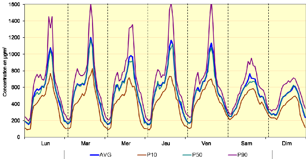
Fig. 22 : Poste de Mesure 41LEB2 (basilique) – Évolution hebdomadaire moyenne pour le NO 2 Période hivernale 2012 - 2013 et période estivale 2012
