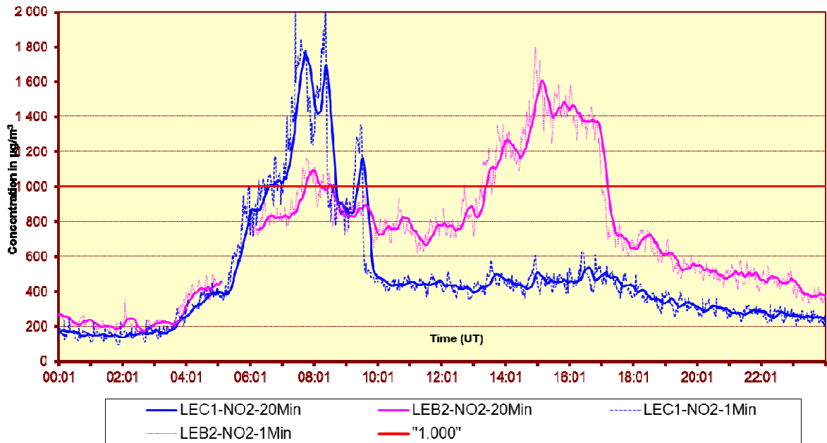
Fig. 4: NO 2 – évolution des valeurs minutes et de la moyenne glissante sur 20 minutes dans les deux postes de mesure du tunnel Léopold II Vendredi 14 septembre 2012 et vendredi 19 octobre 2012
