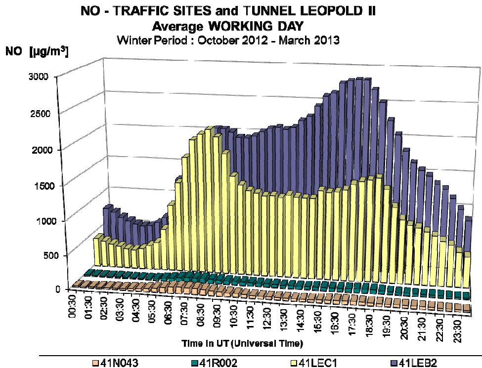
Fig. 34 : NO 2 et NO - Évolution journalière moyenne d'un jour ouvrable moyen ( hiver 2012-2013 ) Postes de mesure trafic à l'air ambiant – Avant Port (N043) et Av. de la Couronne (R002) Postes de mesure du Tunnel Léopold II – LEC1 (Centre) et LEB2 (Basilique)
