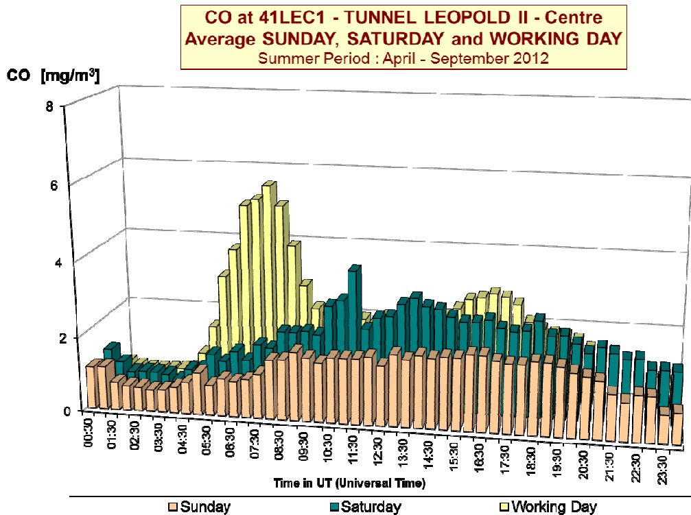
Fig. 19 : CO – évolution journalière moyenne au poste de mesure 41LEC1 (centre) Comparaison entre un dimanche, un samedi et un jour ouvrable moyen Période hivernale 2012-2013 et période estivale 2012
