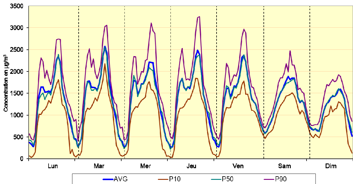
Fig. 26 : Poste de Mesure 41LEB2 (basilique) – Évolution hebdomadaire moyenne pour le NO Période hivernale 2012 - 2013 et période estivale 2012
