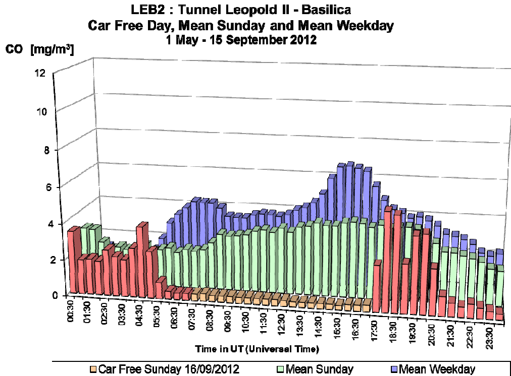
Fig. 32.a : CO in de Leopold II tunnel, richting Basiliek – Dagprofiel autoluwe zondag 16-09-2012, gemiddelde zondag en een gemiddelde werkdag in de periode ‘mei – september 2012’
