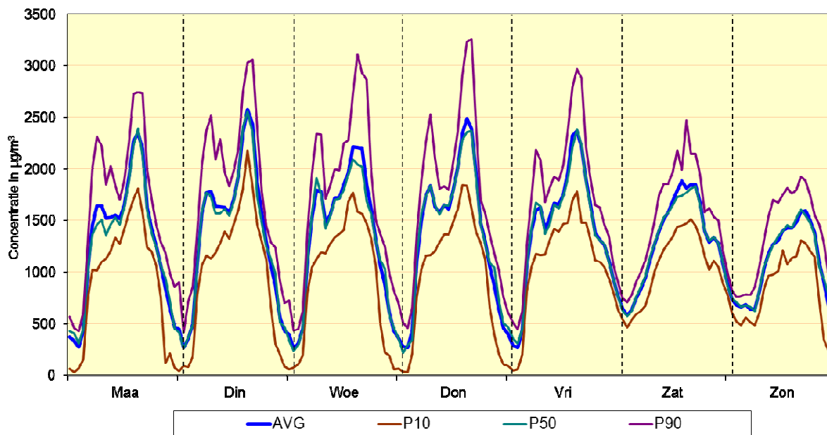
Fig. 26 : Meetpost 41LEB2 (basiliek) - Gemiddeld weekverloop voor NO Vergelijking winterperiode 2012 - 2013 en zomerperiode 2012
