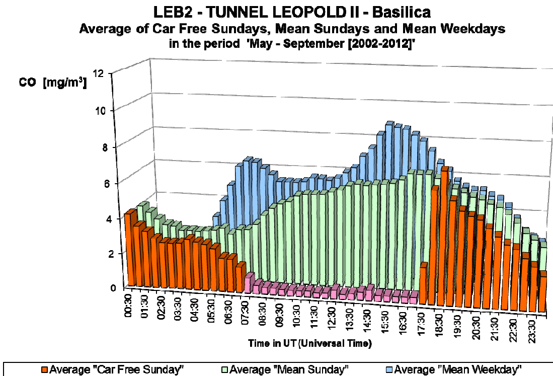
Fig. 32.b : CO in de Leopold II tunnel, richting Basiliek – Gemiddelde Dagprofiel van de elf autoluwe zondagen en van alle zondagen en werkdagen in de periodes ‘mei – september 2002-2012’
