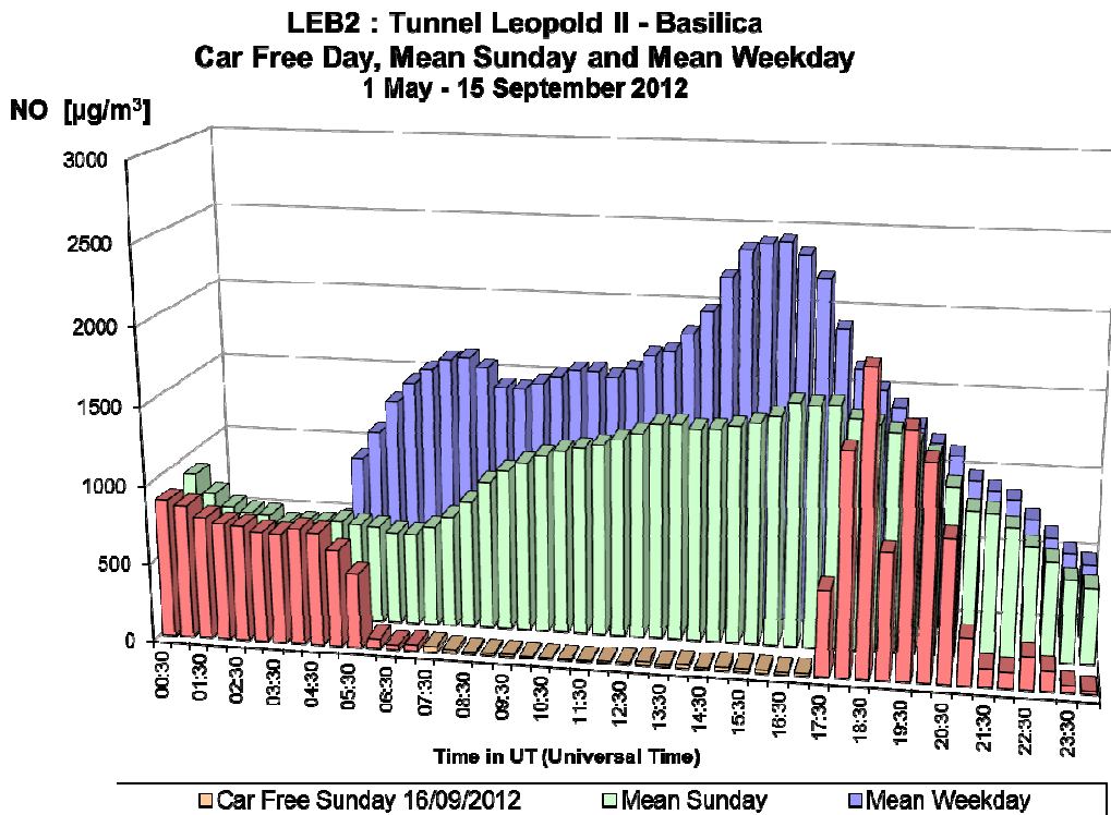
Fig. 30.a : NO in de Leopold II tunnel, richting Basiliek – Dagprofiel autoluwe zondag 16-09-2012, gemiddelde zondag en een gemiddelde werkdag in de periode ‘mei – september 2012’
