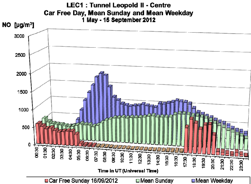
Fig. 29.a : NO in de Leopold II tunnel, richting Centrum – Dagprofiel autoluwe zondag 16-09-2012, gemiddelde zondag en gemiddelde werkdag in de periode ‘mei – september 2012’
