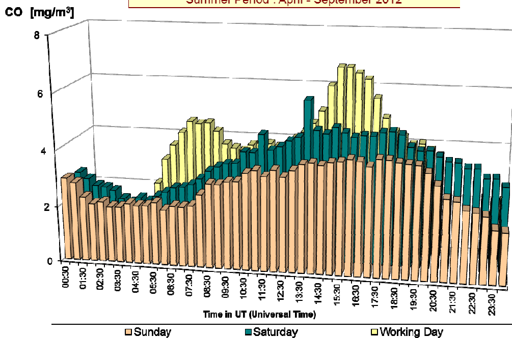
Fig. 20 : CO-dagverloop in de meetpost 41LEB2 (richting basiliek) Vergelijking voor een gemiddelde zondag, zaterdag en werkdag Winterperiode 2012-2013 en zomerperiode 2012
