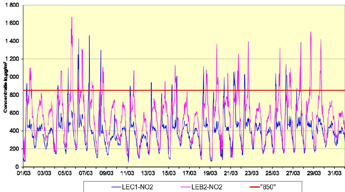
Fig. 1: NO 2 - Evolutie van de uurwaarden en de halfuurswaarden tijdens de maand maart 2013 Meetplaats 41LEC1, richting Centrum - Meetplaats 41LEB2, richting Basiliek
