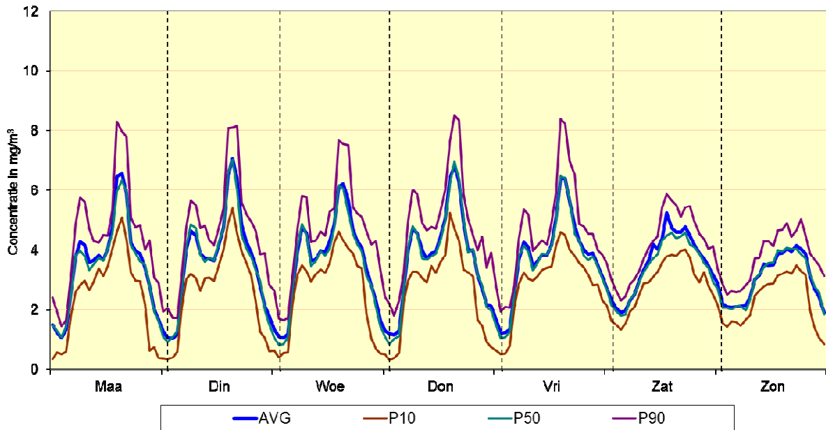
Fig. 24 : Meetpost 41LEB2 (basiliek) - Gemiddeld weekverloop voor CO Vergelijking winterperiode 2012 - 2013 en zomerperiode 2012
