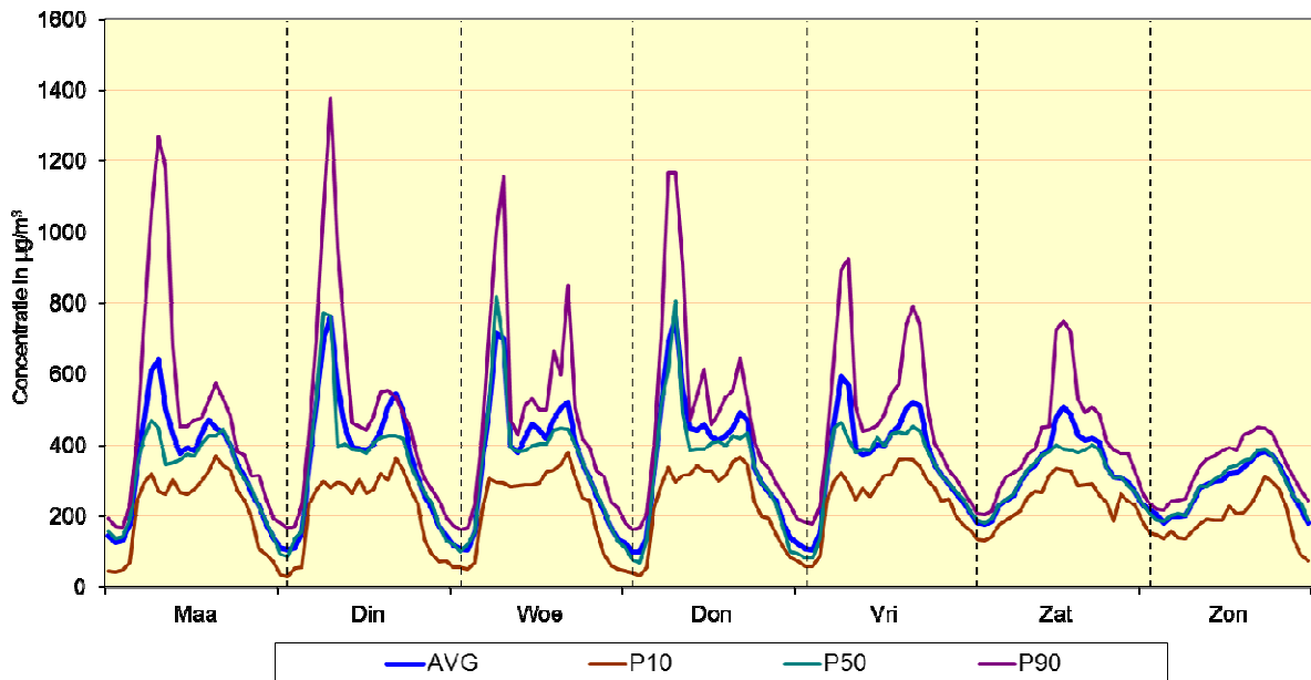
Fig. 21 : Meetpost 41LEC1 (centrum) - Gemiddeld weekverloop voor NO 2 Vergelijking winterperiode 2012 - 2013 en zomerperiode 2012
