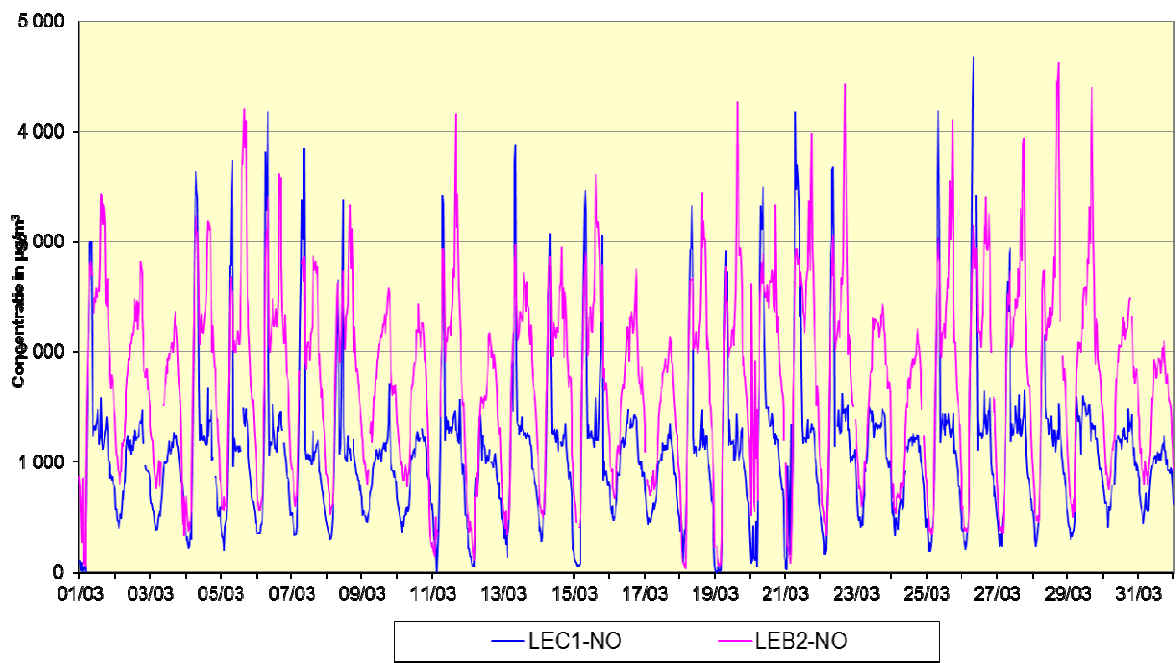
Fig. 2: NO - Evolutie van de uurwaarden en de halfuurswaarden tijdens de maand maart 2013 Meetplaats 41LEC1, richting Centrum - Meetplaats 41LEB2, richting Basiliek
