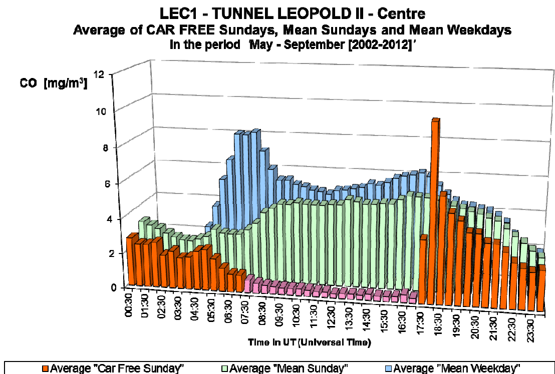
Fig. 31.b : CO in de Leopold II tunnel, richting Centrum – Gemiddelde Dagprofiel van de elf autoluwe zondagen en van alle zondagen en werkdagen in de periodes ‘mei – september 2002-2012’
