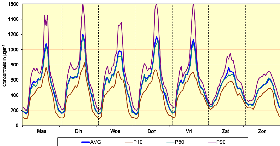
Fig. 22 : Meetpost 41LEB2 (basiliek) - Gemiddeld weekverloop voor NO 2 Vergelijking winterperiode 2012 - 2013 en zomerperiode 2012
