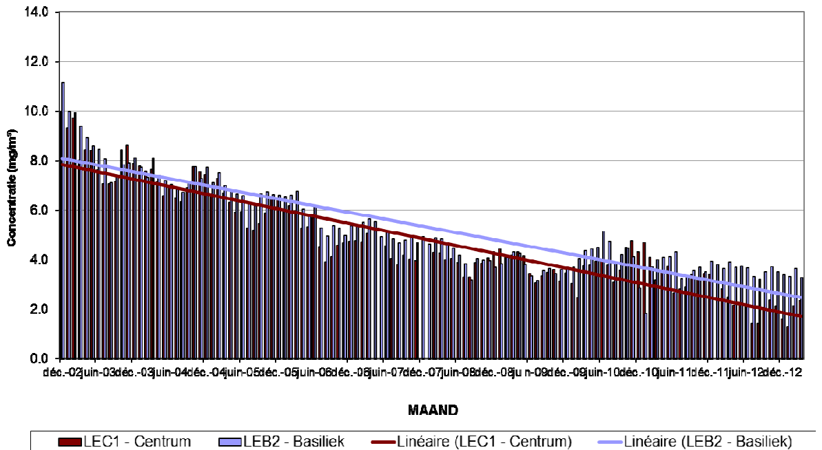
Fig. 10 : NO x en CO - Evolutie maandgemiddelde concentratie in beide meetposten van de Leopold II tunnel. Periode "December 2002 – Maart 2013"
