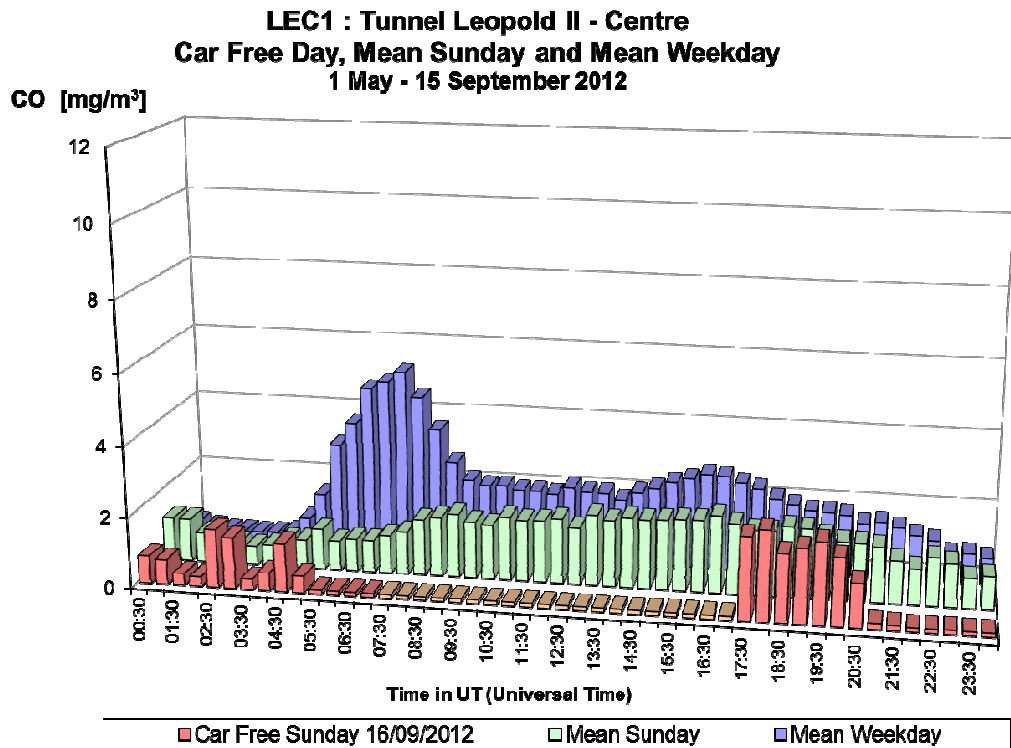
Fig. 31.a : CO in de Leopold II tunnel, richting Centrum – Dagprofiel autoluwe zondag 16-09-2012, gemiddelde zondag en gemiddelde werkdag in de periode ‘mei – september 2012’
