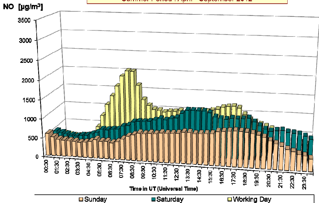
Fig. 17 : NO-dagverloop in de meetpost 41LEC1 (richting centrum) Vergelijking voor een gemiddelde zondag, zaterdag en werkdag Winterperiode 2012-2013 en zomerperiode 2012
