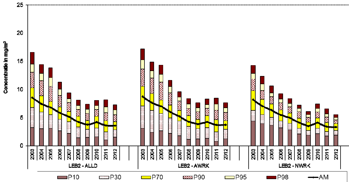
Fig. 6 : CO - Cumulatieve Frequentieverdeling Jurwaarden in beide meetposten van de Leopold II tunnel. Selectie alle dagen , alle werkdagen en alle niet-werkdagen Jaarperiodes 2003 t/m 2012
