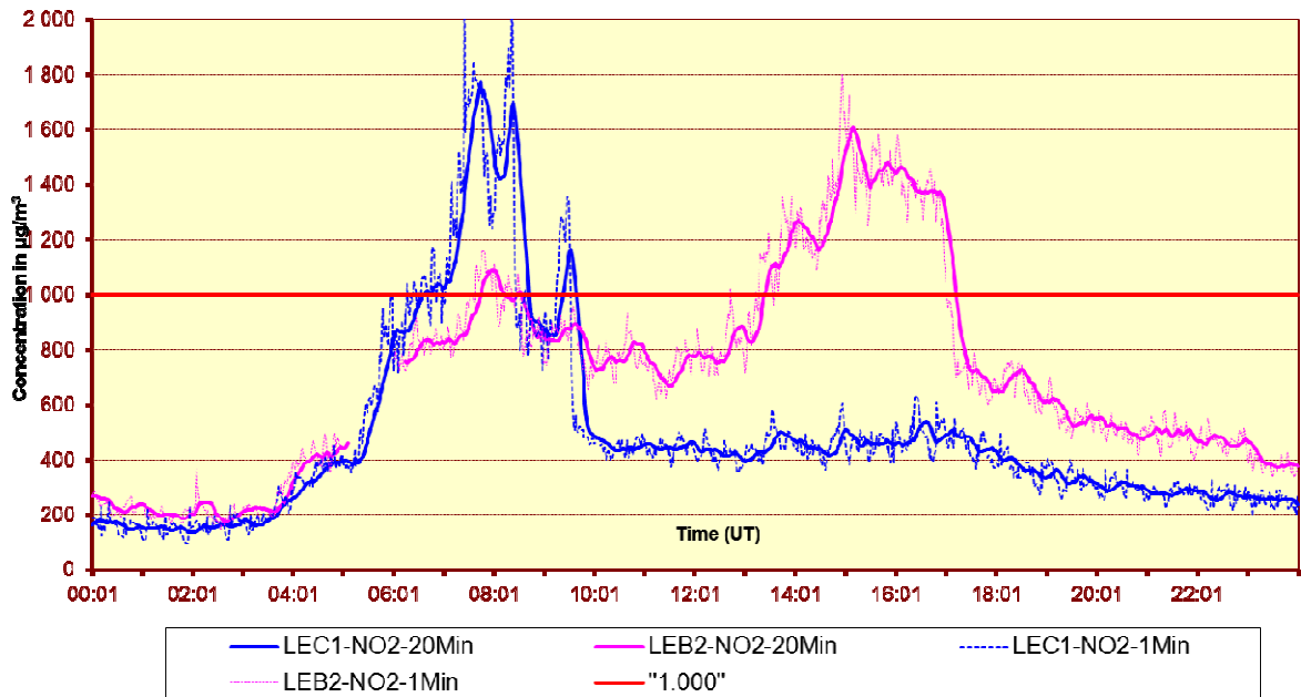
Fig. 4: NO 2 - evolutie minuutwaarden en voortschrijdend 20-minuutsgemiddelde in beide meetposten van de Leopold II tunnel Vrijdag 14 september 2012 en vrijdag 19 oktober 2012
