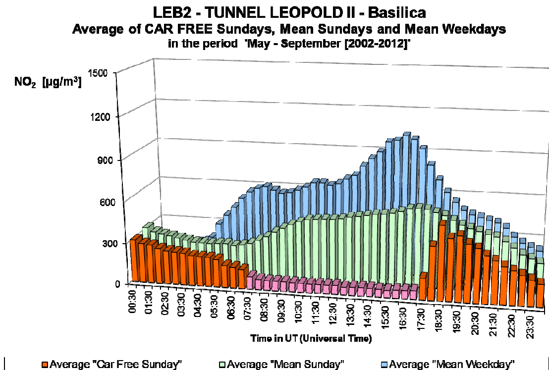
Fig. 28.b : NO 2 in de Leopold II tunnel, richting Basiliek – Gemiddelde Dagprofiel van de elf autoluwe zondagen en van alle zondagen en werkdagen in de periodes ‘mei – september 2002-2012’
