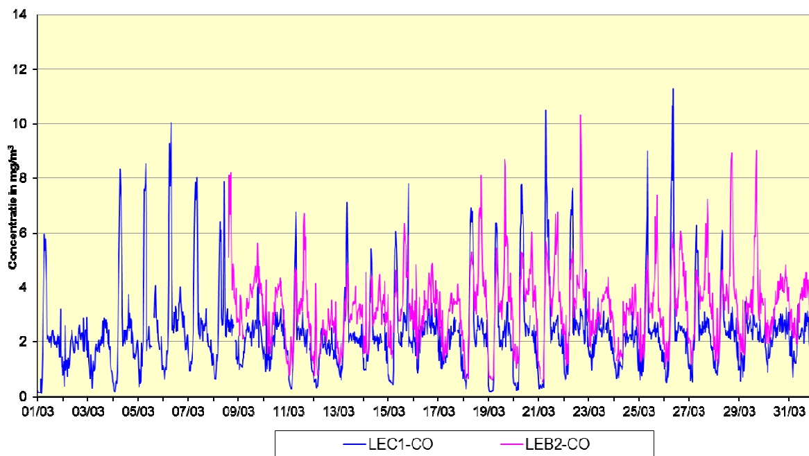
Fig. 3: CO - Evolutie van de uurwaarden en de halfuurswaarden tijdens de maand maart 2013 Meetplaats 41LEC1, richting Centrum - Meetplaats 41LEB2, richting Basiliek
