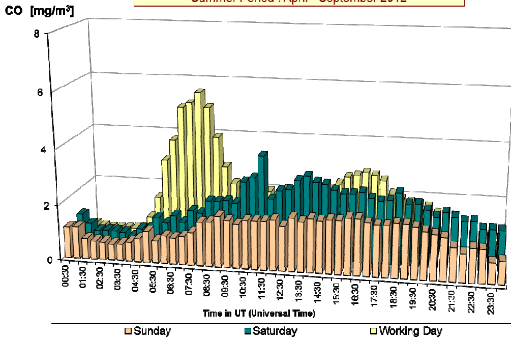
Fig. 19 : CO-dagverloop in de meetpost 41LEC1 (richting centrum) Vergelijking voor een gemiddelde zondag, zaterdag en werkdag Winterperiode 2012-2013 en zomerperiode 2012
