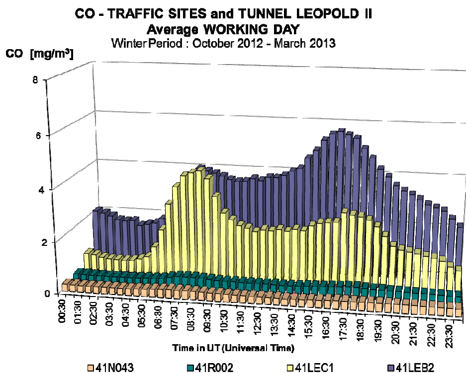
Fig. 33 : CO-dagverloop voor een gemiddelde werkdag tijdens de winter 2012-2013 Meetposten verkeer in de omgevingslucht – Voorhaven (N043) en Kroonlaan (R002) Meetposten in de tunnel Leopold II – LEC1 (centrum) en LEC2 (basiliek)
