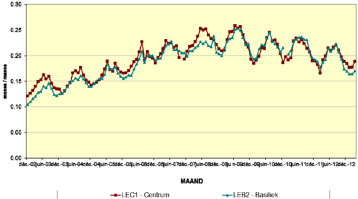
Fig. 11 : Evolutive van de verhouding NO 2 /NO x in beide meetposten van de Leopold II tunnel. Periode "December 2002 – Maart 2013"
