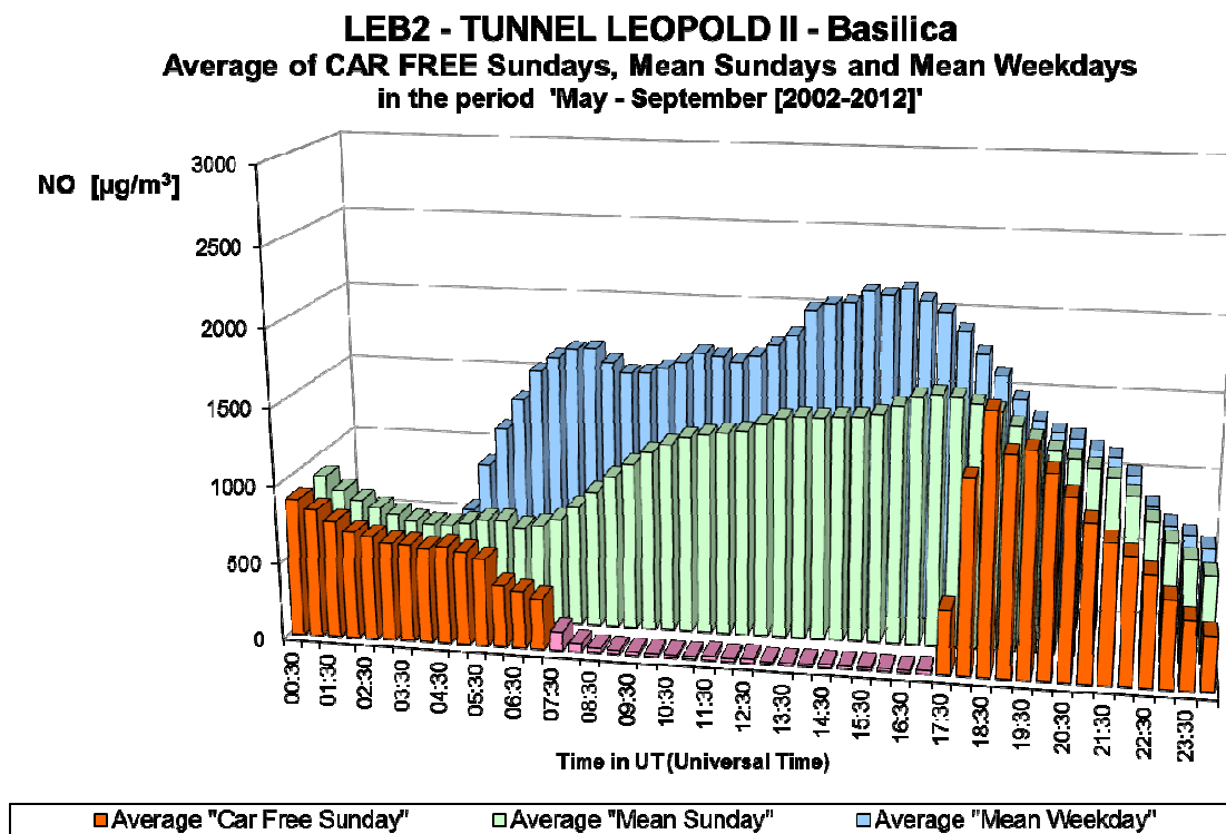
Fig. 30.b : NO in de Leopold II tunnel, richting Basiliek – Gemiddelde Dagprofiel van de elf autoluwe zondagen en van alle zondagen en werkdagen in de periodes ‘mei – september 2002-2012’
