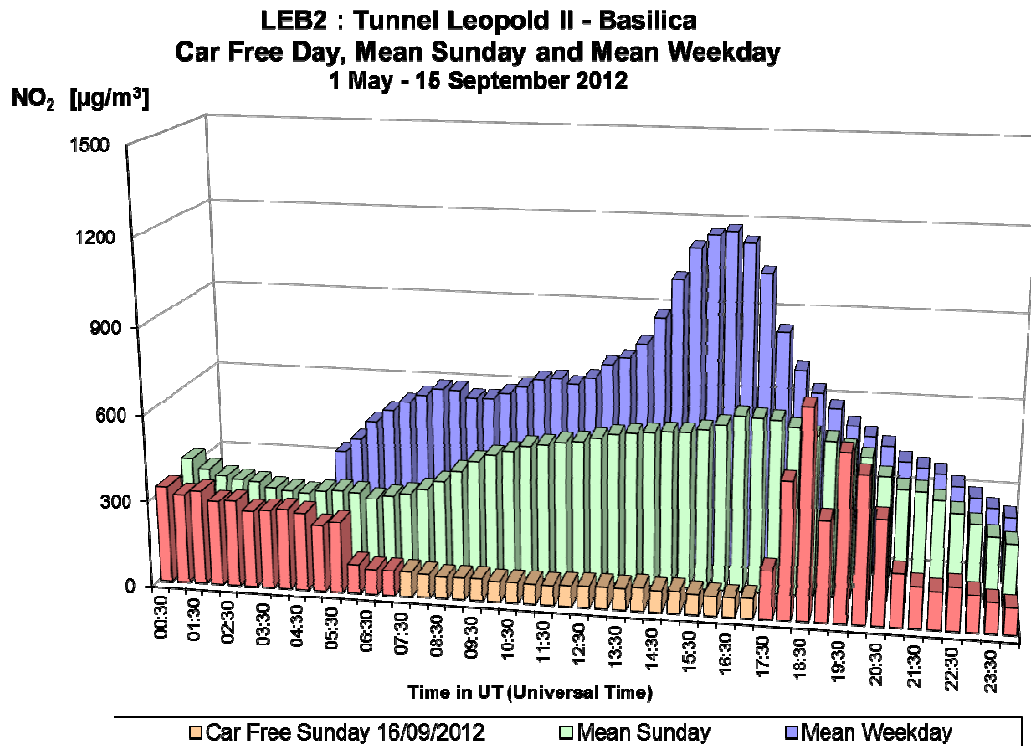
Fig. 28.a : NO 2 in de Leopold II tunnel, richting Basiliek – Dagprofiel autoluwe zondag 16-09-2012, gemiddelde zondag en een gemiddelde werkdag in de periode ‘mei – september 2012’
