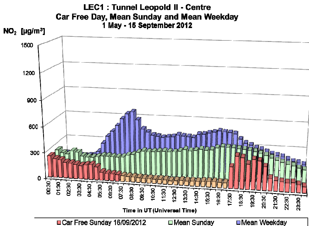
Fig. 27.a : NO 2 in de Leopold II tunnel, richting Centrum – Dagprofiel autoluwe zondag 16-09-2012, gemiddelde zondag en gemiddelde werkdag in de periode ‘mei – september 2012’
