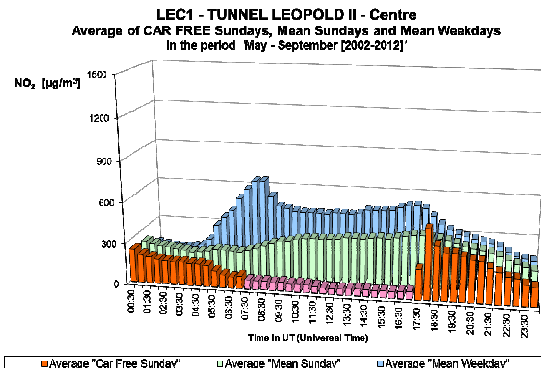
Fig. 27.b : NO 2 in de Leopold II tunnel, richting Centrum – Gemiddelde Dagprofiel van de elf autoluwe zondagen en van alle zondagen en werkdagen in de periodes ‘mei – september 2002-2012’
