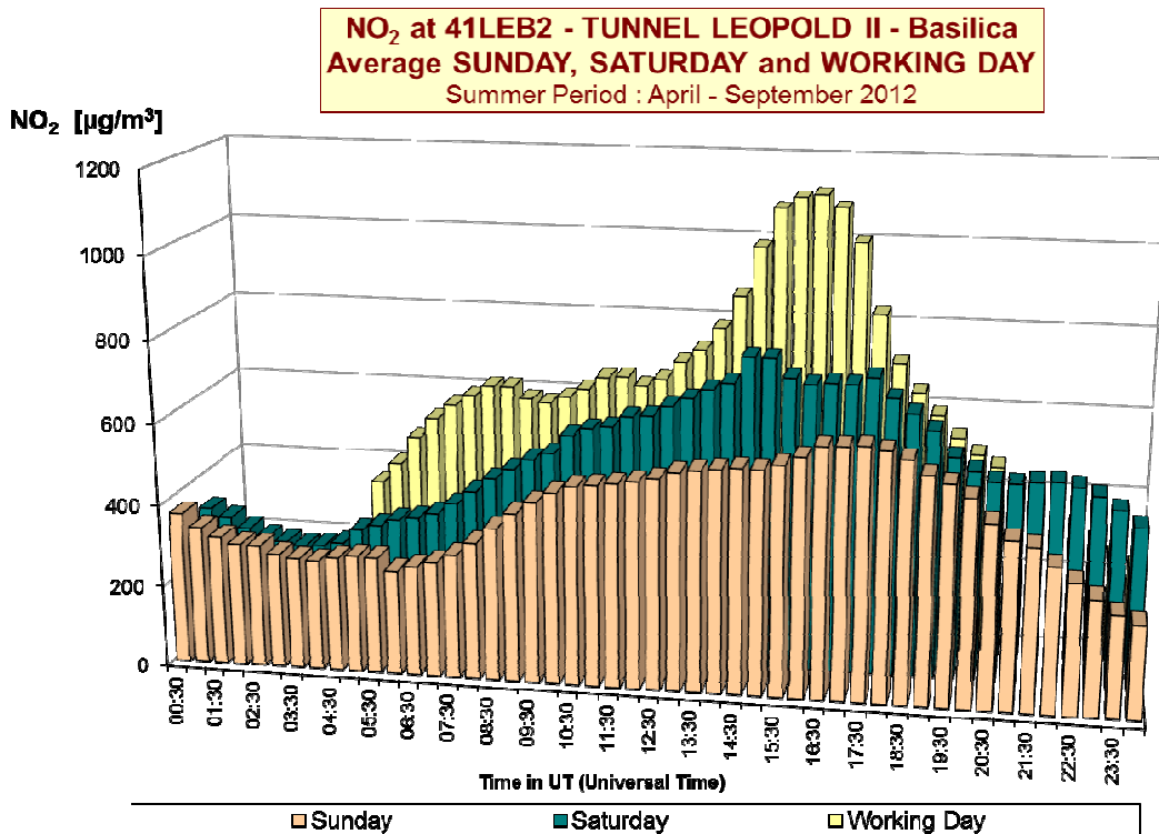
Fig. 16 : NO 2 -dagverloop in de meetpost 41LEB2 (richting basiliek) Vergelijking voor een gemiddelde zondag, zaterdag en werkdag Winterperiode 2012-2013 en zomerperiode 2012
