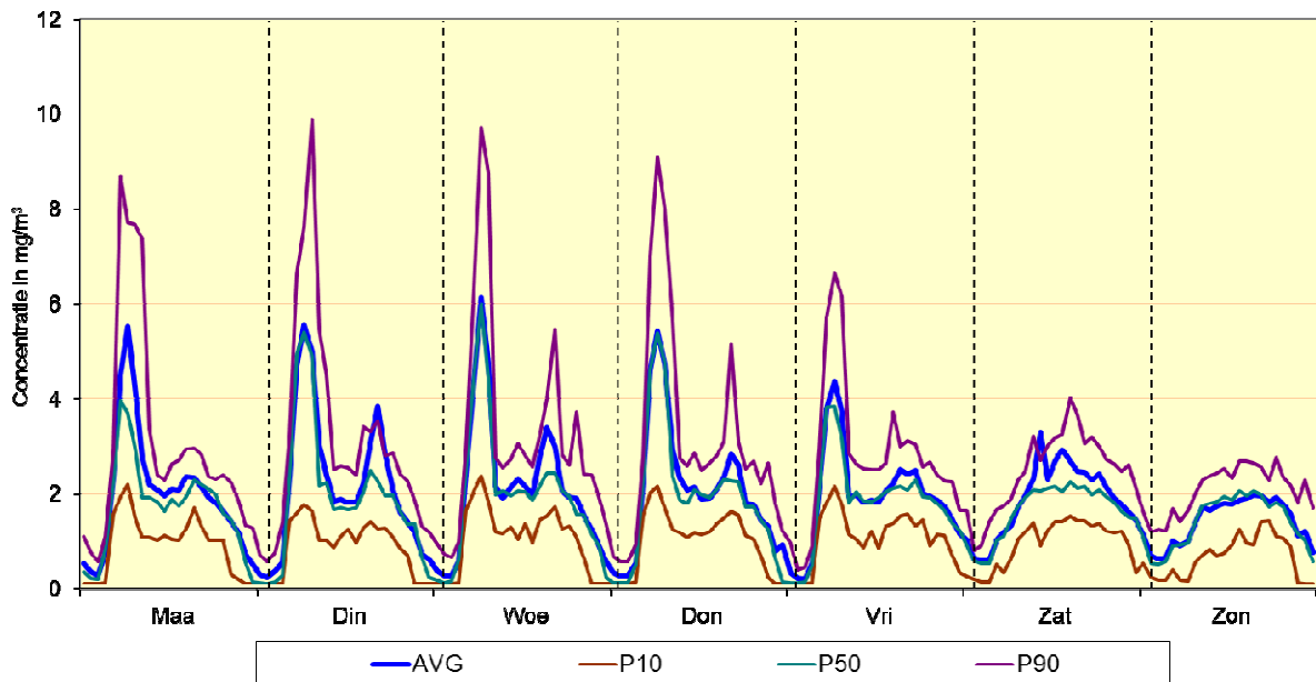
Fig. 23 : Meetpost 41LEC1 (centrum) - Gemiddeld weekverloop voor CO Vergelijking winterperiode 2012 - 2013 en zomerperiode 2012
