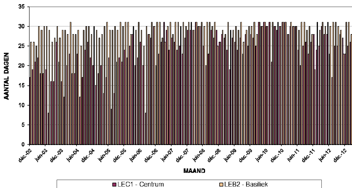
Fig. 14 : NO 2 -Uurwaarden > 400 µg/m 3 . Totaal aantal overschrijdingen per maand en aantal dagen per maand met overschrijding (december 2002 – maart 2013)
