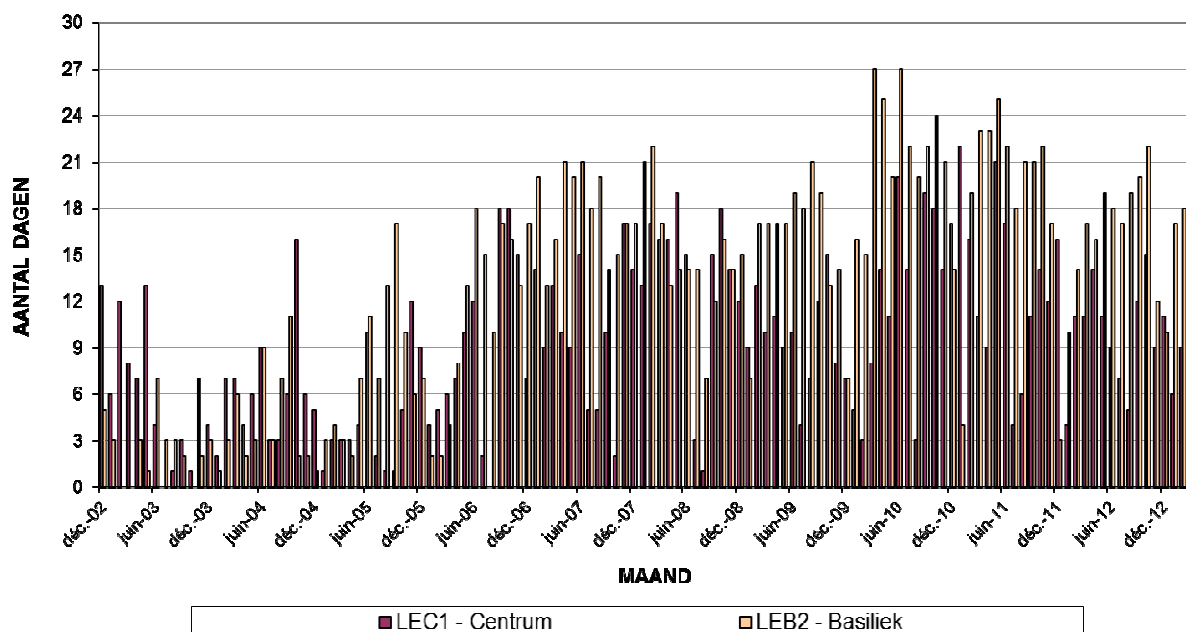
Fig. 12 : NO 2 – 20-Minutsgemiddelden > 1.000 µg/m 3 . Totaal aantal overschrijdingen per maand en aantal dagen per maand met overschrijding (december 2002 – maart 2013)
