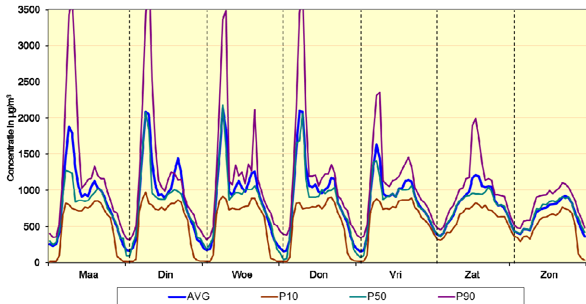
Fig. 25 : Meetpost 41LEC1 (centrum) - Gemiddeld weekverloop voor NO Vergelijking winterperiode 2012 - 2013 en zomerperiode 2012
