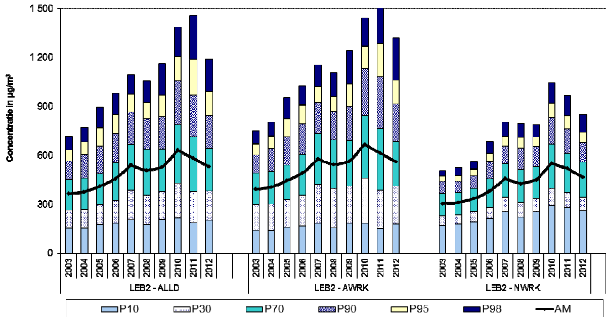
Fig. 5 : NO 2 - Cumulatieve Frequentieverdeling Jurwaarden in beide meetposten van de Leopold II tunnel. Selectie alle dagen , alle werkdagen en alle niet-werkdagen Jaarperiodes 2003 t/m 2012
