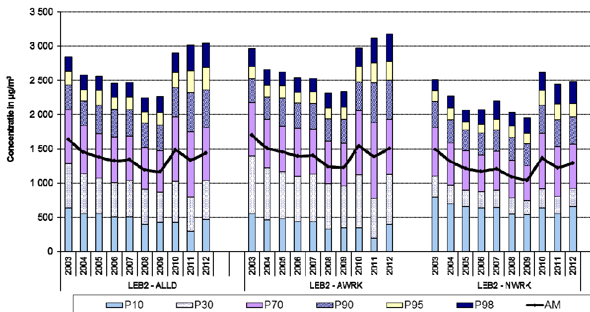
Fig. 7 : NO - Cumulatieve Frequentieverdeling Jurwaarden in beide meetposten van de Leopold II tunnel. Selectie alle dagen , alle werkdagen en alle niet-werkdagen Jaarperiodes 2003 t/m 2012
