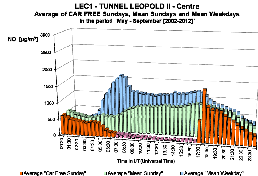
Fig. 29.b : NO in de Leopold II tunnel, richting Centrum – Gemiddelde Dagprofiel van de elf autoluwe zondagen en van alle zondagen en werkdagen in de periodes ‘mei – september 2002-2012’
