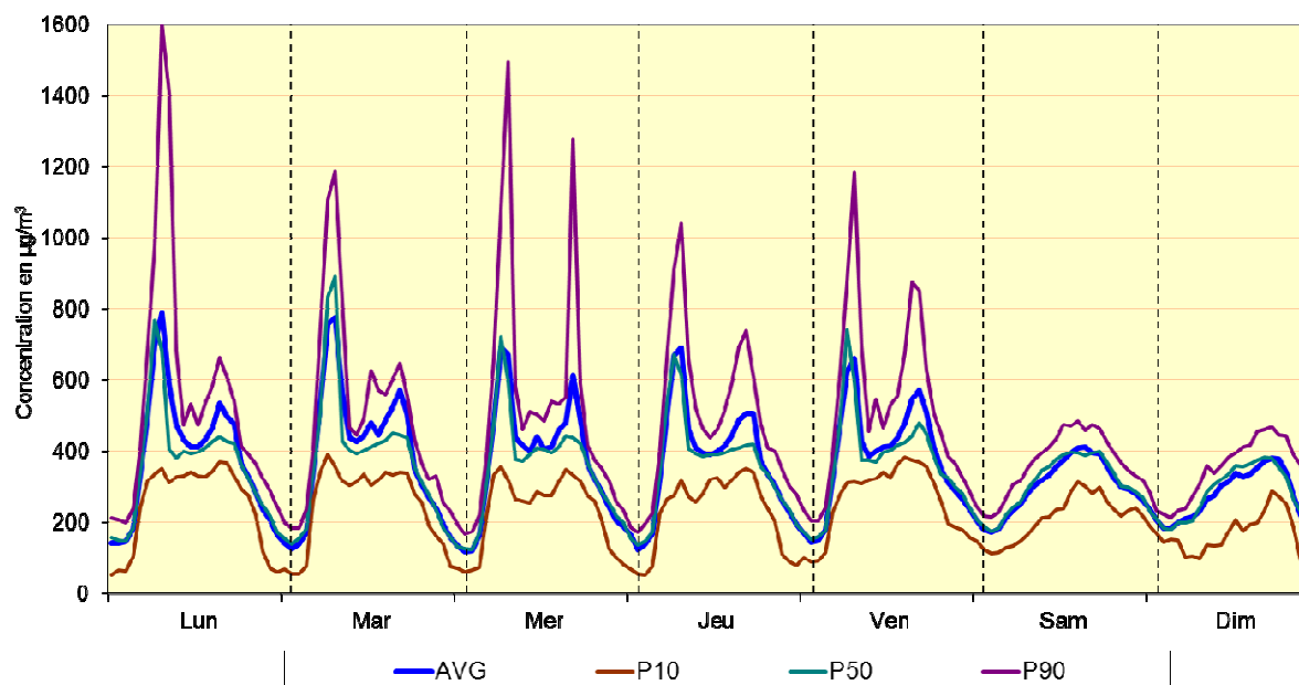
Fig. 21 : Poste de Mesure 41LEC1 (centre) – Évolution hebdomadaire moyenne pour le NO 2 Période hivernale 2012 - 2013 et période estivale 2013
