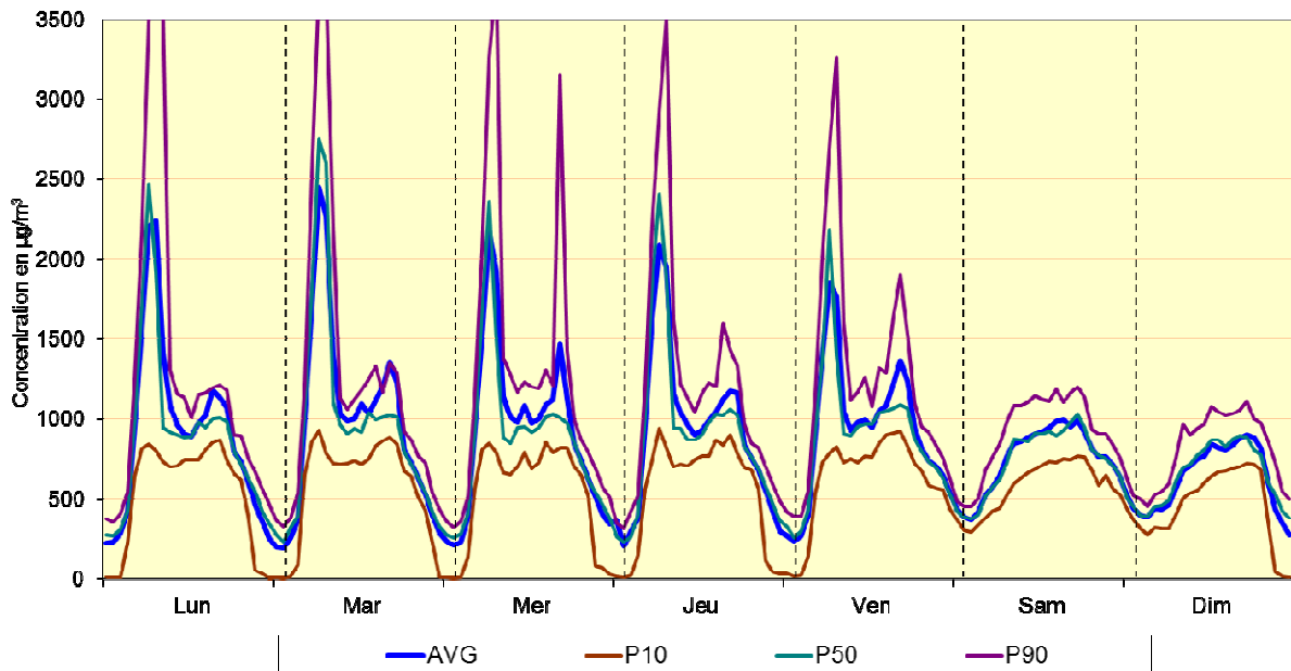
Fig. 25 : Poste de Mesure 41LEC1 (centre) – Évolution hebdomadaire moyenne pour le NO Période hivernale 2012 - 2013 et période estivale 2013
