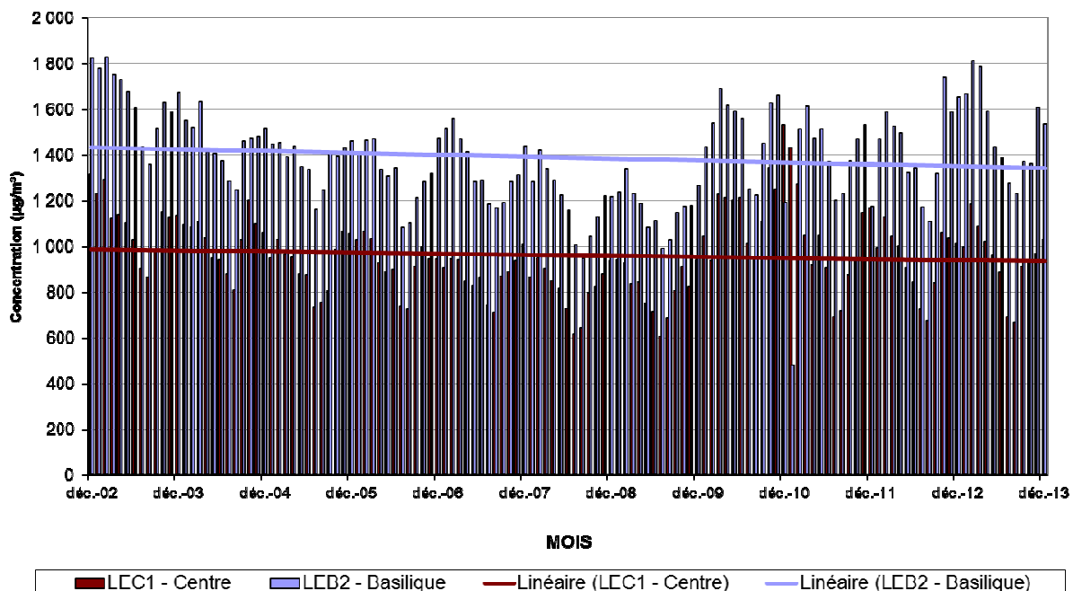
Fig. 9 : NO 2 et NO – Évolution des concentrations moyennes mensuelles dans les deux postes de mesure du tunnel Léopold II. Période – « Décembre 2002 – Décembre 2013 »
