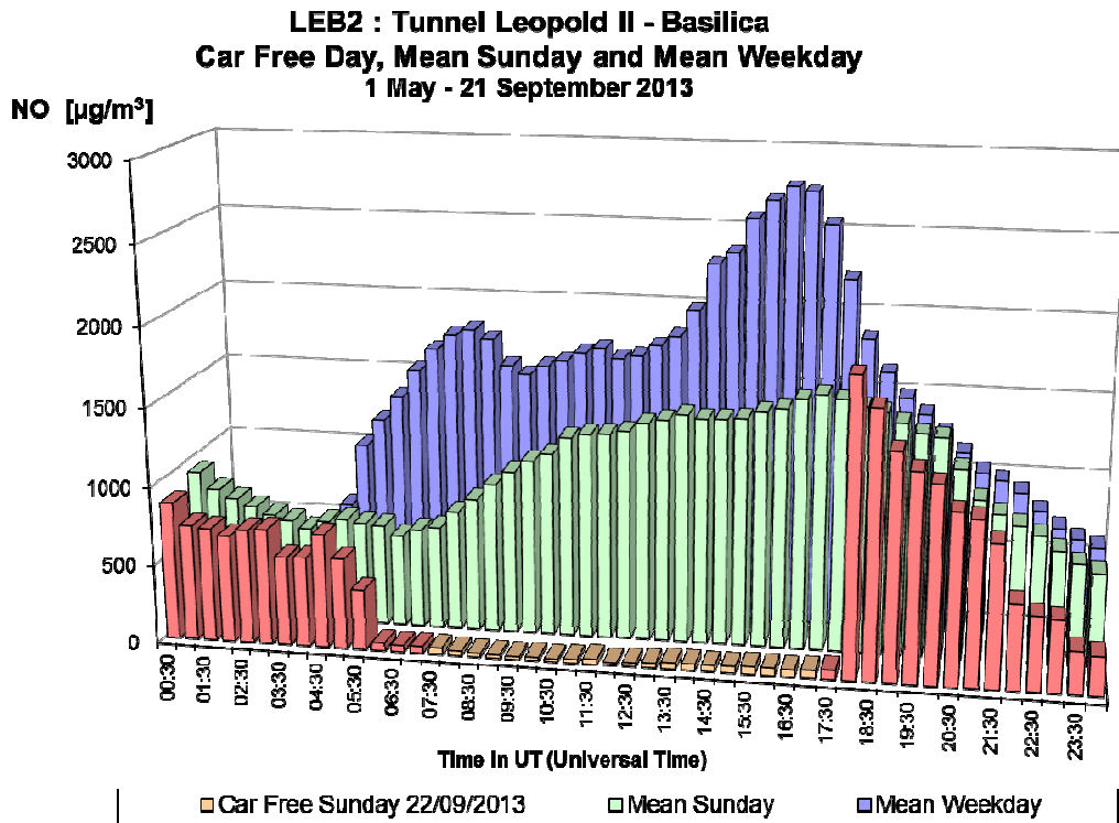
Fig. 30.a : NO dans le tunnel Léopold II, direction Basilique – Profil journalier du dimanche sans voiture, d'un dimanche moyen et d'un jour ouvrable moyen de la période 'mai – septembre 2013'.
