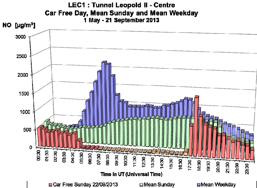
Fig. 29.a : NO dans le tunnel Léopold II, direction Centre – Profil journalier du dimanche sans voiture 22-09-2013, d'un dimanche moyen et d'un jour ouvrable moyen de la période 'mai – septembre 2013'.
