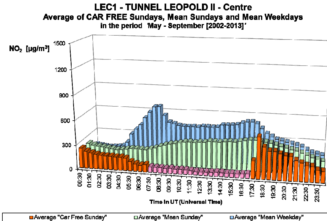
Fig. 27.b : NO 2 dans le tunnel Léopold II, direction Centre – Profil journalier sur les douze dimanches sans voiture et sur tous les dimanches et jours ouvrables des périodes 'mai – septembre 2002-2013'.
