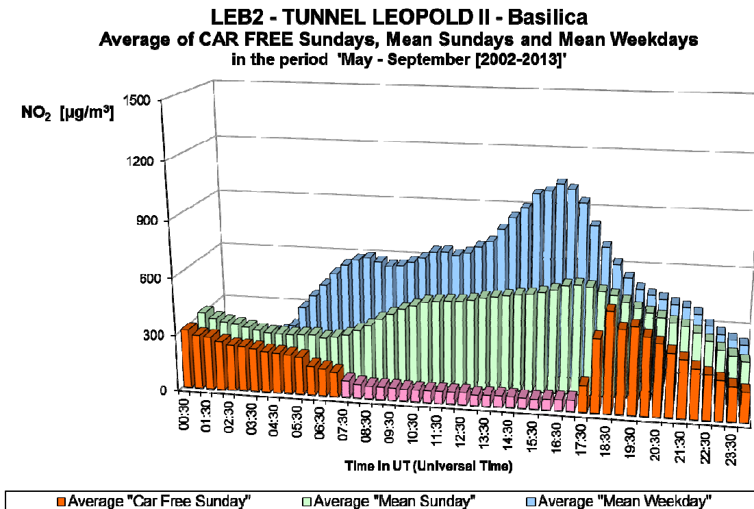
Fig. 28.b : NO 2 dans le tunnel Léopold II, direction Basilique – Profil journalier sur les douze dimanches sans voiture et sur tous les dimanches et jours ouvrables des périodes 'mai – septembre 2002-2013'.
