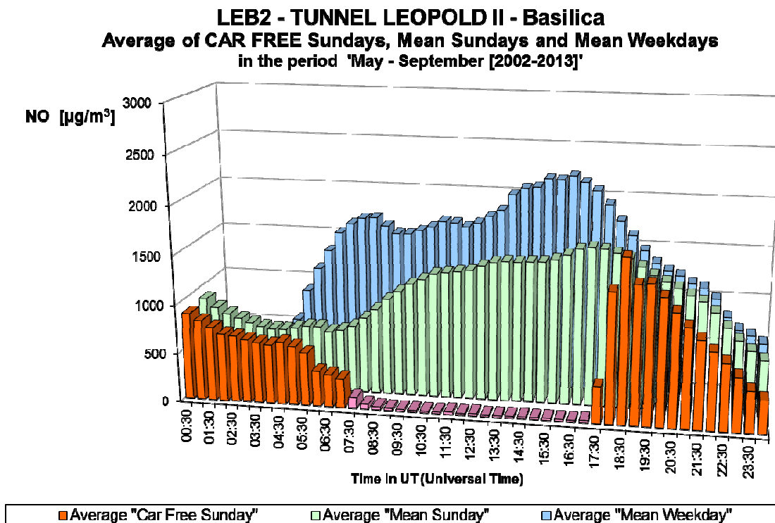
Fig. 30.b : NO dans le tunnel Léopold II, direction Basilique – Profil journalier sur les douze dimanches sans voiture et sur tous les dimanches et jours ouvrables des périodes 'mai – septembre 2002-2013'.
