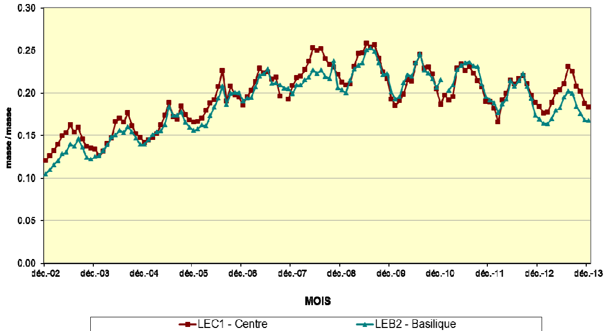
Fig. 11 : Évolution du rapport NO 2 /NO x dans les deux postes de mesure du tunnel Léopold II. Période – « Décembre 2002 – Décembre 2013 »
