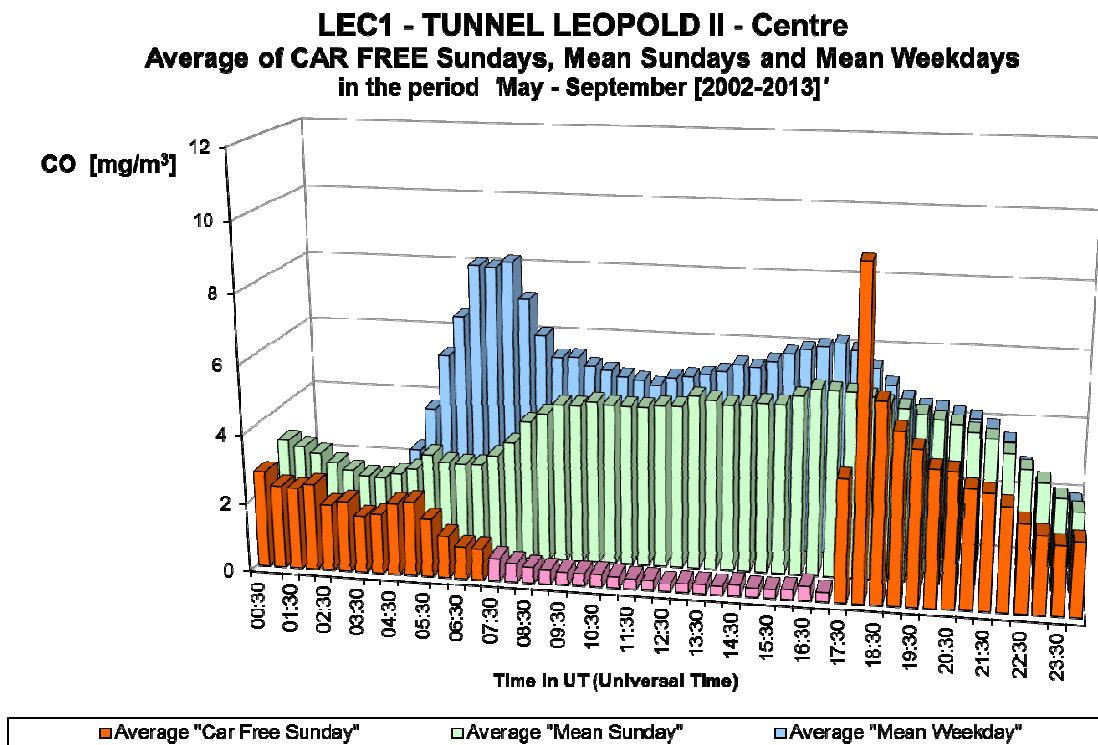
Fig. 31.b : CO dans le tunnel Léopold II, direction Centre – Profil journalier sur les douze dimanches sans voiture et sur tous les dimanches et jours ouvrables des périodes 'mai – septembre 2002-2013'.
