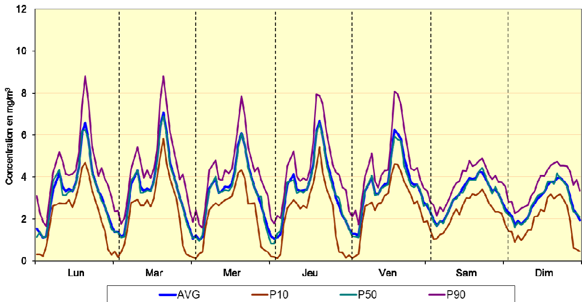
Fig. 24 : Poste de Mesure 41LEB2 (basilique) – Évolution hebdomadaire moyenne pour le CO Période hivernale 2012 - 2013 et période estivale 2013
