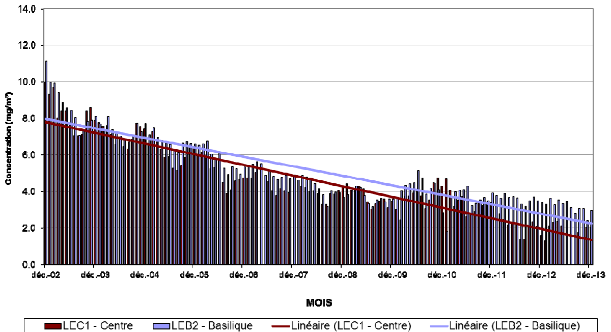
Fig. 10 : NO x et CO – Évolution des concentrations moyennes mensuelles dans les deux postes de mesure du tunnel Léopold II. Période – « Décembre 2002 – Décembre 2013 »
