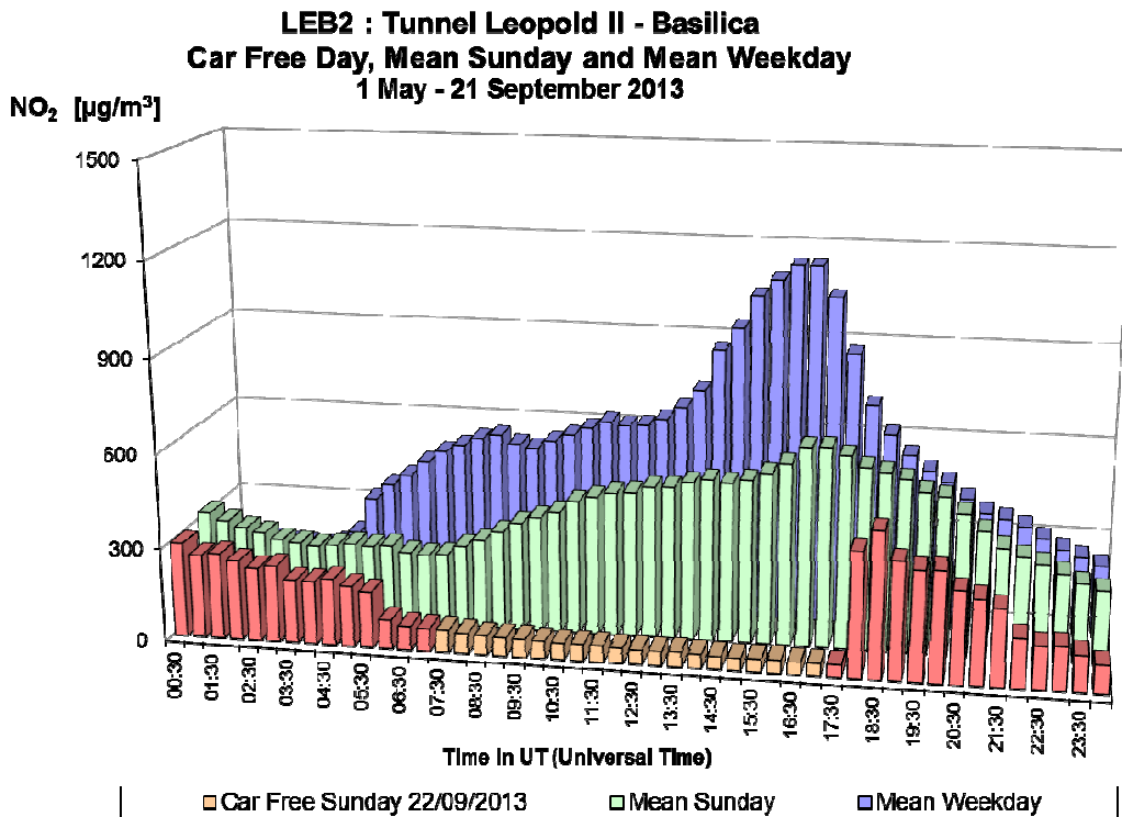
Fig. 28.a : NO 2 dans le tunnel Léopold II, direction Basilique – Profil journalier du dimanche sans voiture, d'un dimanche moyen et d'un jour ouvrable moyen de la période 'mai – septembre 2013'.
