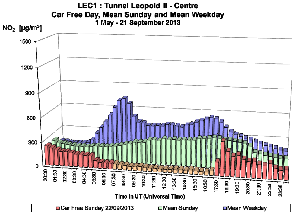
Fig. 27.a : NO 2 dans le tunnel Léopold II, direction Centre – Profil journalier du dimanche sans voiture 22-09-2013, d'un dimanche moyen et d'un jour ouvrable moyen de la période 'mai – septembre 2013'.
