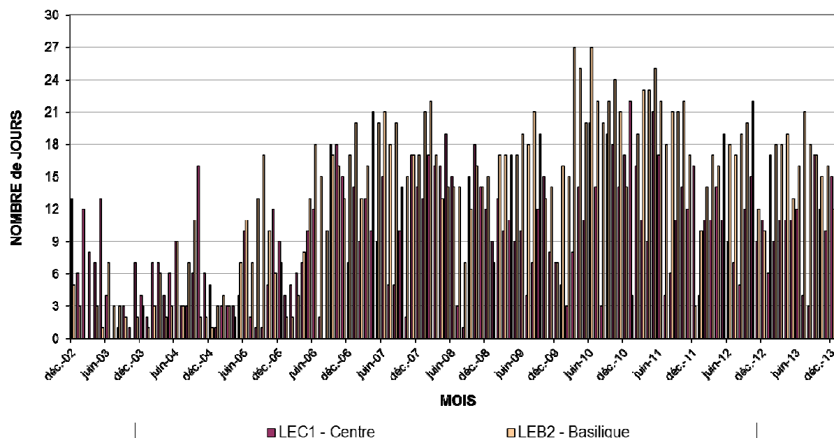
Fig. 12 : NO 2 –Moyennes glissantes sur 20 minutes > 1.000 µg/m 3 . Nombre de dépassements par mois et nombre de jours par mois avec dépassements (décembre 2002 – décembre 2013)
