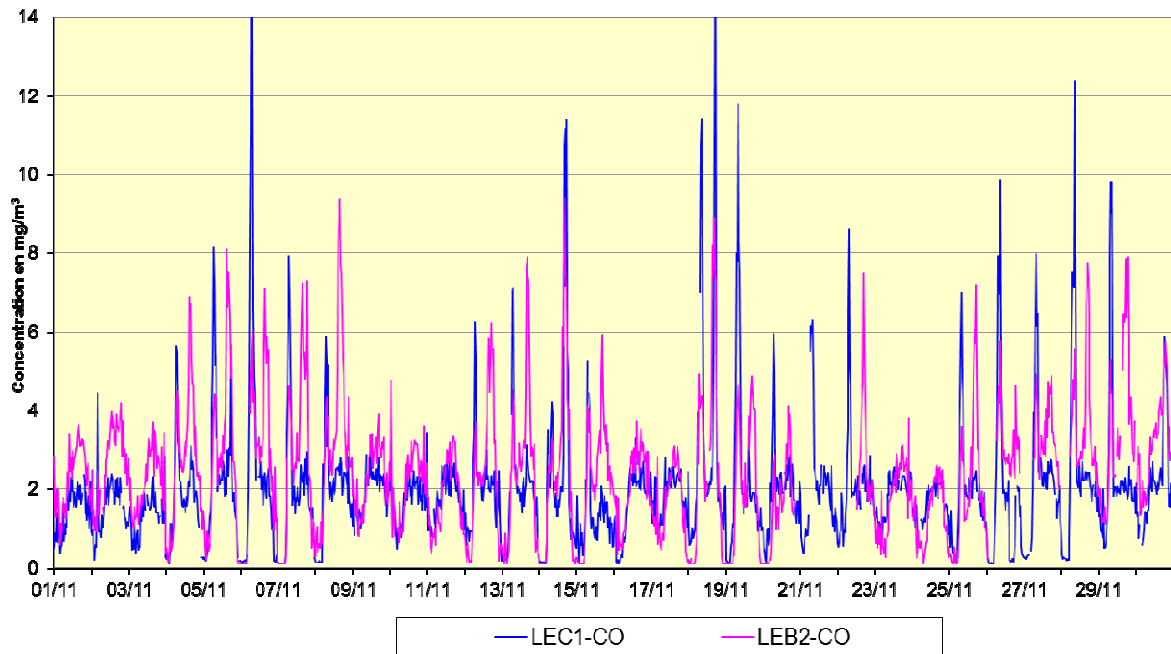
Fig. 3: CO - Évolution des valeurs horaires et semi horaires en novembre 2013 Poste de mesure 41LEC1, direction Centre – Poste de mesure 41LEB2, direction Basilique
