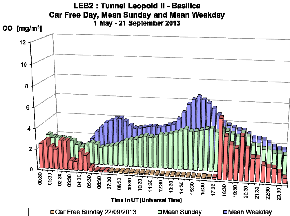
Fig. 32.a : CO dans le tunnel Léopold II, direction Basilique – Profil journalier du dimanche sans voiture, d'un dimanche moyen et d'un jour ouvrable moyen de la période 'mai – septembre 2013'.
