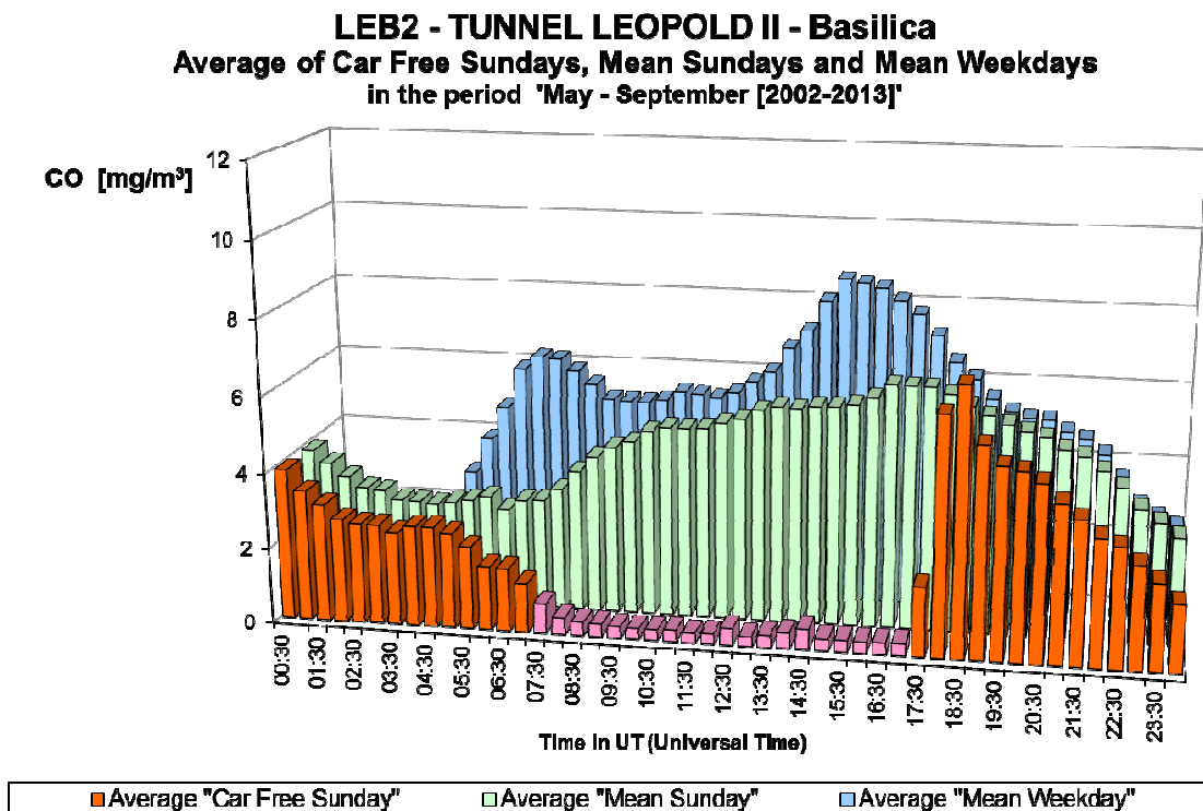
Fig. 32.b : CO dans le tunnel Léopold II, direction Basilique – Profil journalier sur les douze dimanches sans voiture et sur tous les dimanches et jours ouvrables des périodes 'mai – septembre 2002-2013'.
