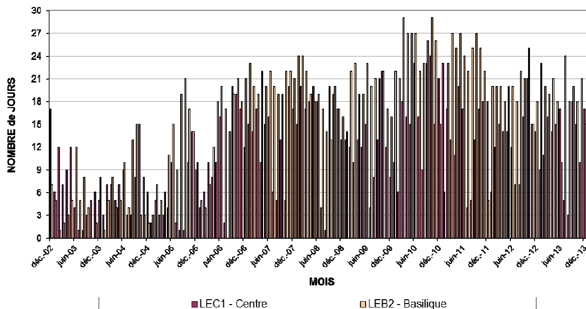
Fig. 13 : NO 2 – Valeurs Semi horaires > 850 µg/m 3 . Nombre de dépassements par mois et nombre de jours par mois avec dépassements (décembre 2002 – décembre 2013)
