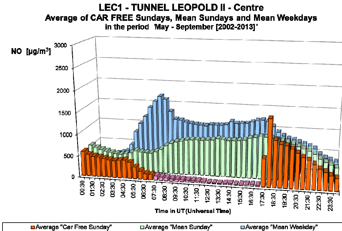
Fig. 29.b : NO dans le tunnel Léopold II, direction Centre – Profil journalier sur les douze dimanches sans voiture et sur tous les dimanches et jours ouvrables des périodes 'mai – septembre 2002-2013'.
