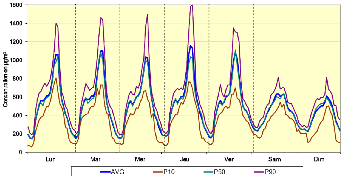
Fig. 22 : Poste de Mesure 41LEB2 (basilique) – Évolution hebdomadaire moyenne pour le NO 2 Période hivernale 2012 - 2013 et période estivale 2013
