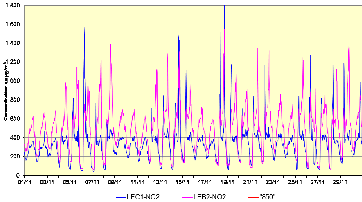
Fig. 1: NO 2 - Évolution des valeurs horaires et semi horaires en novembre 2013 Poste de mesure 41LEC1, direction Centre – Poste de mesure 41LEB2, direction Basilique
