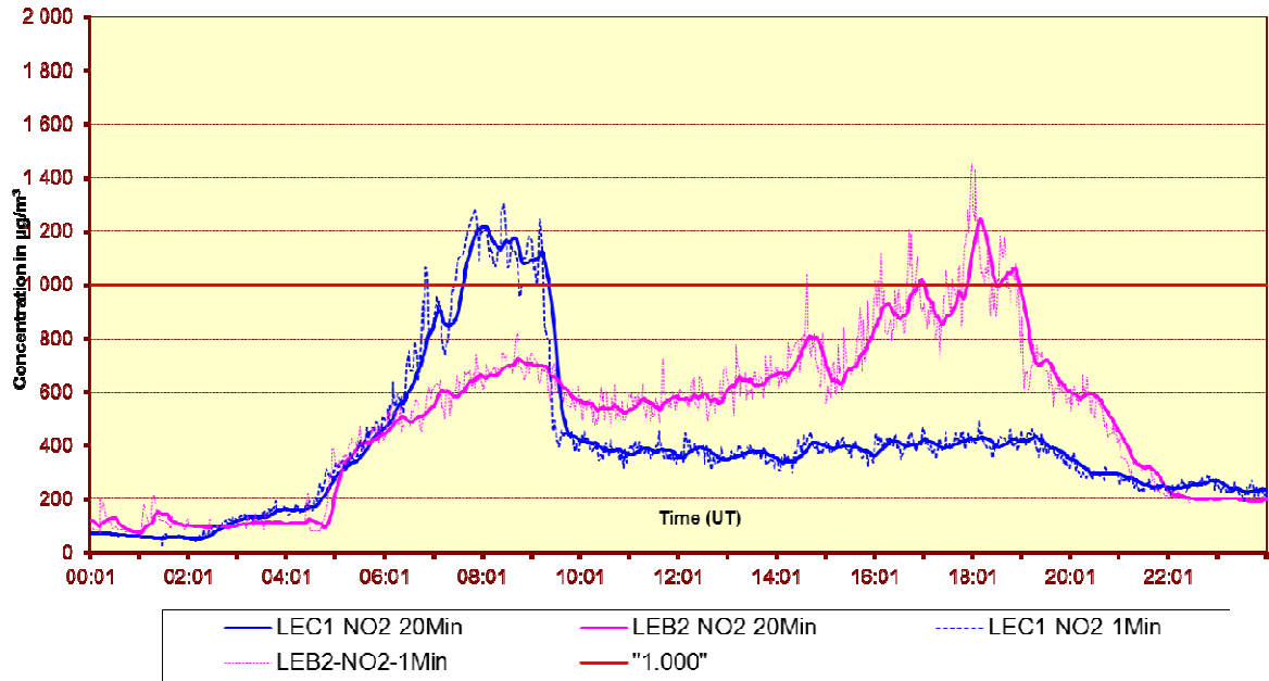
Fig. 4: NO 2 – évolution des valeurs minutes et de la moyenne glissante sur 20 minutes dans les deux postes de mesure du tunnel Léopold II Mardi 01 octobre 2013 et mardi 19 novembre 2013
