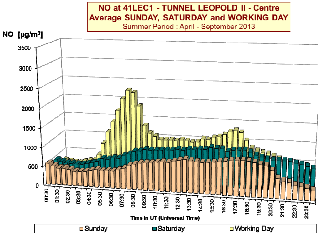
Fig. 17 : NO – évolution journalière moyenne au poste de mesure 41LEC1 (centre) Comparaison entre un dimanche, un samedi et un jour ouvrable moyen Période hivernale 2012-2013 et période estivale 2013
