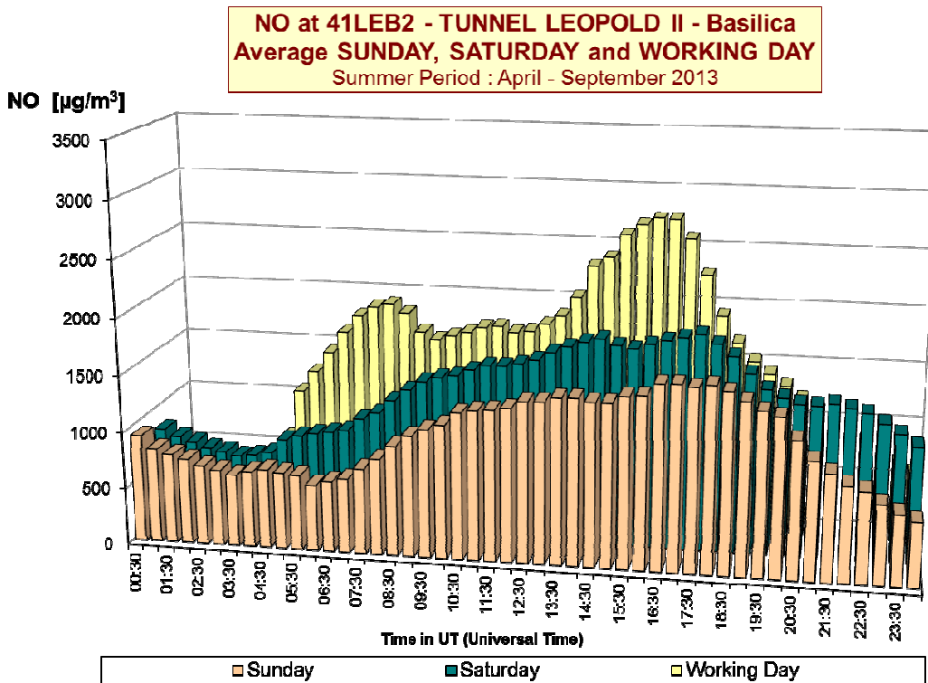
Fig. 18 : NO – évolution journalière moyenne au poste de mesure 41LEB2 (basilique) Comparaison entre un dimanche, un samedi et un jour ouvrable moyen Période hivernale 2012-2013 et période estivale 2013
