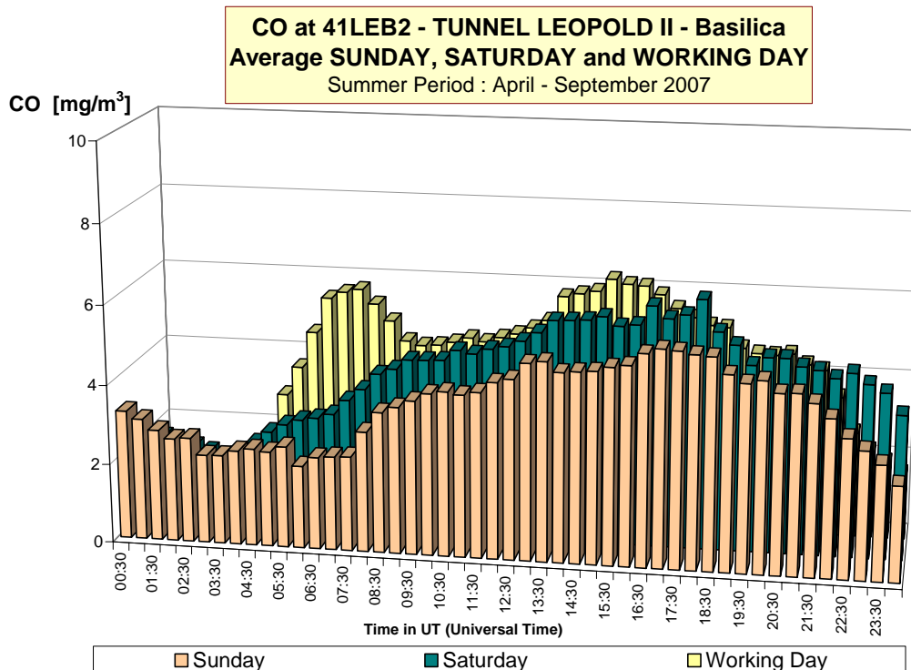
Fig. 20 : CO-dagverloop in de meetpost 41LEB2 (richting basiliek) Vergelijking voor een gemiddelde zondag, zaterdag en werkdag Winterperiode 2008-2009 en zomerperiode 2008
