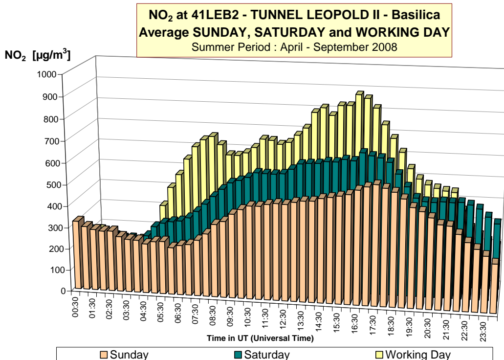
Fig. 16 : NO 2 -dagverloop in de meetpost 41LEB2 (richting basiliek) Vergelijking voor een gemiddelde zondag, zaterdag en werkdag Winterperiode 2008-2009 en zomerperiode 2008
