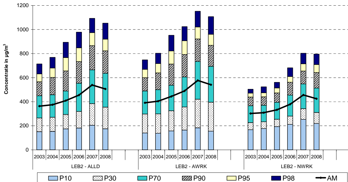
Fig. 5 : NO 2 - Cumulatieve Frequentieverdeling Uurwaarden in beide meetposten van de Leopold II tunnel. Selectie alle dagen , alle werkdagen en alle niet-werkdagen Jaarperiodes 2003 t/m 2008
