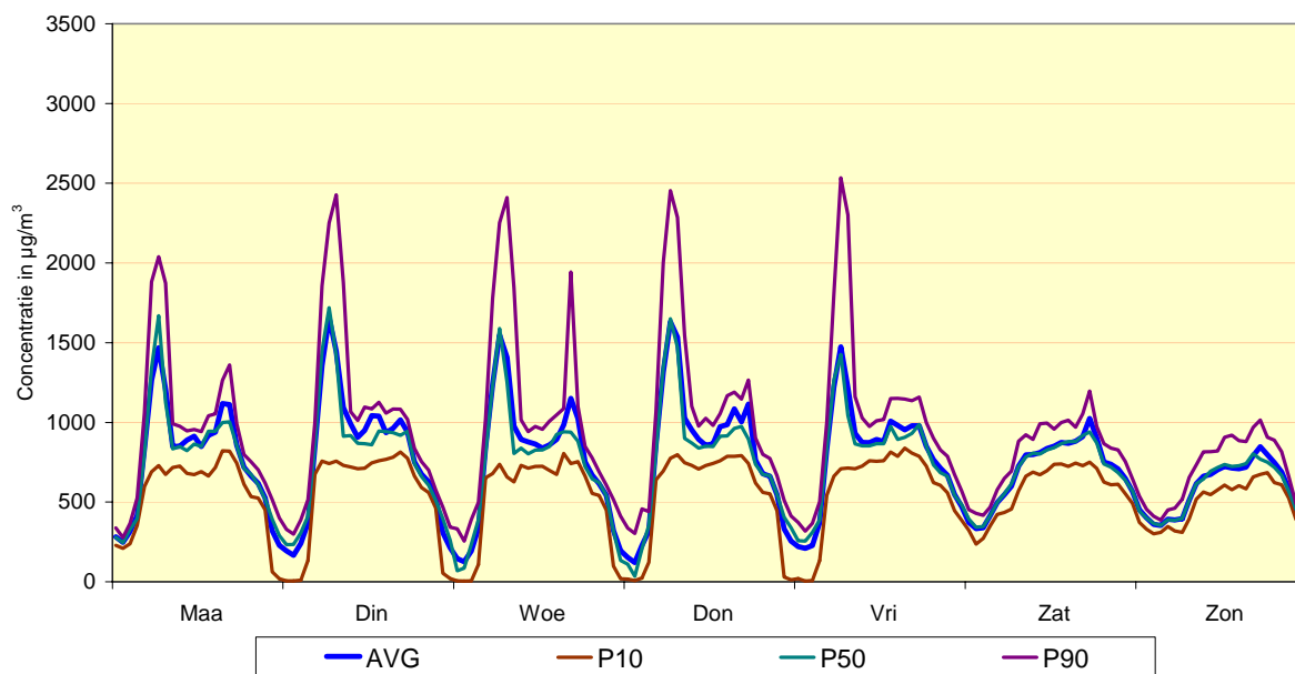
Fig. 25 : Meetpost 41LEC1 (centrum) - Gemiddeld weekverloop voor NO Vergelijking winterperiode 2008 - 2009 en zomerperiode 2008
