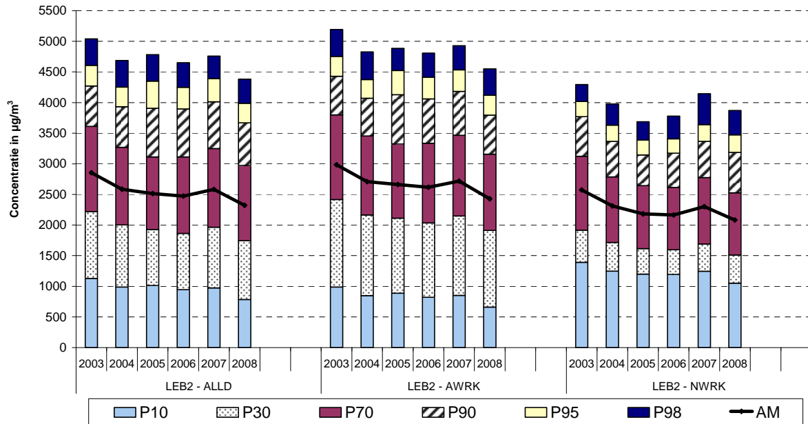
Fig. 8 : NO x - Cumulatieve Frequentieverdeling Uurwaarden in beide meetposten van de Leopold II tunnel. Selectie alle dagen , alle werkdagen en alle niet-werkdagen Jaarperiodes 2003 t/m 2008
