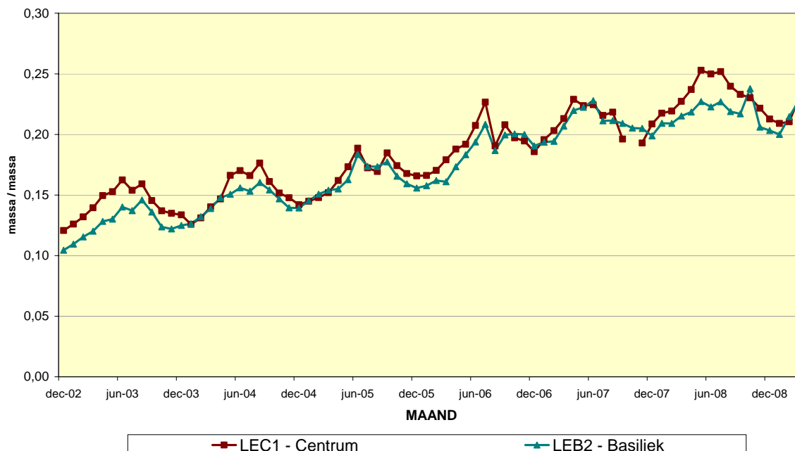
Fig. 11 : Evolutie van de verhouding NO 2 /NO x in beide meetposten van de Leopold II tunnel. Periode "December 2002 – Maart 2009"
