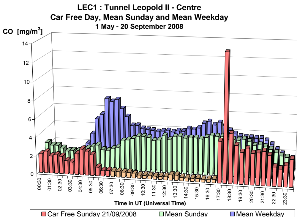
Fig. 31.a : CO in de Leopold II tunnel, richting Centrum – Dagprofiel autoluwte zondag 21-09-2008, gemiddelde zondag en gemiddelde werkdag in de periode ‘mei – september 2008’
