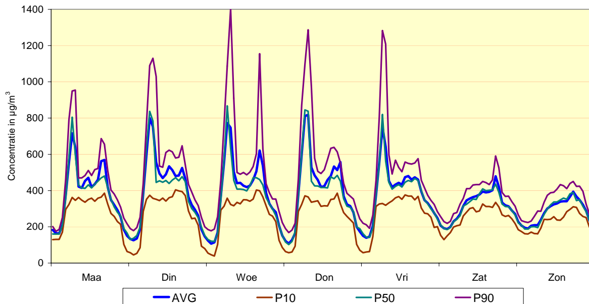
Fig. 21 : Meetpost 41LEC1 (centrum) - Gemiddeld weekverloop voor NO 2 Vergelijking winterperiode 2008 - 2009 en zomerperiode 2008
