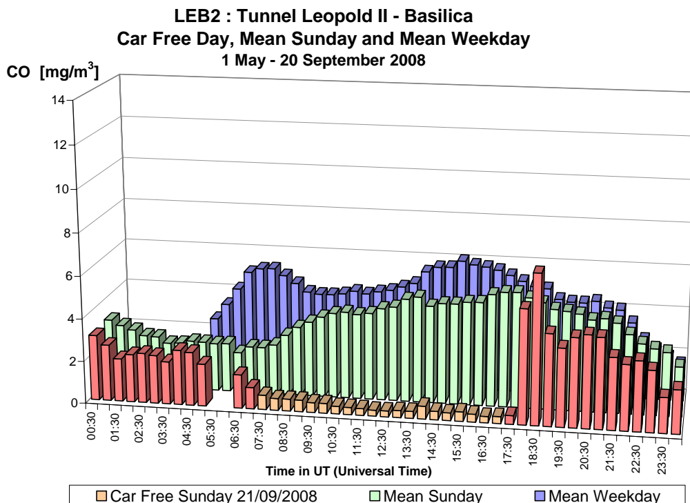
Fig. 32.a : CO in de Leopold II tunnel, richting Basiliek – Dagprofiel autoluwe zondag 21-09-2008, gemiddelde zondag en een gemiddelde werkdag in de periode 'mei – september 2008'
