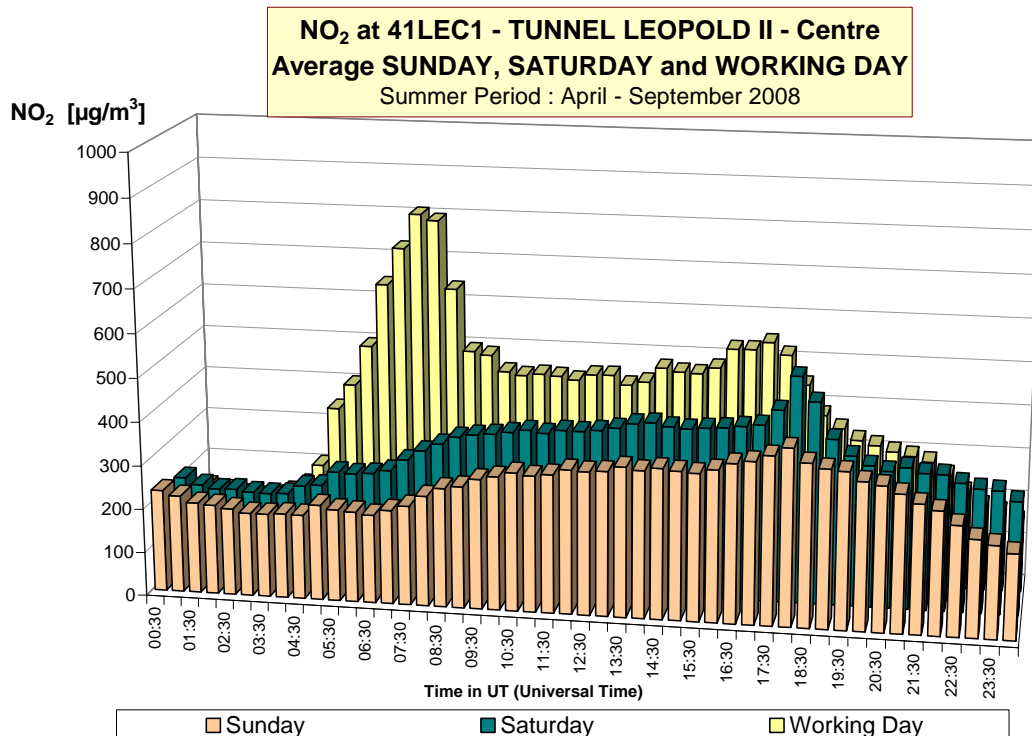
Fig. 15 : NO 2 -dagverloop in de meetpost 41LEC1 (richting centrum) Vergelijking voor een gemiddelde zondag, zaterdag en werkdag Winterperiode 2008-2009 en zomerperiode 2008
