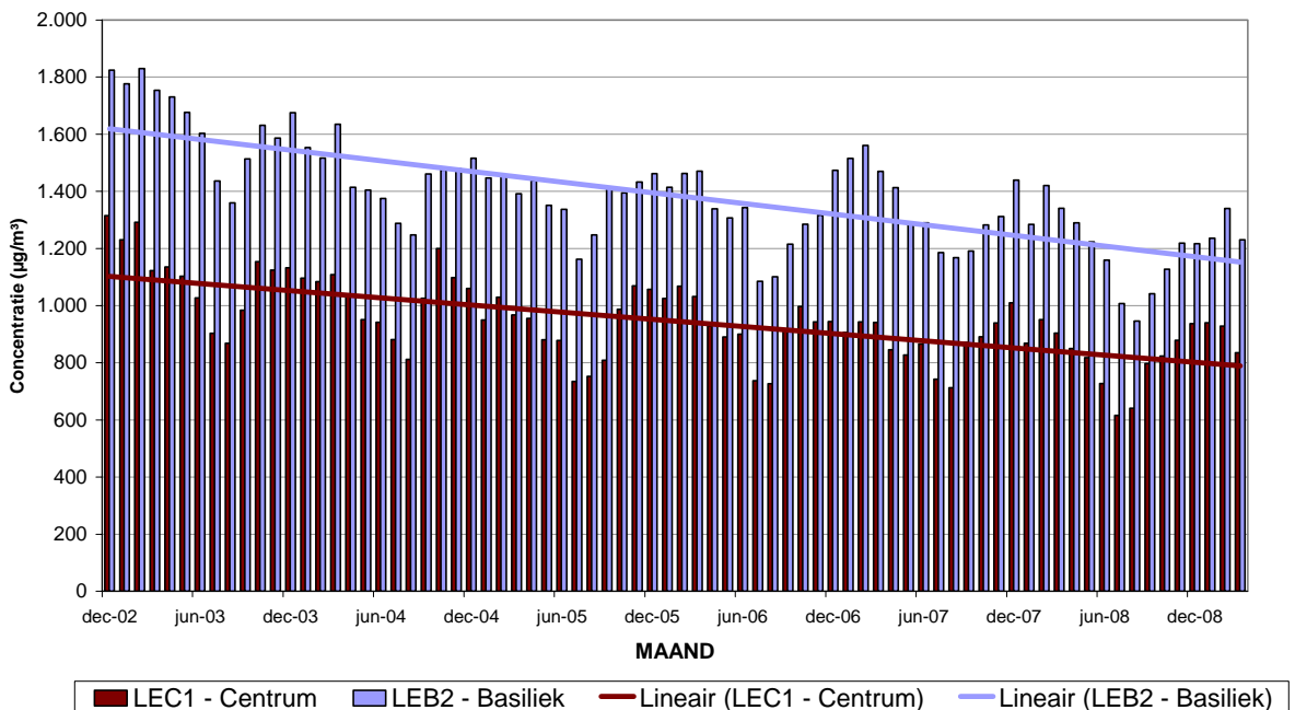
Fig. 9 : NO 2 en NO - Evolutie maandgemiddelde concentratie in beide meetposten van de Leopold II tunnel. Periode "December 2002 – Maart 2009"
