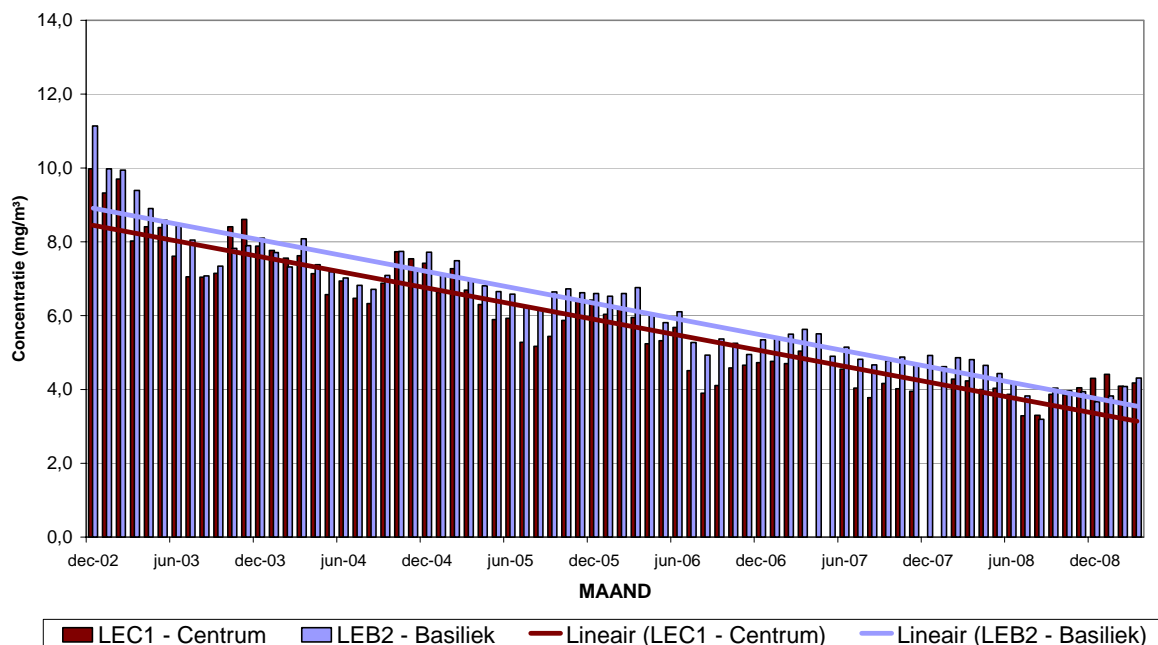
Fig. 10 : NO x en CO - Evolutie maandgemiddelde concentratie in beide meetposten van de Leopold II tunnel. Periode "December 2002 – Maart 2009"
