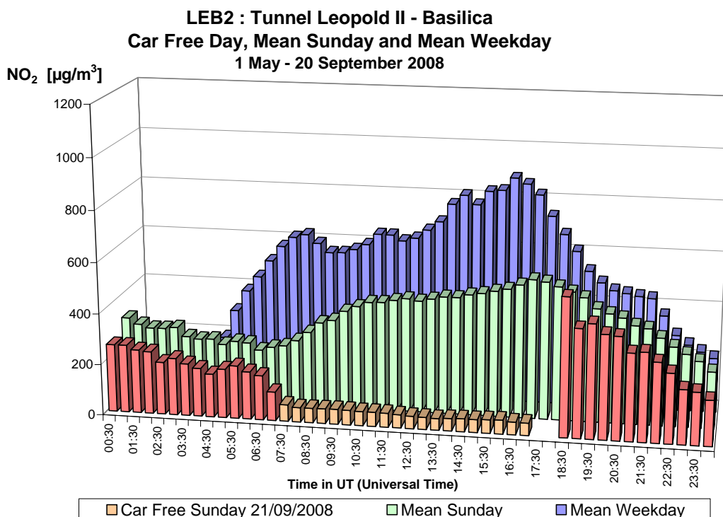
Fig. 28.a : NO 2 in de Leopold II tunnel, richting Basiliek – Dagprofiel autoluwe zondag 21-09-2008, gemiddelde zondag en een gemiddelde werkdag in de periode ‘mei – september 2008’
