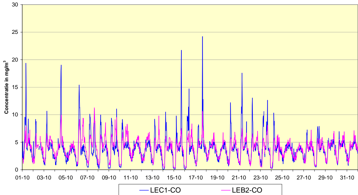
Fig. 3: CO - Evolutie van de uurwaarden en de halfuurwaarden tijdens de maand oktober 2008 Meetplaats 41LEC1, richting Centrum - Meetplaats 41LEB2, richting Basiliek
