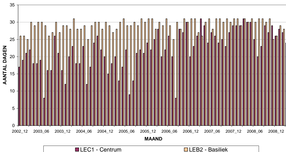
Fig. 14 : NO 2 -Uurwaarden > 400 µg/m 3 . Totaal aantal overschrijdingen per maand en aantal dagen per maand met overschrijding (december 2002 – maart 2009)
