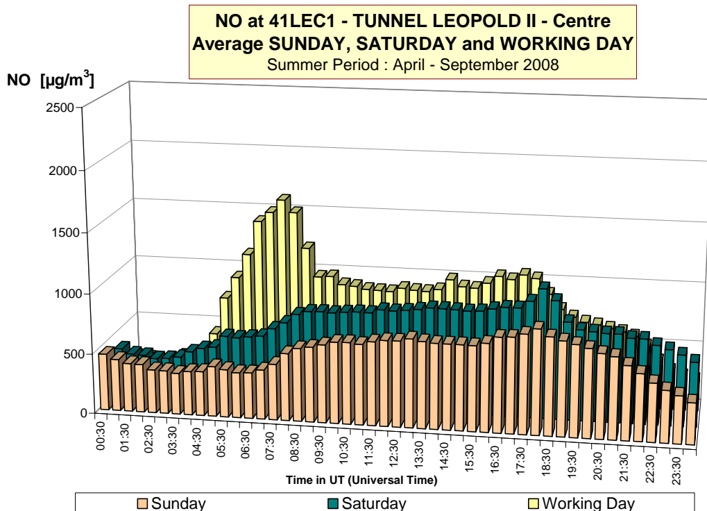
Fig. 17 : NO-dagverloop in de meetpost 41LEC1 (richting centrum) Vergelijking voor een gemiddelde zondag, zaterdag en werkdag Winterperiode 2008-2009 en zomerperiode 2008
