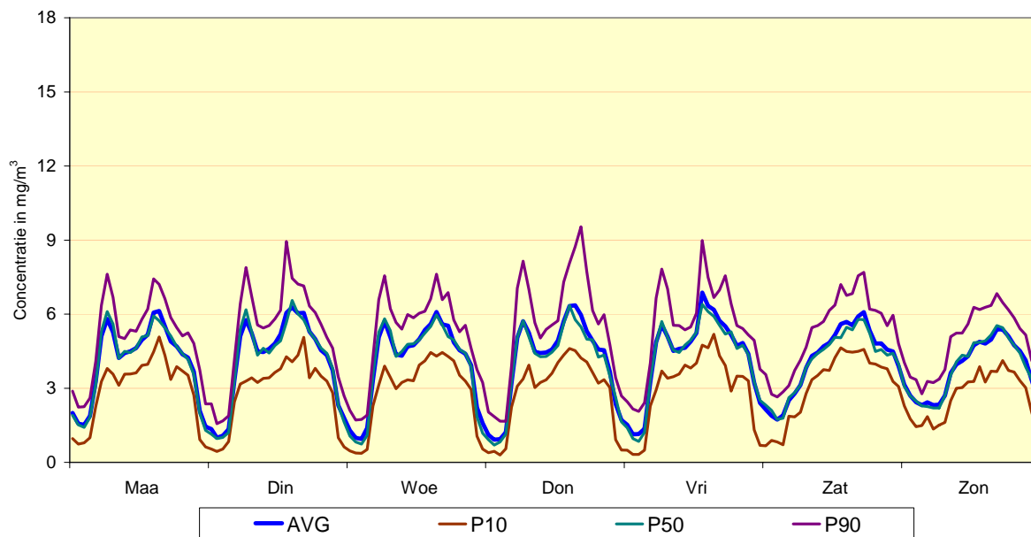
Fig. 24 : Meetpost 41LEB2 (basiliek) - Gemiddeld weekverloop voor CO Vergelijking winterperiode 2008 - 2009 en zomerperiode 2008
