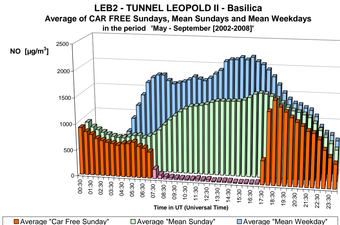
Fig. 30.b : NO in de Leopold II tunnel, richting Basiliek – Gemiddelde Dagprofiel van de zeven autoluwe zondagen en van alle zondagen en werkdagen in de periodes ‘mei – september 2002-2008’
