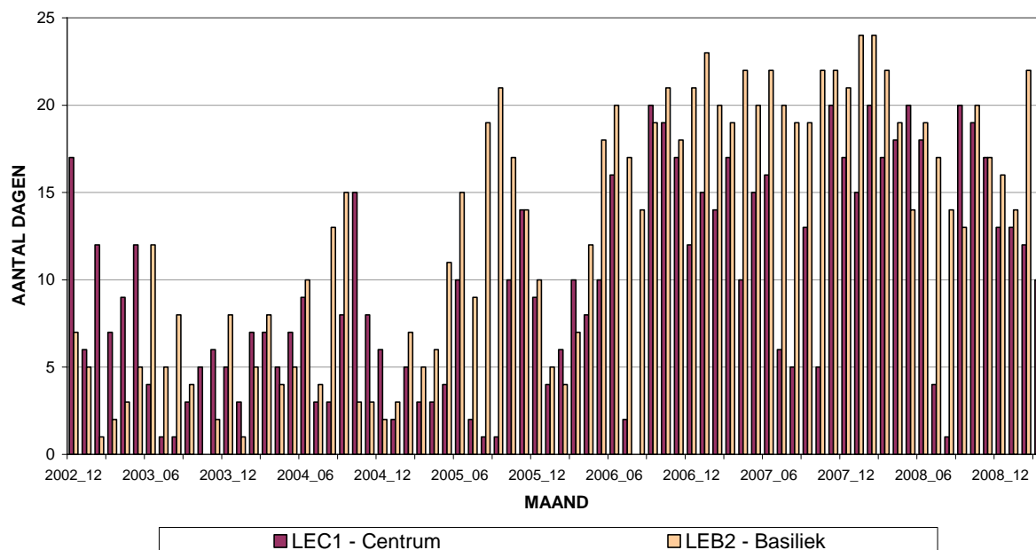
Fig. 13 : NO 2 – Halfuurswaarden > 850 µg/m 3 . Totaal aantal overschrijdingen per maand en aantal dagen per maand met overschrijding (december 2002 – maart 2009)
