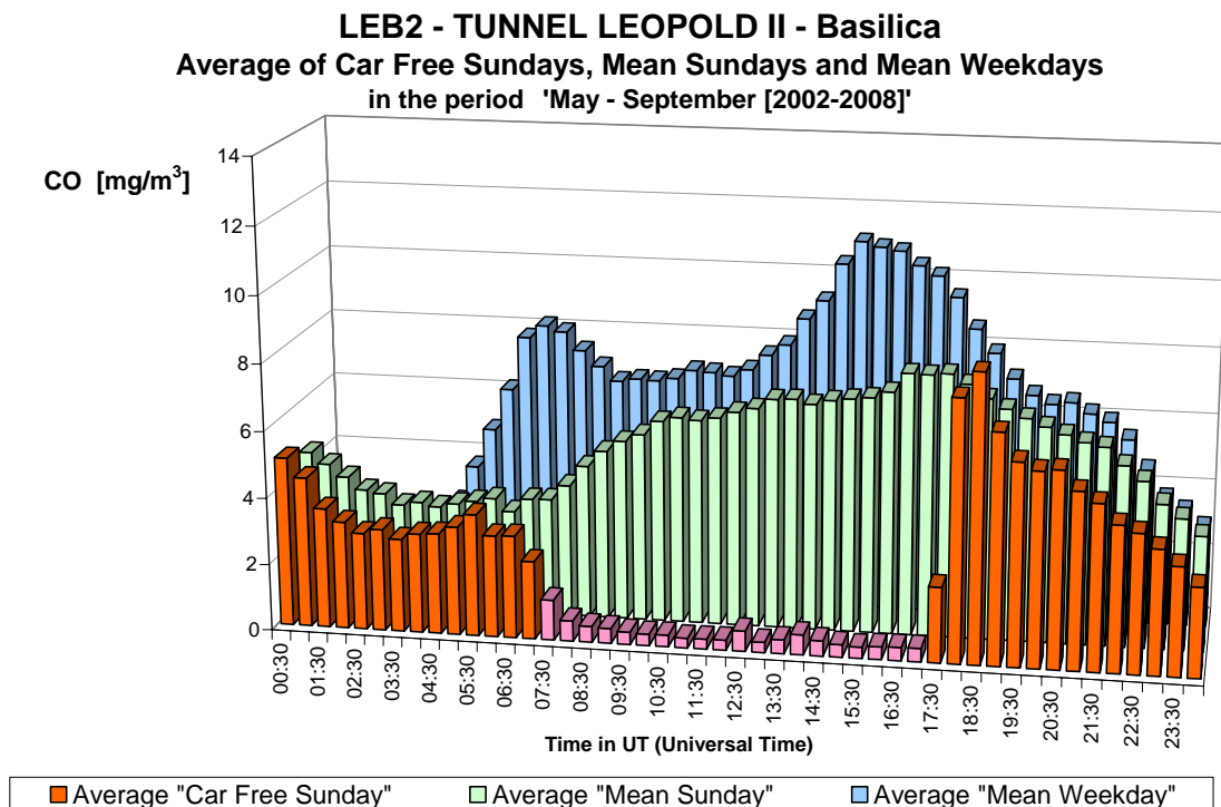
Fig. 32.b : CO in de Leopold II tunnel, richting Basiliek – Gemiddelde Dagprofiel van de zeven autoluwe zondagen en van alle zondagen en werkdagen in de periodes 'mei – september 2002-2008'
