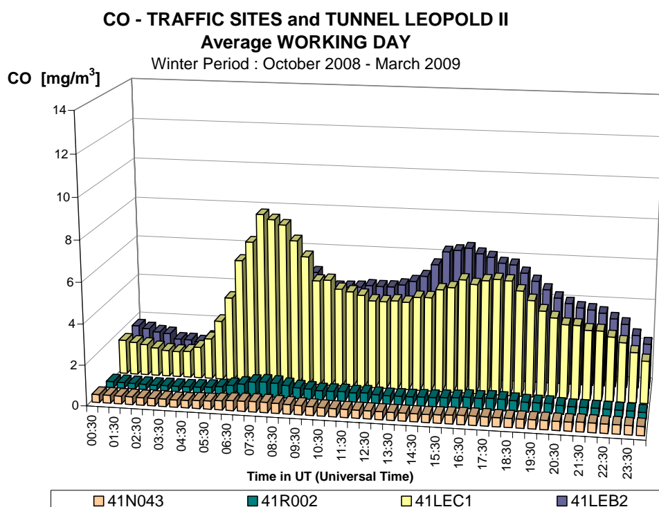
Fig. 33 : CO-dagverloop voor een gemiddelde werkdag tijdens de winter 2008-2009 Meetposten verkeer in de omgevingslucht – Voorhaven (N043) en Kroonlaan (R002) Meetposten in de tunnel Leopold II – LEC1 (centrum) en LEC2 (basiliek)
