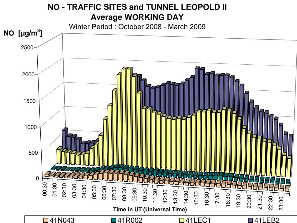
Fig. 34 : Dagverloop NO 2 en NO voor een gemiddelde werkdag tijdens de winter 2008-2009 Meetposten verkeer in de omgevingslucht – Voorhaven (N043) en Kroonlaan (R002) Meetposten in de tunnel Leopold II – LEC1 (centrum) en LEC2 (basiliek)
