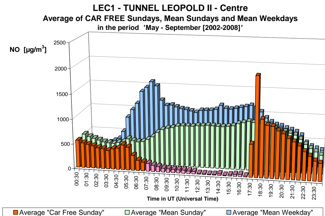
Fig. 29.b : NO in de Leopold II tunnel, richting Centrum – Gemiddelde Dagprofiel van de zeven autoluwe zondagen en van alle zondagen en werkdagen in de periodes ‘mei – september 2002-2008’
