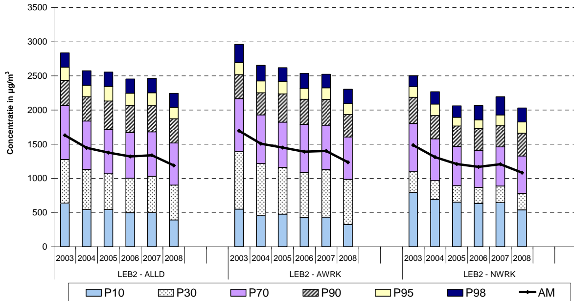
Fig. 7 : NO - Cumulatieve Frequentieverdeling Uurwaarden in beide meetposten van de Leopold II tunnel. Selectie alle dagen , alle werkdagen en alle niet-werkdagen Jaarperiodes 2003 t/m 2008
