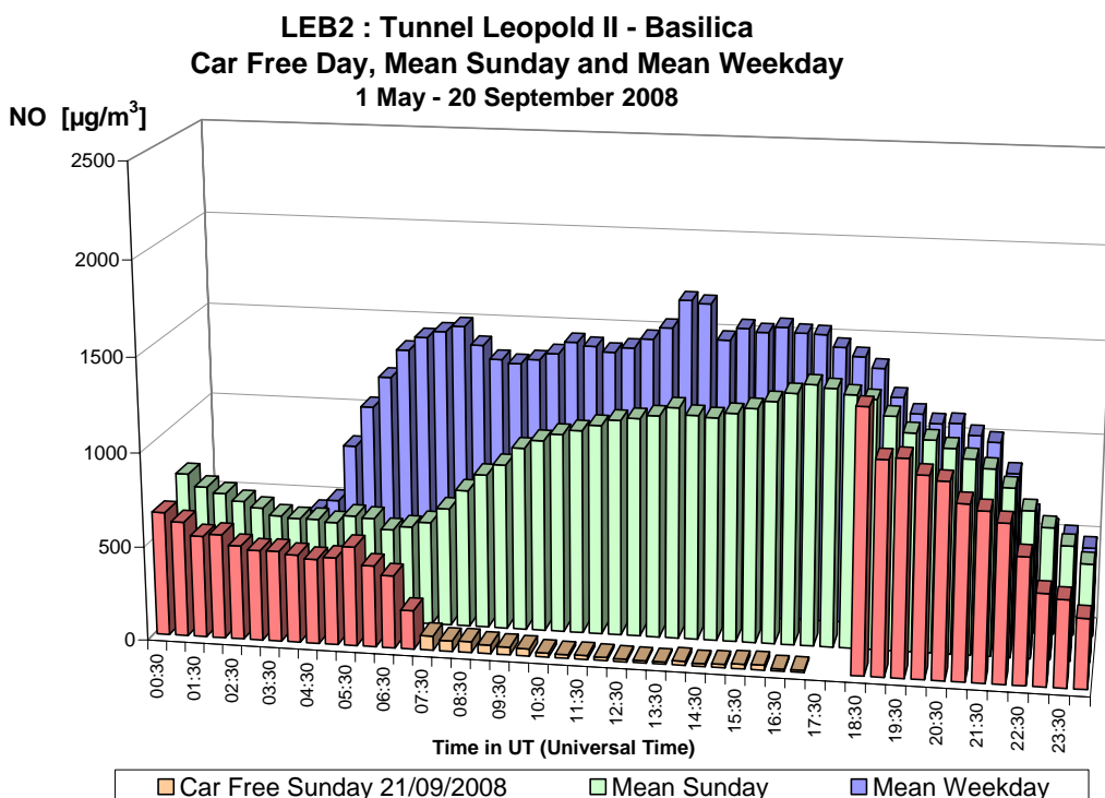
Fig. 30.a : NO in de Leopold II tunnel, richting Basiliek – Dagprofiel autoluwe zondag 21-09-2008, gemiddelde zondag en een gemiddelde werkdag in de periode ‘mei – september 2008’
