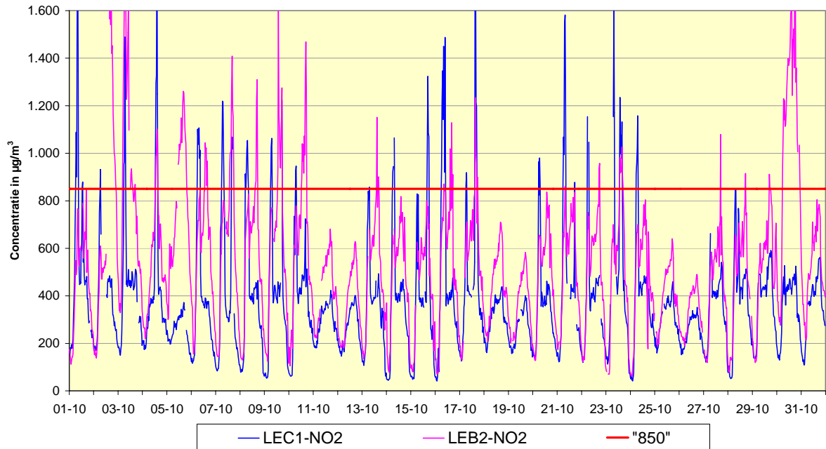
Fig. 1: NO 2 - Evolutie van de uurwaarden en de halfuurwaarden tijdens de maand oktober 2008 Meetplaats 41LEC1, richting Centrum - Meetplaats 41LEB2, richting Basiliek
