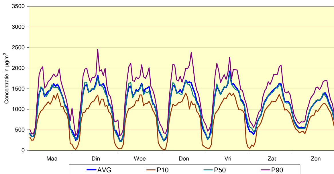
Fig. 26 : Meetpost 41LEB2 (basiliek) - Gemiddeld weekverloop voor NO Vergelijking winterperiode 2008 - 2009 en zomerperiode 2008
