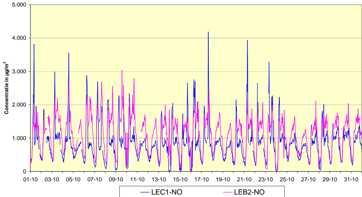
Fig. 2: NO - Evolutie van de uurwaarden en de halfuurwaarden tijdens de maand oktober 2008 Meetplaats 41LEC1, richting Centrum - Meetplaats 41LEB2, richting Basiliek
