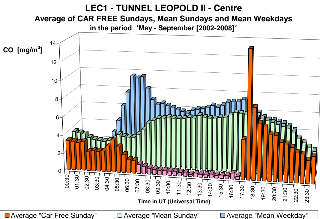
Fig. 31.b : CO in de Leopold II tunnel, richting Centrum – Gemiddelde Dagprofiel van de zeven autoluwte zondagen en van alle zondagen en werkdagen in de periodes ‘mei – september 2002-2008’
