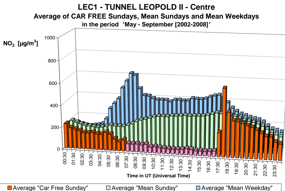
Fig. 27.b : NO 2 in de Leopold II tunnel, richting Centrum – Gemiddelde Dagprofiel van de zeven autoluwe zondagen en van alle zondagen en werkdagen in de periodes ‘mei – september 2002-2008’
