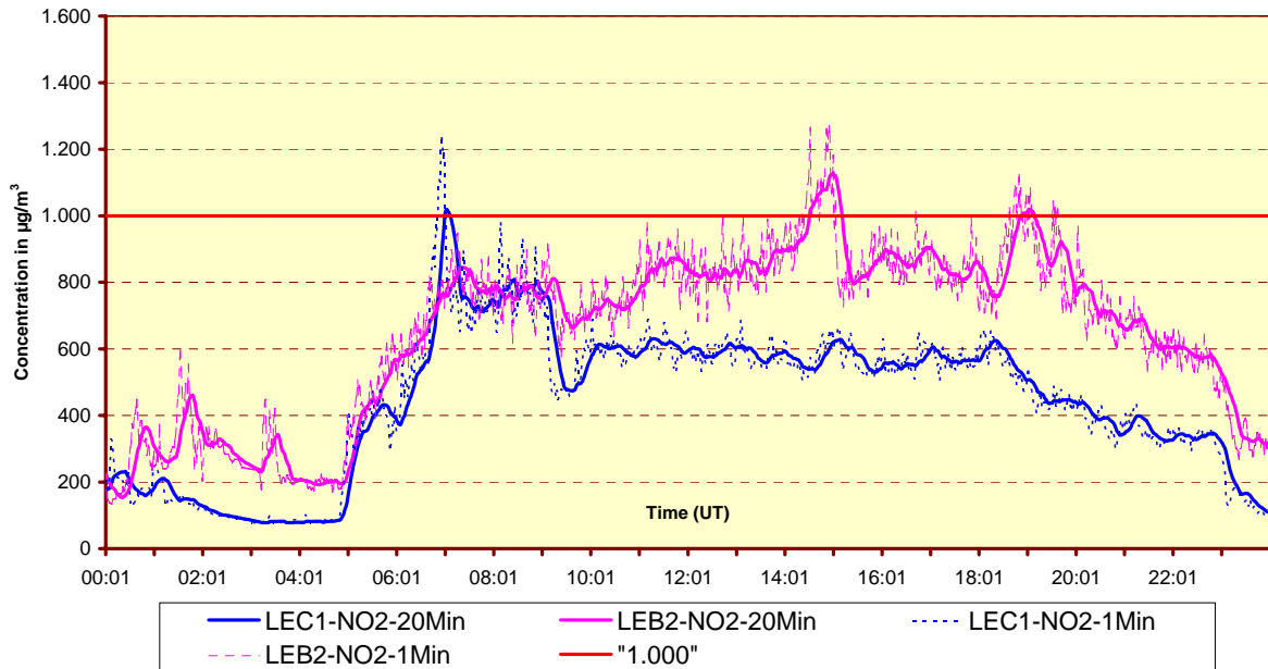
Fig. 4: NO 2 - evolutie minuutwaarden en voortschrijdend 20-minuutsgemiddelde in beide meetposten van de Leopold II tunnel Dinsdag 2 december 2008 en woensdag 18 februari 2009
