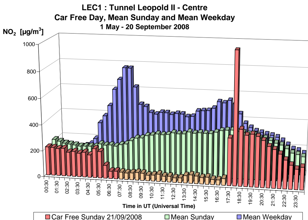
Fig. 27.a : NO 2 in de Leopold II tunnel, richting Centrum – Dagprofiel autoluwe zondag 21-09-2008, gemiddelde zondag en gemiddelde werkdag in de periode ‘mei – september 2008’
