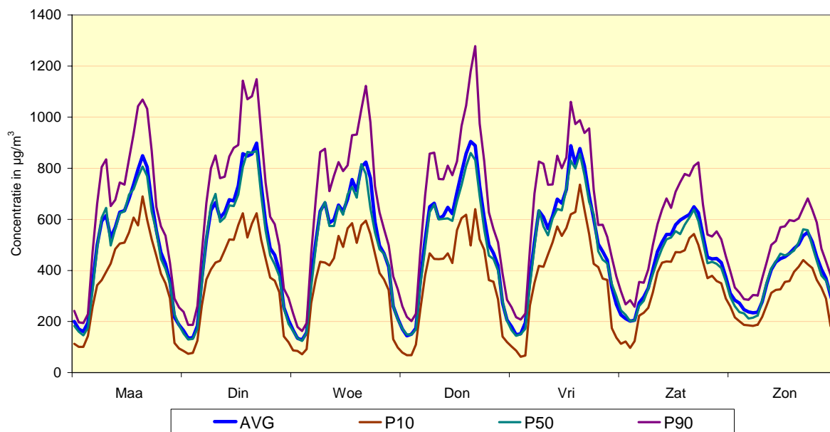
Fig. 22 : Meetpost 41LEB2 (basiliek) - Gemiddeld weekverloop voor NO 2 Vergelijking winterperiode 2008 - 2009 en zomerperiode 2008
