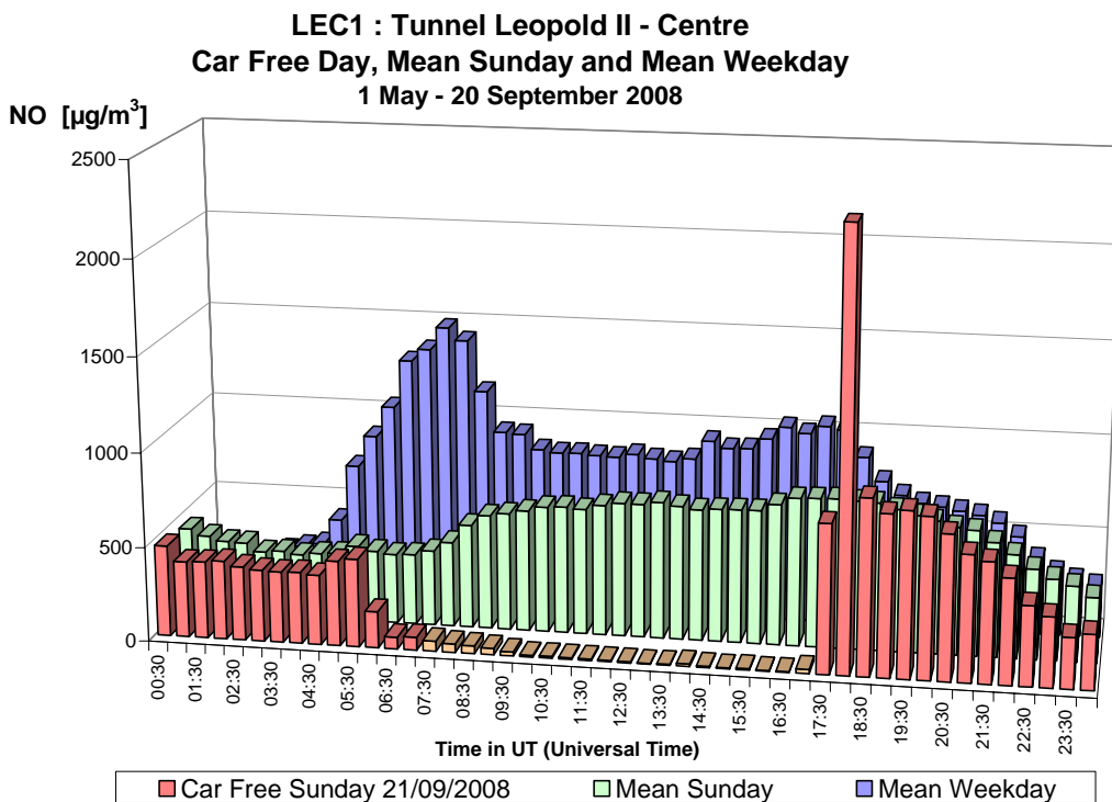
Fig. 29.a : NO in de Leopold II tunnel, richting Centrum – Dagprofiel autoluwe zondag 21-09-2008, gemiddelde zondag en gemiddelde werkdag in de periode ‘mei – september 2008’
