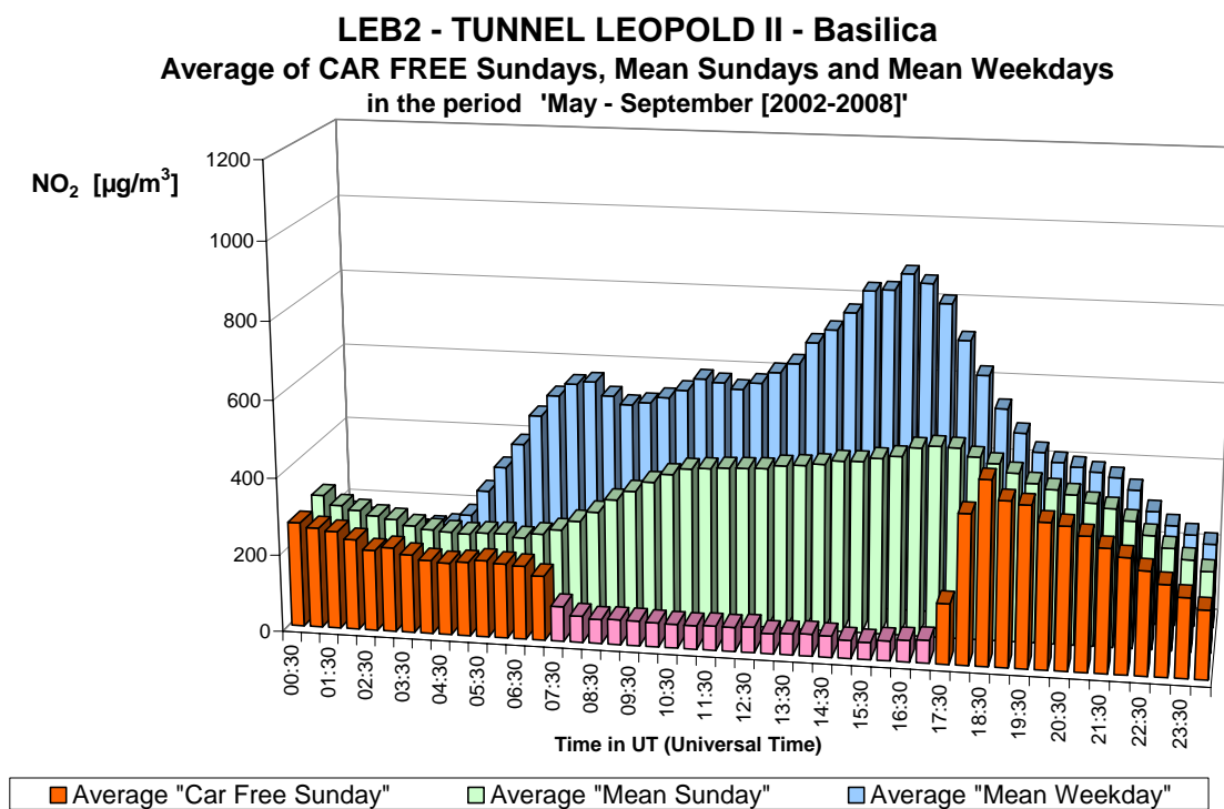
Fig. 28.b : NO 2 in de Leopold II tunnel, richting Basiliek – Gemiddelde Dagprofiel van de zeven autoluwe zondagen en van alle zondagen en werkdagen in de periodes ‘mei – september 2002-2008’
