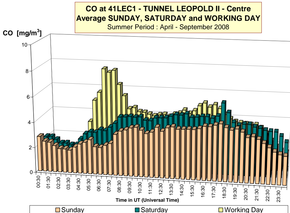
Fig. 19 : CO-dagverloop in de meetpost 41LEC1 (richting centrum) Vergelijking voor een gemiddelde zondag, zaterdag en werkdag Winterperiode 2008-2009 en zomerperiode 2008
