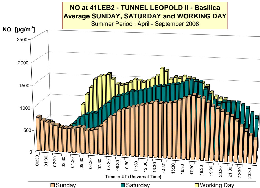
Fig. 18 : NO-dagverloop in de meetpost 41LEB2 (richting basiliek) Vergelijking voor een gemiddelde zondag, zaterdag en werkdag Winterperiode 2008-2009 en zomerperiode 2008
