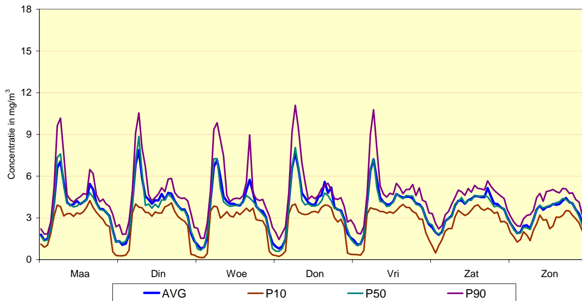
Fig. 23 : Meetpost 41LEC1 (centrum) - Gemiddeld weekverloop voor CO Vergelijking winterperiode 2008 - 2009 en zomerperiode 2008
