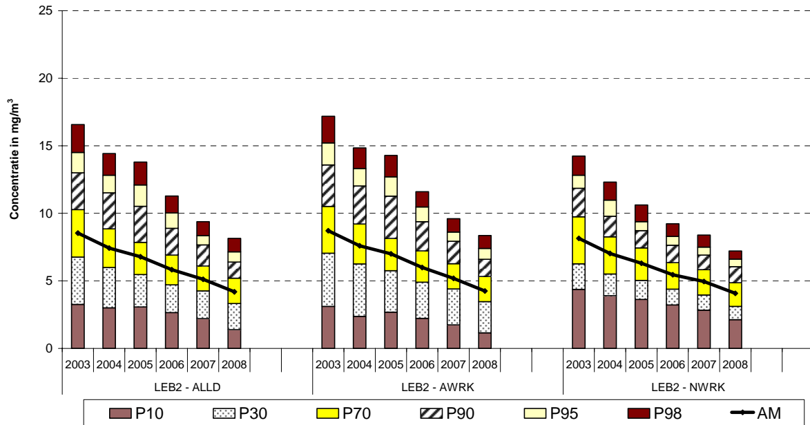
Fig. 6 : CO - Cumulatieve Frequentieverdeling Uurwaarden in beide meetposten van de Leopold II tunnel. Selectie alle dagen , alle werkdagen en alle niet-werkdagen Jaarperiodes 2003 t/m 2008
