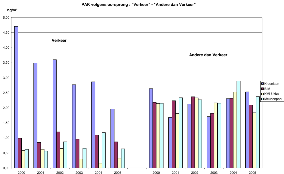
Fig. 4.60: Evolutie van de concentratie van vaste PAK-deeltjes in 4 verschillende meetposten Onderscheid volgens oorsprong "Verkeer" en "niet-Verkeer" Periode : 2000 - 2005
