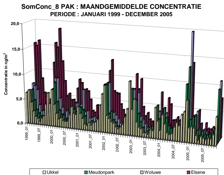
Fig. 4.59: Evolutie van de maandgemiddelde concentratie voor de somconcentratie van 8 verschillende PAK's in vier meetposten. Periode : januari 1999 - december 2005
