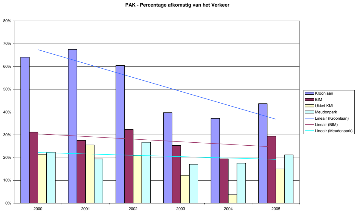
Fig. 4.61: Evolutie percentage vaste PAK-deeltjes afkomstig van het verkeer Periode : 2000 - 2005
