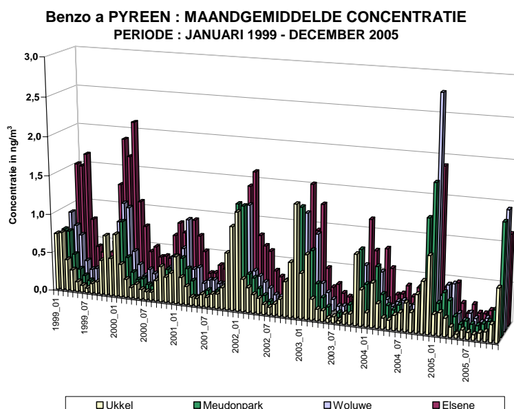
Fig. 4.58: Evolutie van de maandgemiddelde concentratie voor benzo a pyreen in vier meetposten. Periode : januari 1999 - december 2005
