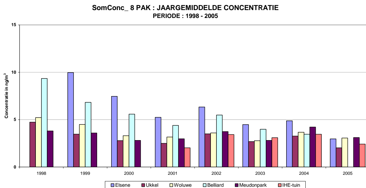
Fig. 4.57: Evolutie van de jaargemiddelde concentratie voor de somconcentratie van 8 verschillende polycyclische aromatische koolwaterstoffen. Periode : 1998 - 2005
