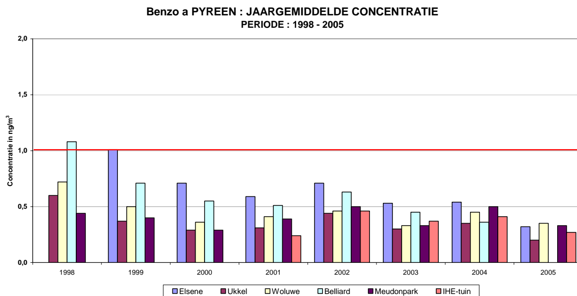
Fig. 4.56: Evolutie van de jaargemiddelde concentratie voor benzo a pyreen Periode : 1998 - 2005
