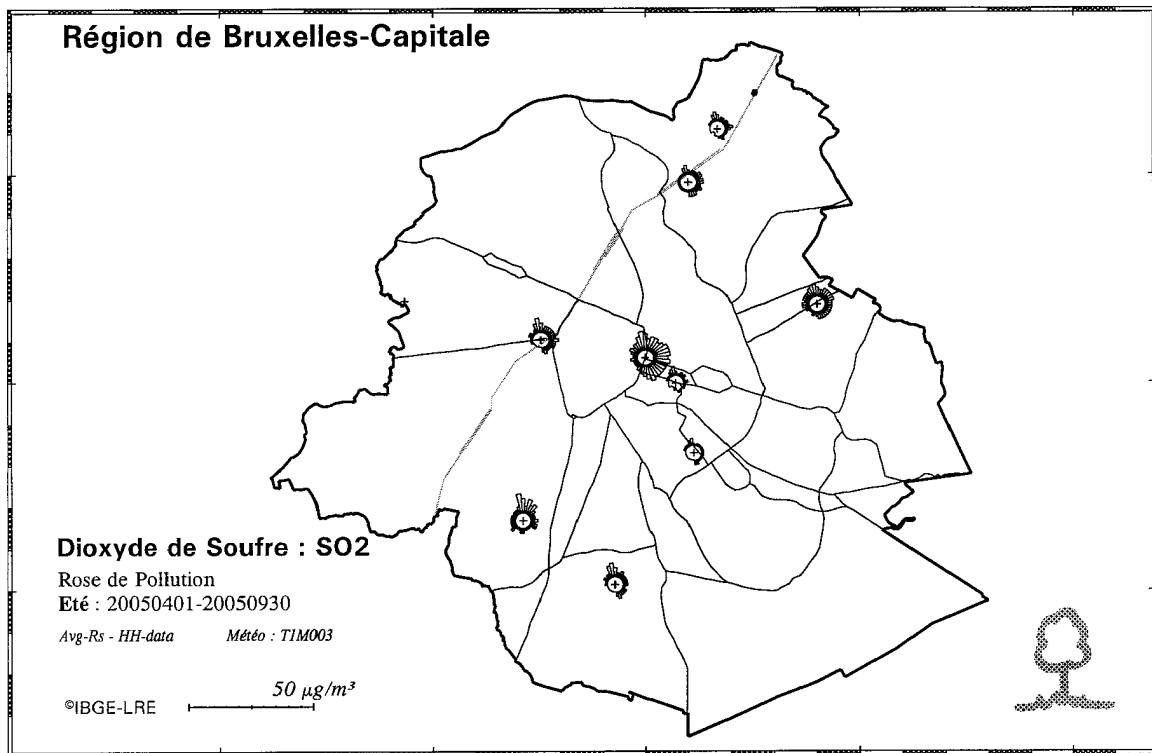
Fig. 4.72: SO 2 roses de pollution - dispersion spatiale de la concentration pendant l'hiver et l'été
