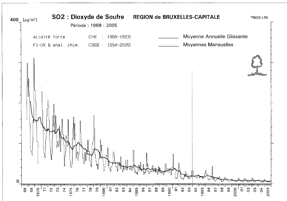
Fig. 4.71: SO 2 - évolution de la concentration à long terme (1968-2005)
