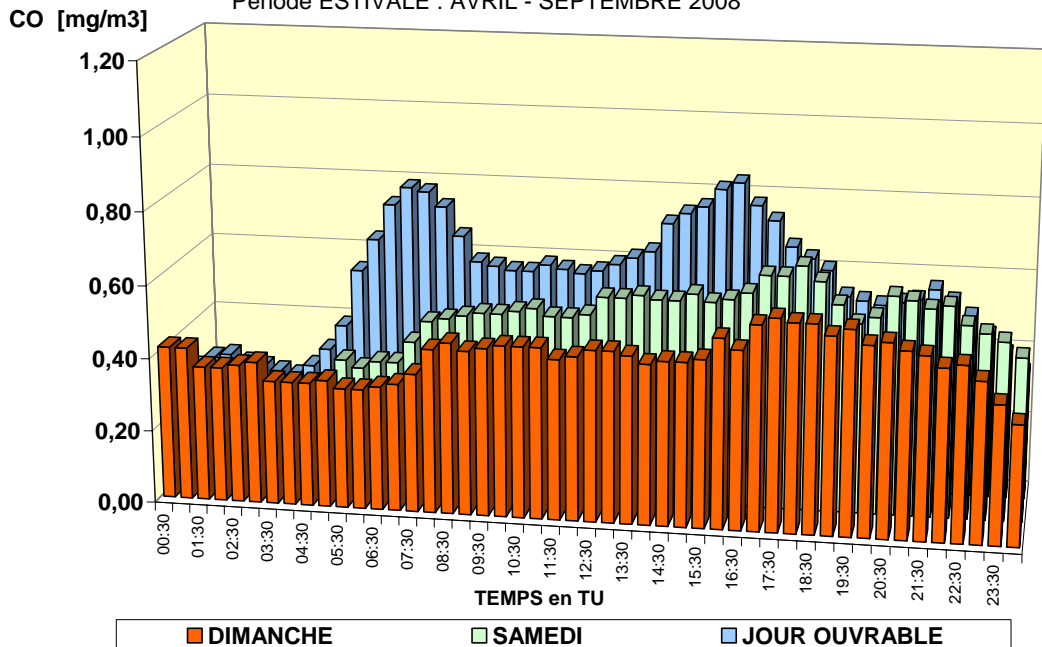
Fig. 4.103: Évolution journalière moyenne en CO pendant l'hiver et l'été (dimanche, samedi et jour ouvrable) - Poste de mesure Arts-Loi (B003)
