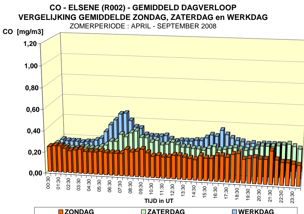
Fig. 4.104: Gemiddeld CO-dagverloop tijdens winter en zomer (zondag, zaterdag, werkdag) Meetpost Elsene-Kroonlaan (R002)
