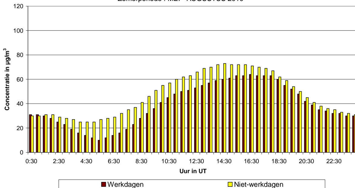
Fig. 49.a : Voorhaven : Gemiddeld dagverloop van de O 3 -concentratie op werkdagen en niet-werkdagen tijdens de periode mei - augustus 2010
