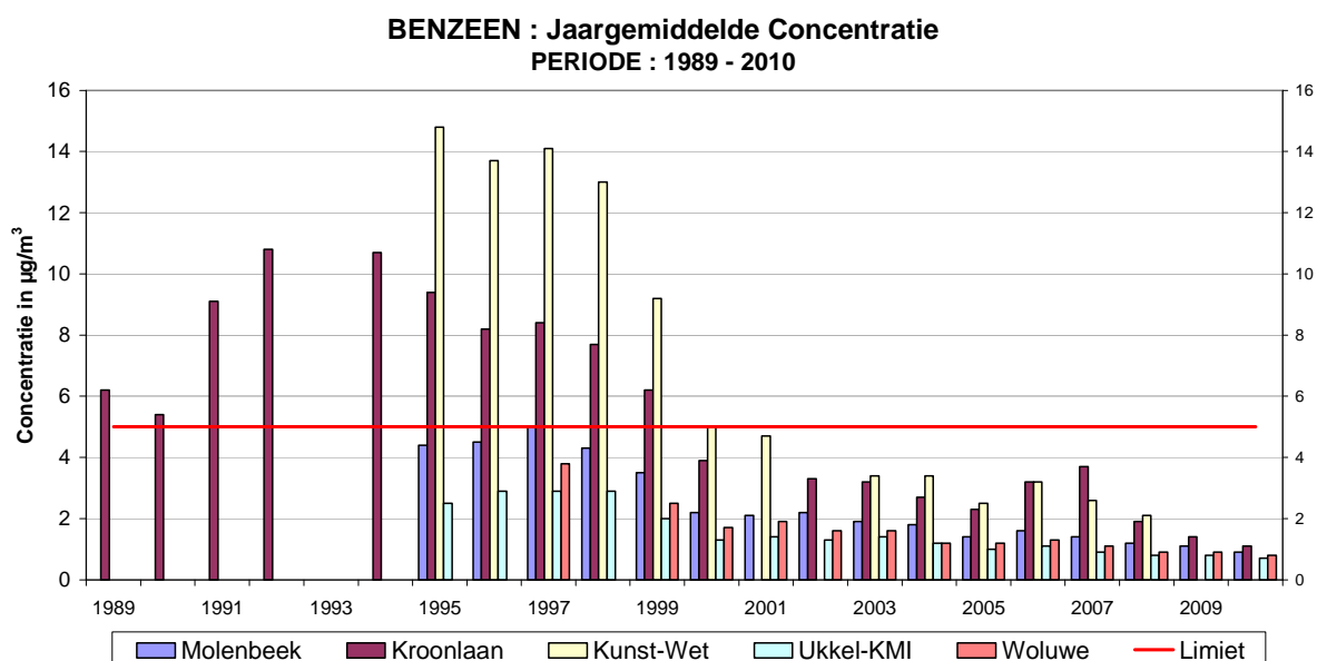
Fig. 28 : Benzeen - Evolutie jaargemiddelde concentratie Periode : Januari – December (1989-2009) en 'Januari – September 2010'
