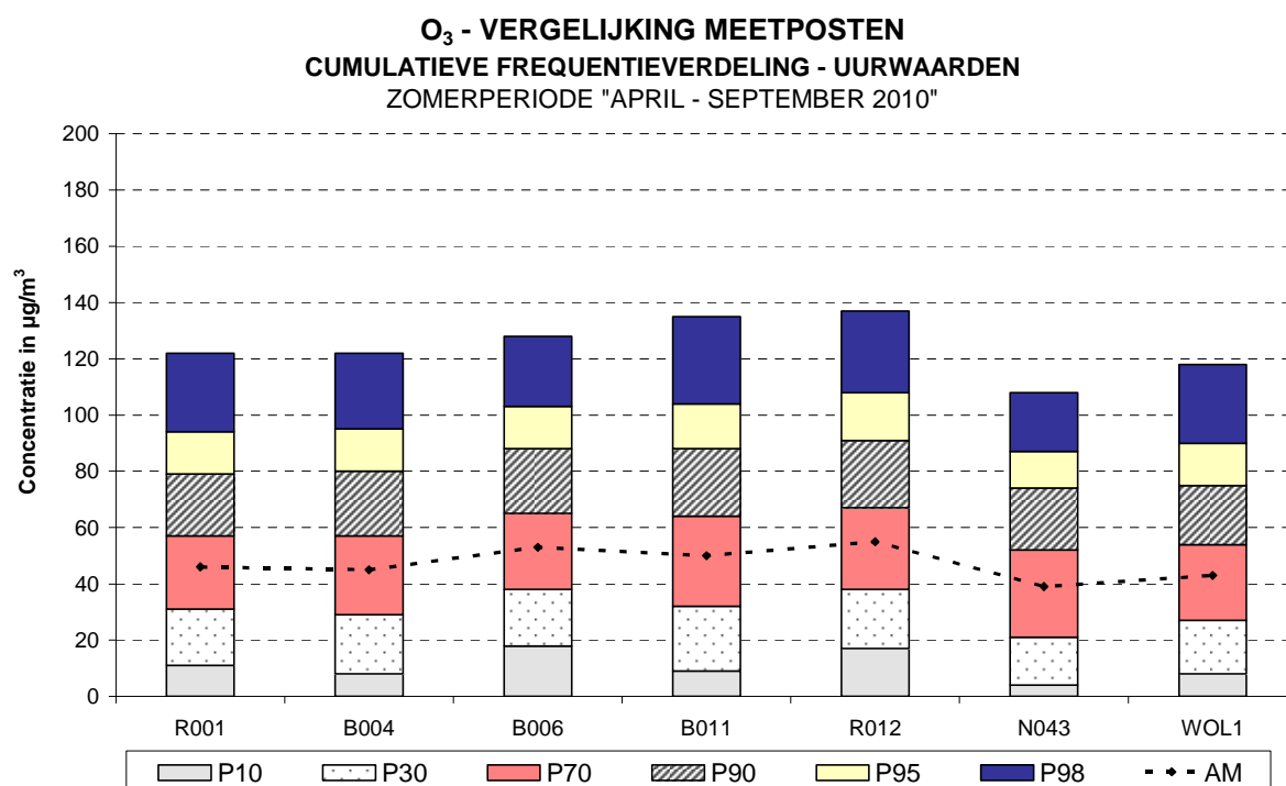
Fig. 32 : Ozon - Cumulatieve frequentieverdeling uurwaarden : april - september 2010
