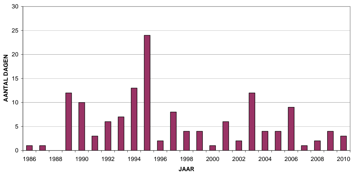
Fig. 17 : Ozon - Evolutie aantal overschrijdingsdagen in het Brussels Hoofdstedelijk Gewest
