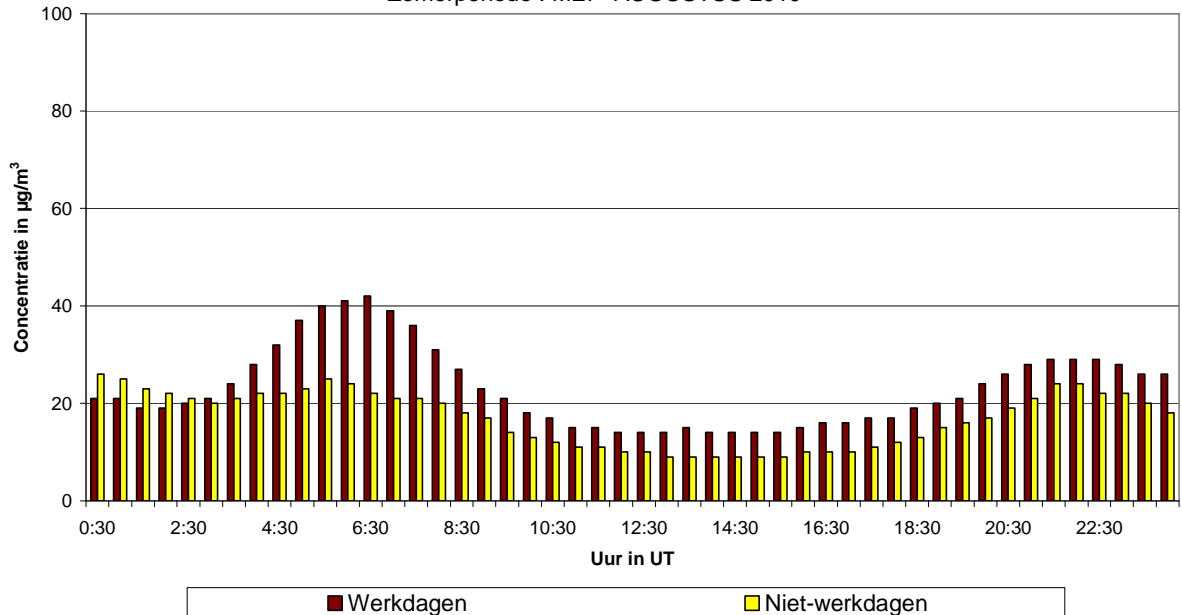
Fig. 47.b : St.-Agatha-Berchem : Gemiddeld dagverloop van de NO 2 -concentratie op werkdagen en niet-werkdagen tijdens de periode mei – augustus 2010
