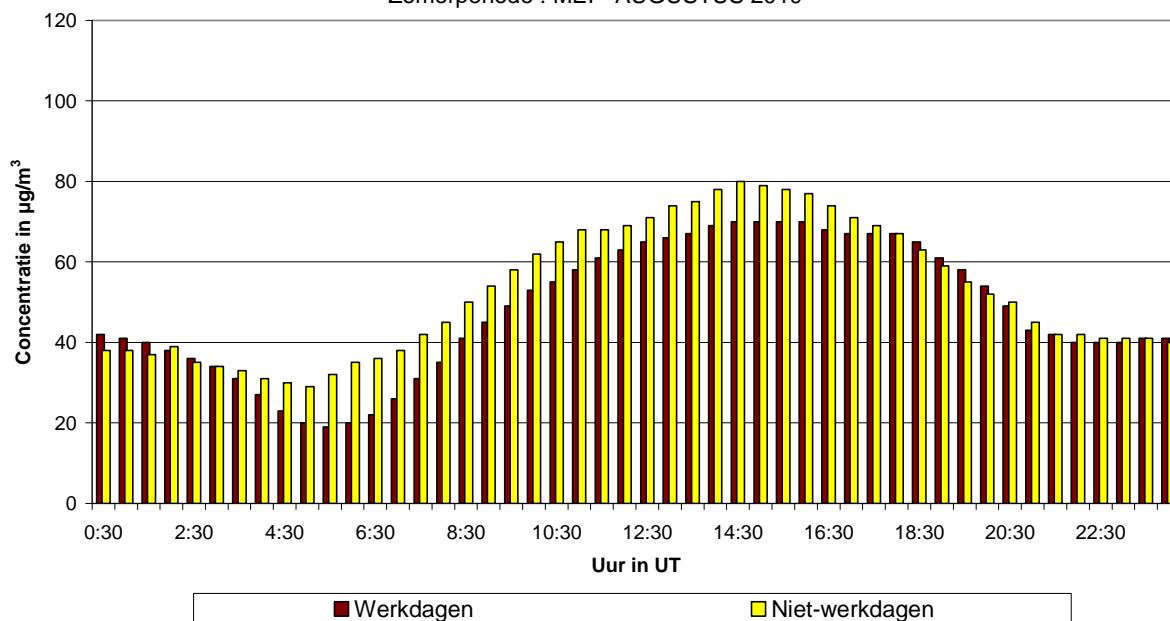
Fig. 48.a : Molenbeek : Gemiddeld dagverloop van de O 3 -concentratie op werkdagen en niet-werkdagen tijdens de periode mei - augustus 2010
