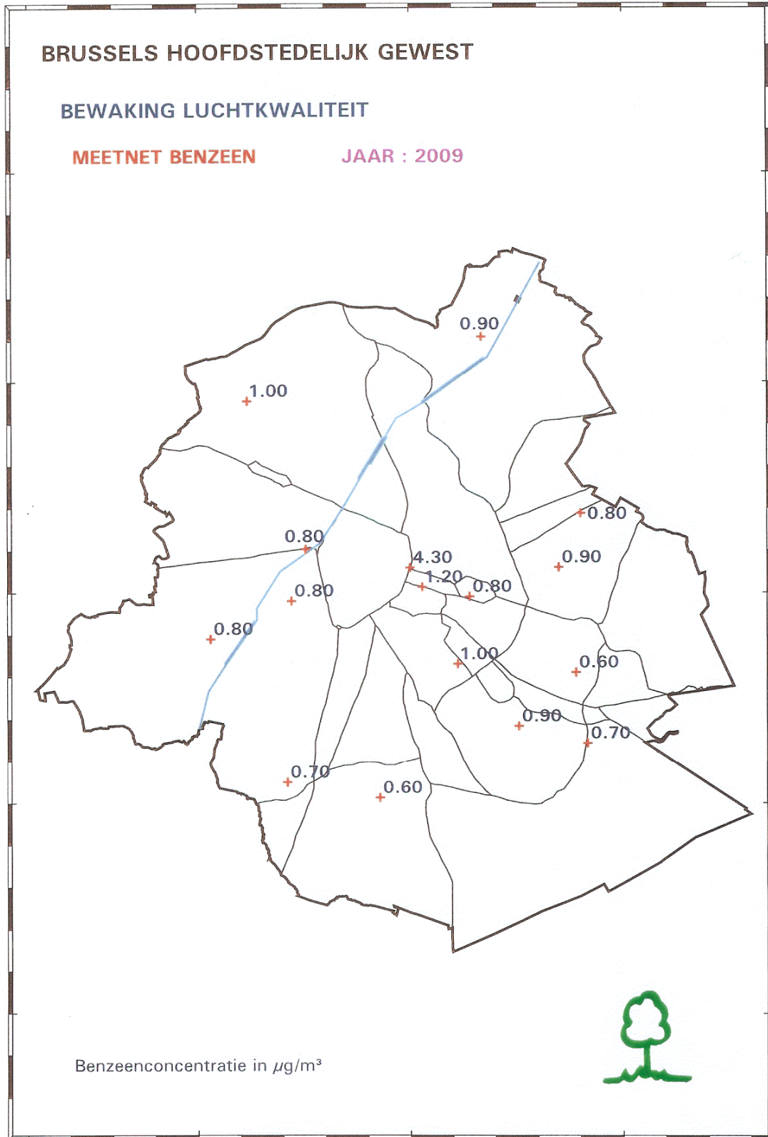
Fig. 31 : Benzeen – Ruimtelijke spreiding jaargemiddelde concentratie in 2009
