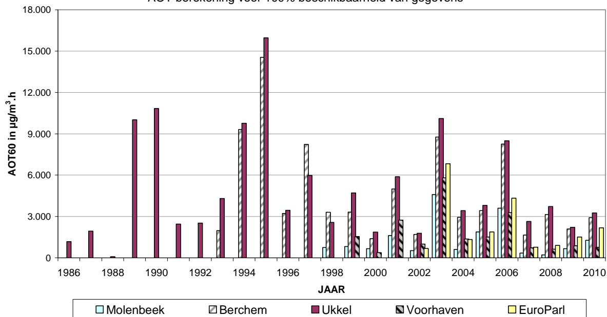
Fig. 24: Evolutie AOT60 in de tijd (1986-2010) Periode: JANUARI – DECEMBER (1986 – 2009) 2010 : Januari - September
