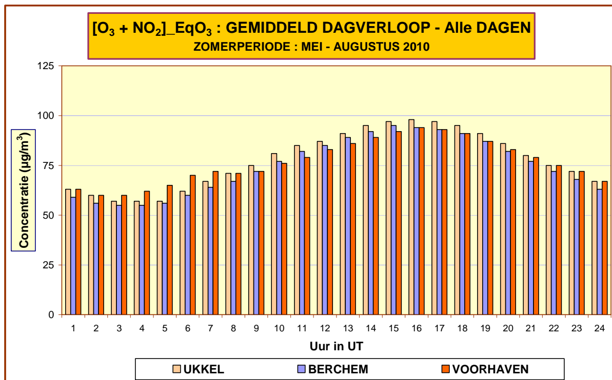
Fig. 67: [O 3 + NO 2 ] – Evolutie Dagverloop – Vergelijking tussen 3 meetposten Periode “mei –augustus 2010”
