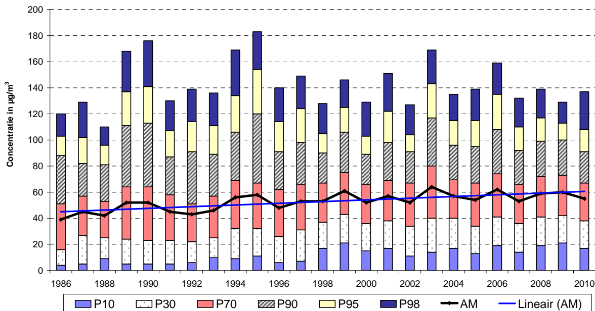
Fig. 70: Ozon te Ukkel – Uurgemiddelde concentratie – evolutie over langere termijn Zomerperiodes 1986 - 2010
