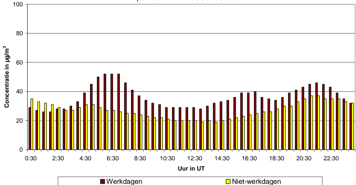
Fig. 50.b : St.-Lambr.-Woluwe : Gemiddeld dagverloop van de NO 2 -concentratie op werkdagen en niet-werkdagen tijdens de periode mei – augustus 2010
