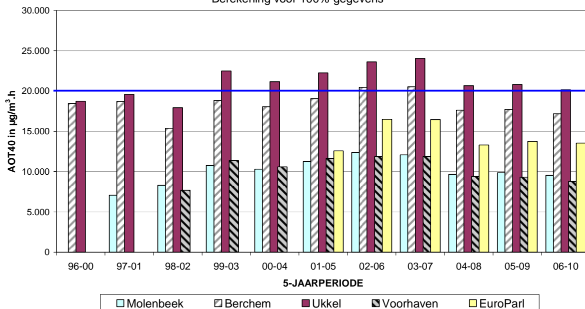
Fig. 16: Evolutie AOT40-AS in de tijd (1996-2010) AOT over de periode April – September, 8-20 h MET - Midden-Europese tijd Resultaten per jaar en gemiddeld over 5 jaar
