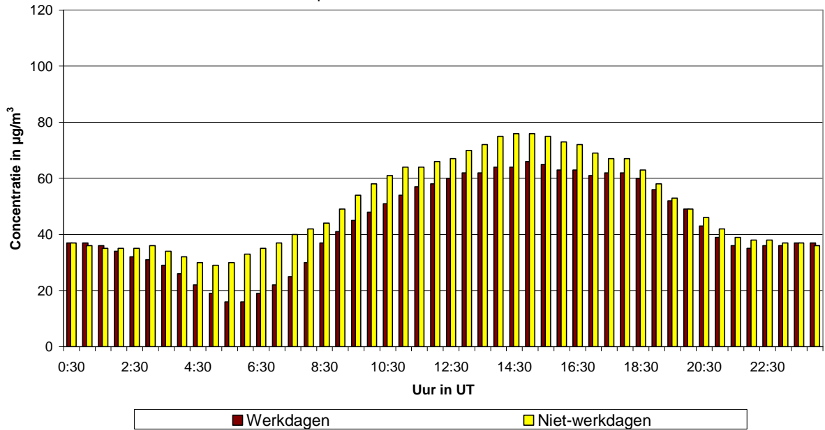
Fig. 50.a : St.-Lambr.-Woluwe : Gemiddeld dagverloop van de O 3 -concentratie op werkdagen en niet-werkdagen tijdens de periode mei - augustus 2010
