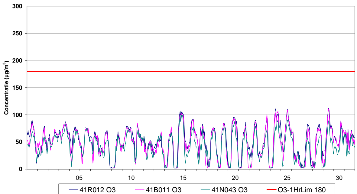
Fig. 3 : Evolutie van de uurwaarden voor ozon – Ukkel, Berchem en Voorhaven – Mei 2010
