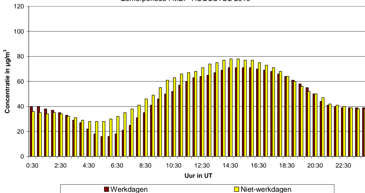
Fig. 52.a : St.-Katelijne : Gemiddeld dagverloop van de O 3 -concentratie op werkdagen en niet-werkdagen tijdens de periode mei - augustus 2010
