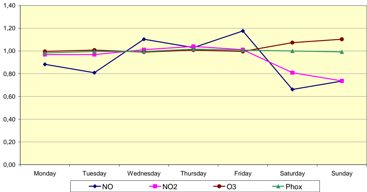
Fig. 59.a : Meetpost te Ukkel – Gemiddeld weekpatroon voor NO, NO 2 , O 3 en [NO 2 +O 3 ] over drie opeenvolgende zomerperiodes 'april – september' 2008, 2009 en 2010
