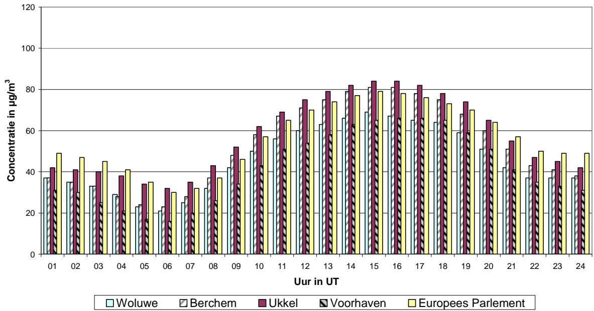
Fig. 8 : Gemiddeld dagverloop van de O 3 -concentratie in de periode mei – augustus 2010
