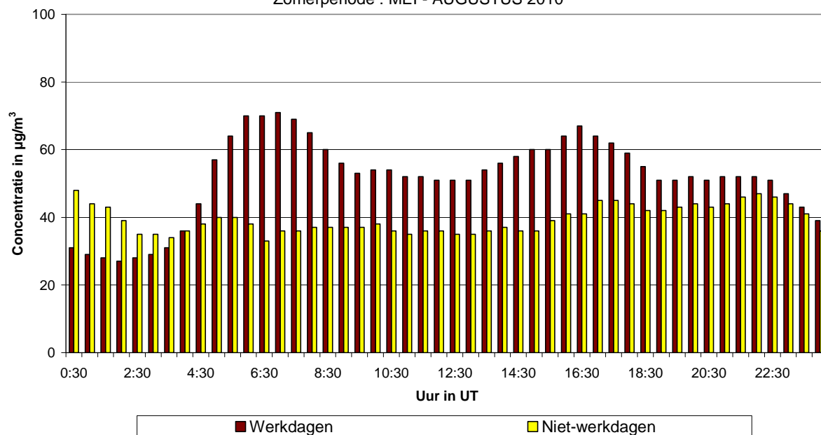
Fig. 54.a : Kroonlaan te Elsene : Gemiddeld dagverloop van de NO 2 -concentratie op werkdagen en niet-werkdagen tijdens de periode mei - augustus 2010
