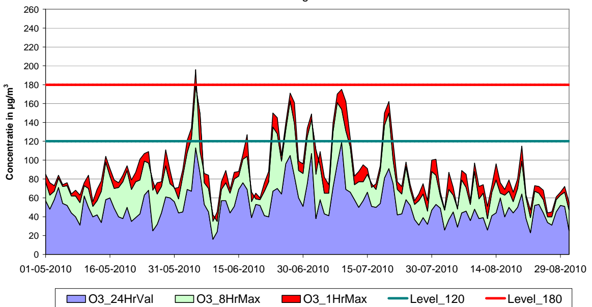
Fig. 22 : Ozon - Evolutie Dagwaarde (24HrVal), maximale 8-uurwaarde (8HrMax) en maximale uurwaarde (1HMax). Periode : mei - augustus 2010 Meetposten te Ukkel en St.-Agatha-Berchem
