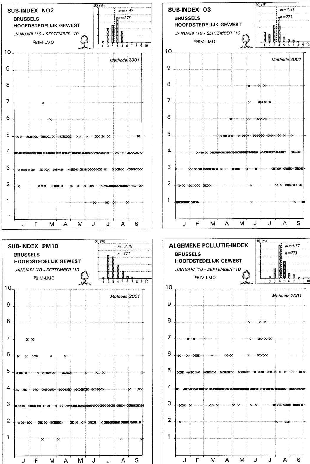
Fig. 60 : Subindexen voor NO 2 , O 3 en PM10 – Index Algemene Luchtkwaliteit Januari – September 2010
