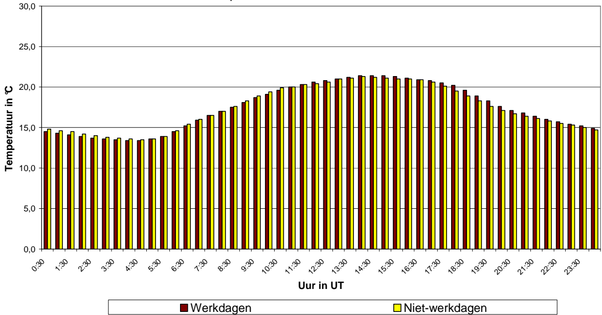
Fig. 55.a : Ukkel : Gemiddeld dagverloop van de temperatuur op werkdagen en niet-werkdagen tijdens de periode mei – augustus 2010
