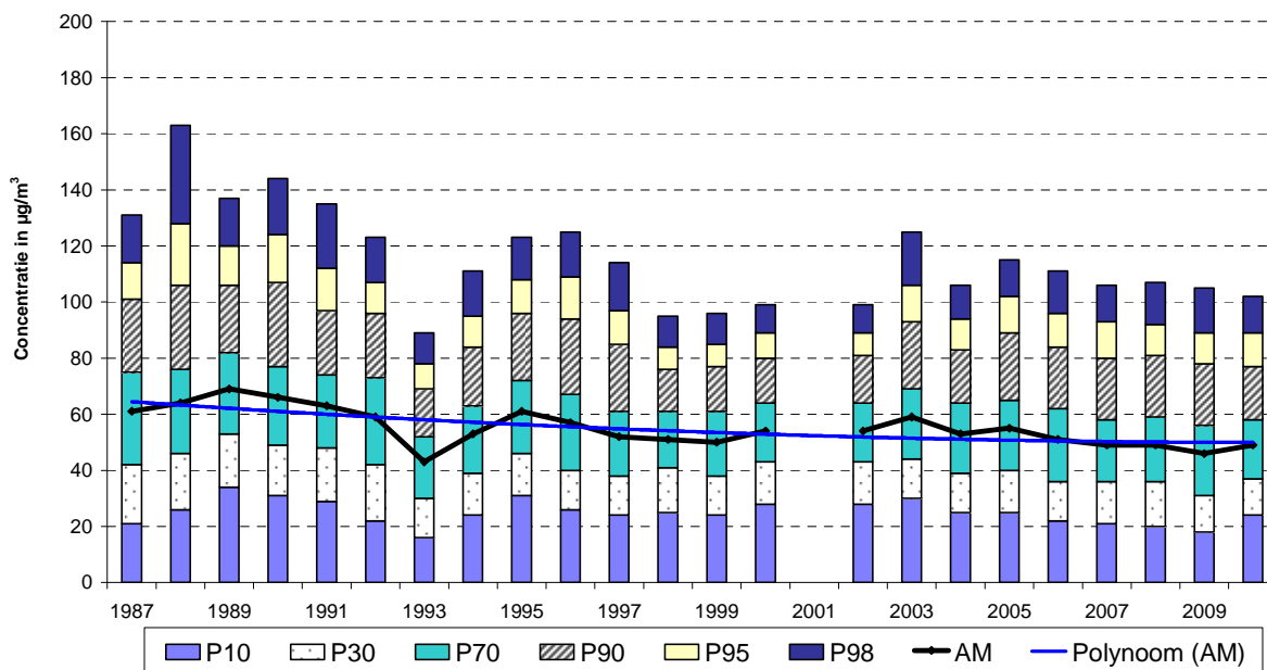
Fig. 40 : Elsene – Evolutie NO 2 -uurwaarden (1987-2010) Zomerperiode “april – september”
