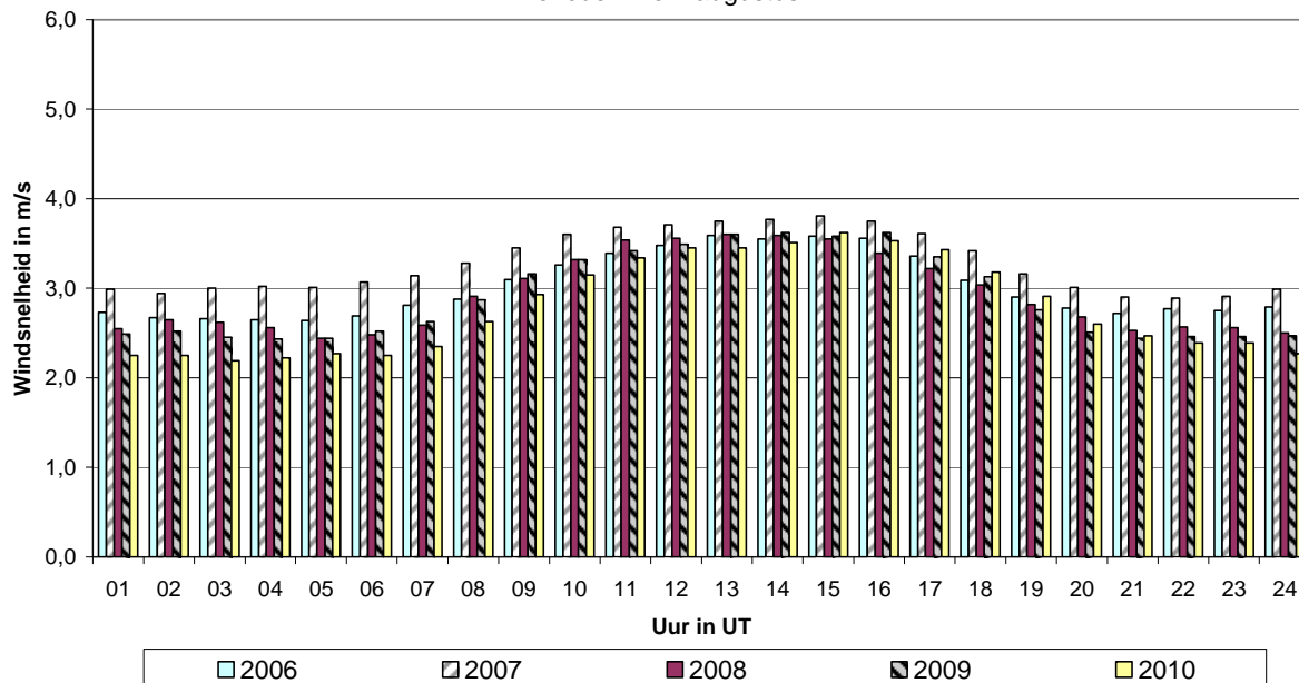
Fig. 38 : Gemiddeld dagverloop windsnelheid te Ukkel (M003) Zomerperiodes mei-augustus 2006, 2007, 2008, 2009 en 2010
