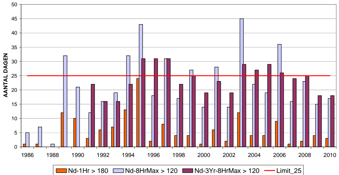
Fig. 21 : Ozon : aantal dagen met overschrijdingen in het Gewest
