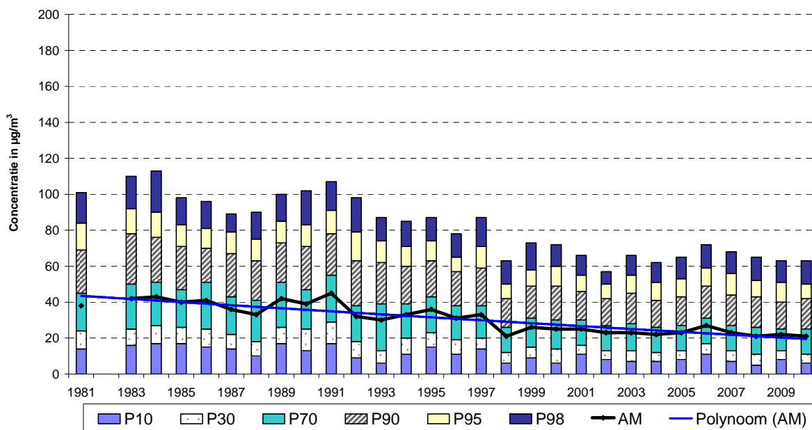
Fig. 41 : Ukkel – Evolutie NO 2 -uurwaarden (1981-2010) Zomerperiode “april – september”
