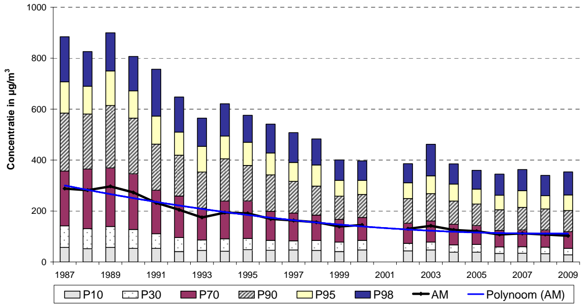
Fig. 72: NO x – Kroonlaan te Elsene ( canyon street ) - Uurgemiddelde concentratie Evolutie over langere termijn - Jaarperiodes 1987 – 2009
