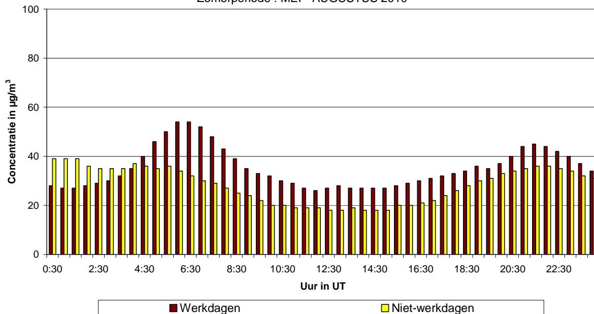
Fig. 52.b : St.-Katelijne : Gemiddeld dagverloop van de NO 2 -concentratie op werkdagen en niet-werkdagen tijdens de periode mei – augustus 2010
