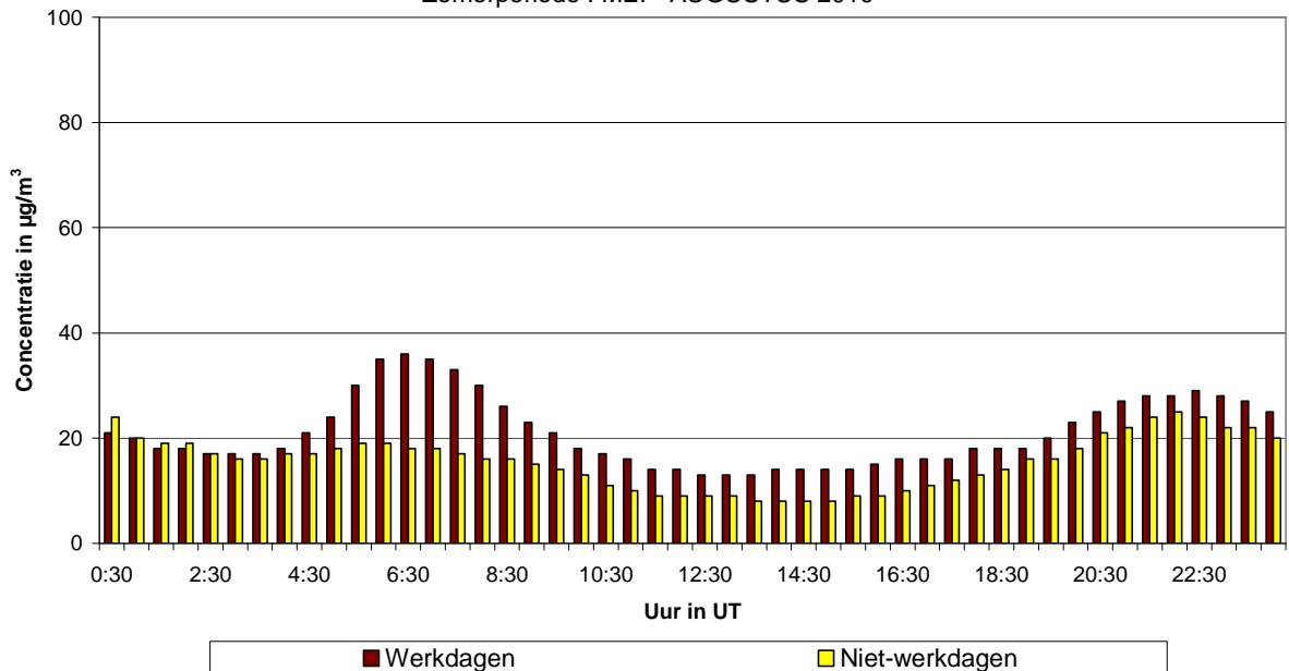
Fig. 46.b : Ukkel : Gemiddeld dagverloop van de NO 2 -concentratie op werkdagen en niet-werkdagen tijdens de periode mei – augustus 2010
