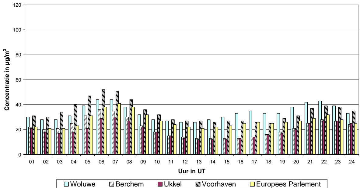
Fig. 9 : Gemiddeld dagverloop van de NO 2 -concentratie in de periode mei – augustus 2010
