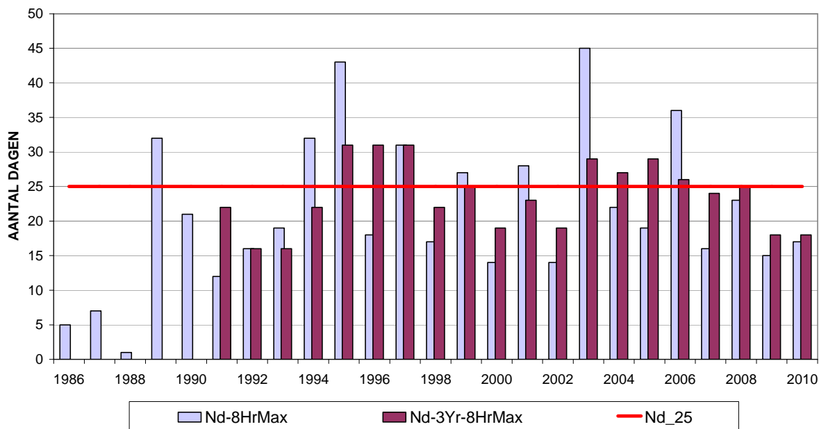
Fig. 14 : Ozon - Evolutie aantal overschrijdingsdagen in het Brussels Hoofdstedelijk Gewest Streefwaarde voor de gezondheid: Maximale 8-uurwaarde > 120 µg/m 3 Periode : Januari – December (1986-2009). [2010]: Januari – September
