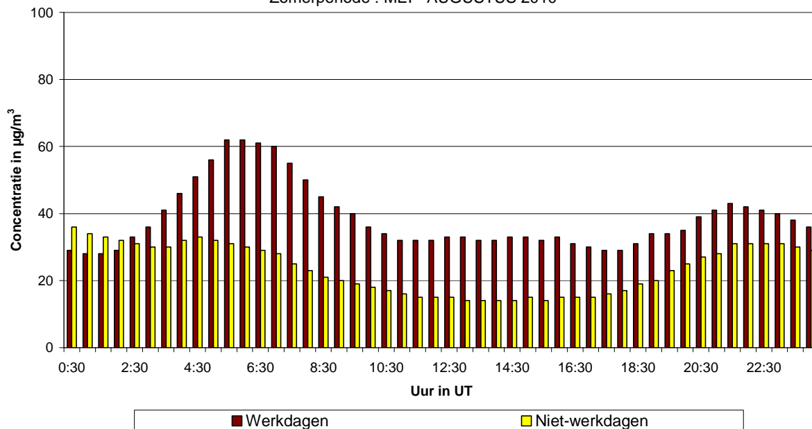
Fig. 49.b : Voorhaven : Gemiddeld dagverloop van de NO 2 -concentratie op werkdagen en niet-werkdagen tijdens de periode mei – augustus 2010
