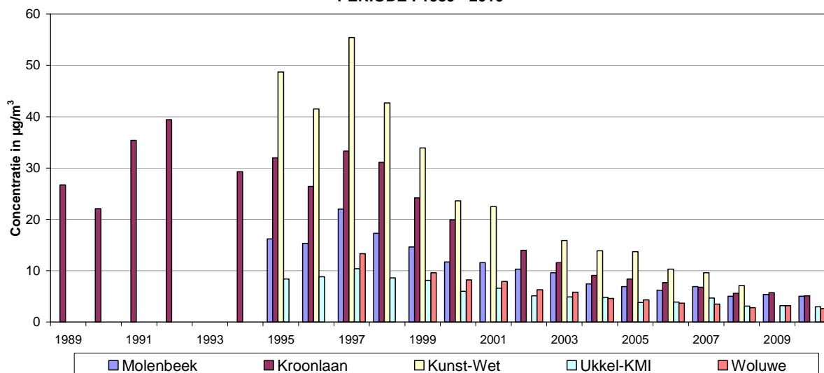
Fig. 29 : Toluene - Evolutie jaargemiddelde concentratie Periode : Januari – December (1989-2009) en 'Januari – September 2010'
