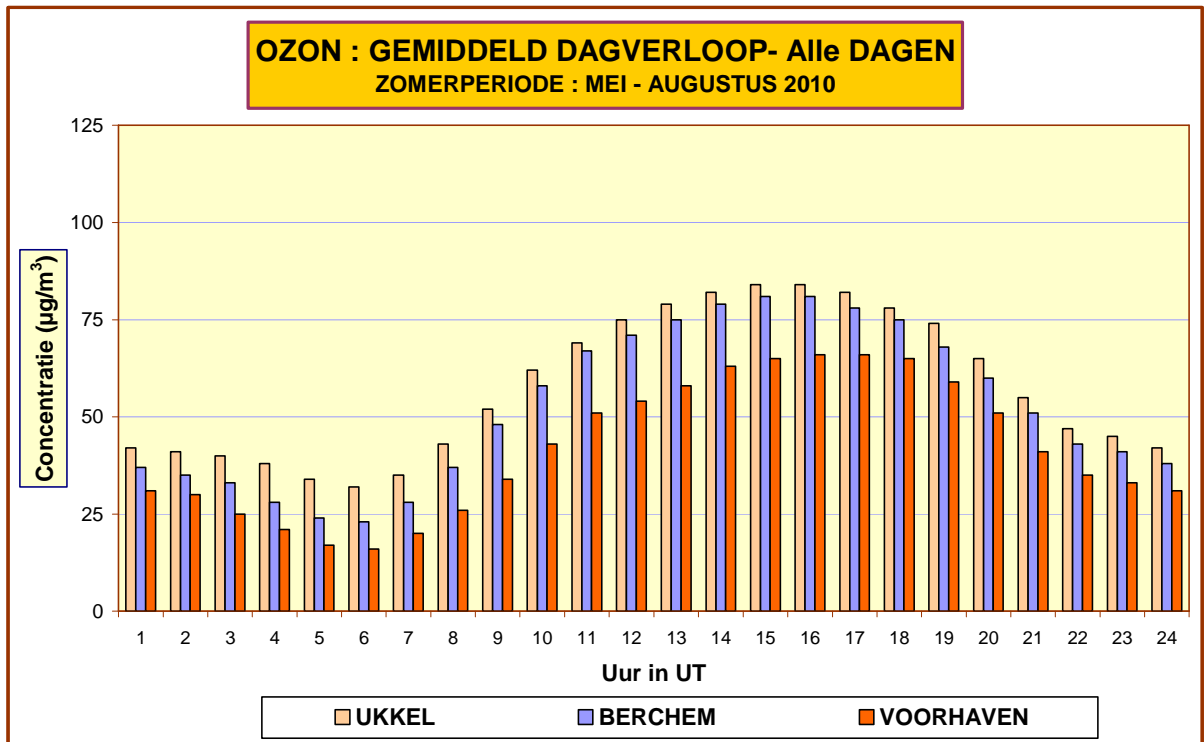
Fig. 65: Ozon – Evolutie Dagverloop – Vergelijking tussen 3 meetposten Periode “mei –augustus 2010”
