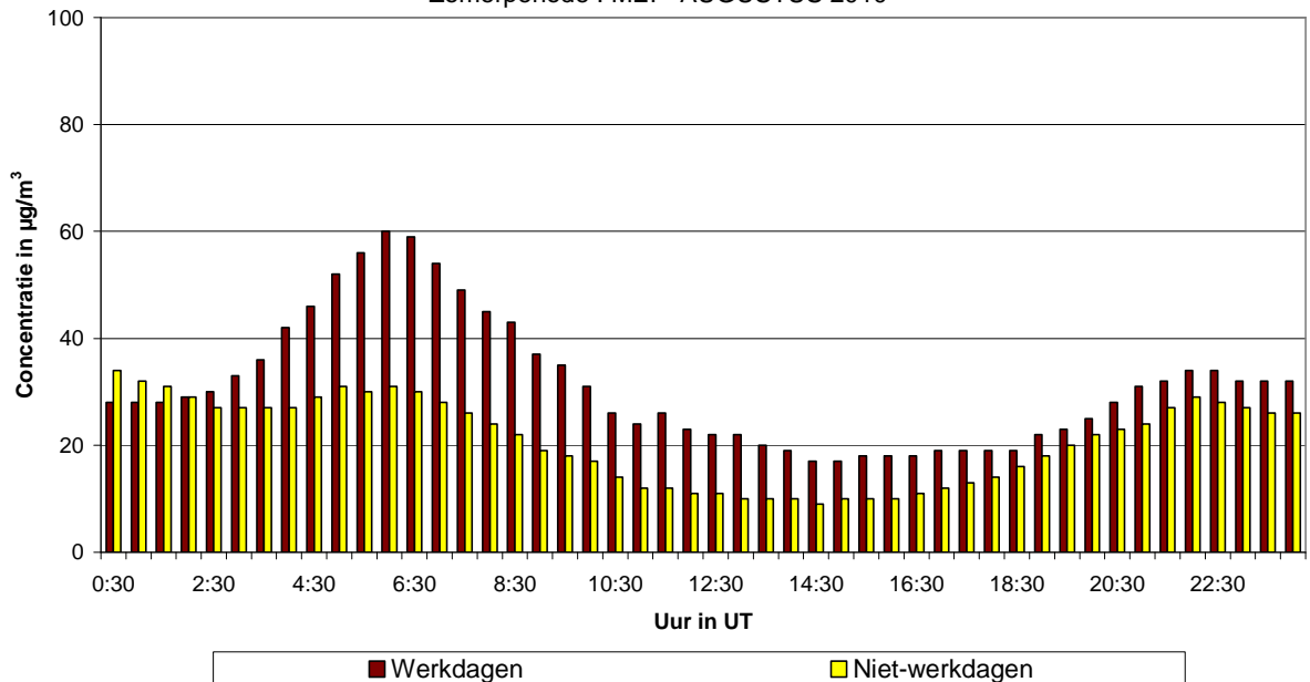
Fig. 53.b : Meudonpark : Gemiddeld dagverloop van de NO 2 -concentratie op werkdagen en niet-werkdagen tijdens de periode mei – augustus 2010
