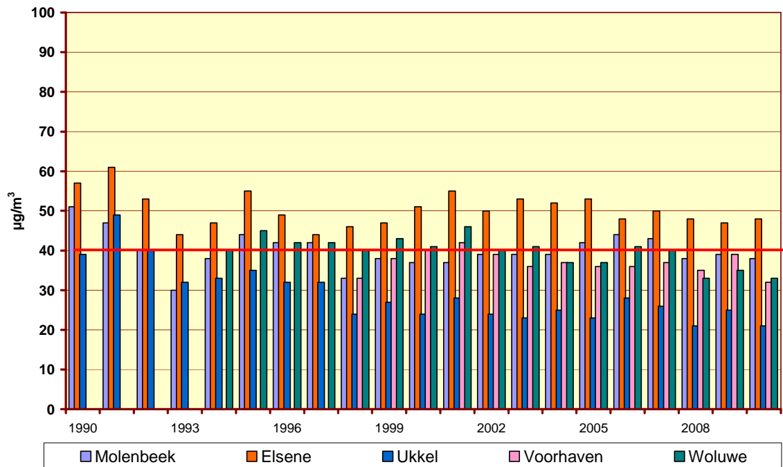
Fig. 27.c : NO 2 - Evolutie gemiddelde concentratie op 'Zaterdag' Jaarperiodes 1990-2009 en "Januari - September 2010"
