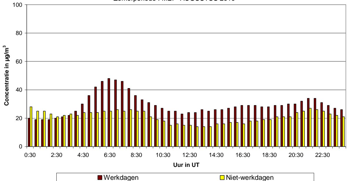
Fig. 51.b : Europees Parlement : Gemiddeld dagverloop van de NO 2 -concentratie op werkdagen en niet-werkdagen tijdens de periode mei – augustus 2010
