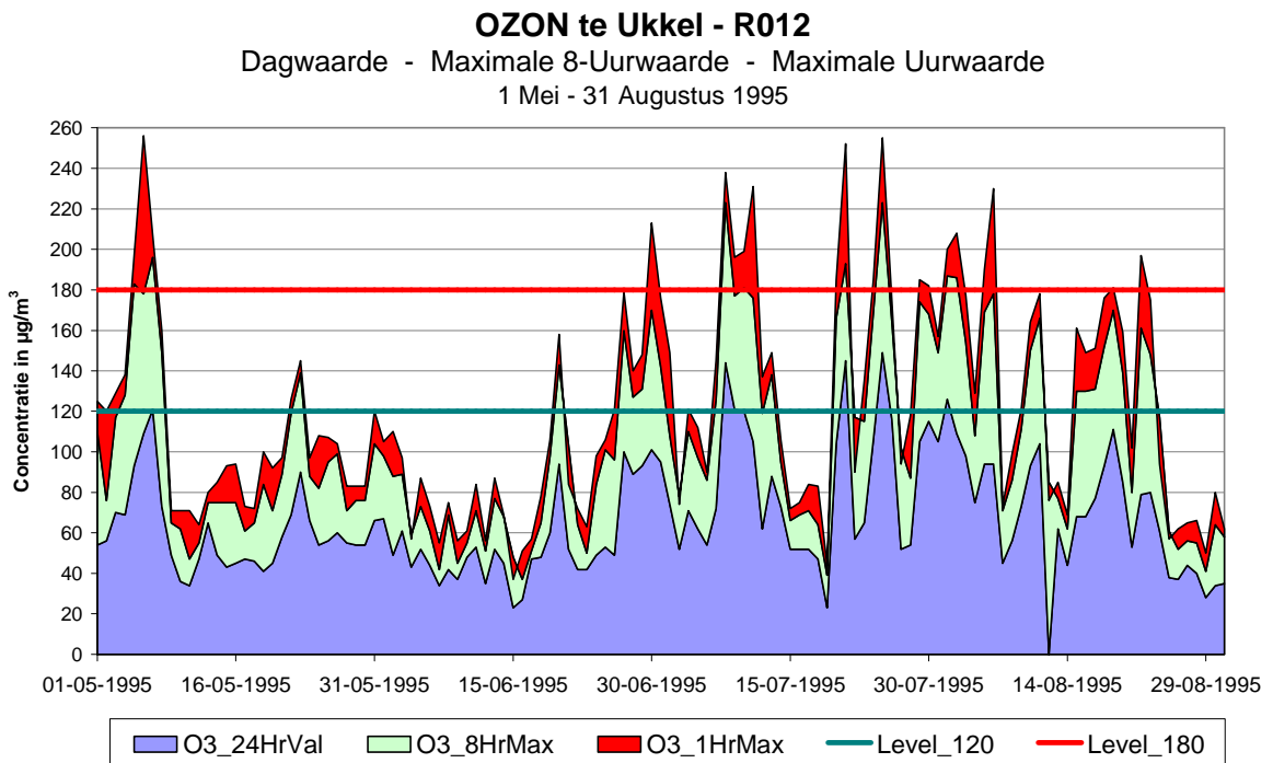
Fig. 23 : Ozon te Ukkel - Evolutie Dagwaarde (24HrMax), maximale 8-uurwaarde (8HrMax) en maximale uurwaarde (1HrMax). Vergelijking zomerperiode 2003 en 1995
