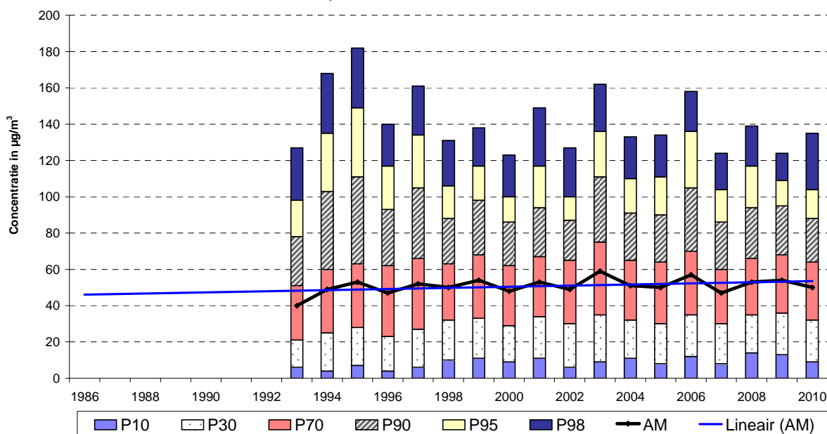
Fig. 34 : Evolutie O 3 -uurwaarden te St.-Ag.-Berchem (1993-2010) Zomerperiode "april – september"
