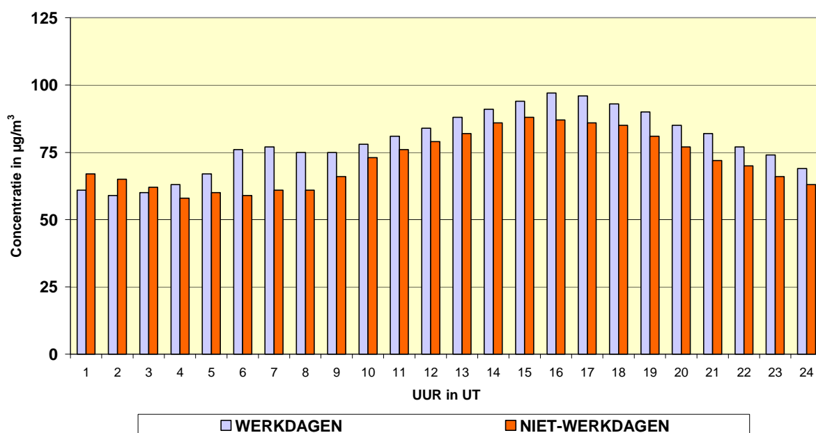
Fig. 69: [O 3 + NO 2 ] – Evolutie Dagverloop voor werkdagen en niet-werkdagen Meetposten Ukkel en Voorhaven - Periode “mei – augustus 2010”
