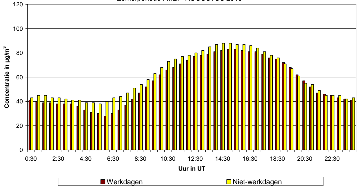
Fig. 46.a : Ukkel : Gemiddeld dagverloop van de O 3 -concentratie op werkdagen en niet-werkdagen tijdens de periode mei - augustus 2010
