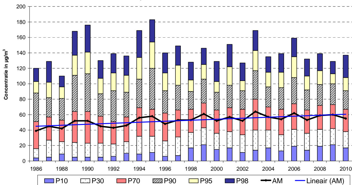
Fig. 33 : Evolutie O 3 -uurwaarden te Ukkel (1986-2010) Zomerperiode "april – september"
