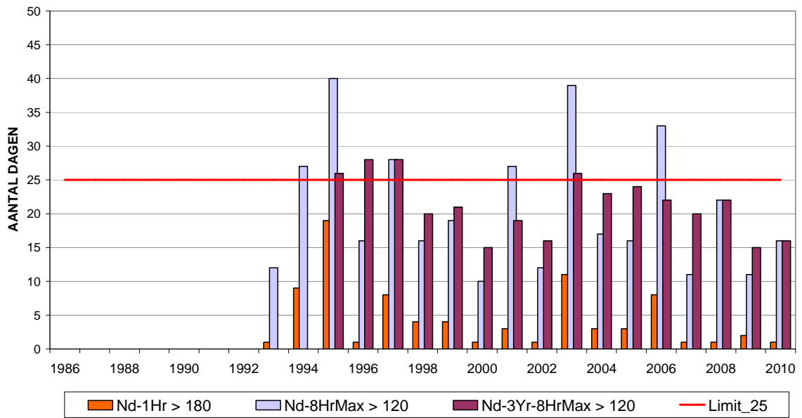
Fig. 20 : Ozon te St.-Ag.-Berchem : aantal dagen met overschrijdingen
