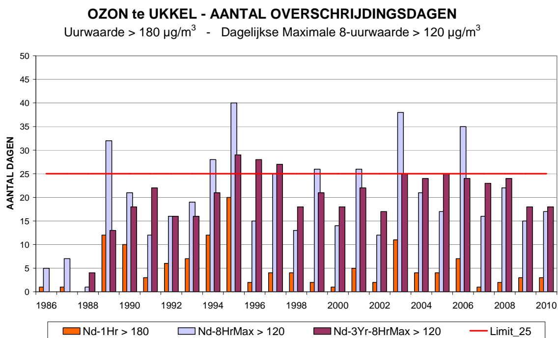
Fig. 19 : Ozon te Ukkel : aantal dagen met overschrijdingen Jaarperiodes: 1 januari – 31 december (1986-2009) Voorlopige resultaten voor het jaar 2010 (1 januari – 30 september)
