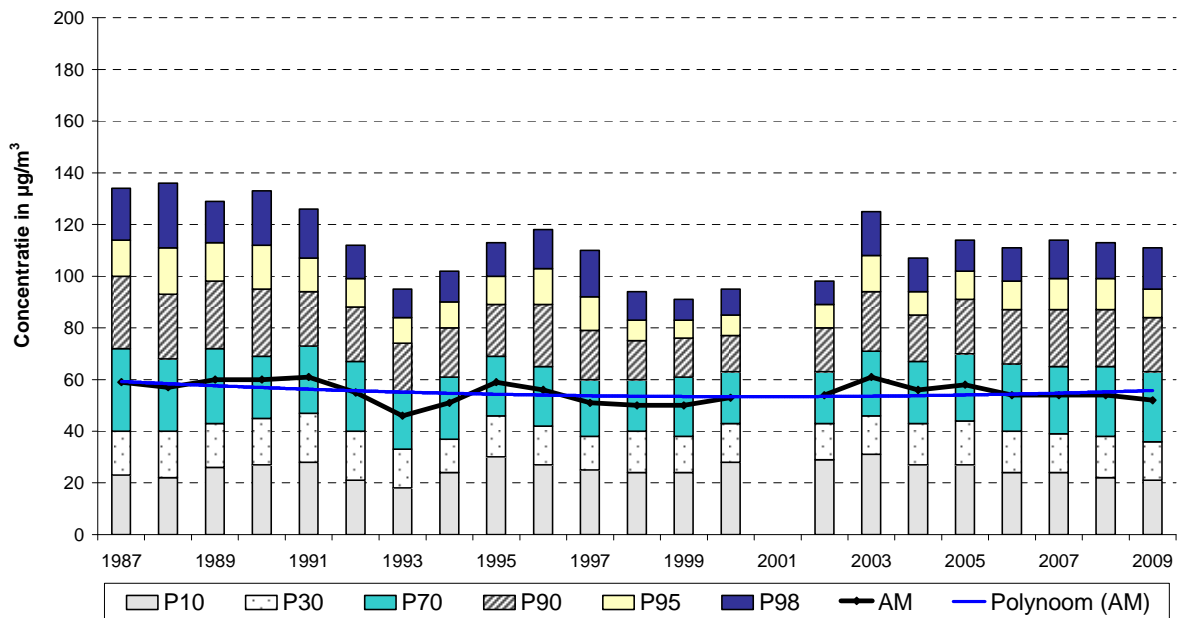
Fig. 73: NO 2 – Kroonlaan te Elsene ( canyon street ) - Uurgemiddelde concentratie Evolutie over langere termijn - Jaarperiodes 1987 – 2009
