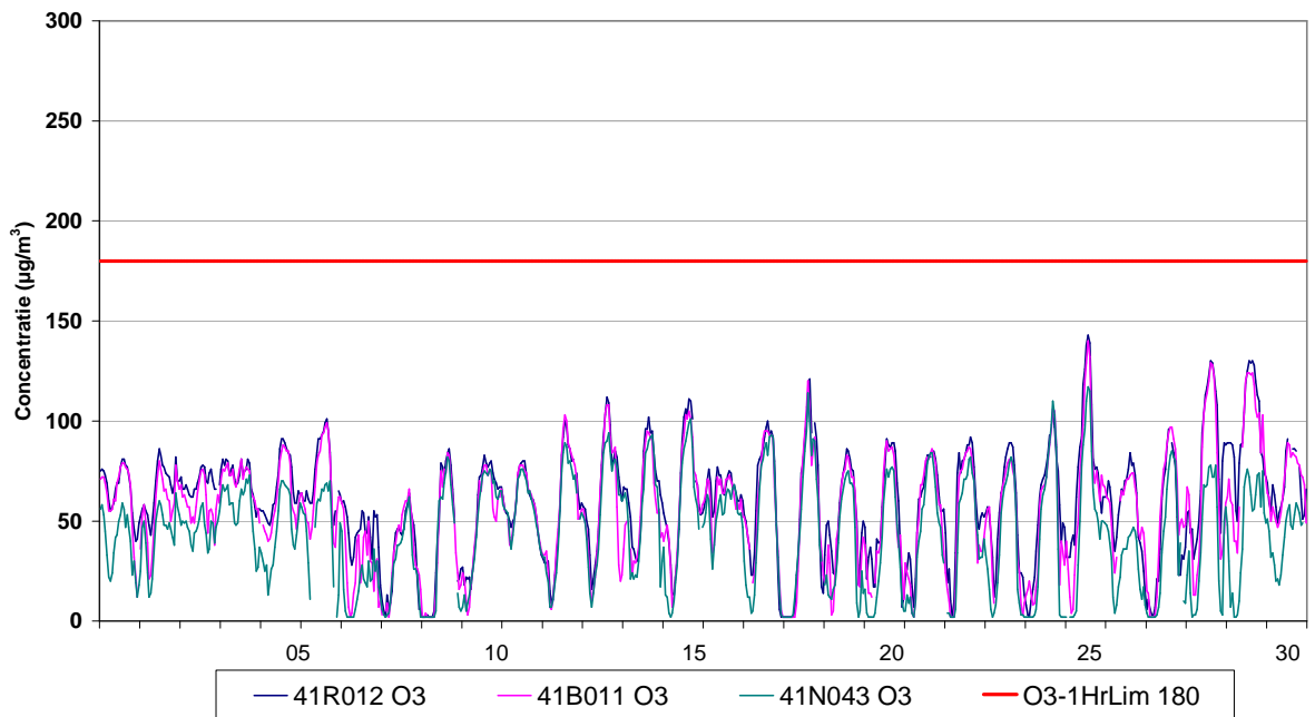
Fig. 2 : Evolutie van de uurwaarden voor ozon – Ukkel, Berchem en Voorhaven – April 2010
