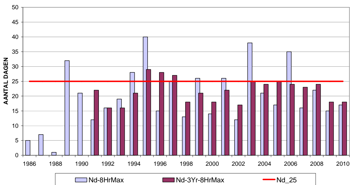
Fig. 12 : Ozon - Evolutie aantal overschrijdingsdagen in de meetpost te Ukkel Streefwaarde voor de gezondheid: Maximale 8-uurwaarde > 120 µg/m 3 Periode : Januari – December (1986-2009). [2010]: Januari – September
