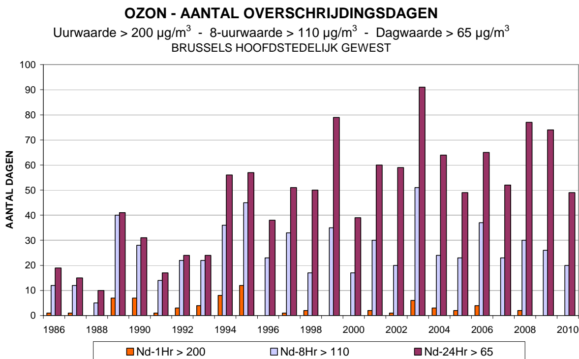
Fig. 25 : Ozon : aantal dagen met overschrijdingen (richtlijn 92/72/EG) Periode : januari - december (1986 t/m 2009) 2010 : Januari - September
