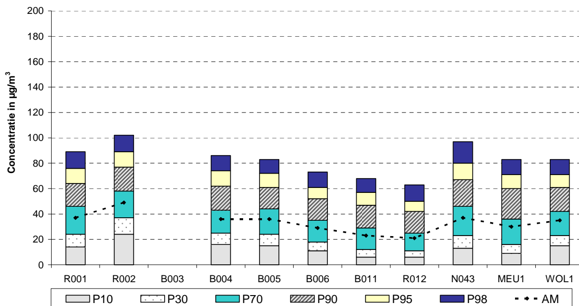
Fig. 39 : NO 2 - Cumulatieve frequentieverdeling uurwaarden: april - september 2010
