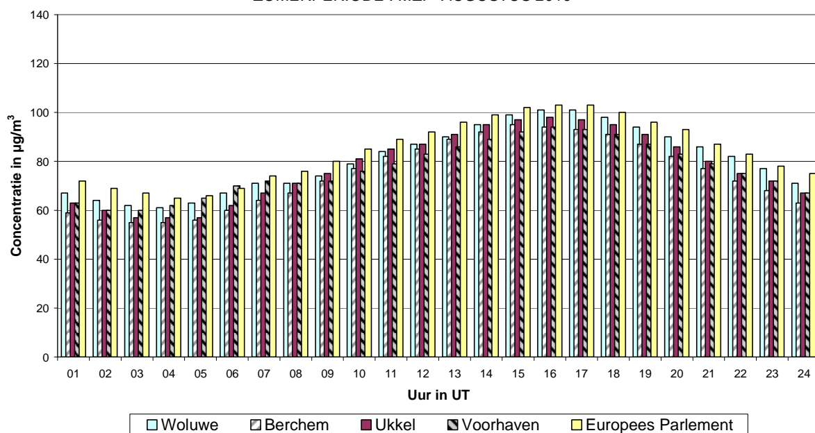
Fig. 10 : Gemiddeld dagverloop voor de som van de gasvormige oxidantia [O 3 + NO 2 ], uitgedrukt als equivalent massaconcentratie ozon, tijdens de periode mei – augustus 2010
