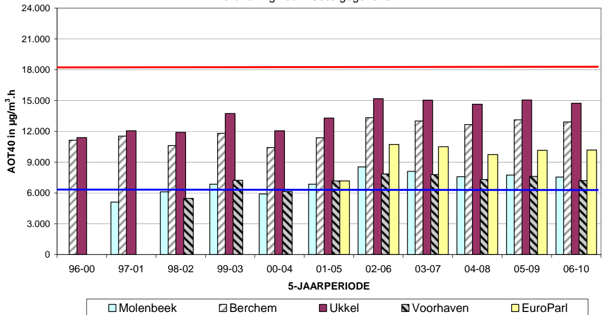
Fig. 15: Evolutie AOT40-MJ in de tijd (1996-2010)
