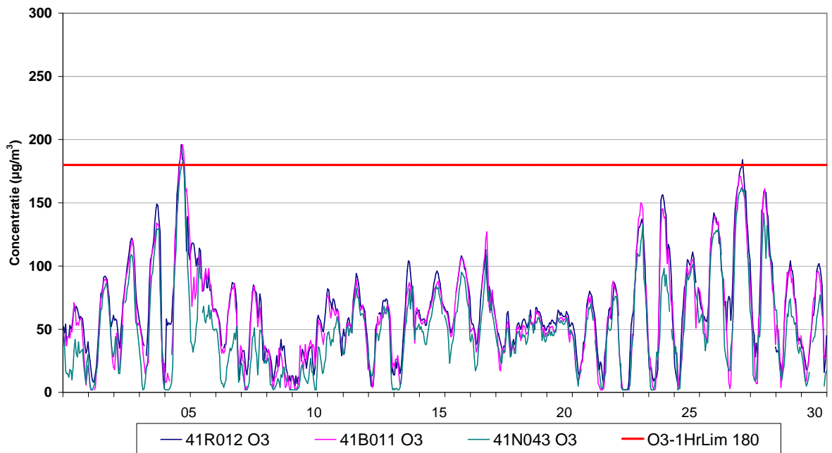
Fig. 4 : Evolutie van de uurwaarden voor ozon – Ukkel, Berchem en Voorhaven – Juni 2010
