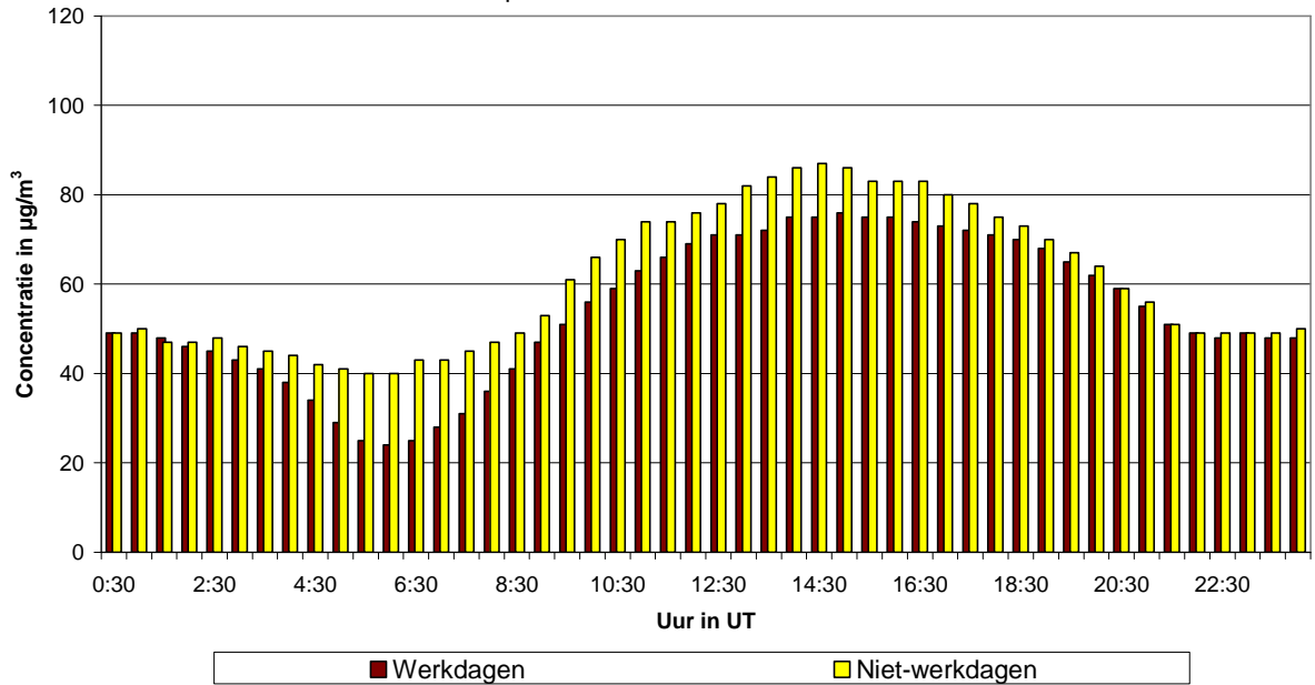
Fig. 51.a : Europees Parlement : Gemiddeld dagverloop van de O 3 -concentratie op werkdagen en niet-werkdagen tijdens de periode mei - augustus 2010
