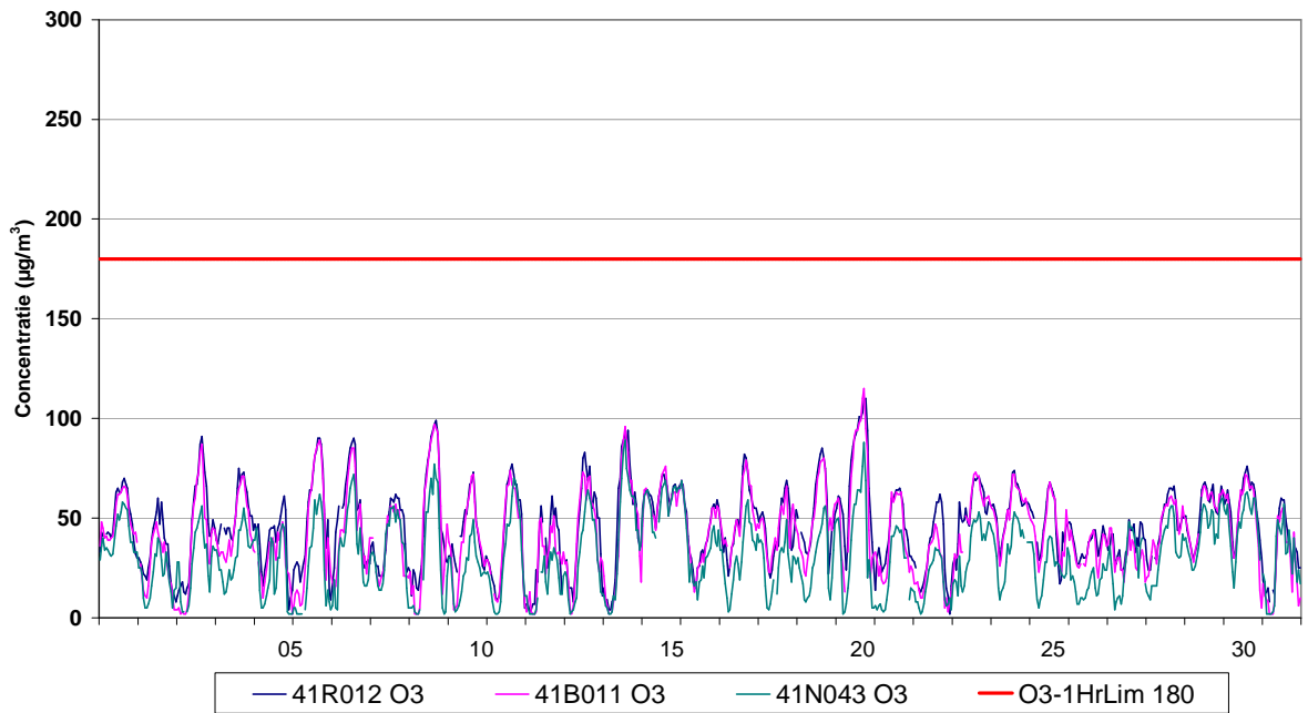
Fig. 6 : Evolutie van de uurwaarden voor ozon – Ukkel, Berchem en Voorhaven – Augustus 2010
