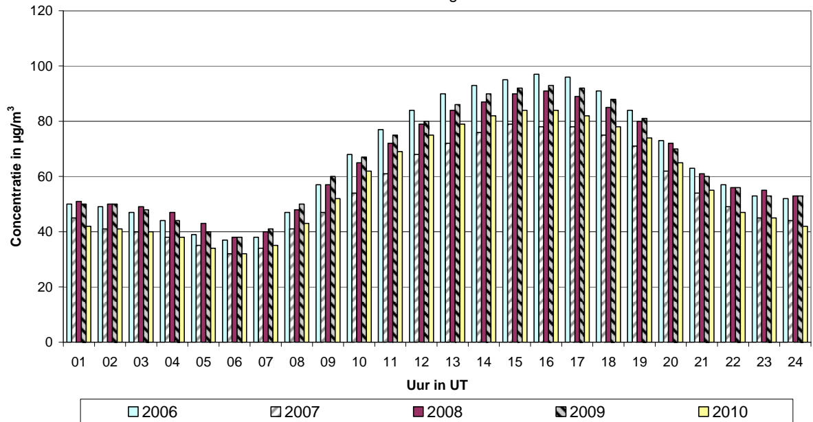
Fig. 35 : Gemiddeld dagverloop O 3 -concentratie te Ukkel (R012) Evolutie tijdens recente zomerperiodes (2006-2010)
