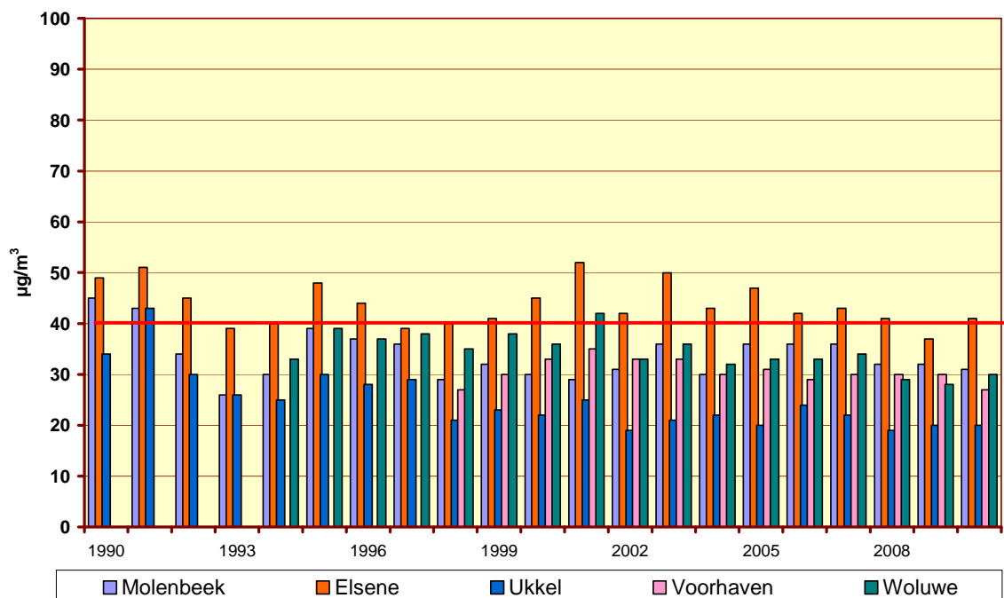
Fig. 27.d : NO 2 - Evolutie gemiddelde concentratie op 'Zondagen' Jaarperiodes 1990-2009 en "Januari - September 2010"
