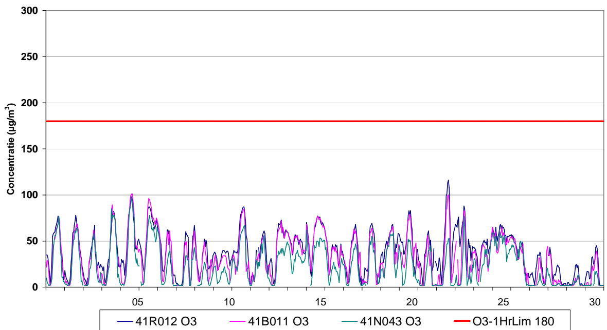
Fig. 7 : Evolutie van de uurwaarden voor ozon – Ukkel, Berchem en Voorhaven – September 2010
