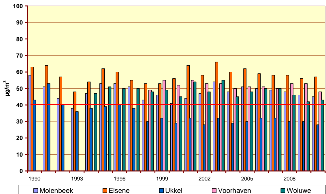
Fig. 27.b : NO 2 - Evolutie gemiddelde concentratie op 'werkdagen' Jaarperiodes 1990-2009 en "Januari – September 2010"
