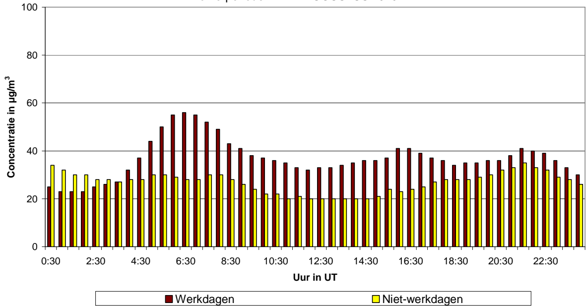
Fig. 53.a : Eastman-Belliard : Gemiddeld dagverloop van de NO 2 -concentratie op werkdagen en niet-werkdagen tijdens de periode mei - augustus 2010
