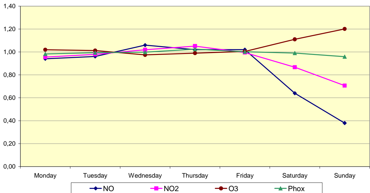
Fig. 59.b : Meetpost te Molenbeek – Gemiddeld weekpatroon voor NO, NO 2 , O 3 en [NO 2 +O 3 ] over drie opeenvolgende zomerperiodes 'april – september' 2008, 2009 en 2010
