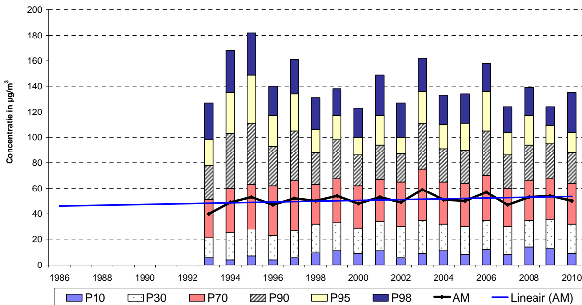
Fig. 71: Ozon te St.-Ag.-Berchem – Uurgemiddelde concentratie – evolutie over langere termijn Zomerperiodes 1993 - 2010
