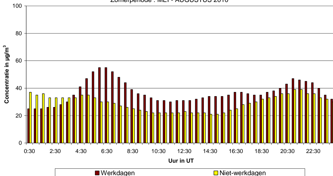
Fig. 48.b : Molenbeek : Gemiddeld dagverloop van de NO 2 -concentratie op werkdagen en niet-werkdagen tijdens de periode mei - augustus 2010
