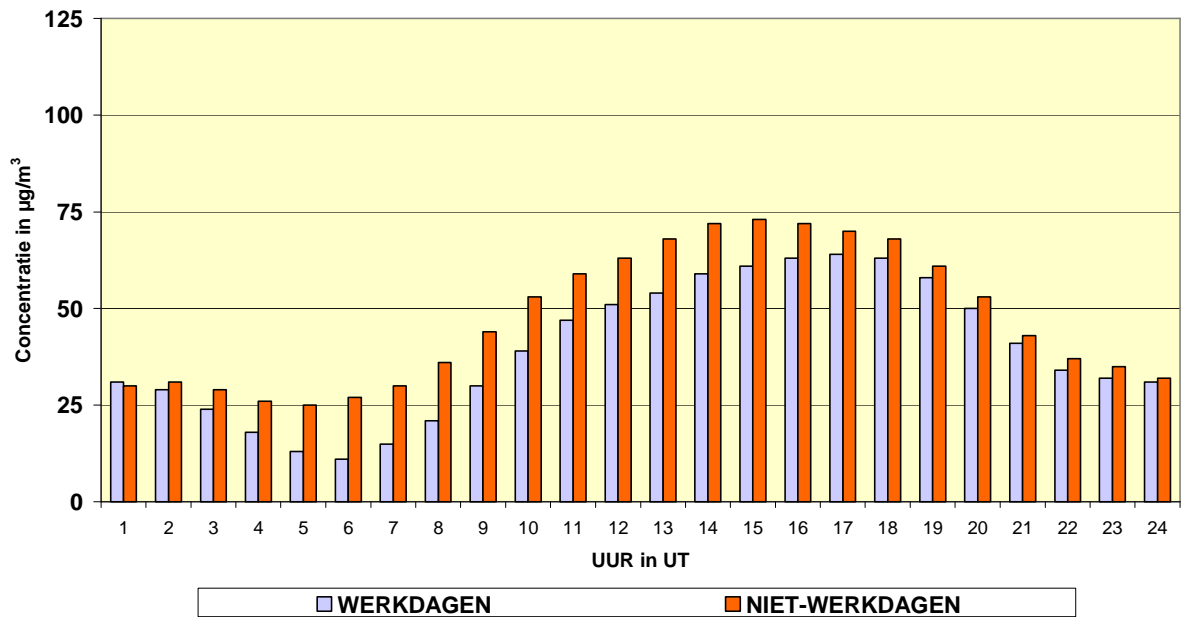
Fig. 68: Ozon – Evolutie Dagverloop voor werkdagen en niet-werkdagen Meetposten Ukkel en Voorhaven - Periode “mei – augustus 2010”
