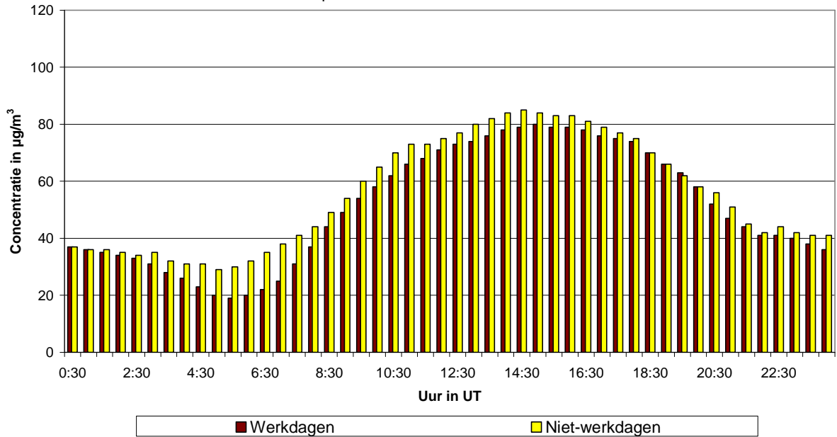
Fig. 47.a : St.-Agatha-Berchem : Gemiddeld dagverloop van de O 3 -concentratie op werkdagen en niet-werkdagen tijdens de periode mei - augustus 2010
