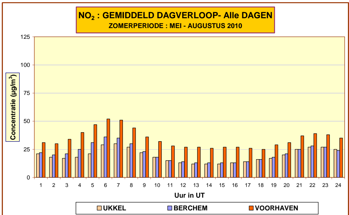
Fig. 66: NO 2 – Evolutie Dagverloop – Vergelijking tussen 3 meetposten Periode “mei –augustus 2010”
