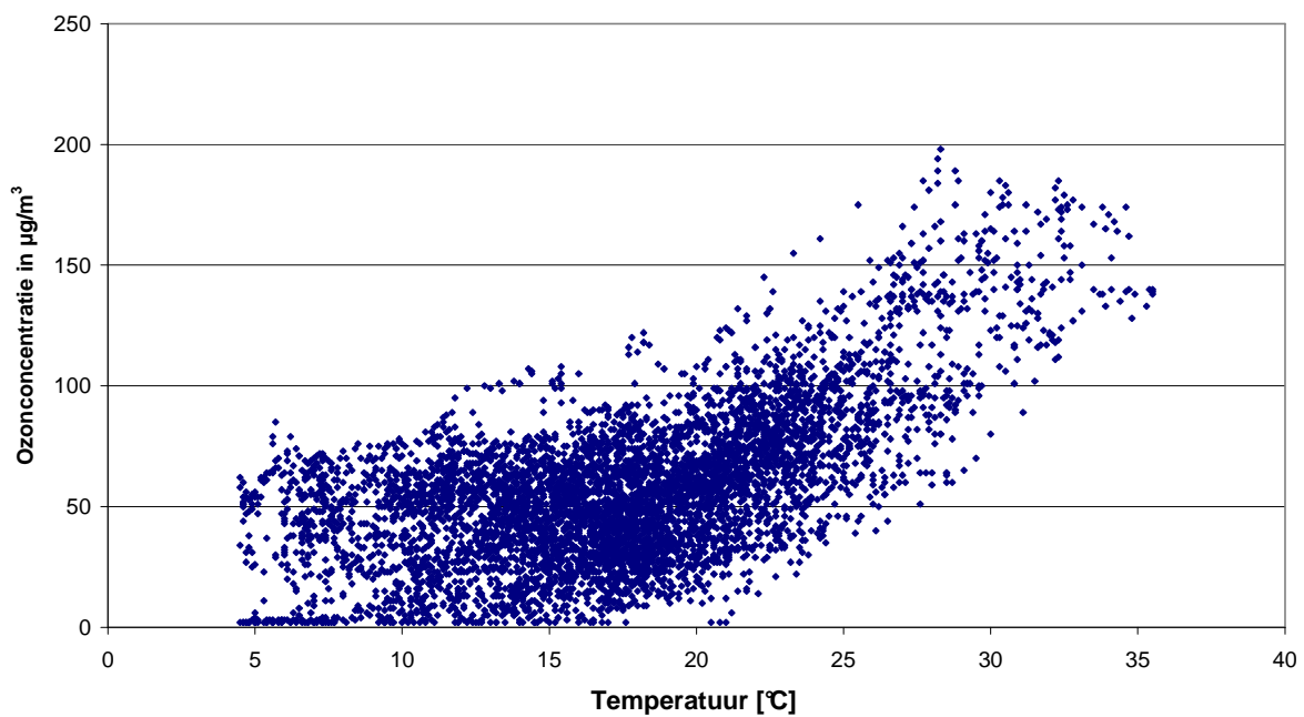
Fig. 42 : Ukkel : Ozonconcentraties versus temperatuur (mei - augustus 2010)
