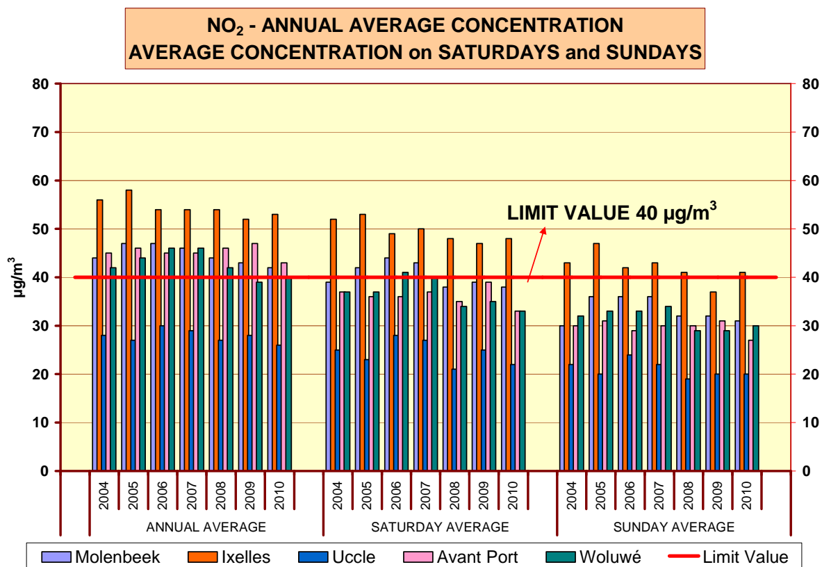
Fig. 26 : NO 2 – Vergelijking jaargemiddelde concentratie met de gemiddelde concentratie op 'Zaterdag' en 'Zondag' voor een selectie van meetposten. Jaarperiodes 2004-2009 en "Januari – September 2010"
