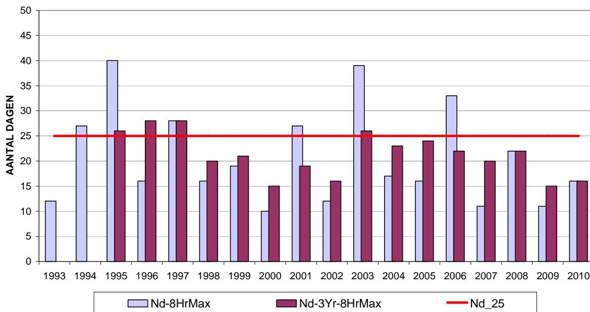
Fig. 13 : Ozon - Evolutie aantal overschrijdingsdagen in de meetpost te Berchem Streefwaarde voor de gezondheid: Maximale 8-uurwaarde > 120 µg/m 3 Periode : Januari – December (1993-2009). [2010]: Januari – September
