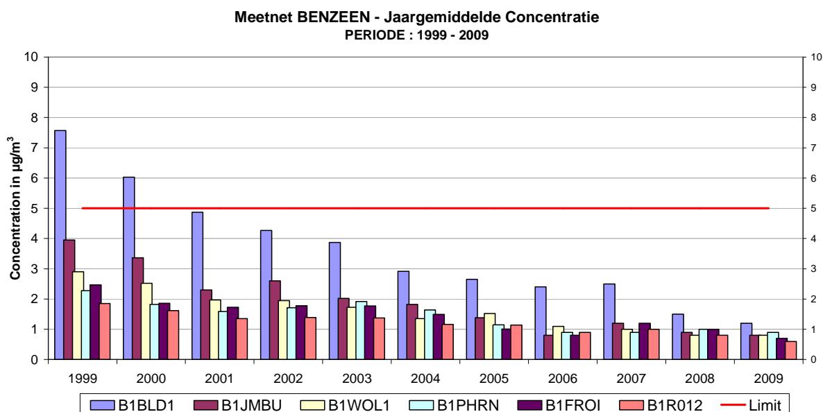
Fig. 30 : Benzeen – Evolutie jaargemiddelde concentratie in een aantal meetpunten van het benzeenmeetnet – Periode : 1999 - 2009
