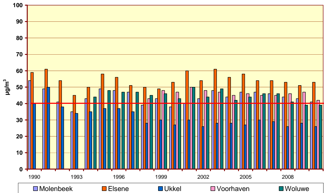
Fig. 27.a : NO 2 - Evolutie jaargemiddelde concentratie Jaarperiodes 1990-2009 en "Januari – September 2010"
