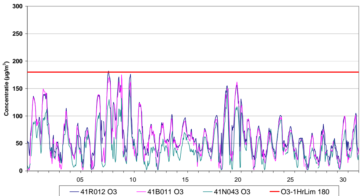
Fig. 5 : Evolutie van de uurwaarden voor ozon – Ukkel, Berchem en Voorhaven – Juli 2010
