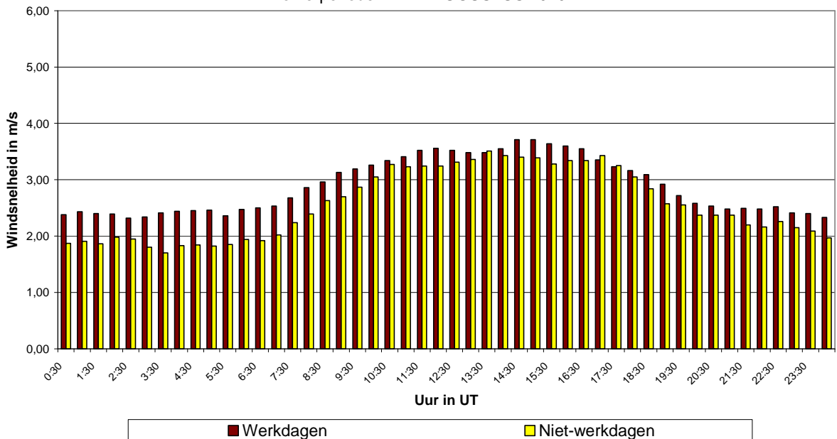
Fig. 55.b : Ukkel : Gemiddeld dagverloop van de windsnelheid op werkdagen en niet-werkdagen tijdens de periode mei – augustus 2010
