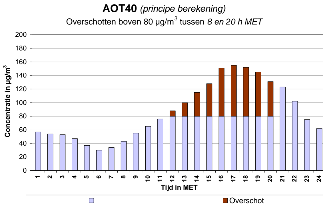
Fig. 7 : AOT40 : Voorstelling overschotten boven 80 \mu\text{g}/\text{m}^3 tussen 8 en 20 h MET
