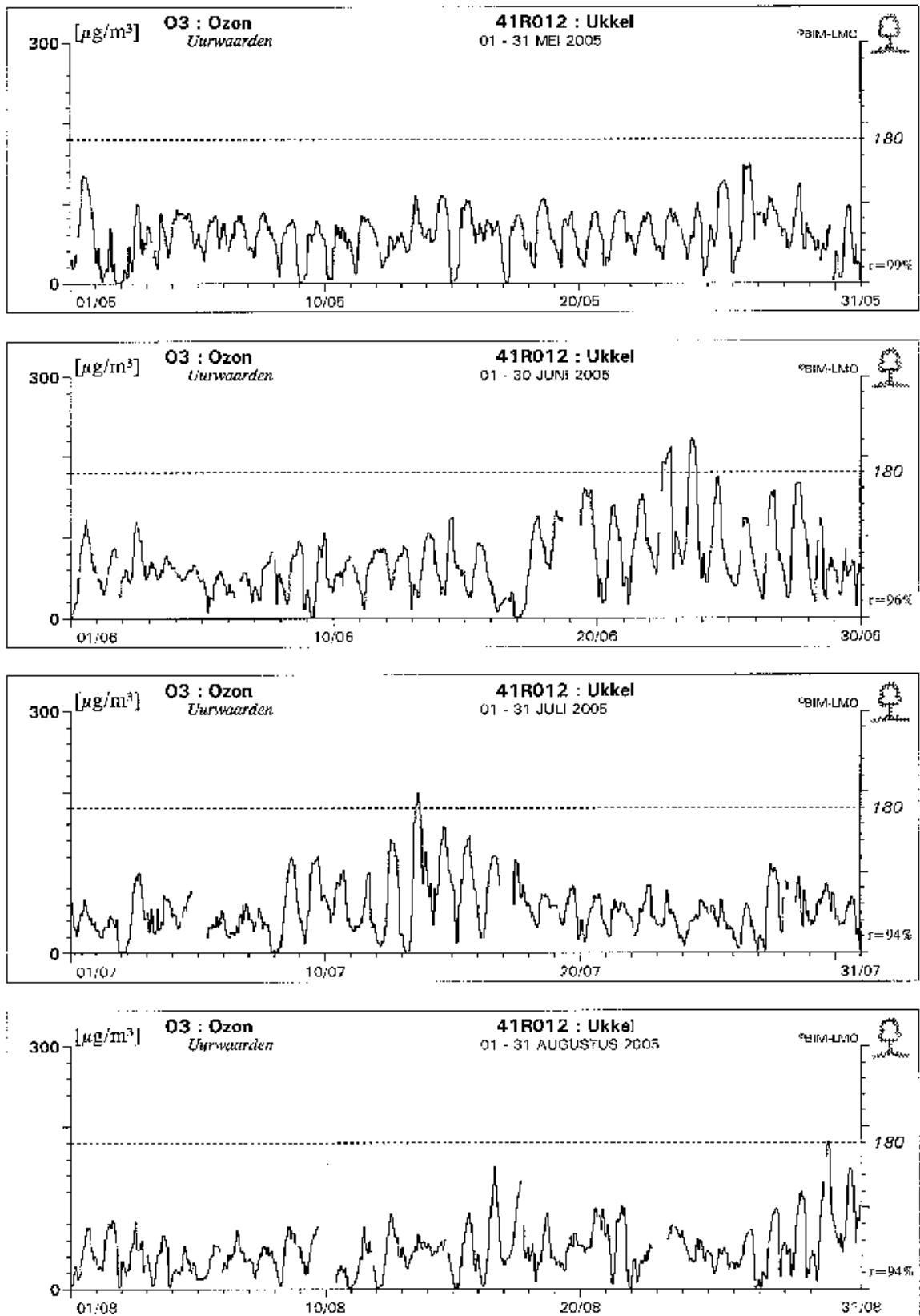
Fig. 2 : Evolutie O 3 -concentratie te Ukkel tijdens de maanden mei, juni, juli en augustus 2005
