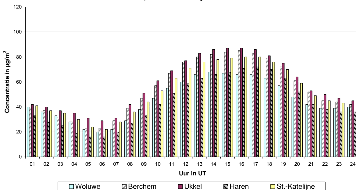
Fig. 4 : Gemiddeld dagverloop van de O 3 -concentratie in de periode mei - augustus 2005
