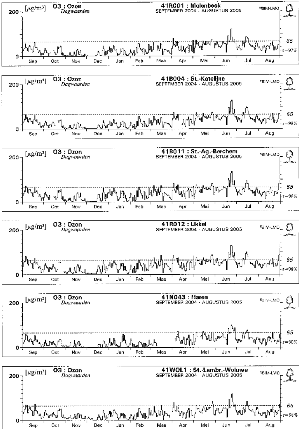
Fig. 3 : Evolutie O 3 -dagwaarden in het Brussels Hoofdstedelijk Gewest Periode : september 2004 – augustus 2005
