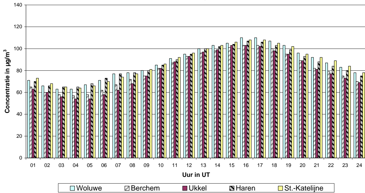
Fig. 6 : Gemiddeld dagverloop gasvormige oxidantia [O 3 + NO 2 ] in de periode mei – augustus 2005
