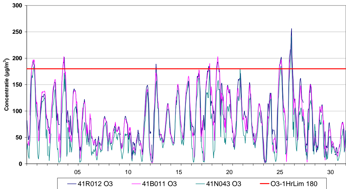
Fig. 4 : Evolutie van de uurwaarden voor ozon – Ukkel, Berchem en Haren – Juli 2006
