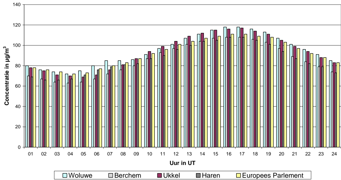
Fig. 8 : Gemiddeld dagverloop voor de som van de gasvormige oxidantia [O 3 + NO 2 ], uitgedrukt als equivalent massaconcentratie ozon, tijdens de periode mei – augustus 2006
