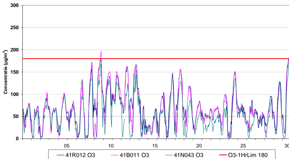
Fig. 3 : Evolutie van de uurwaarden voor ozon – Ukkel, Berchem en Haren – Juni 2006
