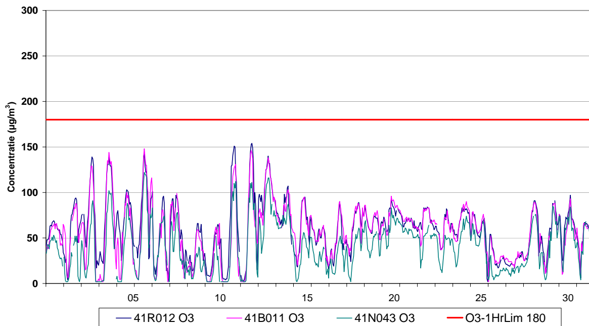
Fig. 2 : Evolutie van de uurwaarden voor ozon – Ukkel, Berchem en Haren – Mei 2006
