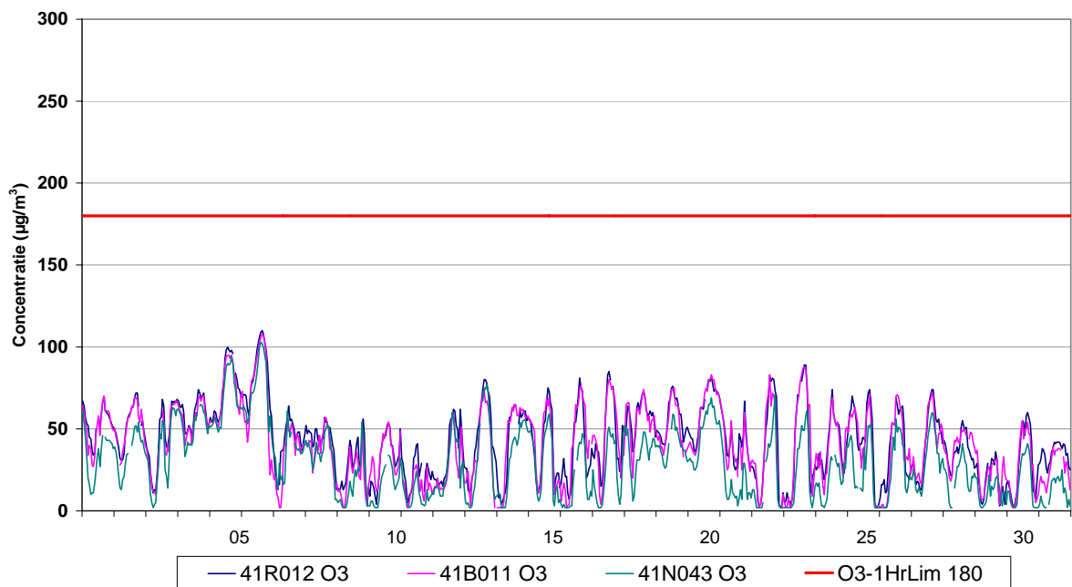
Fig. 5 : Evolutie van de uurwaarden voor ozon – Ukkel, Berchem en Haren – Augustus 2006
