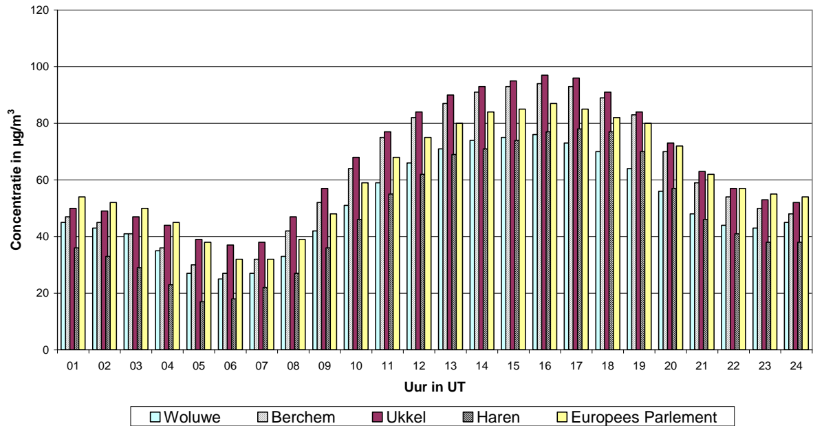
Fig. 6 : Gemiddeld dagverloop van de O 3 -concentratie in de periode mei – augustus 2006
