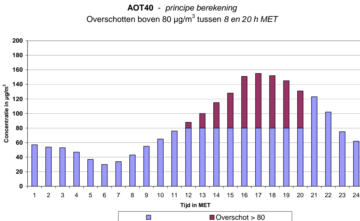
Fig. 9 : AOT40 : Voorstelling overschotten boven 80 \mu\text{g}/\text{m}^3 tussen 8:00 en 20:00 h MET
