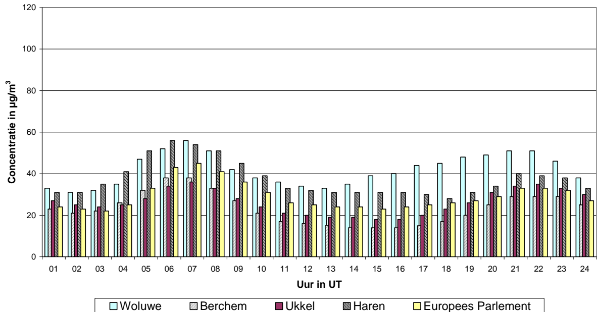
Fig. 7 : Gemiddeld dagverloop van de NO 2 -concentratie in de periode mei – augustus 2006
