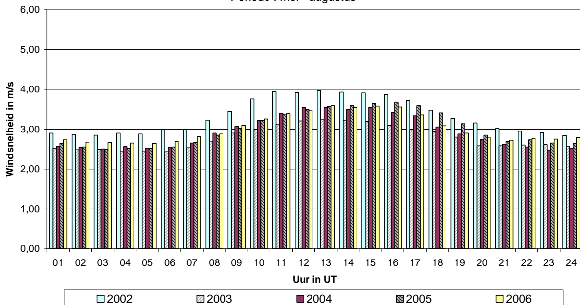
Gemiddeld dagverloop Windsnelheid Vergelijking 2002, 2003, 2004, 2005 en 2006 Periode : mei - augustus
