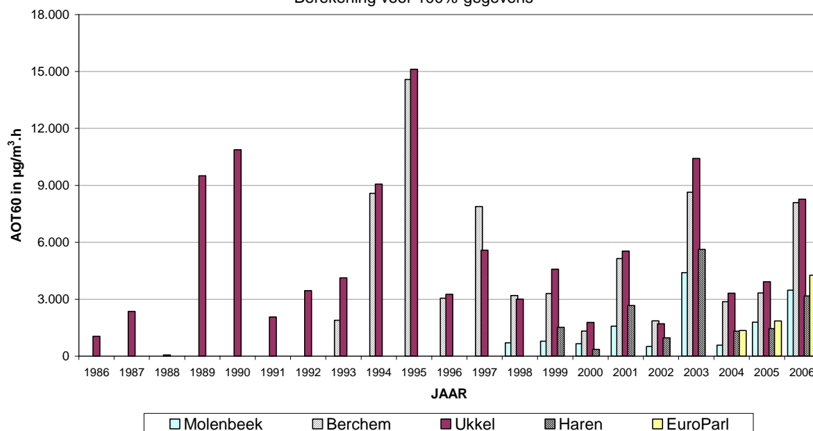
Fig. 18: Evolutie AOT60 in de tijd (1986-2006) Periode: JANUARI – DECEMBER (1986 – 2005) 2006 : januari - september
