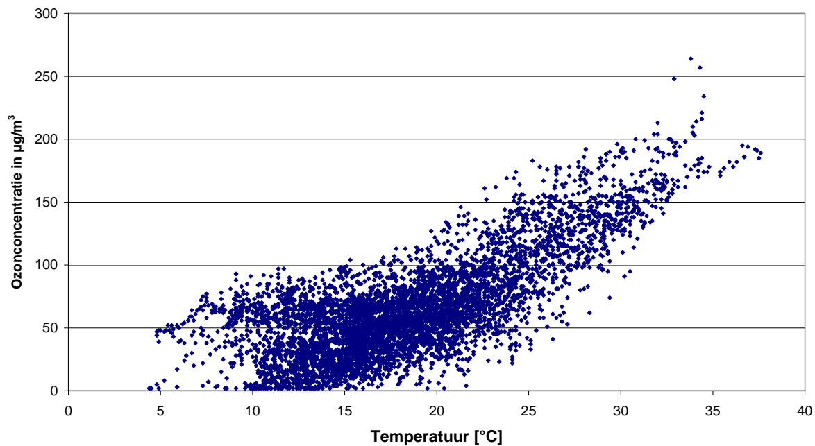
Fig. 36 : Ukkel : Ozonconcentraties versus temperatuur (mei - augustus 2006)
