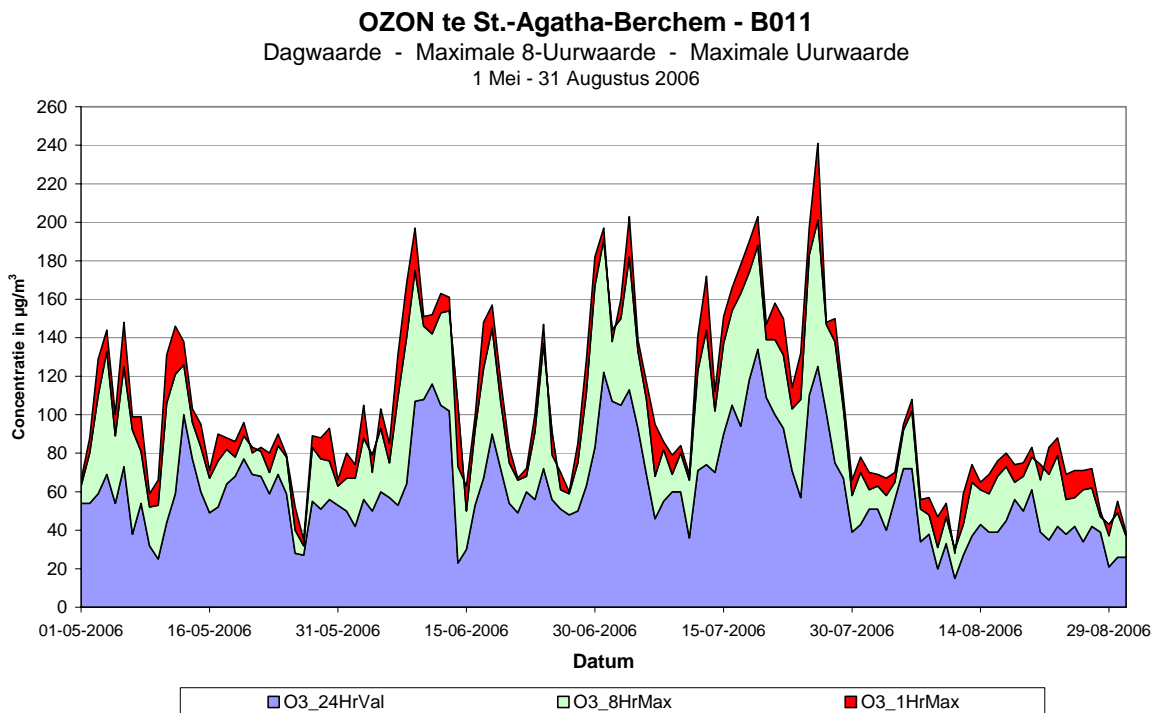
Fig. 16 : Ozon - Evolutie Dagwaarde (24HrVal), maximale 8-uurwaarde (8HrMax) en maximale uurwaarde (1HMax). Periode : mei - augustus 2006 Meetposten te Ukkel en St.-Agatha-Berchem
