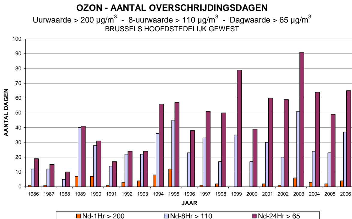
Fig. 19 : Ozon : aantal dagen met overschrijdingen (richtlijn 92/72/EG) Periode : januari - december (1986 t/m 2005) 2006 : januari - september
