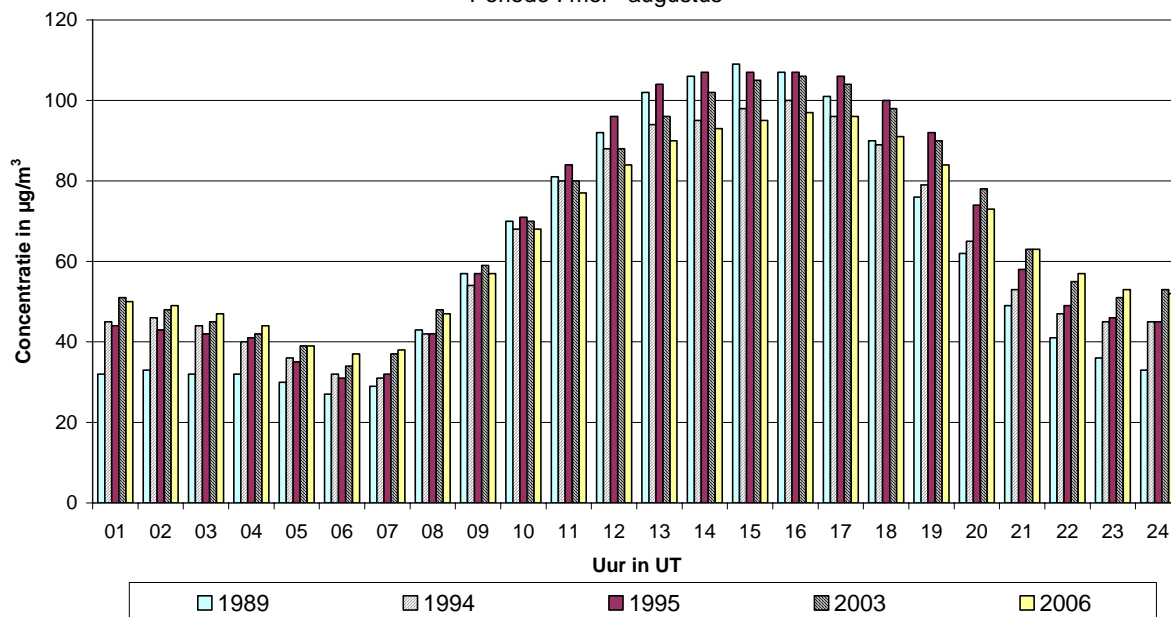
Fig. 31 : Gemiddeld dagverloop O 3 -concentratie te Ukkel (R012) Evolutie tijdens de ozonrijke zomerperiodes (1989-1994-1995-2003-2006)
