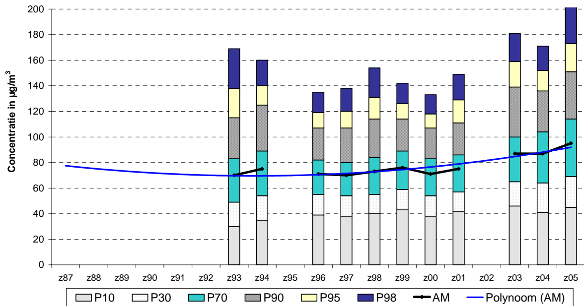
Fig. 35 : Kunst-Wet – Evolutive NO 2 -uurwaarden (1991-2006) Zomerperiode "april – september"
