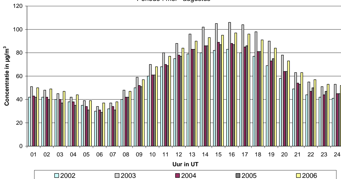
Fig. 30 : Gemiddeld dagverloop O 3 -concentratie te Ukkel (R012) Evolutie tijdens recente zomerperiodes (2002-2006)
