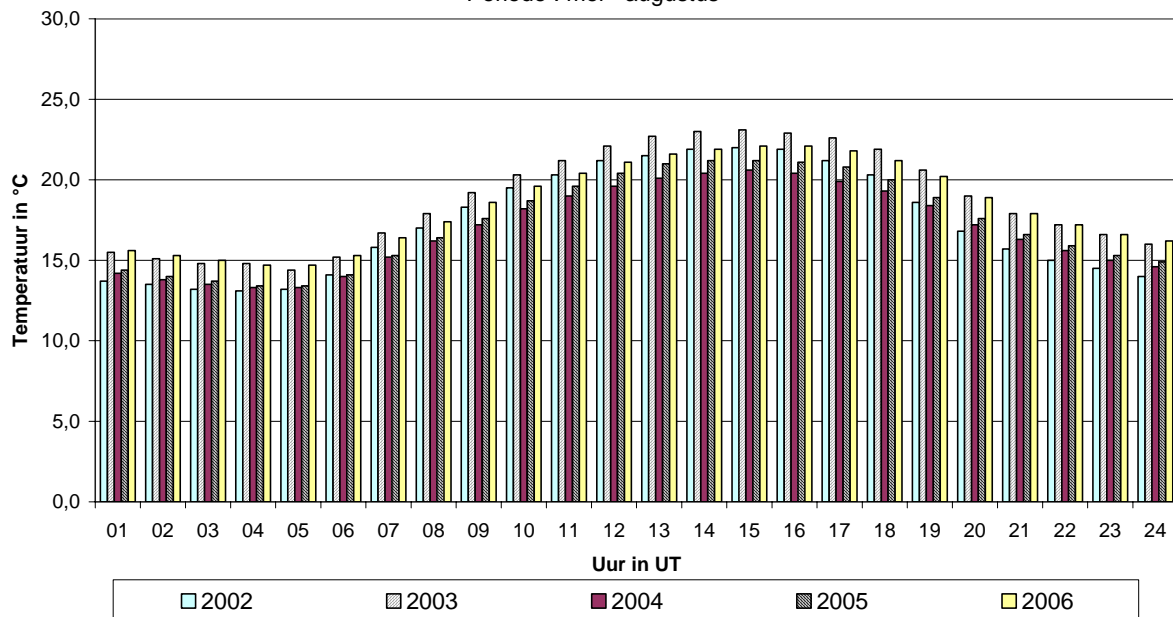
Gemiddeld dagverloop Temperatuur Vergelijking 2002, 2003, 2004, 2005 en 2006 Periode : mei - augustus
