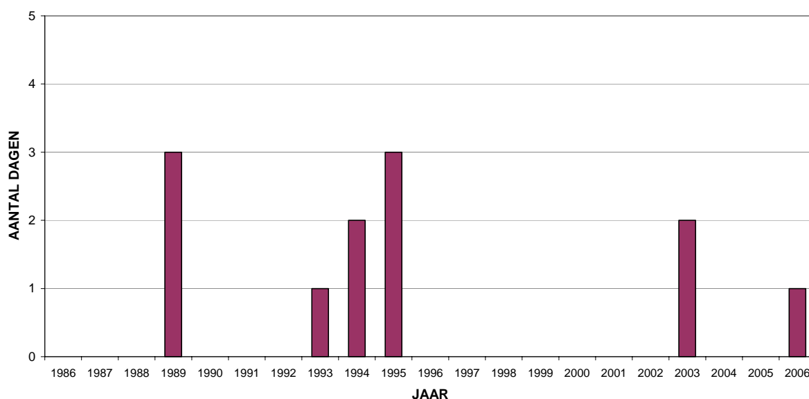
Fig. 14 : Ozon - Evolutie aantal overschrijdingsdagen in het Brussels Hoofdstedelijk Gewest Alarmdrempel: Uurwaarde > 240 µg/m 3
