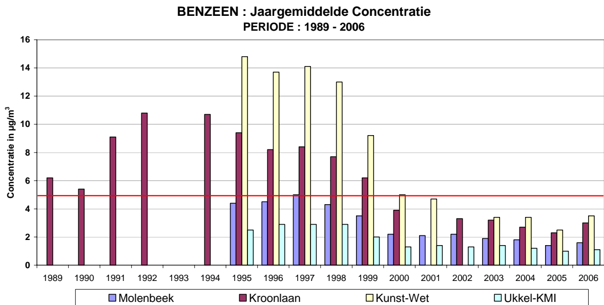
Fig. 22 : Benzeen - Evolutie jaargemiddelde concentratie Periode : januari – december (1989-2005) 2006 : januari - september
