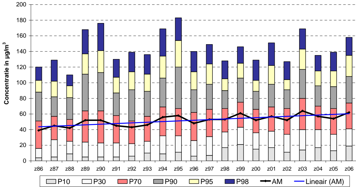
Fig. 28 : Evolutive O 3 -uurwaarden te Ukkel (1986-2006) Zomerperiode "april – september"
