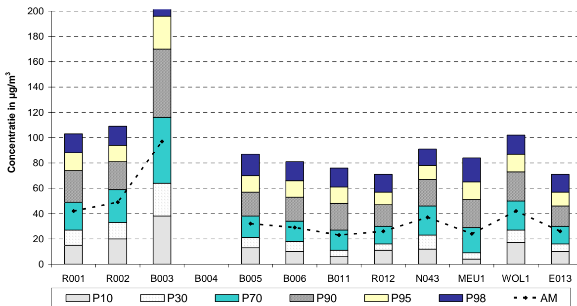
Fig. 27 : NO 2 - Cumulatieve frequentieverdeling halfuurswaarden: mei - augustus 2006
