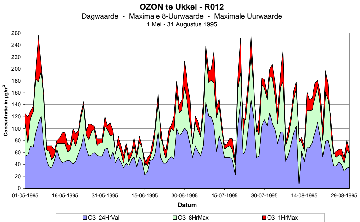
Fig. 17 : Ozon te Ukkel - Evolutie Dagwaarde (24HrMax), maximale 8-uurwaarde (8HrMax) en maximale uurwaarde (1HrMax). Vergelijking zomerperiode 2003 en 1995
