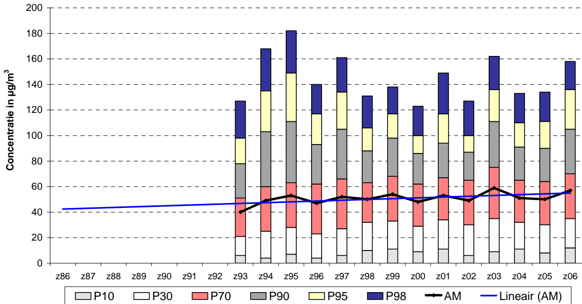
Fig. 29 : Evolutive O 3 -uurwaarden te St.-Ag.-Berchem (1993-2006) Zomerperiode "april – september"
