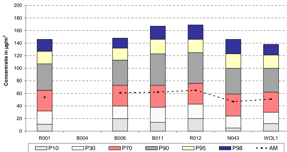
Fig. 26 : Ozon - Cumulatieve frequentieverdeling halfuurswaarden : mei - augustus 2006
