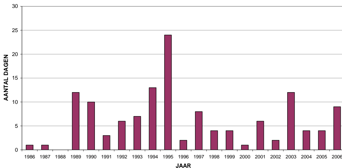
Fig. 13 : Ozon - Evolutie aantal overschrijdingsdagen in het Brussels Hoofdstedelijk Gewest Informatiedrempel: Uurwaarde > 180 µg/m 3
