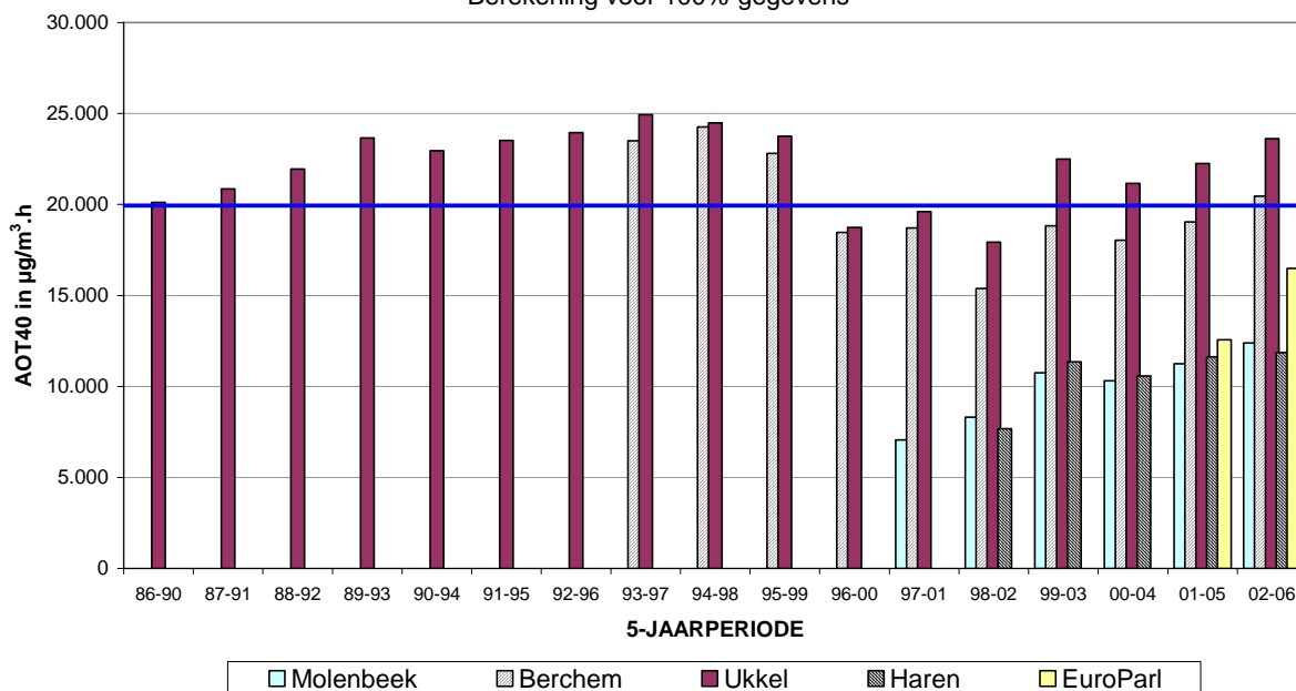
Fig. 12: Evolutie AOT40-AS in de tijd (1986-2006) AOT over de periode April – September, 8-20 h MET - Midden-Europese tijd Resultaten per jaar en gemiddeld over 5 jaar
