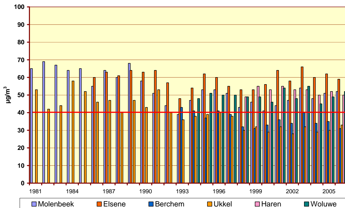
Fig. 20 : NO 2 - Evolutie jaargemiddelde concentratie ( alle dagen ) en gemiddelde concentratie op ' werkdagen ' – Periode 1981-2006
