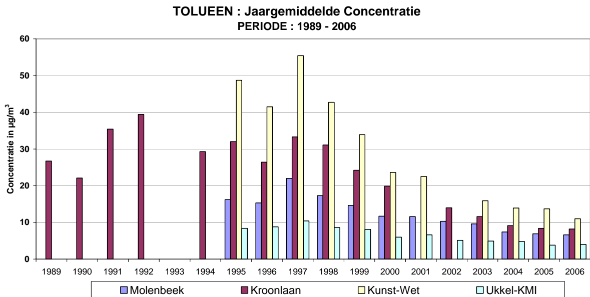
Fig. 23 : Tolueen - Evolutie jaargemiddelde concentratie Periode : januari – december (1989-2005) 2006 : januari - september
