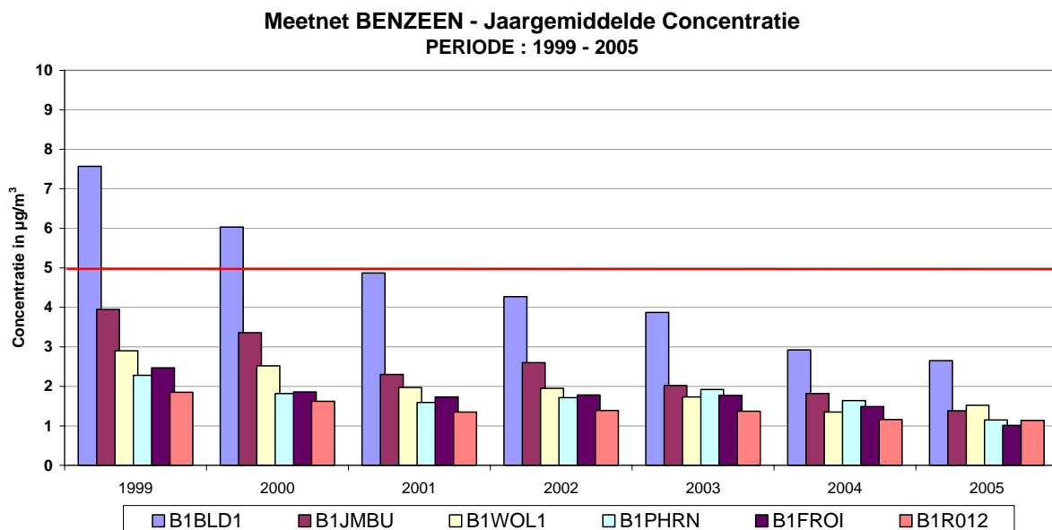
Fig. 24 : Benzeen – Evolutie jaargemiddelde concentratie in een aantal meetpunten van het benzeenmeetnet – Periode : 1999 - 2005
