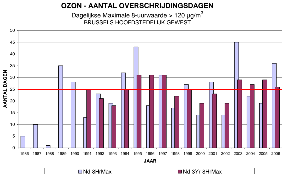
Fig. 10 : Ozon - Evolutie aantal overschrijdingsdagen in het Brussels Hoofdstedelijk Gewest Streefwaarde voor de gezondheid: Maximale 8-uurwaarde > 120 µg/m 3 Periode : Januari – December (1986-2005) [2006]: januari – september
