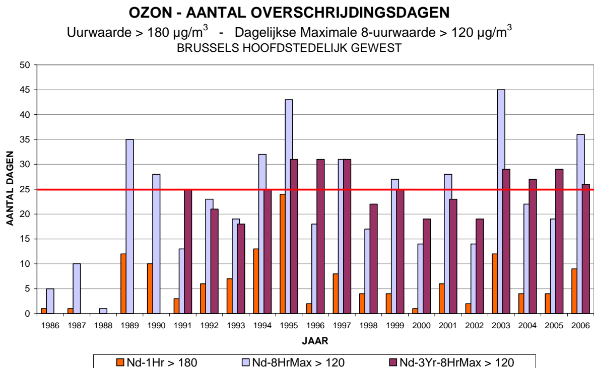
Fig. 15 : Ozon : aantal dagen met overschrijdingen in het Gewest Jaarperiodes : 1 januari – 31 december (1986-2005) Voorlopige resultaten voor het jaar 2006 (1 januari – 30 september)
