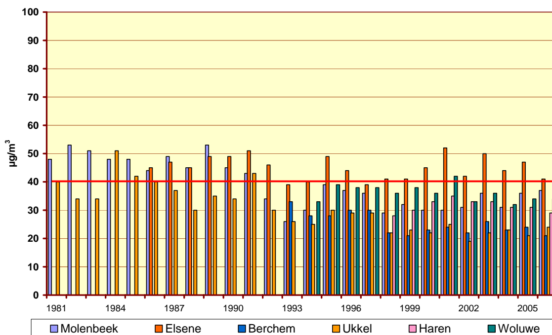
Fig. 21 : NO 2 - Evolutive gemiddelde concentratie op 'Zaterdag' en 'Zondag' Periode 1981-2006
