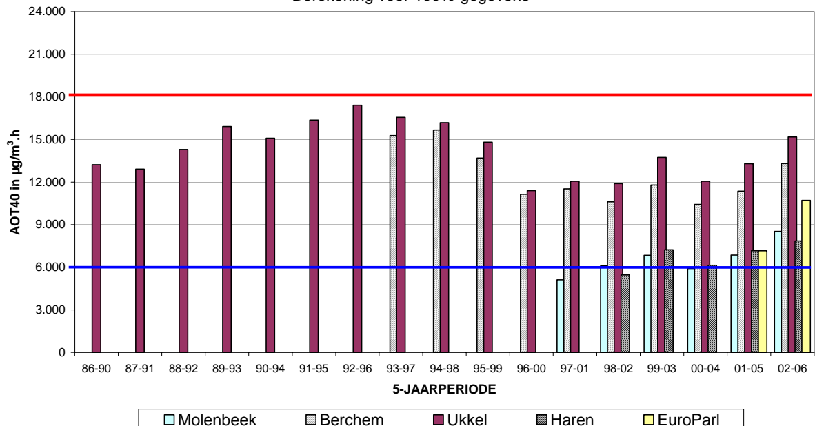
Fig. 11: Evolutie AOT40-MJ in de tijd (1986-2006) AOT40 over de periode Mei – Juli, 8-20 h MET - Midden-Europese tijd Resultaten per jaar en gemiddeld over 5 jaar
