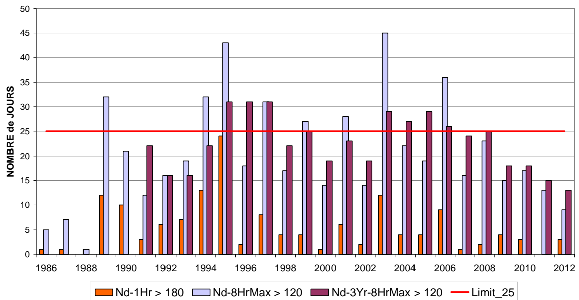
Fig. 21 : Ozone : nombre de jours avec dépassements en Région de Bruxelles-Capitale Périodes annuelles : 1 janvier – 31 décembre (1986 – 2011) Données partielles pour l'année 2012 (1 er janvier – 30 septembre)
