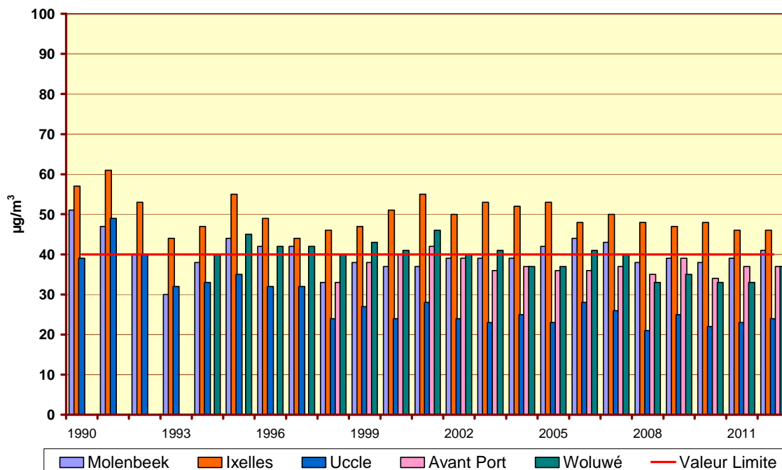
Fig. 27.c : NO 2 – Évolution de la concentration moyenne les 'Samedis' Périodes annuelles 1990 – 2011 et « Octobre 2011 – Septembre 2012 »
