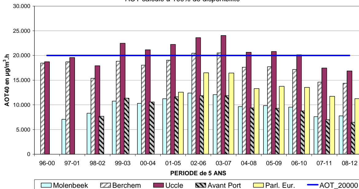
Fig. 16 : Évolution AOT40-AS dans le temps (1996-2012) AOT40 pour la période Avril – Septembre, 8-20 h d'Europe centrale Résultats par an et moyenné sur 5 ans
