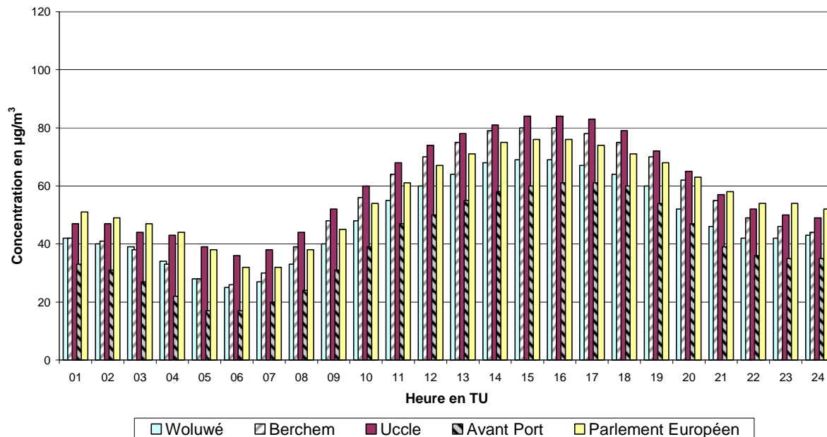
Fig. 8 : Évolution journalière moyenne des concentrations en O 3 durant la période mai-août 2012
