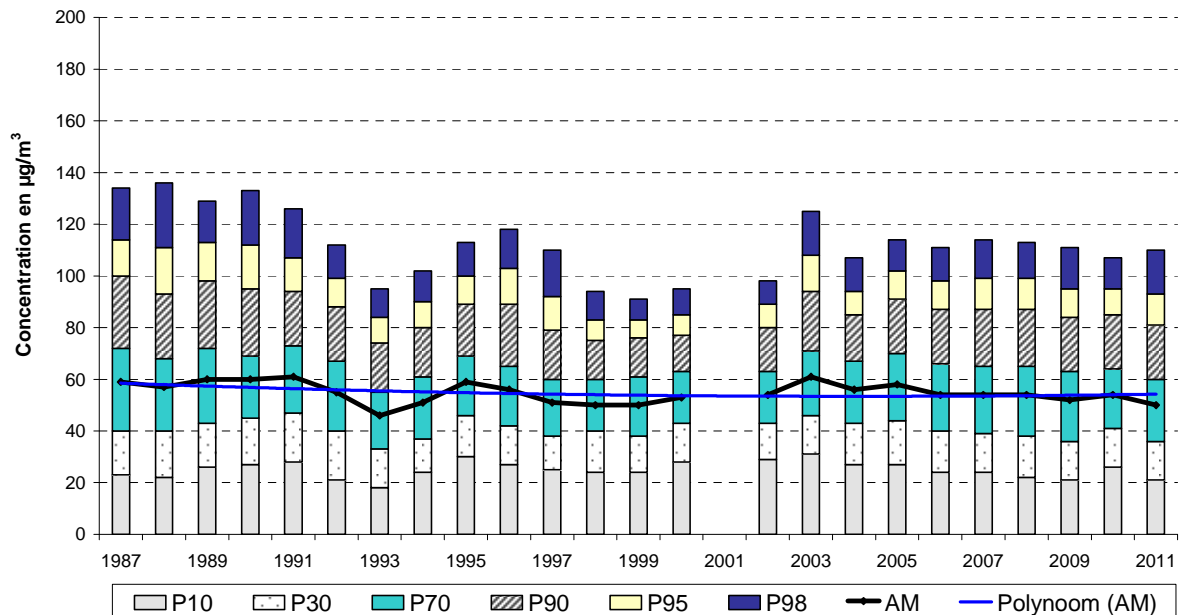
Fig. 73 : NO x à Ixelles – Avenue de la Couronne ( canyon street ) – Valeurs horaires Évolution à long terme - Périodes annuelles 1987 - 2011
