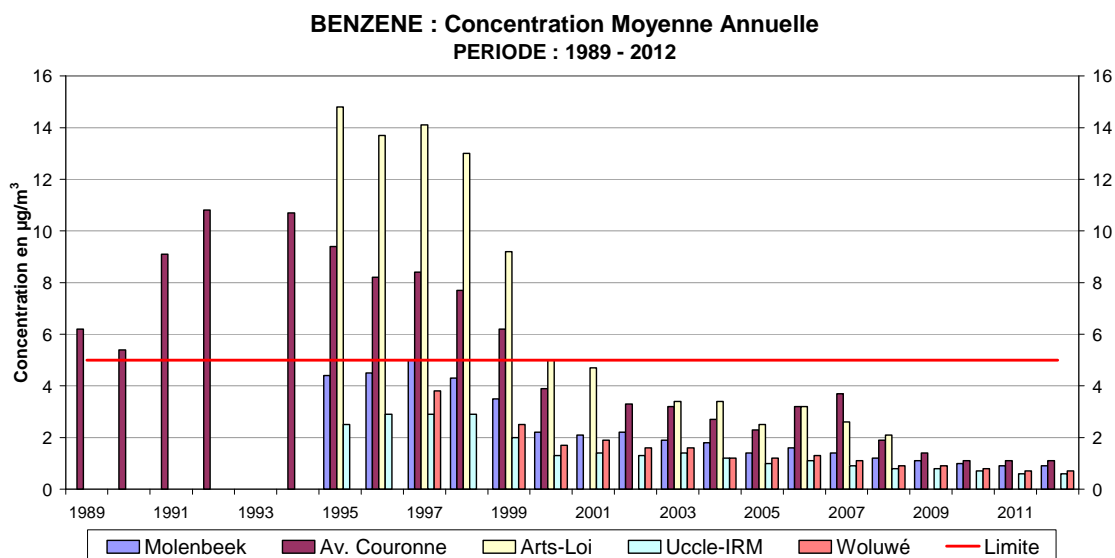
Fig. 28 : Benzène – Évolution de la concentration moyenne annuelle Période : Janvier – Décembre (1989-2011) et 'Octobre 2011 – Septembre 2012'
