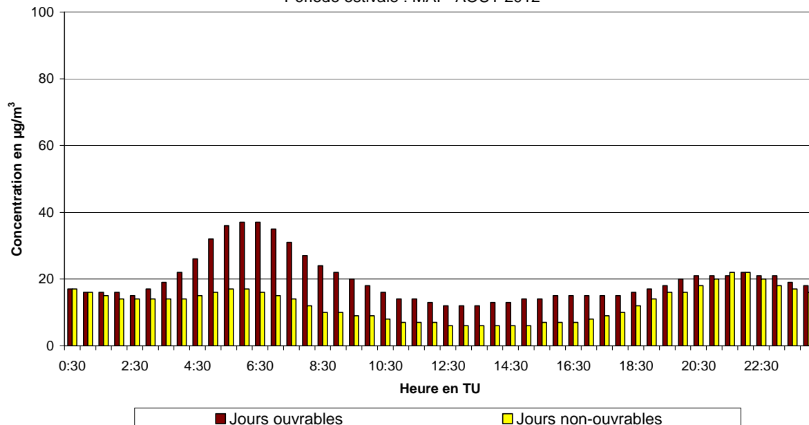
Fig. 47.b : Berchem-Ste-Agathe : Évolution journalière moyenne de la concentration en NO 2 les jours ouvrables et non-ouvrables pendant le période mai – août 2012
