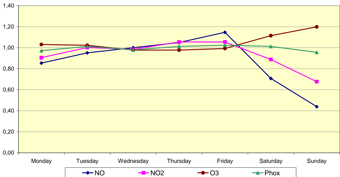
Fig. 59.b : Poste de mesure à Molenbeek – Profil hebdomadaire moyen des concentrations en NO, NO 2 , O 3 et [NO 2 +O 3 ] sur trois périodes estivales successives : 'avril – septembre' 2010, 2011 et 2012
