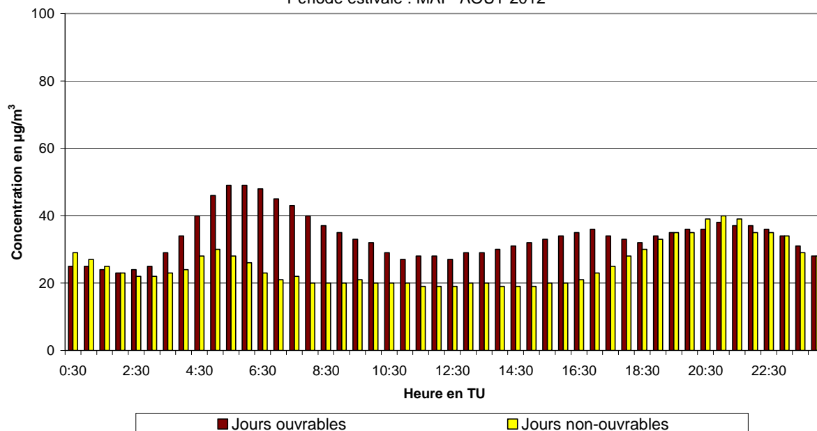
Fig. 48.b : Molenbeek : Évolution journalière moyenne de la concentration en NO 2 les jours ouvrables et non-ouvrables pendant la période mai – août 2012
