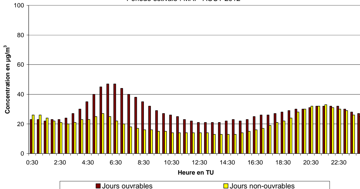
Fig. 52.b : Ste-Catherine : Évolution journalière moyenne de la concentration en NO 2 les jours ouvrables et non-ouvrables pendant la période mai – août 2012
