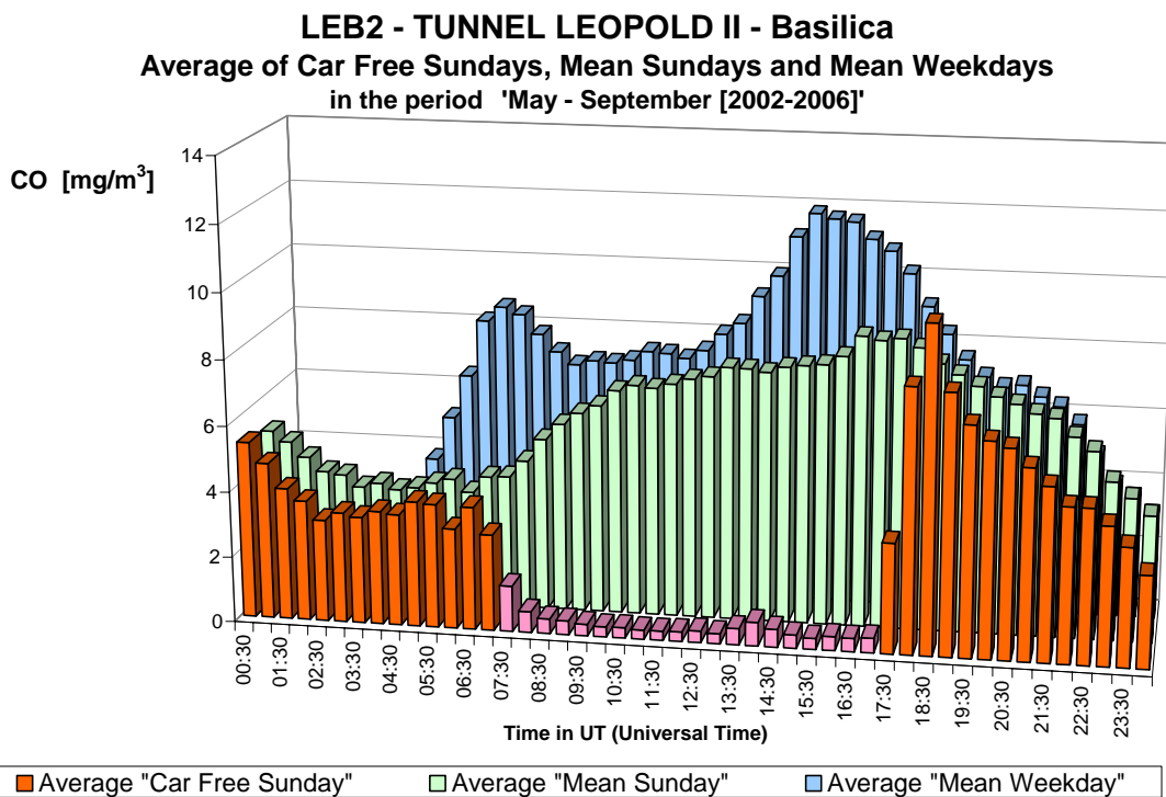
Fig. 32.b : CO in de Leopold II tunnel, richting Basiliek – Gemiddelde Dagprofiel van de vijf autoluwe zondagen en van alle zondagen en werkdagen in de periodes 'mei – september 2002-2006'
