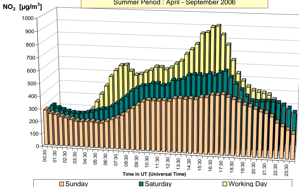
Fig. 16 : NO 2 -dagverloop in de meetpost 41LEB2 (richting basiliek) Vergelijking voor een gemiddelde zondag, zaterdag en werkdag Winterperiode 2006-2007 en zomerperiode 2006
