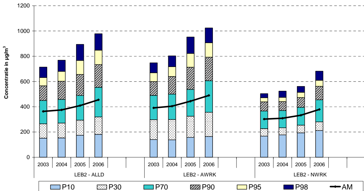
Fig. 5 : NO 2 - Cumulatieve Frequentieverdeling Uurwaarden in beide meetposten van de Leopold II tunnel. Selectie alle dagen , alle werkdagen en alle niet-werkdagen Jaarperiodes 2003, 2004, 2005 en 2006
