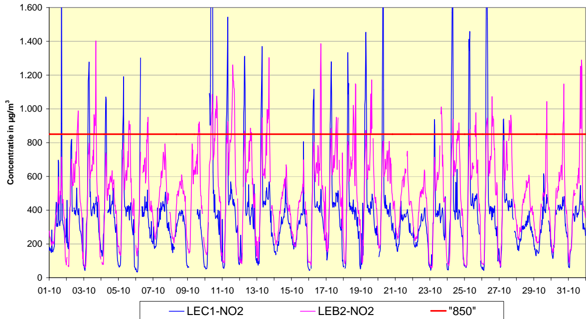
Fig. 1: NO 2 - Evolutie van de uurwaarden en de halfuurwaarden tijdens de maand oktober 2006 Meetplaats 41LEC1, richting Centrum - Meetplaats 41LEB2, richting Basiliek
