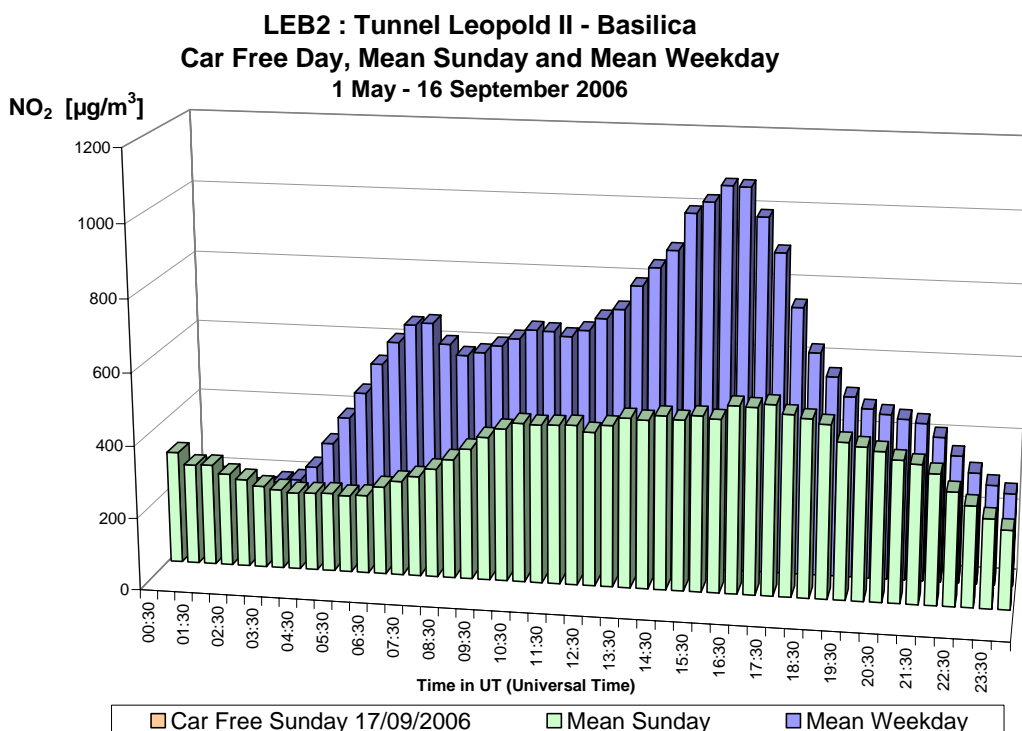
Fig. 28.a : NO 2 in de Leopold II tunnel, richting Basiliek – Dagprofiel van een gemiddelde zondag en een gemiddelde werkdag in de periode 'mei – september 2006' Wegens technische problemen geen gegevens voor de autoluwe zondag 17-09-2006
