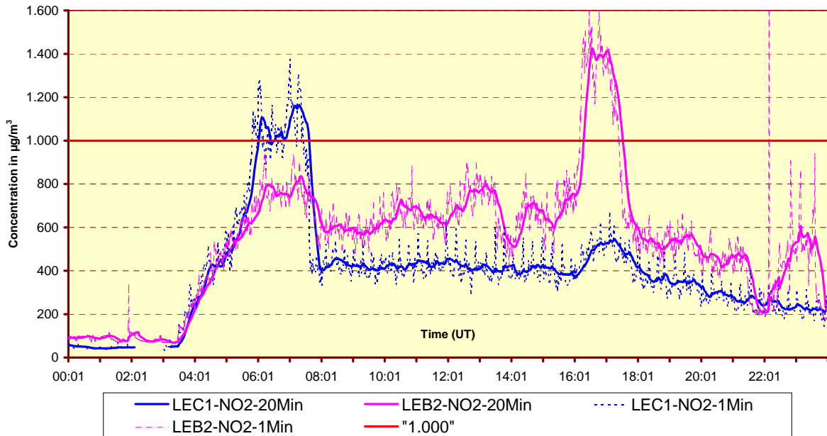
Fig. 4: NO 2 - evolutie minuutwaarden en voortschrijdend 20-minuutsgemiddelde in beide meetposten van de Leopold II tunnel Dinsdag 03 oktober en maandag 16 oktober 2006
