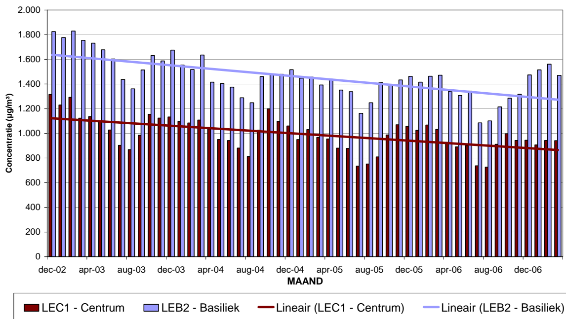
Fig. 9 : NO 2 en NO - Evolutie maandgemiddelde concentratie in beide meetposten van de Leopold II tunnel. Periode "December 2002 – Maart 2007"
