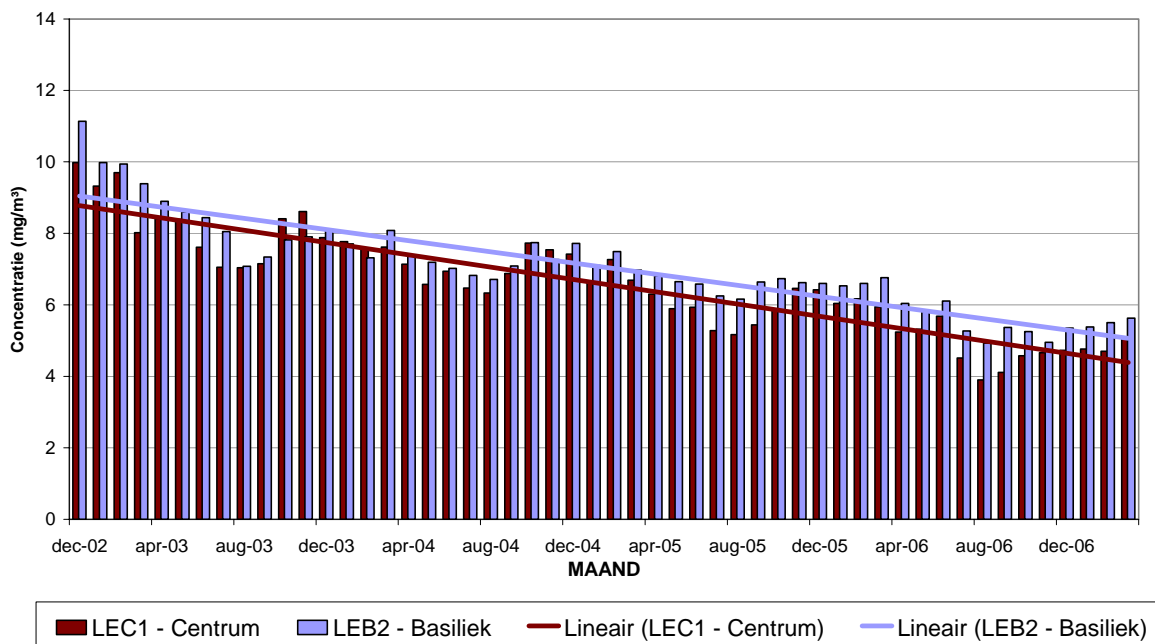
Fig. 10 : NO x en CO - Evolutie maandgemiddelde concentratie in beide meetposten van de Leopold II tunnel. Periode "December 2002 – Maart 2007"
