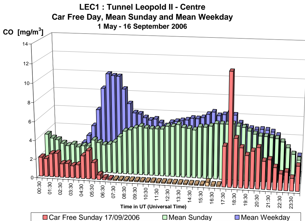
Fig. 31.a : CO in de Leopold II tunnel, richting Centrum – Dagprofiel autoluwe zondag 17-09-2006, gemiddelde zondag en gemiddelde werkdag in de periode 'mei – september 2006'
