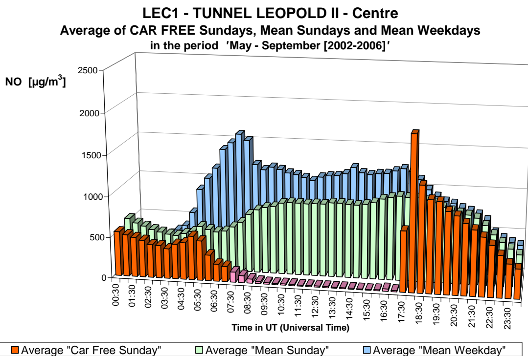
Fig. 29.b : NO in de Leopold II tunnel, richting Centrum – Gemiddelde Dagprofiel van de vijf autoluwe zondagen en van alle zondagen en werkdagen in de periodes 'mei – september 2002-2006'
