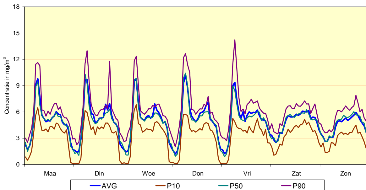
Fig. 23 : Meetpost 41LEC1 (centrum) - Gemiddeld weekverloop voor CO Vergelijking winterperiode 2006 - 2007 en zomerperiode 2006
