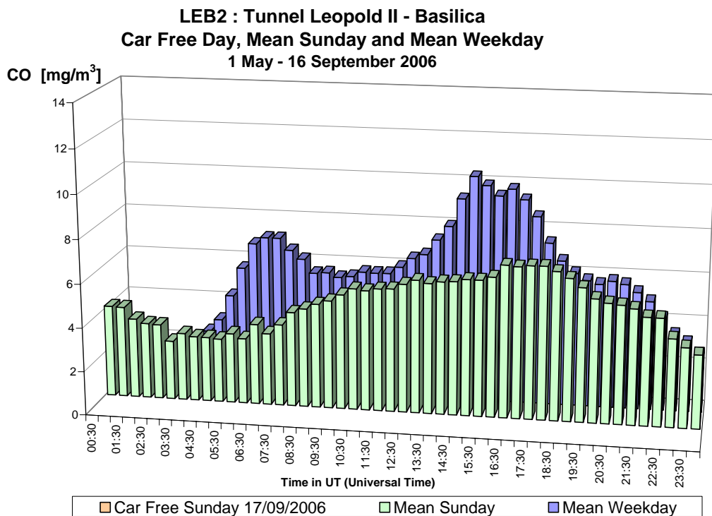
Fig. 32.a : CO in de Leopold II tunnel, richting Basiliek – Dagprofiel van een gemiddelde zondag en een gemiddelde werkdag in de periode 'mei – september 2006' Wegens technische problemen geen gegevens voor de autoluwe zondag 17-09-2006
