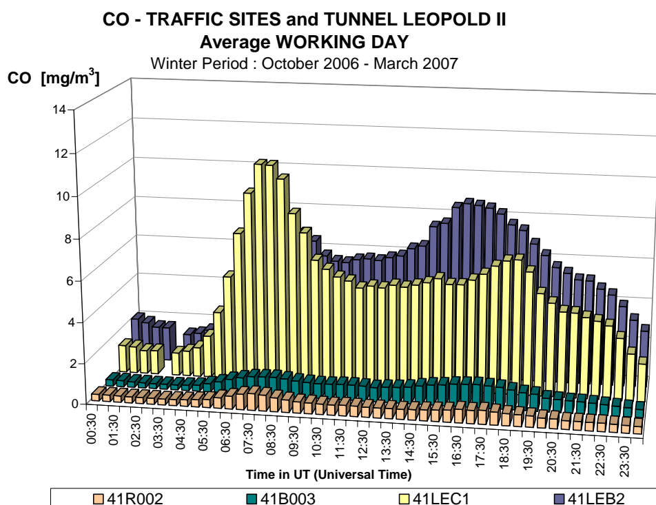
Fig. 33 : CO-dagverloop voor een gemiddelde werkdag tijdens de winter 2006-2007 Meetposten verkeer in de omgevingslucht - Kroonlaan (R002) en Kunst-Wet (B003) Meetposten in de tunnel Leopold II – LEC1 (centrum) en LEC2 (basiliek)
