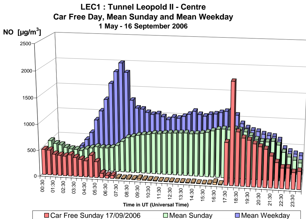
Fig. 29.a : NO in de Leopold II tunnel, richting Centrum – Dagprofiel autoluwe zondag 17-09-2006, gemiddelde zondag en gemiddelde werkdag in de periode 'mei – september 2006'
