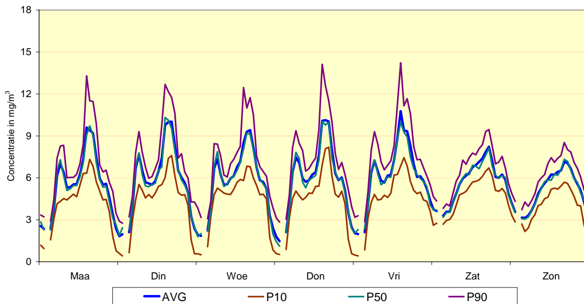
Fig. 24 : Meetpost 41LEB2 (basiliek) - Gemiddeld weekverloop voor CO Vergelijking winterperiode 2006 - 2007 en zomerperiode 2006
