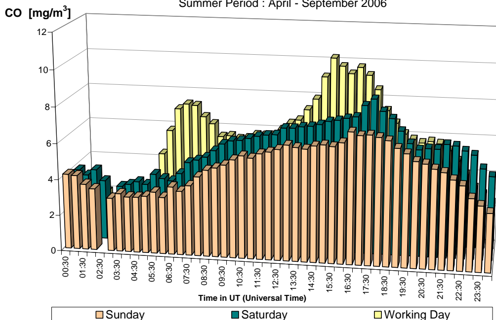
Fig. 20 : CO-dagverloop in de meetpost 41LEB2 (richting basiliek) Vergelijking voor een gemiddelde zondag, zaterdag en werkdag Winterperiode 2006-2007 en zomerperiode 2006
