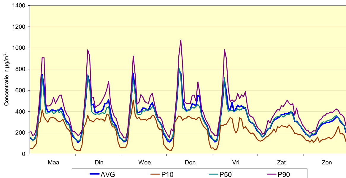
Fig. 21 : Meetpost 41LEC1 (centrum) - Gemiddeld weekverloop voor NO 2 Vergelijking winterperiode 2006 - 2007 en zomerperiode 2006
