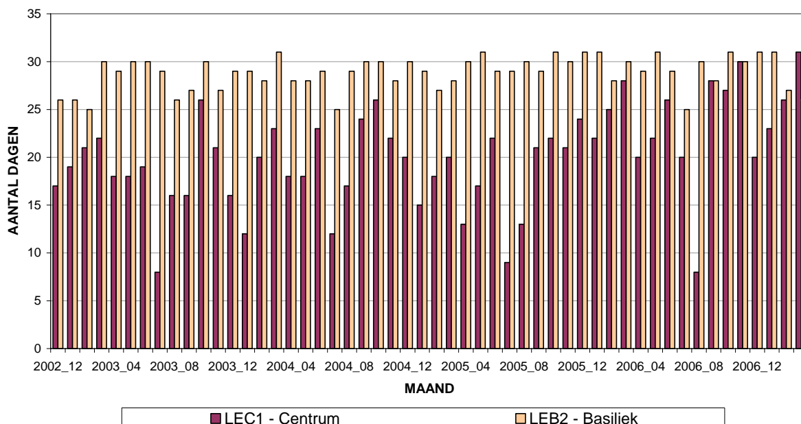
Fig. 14 : NO 2 -Uurwaarden > 400 µg/m 3 . Totaal aantal overschrijdingen per maand en aantal dagen per maand met overschrijding (december 2002 – maart 2007)
