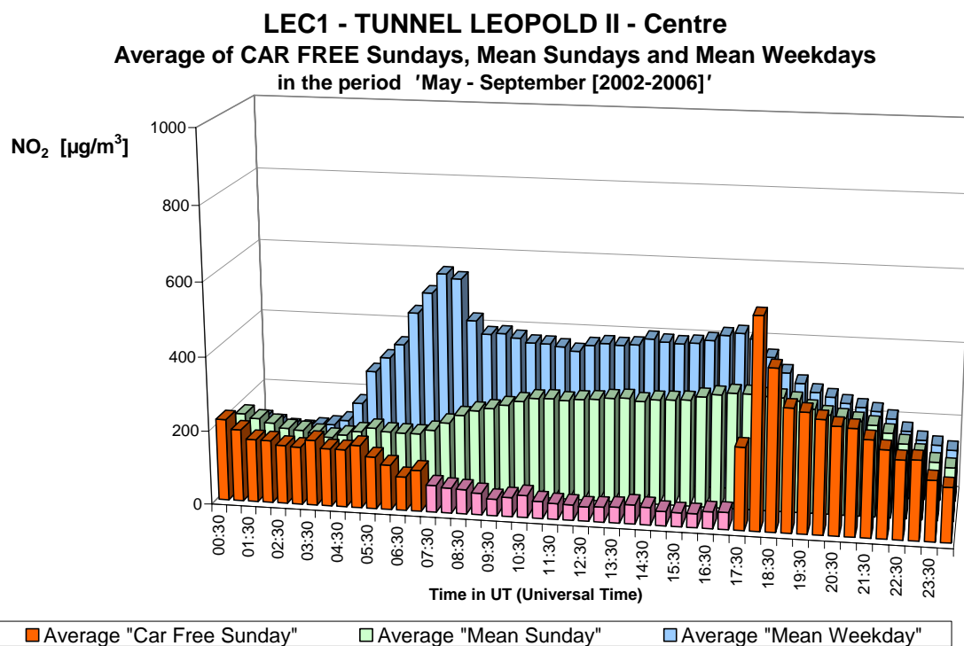
Fig. 27.b : NO 2 in de Leopold II tunnel, richting Centrum – Gemiddelde Dagprofiel van de vijf autoluwe zondagen en van alle zondagen en werkdagen in de periodes ‘mei – september 2002-2006’
