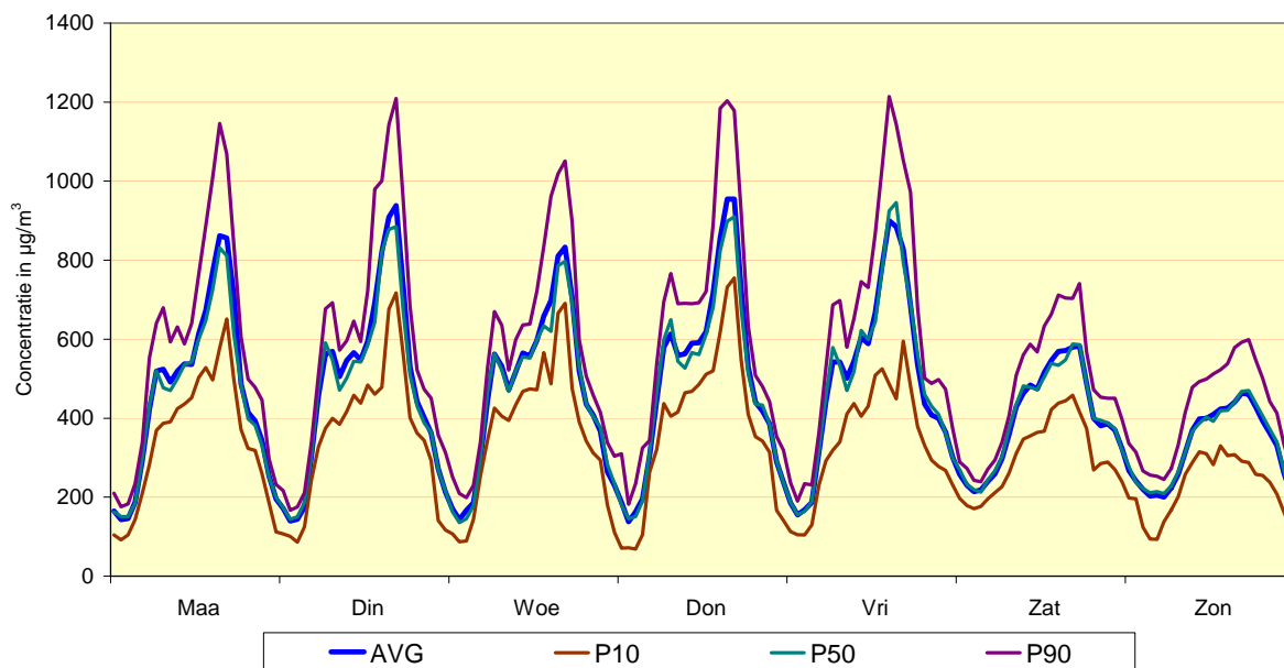
Fig. 22 : Meetpost 41LEB2 (basiliek) - Gemiddeld weekverloop voor NO 2 Vergelijking winterperiode 2006 - 2007 en zomerperiode 2006
