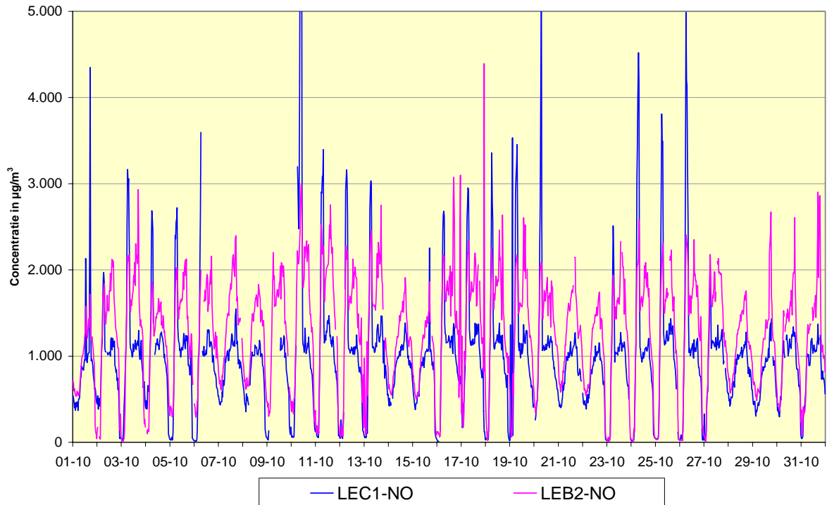
Fig. 2: NO - Evolutie van de uurwaarden en de halfuurswaarden tijdens de maand oktober 2006 Meetplaats 41LEC1, richting Centrum - Meetplaats 41LEB2, richting Basiliek
