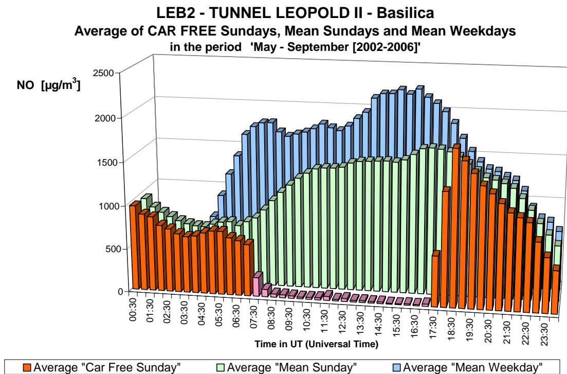
Fig. 30.b : NO in de Leopold II tunnel, richting Basiliek – Gemiddelde Dagprofiel van de vijf autoluwe zondagen en van alle zondagen en werkdagen in de periodes 'mei – september 2002-2006'
