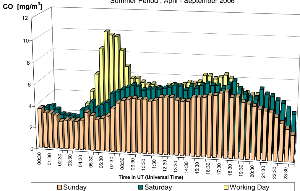
Fig. 19 : CO-dagverloop in de meetpost 41LEC1 (richting centrum) Vergelijking voor een gemiddelde zondag, zaterdag en werkdag Winterperiode 2006-2007 en zomerperiode 2006
