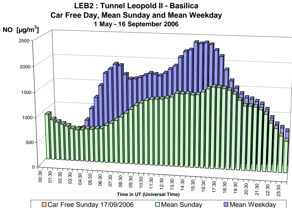
Fig. 30.a : NO in de Leopold II tunnel, richting Basiliek – Dagprofiel van een gemiddelde zondag en een gemiddelde werkdag in de periode 'mei – september 2006' Wegens technische problemen geen gegevens voor de autoluwe zondag 17-09-2006
