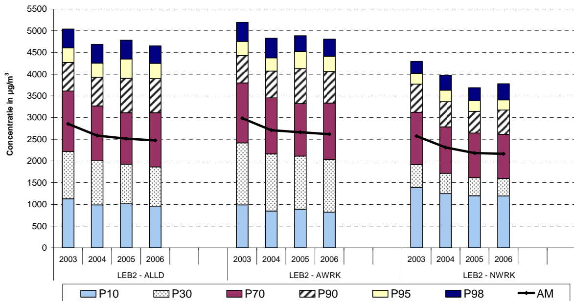
Fig. 8 : NO x - Cumulatieve Frequentieverdeling Uurwaarden in beide meetposten van de Leopold II tunnel. Selectie alle dagen , alle werkdagen en alle niet-werkdagen Jaarperiodes 2003, 2004, 2005 en 2006
