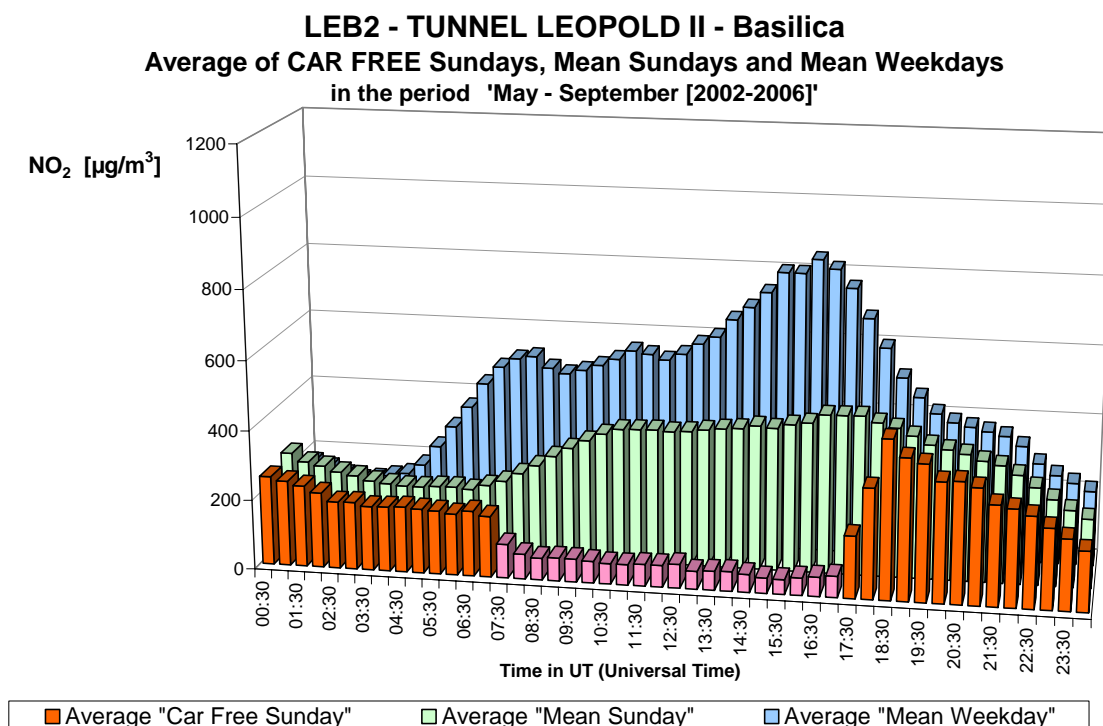
Fig. 28.b : NO 2 in de Leopold II tunnel, richting Basiliek – Gemiddelde Dagprofiel van de vijf autoluwe zondagen en van alle zondagen en werkdagen in de periodes 'mei – september 2002-2006'
