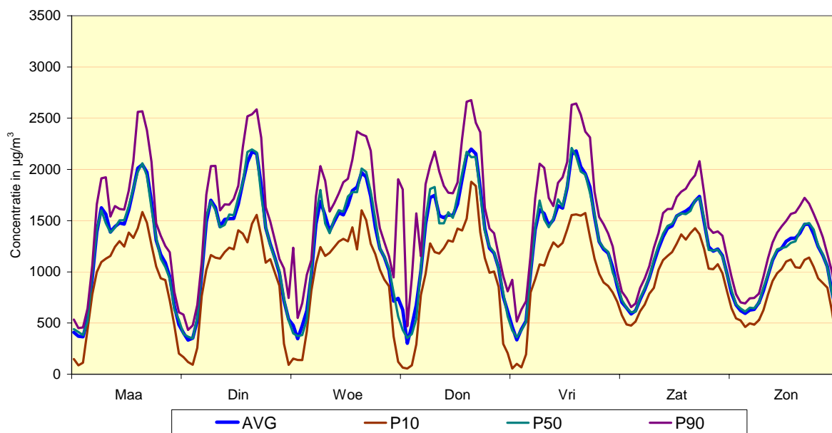
Fig. 26 : Meetpost 41LEB2 (basiliek) - Gemiddeld weekverloop voor NO Vergelijking winterperiode 2006 - 2007 en zomerperiode 2006
