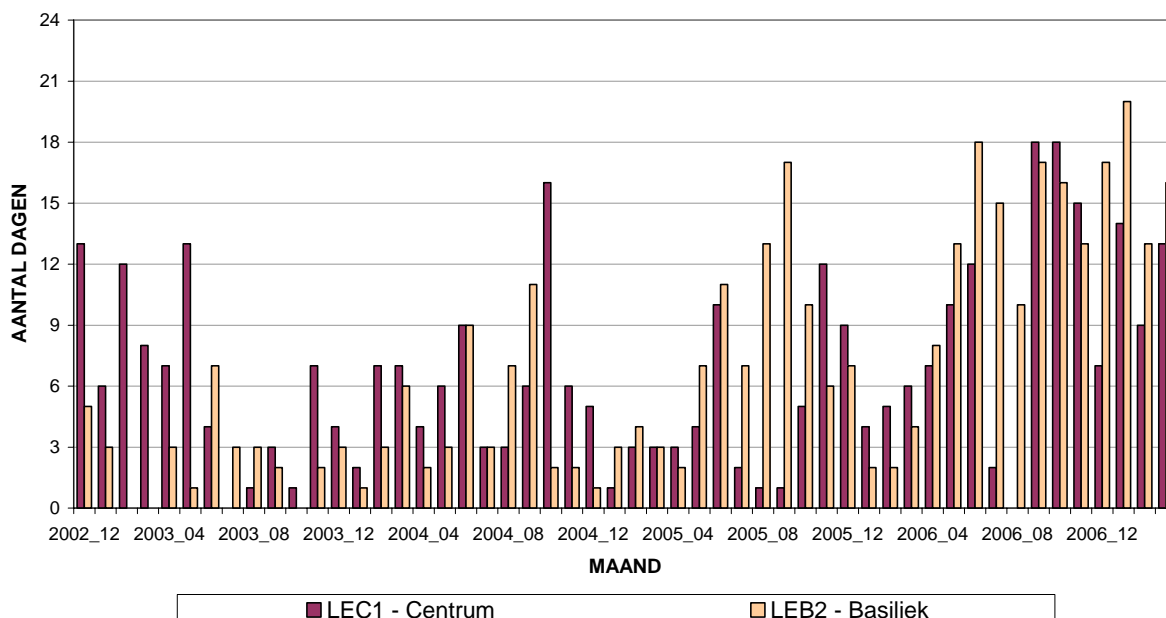
Fig. 12 : NO 2 – 20-Minutsgemiddelden > 1.000 µg/m 3 . Totaal aantal overschrijdingen per maand en aantal dagen per maand met overschrijding (december 2002 – maart 2007)
