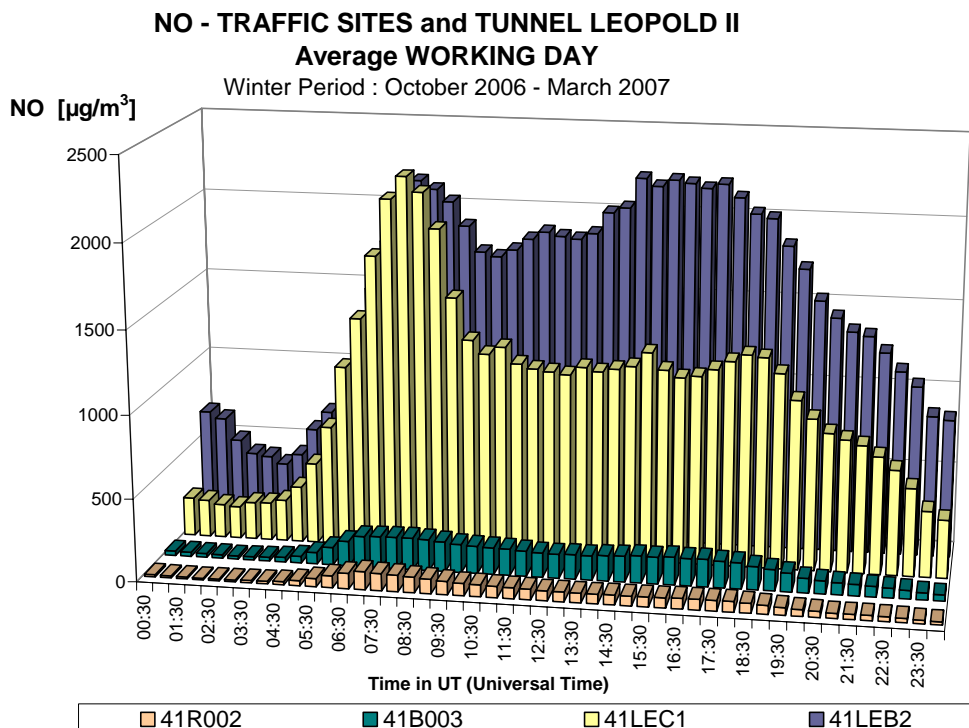
Fig. 34 : Dagverloop NO 2 en NO voor een gemiddelde werkdag tijdens de winter 2006-2007 Meetposten verkeer in de omgevingslucht - Kroonlaan (R002) en Kunst-Wet (B003) Meetposten in de tunnel Leopold II – LEC1 (centrum) en LEC2 (basiliek)
