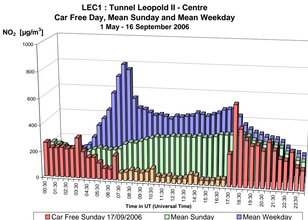
Fig. 27.a : NO 2 in de Leopold II tunnel, richting Centrum – Dagprofiel autoluwe zondag 17-09-2006, gemiddelde zondag en gemiddelde werkdag in de periode ‘mei – september 2006’
