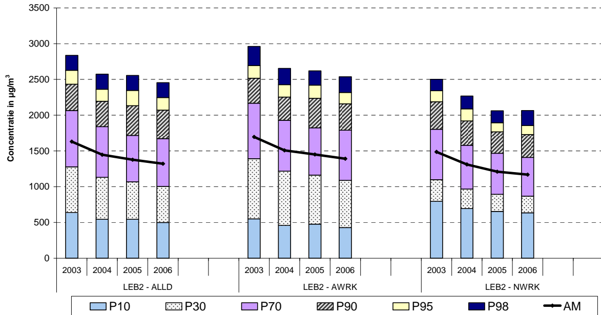
Fig. 7 : NO - Cumulatieve Frequentieverdeling Uurwaarden in beide meetposten van de Leopold II tunnel. Selectie alle dagen , alle werkdagen en alle niet-werkdagen Jaarperiodes 2003, 2004, 2005 en 2006
