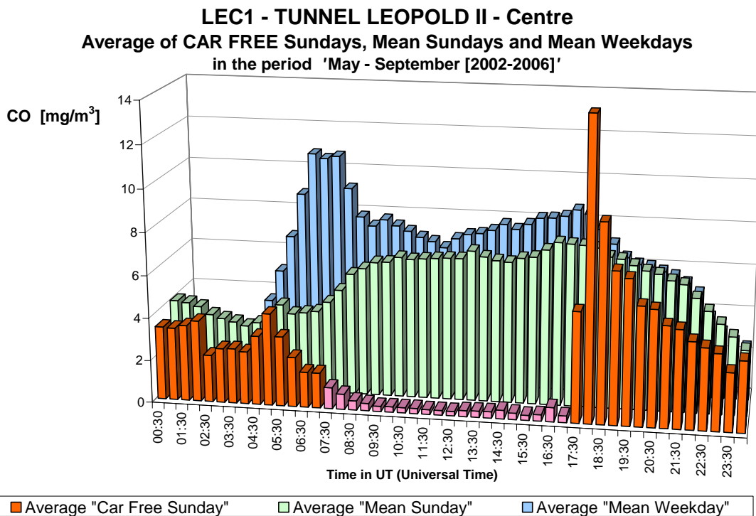
Fig. 31.b : CO in de Leopold II tunnel, richting Centrum – Gemiddelde Dagprofiel van de vijf autoluwe zondagen en van alle zondagen en werkdagen in de periodes 'mei – september 2002-2006'
