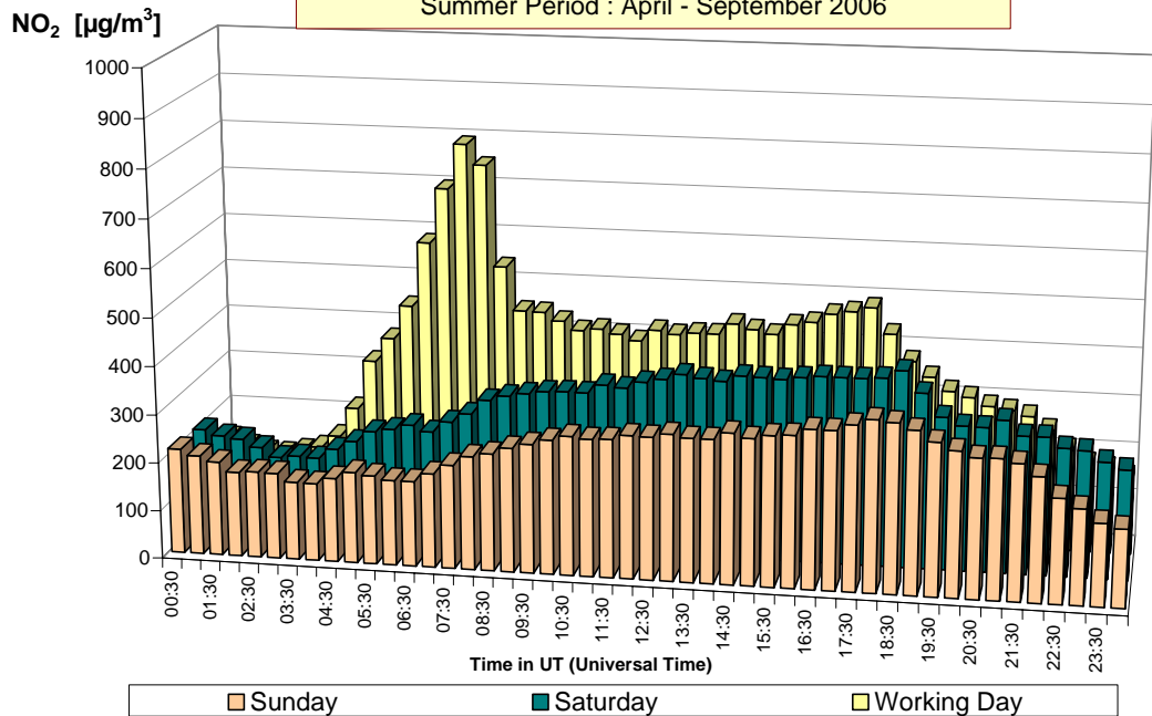
Fig. 15 : NO 2 -dagverloop in de meetpost 41LEC1 (richting centrum) Vergelijking voor een gemiddelde zondag, zaterdag en werkdag Winterperiode 2006-2007 en zomerperiode 2006
