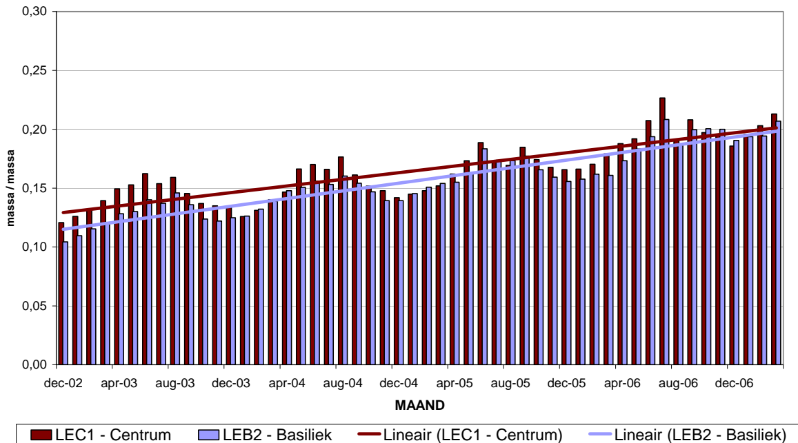
Fig. 11 : Evolutie van de verhouding NO 2 /NO x in beide meetposten van de Leopold II tunnel. Periode "December 2002 – Maart 2007"
