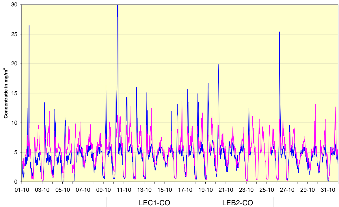
Fig. 3: CO - Evolutie van de uurwaarden en de halfuurswaarden tijdens de maand oktober 2006 Meetplaats 41LEC1, richting Centrum - Meetplaats 41LEB2, richting Basiliek
