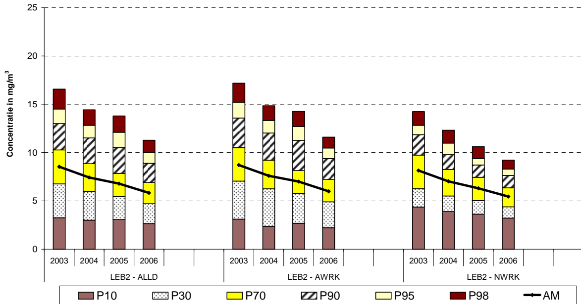
Fig. 6 : CO - Cumulatieve Frequentieverdeling Urwaarden in beide meetposten van de Leopold II tunnel. Selectie alle dagen , alle werkdagen en alle niet-werkdagen Jaarperiodes 2003, 2004, 2005 en 2006
