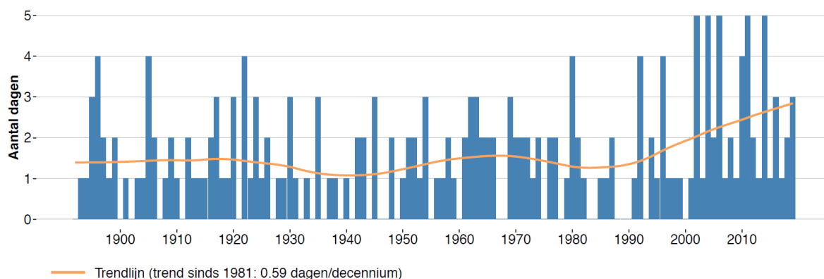
Figuur 2.8 : Aantal dagen tijdens de zomer (juni tot augustus) waarop de neerslaghoeveelheden in Ukkel 20 mm of meer bereikten, periode 1892-2019
