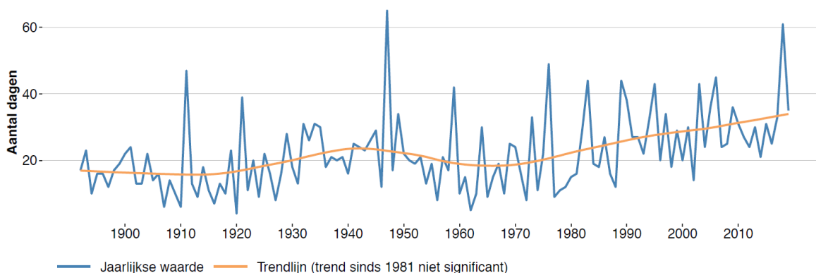
Figuur 2.7 : Jaarlijks aantal zomerdagen in Ukkel tijdens de periode 1892-2019 (Tmax ≥ 25°C)
