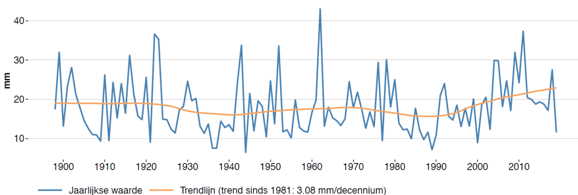
Figuur 2.9 : Jaarlijkse maximale neerslaghoeveelheid gevallen in één uur in Ukkel periode 1898 tot 2019
