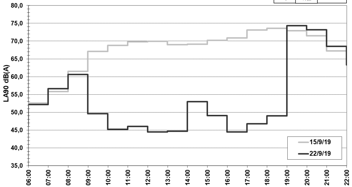
AUD_E411 Bruit de fond en dB(A)
