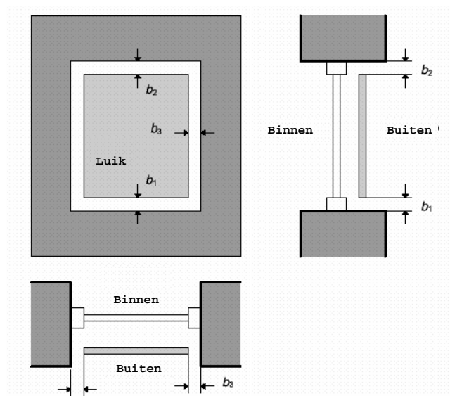
Figuur [19]: Karakteristieken van lichtspleten rond gesloten luiken
