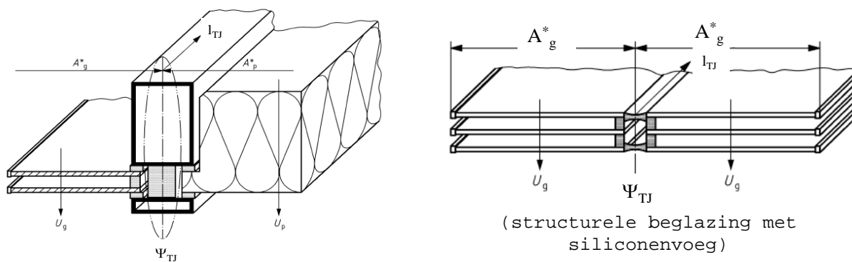
Figuur [28]: Verbindingen beschouwd als lineaire aansluiting
