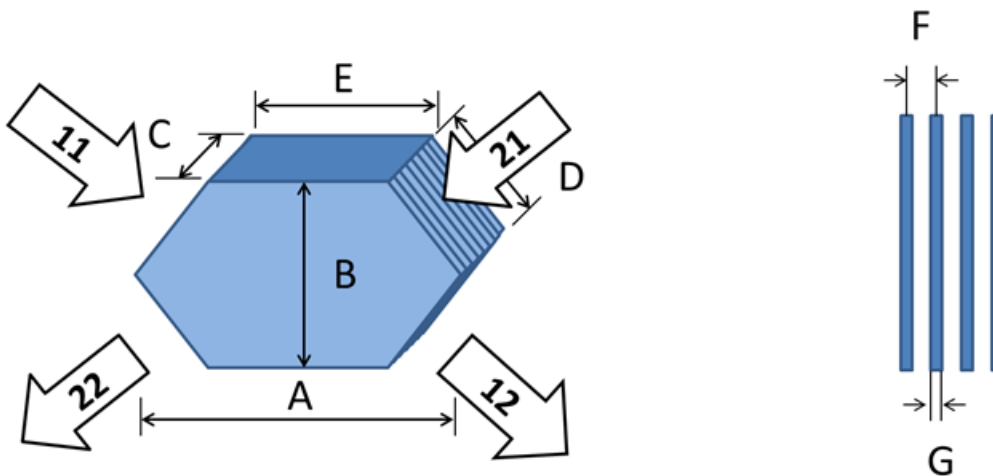
Figuur [6]: Tegenstroomwarmtewisselaar
