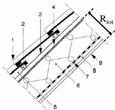
Figuur [50]: Warmteweerstand van een pannen- of leiidak
