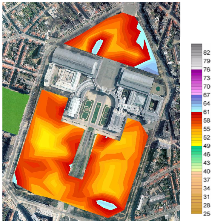
Afbeelding 2: L_{Aeq} -geluidsniveaus dB(A) - 2003. Bron: ACOUSTIC TECHNOLOGIES NV 2003
