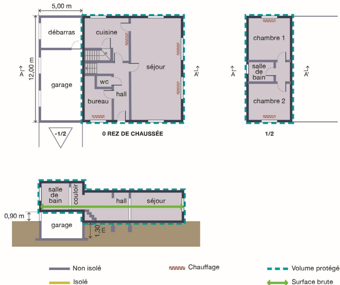
Figure 36 – Plan au sol d'une villa (split-level) avec garage et remise semi-enterrés
