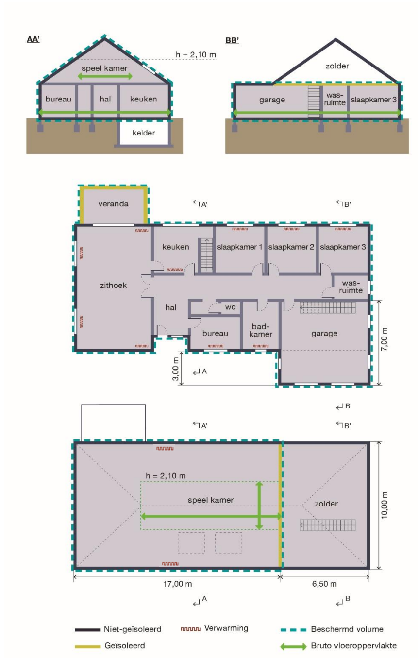
Afbeelding 35 – Boveanzicht van een 4-gevelvilla met speelruimte op de zolder
