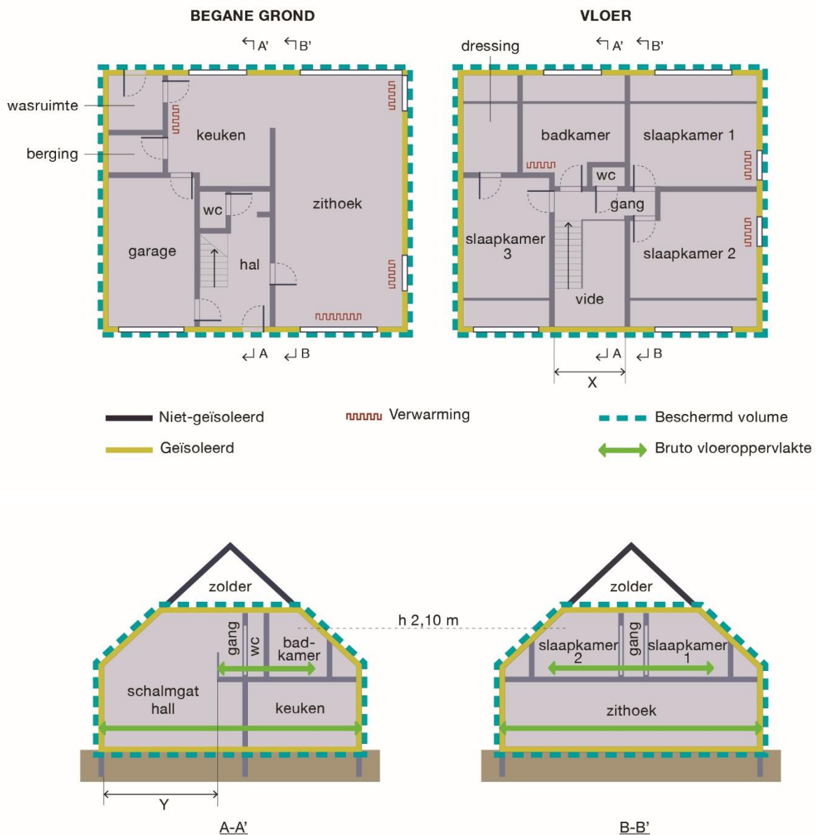
Afbeelding 31 – Boveenaanzicht en doorsnede van een geïsoleerd huis
