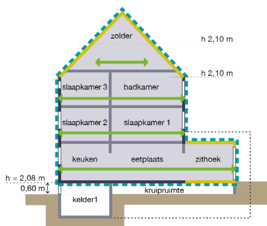
Afbeelding 32 – Bovenaanzicht en doorsnede van een gerenoveerde rijwoning
