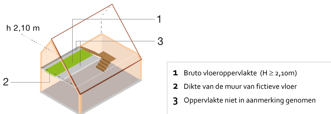
Afbeelding 30 – Bruto vloeroppervlakte van een mezzanine
