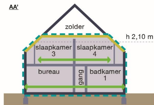
Afbeelding 33 – Bovenanzicht en doorsnede van een villa met 4 gevels
