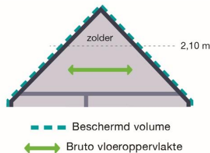
Afbeelding 28 – Bruto vloeroppervlakte onder een hellend dak
