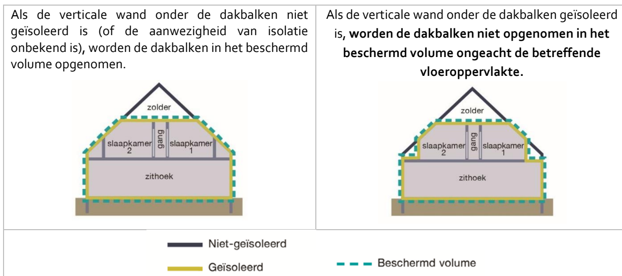
Afbeelding 26 – Dakbalken, nissen
