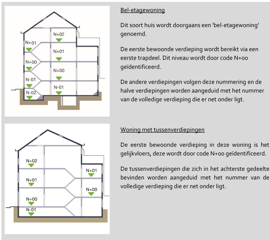
Afbeelding 4 – Appartementscode: beginniveau
