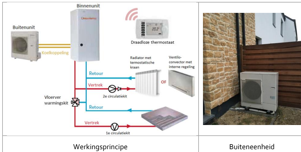
Afbeelding 18 – De (buiten)lucht/water-warmtepomp
