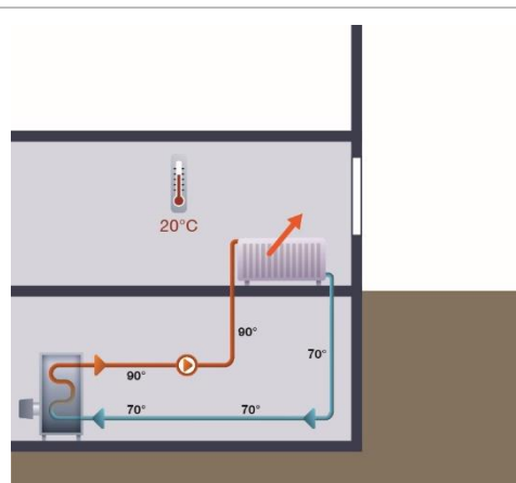
Schema 8 – Schematische weergave van een regeling met constante temperatuur (bron: Energie +)
