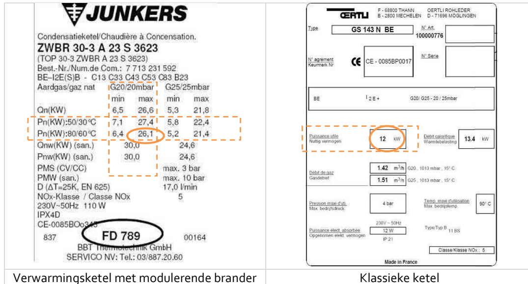
Afbeelding 31 – Vermogensaanduiding op een kenplaat
