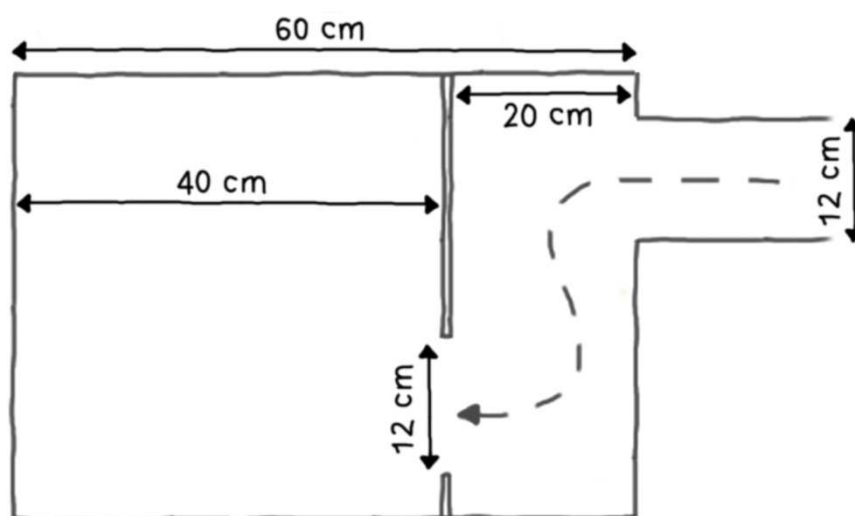
Model met toegangssas - © S. Gérard
