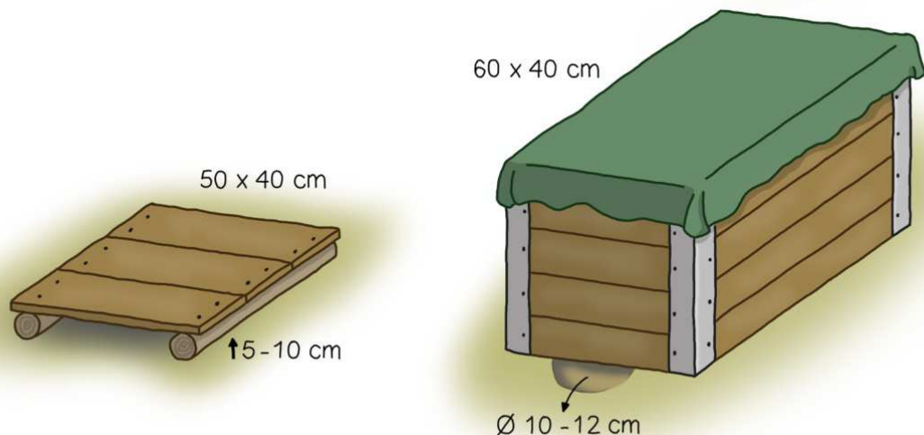
Eenvoudig model: afmetingen van de plankenvloer en de externe bekisting - © S.Gérard
