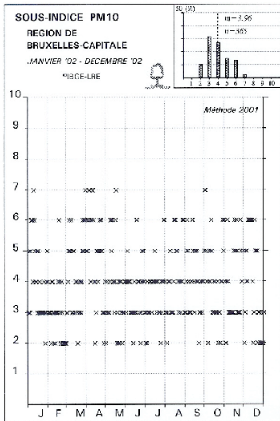
Fig. 5.1: Les sous-indices pour NO 2 , O 3 et PM 10 – Indice général de la qualité de l'air
