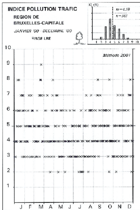
Fig. 5.2: Les sous-indices NO x et CO - Indice trafic
