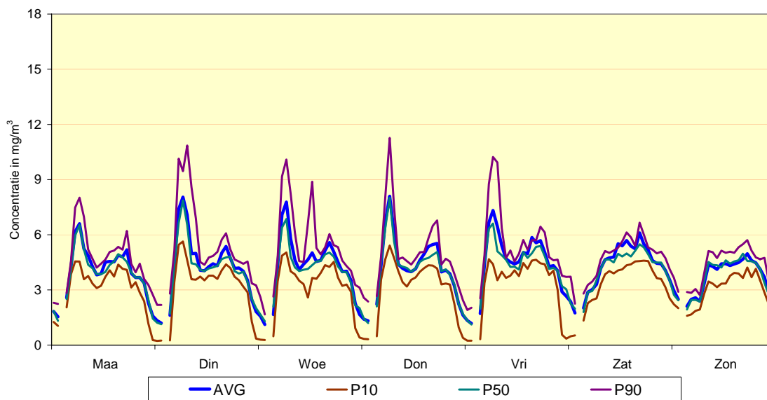
Fig. 23 : Meetpost 41LEC1 (centrum) - Gemiddeld weekverloop voor CO Vergelijking winterperiode 2007 - 2008 en zomerperiode 2007
