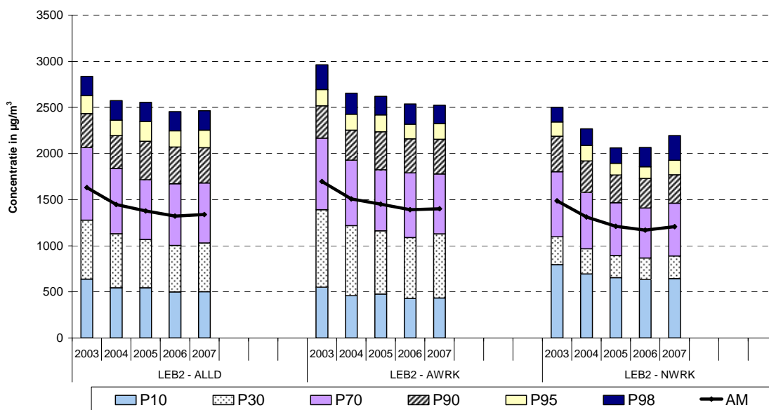
Fig. 7 : NO - Cumulatieve Frequentieverdeling Uurwaarden in beide meetposten van de Leopold II tunnel. Selectie alle dagen , alle werkdagen en alle niet-werkdagen Jaarperiodes 2003 t/m 2007
