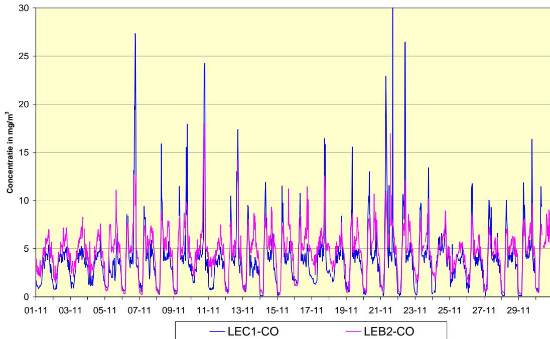
Fig. 3: CO - Evolutie van de uurwaarden en de halfuurswaarden tijdens de maand november 2007 Meetplaats 41LEC1, richting Centrum - Meetplaats 41LEB2, richting Basiliek
