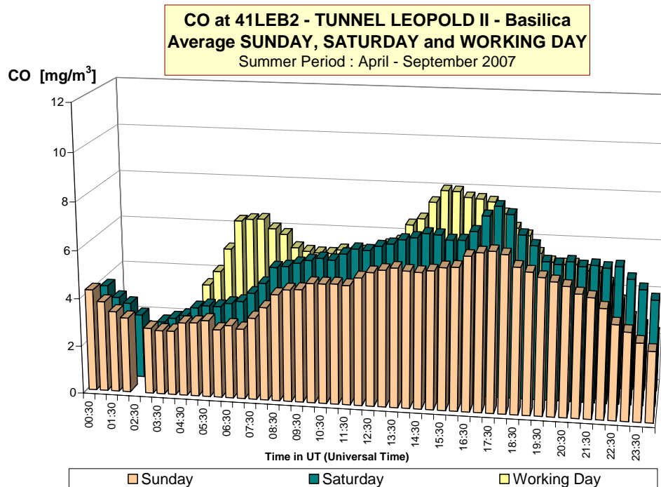
Fig. 20 : CO-dagverloop in de meetpost 41LEB2 (richting basiliek) Vergelijking voor een gemiddelde zondag, zaterdag en werkdag Winterperiode 2007-2008 en zomerperiode 2007
