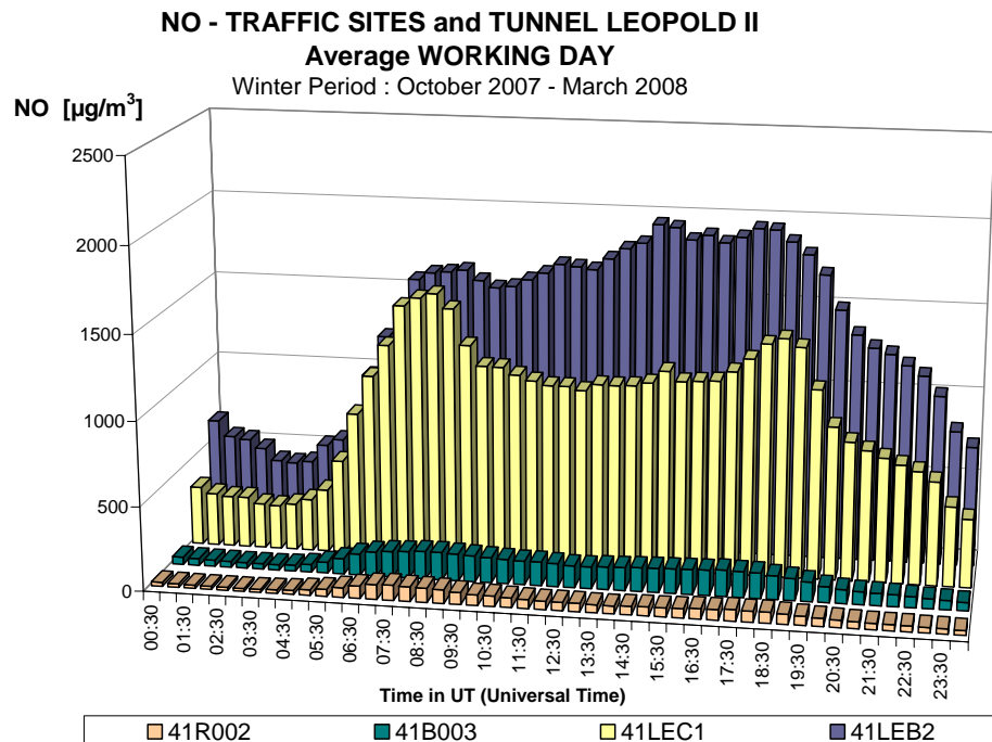
Fig. 34 : Dagverloop NO 2 en NO voor een gemiddelde werkdag tijdens de winter 2007-2008 Meetposten verkeer in de omgevingslucht - Kroonlaan (R002) en Kunst-Wet (B003) Meetposten in de tunnel Leopold II – LEC1 (centrum) en LEC2 (basiliek)
