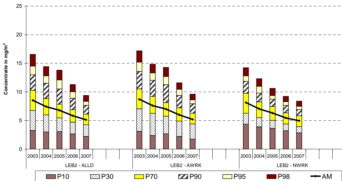
Fig. 6 : CO - Cumulatieve Frequentieverdeling Uurwaarden in beide meetposten van de Leopold II tunnel. Selectie alle dagen , alle werkdagen en alle niet-werkdagen Jaarperiodes 2003 t/m 2007
