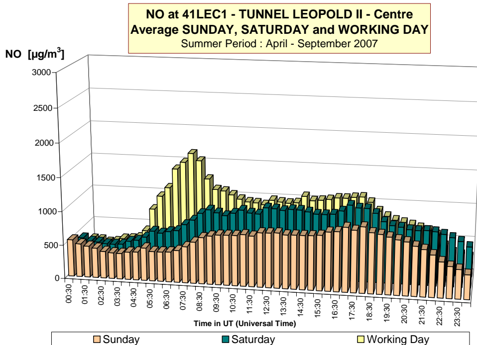
Fig. 17 : NO-dagverloop in de meetpost 41LEC1 (richting centrum) Vergelijking voor een gemiddelde zondag, zaterdag en werkdag Winterperiode 2007-2008 en zomerperiode 2007
