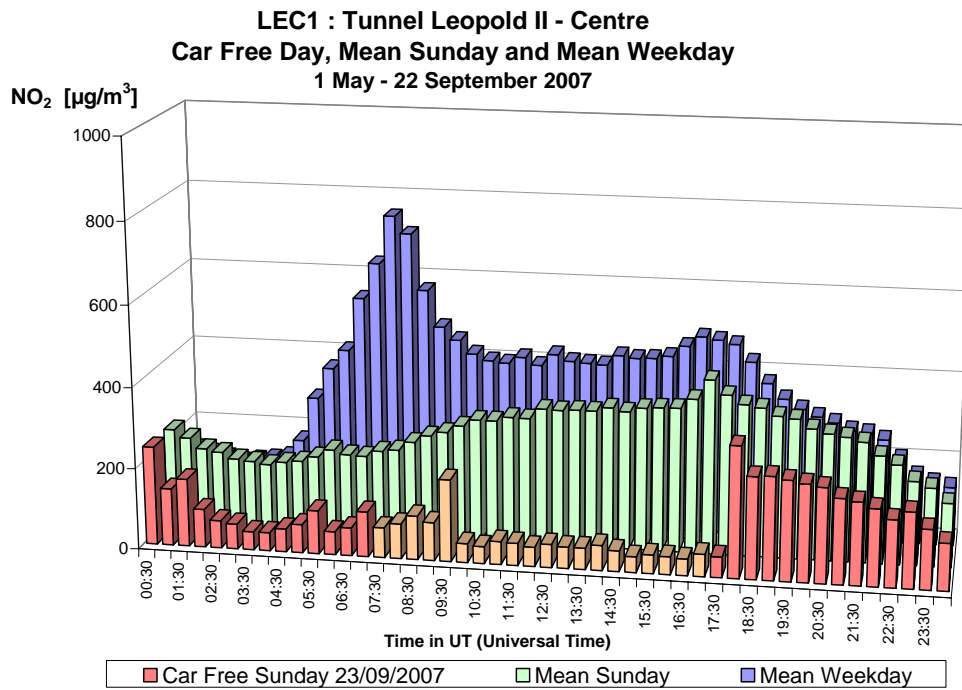
Fig. 27.a : NO 2 in de Leopold II tunnel, richting Centrum – Dagprofiel autoluwe zondag 23-09-2007, gemiddelde zondag en gemiddelde werkdag in de periode 'mei – september 2007'
