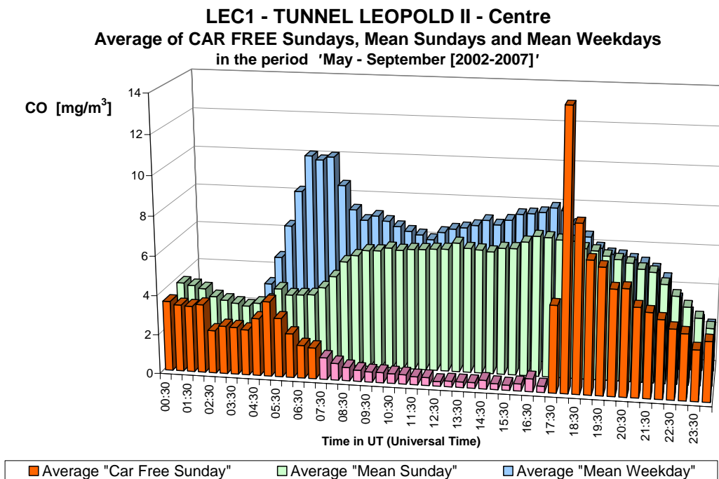
Fig. 31.b : CO in de Leopold II tunnel, richting Centrum – Gemiddelde Dagprofiel van de zes autoluwe zondagen en van alle zondagen en werkdagen in de periodes 'mei – september 2002-2007'
