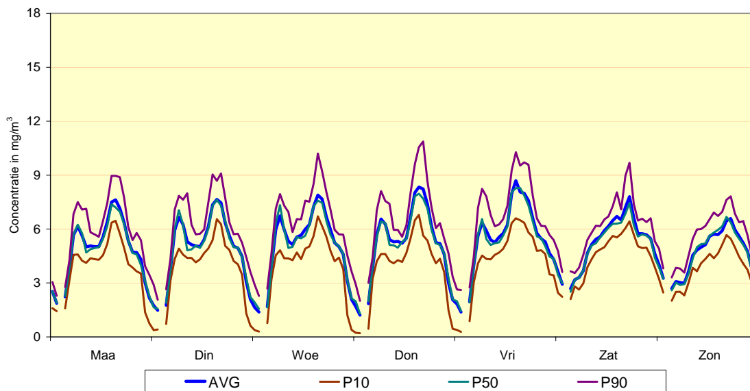
Fig. 24 : Meetpost 41LEB2 (basiliek) - Gemiddeld weekverloop voor CO Vergelijking winterperiode 2007 - 2008 en zomerperiode 2007
