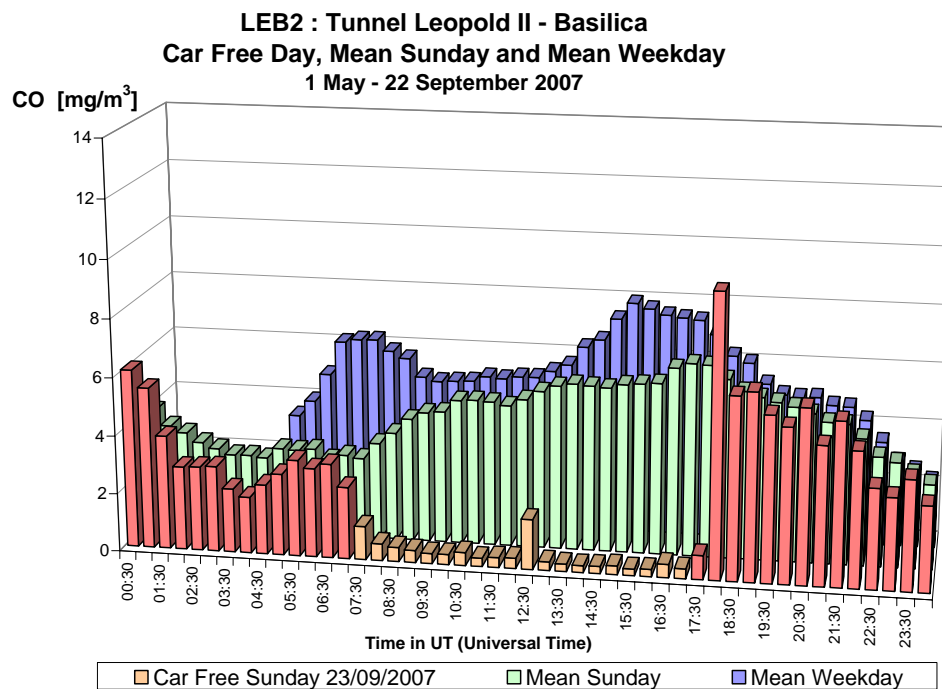
Fig. 32.a : CO in de Leopold II tunnel, richting Basiliek – Dagprofiel autoluwe zondag 23-09-2007, gemiddelde zondag en een gemiddelde werkdag in de periode 'mei – september 2007'
