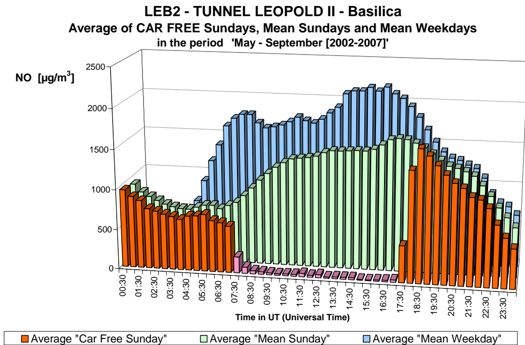
Fig. 30.b : NO in de Leopold II tunnel, richting Basiliek – Gemiddelde Dagprofiel van de zes autoluwe zondagen en van alle zondagen en werkdagen in de periodes 'mei – september 2002-2007'
