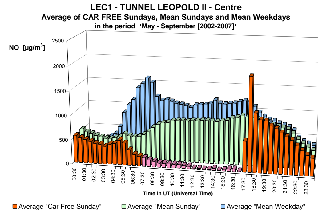
Fig. 29.b : NO in de Leopold II tunnel, richting Centrum – Gemiddelde Dagprofiel van de zes autoluwe zondagen en van alle zondagen en werkdagen in de periodes 'mei – september 2002-2007'
