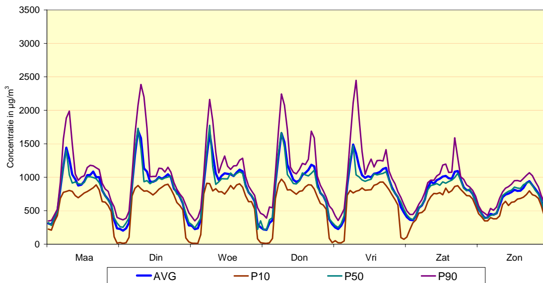
Fig. 25 : Meetpost 41LEC1 (centrum) - Gemiddeld weekverloop voor NO Vergelijking winterperiode 2007 - 2008 en zomerperiode 2007
