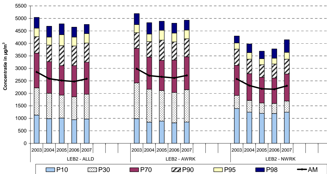
Fig. 8 : NO x - Cumulatieve Frequentieverdeling Uurwaarden in beide meetposten van de Leopold II tunnel. Selectie alle dagen , alle werkdagen en alle niet-werkdagen Jaarperiodes 2003 t/m 2007
