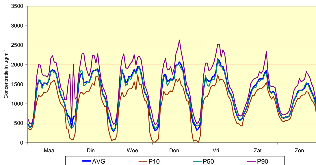
Fig. 26 : Meetpost 41LEB2 (basiliek) - Gemiddeld weekverloop voor NO Vergelijking winterperiode 2007 - 2008 en zomerperiode 2007
