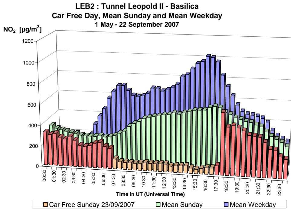
Fig. 28.a : NO 2 in de Leopold II tunnel, richting Basiliek – Dagprofiel autoluwe zondag 23-09-2007, gemiddelde zondag en een gemiddelde werkdag in de periode 'mei – september 2007'
