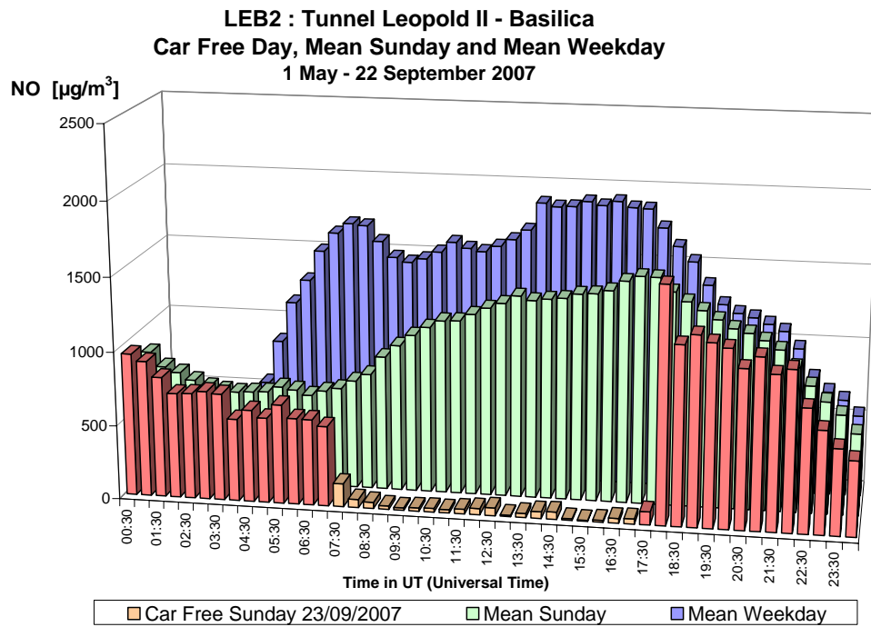
Fig. 30.a : NO in de Leopold II tunnel, richting Basiliek – Dagprofiel autoluwe zondag 23-09-2007, gemiddelde zondag en een gemiddelde werkdag in de periode 'mei – september 2007'
