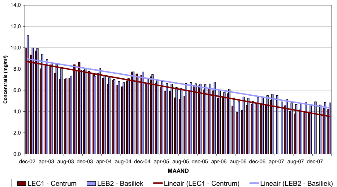
Fig. 10 : NO x en CO - Evolutie maandgemiddelde concentratie in beide meetposten van de Leopold II tunnel. Periode "December 2002 – Maart 2008"
