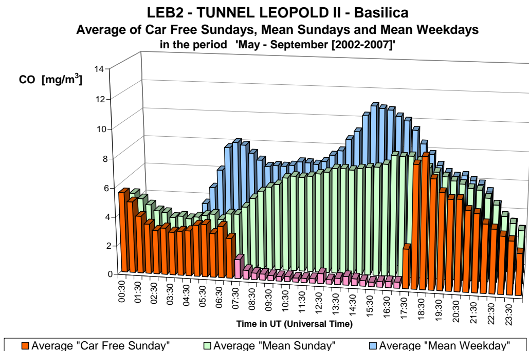
Fig. 32.b : CO in de Leopold II tunnel, richting Basiliek – Gemiddelde Dagprofiel van de vijf autoluwe zondagen en van alle zondagen en werkdagen in de periodes 'mei – september 2002-2007'
