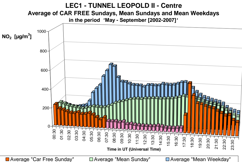
Fig. 27.b : NO 2 in de Leopold II tunnel, richting Centrum – Gemiddelde Dagprofiel van de zes autoluwe zondagen en van alle zondagen en werkdagen in de periodes 'mei – september 2002-2007'
