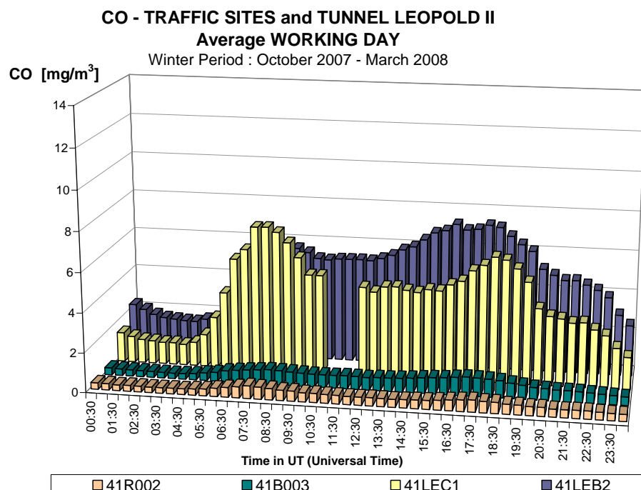
Fig. 33 : CO-dagverloop voor een gemiddelde werkdag tijdens de winter 2007-2008 Meetposten verkeer in de omgevingslucht - Kroonlaan (R002) en Kunst-Wet (B003) Meetposten in de tunnel Leopold II – LEC1 (centrum) en LEC2 (basiliek)
