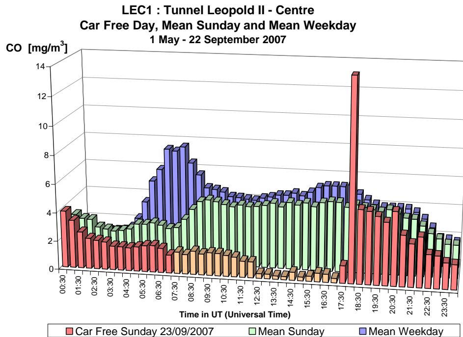
Fig. 31.a : CO in de Leopold II tunnel, richting Centrum – Dagprofiel autoluwe zondag 23-09-2007, gemiddelde zondag en gemiddelde werkdag in de periode 'mei – september 2007'
