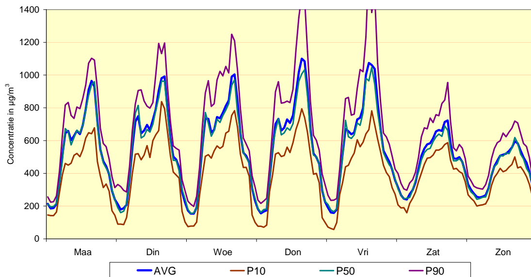
Fig. 22 : Meetpost 41LEB2 (basiliek) - Gemiddeld weekverloop voor NO 2 Vergelijking winterperiode 2007 - 2008 en zomerperiode 2007
