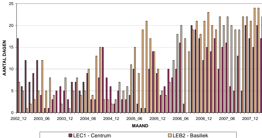
Fig. 13 : NO 2 – Halfuurswaarden > 850 µg/m 3 . Totaal aantal overschrijdingen per maand en aantal dagen per maand met overschrijding (december 2002 – maart 2008)
