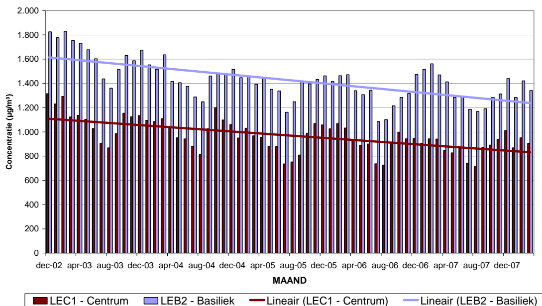
Fig. 9 : NO 2 en NO - Evolutie maandgemiddelde concentratie in beide meetposten van de Leopold II tunnel. Periode "December 2002 – Maart 2008"
