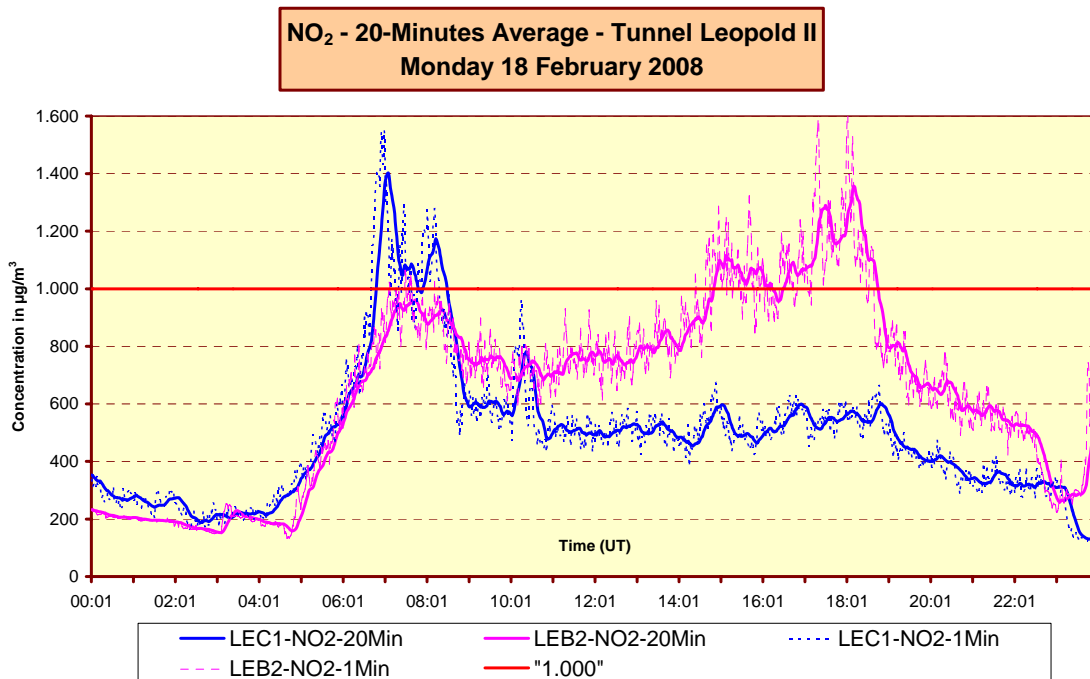
Fig. 4: NO 2 - evolutie minuutwaarden en voortschrijdend 20-minuutsgemiddelde in beide meetposten van de Leopold II tunnel Dinsdag 22 januari en maandag 18 februari 2008
