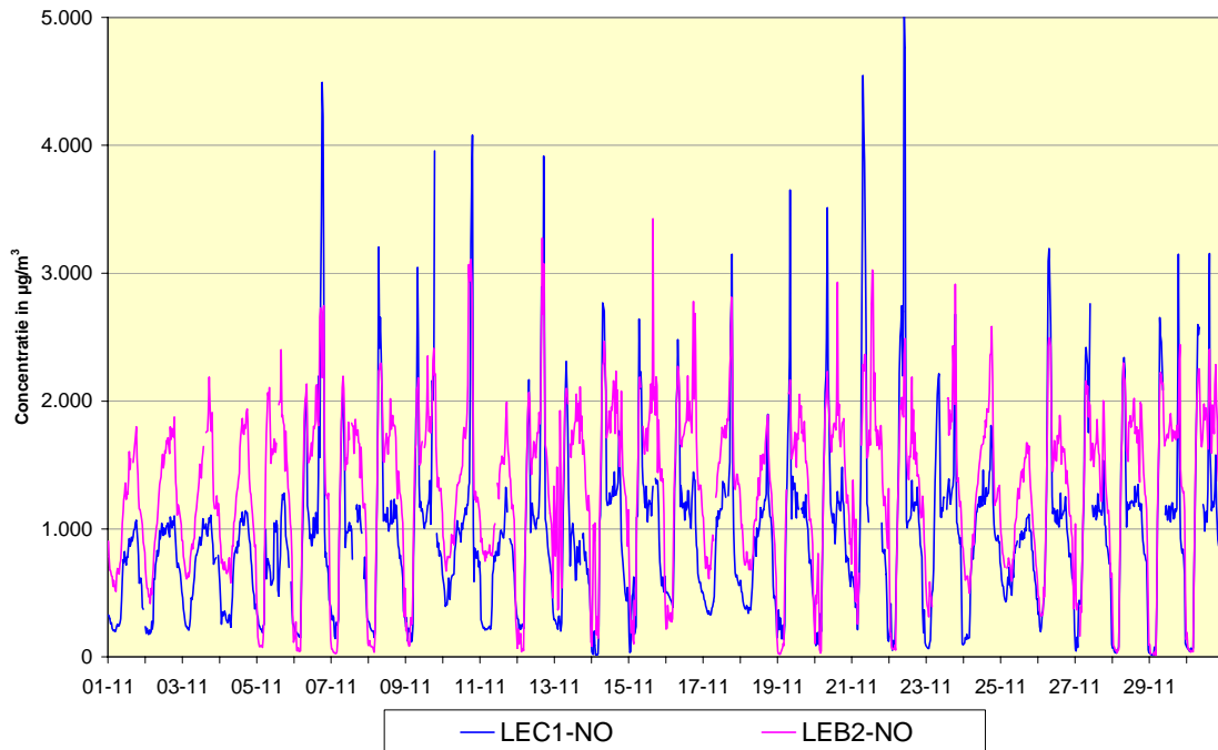
Fig. 2: NO - Evolutie van de uurwaarden en de halfuurswaarden tijdens de maand november 2007 Meetplaats 41LEC1, richting Centrum - Meetplaats 41LEB2, richting Basiliek
