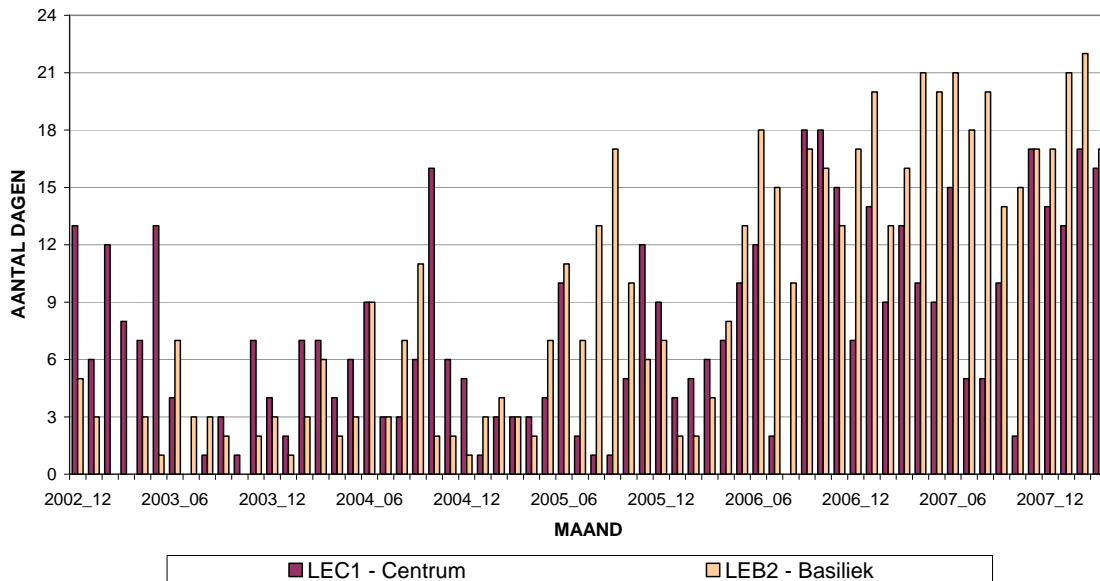
Fig. 12 : NO 2 – 20-Minuutsgemiddelden > 1.000 µg/m 3 . Totaal aantal overschrijdingen per maand en aantal dagen per maand met overschrijding (december 2002 – maart 2008)
