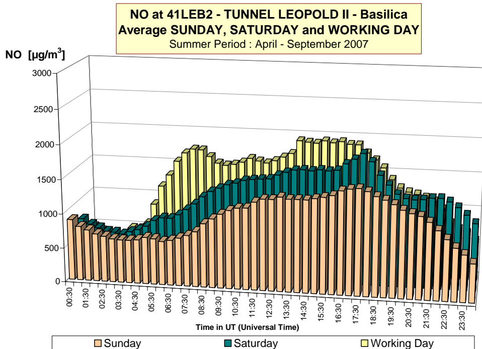
Fig. 18 : NO-dagverloop in de meetpost 41LEB2 (richting basiliek) Vergelijking voor een gemiddelde zondag, zaterdag en werkdag Winterperiode 2007-2008 en zomerperiode 2007
