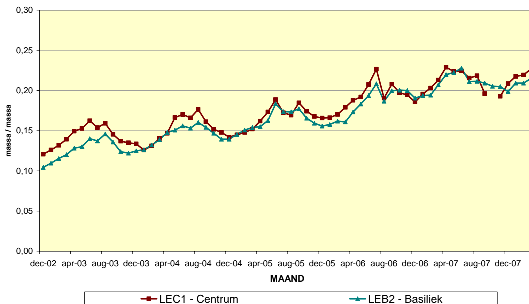
Fig. 11 : Evolutive van de verhouding NO 2 /NO x in beide meetposten van de Leopold II tunnel. Periode "December 2002 – Maart 2008"
