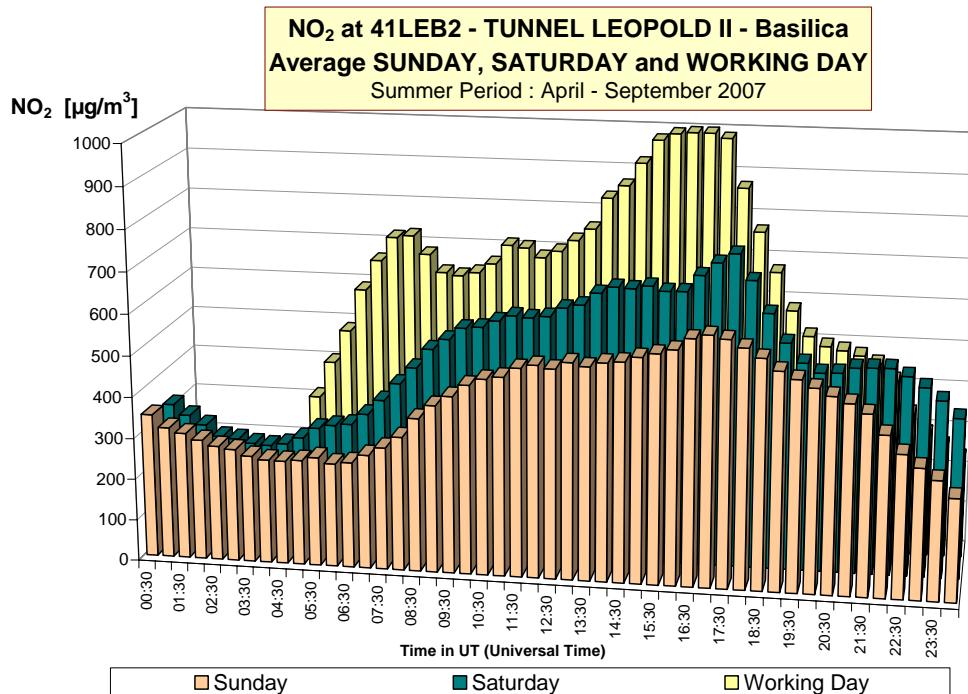
Fig. 16 : NO 2 -dagverloop in de meetpost 41LEB2 (richting basiliek) Vergelijking voor een gemiddelde zondag, zaterdag en werkdag Winterperiode 2007-2008 en zomerperiode 2007
