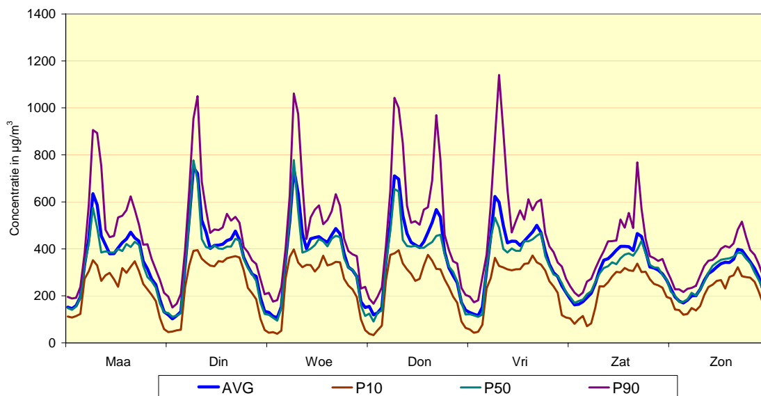
Fig. 21 : Meetpost 41LEC1 (centrum) - Gemiddeld weekverloop voor NO 2 Vergelijking winterperiode 2007 - 2008 en zomerperiode 2007
