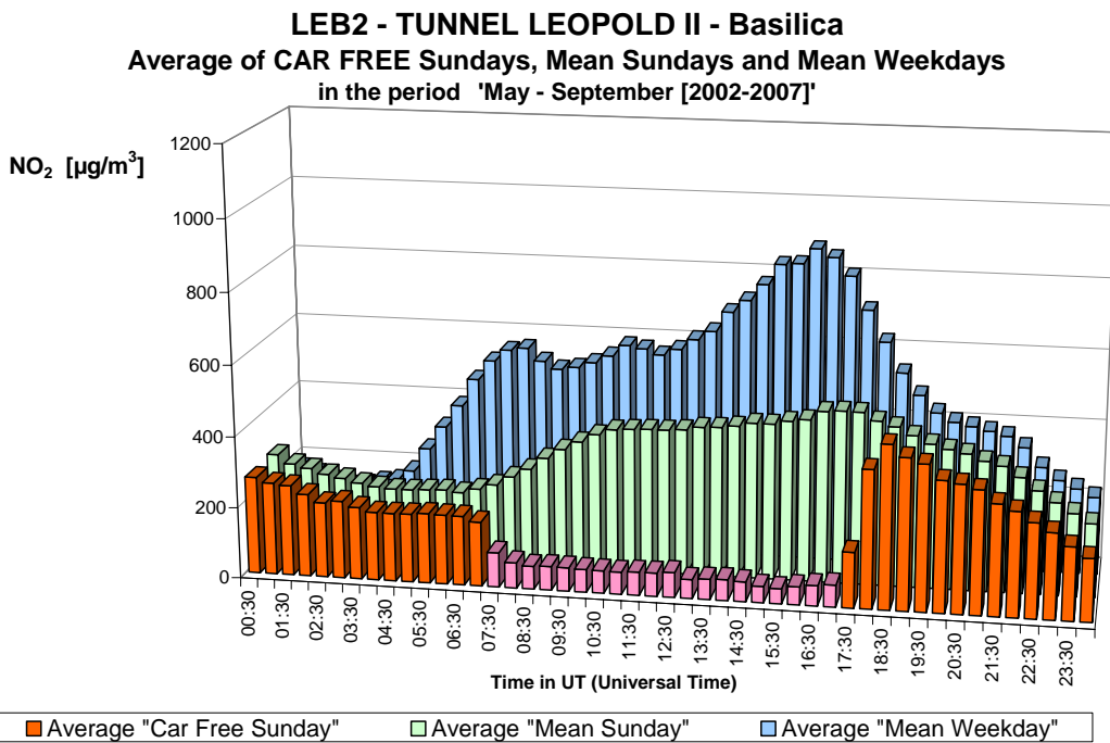
Fig. 28.b : NO 2 in de Leopold II tunnel, richting Basiliek – Gemiddelde Dagprofiel van de zes autoluwe zondagen en van alle zondagen en werkdagen in de periodes 'mei – september 2002-2007'
