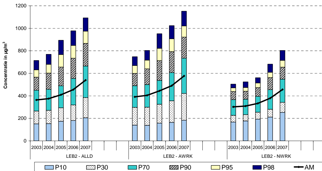
Fig. 5 : NO 2 - Cumulatieve Frequentieverdeling Uurwaarden in beide meetposten van de Leopold II tunnel. Selectie alle dagen , alle werkdagen en alle niet-werkdagen Jaarperiodes 2003 t/m 2007
