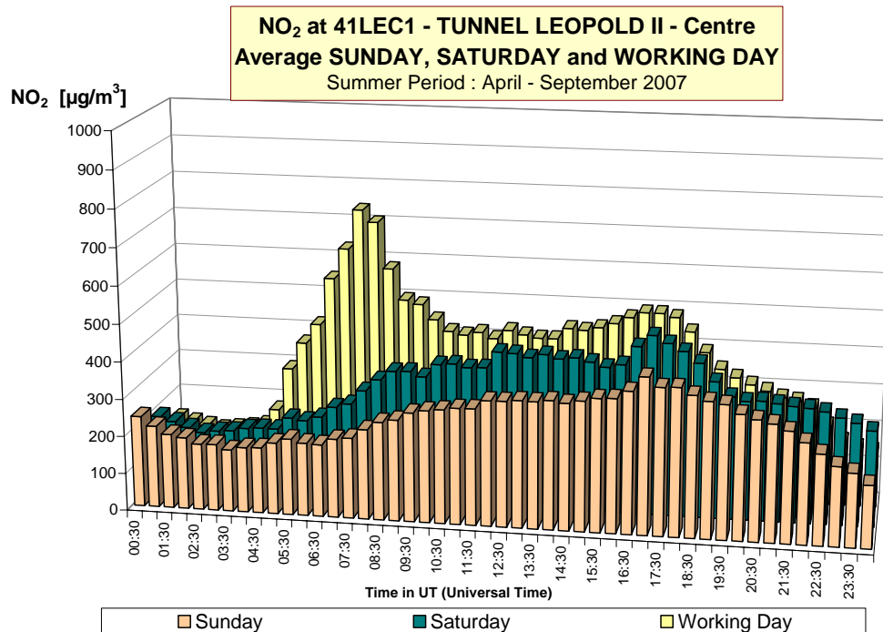
Fig. 15 : NO 2 -dagverloop in de meetpost 41LEC1 (richting centrum) Vergelijking voor een gemiddelde zondag, zaterdag en werkdag Winterperiode 2007-2008 en zomerperiode 2007
