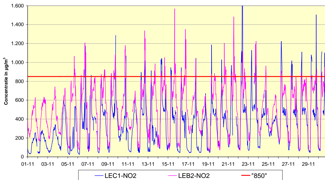
Fig. 1: NO 2 - Evolutie van de uurwaarden en de halfuurswaarden tijdens de maand november 2007 Meetplaats 41LEC1, richting Centrum - Meetplaats 41LEB2, richting Basiliek
