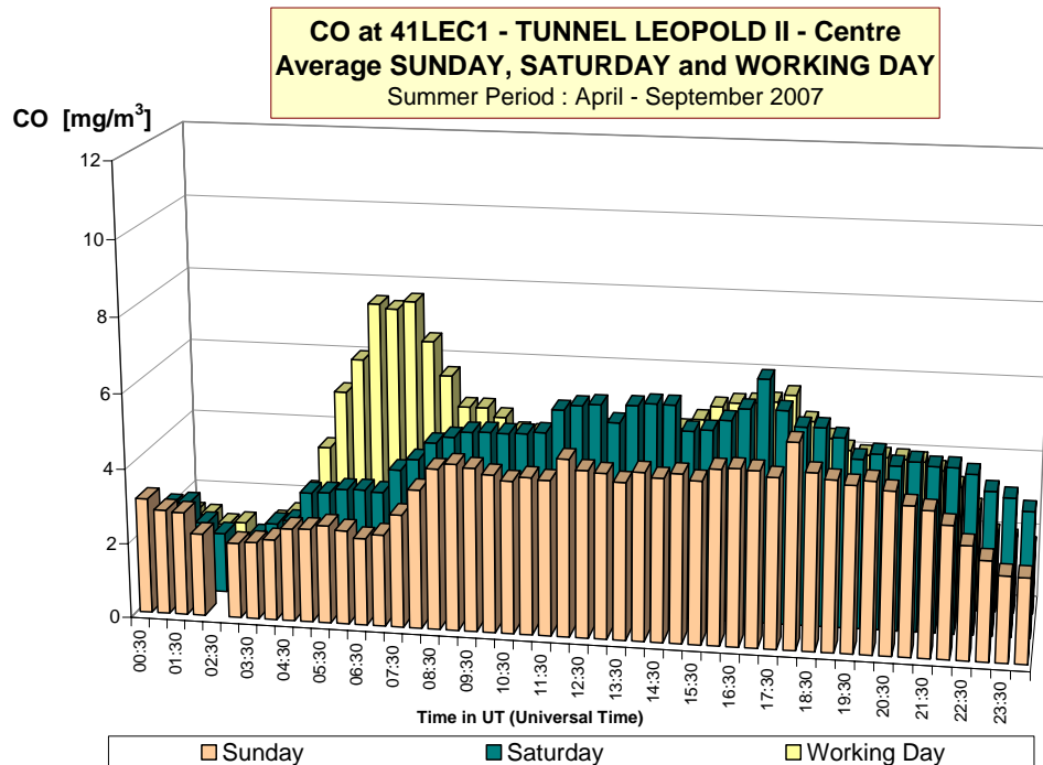
Fig. 19 : CO-dagverloop in de meetpost 41LEC1 (richting centrum) Vergelijking voor een gemiddelde zondag, zaterdag en werkdag Winterperiode 2007-2008 en zomerperiode 2007
