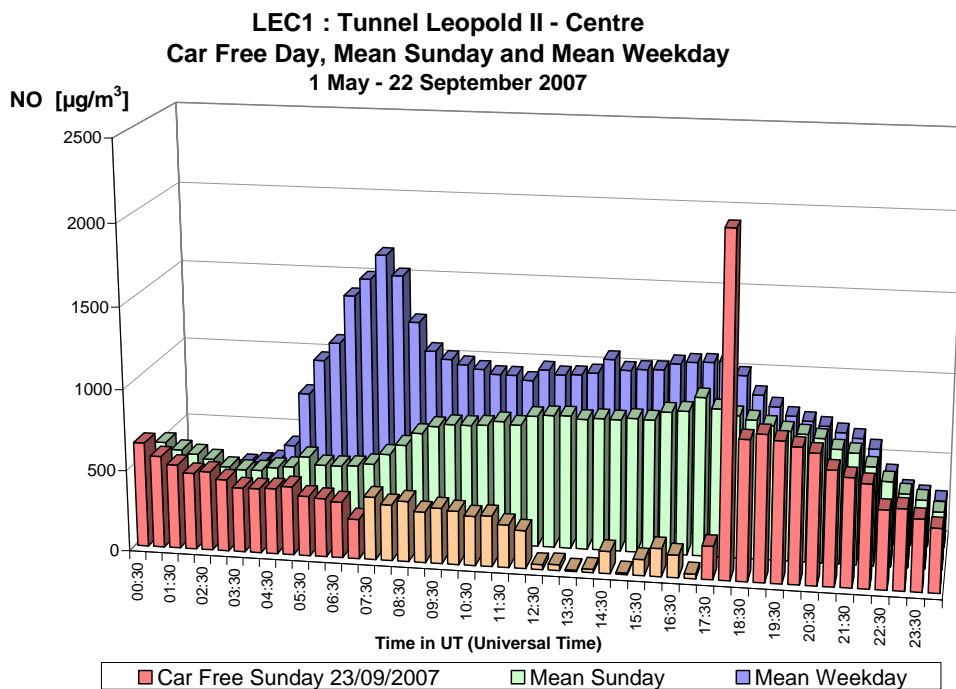
Fig. 29.a : NO in de Leopold II tunnel, richting Centrum – Dagprofiel autoluwe zondag 23-09-2007, gemiddelde zondag en gemiddelde werkdag in de periode 'mei – september 2007'
