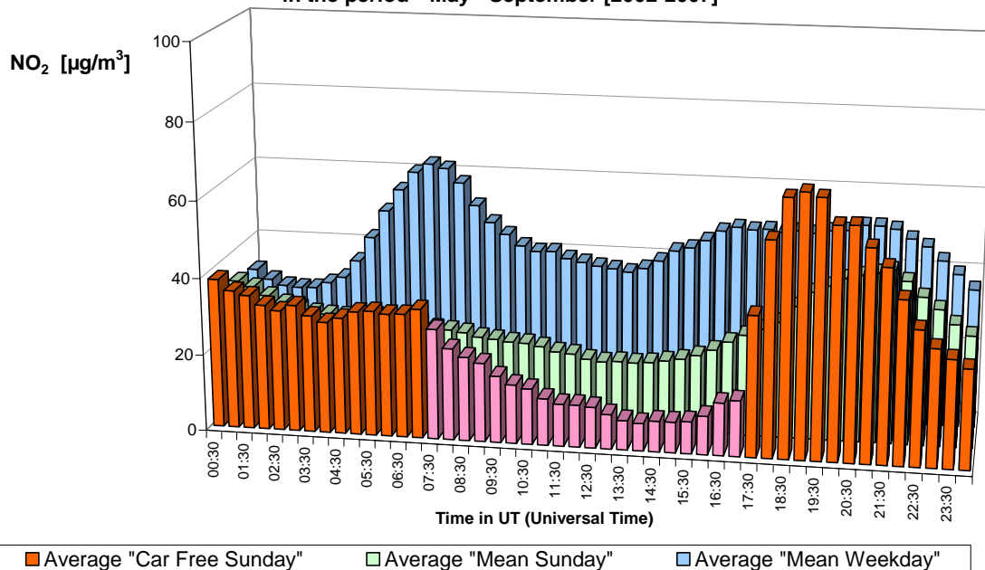
Fig. 16.b : NO 2 à Woluwé – Profil journalier sur les six dimanches sans voiture et sur tous les dimanches et jours ouvrables des périodes 'mai – septembre 2002-2007'.
