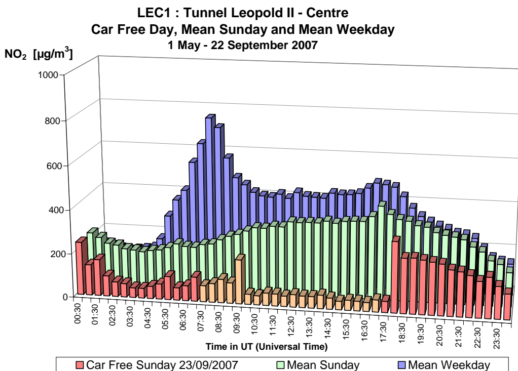
Fig. 2.a : NO 2 dans le tunnel Léopold II, direction Centre – Profil journalier du dimanche sans voiture 23-09-2007, d'un dimanche moyen et d'un jour ouvrable moyen de la période 'mai – septembre 2007'.
