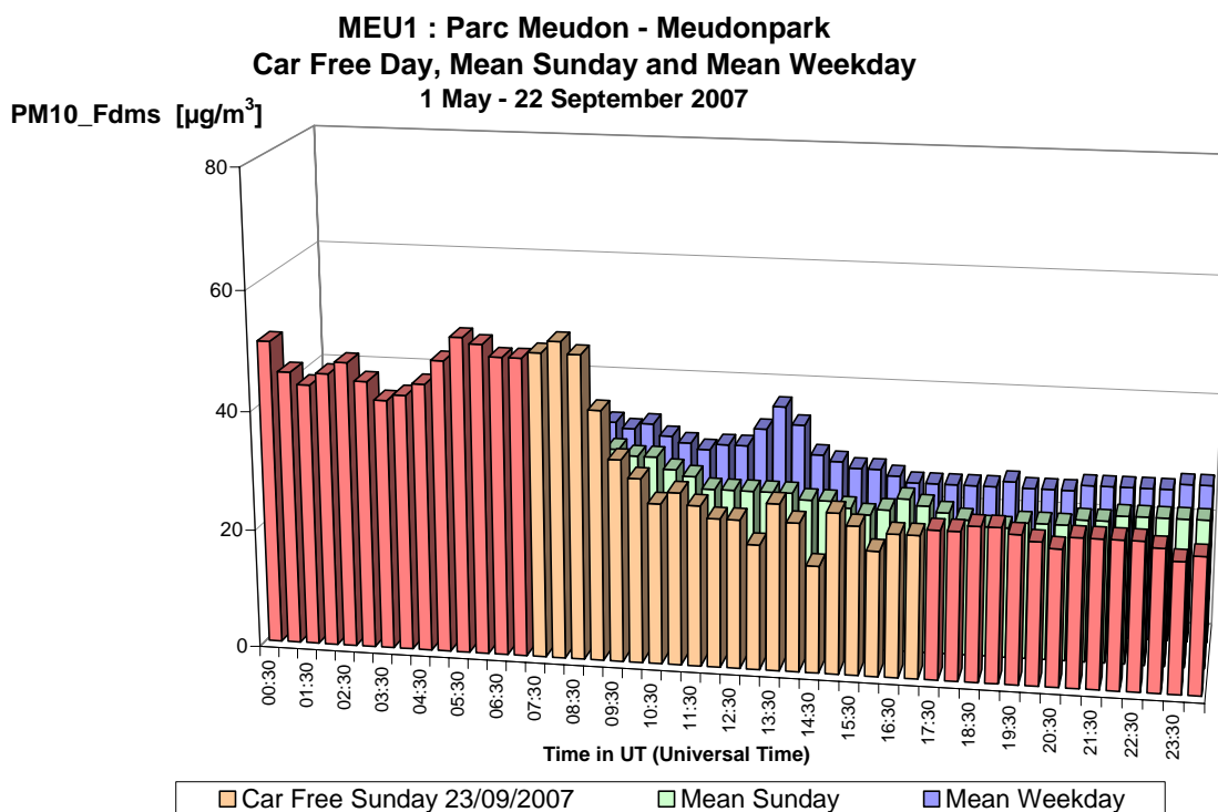
Fig. 34.a : PM10 au Parc Meudon – Profil journalier du dimanche sans voiture 23-09-2007, d'un dimanche moyen et d'un jour ouvrable moyen de la période 'mai – septembre 2007'
