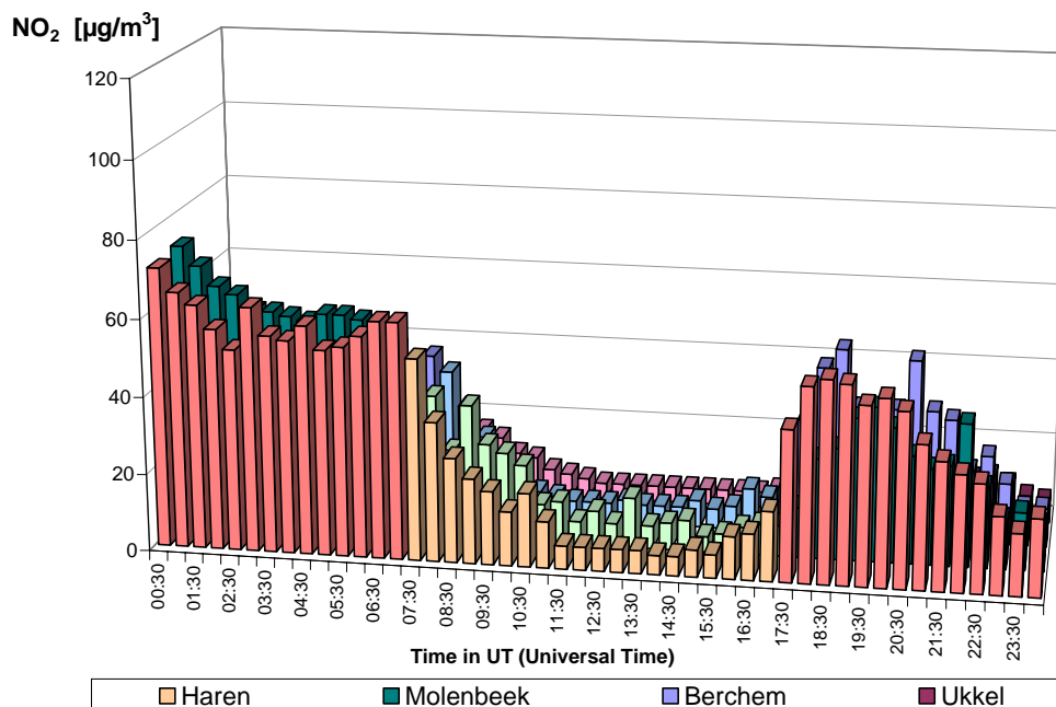
Fig. 22.b: Dimanche sans voiture 23 septembre 2007 – Profil journalier complémentaire en NO 2 Situation à 4 endroits différents : Haren, Molenbeek, Berchem et Uccle
