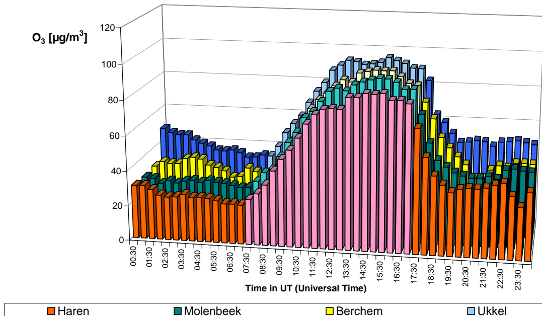
Fig. 23.a: Moyenne sur les six dimanches sans voiture – Profil journalier en O 3 Situation à 4 endroits différents : Haren, Molenbeek, Berchem et Uccle
