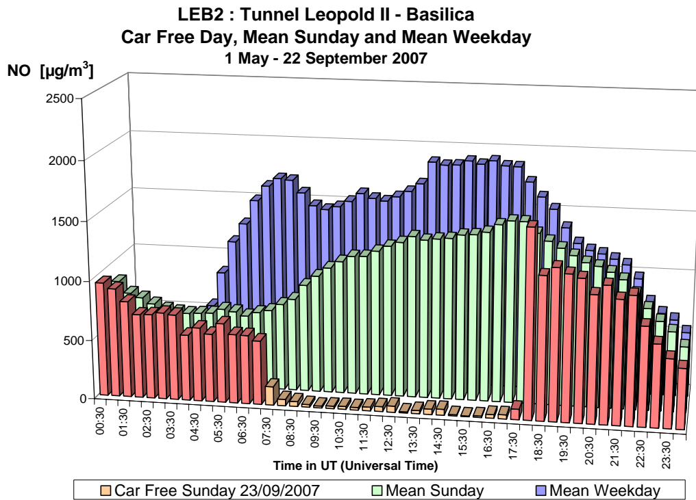
Fig. 5.a : NO dans le tunnel Léopold II, direction Basilique – Profil journalier du dimanche sans voiture 23-09-2007, d'un dimanche moyen et d'un jour ouvrable moyen de la période 'mai – septembre 2007'.
