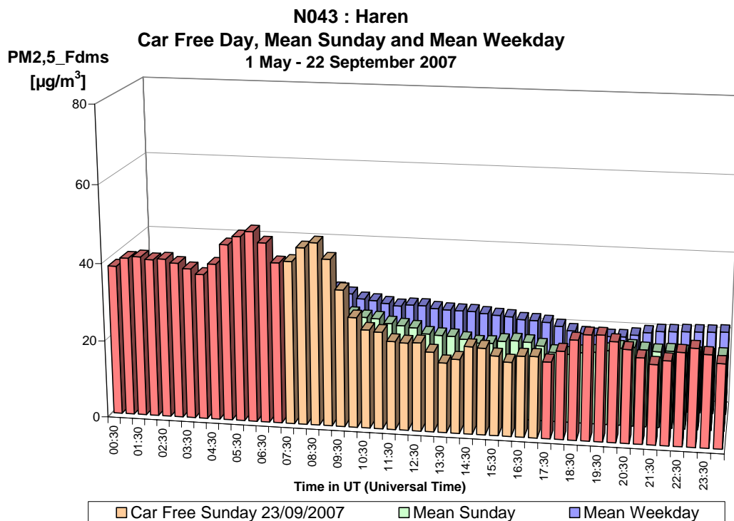
Fig. 38 : PM 2,5 à Haren – Profil journalier du dimanche sans voiture 23-09-2007, d'un dimanche moyen et d'un jour ouvrable moyen de la période 'mai – septembre 2007'
