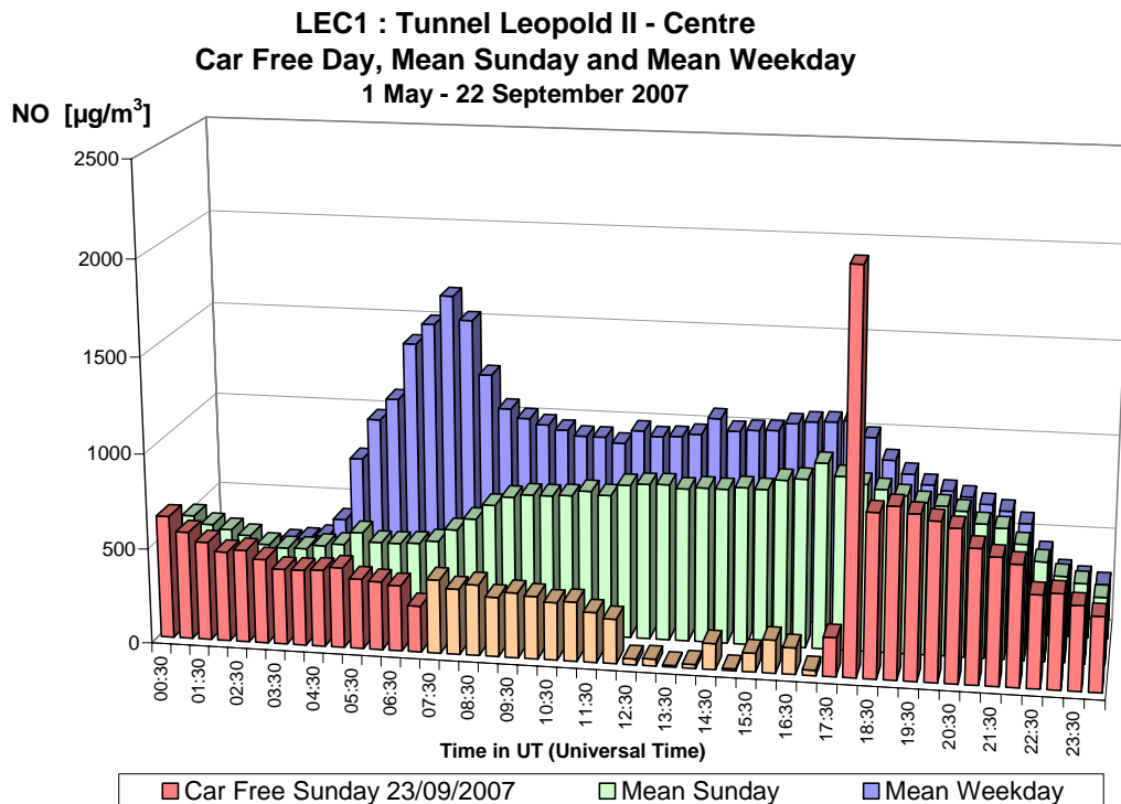
Fig. 1.a : NO dans le tunnel Léopold II, direction Centre – Profil journalier du dimanche sans voiture 23-09-2007, d'un dimanche moyen et d'un jour ouvrable moyen de la période 'mai – septembre 2007'.
