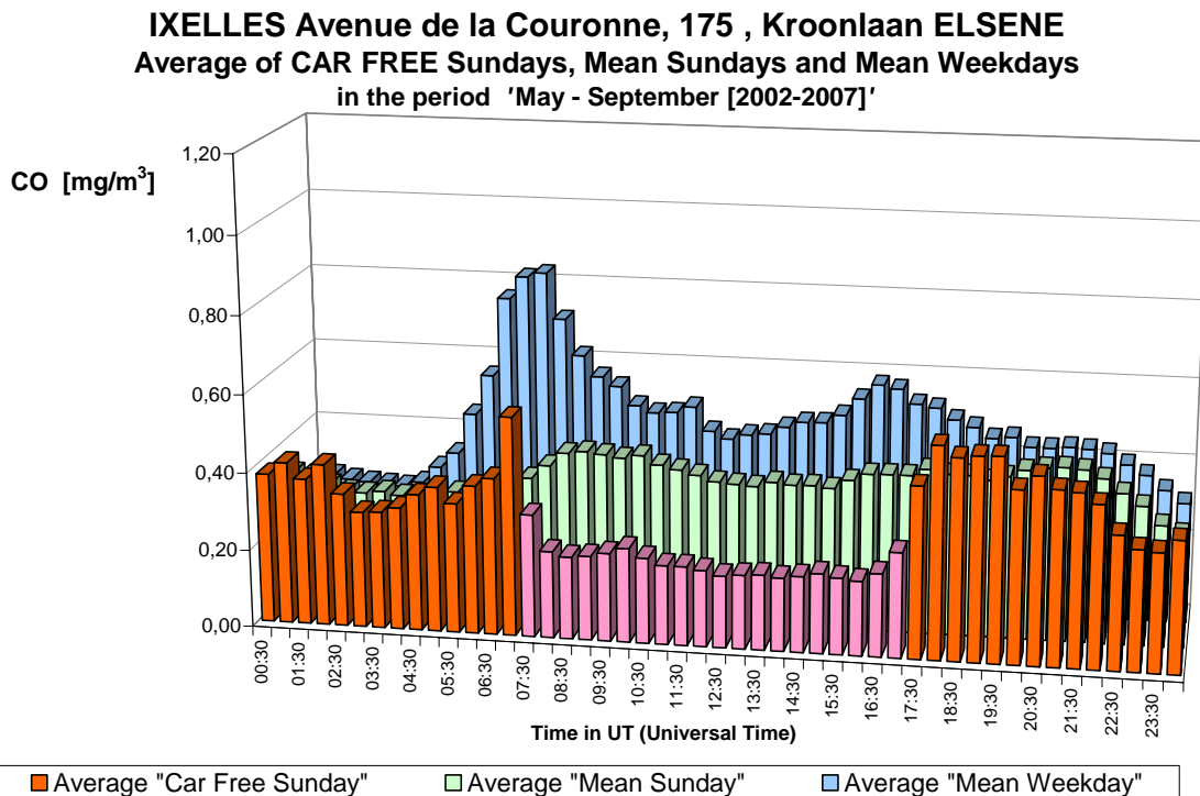
Fig. 25.b : CO à Ixelles (Av. de la Couronne) – Profil journalier sur les six dimanches sans voiture et sur tous les dimanches et jours ouvrables des périodes 'mai – septembre 2002-2007'.
