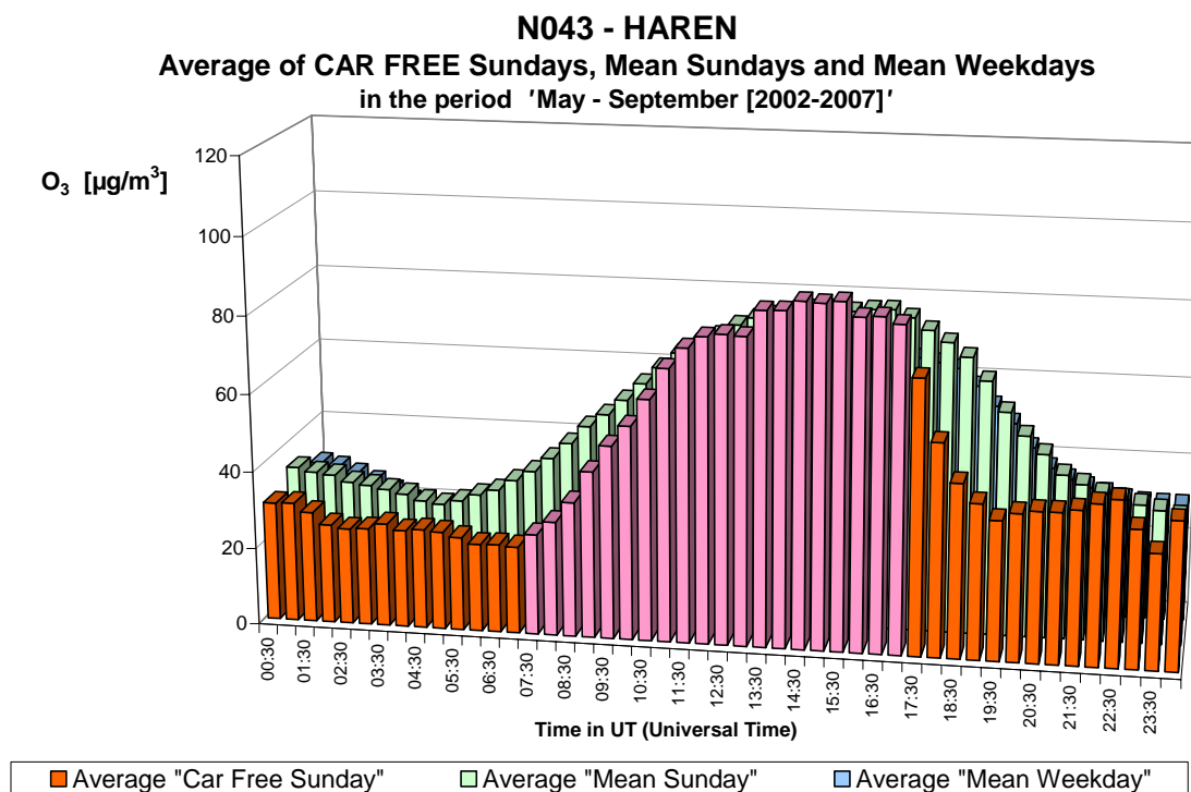
Fig. 21.b : O 3 à Berchem – Profil journalier sur les six dimanches sans voiture et sur tous les dimanches et jours ouvrables des périodes 'mai – septembre 2002-2007'.
