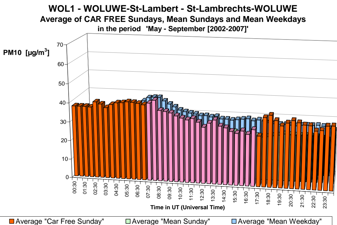
Fig. 35.b : PM10 à Woluwé-St-Lambert – Profil journalier sur les six dimanches sans voiture et sur tous les dimanches et jours ouvrables des périodes 'mai – septembre 2002-2007'.
