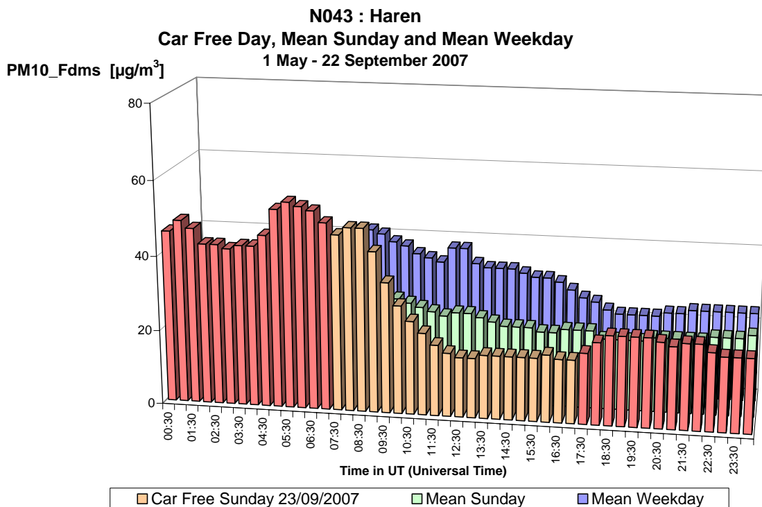
Fig. 33.a : PM10 à Haren – Profil journalier du dimanche sans voiture 23-09-2007, d'un dimanche moyen et d'un jour ouvrable moyen de la période 'mai – septembre 2007'
