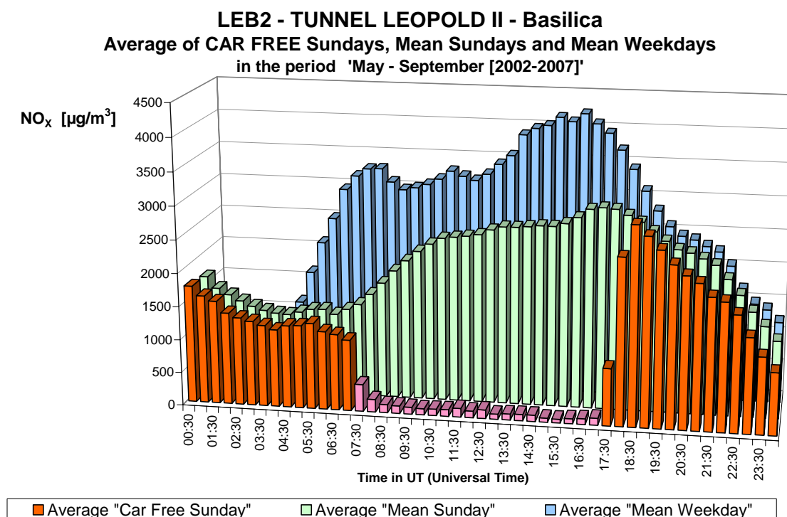
Fig. 7.b : NO x dans le tunnel Léopold II, direction Basilique – Profil journalier sur les six dimanches sans voiture et sur tous les dimanches et jours ouvrables des périodes 'mai – septembre 2002-2007'.
