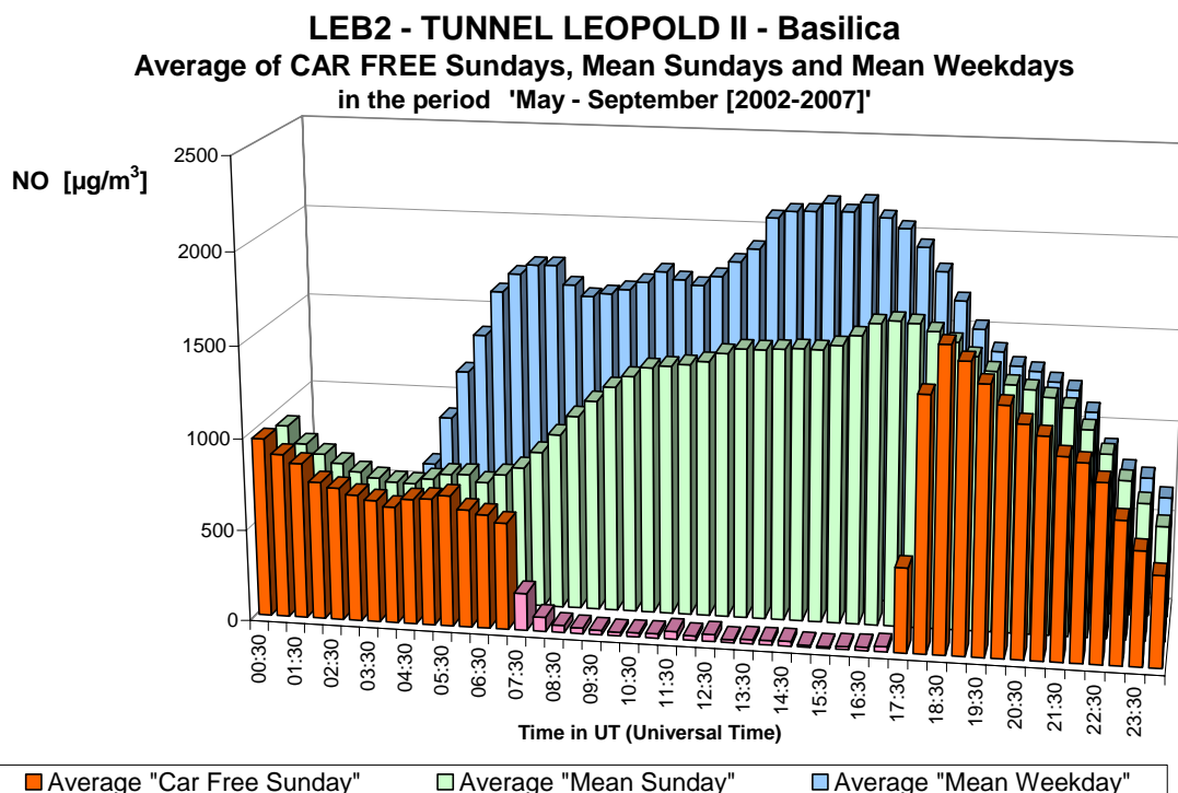
Fig. 5.b : NO dans le tunnel Léopold II, direction Basilique – Profil journalier sur les six dimanches sans voiture et sur tous les dimanches et jours ouvrables des périodes 'mai – septembre 2002-2007'.
