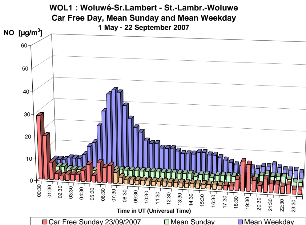
Fig. 15.a : NO à Woluwé – Profil journalier du dimanche sans voiture 23-09-2007, d'un dimanche moyen et d'un jour ouvrable moyen de la période 'mai – septembre 2007'.
