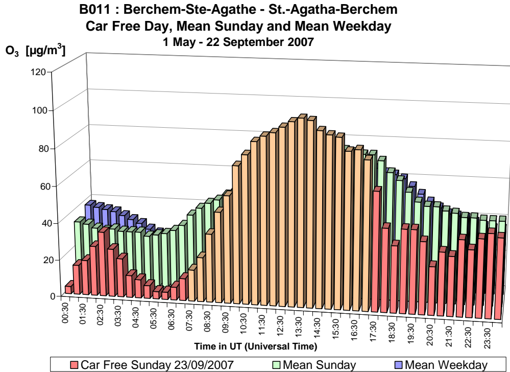
Fig. 20.a : O 3 à Berchem – Profil journalier du dimanche sans voiture 23-09-2007, d'un dimanche moyen et d'un jour ouvrable moyen de la période 'mai – septembre 2007'.
