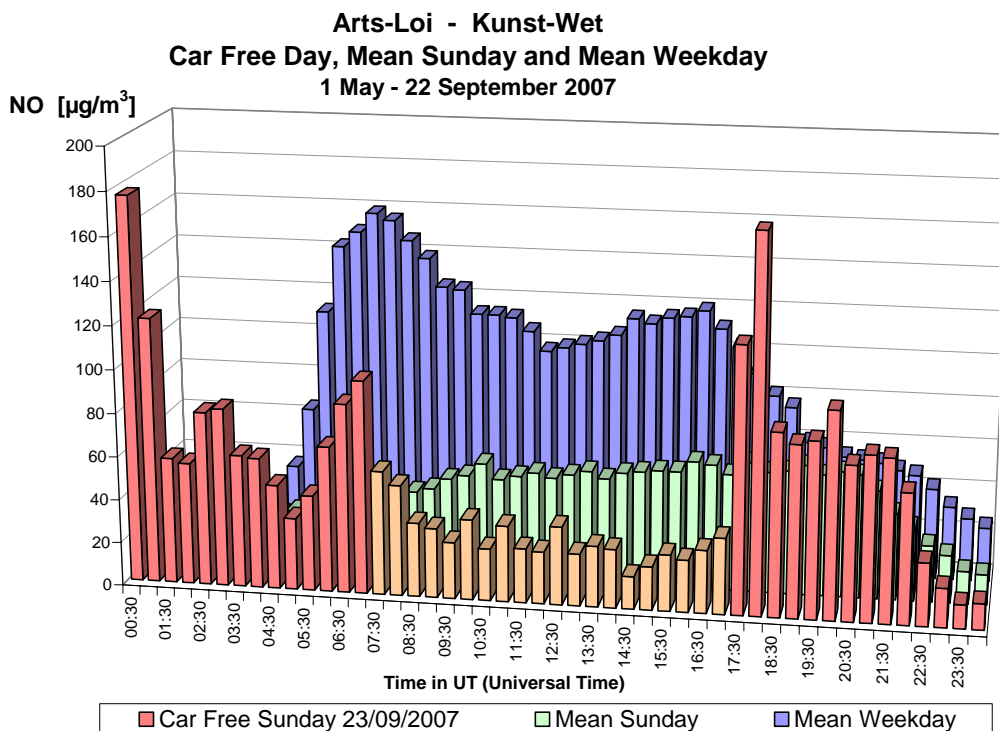
Fig. 9.a : NO au poste de mesure Arts-Loi – Profil journalier du dimanche sans voiture 23-09-2007, d'un dimanche moyen et d'un jour ouvrable moyen de la période 'mai – septembre 2007'.
