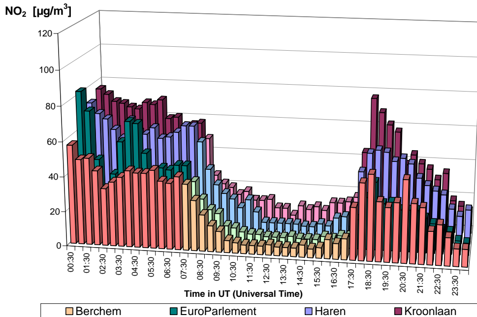
Fig. 17.a : Dimanche sans voiture du 23-09-2007 – Comparaison du profil journalier en NO 2 à 4 endroits différents – Berchem, Parlement européen, Haren et Av. de la Couronne à Ixelles
