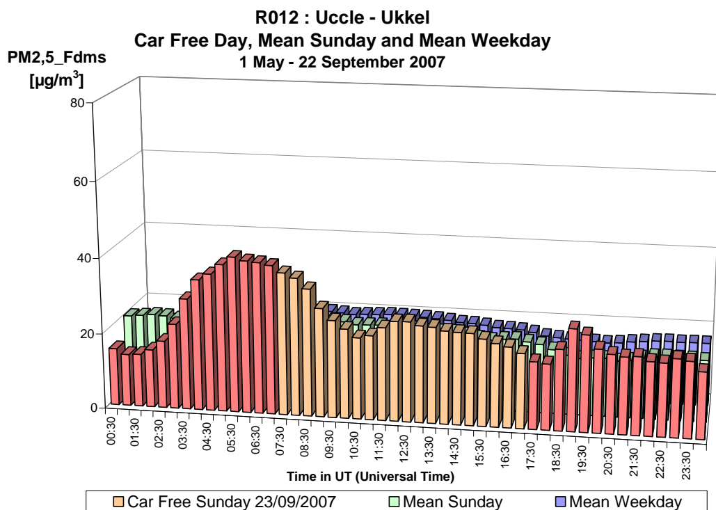
Fig. 37 : PM 2,5 à Uccle – Profil journalier du dimanche sans voiture 23-09-2007, d'un dimanche moyen et d'un jour ouvrable moyen de la période 'mai – septembre 2007'
