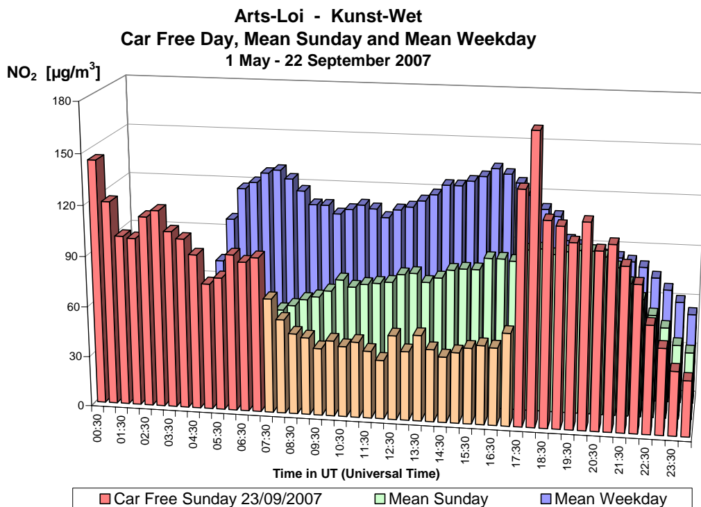
Fig. 10.a : NO 2 au poste de mesure Arts-Loi – Profil journalier du dimanche sans voiture 23-09-2007, d'un dimanche moyen et d'un jour ouvrable moyen de la période mai – septembre 2007.
