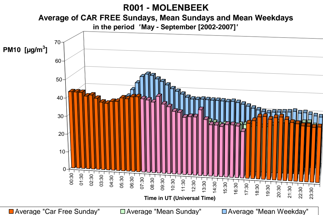
Fig. 30.b : PM10 à Molenbeek – Profil journalier sur les six dimanches sans voiture et sur tous les dimanches et jours ouvrables des périodes 'mai – septembre 2002-2007'.
