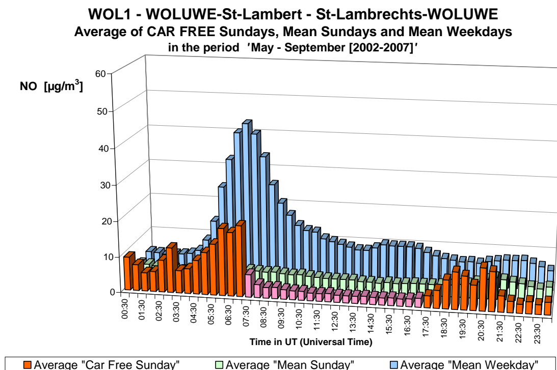
Fig. 15.b : NO à Woluwé – Profil journalier sur les six dimanches sans voiture et sur tous les dimanches et jours ouvrables des périodes 'mai – septembre 2002-2007'.
