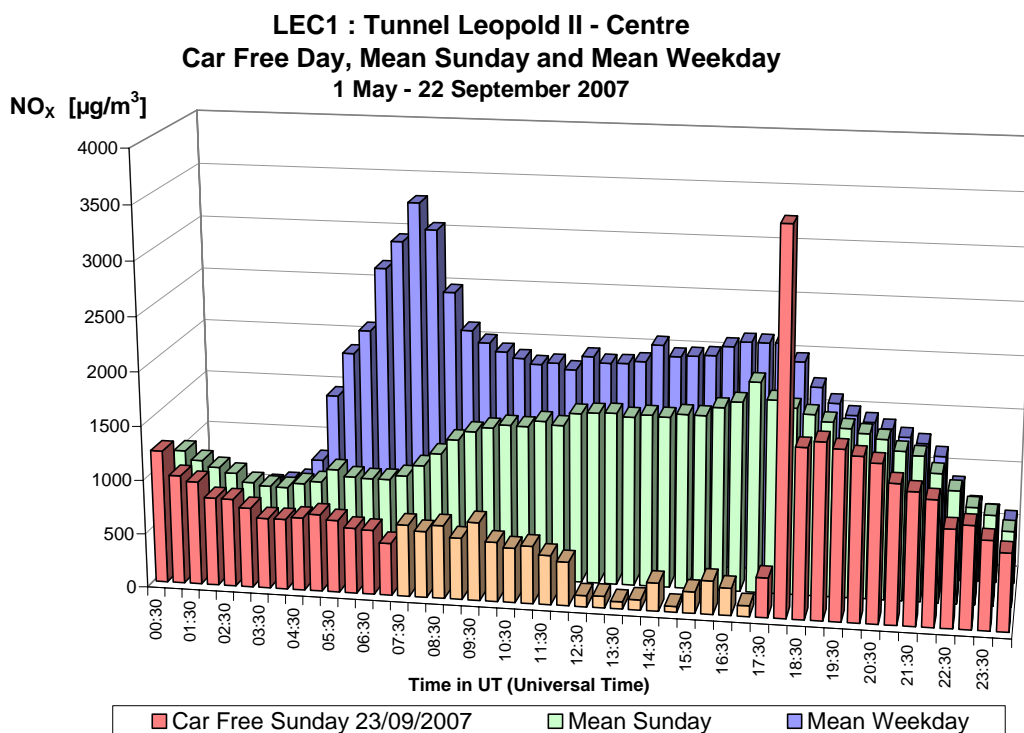
Fig. 3.a : NO x dans le tunnel Léopold II, direction Centre – Profil journalier du dimanche sans voiture 23-09-2007, d'un dimanche moyen et d'un jour ouvrable moyen de la période 'mai – septembre 2007'.
