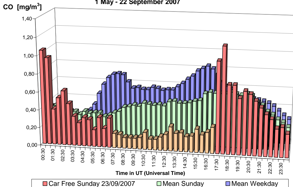
Fig. 24.a : CO au poste de mesure Arts-Loi – Profil journalier du dimanche sans voiture 23-09-2007, d'un dimanche moyen et d'un jour ouvrable moyen de la période 'mai – septembre 2007'.
