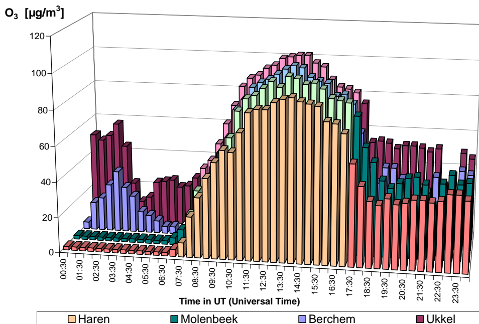
Fig. 22.a: Dimanche sans voiture 23 septembre 2007 – Profil journalier O 3 Situation à 4 endroits différents : Haren, Molenbeek, Berchem et Uccle
