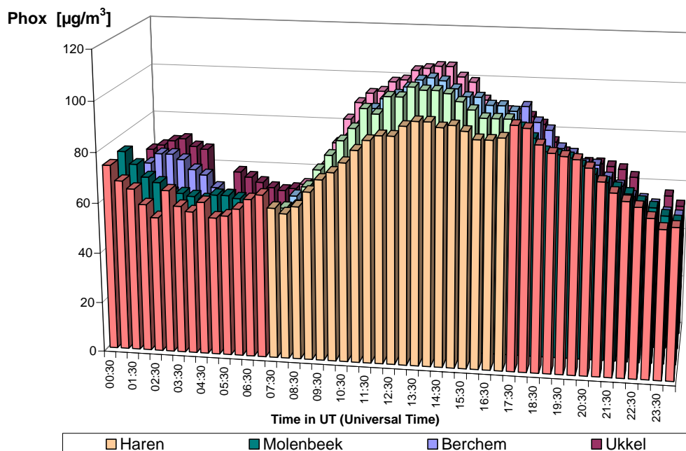
Fig. 22.c: Dimanche sans voiture 23 septembre 2007 – Profil journalier de la somme [O 3 + NO 2 ], exprimée en quantités équivalentes ozone. Situation à 4 endroits différents : Haren, Molenbeek, Berchem et Uccle
