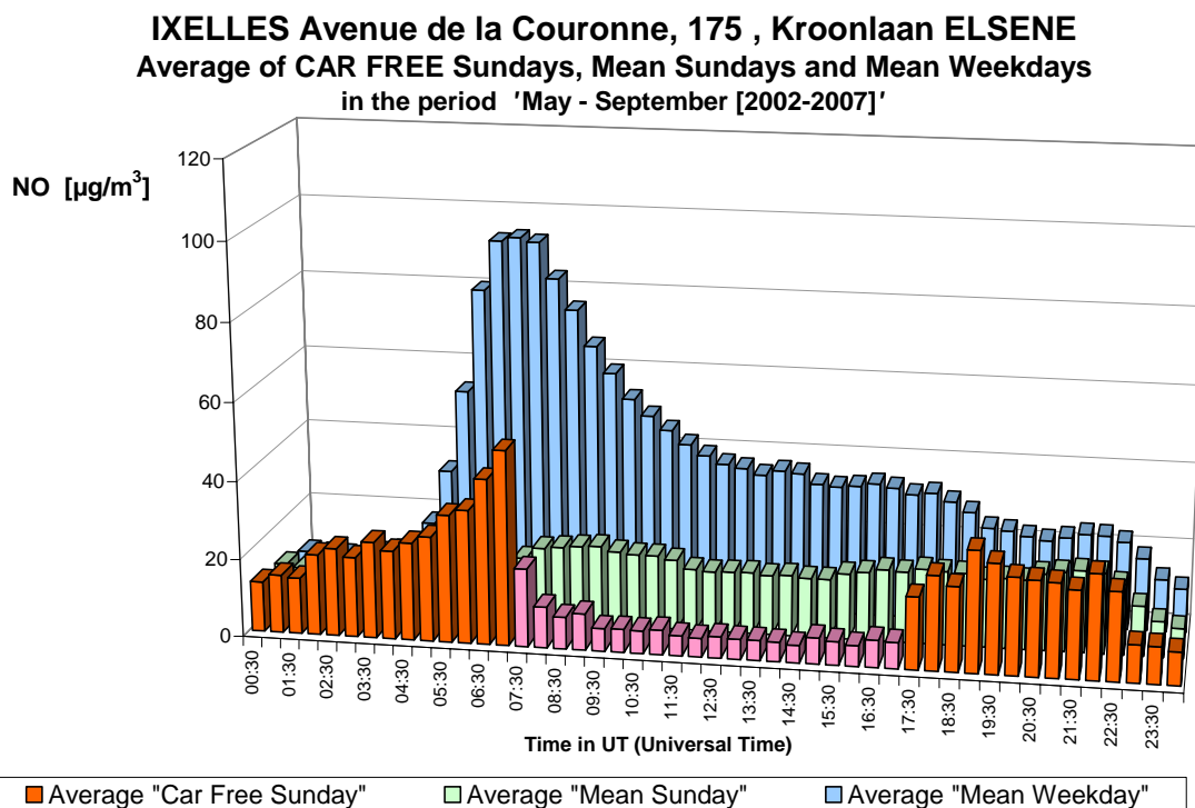
Fig. 11.b : NO à Ixelles (Av. de la Couronne) – Profil journalier sur les six dimanches sans voiture et sur tous les dimanches et jours ouvrables des périodes 'mai – septembre 2002-2007'.
