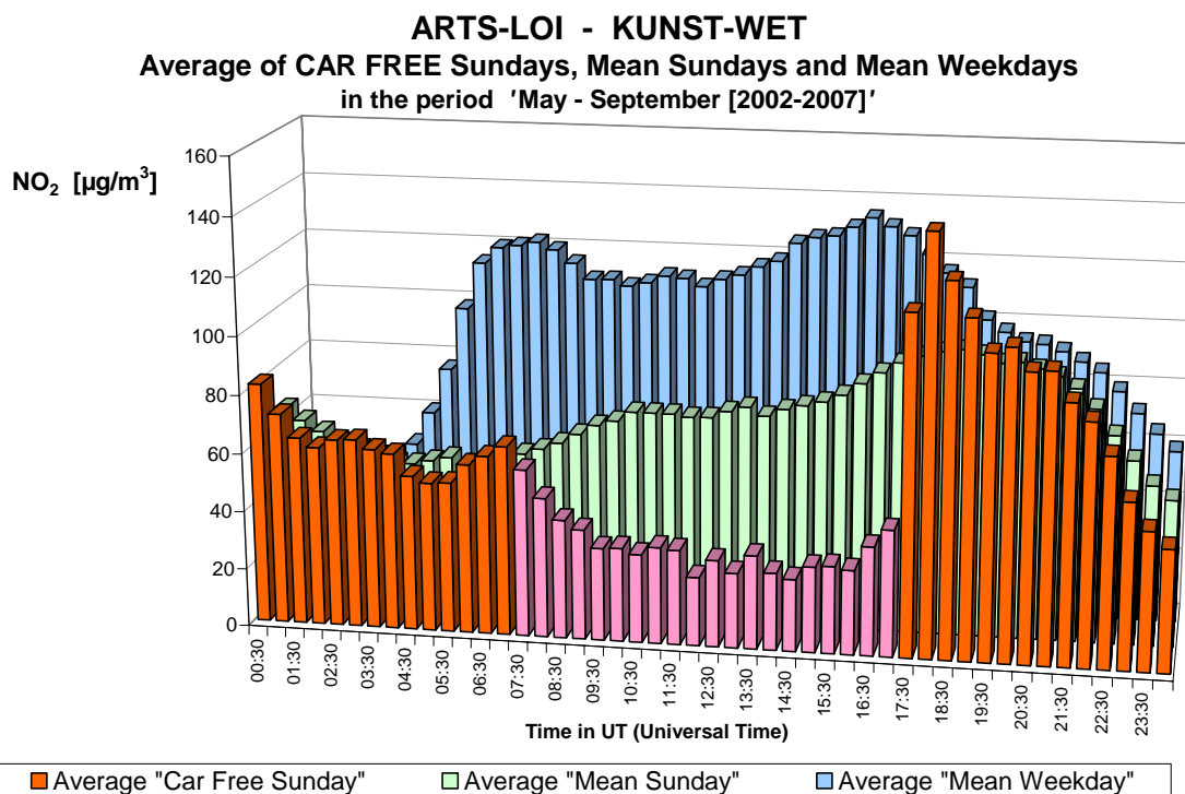
Fig. 10.b : NO 2 au poste de mesure Arts-Loi – Profil journalier sur les six dimanches sans voiture et sur tous les dimanches et jours ouvrables des périodes 'mai – septembre 2002-2007'.
