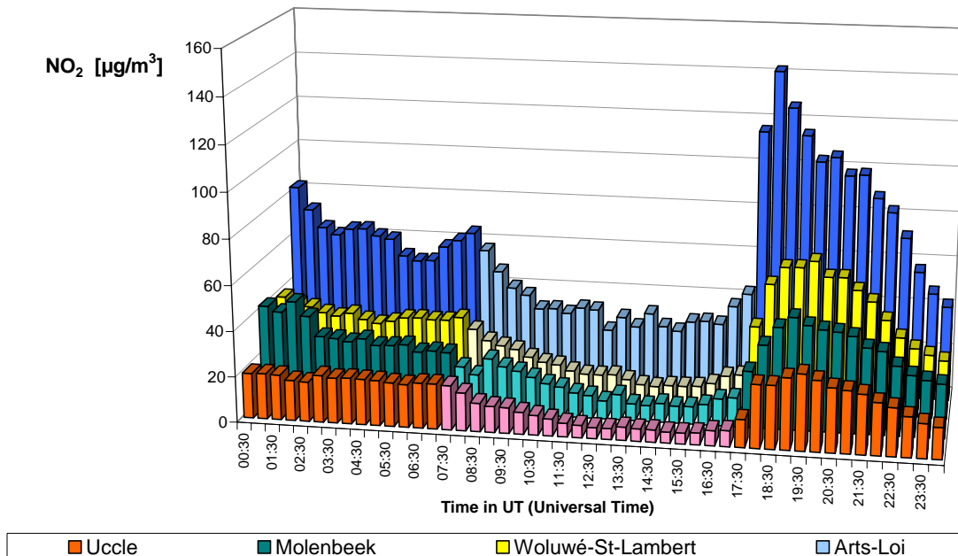
Fig. 18.b : Situation moyenne des 6 dimanches sans voiture– Comparaison du profil journalier en NO 2 à 4 endroits différents– Uccle, Molenbeek, Woluwé-St-Lambert et Arts-Loi
