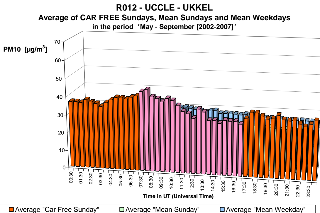
Fig. 32.b : PM10 à Uccle – Profil journalier sur les six dimanches sans voiture et sur tous les dimanches et jours ouvrables des périodes 'mai – septembre 2002-2007'.
