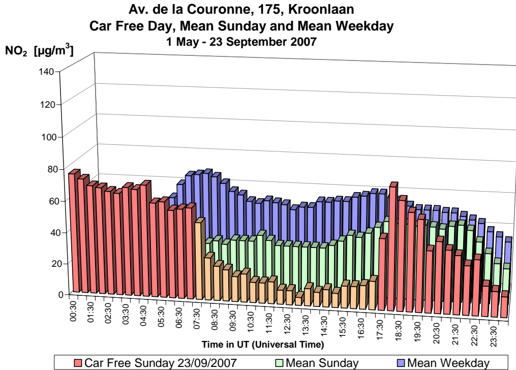
Fig. 12.a : NO 2 à Ixelles (Av. de la Couronne) – Profil journalier du dimanche sans voiture 23-09-2007, d'un dimanche moyen et d'un jour ouvrable moyen de la 'période mai – septembre 2007'.
