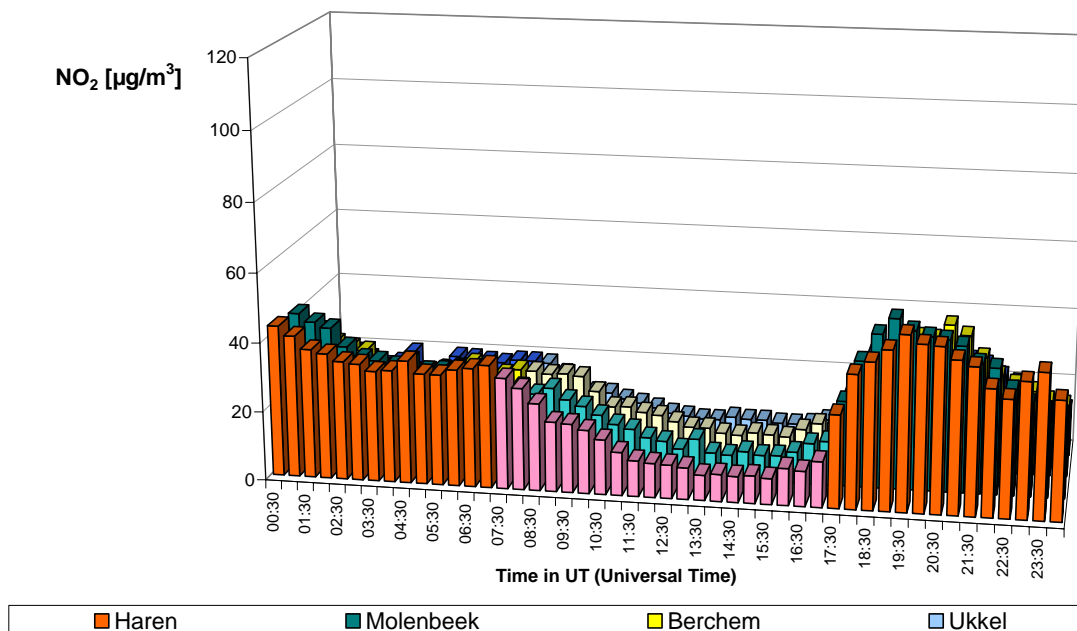
Fig. 23.b: Moyenne sur les six dimanches sans voiture – Profil journalier complémentaire en NO 2 Situation à 4 endroits différents : Haren, Molenbeek, Berchem et Uccle
