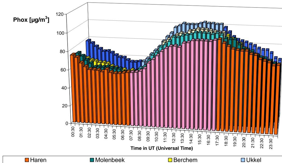
Fig. 23.c: Moyenne sur les six dimanches sans voiture – Profil journalier de la somme [O 3 + NO 2 ], exprimée en quantités équivalentes ozone Situation à 4 endroits différents : Haren, Molenbeek, Berchem et Uccle
