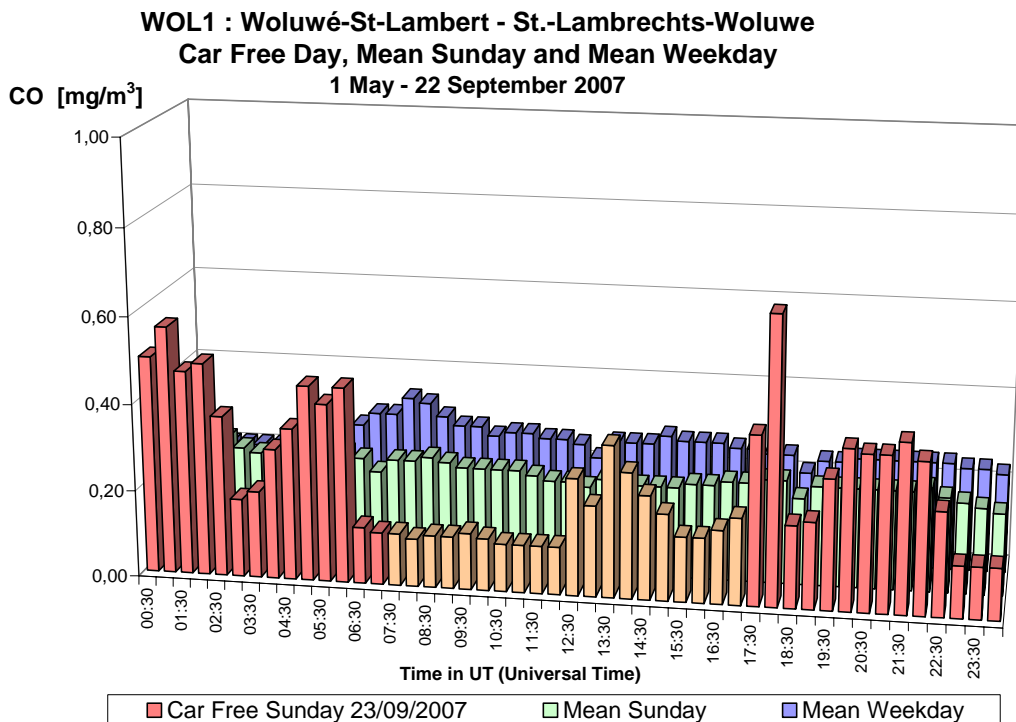
Fig. 26.a : CO à Woluwé – Profil journalier du dimanche sans voiture 23-09-2007, d'un dimanche moyen et d'un jour ouvrable moyen de la période 'mai – septembre 2007'.
