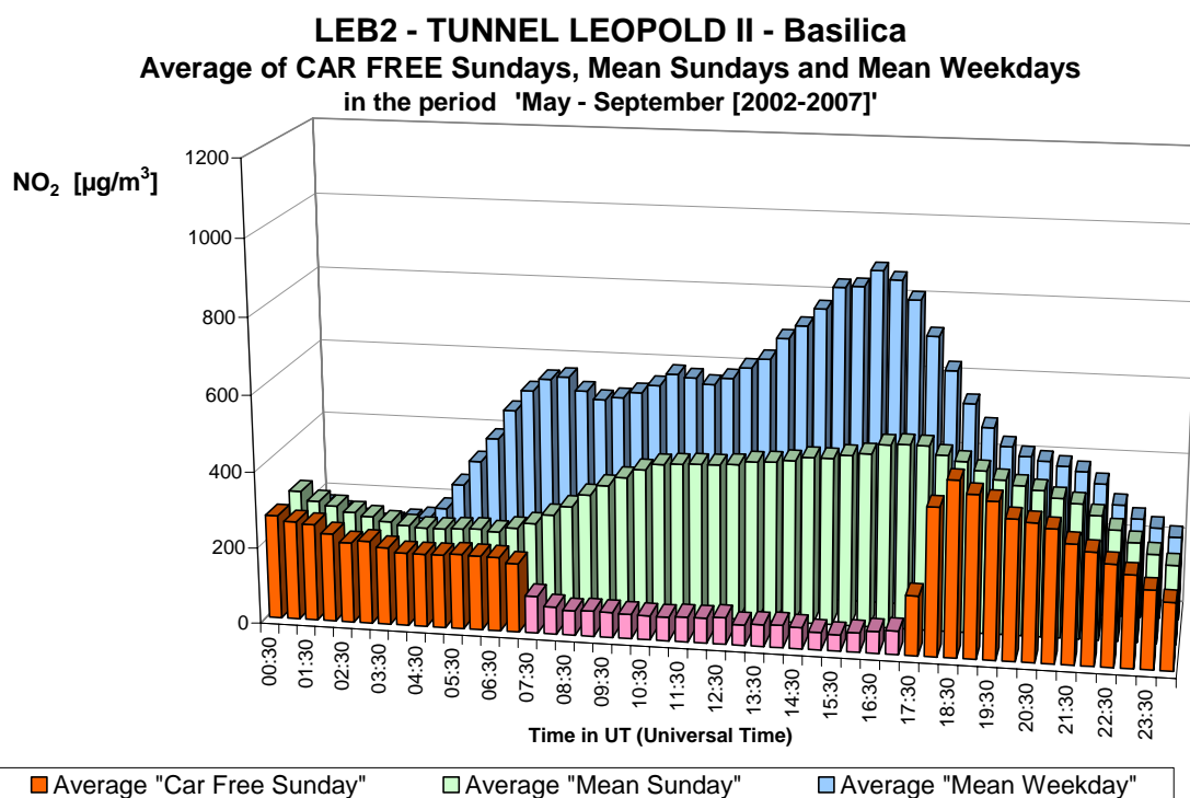
Fig. 6.b : NO 2 dans le tunnel Léopold II, direction Basilique – Profil journalier sur les six dimanches sans voiture et sur tous les dimanches et jours ouvrables des périodes 'mai – septembre 2002-2007'.
