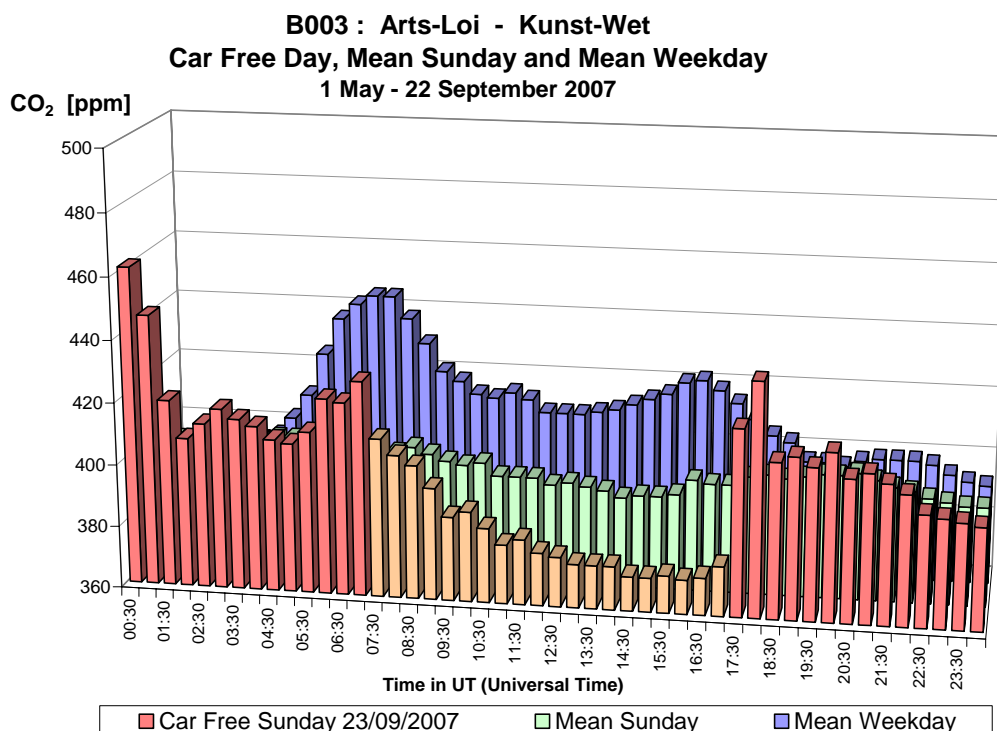
Fig. 27.a : CO 2 au poste de mesure Arts-Loi – Profil journalier du dimanche sans voiture 23-09-2007, d'un dimanche moyen et d'un jour ouvrable moyen de la période 'mai – septembre 2007'.
