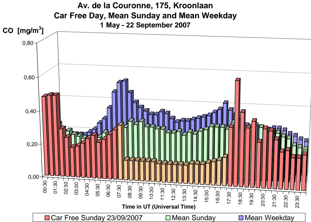
Fig. 25.a : CO à Ixelles (Av. de la Couronne) – Profil journalier du dimanche sans voiture 23-09-2007, d'un dimanche moyen et d'un jour ouvrable moyen de la période 'mai – septembre 2007'.
