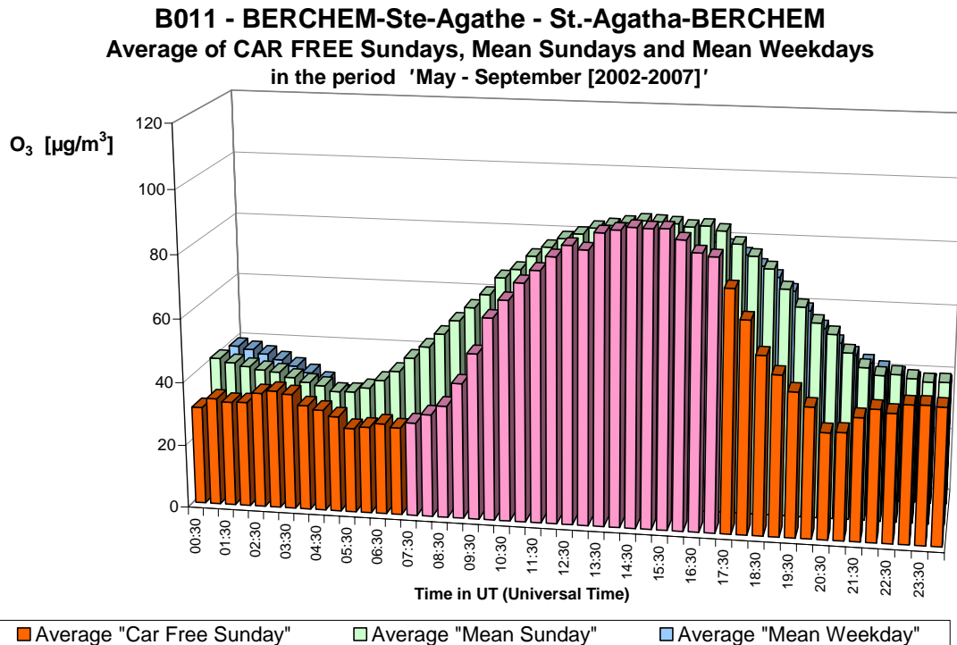
Fig. 20.b : O 3 à Berchem – Profil journalier sur les six dimanches sans voiture et sur tous les dimanches et jours ouvrables des périodes 'mai – septembre 2002-2007'.
