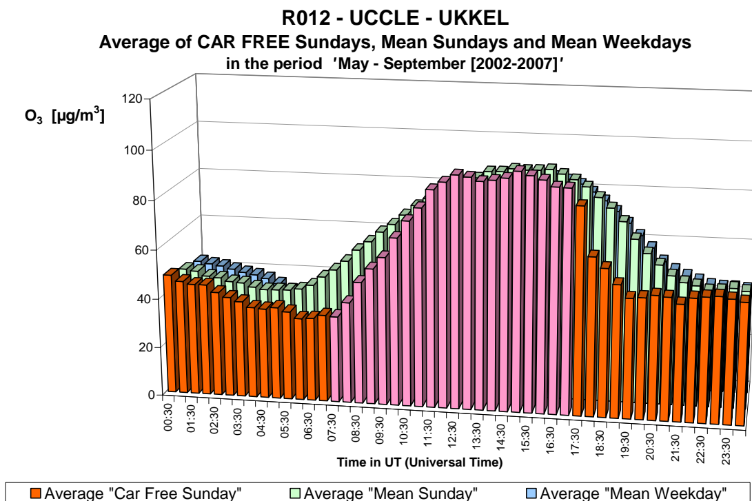
Fig. 19.b : O 3 à Uccle – Profil journalier sur les six dimanches sans voiture et sur tous les dimanches et jours ouvrables des périodes 'mai – septembre 2002-2007'.
