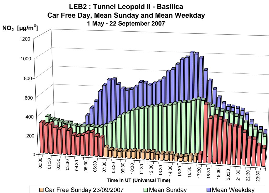
Fig. 6.a : NO 2 dans le tunnel Léopold II, direction Basilique – Profil journalier du dimanche sans voiture 23-09-2007, d'un dimanche moyen et d'un jour ouvrable moyen de la période 'mai – septembre 2007'.
