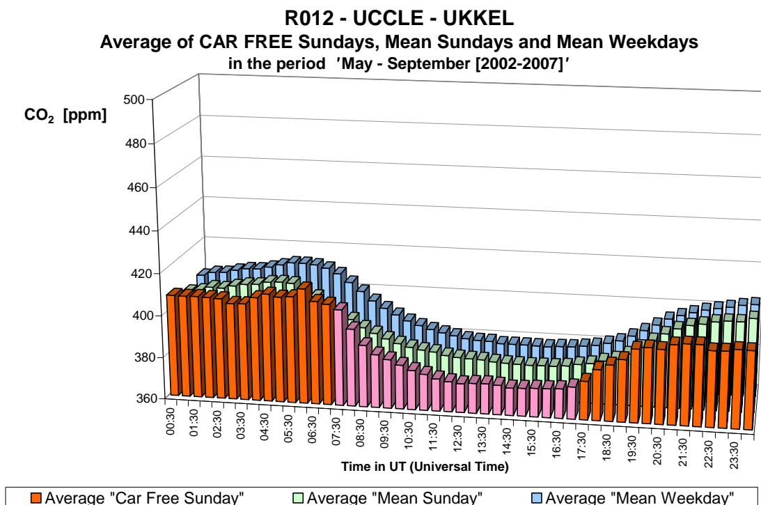
Fig. 29.b : CO 2 à Uccle – Profil journalier sur les six dimanches sans voiture et sur tous les dimanches et jours ouvrables des périodes 'mai – septembre 2002-2007'.
