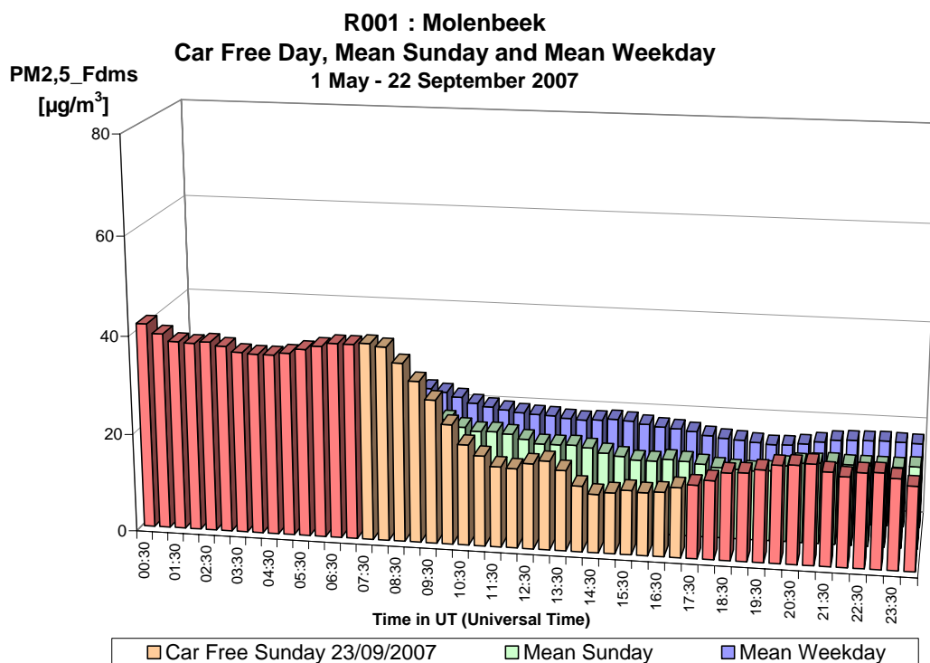
Fig. 36 : PM 2,5 à Molenbeek – Profil journalier du dimanche sans voiture, d'un dimanche moyen et d'un jour ouvrable moyen de la période 'mai – septembre 2007'
