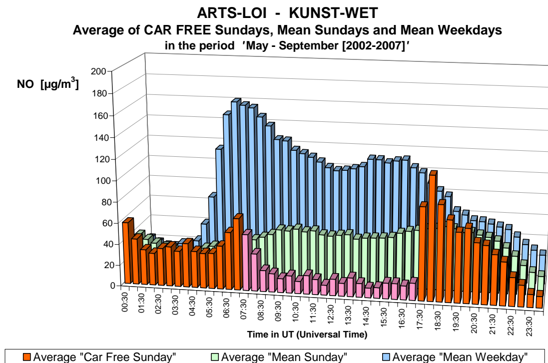
Fig. 9.b : NO au poste de mesure Arts-Loi – Profil journalier sur les six dimanches sans voiture et sur tous les dimanches et jours ouvrables des périodes 'mai – septembre 2002-2007'.
