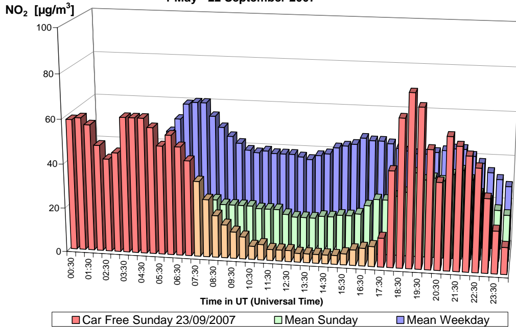
Fig. 16.a : NO 2 à Woluwé – Profil journalier du dimanche sans voiture 23-09-2007, d'un dimanche moyen et d'un jour ouvrable moyen de la période 'mai – septembre 2007'.
