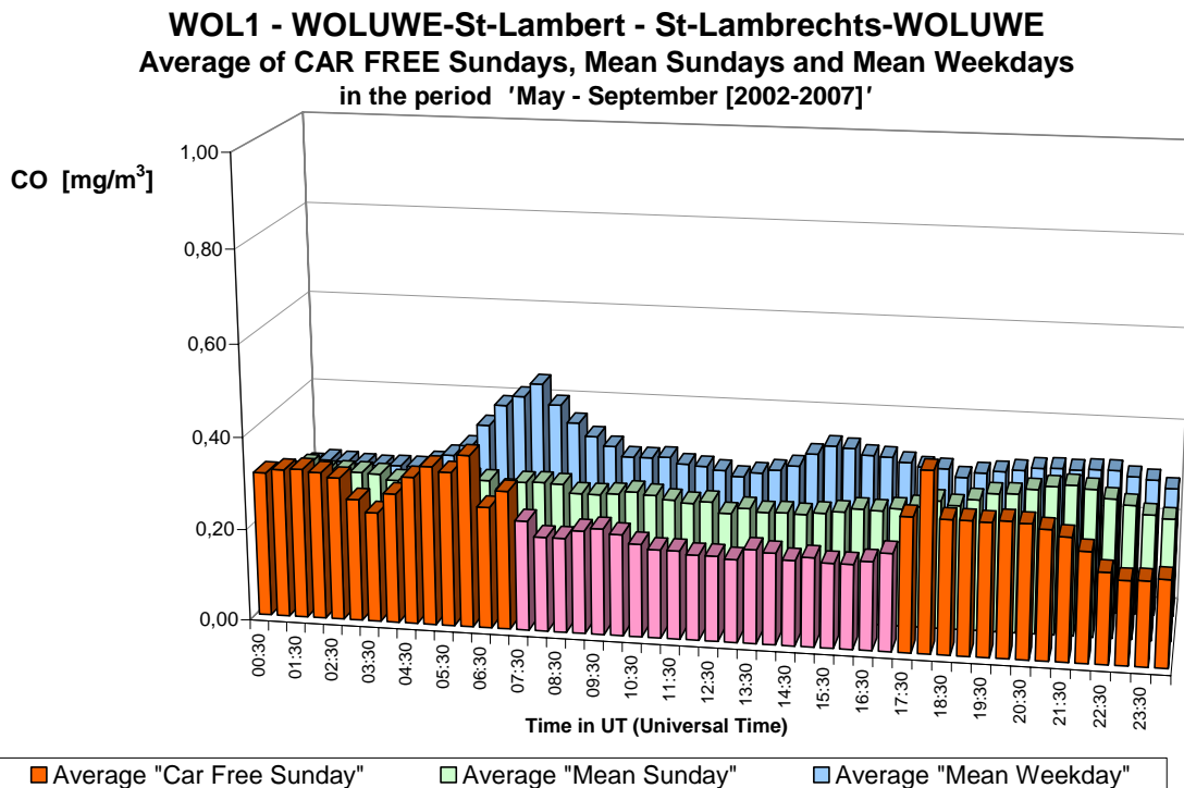
Fig. 26.b : CO à Woluwé – Profil journalier sur les six dimanches sans voiture et sur tous les dimanches et jours ouvrables des périodes 'mai – septembre 2002-2007'.
