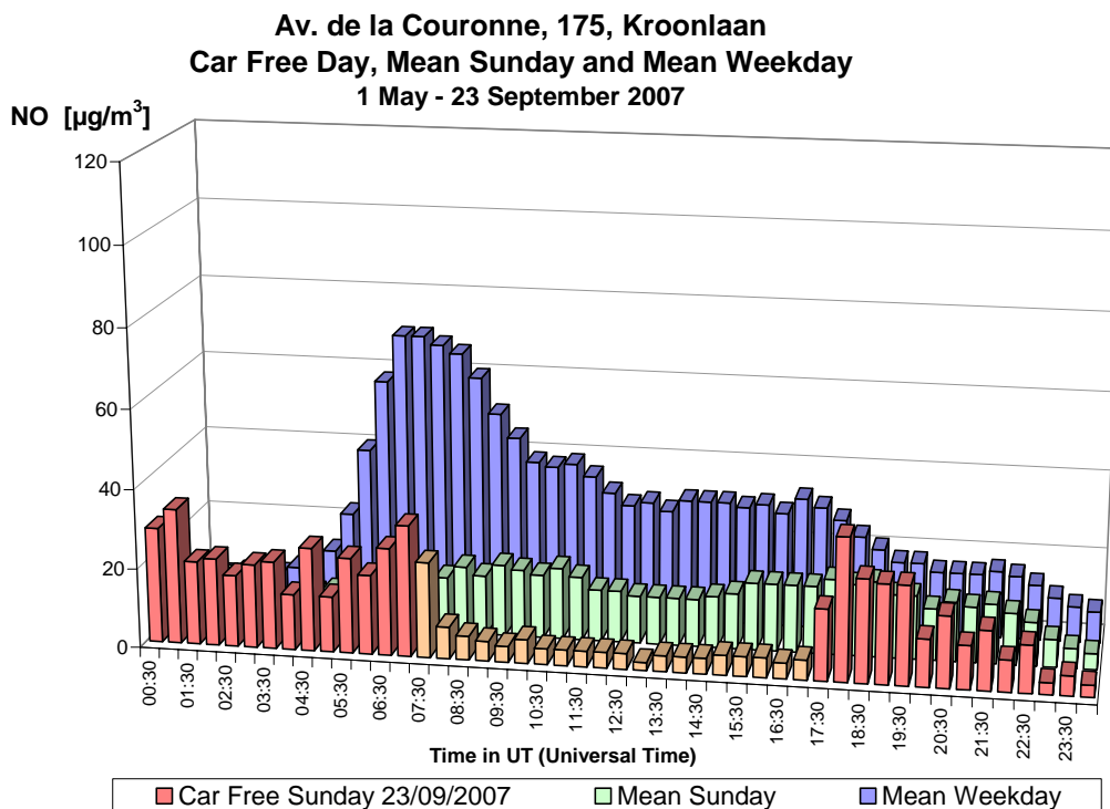
Fig. 11.a : NO à Ixelles (Av. de la Couronne) – Profil journalier du dimanche sans voiture 23-09-2007, d'un dimanche moyen et d'un jour ouvrable moyen de la 'période'.
