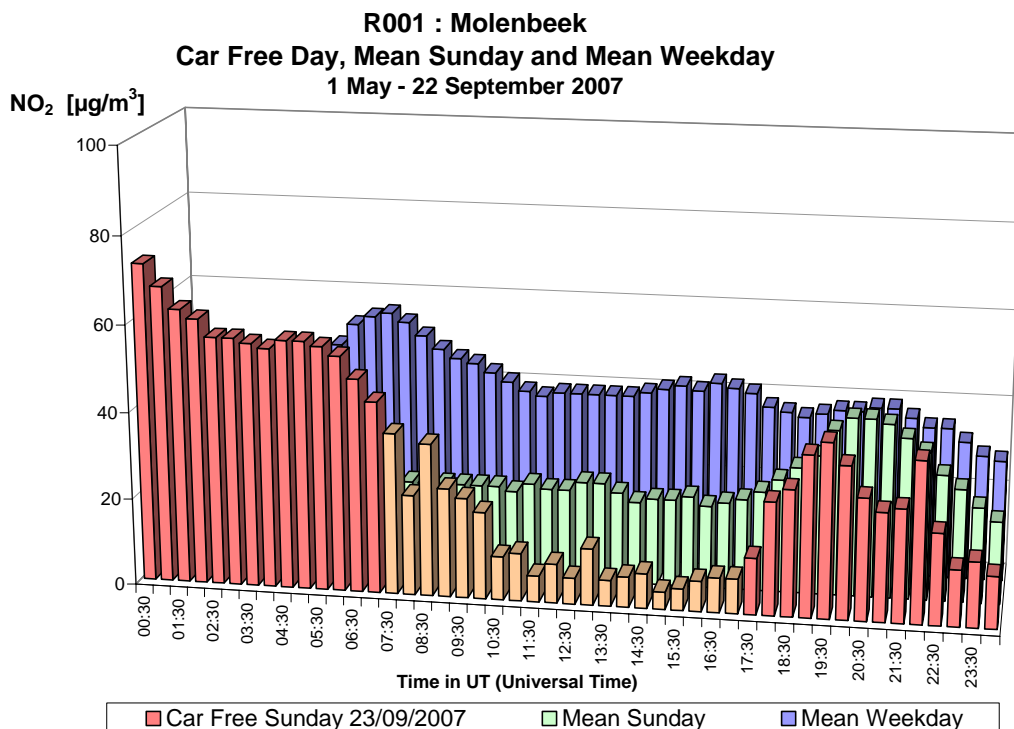
Fig. 14.a : NO 2 à Molenbeek – Profil journalier du dimanche sans voiture 23-09-2007, d'un dimanche moyen et d'un jour ouvrable moyen de la période 'mai – septembre 2007'.
