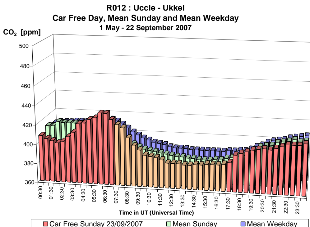
Fig. 29.a : CO 2 à Uccle – Profil journalier du dimanche sans voiture 23-09-2007, d'un dimanche moyen et d'un jour ouvrable moyen de la période 'mai – septembre 2007'.
