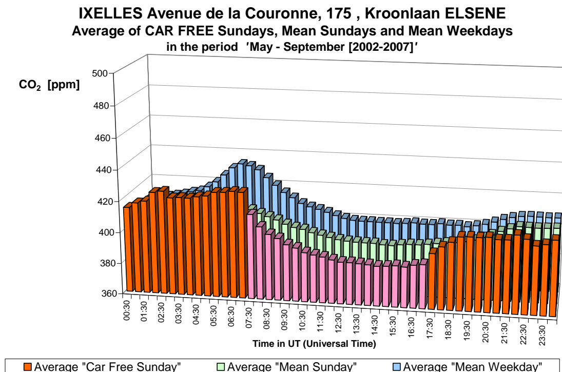
Fig. 28.b : CO 2 à Ixelles (Av. de la Couronne) – Profil journalier sur les six dimanches sans voiture et sur tous les dimanches et jours ouvrables des périodes 'mai – septembre 2002-2007'.
