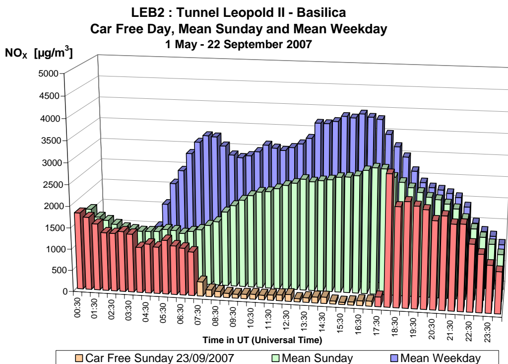
Fig. 7.a: NO x dans le tunnel Léopold II, direction Basilique – Profil journalier du dimanche sans voiture 23-09-2007, d'un dimanche moyen et d'un jour ouvrable moyen de la période 'mai – septembre 2007'.
