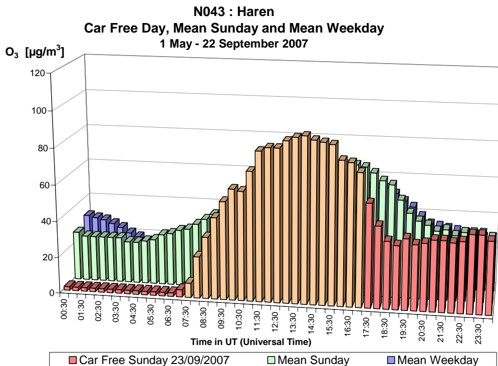
Fig. 21.a : O 3 à Haren – Profil journalier du dimanche sans voiture 23-09-2007, d'un dimanche moyen et d'un jour ouvrable moyen de la période 'mai – septembre 2007'.
