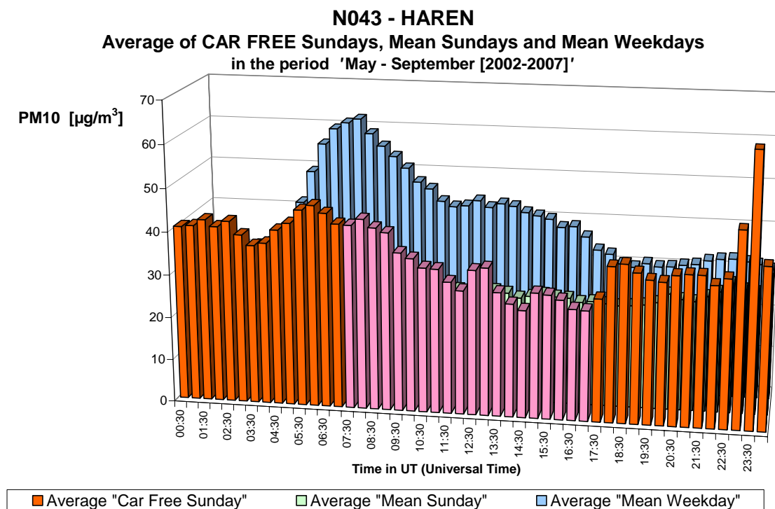
Fig. 33.b : PM10 à Haren – Profil journalier sur les six dimanches sans voiture et sur tous les dimanches et jours ouvrables des périodes 'mai – septembre 2002-2007'.
