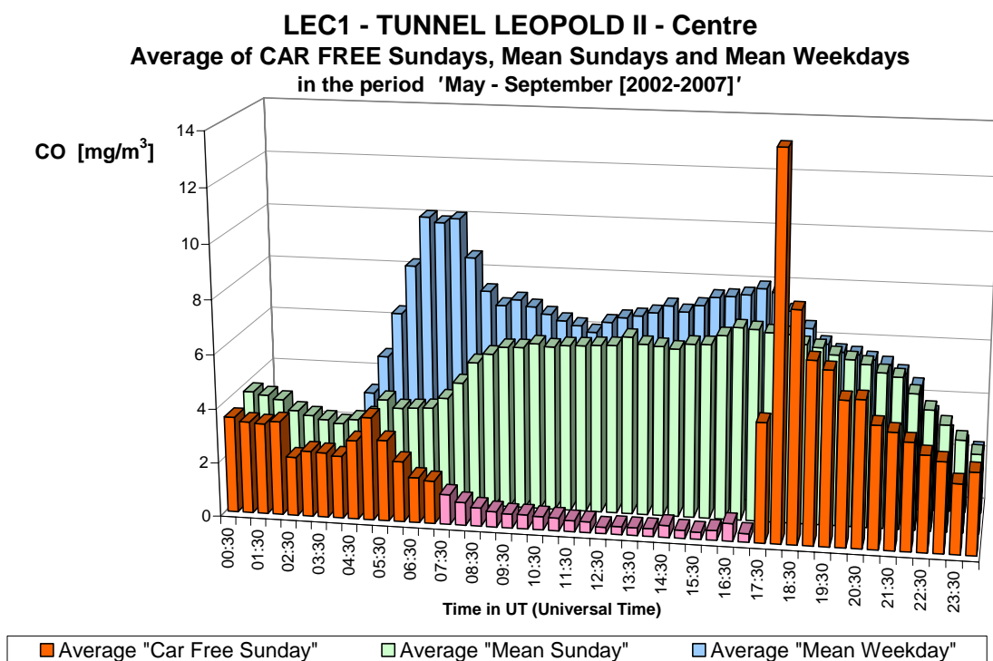
Fig. 4.b : CO dans le tunnel Léopold II, direction Centre – Profil journalier sur les six dimanches sans voiture et sur tous les dimanches et jours ouvrables des périodes 'mai – septembre 2002-2007'.
