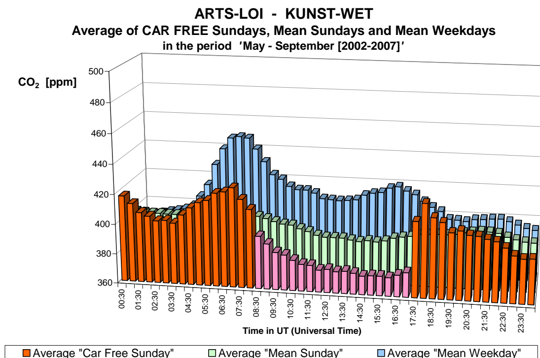
Fig. 27.b : CO 2 au poste de mesure Arts-Loi – Profil journalier sur les six dimanches sans voiture et sur tous les dimanches et jours ouvrables des périodes 'mai – septembre 2002-2007'.
