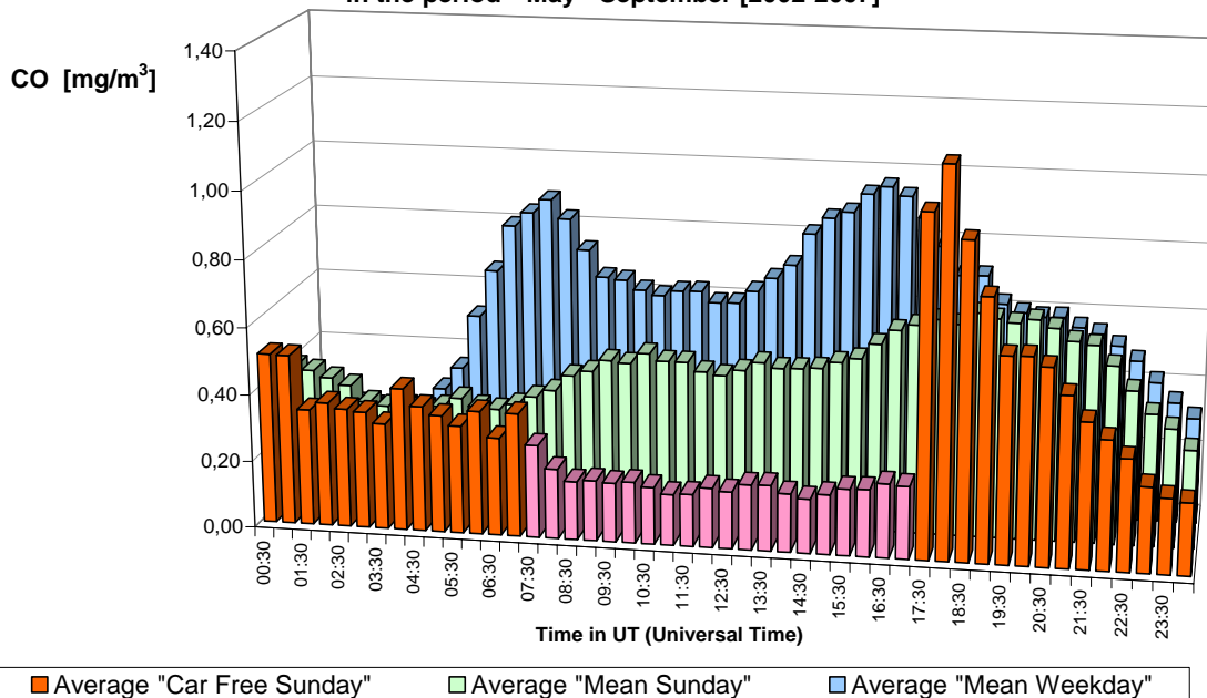
Fig. 24.b : CO au poste de mesure Arts-Loi – Profil journalier sur les six dimanches sans voiture et sur tous les dimanches et jours ouvrables des périodes 'mai – septembre 2002-2007'.
