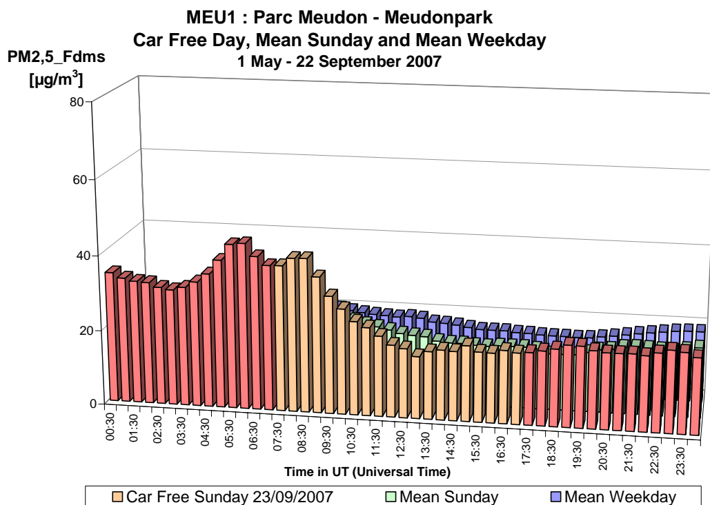
Fig. 39 : PM 2,5 au Parc Meudon – Profil journalier du dimanche sans voiture 23-09-2007, d'un dimanche moyen et d'un jour ouvrable moyen de la période 'mai – septembre 2007'
