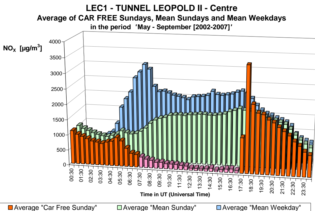
Fig. 3.b : NO x dans le tunnel Léopold II, direction Centre – Profil journalier sur les six dimanches sans voiture et sur tous les dimanches et jours ouvrables des périodes 'mai – septembre 2002-2007'.
