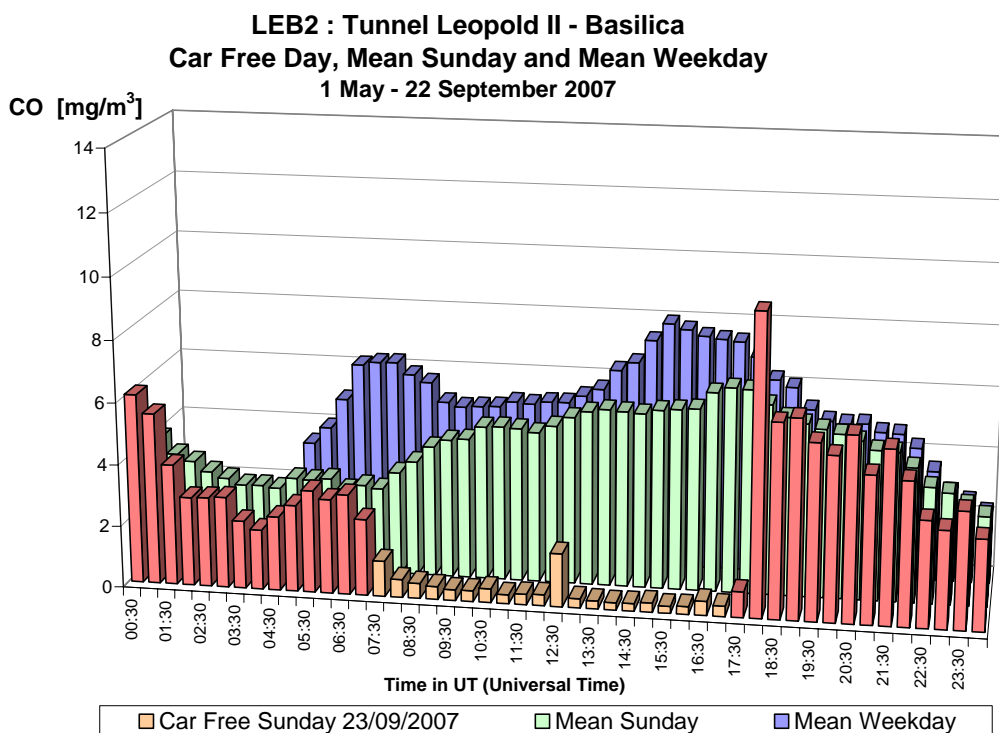
Fig. 8.a : CO dans le tunnel Léopold II, direction Basilique – Profil journalier du dimanche sans voiture 23-09-2007, d'un dimanche moyen et d'un jour ouvrable moyen de la période 'mai – septembre 2007'.
