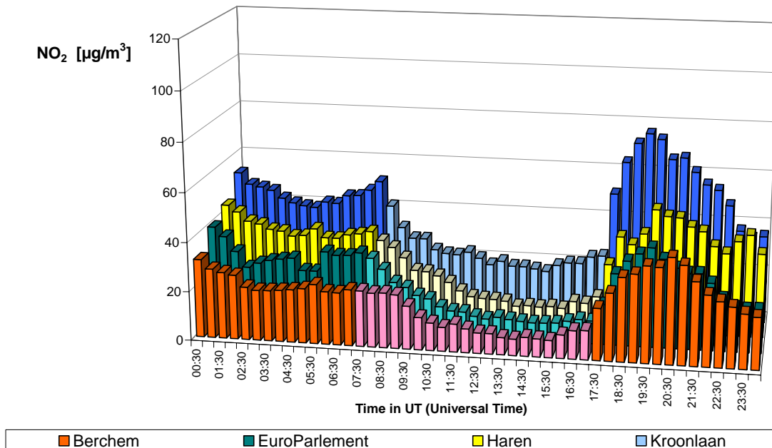
Fig. 17.b : Situation moyenne des 6 dimanches sans voiture – Comparaison du profil journalier en NO 2 à 4 endroits différents – Berchem, Parlement européen, Haren et Av. de la Couronne à Ixelles
