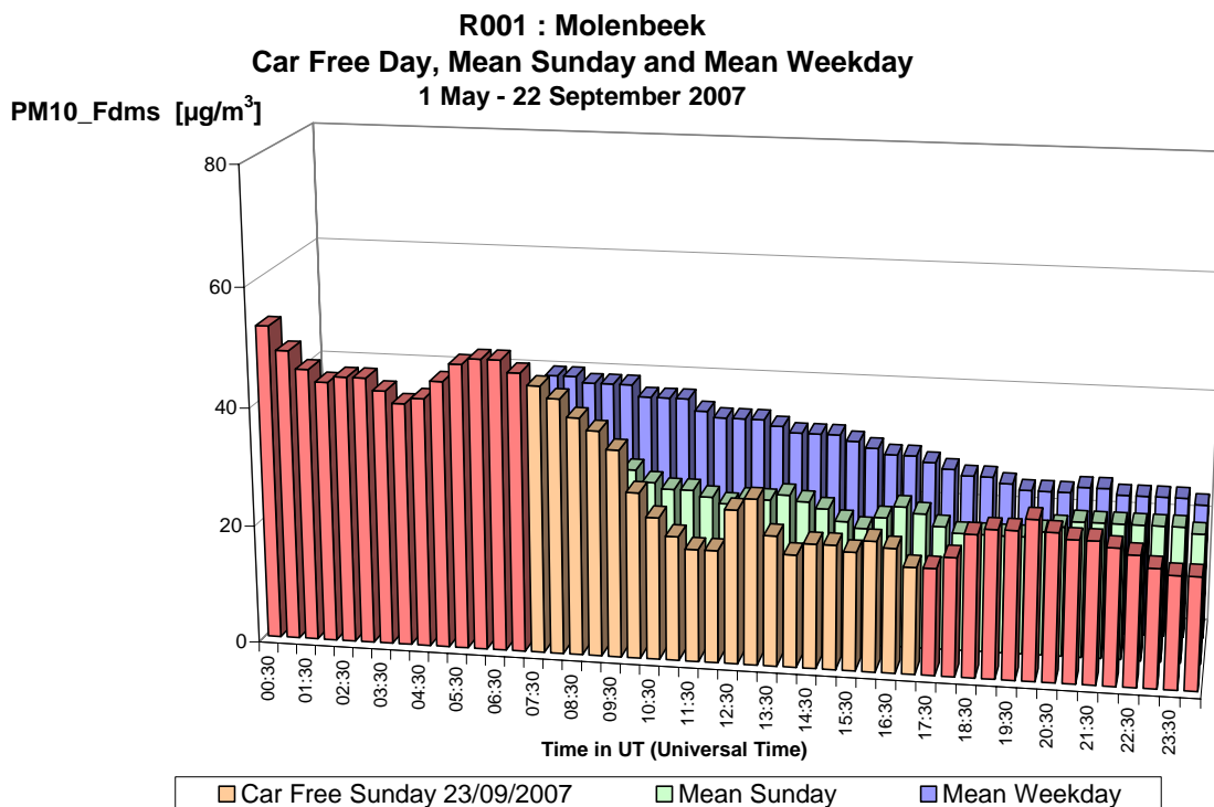
Fig. 30.a : PM10 à Molenbeek – Profil journalier du dimanche sans voiture 23-09-2007, d'un dimanche moyen et d'un jour ouvrable moyen de la période 'mai – septembre 2007'
