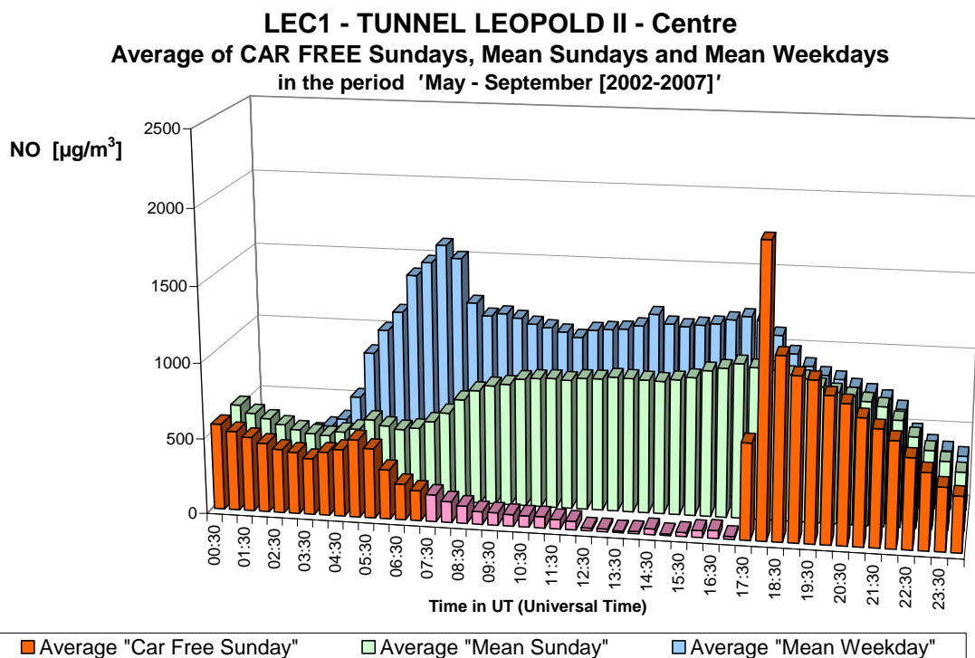
Fig. 1.b : NO dans le tunnel Léopold II, direction Centre – Profil journalier sur les six dimanches sans voiture et sur tous les dimanches et jours ouvrables des périodes 'mai – septembre 2002-2007'.
