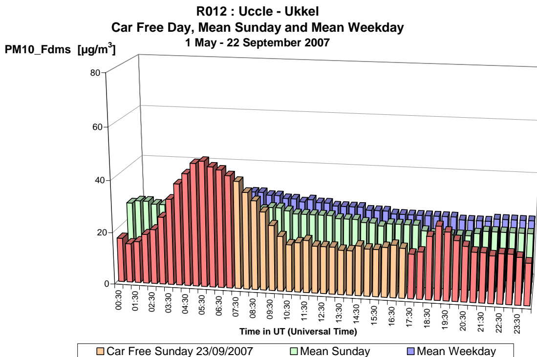
Fig. 32.a : PM10 à Uccle – Profil journalier du dimanche sans voiture 23-09-2007, d'un dimanche moyen et d'un jour ouvrable moyen de la période 'mai – septembre 2007'
