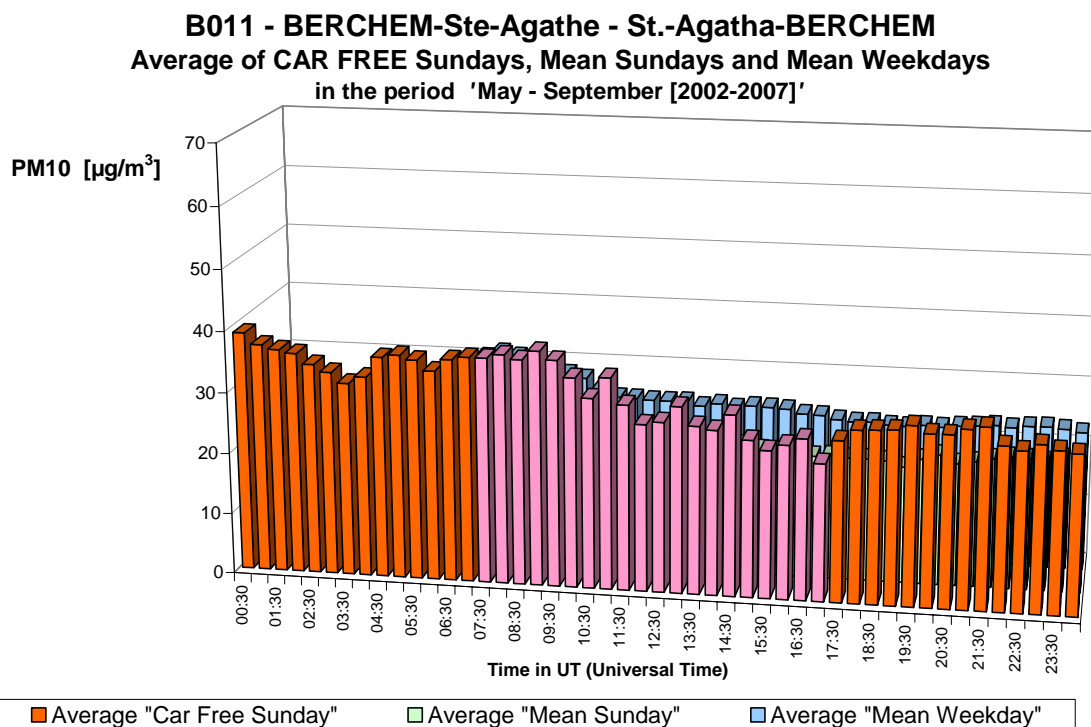
Fig. 31.b : PM10 à Berchem-Ste-Agathe – Profil journalier sur les six dimanches sans voiture et sur tous les dimanches et jours ouvrables des périodes 'mai – septembre 2002-2007'.
