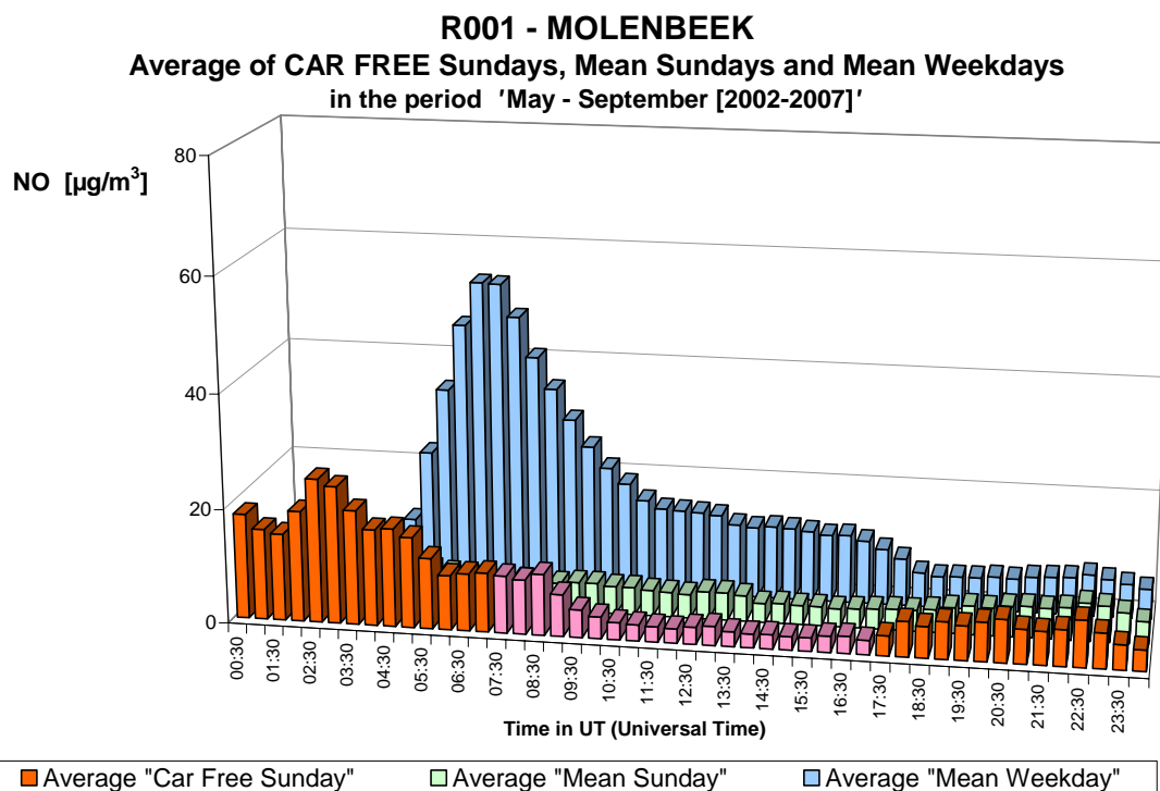
Fig. 13.b : NO à Molenbeek – Profil journalier sur les six dimanches sans voiture et sur tous les dimanches et jours ouvrables des périodes 'mai – septembre 2002-2007'.
