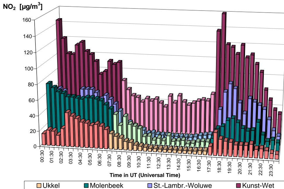
Fig. 18.a : Dimanche sans voiture du 23-09-2007 – Comparaison du profil journalier en NO 2 à 4 endroits différents– Uccle, Molenbeek, Woluwé-St-Lambert et Arts-Loi
