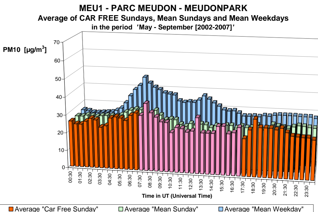
Fig. 34.b : PM10 au Parc Meudon – Profil journalier sur les six dimanches sans voiture et sur tous les dimanches et jours ouvrables des périodes 'mai – septembre 2002-2007'.
