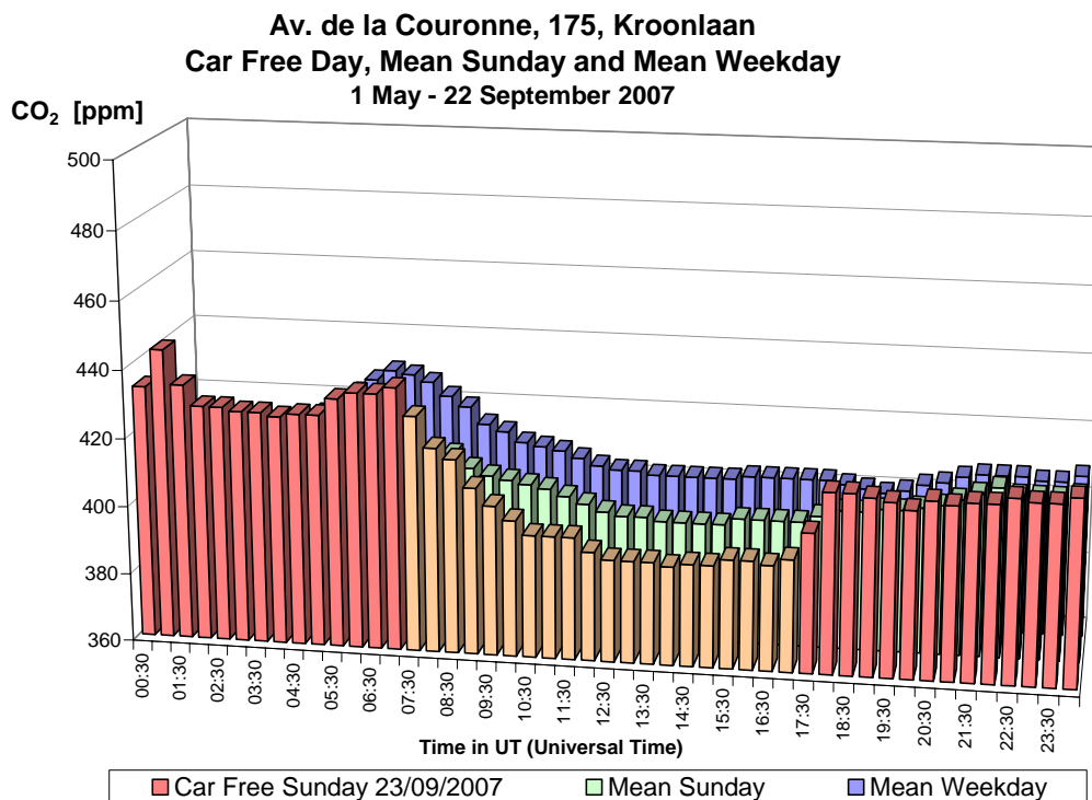
Fig. 28.a : CO 2 à Ixelles (Av. de la Couronne) – Profil journalier du dimanche sans voiture 23-09-2007, d'un dimanche moyen et d'un jour ouvrable moyen de la période 'mai – septembre 2007'.
