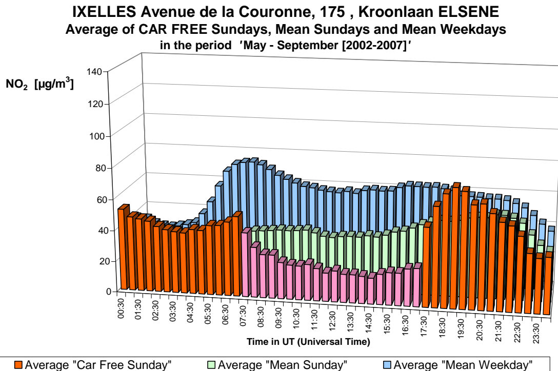
Fig. 12.b : NO 2 à Ixelles (Av. de la Couronne) – Profil journalier sur les six dimanches sans voiture et sur tous les dimanches et jours ouvrables des périodes 'mai – septembre 2002-2007'.
