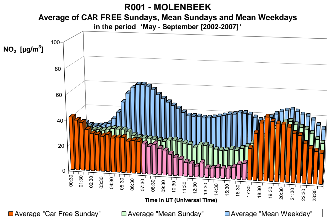
Fig. 14.b : NO 2 à Molenbeek – Profil journalier sur les six dimanches sans voiture et sur tous les dimanches et jours ouvrables des périodes 'mai – septembre 2002-2007'.
