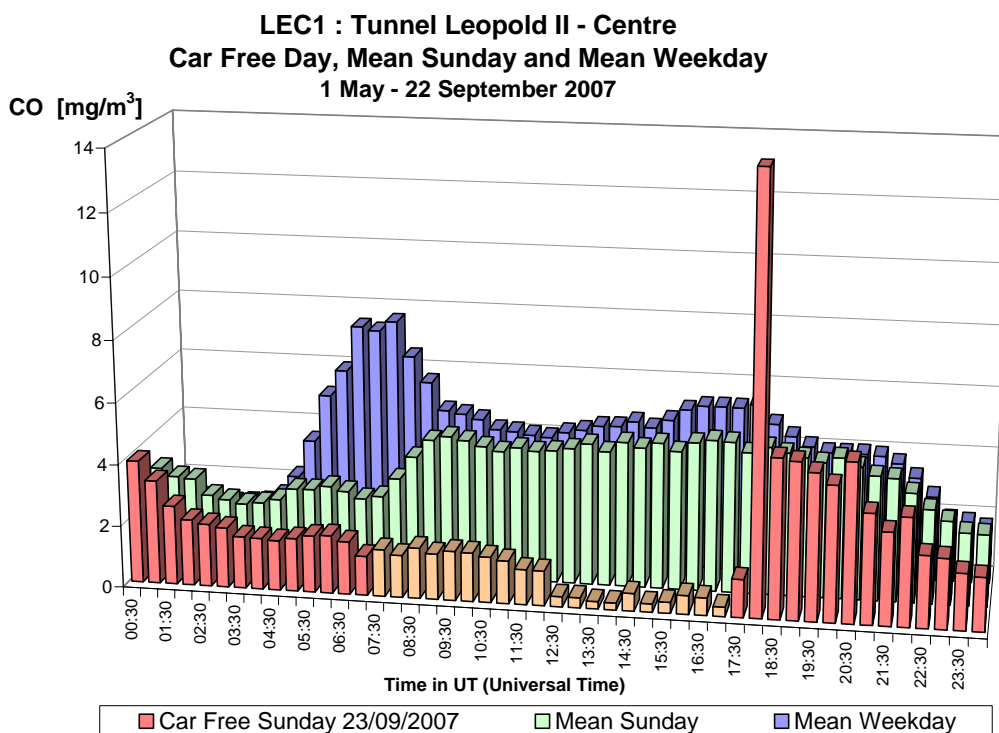
Fig. 4.a : CO dans le tunnel Léopold II, direction Centre – Profil journalier du dimanche sans voiture 23-09-2007, d'un dimanche moyen et d'un jour ouvrable moyen de la période 'mai – septembre 2007'.
