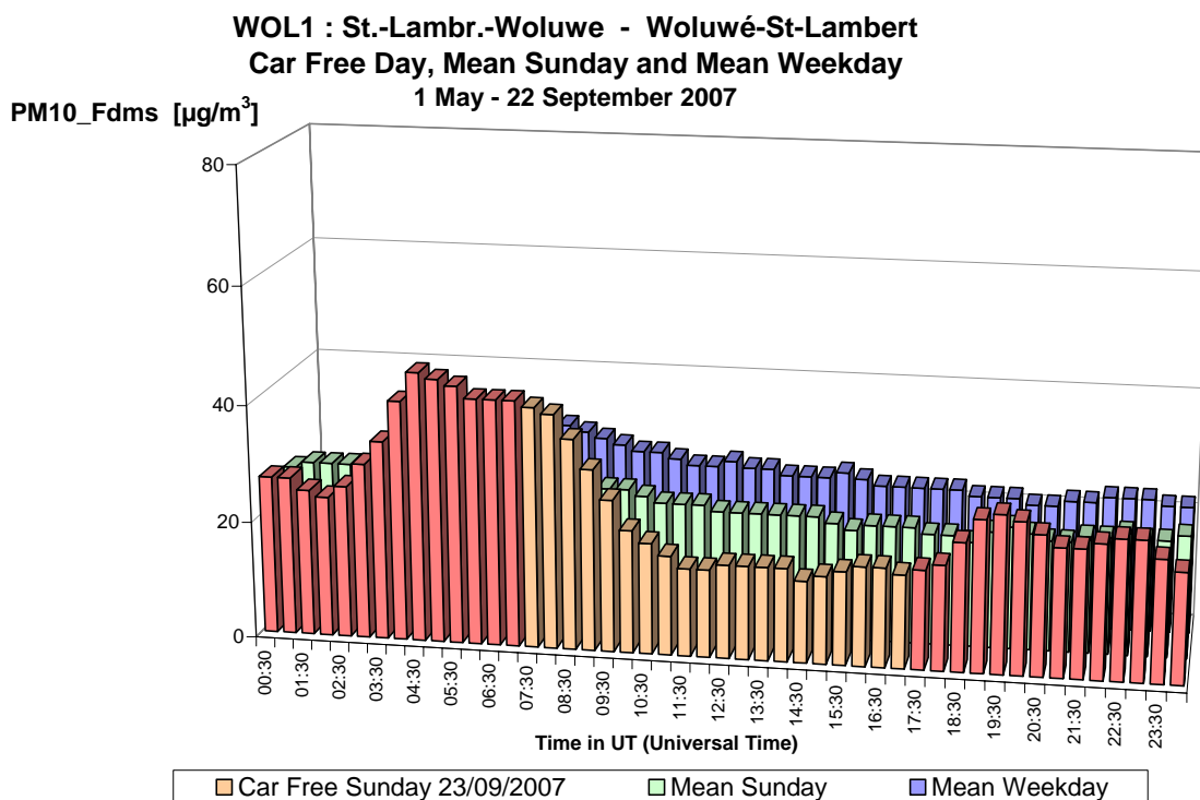
Fig. 35.a : PM10 à Woluwé-St-Lambert – Profil journalier du dimanche sans voiture 23-09-2007, d'un dimanche moyen et d'un jour ouvrable moyen de la période 'mai – septembre 2007'
