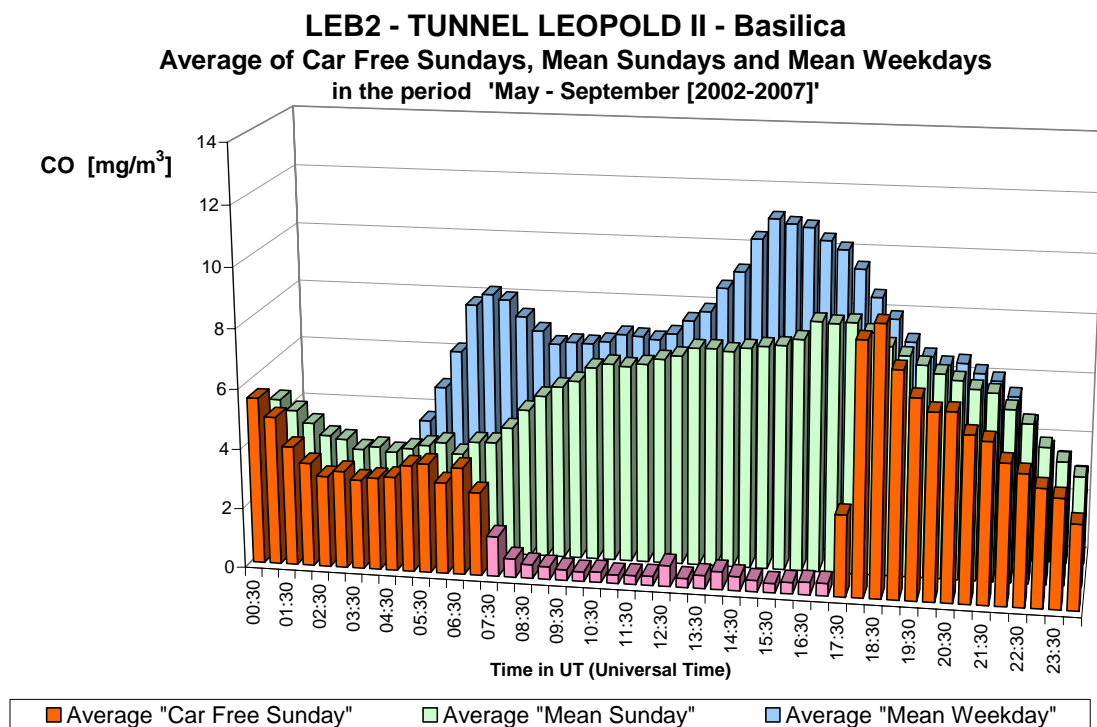
Fig. 8.b : CO dans le tunnel Léopold II, direction Basilique – Profil journalier sur les six dimanches sans voiture et sur tous les dimanches et jours ouvrables des périodes 'mai – septembre 2002-2007'.
