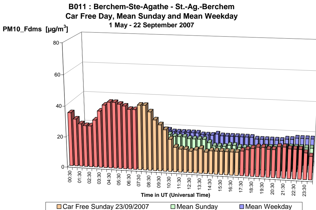
Fig. 31.a : PM10 à Berchem-Ste-Agathe – Profil journalier du dimanche sans voiture 23-09-2007, d'un dimanche moyen et d'un jour ouvrable moyen de la période 'mai – septembre 2007'
