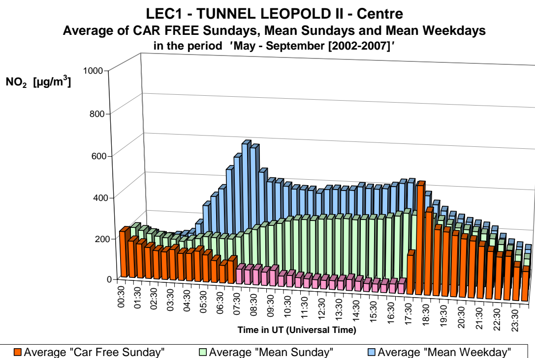
Fig. 2.b : NO 2 dans le tunnel Léopold II, direction Centre – Profil journalier sur les six dimanches sans voiture et sur tous les dimanches et jours ouvrables des périodes 'mai – septembre 2002-2007'.
