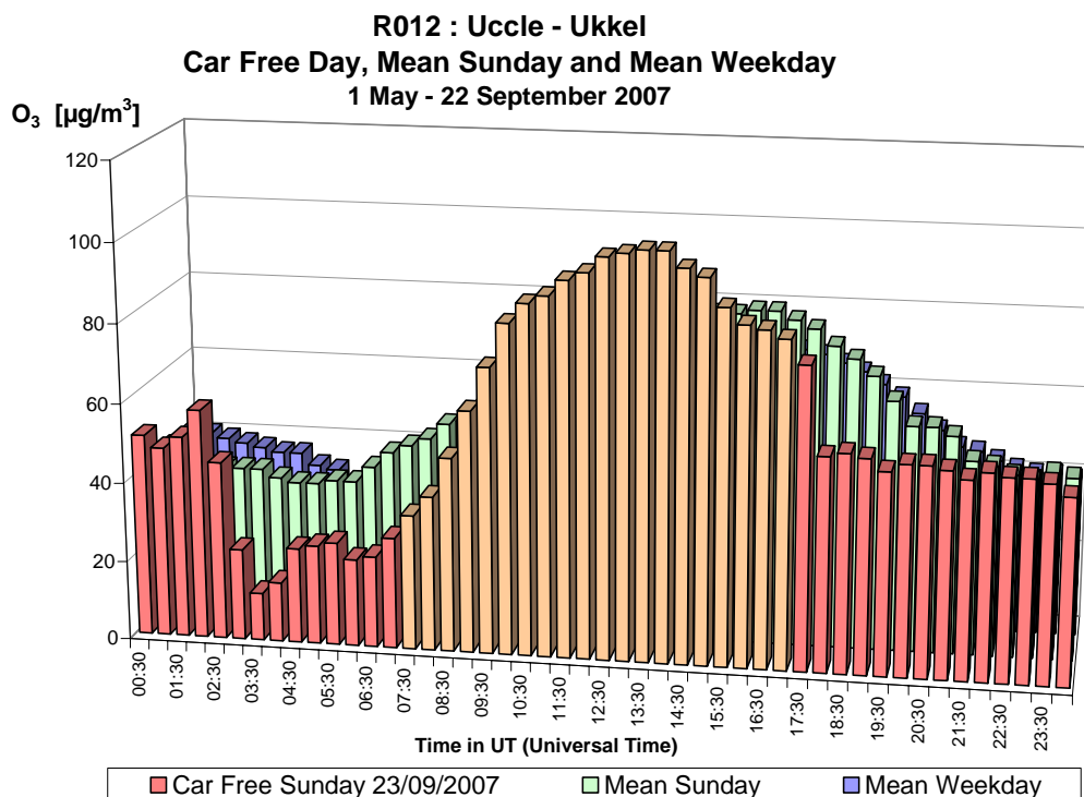
Fig. 19.a : O 3 à Uccle – Profil journalier du dimanche sans voiture 23-09-2007, d'un dimanche moyen et d'un jour ouvrable moyen de la période 'mai – septembre 2007'.
