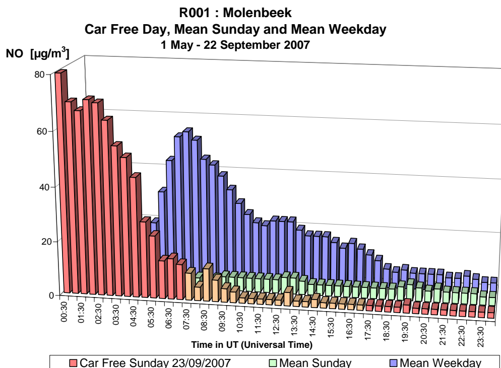
Fig. 13.a : NO à Molenbeek – Profil journalier du dimanche sans voiture 23-09-2007, d'un dimanche moyen et d'un jour ouvrable moyen de la période 'mai – septembre 2007'.
