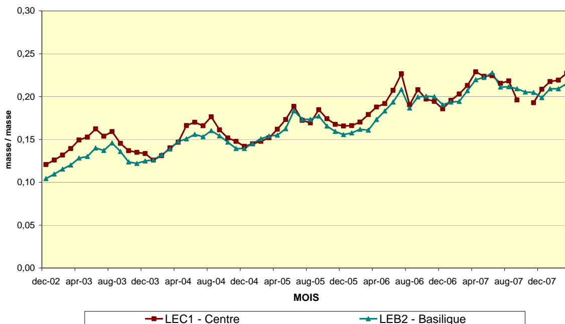
Fig. 11 : Évolution du rapport NO 2 /NO x dans les deux postes de mesure du tunnel Léopold II. Période – « Décembre 2002 – Mars 2008 »
