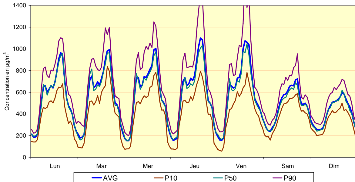
Fig. 22 : Poste de Mesure 41LEB2 (basilique) – Évolution hebdomadaire moyenne pour le NO 2 Période hivernale 2007 - 2008 et période estivale 2007
