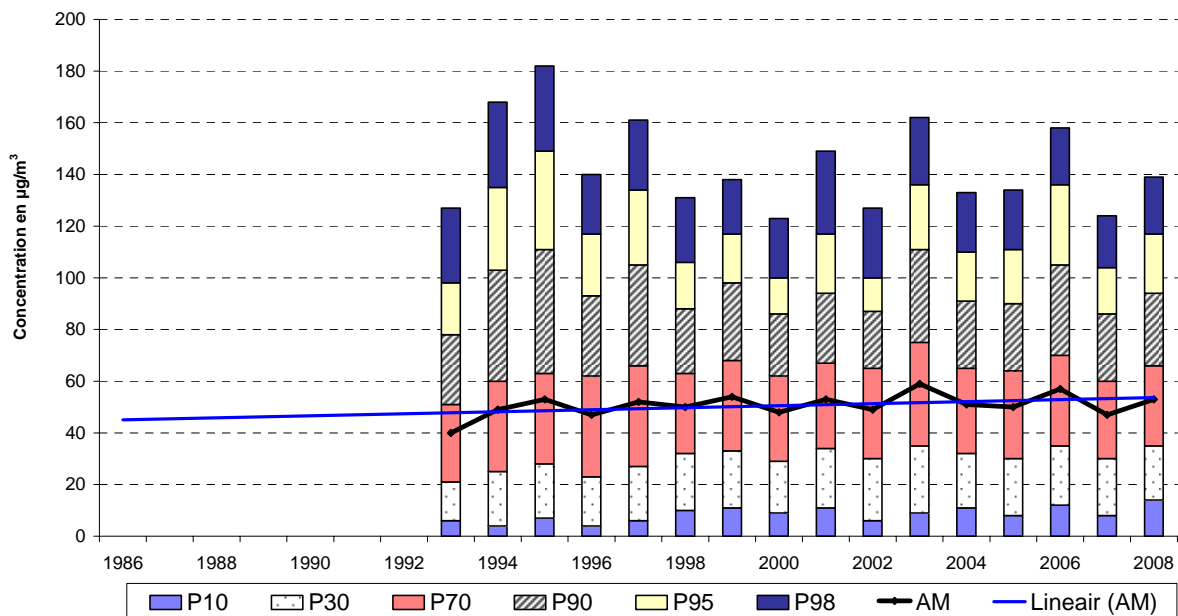
Fig. 34 : Berchem-Ste-Agathe - Évolution des Valeurs Horaires en Ozone (1993-2008) Période estivale « avril – septembre »
