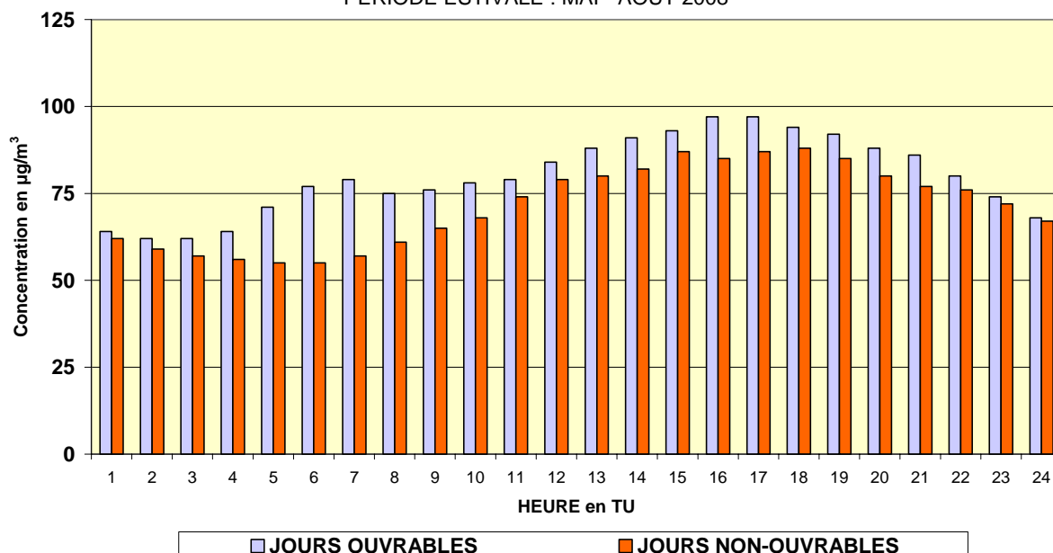
Fig. 70 : [O 3 + NO 2 ] – Évolution journalière moyenne les jours ouvrables et les jours non ouvrables Postes de mesure d'Uccle et de Haren (trafic) - Période « mai –août 2008 »
