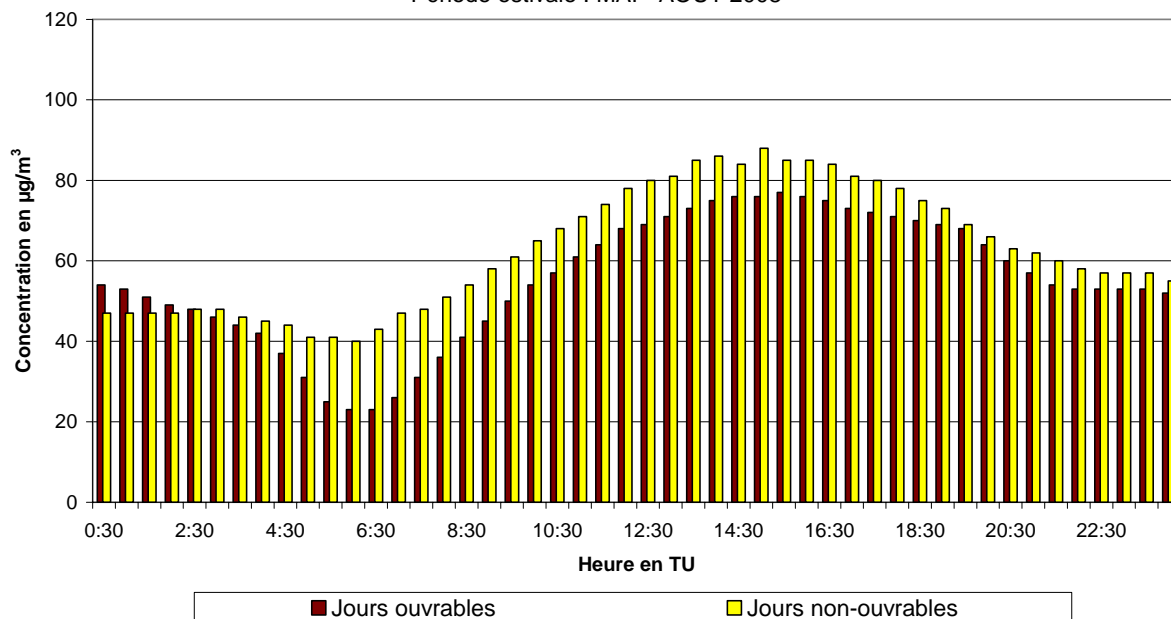
Fig. 51.a : Parlement Européen : Évolution journalière moyenne de la concentration en O 3 les jours ouvrables et non-ouvrables pendant la période mai - août 2008
