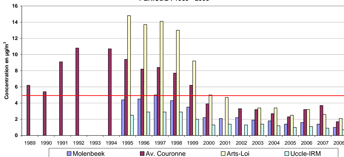
Fig. 28 : Benzène – Évolution de la concentration moyenne annuelle Période : janvier – décembre (1989-2007) 2008 : Janvier - Septembre
