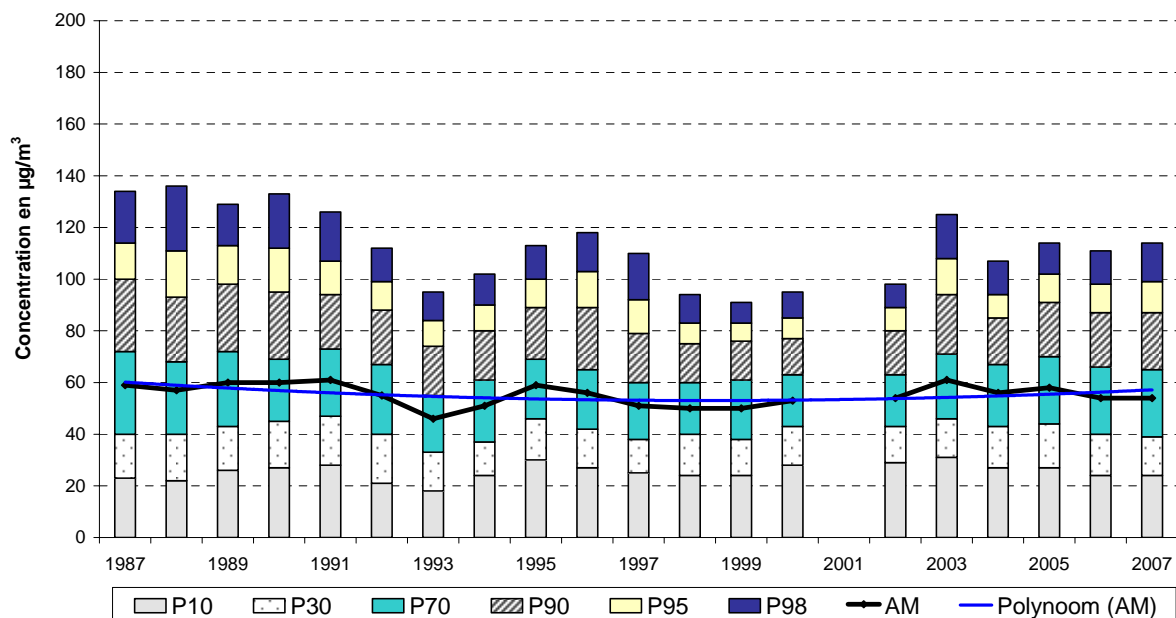
Fig. 74 : NO x à Ixelles – Avenue de la Couronne ( canyon street ) – Valeurs horaires Évolution à long terme - Périodes annuelles 1987 - 2007
