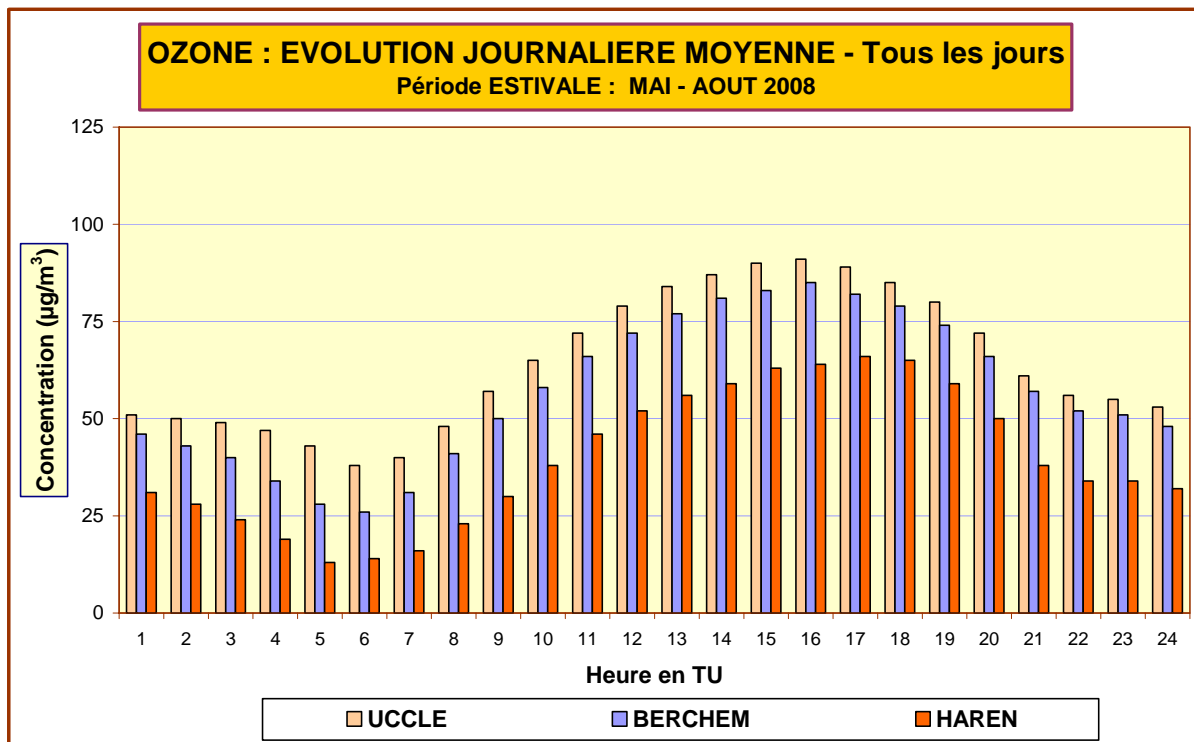
Fig. 66 : Ozone – Évolution journalière moyenne – Comparaison entre 3 postes de mesure Période « mai –août 2008 »
