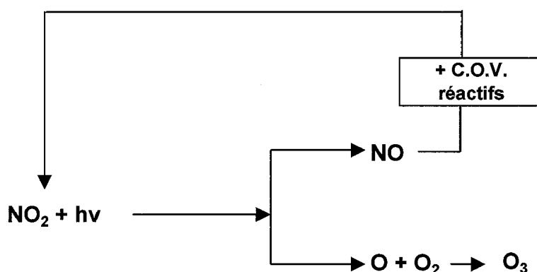
Fig. 64 : formation excessive d'ozone (schéma simplifié)
