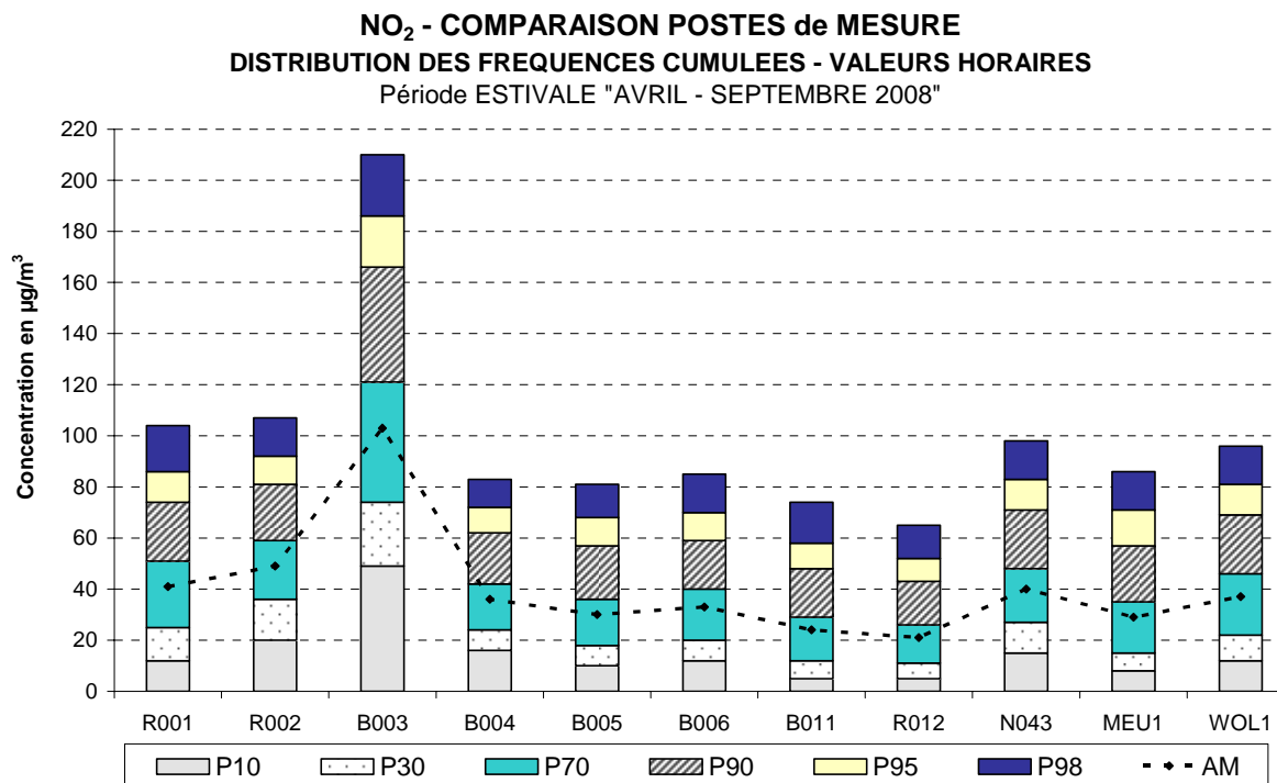
Fig.39 : NO 2 - Distribution de fréquences cumulées - valeurs horaires: avril - septembre 2008
