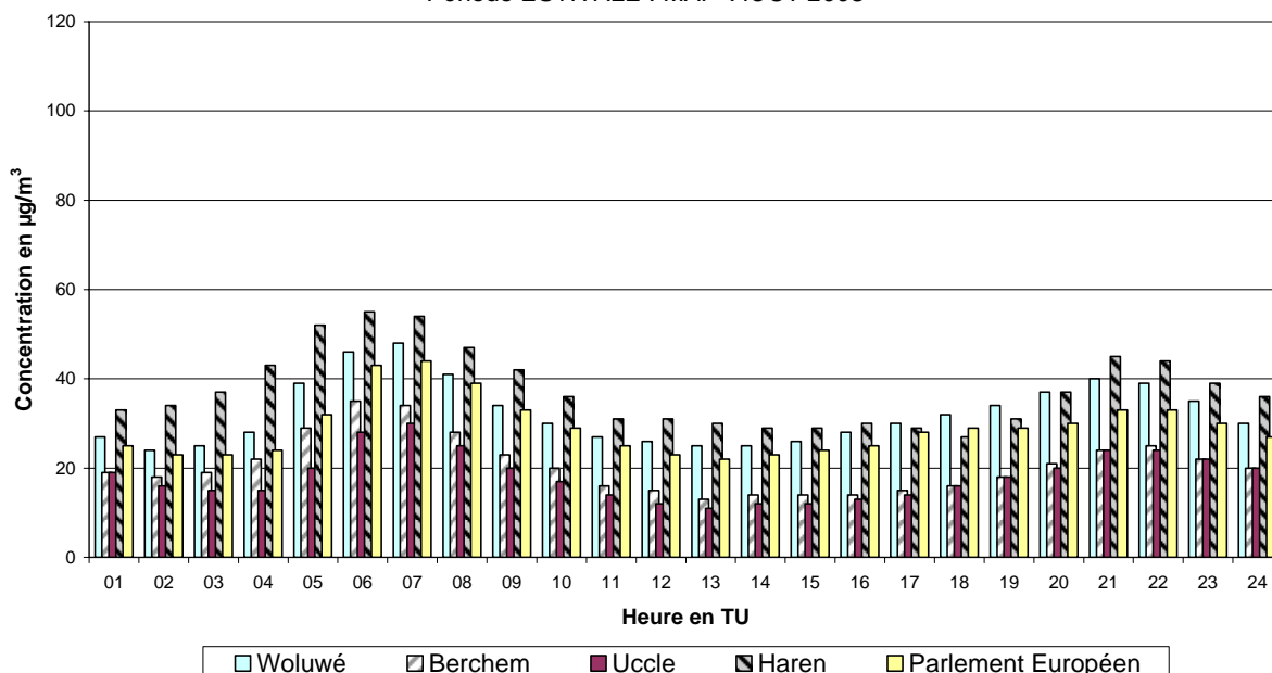
Fig. 9 : Évolution journalière moyenne des concentrations en NO 2 durant la période mai-août 2008
