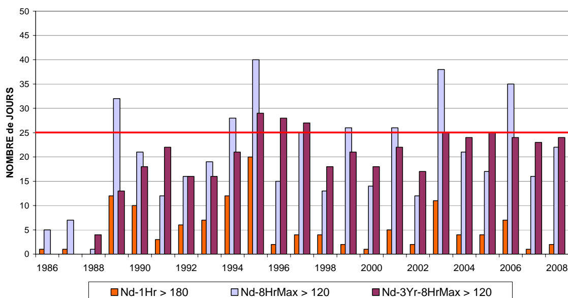
Fig. 19 : Ozone à Uccle : nombre de jours avec dépassements Périodes annuelles : 1 janvier – 31 décembre (1986 – 2007) Données partielles pour l'année 2008 (1 er janvier – 30 septembre)
