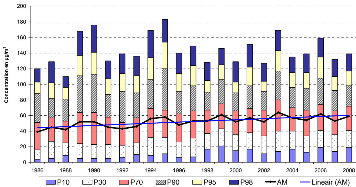
Fig. 33 : Uccle - Évolution des Valeurs Horaires en Ozone (1986-2008) Période estivale « avril – septembre »
