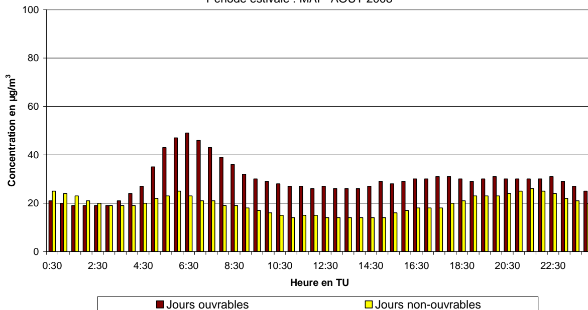
Fig. 53.a : Eastman-Belliard : Évolution journalière moyenne de la concentration en NO 2 les jours ouvrables et non-ouvrables pendant la période mai - août 2008
