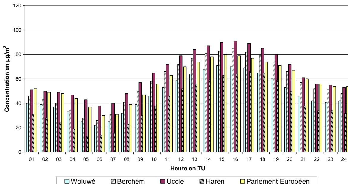
Fig. 8 : Évolution journalière moyenne des concentrations en O 3 durant la période mai-août 2008
