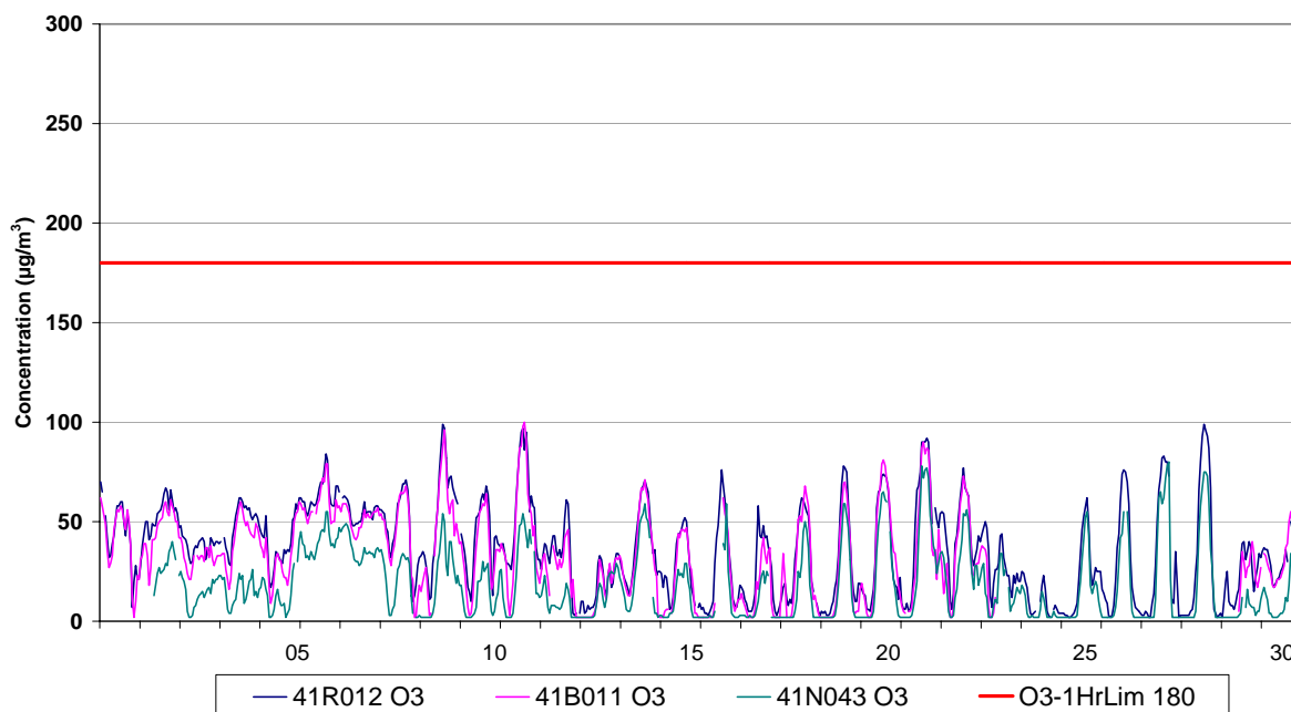
Fig. 7 : Évolution des concentrations horaires en Ozone – Uccle, Berchem et Haren – Septembre 2008
