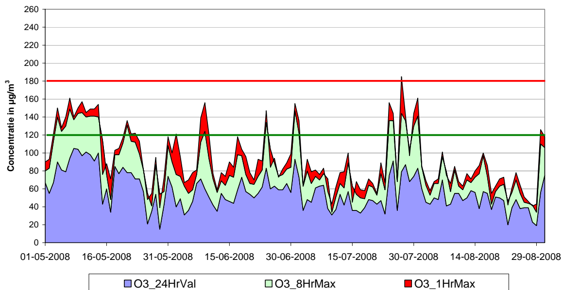
Fig. 22 : Ozone – Évolution Valeur Journalière (24HrVal), valeur maximale sur 8 heures (8HrMax) et valeur maximale horaire (1HrMax). Période : mai – août 2008. Postes de mesure à Uccle et Berchem-Ste-Agathe
