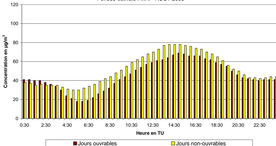
Fig. 50.a : Woluwé-St-Lambert : Évolution journalière moyenne de la concentration en O 3 les jours ouvrables et non-ouvrables pendant la période mai - août 2008
