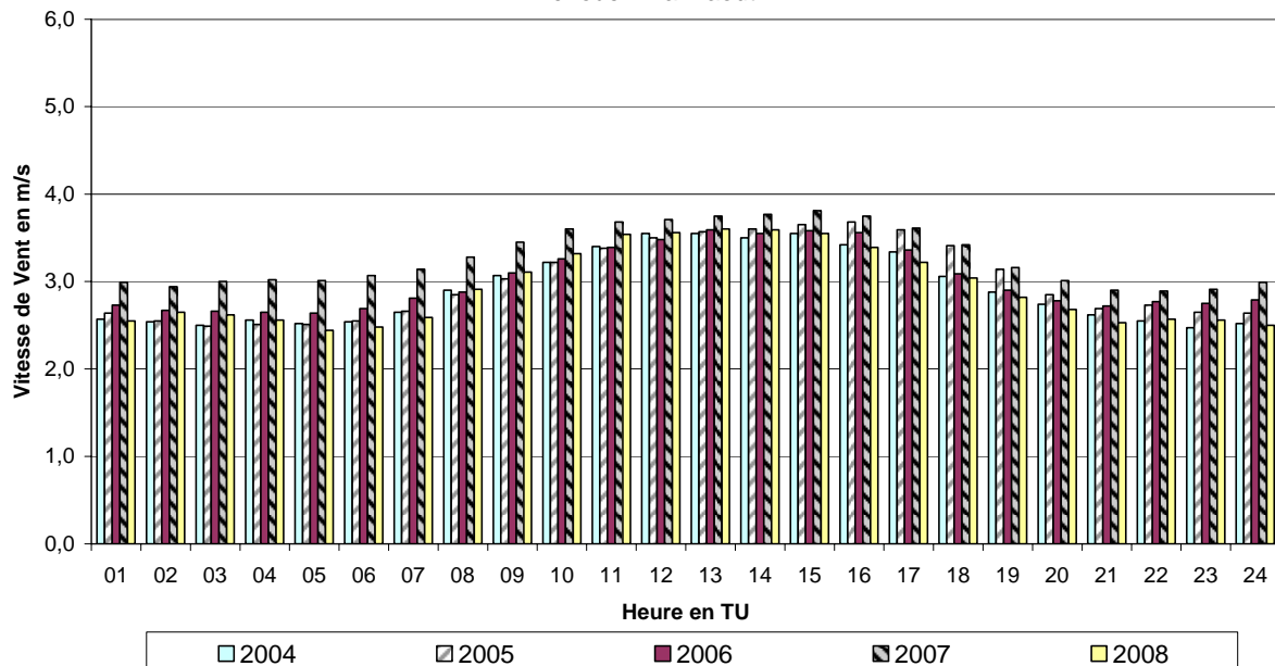
Fig. 38 : Vitesse de vent - évolution journalière moyenne Périodes estivales « mai – août » 2004, 2005, 2006, 2007 et 2008
