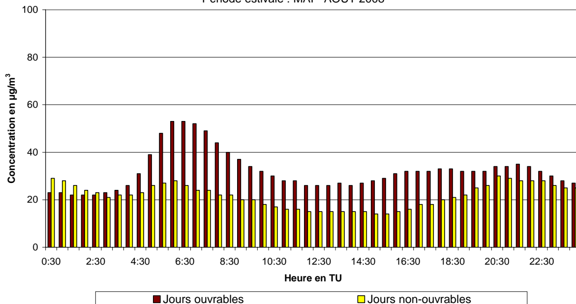
Fig. 51.b : Parlement Européen : Évolution journalière moyenne de la concentration en NO 2 les jours ouvrables et non-ouvrables pendant la période mai – août 2008
