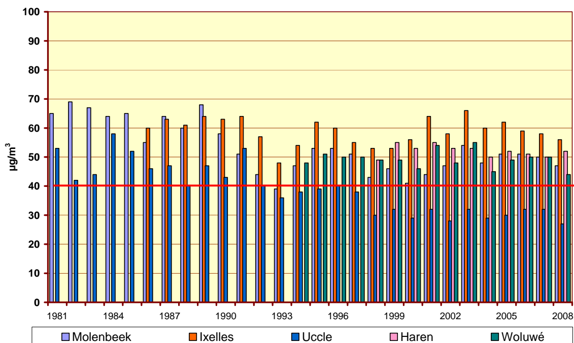
Fig. 26 : NO 2 – Évolution de la concentration moyenne annuelle ( tous les jours ) et de la concentration moyenne les ' jours ouvrables ' – Période 1981 - 2008
