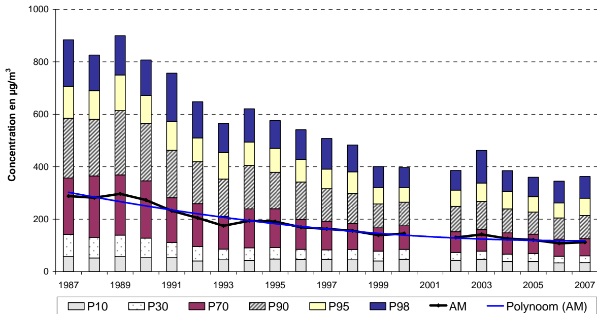
Fig. 73 : NO x à Ixelles – Avenue de la Couronne ( canyon street ) – Valeurs horaires Évolution à long terme - Périodes annuelles 1987 - 2007
