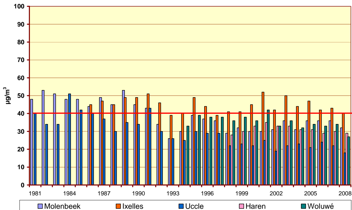
Fig. 27 : NO 2 – Évolution de la concentration moyenne les 'Samedis' et 'Dimanches' Période 1981 - 2008
