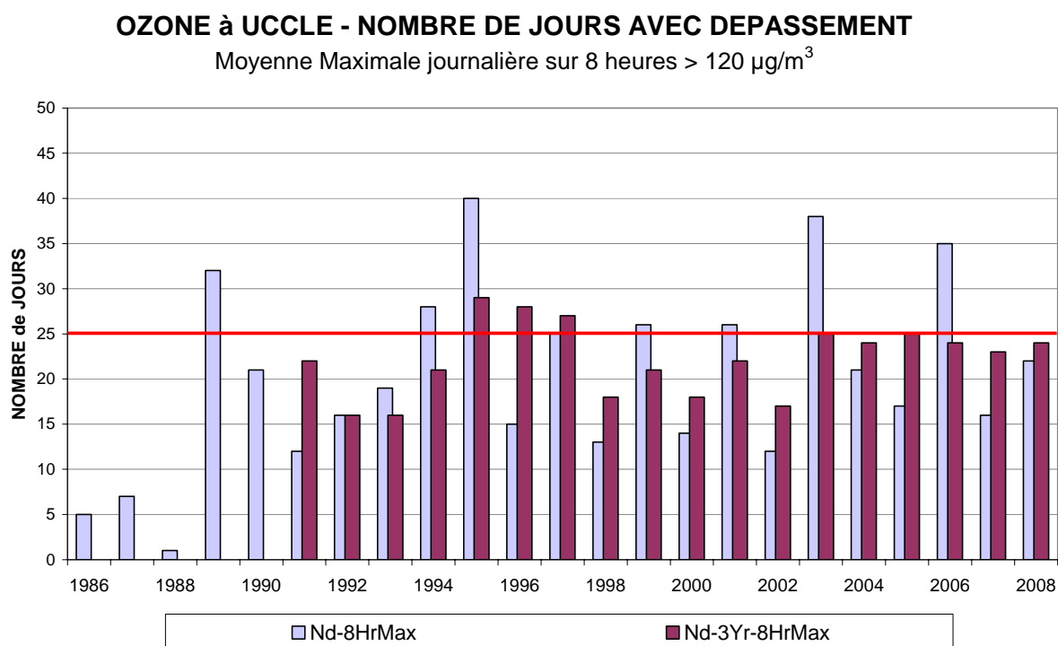
Fig. 12: Ozone – évolution du nombre de jours avec dépassement à Uccle. Valeur cible pour la Santé Publique. Valeur maximale sur 8 heures > 120 \mu\text{g}/\text{m}^3 . Période : Janvier – Décembre (1986-2007). [2008] : Janvier - Septembre
