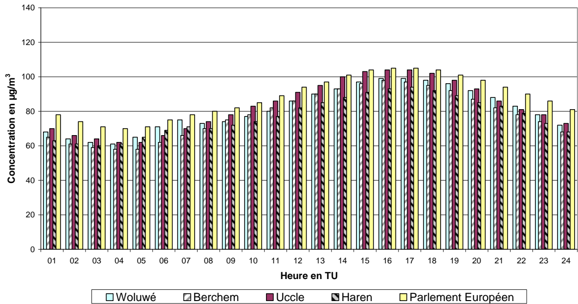
Fig. 10 : Évolution journalière moyenne des concentrations en [O 3 + NO 2 ], exprimées en équivalent O 3 , durant la période mai – août 2008
