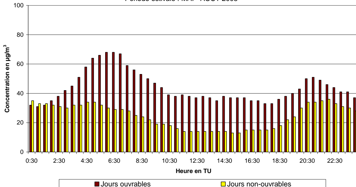
Fig. 49.b : Haren : Évolution journalière moyenne de la concentration en NO 2 les jours ouvrables et non-ouvrables pendant la période mai – août 2008
