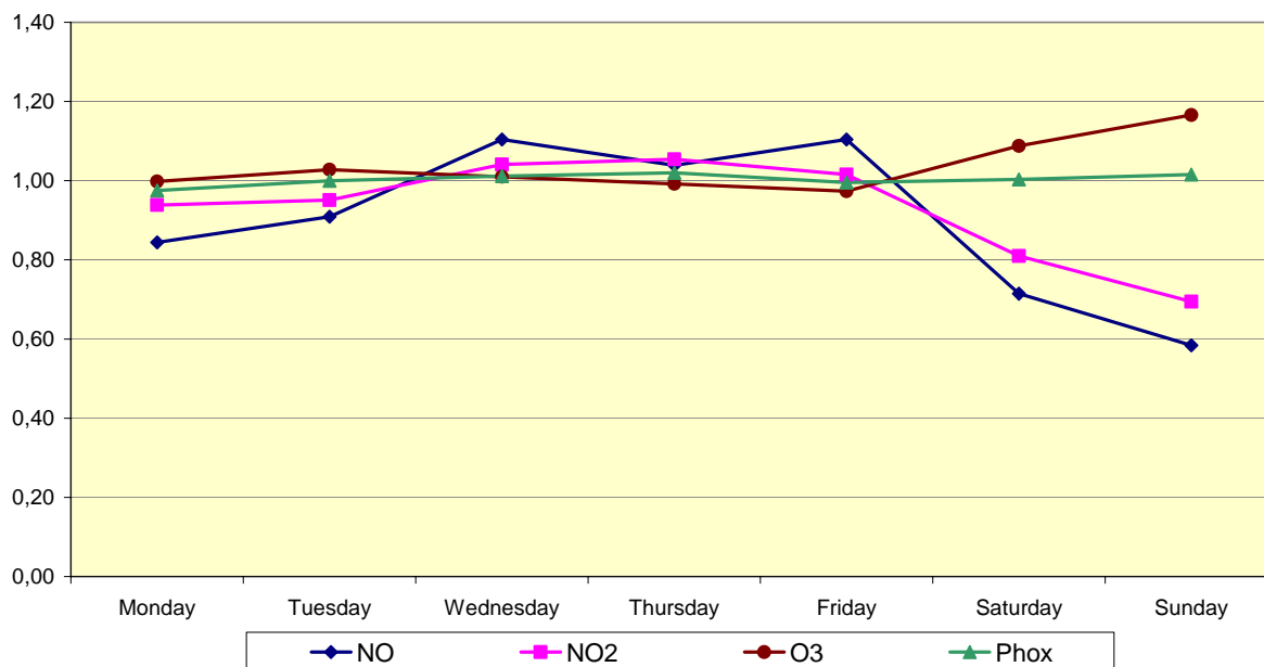
Fig. 59.a : Poste de mesure à Uccle – Profil hebdomadaire moyen des concentrations en NO, NO 2 , O 3 et [NO 2 +O 3 ] sur trois périodes estivales successives : 'avril – septembre' 2006, 2007 et 2008
