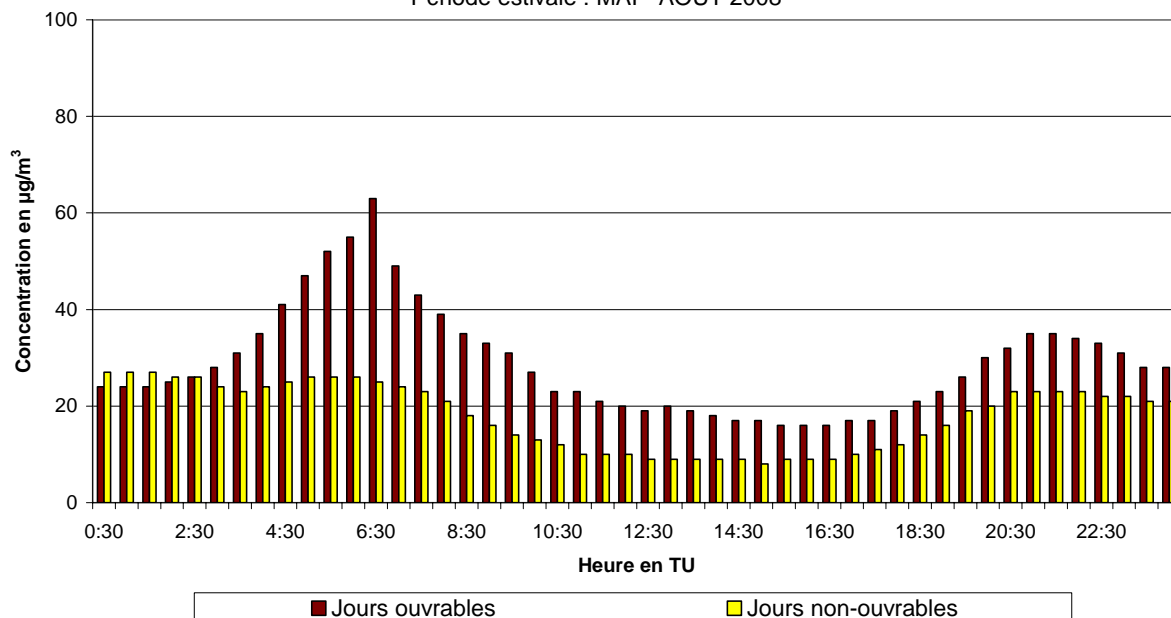
Fig. 53.b : Parc Meudon : Évolution journalière moyenne de la concentration en NO 2 les jours ouvrables et non-ouvrables pendant la période mai – août 2008
