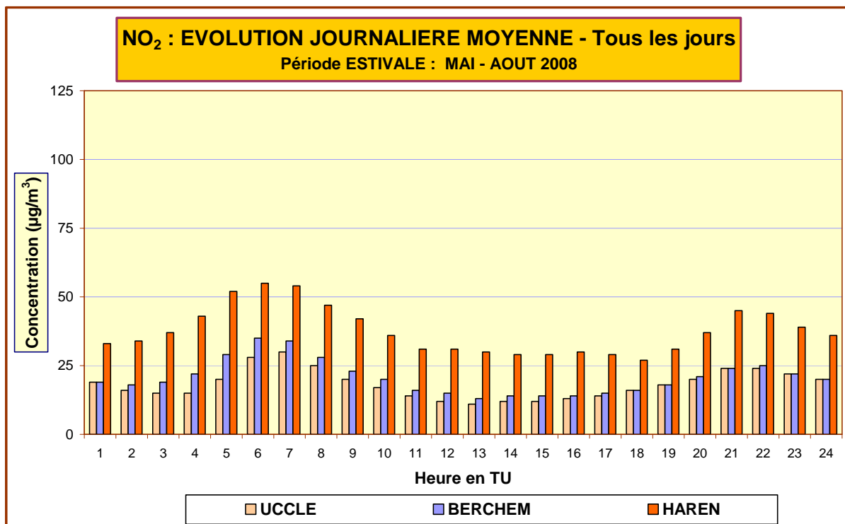
Fig. 67 : NO 2 – Évolution journalière moyenne – Comparaison entre 3 postes de mesure Période « mai –août 2008 »
