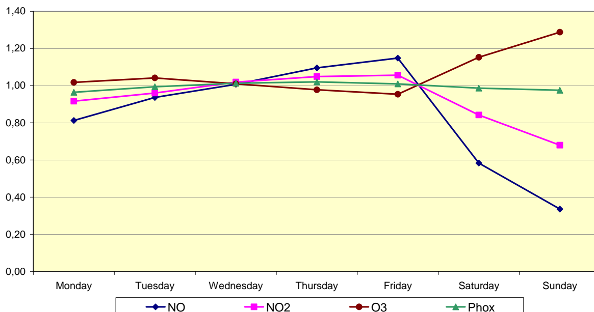
Fig. 59.b : Poste de mesure à Molenbeek – Profil hebdomadaire moyen des concentrations en NO, NO 2 , O 3 et [NO 2 +O 3 ] sur trois périodes estivales successives : 'avril – septembre' 2006, 2007 et 2008
