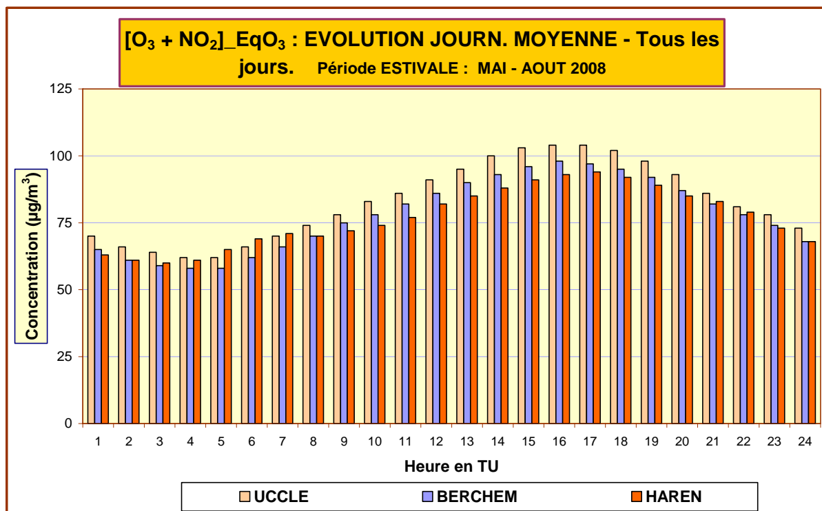
Fig. 68 : [O 3 + NO 2 ] – Évolution journalière moyenne – Comparaison entre 3 postes de mesure Période « mai –août 2008 »
