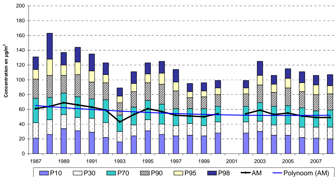
Fig. 40 : Ixelles – Évolution de Valeurs Horaires en NO 2 Période estivale « avril – septembre » (1991-2008)
