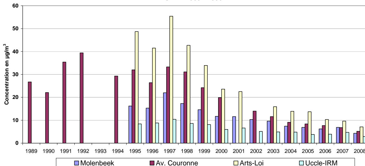
Fig. 29 : Toluène – Évolution de la concentration moyenne annuelle Période : janvier – décembre (1989-2007) 2008 : Janvier - Septembre
