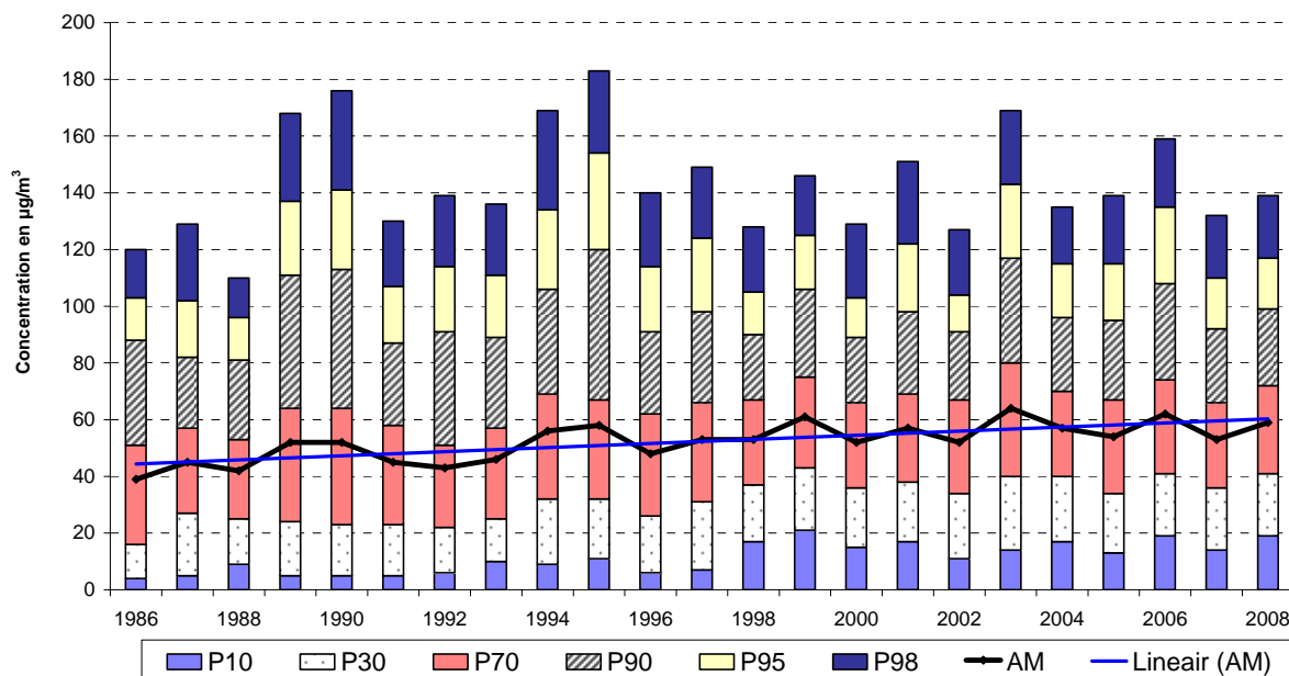
Fig. 71 : Ozone à Uccle – Valeurs horaires –évolution à long terme Périodes estivales 1986 - 2008
