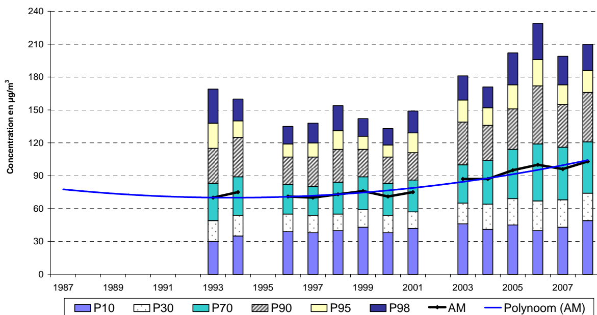
Fig. 41 : Arts-Loi – Évolution de Valeurs Horaires en NO 2 Période estivale « avril – septembre » (1993-2008)
