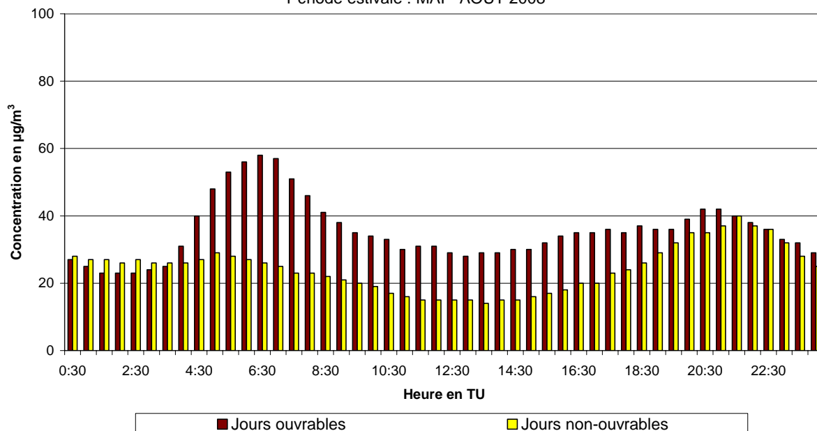
Fig. 50.b : Woluwé-St-Lambert : Évolution journalière moyenne de la concentration en NO 2 les jours ouvrables et non-ouvrables pendant la période mai – août 2008
