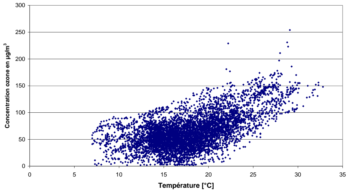
Fig. 42 : Uccle : Concentrations en ozone en fonction de la température (mai - août 2008)
