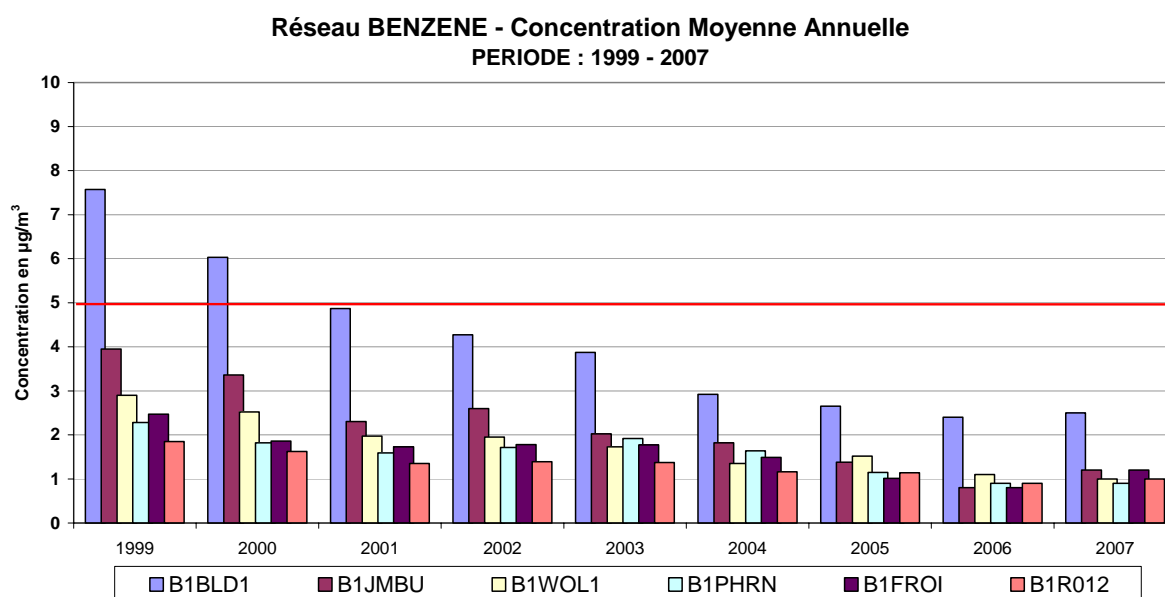
Fig. 30 : Réseau Benzène – Évolution de la concentration moyenne annuelle dans quelques postes de mesure. Période 1999 - 2007
