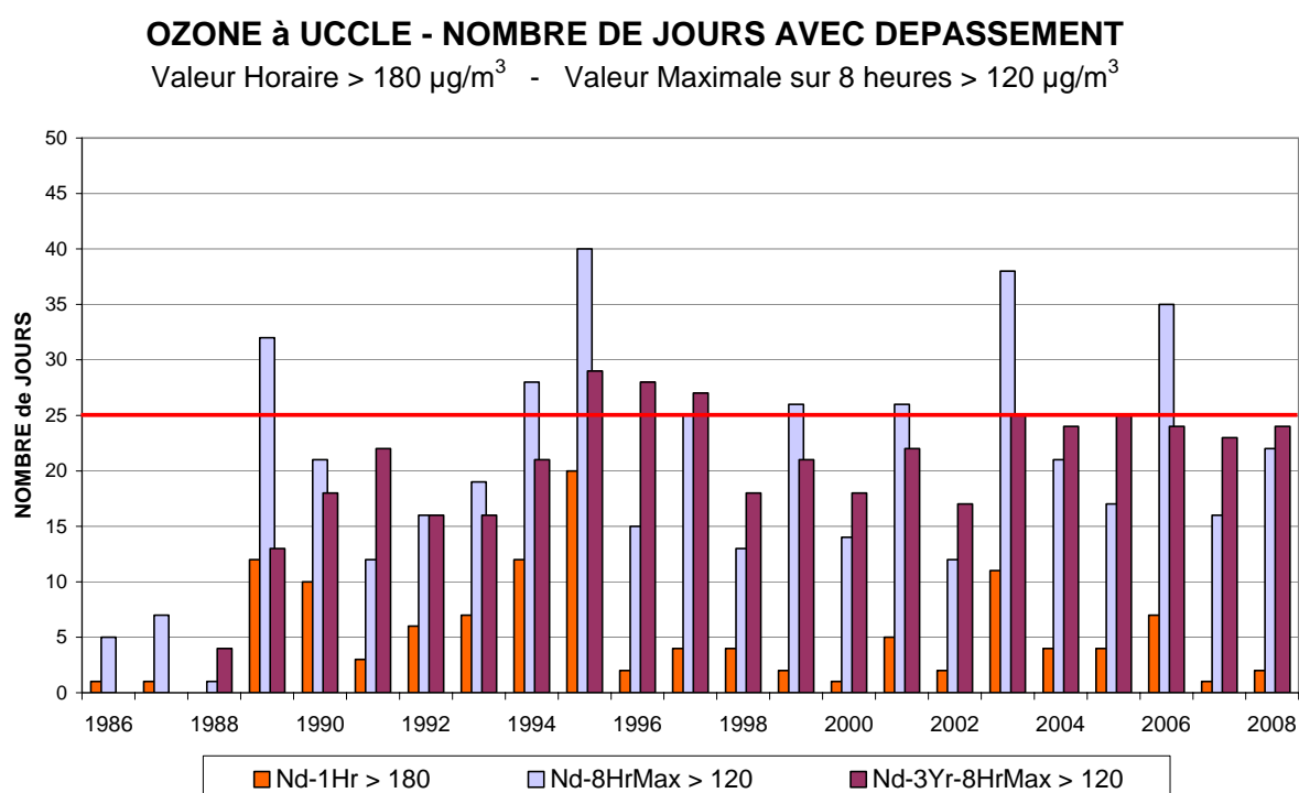
Fig. 63 : Ozone – nombre de jours avec dépassements à Uccle Nombre de jours avec des valeurs horaires supérieures à 180 \mu\text{g}/\text{m}^3 et des valeurs maximales sur 8 heures supérieures à 120 \mu\text{g}/\text{m}^3 (par an et moyenné sur 3 ans)
