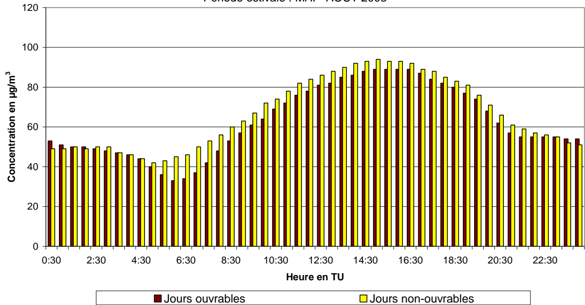
Fig. 46.a : Uccle : Évolution journalière moyenne de la concentration en O 3 les jours ouvrables et non-ouvrables pendant la période mai - août 2008
