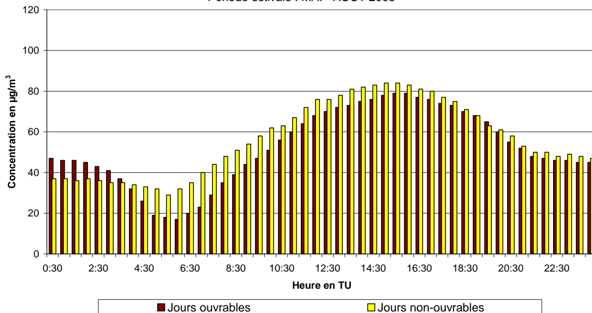
Fig. 52.a : Ste-Catherine : Évolution journalière moyenne de la concentration en O 3 les jours ouvrables et non-ouvrables pendant la période mai - août 2008
