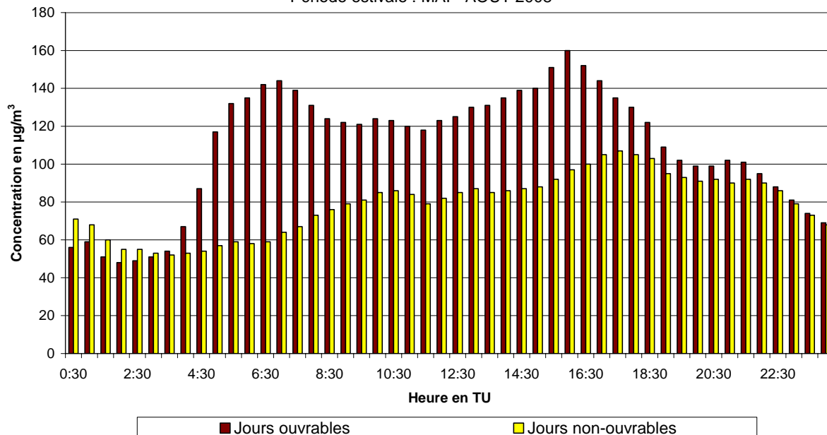
Fig. 54.b : Arts-Loi : Évolution journalière moyenne de la concentration en NO 2 les jours ouvrables et non-ouvrables pendant la période mai - août 2008
