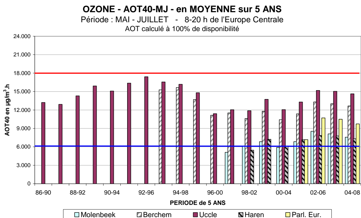
Fig. 62 : Évolution AOT-MJ, moyenné sur 5 ans
