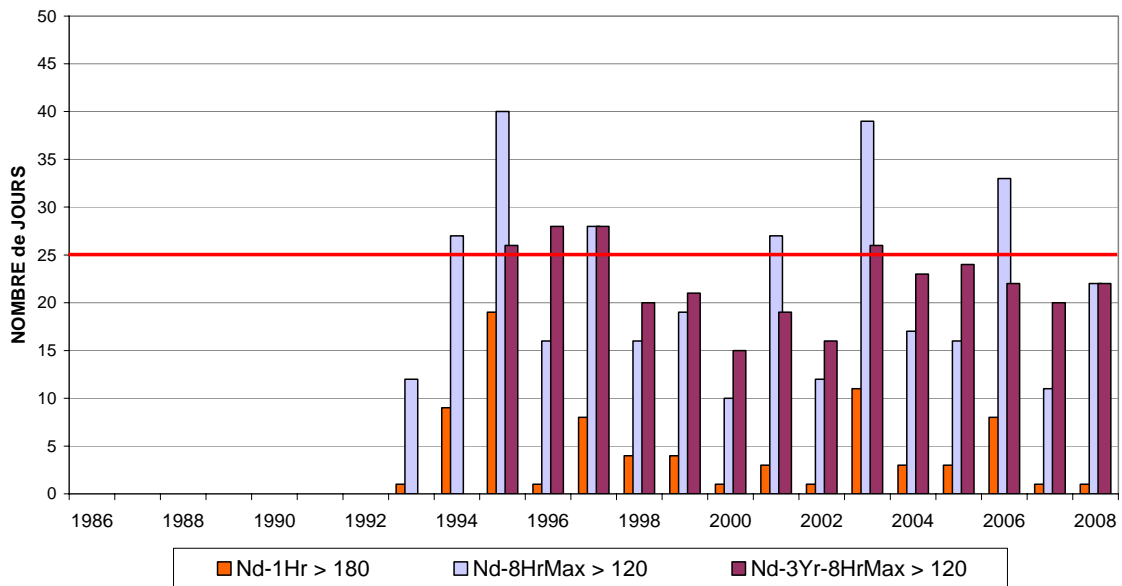
Fig. 20 : Ozone à Berchem : nombre de jours avec dépassements Périodes annuelles : 1 janvier – 31 décembre (1986 – 2007) Données partielles pour l'année 2008 (1 er janvier – 30 septembre)
