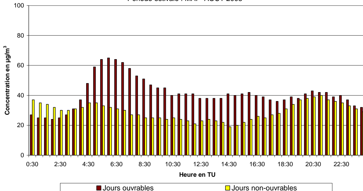
Fig. 48.b : Molenbeek : Évolution journalière moyenne de la concentration en \text{NO}_2 les jours ouvrables et non-ouvrables pendant la période mai – août 2008
