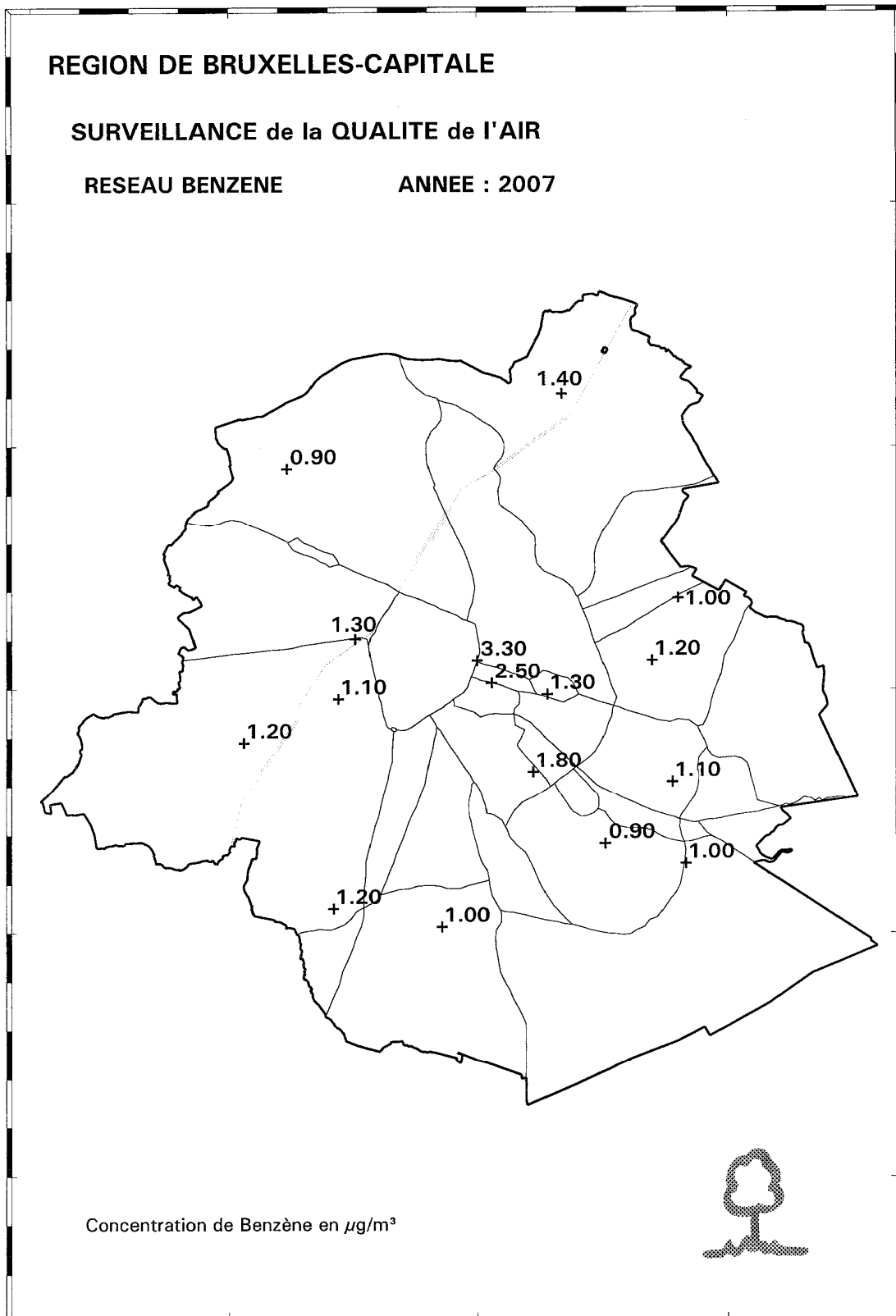
Fig. 31 : Benzène – Distribution spatiale de concentration moyenne annuelle en 2007
