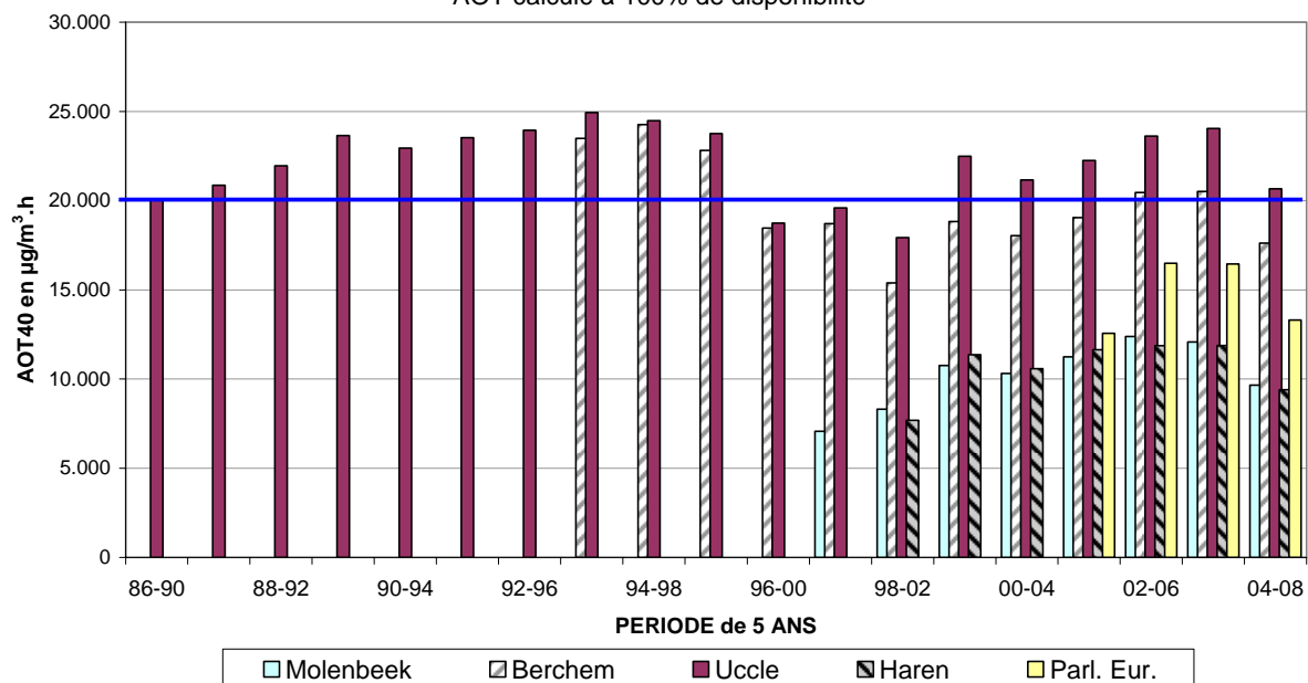
Fig. 16 : Évolution AOT40-AS dans le temps (1986-2008) AOT40 pour la période Avril – Septembre, 8-20 h d'Europe centrale Résultats par an et moyenné sur 5 ans
