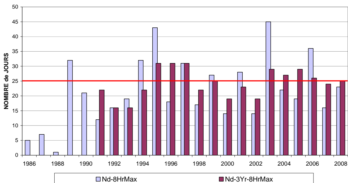
Fig. 14: Ozone – évolution du nombre de jours avec dépassement dans la Région. Valeur cible pour la Santé Publique. Valeur maximale sur 8 heures > 120 µg/m 3 . Période : Janvier – Décembre (1986-2007). [2008] : Janvier - Septembre
