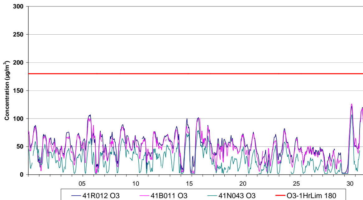
Fig. 6 : Évolution des concentrations horaires en Ozone – Uccle, Berchem et Haren – Août 2008
