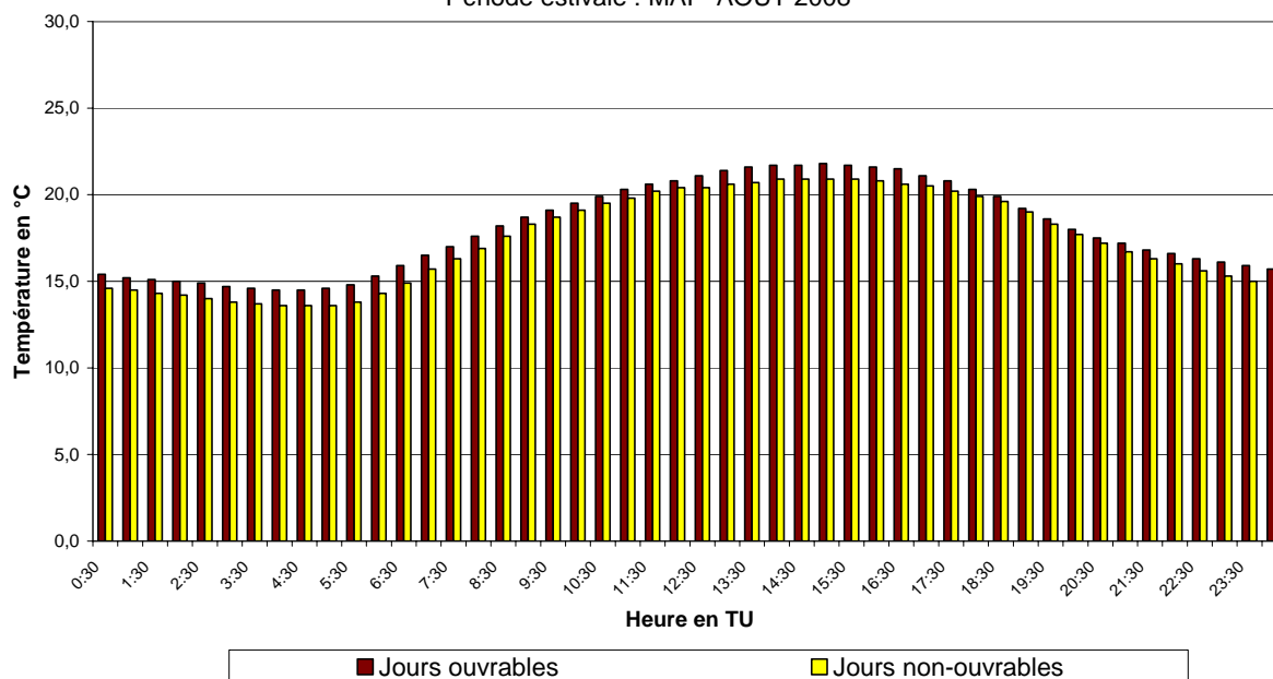
Fig. 55.a : Uccle : Évolution journalière moyenne de la température les jours ouvrables et non-ouvrables pendant la période mai – août 2008
