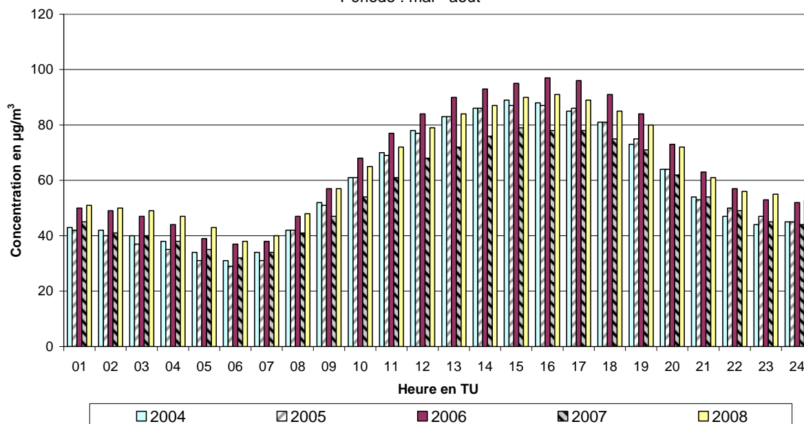
Fig. 35 : Évolution journalière moyenne en ozone à Uccle (R012) Comparaison des niveaux durant les périodes estivales récentes (2004 à 2008)
