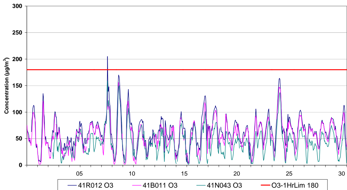
Fig. 4 : Évolution des concentrations horaires en Ozone – Uccle, Berchem et Haren – Juin 2008
