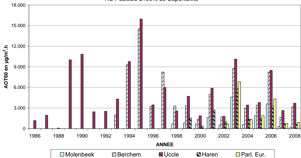
Fig. 24: Évolution AOT60 dans le temps (1986-2008)
