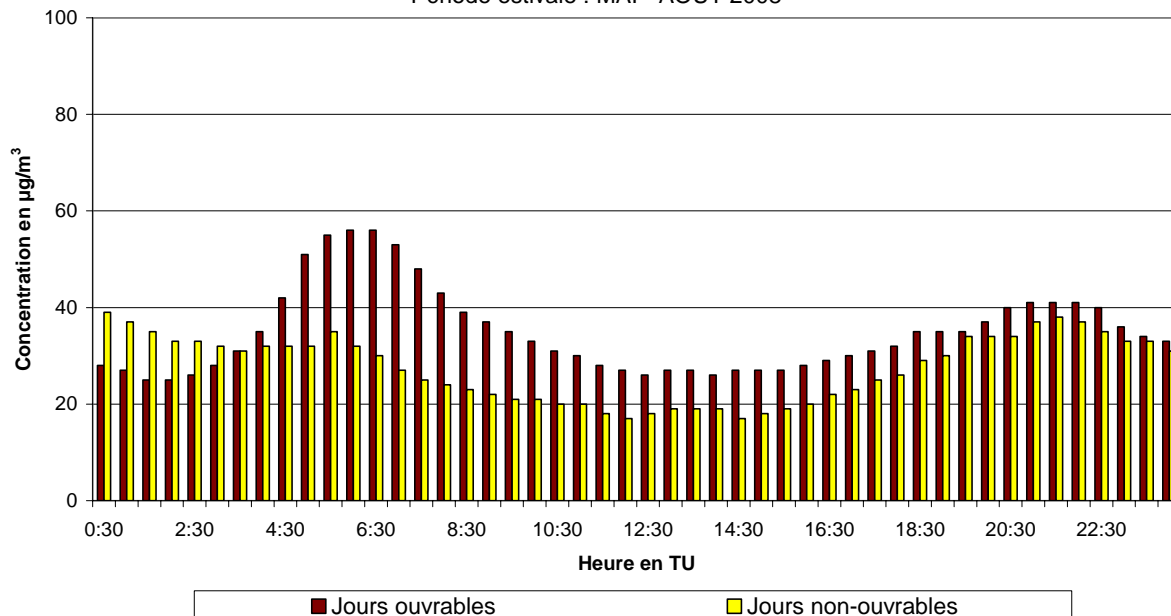
Fig. 52.b : Ste-Catherine : Évolution journalière moyenne de la concentration en NO 2 les jours ouvrables et non-ouvrables pendant la période mai – août 2008
