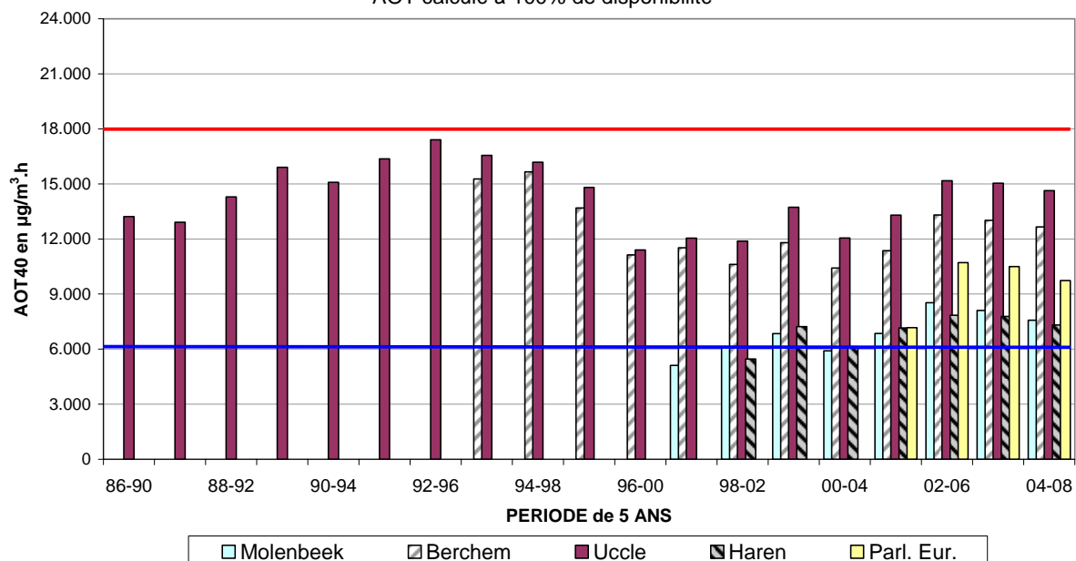
Fig. 15 : Évolution AOT40-MJ dans le temps (1986-2008) AOT40 pour la période Mai – Juillet, 8-20 h d'Europe centrale Résultats par an et moyenné sur 5 ans
