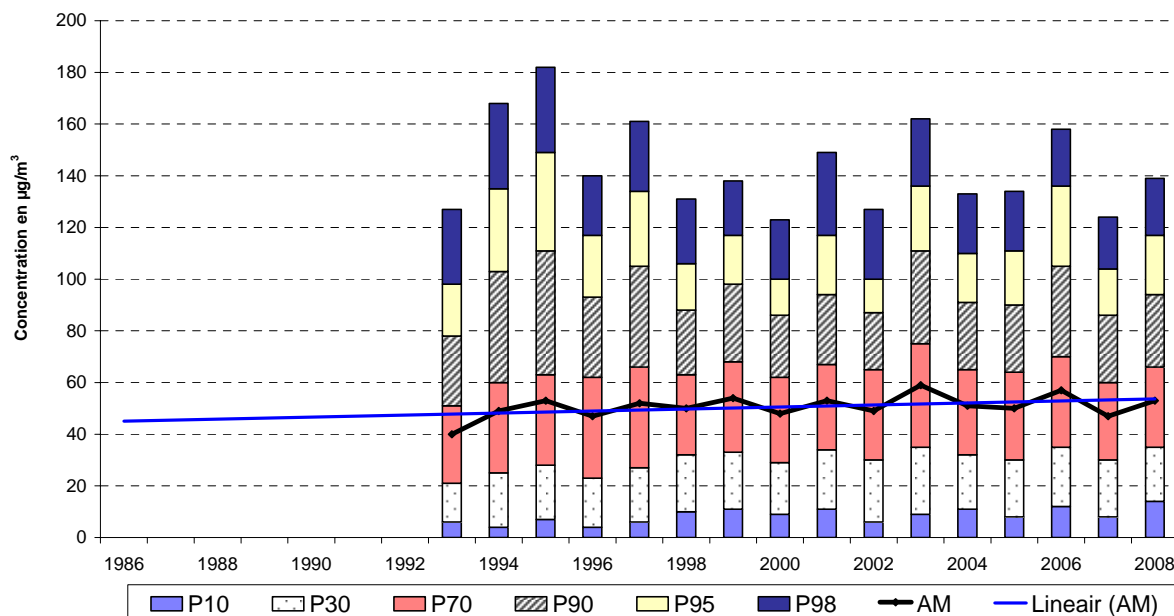
Fig. 72 : Ozone à Berchem-Ste-Agathe – Valeurs horaires –évolution à long terme Périodes estivales 1993 - 2008
