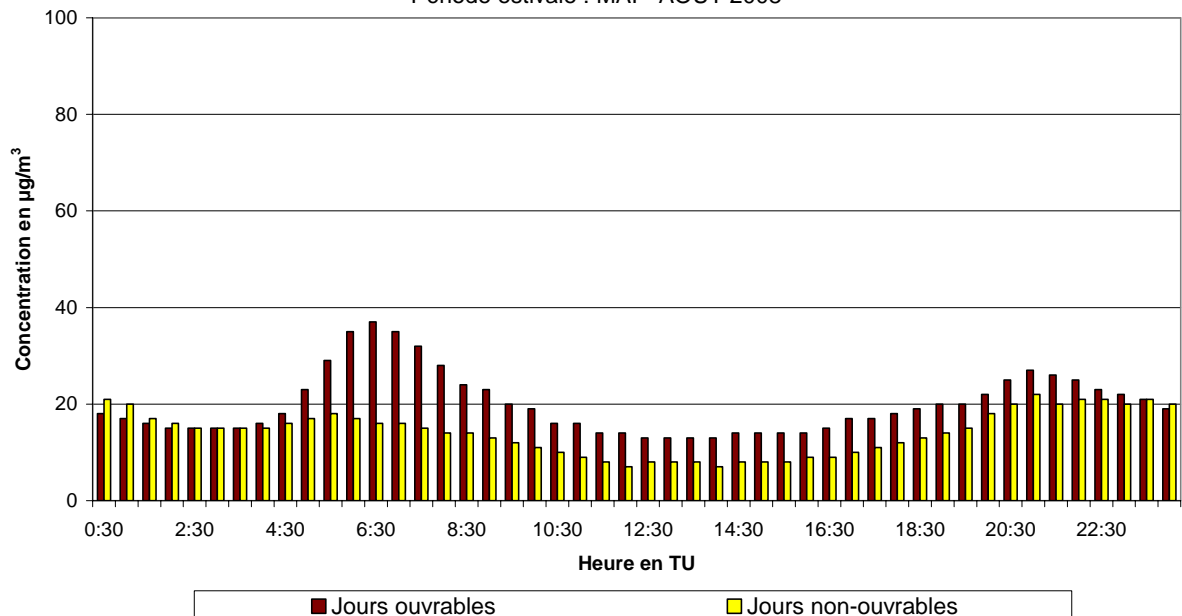
Fig. 46.b : Uccle : Évolution journalière moyenne de la concentration en NO 2 les jours ouvrables et non-ouvrables pendant la période mai – août 2008
