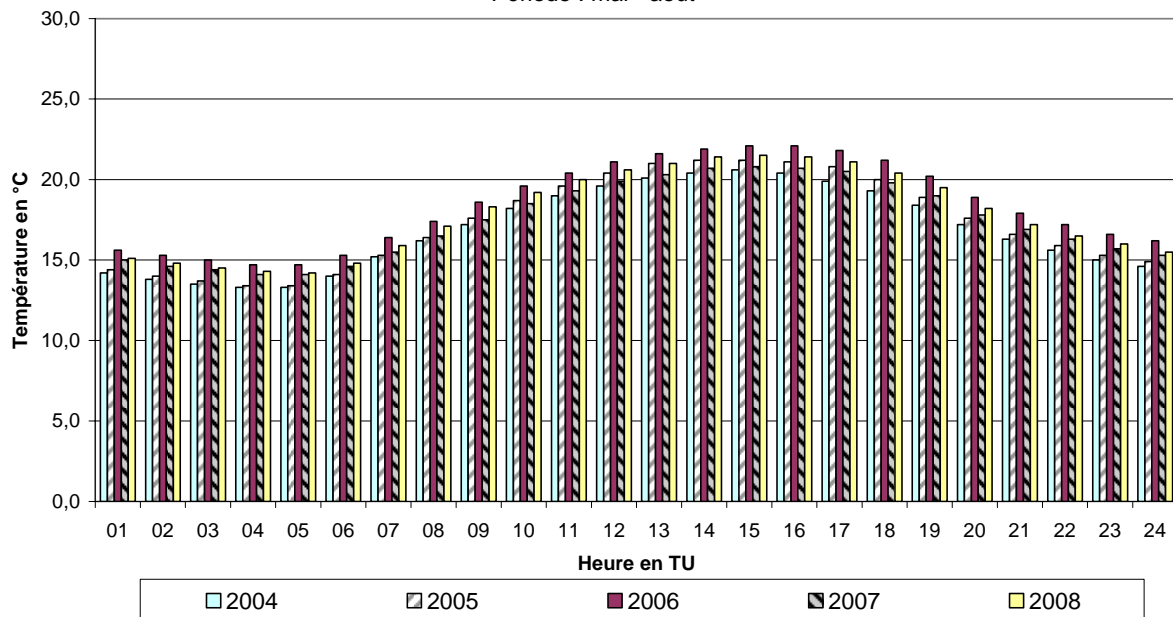
Fig. 37 : Température - évolution journalière moyenne Périodes estivales « mai – août » 2004, 2005, 2006, 2007 et 2008
