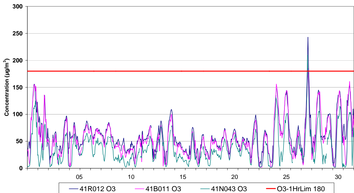
Fig. 5 : Évolution des concentrations horaires en Ozone – Uccle, Berchem et Haren – Juillet 2008
