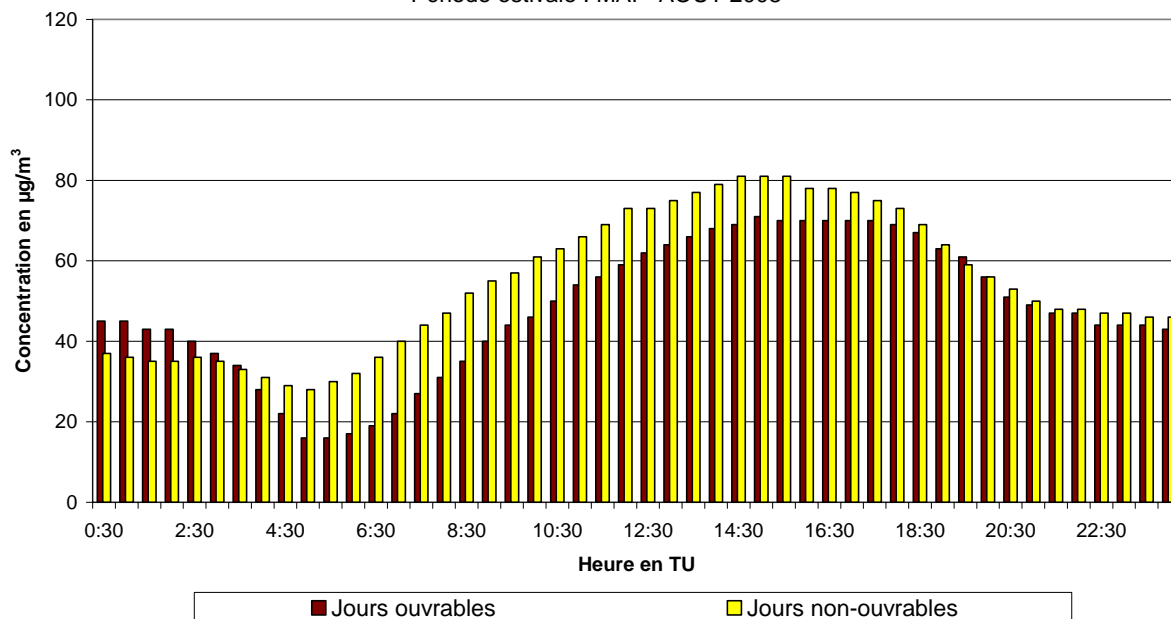
Fig. 48.a : Molenbeek : Évolution journalière moyenne de la concentration en \text{O}_3 les jours ouvrables et non-ouvrables pendant la période mai- août 2008
