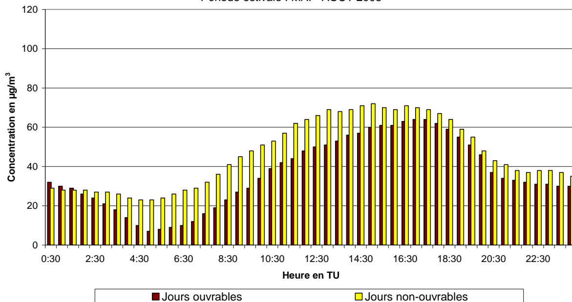
Fig. 49.a : Haren : Évolution journalière moyenne de la concentration en O 3 les jours ouvrables et non-ouvrables pendant la période mai - août 2008
