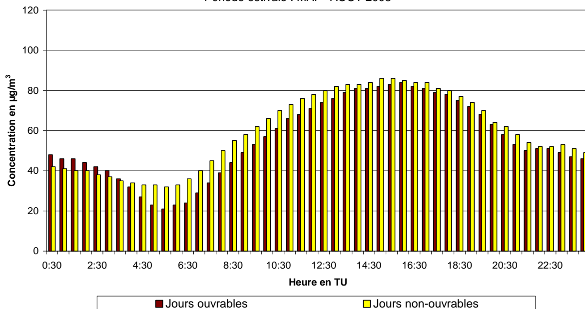
Fig. 47.a : Berchem-Ste-Agathe : Évolution journalière moyenne de la concentration en \text{O}_3 les jours ouvrables et non-ouvrables pendant la période mai - août 2008
