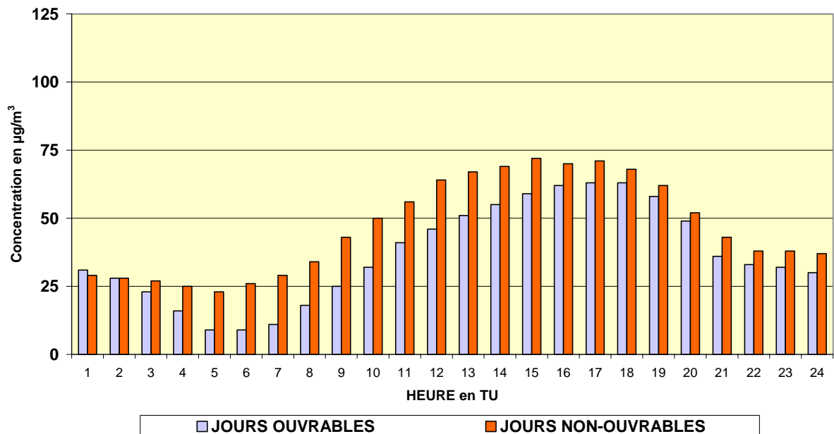
Fig. 69 : Ozone – Évolution journalière moyenne les jours ouvrables et les jours non ouvrables Postes de mesure d'Uccle et de Haren (trafic) - Période « mai –août 2008 »
