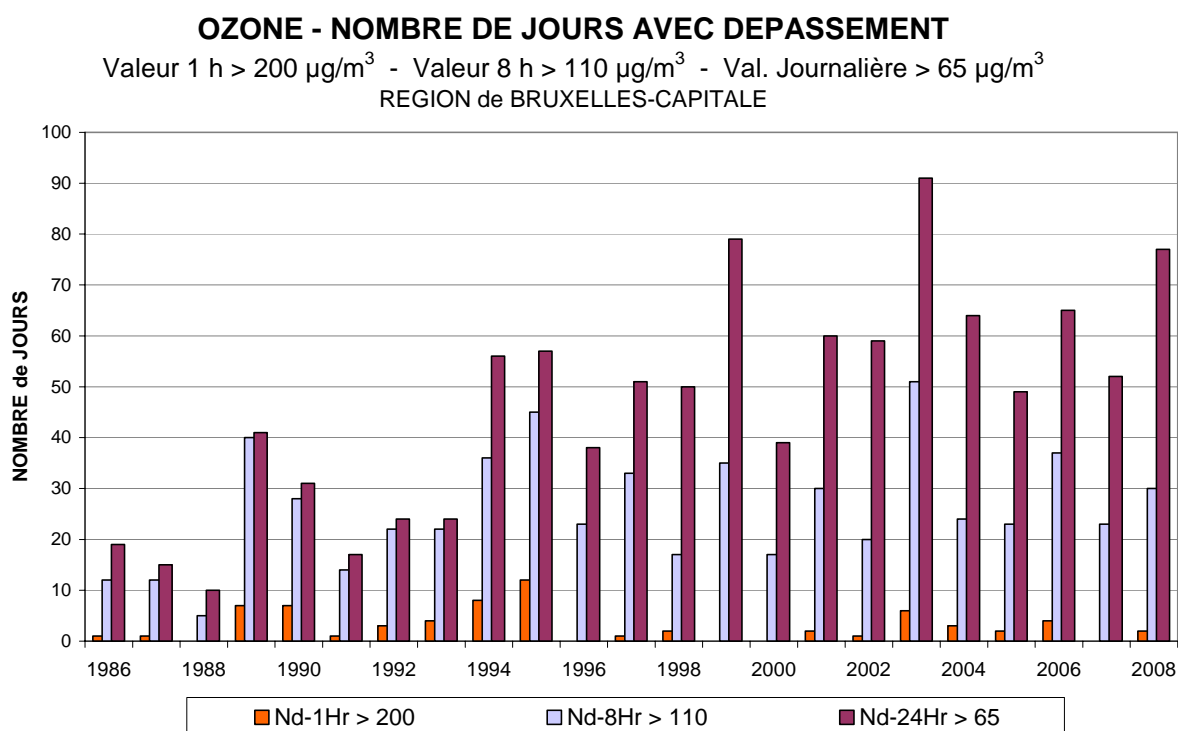
Fig. 25 : Ozone : nombre de jours avec dépassements (directive 92/72/CE) Période : janvier - décembre (1986 à 2007) 2008 : Janvier - Septembre
