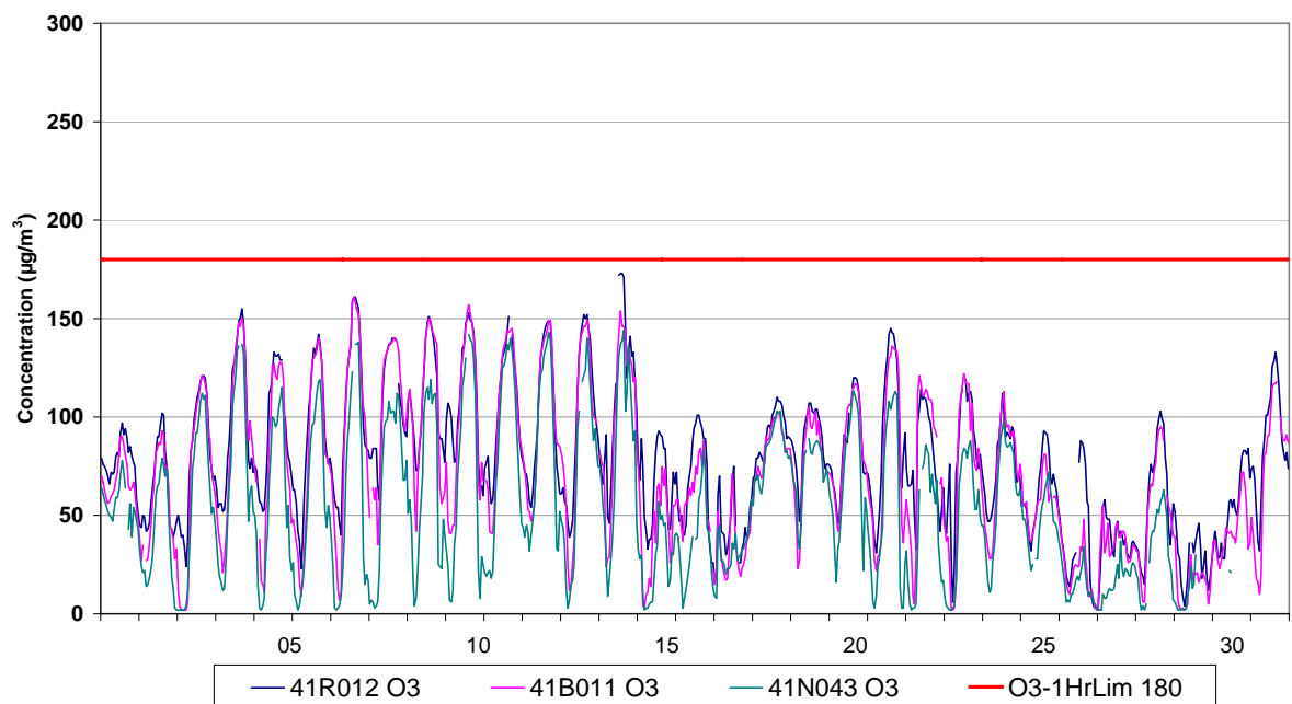
Fig. 3 : Évolution des concentrations horaires en Ozone – Uccle, Berchem et Haren – Mai 2008
