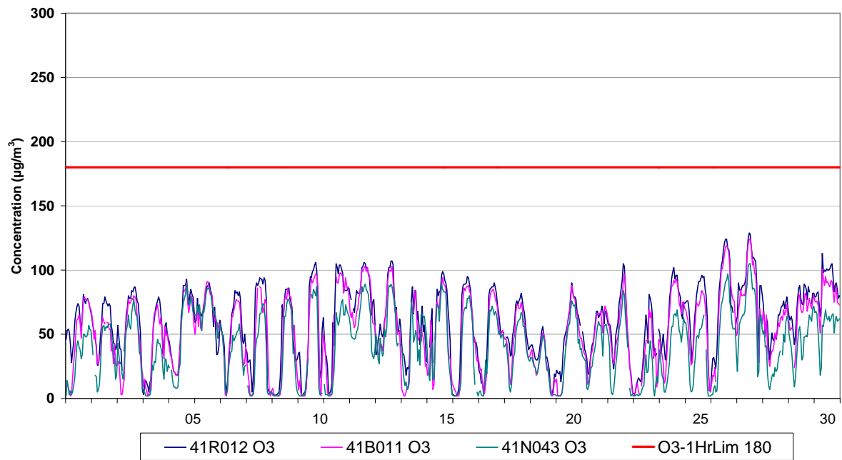
Fig. 2 : Évolution des concentrations horaires en Ozone – Uccle, Berchem et Haren – Avril 2008
