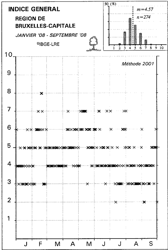
Fig. 60 : Les sous-indices pour NO 2 , O 3 et PM10 - Indice général (2008)
