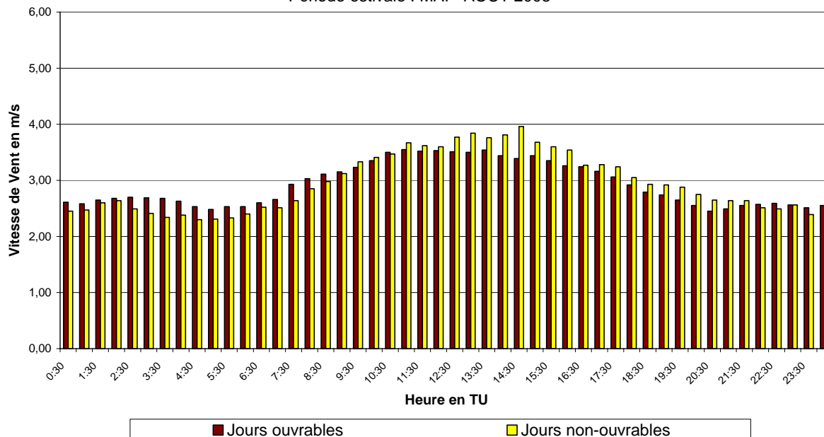
Fig. 55.b : Uccle : Évolution journalière moyenne de la vitesse de vent les jours ouvrables et non-ouvrables pendant la période mai – août 2008
