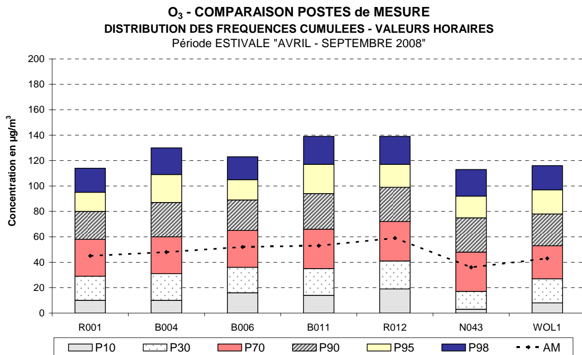
Fig. 32 : Ozone - Distribution de fréquences cumulées - valeurs horaires: avril - septembre 2008
