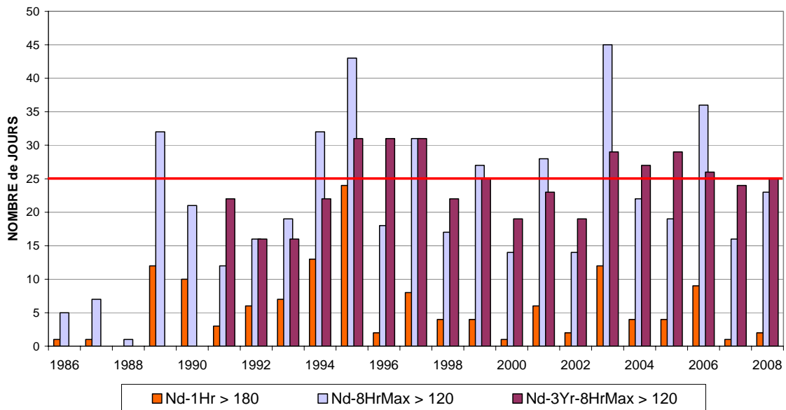
Fig. 21 : Ozone : nombre de jours avec dépassements en Région de Bruxelles-Capitale Périodes annuelles : 1 janvier – 31 décembre (1986 – 2007) Données partielles pour l'année 2008 (1 er janvier – 30 septembre)
