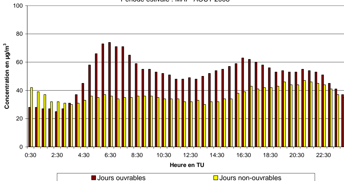
Fig. 54.a : Avenue de la Couronne à Ixelles : Évolution journalière moyenne de la concentration en NO 2 les jours ouvrables et non-ouvrables pendant la période mai - août 2008
