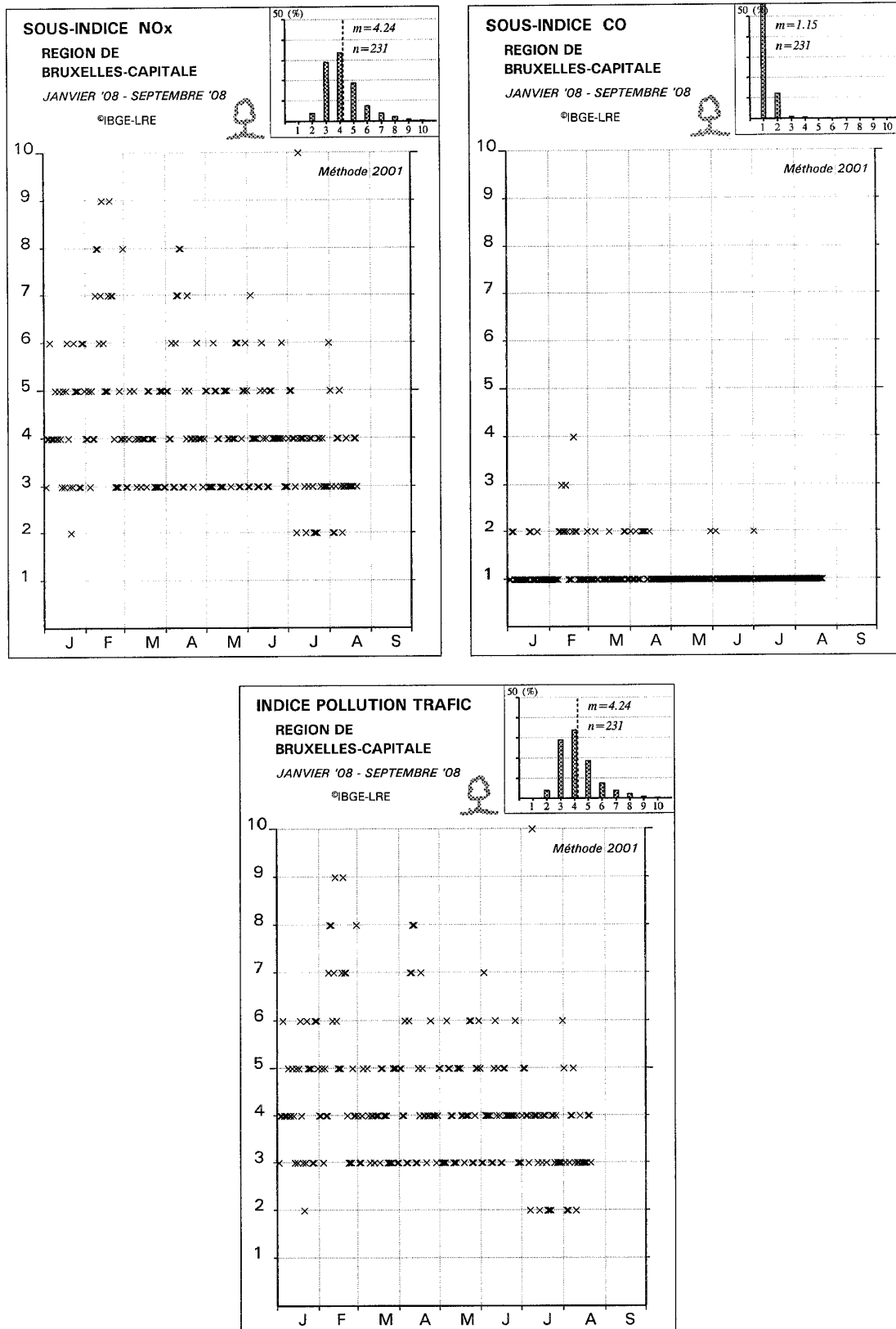
Fig. 61 : Sous-indices pour NO x et CO – Indice trafic (2008)
