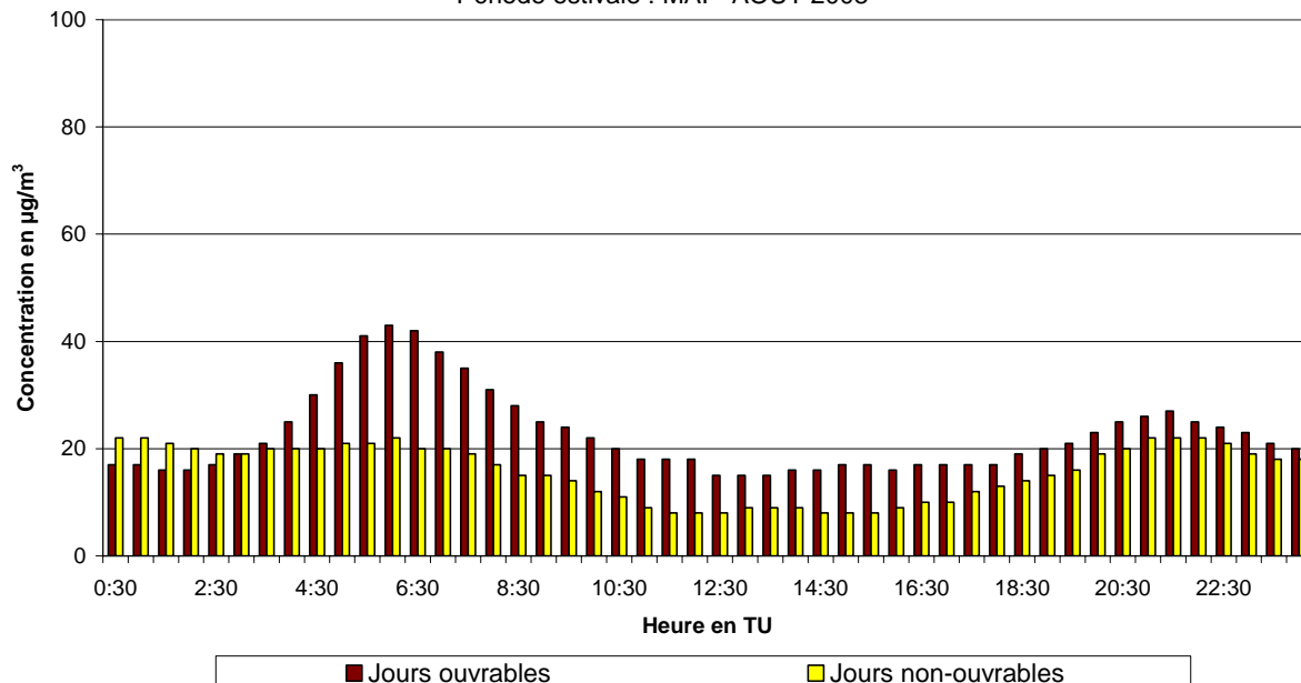
Fig. 47.b : Berchem-Ste-Agathe : Évolution journalière moyenne de la concentration en \text{NO}_2 les jours ouvrables et non-ouvrables pendant le période mai – août 2008
