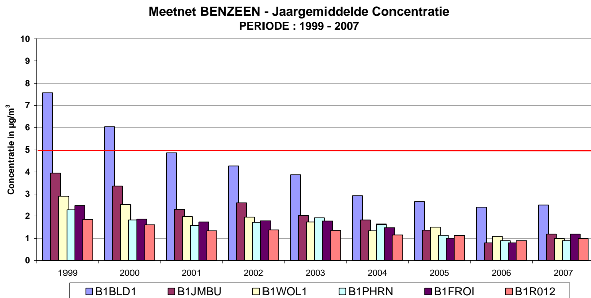
Fig. 30 : Benzeen – Evolutie jaargemiddelde concentratie in een aantal meetpunten van het benzeenmeetnet – Periode : 1999 - 2007
