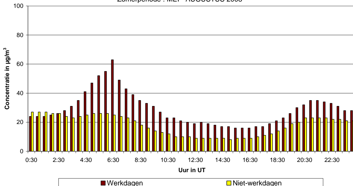
Fig. 53.b : Meudonpark : Gemiddeld dagverloop van de NO 2 -concentratie op werkdagen en niet-werkdagen tijdens de periode mei – augustus 2008
