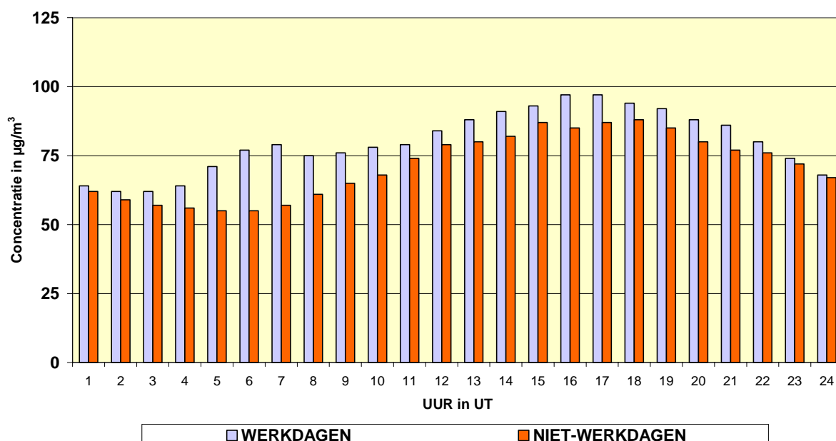
Fig. 70: [O 3 + NO 2 ] – Evolutie Dagverloop voor werkdagen en niet-werkdagen Meetposten te Ukkel en Haren - Periode “mei – augustus 2008”
