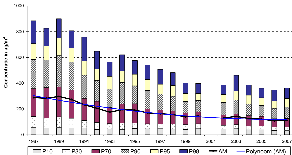
Fig. 73: NO x – Kroonlaan te Elsene ( canyon street ) - Uurgemiddelde concentratie Evolutie over langere termijn - Jaarperiodes 1987 – 2007
