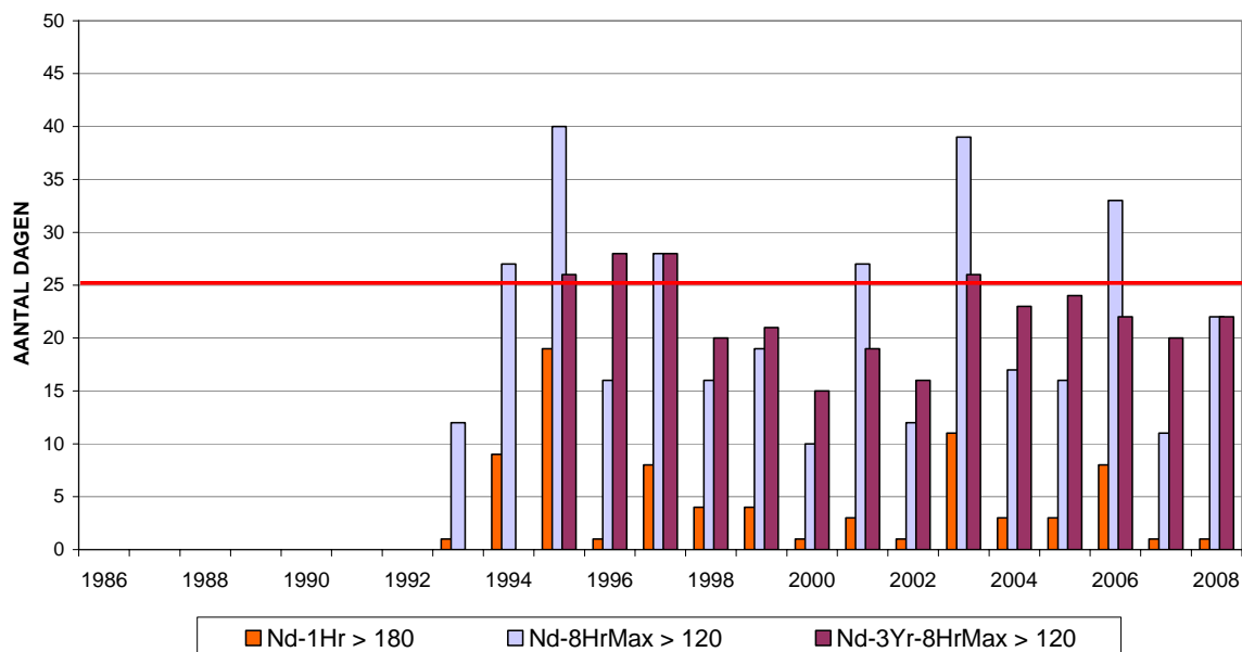
Fig. 20 : Ozon te St.-Ag.-Berchem : aantal dagen met overschrijdingen Jaarperioden: 1 januari – 31 december (1986-2007) Voorlopige resultaten voor het jaar 2008 (1 januari – 30 september)
