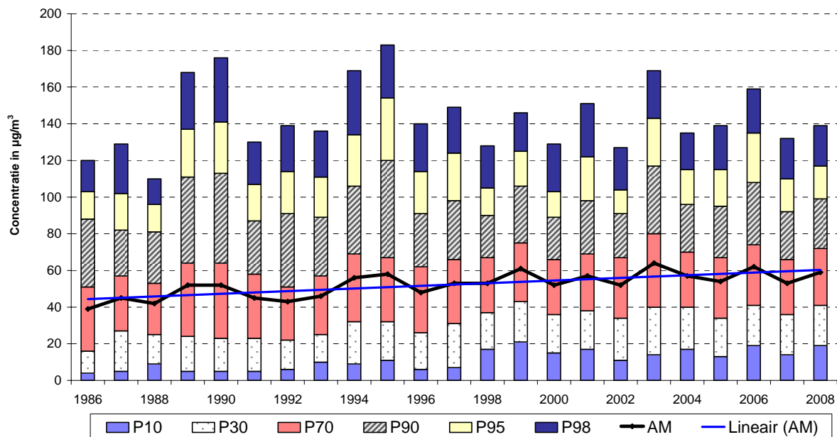
Fig. 33 : Evolutive O 3 -uurwaarden te Ukkel (1986-2008) Zomerperiode "april – september"
