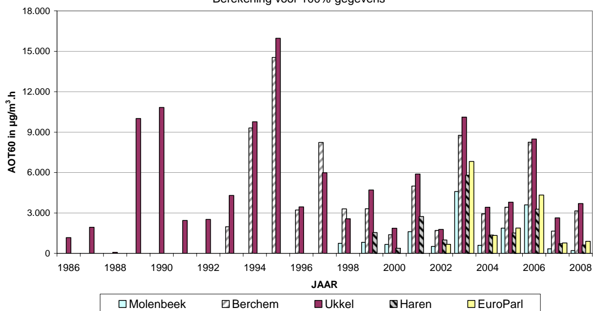
Fig. 24: Evolutie AOT60 in de tijd (1986-2008) Periode: JANUARI – DECEMBER (1986 – 2007) 2008 : Januari - September
