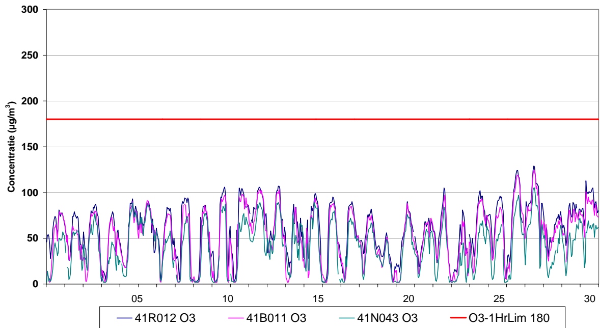
Fig. 2 : Evolutie van de uurwaarden voor ozon – Ukkel, Berchem en Haren – April 2008
