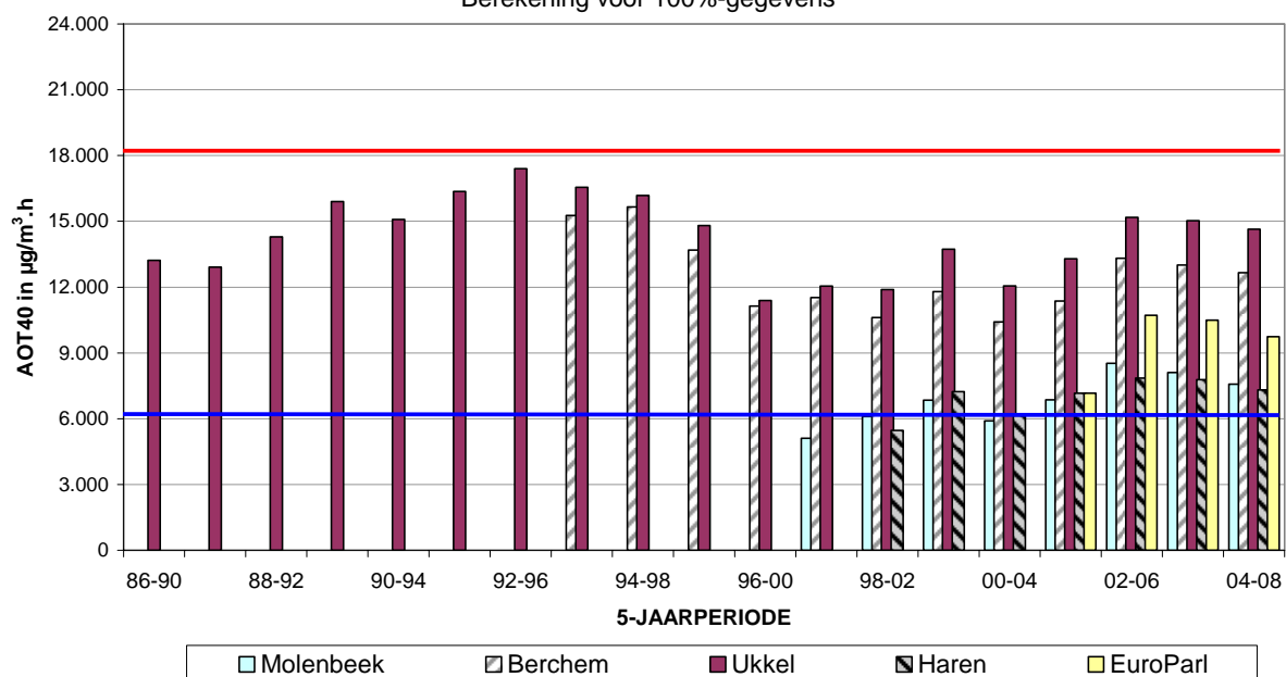
Fig. 15: Evolutie AOT40-MJ in de tijd (1986-2008) AOT40 over de periode Mei – Juli, 8-20 h MET - Midden-Europese tijd Resultaten per jaar en gemiddeld over 5 jaar
