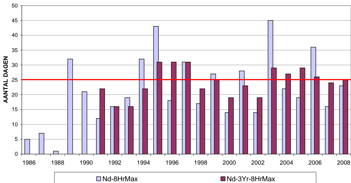
Fig. 14 : Ozon - Evolutie aantal overschrijdingsdagen in het Brussels Hoofdstedelijk Gewest Streefwaarde voor de gezondheid: Maximale 8-uurwaarde > 120 µg/m 3 Periode : Januari – December (1986-2007). [2008]: Januari – September
