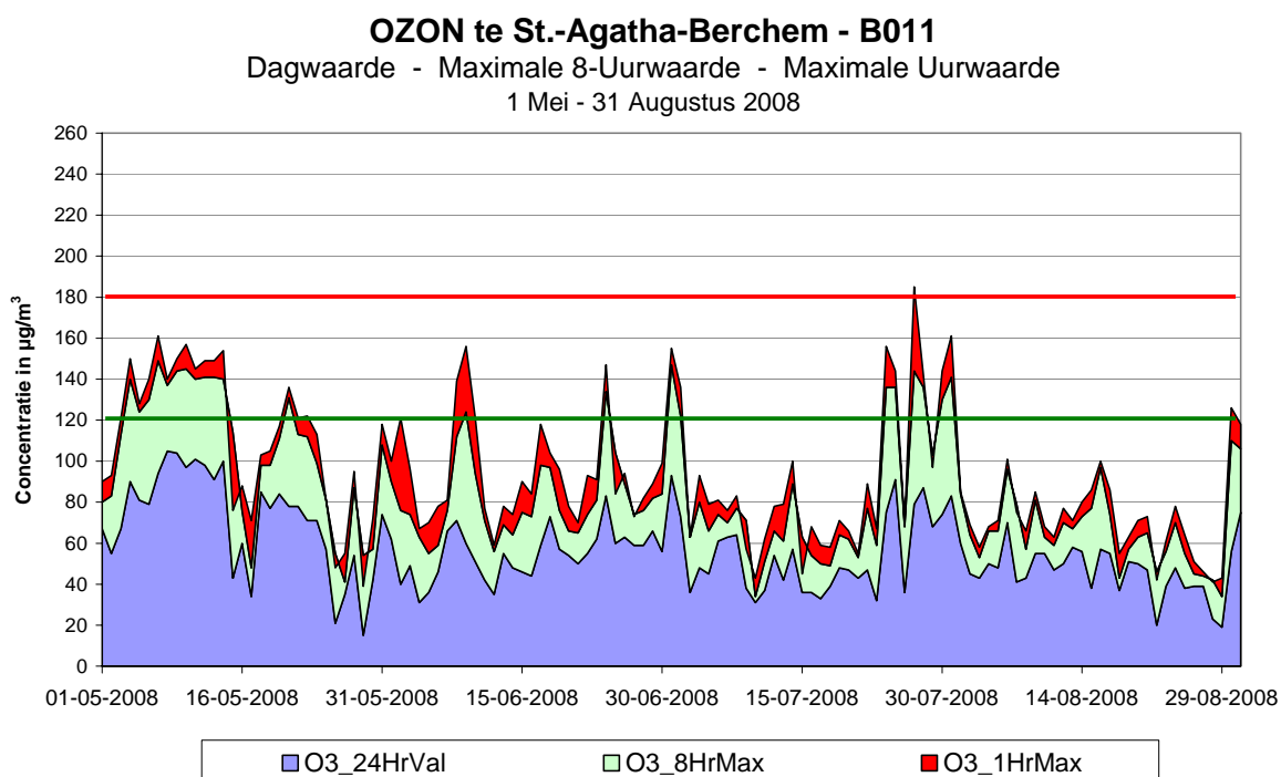
Fig. 22 : Ozon - Evolutie Dagwaarde (24HrVal), maximale 8-uurwaarde (8HrMax) en maximale uurwaarde (1HMax). Periode : mei - augustus 2008 Meetposten te Ukkel en St.-Agatha-Berchem
