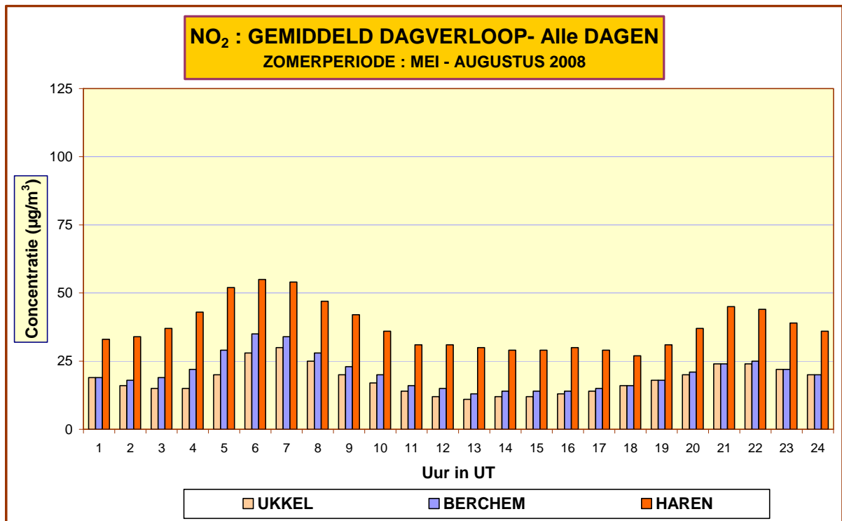
Fig. 67: NO 2 – Evolutie Dagverloop – Vergelijking tussen 3 meetposten Periode “mei –augustus 2008”
