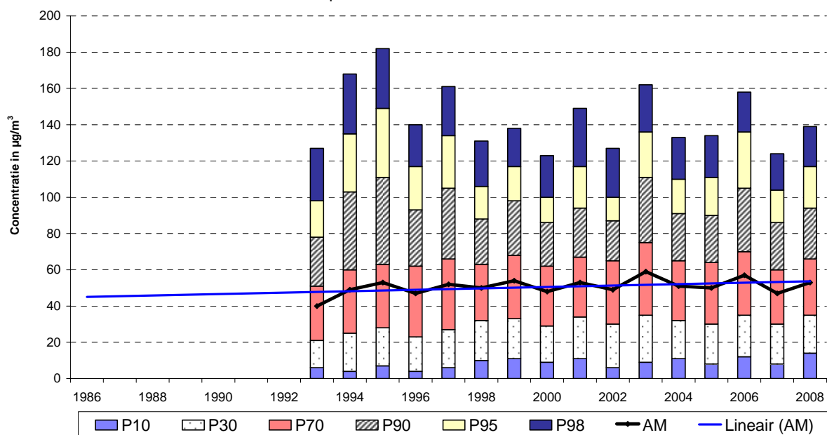
Fig. 72: Ozon te St.-Ag.-Berchem – Uurgemiddelde concentratie – evolutie over langere termijn Zomerperiodes 1993 - 2008
