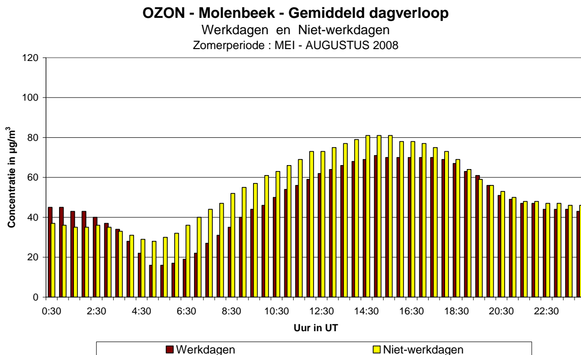
Fig. 48.a : Molenbeek : Gemiddeld dagverloop van de \text{O}_3 -concentratie op werkdagen en niet-werkdagen tijdens de periode mei - augustus 2008
