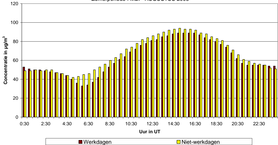
Fig. 46.a : Ukkel : Gemiddeld dagverloop van de O 3 -concentratie op werkdagen en niet-werkdagen tijdens de periode mei - augustus 2008
