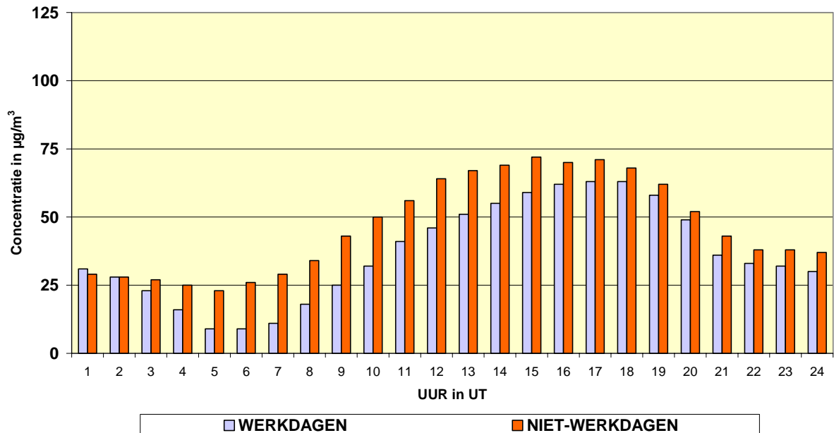
Fig. 69: Ozon – Evolutie Dagverloop voor werkdagen en niet-werkdagen Meetposten te Ukkel en Haren - Periode “mei – augustus 2008”
