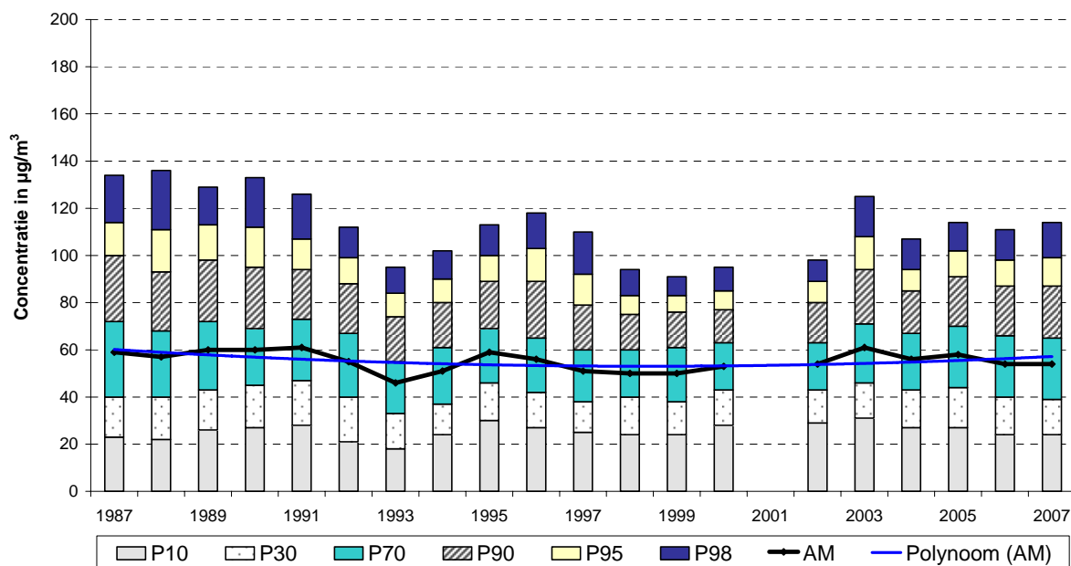
Fig. 74: NO 2 – Kroonlaan te Elsene ( canyon street ) - Uurgemiddelde concentratie Evolutie over langere termijn - Jaarperiodes 1987 – 2007
