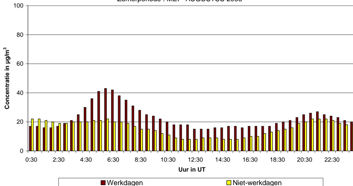
Fig. 47.b : St.-Agatha-Berchem : Gemiddeld dagverloop van de NO 2 -concentratie op werkdagen en niet-werkdagen tijdens de periode mei - augustus 2008
