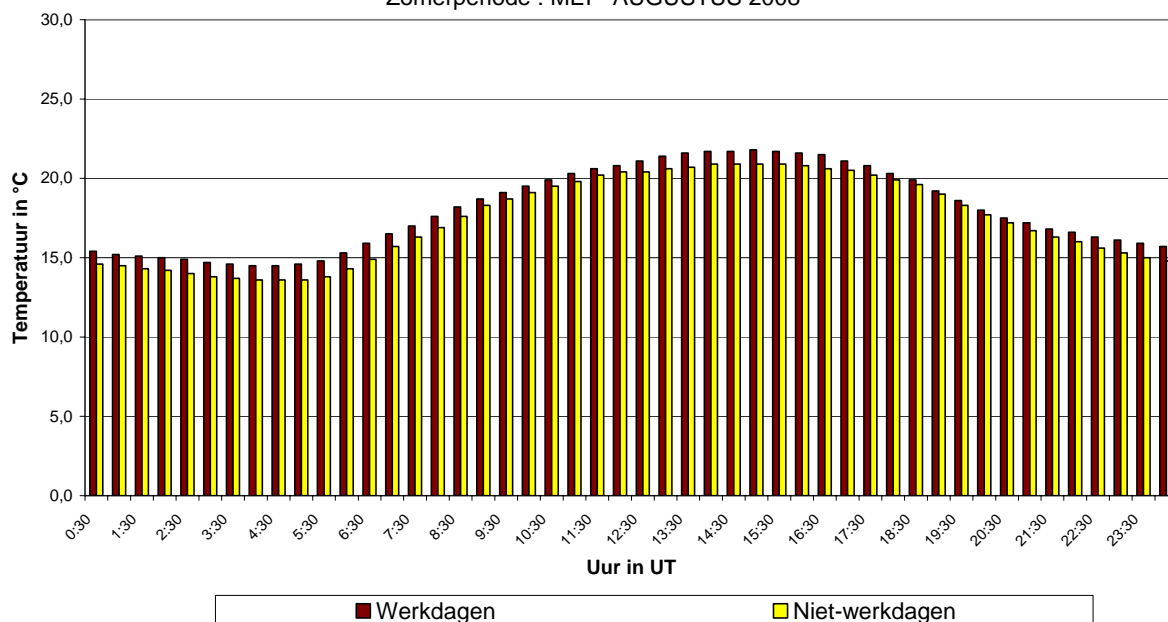
Fig. 55.a : Ukkel : Gemiddeld dagverloop van de temperatuur op werkdagen en niet-werkdagen tijdens de periode mei – augustus 2008
