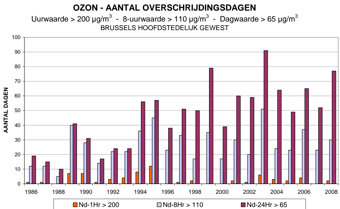
Fig. 25 : Ozon : aantal dagen met overschrijdingen (richtlijn 92/72/EG) Periode : januari - december (1986 t/m 2007) 2008 : Januari - September
