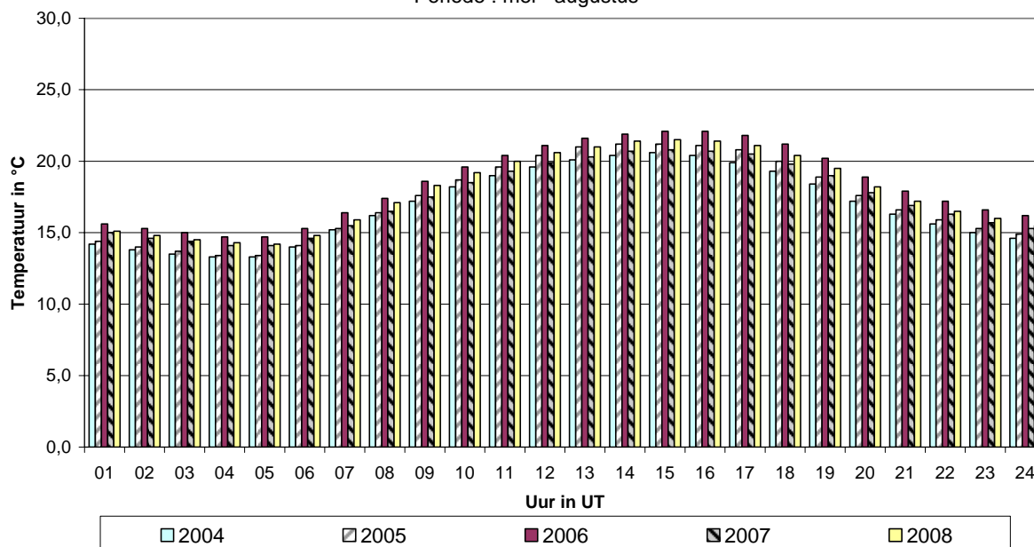
Fig. 37 : Gemiddeld dagverloop temperatuur te Ukkel (M003) Zomerperiodes mei-augustus 2004, 2005, 2006, 2007 en 2008
