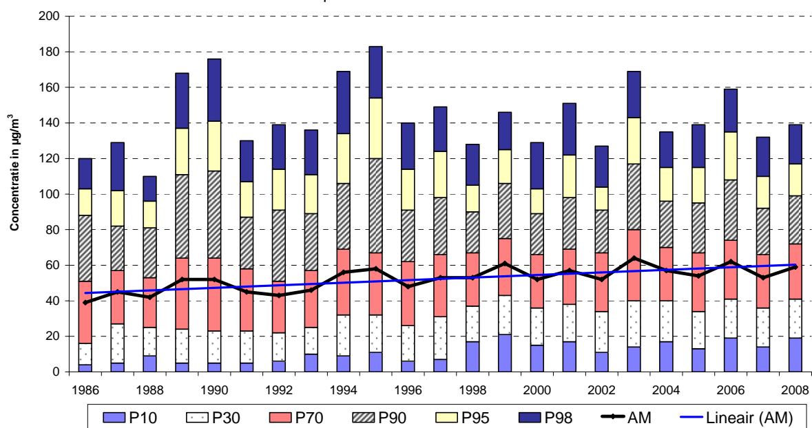
Fig. 71: Ozon te Ukkel – Uurgemiddelde concentratie – evolutie over langere termijn Zomerperiodes 1986 - 2008
