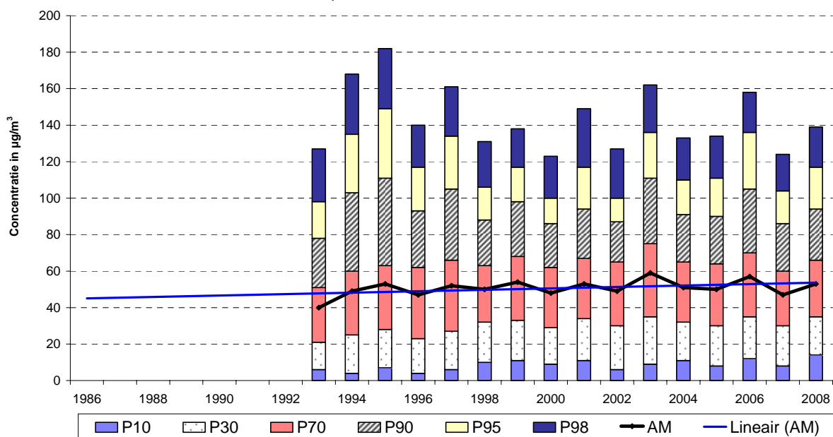
Fig. 34 : Evolutive O 3 -uurwaarden te St.-Ag.-Berchem (1993-2008) Zomerperiode "april – september"
