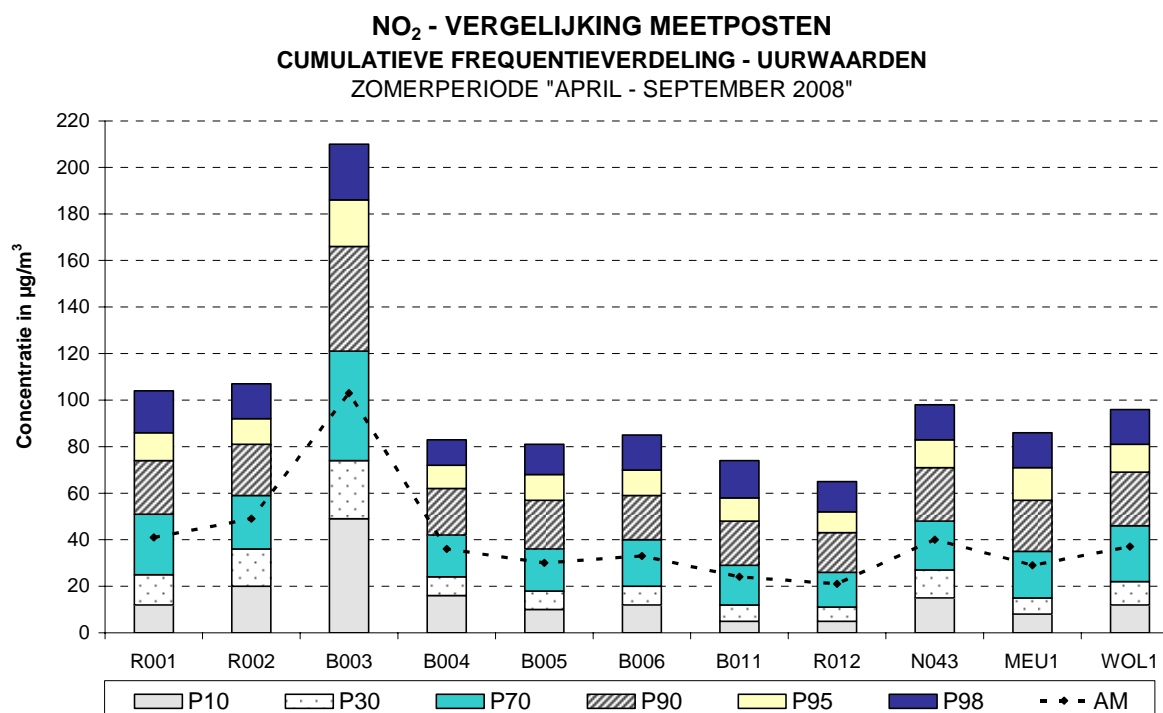
Fig. 39 : NO 2 - Cumulatieve frequentieverdeling uurwaarden: april - september 2008
