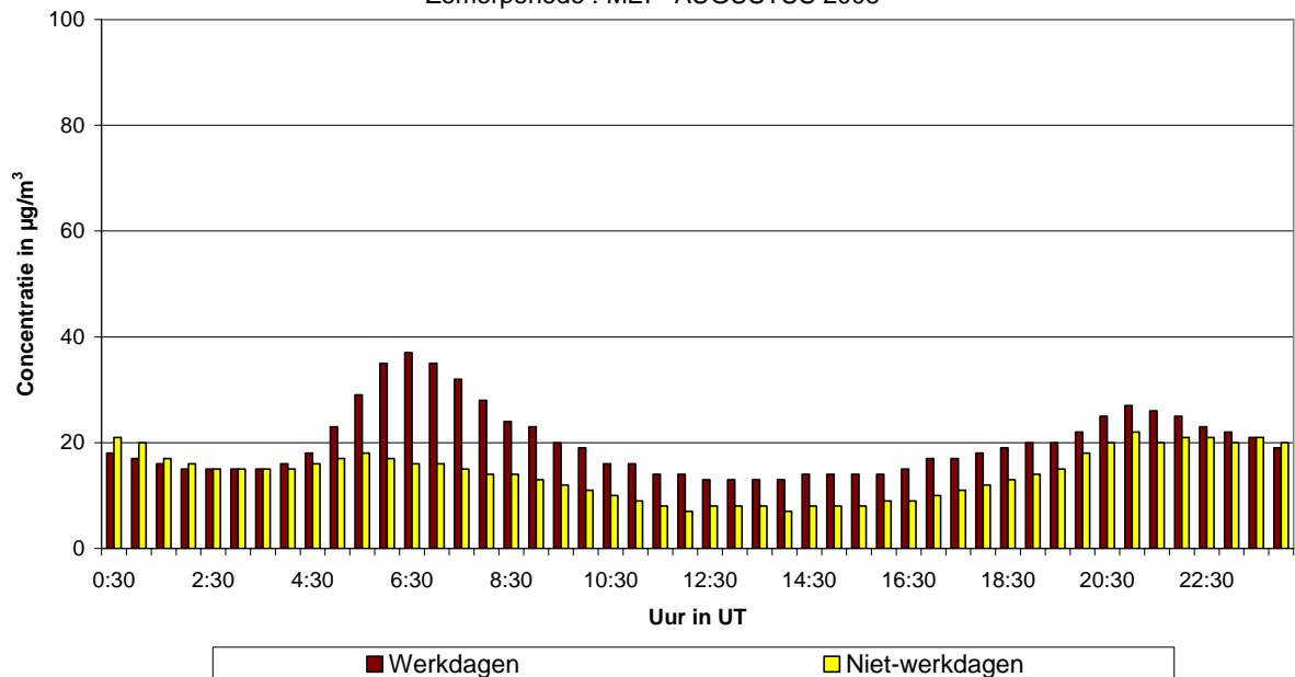
Fig. 46.b : Ukkel : Gemiddeld dagverloop van de NO 2 -concentratie op werkdagen en niet-werkdagen tijdens de periode mei - augustus 2008
