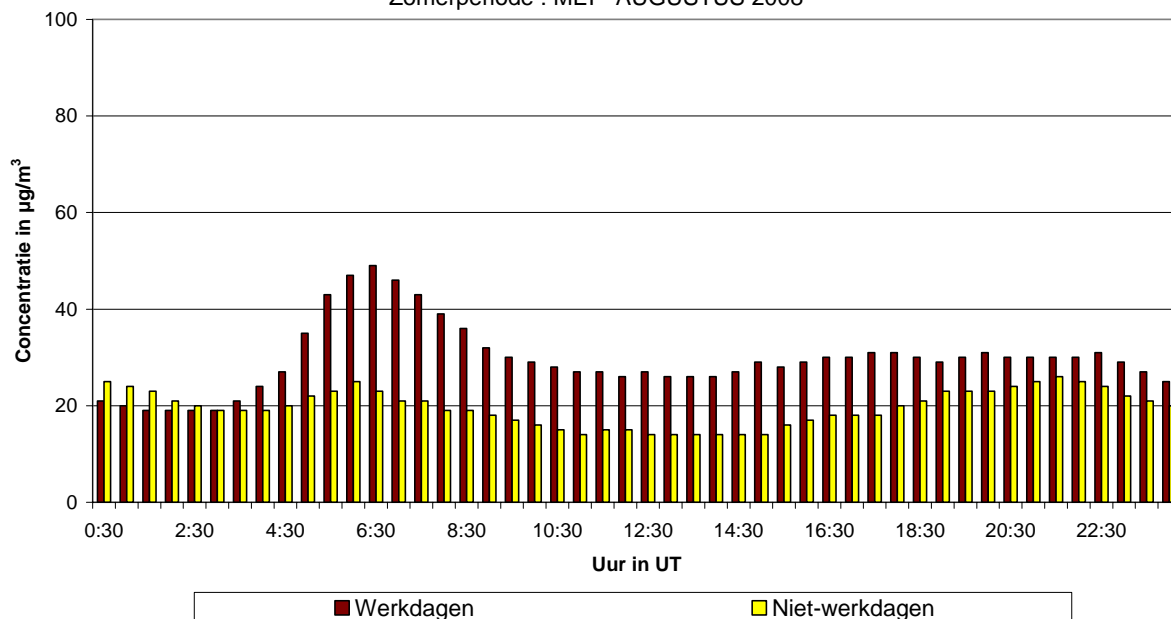
Fig. 53.a : Eastman-Belliard : Gemiddeld dagverloop van de NO 2 -concentratie op werkdagen en niet-werkdagen tijdens de periode mei - augustus 2008
