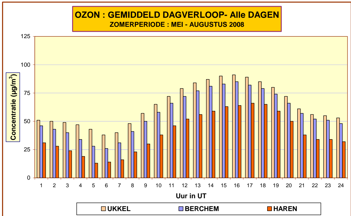
Fig. 66: Ozon – Evolutie Dagverloop – Vergelijking tussen 3 meetposten Periode “mei –augustus 2008”
