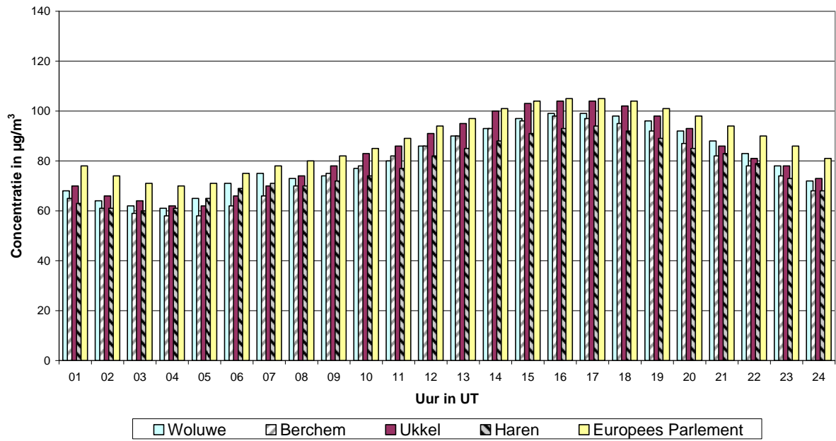
Fig. 10 : Gemiddeld dagverloop voor de som van de gasvormige oxidantia [O 3 + NO 2 ], uitgedrukt als equivalent massaconcentratie ozon, tijdens de periode mei – augustus 2008
