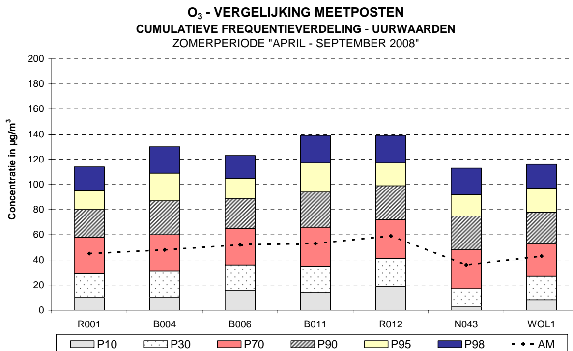
Fig. 32 : Ozon - Cumulatieve frequentieverdeling uurwaarden : april - september 2008
