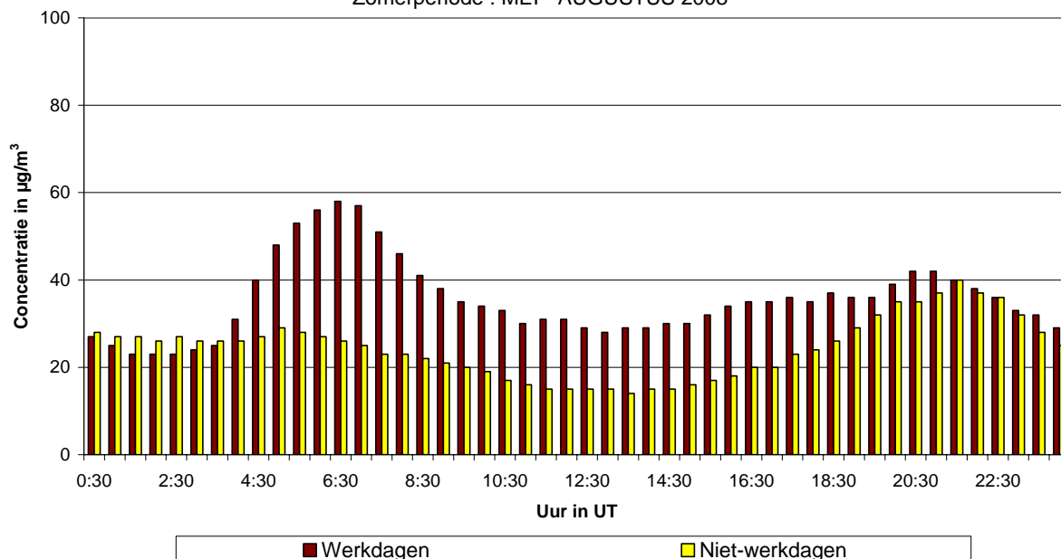
Fig. 50.b : St.-Lambr.-Woluwe : Gemiddeld dagverloop van de NO 2 -concentratie op werkdagen en niet-werkdagen tijdens de periode mei - augustus 2008
