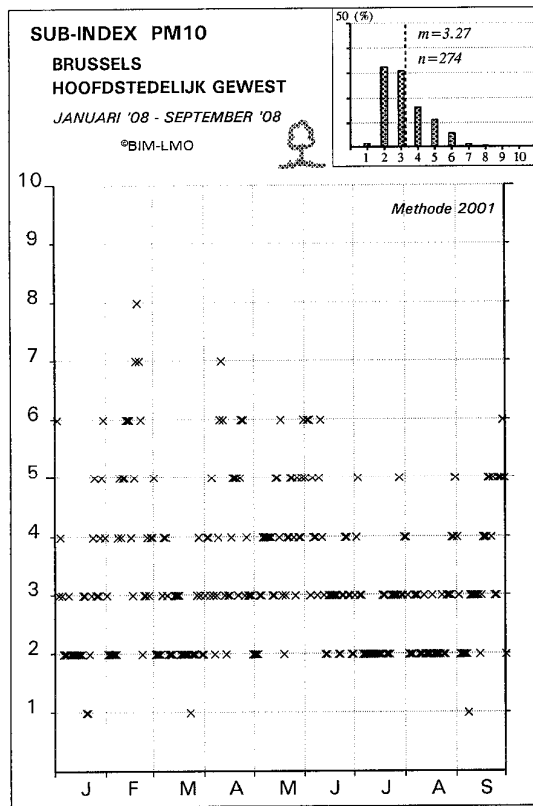
Fig. 60 : Subindexen voor NO 2 , O 3 en PM10 – Index Algemene Luchtkwaliteit (2008)
