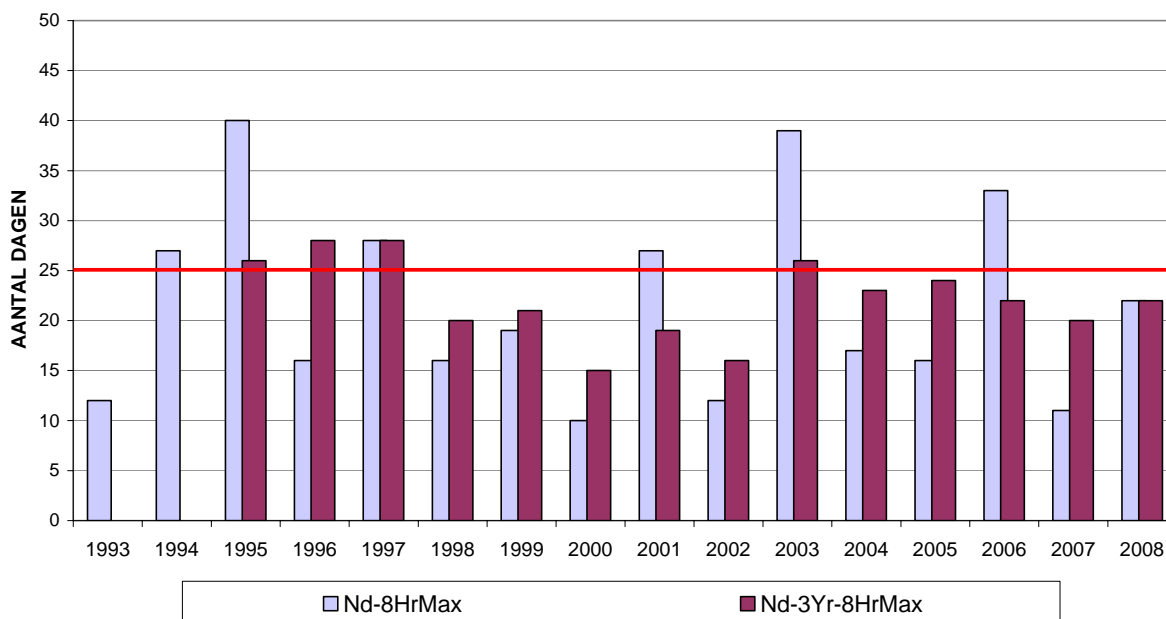
Fig. 13 : Ozon - Evolutie aantal overschrijdingsdagen in de meetpost te Berchem Streefwaarde voor de gezondheid: Maximale 8-uurwaarde > 120 µg/m 3 Periode : Januari – December (1986-2007). [2008]: Januari – September
