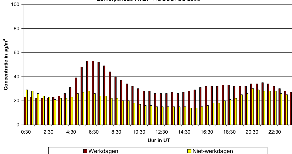
Fig. 51.b : Europees Parlement : Gemiddeld dagverloop van de NO 2 -concentratie op werkdagen en niet-werkdagen tijdens de periode mei – augustus 2008
