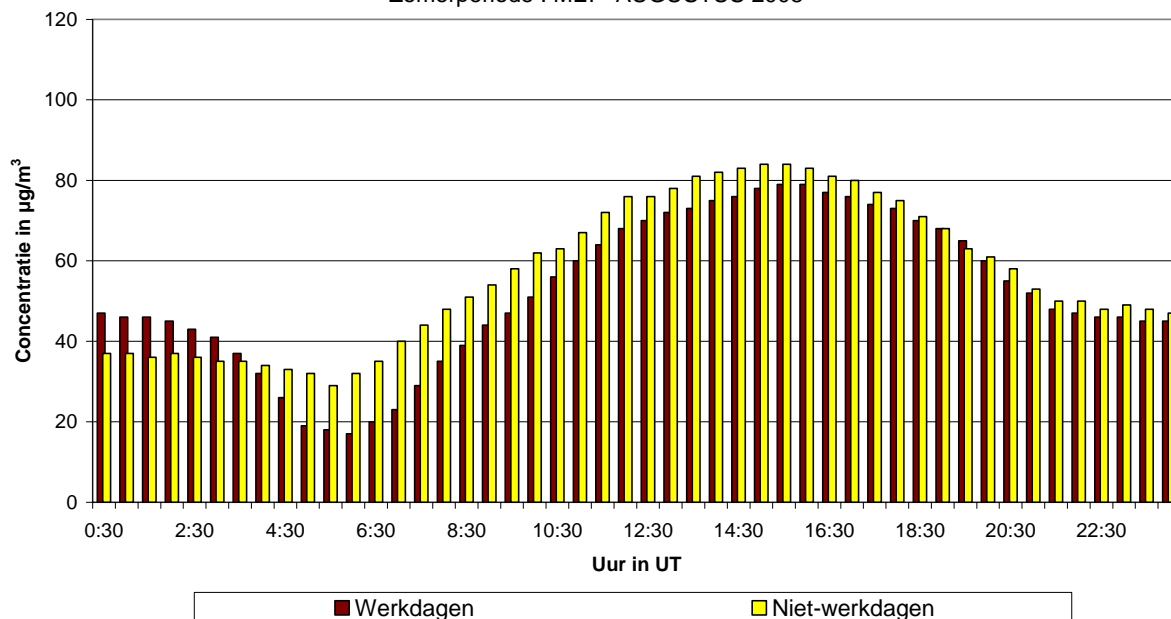
Fig. 52.a : St.-Katelijne : Gemiddeld dagverloop van de O 3 -concentratie op werkdagen en niet-werkdagen tijdens de periode mei - augustus 2008
