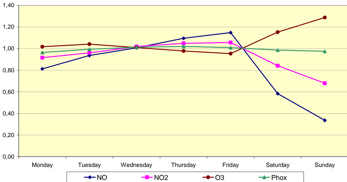
Fig. 59.b : Meetpost te Molenbeek – Gemiddeld weekpatroon voor NO, NO 2 , O 3 en [NO 2 +O 3 ] over drie opeenvolgende zomerperiodes 'april – september' 2006, 2007 en 2008
