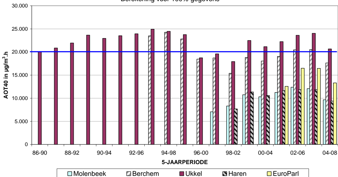
Fig. 16: Evolutie AOT40-AS in de tijd (1986-2008) AOT over de periode April – September, 8-20 h MET - Midden-Europese tijd Resultaten per jaar en gemiddeld over 5 jaar
