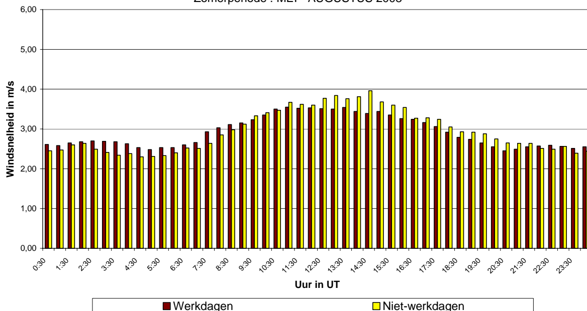
Fig. 55.b : Ukkel : Gemiddeld dagverloop van de windsnelheid op werkdagen en niet-werkdagen tijdens de periode mei – augustus 2008
