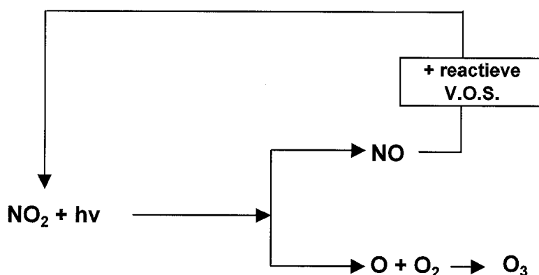
Fig. 64: vereenvoudigd reactieschema voor excessieve ozonvorming
