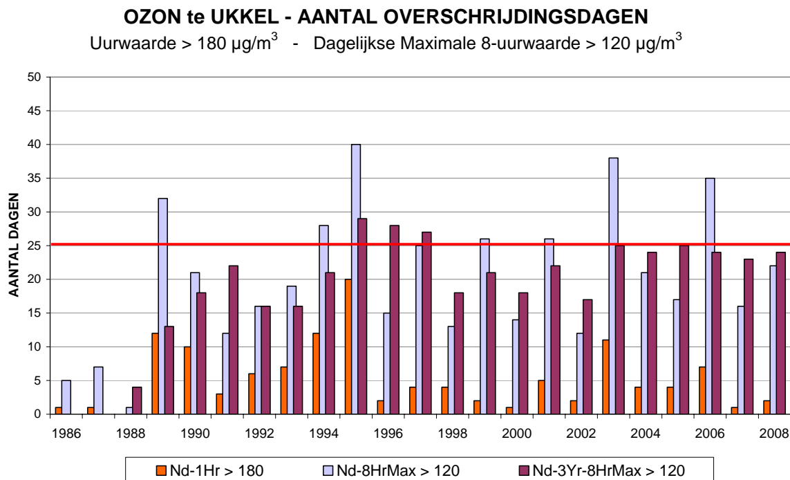
Fig. 19 : Ozon te Ukkel : aantal dagen met overschrijdingen Jaarperiodes: 1 januari – 31 december (1986-2007) Voorlopige resultaten voor het jaar 2008 (1 januari – 30 september)
