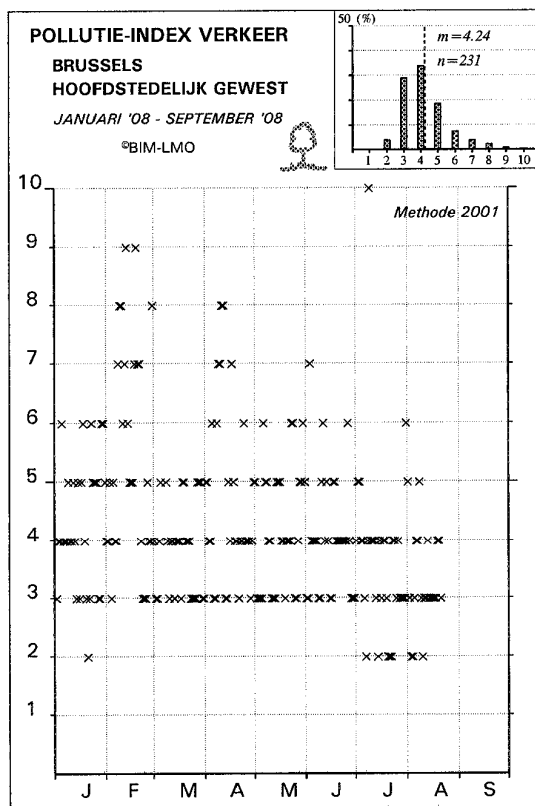
Fig. 61 : Subindexen NO x en CO – Verkeersindex (2008)
