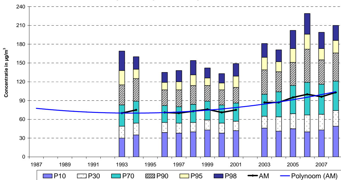
Fig. 41 : Kunst-Wet – Evolutie NO 2 -uurwaarden (1991-2008) Zomerperiode "april – september"
