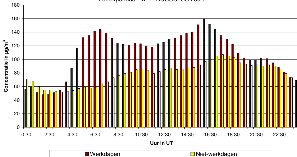
Fig. 54.b : Kunst-Wet : Gemiddeld dagverloop van de NO 2 -concentratie op werkdagen en niet-werkdagen tijdens de periode mei - augustus 2008
