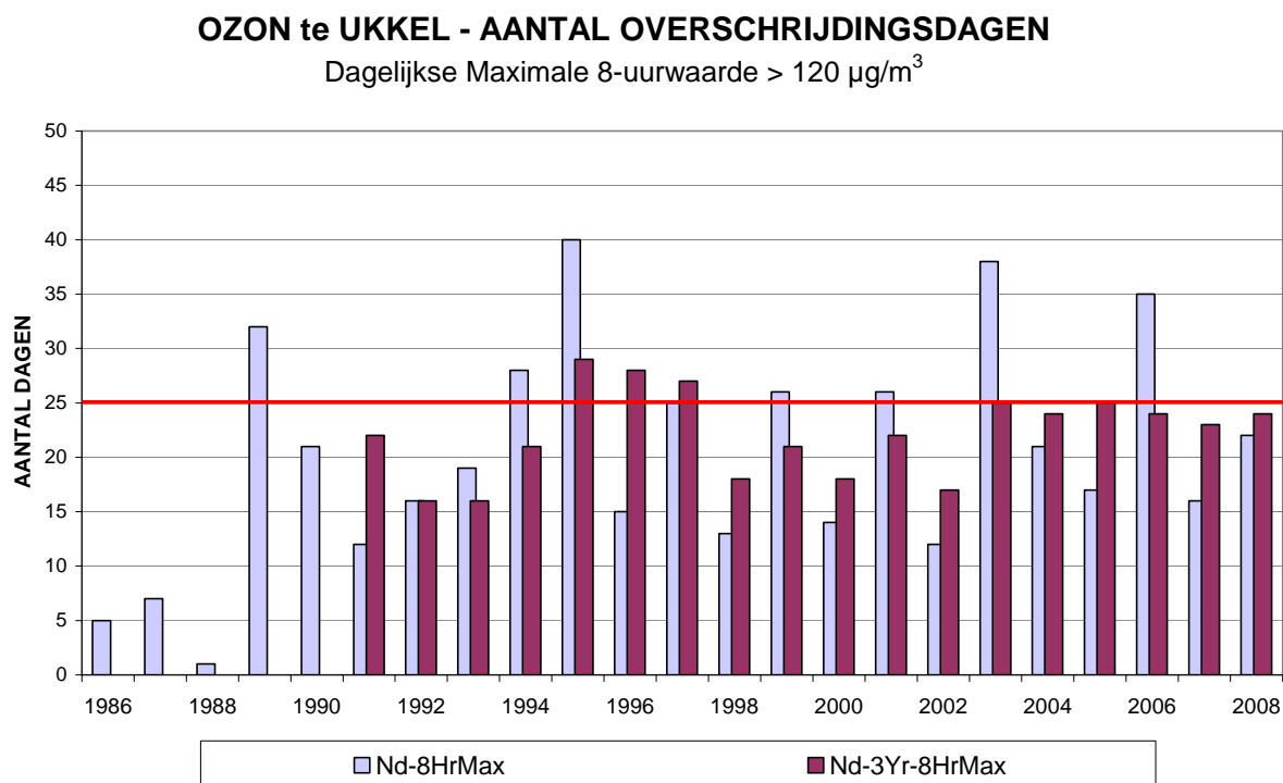
Fig. 12 : Ozon - Evolutie aantal overschrijdingsdagen in de meetpost te Ukkel Streefwaarde voor de gezondheid: Maximale 8-uurwaarde > 120 \mu\text{g}/\text{m}^3 Periode : Januari – December (1986-2007). [2008]: Januari – September
