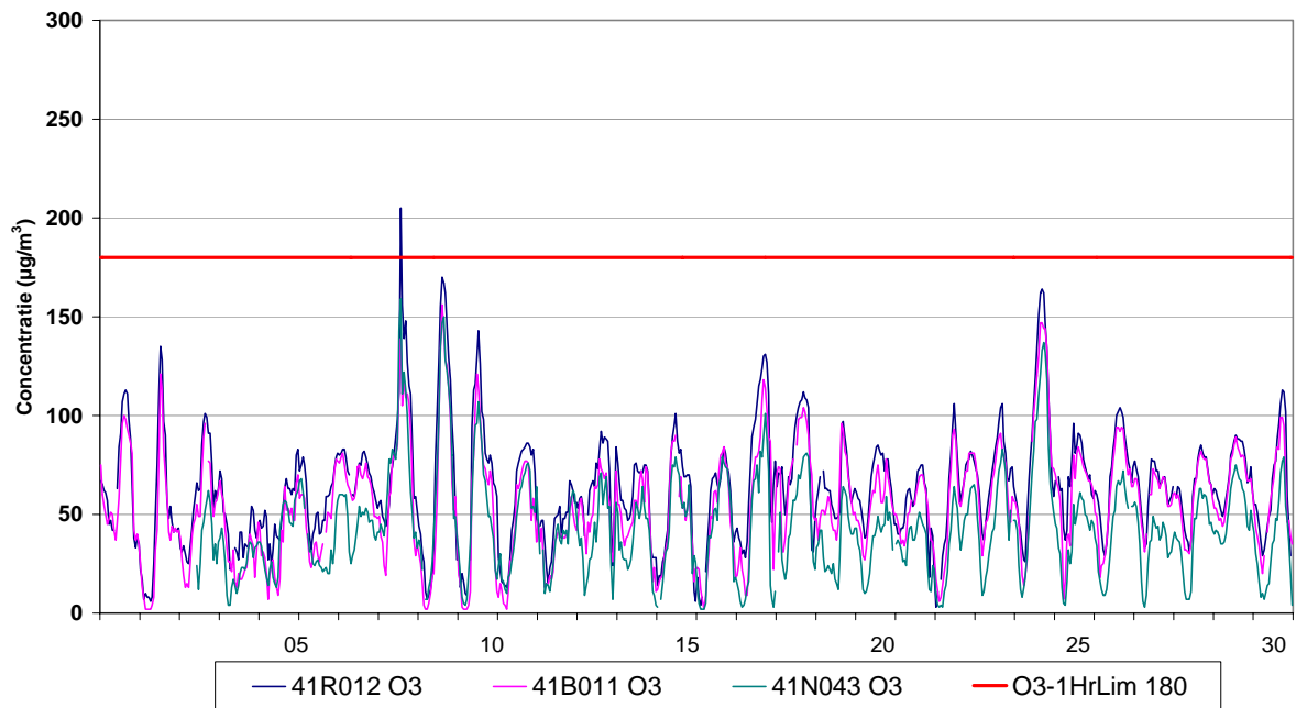
Fig. 4 : Evolutie van de uurwaarden voor ozon – Ukkel, Berchem en Haren – Juni 2008
