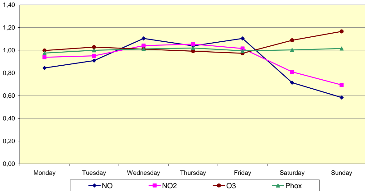
Fig. 59.a : Meetpost te Ukkel – Gemiddeld weekpatroon voor NO, NO 2 , O 3 en [NO 2 +O 3 ] over drie opeenvolgende zomerperiodes 'april – september' 2006, 2007 en 2008
