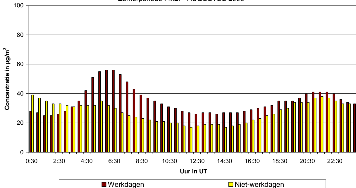
Fig. 52.b : St.-Katelijne : Gemiddeld dagverloop van de NO 2 -concentratie op werkdagen en niet-werkdagen tijdens de periode mei – augustus 2008
