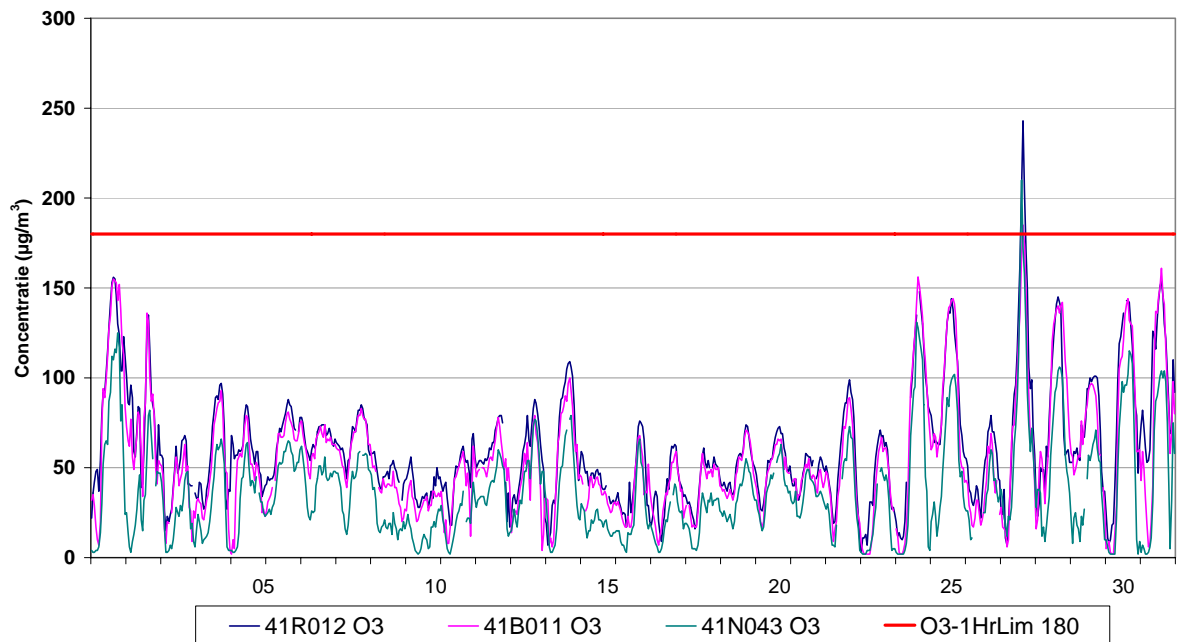
Fig. 5 : Evolutie van de uurwaarden voor ozon – Ukkel, Berchem en Haren – Juli 2008
