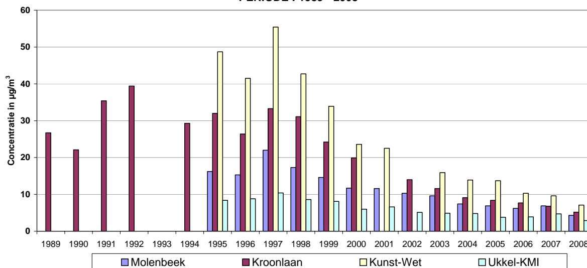
Fig. 29 : Toluene - Evolutive jaargemiddelde concentratie Periode : januari – december (1989-2007) 2008 : Januari - September
