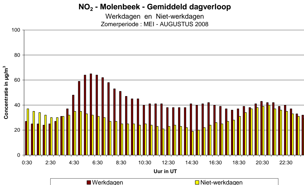
Fig. 48.b : Molenbeek : Gemiddeld dagverloop van de \text{NO}_2 -concentratie op werkdagen en niet-werkdagen tijdens de periode mei – augustus 2008
