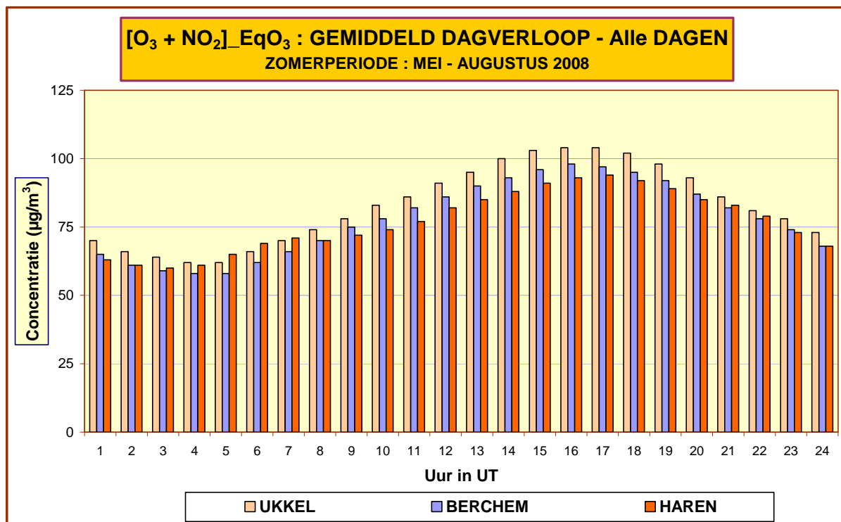
Fig. 68: [O 3 + NO 2 ] – Evolutie Dagverloop – Vergelijking tussen 3 meetposten Periode “mei – augustus 2008”
