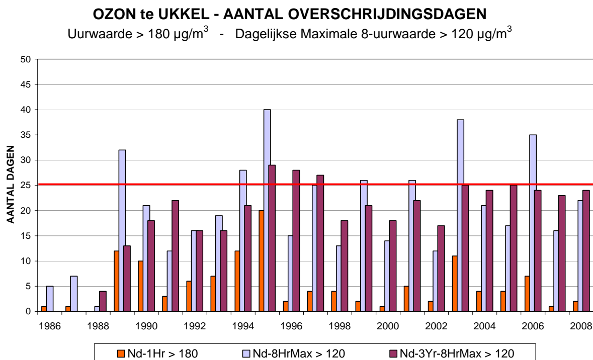
Fig. 63: Ozon: aantal dagen met overschrijdingen te Ukkel Aantal dagen met een uurwaarde hoger dan 180 \mu\text{g}/\text{m}^3 en met een maximale 8-uurwaarde hoger dan 120 \mu\text{g}/\text{m}^3 (per jaar en gemiddeld over 3 jaar)
