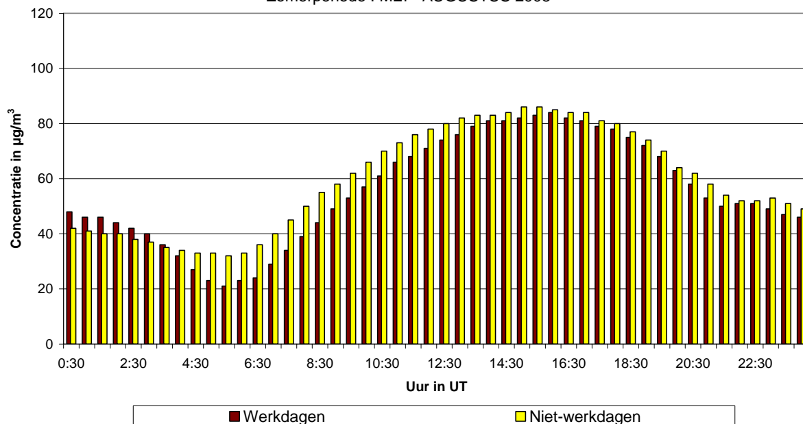
Fig. 47.a : St.-Agatha-Berchem : Gemiddeld dagverloop van de O 3 -concentratie op werkdagen en niet-werkdagen tijdens de periode mei - augustus 2008
