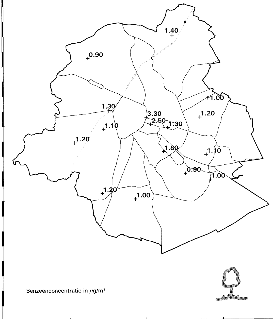
Fig. 31 : Benzeen – Ruimtelijke spreiding jaargemiddelde concentratie in 2007
