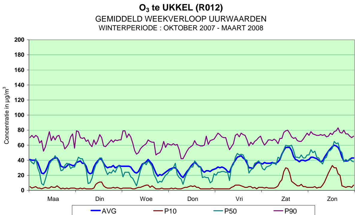
Fig. 56 : Ozon te Ukkel - Gemiddeld weekverloop tijdens zomer en winter
