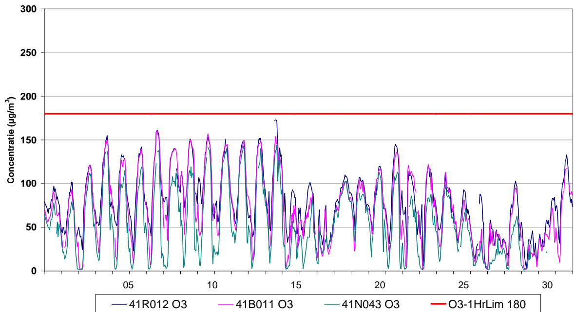
Fig. 3 : Evolutie van de uurwaarden voor ozon – Ukkel, Berchem en Haren – Mei 2008
