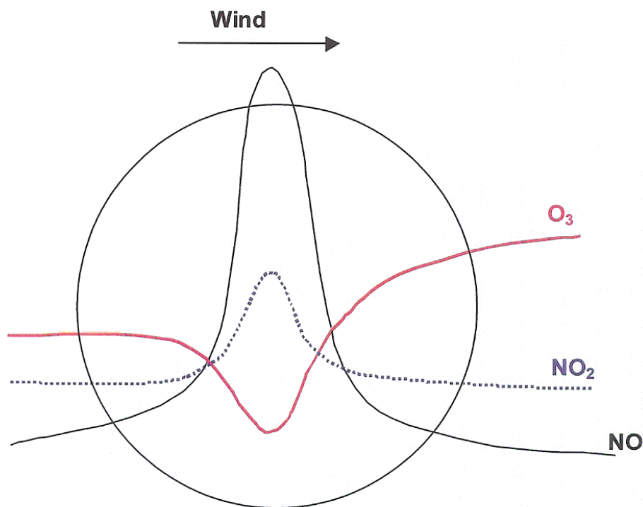
Fig. 65 : Overmaat NO in het centrum zorgt voor een belangrijke ozonafbraak. In de rand en windafwaarts van het brongebied haalt de ozonvorming de bovenhand op de ozonafbraak
