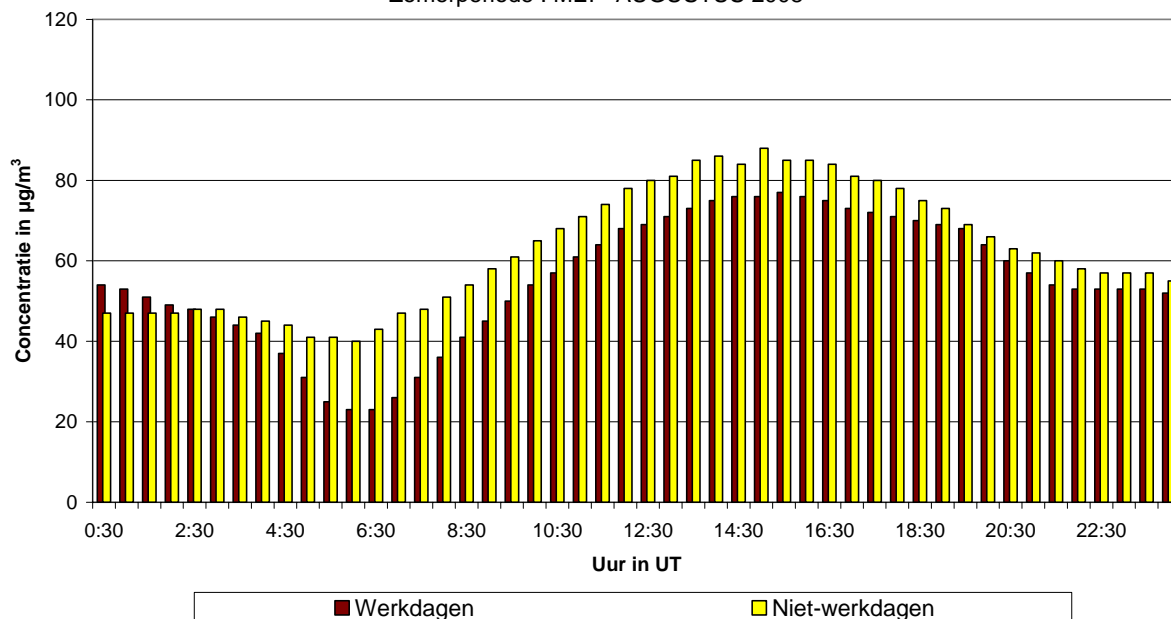
Fig. 51.a : Europees Parlement : Gemiddeld dagverloop van de O 3 -concentratie op werkdagen en niet-werkdagen tijdens de periode mei - augustus 2008
