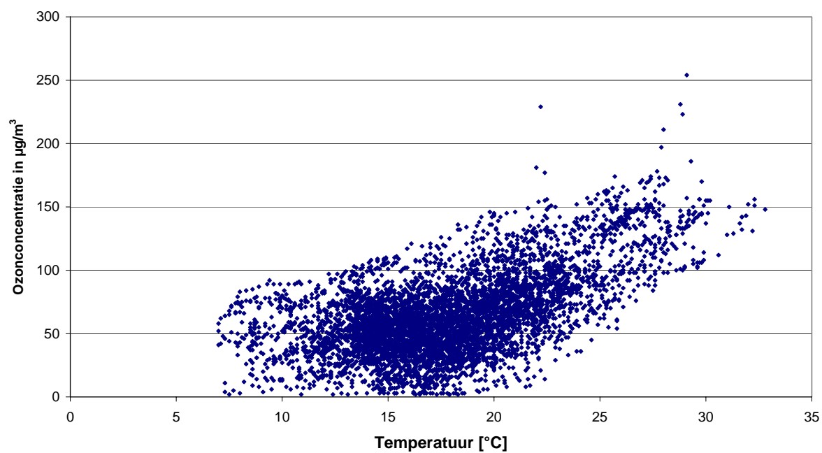
Fig. 42 : Ukkel : Ozonconcentraties versus temperatuur (mei - augustus 2008)
