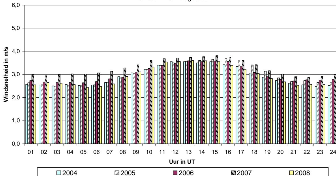
Fig. 38 : Gemiddeld dagverloop windsnelheid te Ukkel (M003) Zomerperiodes mei-augustus 2004, 2005, 2006, 2007 en 2008
