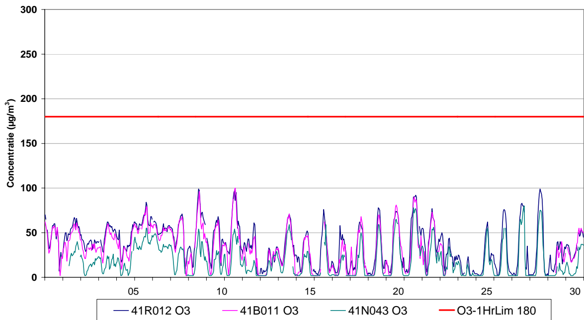
Fig. 7 : Evolutie van de uurwaarden voor ozon – Ukkel, Berchem en Haren – September 2008
