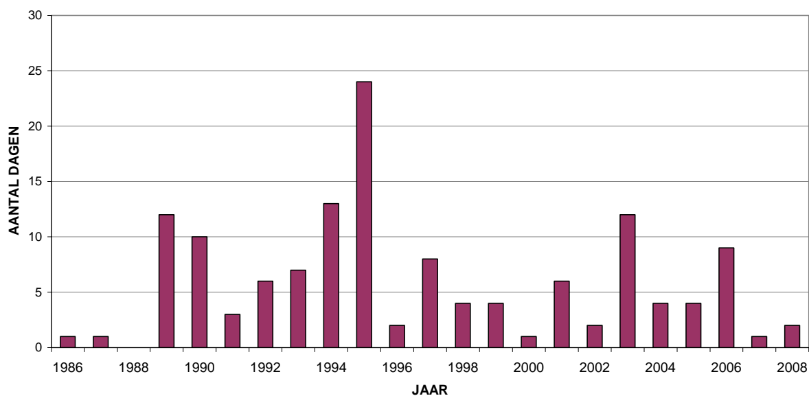
Fig. 17 : Ozon - Evolutie aantal overschrijdingsdagen in het Brussels Hoofdstedelijk Gewest Informatiedrempel: Uurwaarde > 180 \mu\text{g}/\text{m}^3
