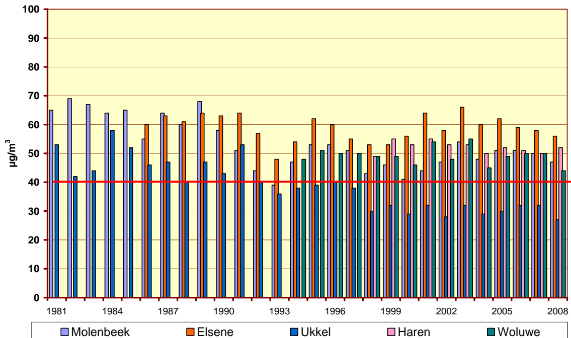
Fig. 26 : NO 2 - Evolutie jaargemiddelde concentratie ( alle dagen ) en gemiddelde concentratie op ' werkdagen ' – Periode 1981-2008
