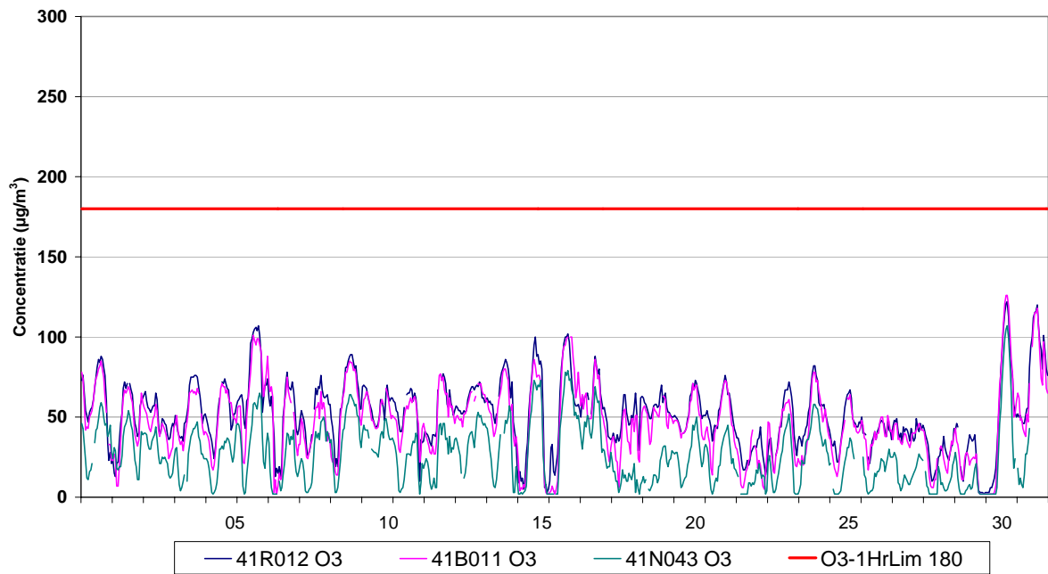
Fig. 6 : Evolutie van de uurwaarden voor ozon – Ukkel, Berchem en Haren – Augustus 2008
