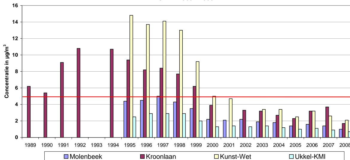
Fig. 28 : Benzeen - Evolutie jaargemiddelde concentratie Periode : januari – december (1989-2007) 2008 : Januari - September
