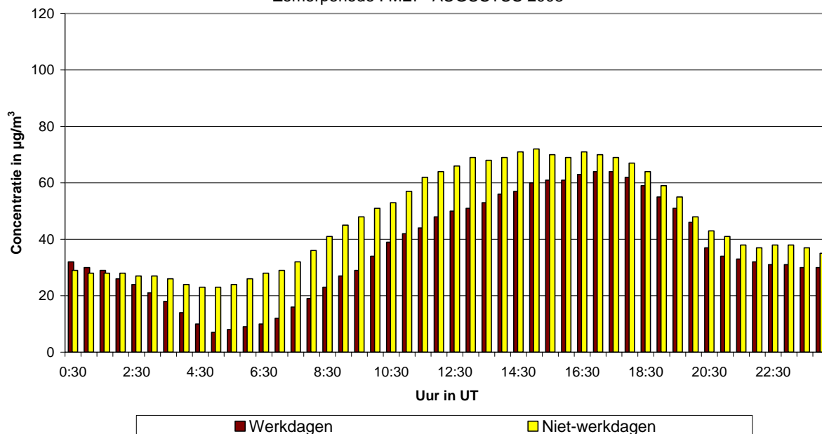
Fig. 49.a : Haren : Gemiddeld dagverloop van de O 3 -concentratie op werkdagen en niet-werkdagen tijdens de periode mei - augustus 2008
