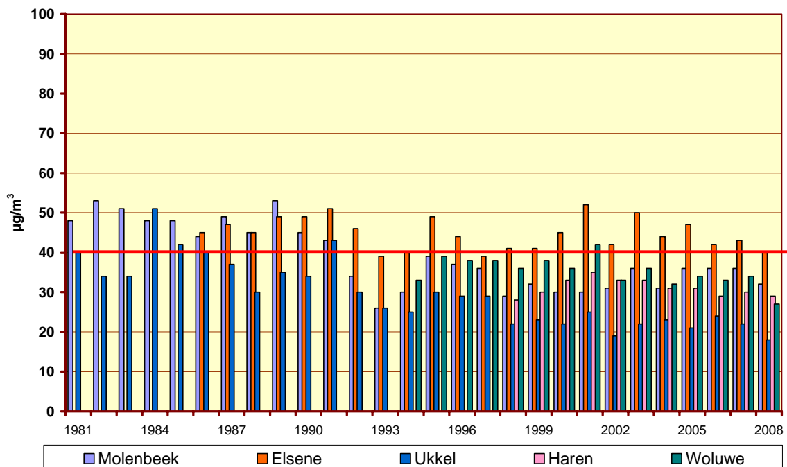
Fig. 27 : NO 2 - Evolutive gemiddelde concentratie op 'Zaterdag' en 'Zondag' Periode 1981-2008
