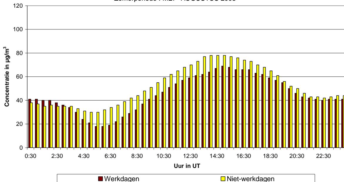
Fig. 50.a : St.-Lambr.-Woluwe : Gemiddeld dagverloop van de O 3 -concentratie op werkdagen en niet-werkdagen tijdens de periode mei - augustus 2008
