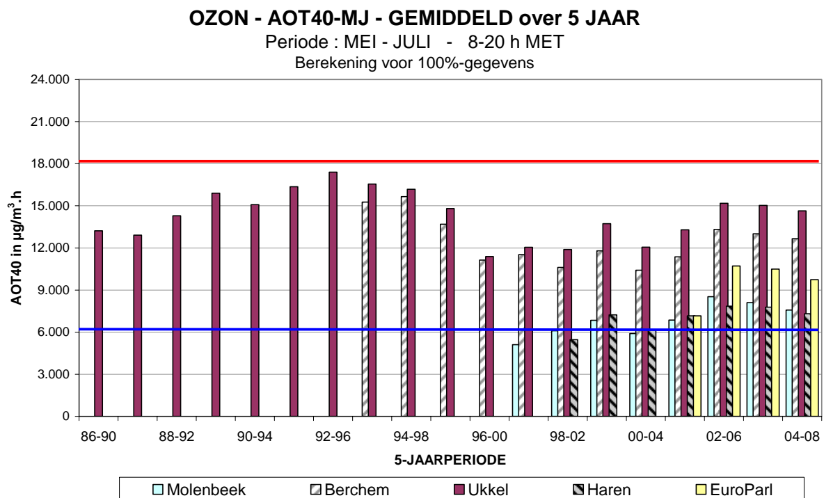
Fig. 62: Evolutie van de AOT40-MJ, gemiddeld over 5 jaar
