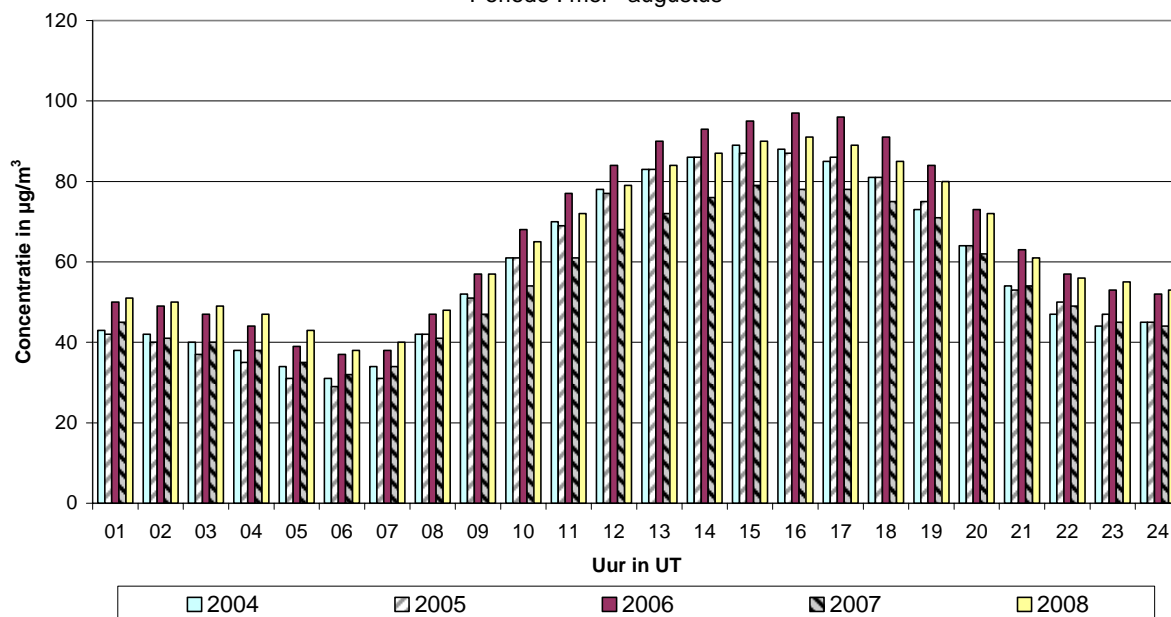
Fig. 35 : Gemiddeld dagverloop O 3 -concentratie te Ukkel (R012) Evolutie tijdens recente zomerperiodes (2004-2008)
