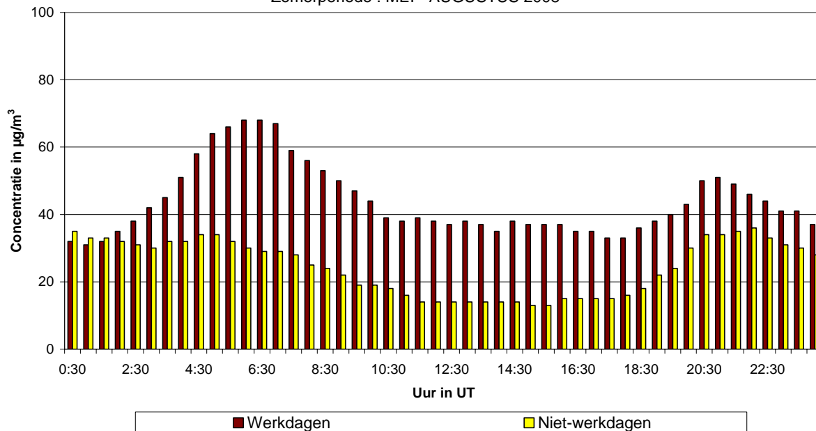
Fig. 49.b : Haren : Gemiddeld dagverloop van de NO 2 -concentratie op werkdagen en niet-werkdagen tijdens de periode mei - augustus 2008
