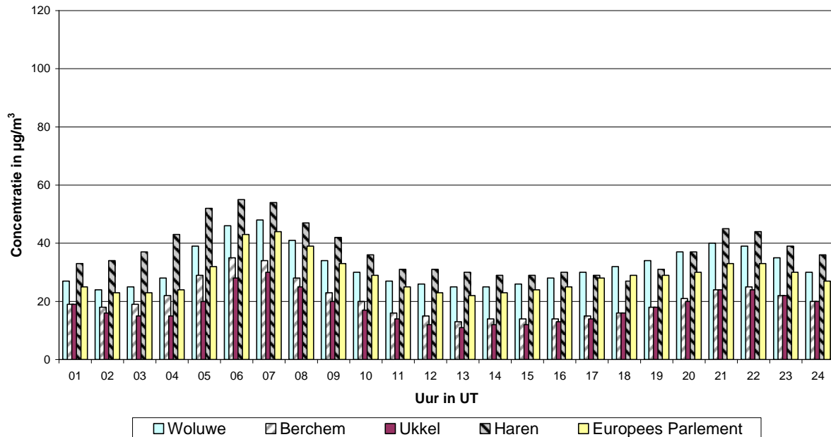
Fig. 9 : Gemiddeld dagverloop van de NO 2 -concentratie in de periode mei – augustus 2008
