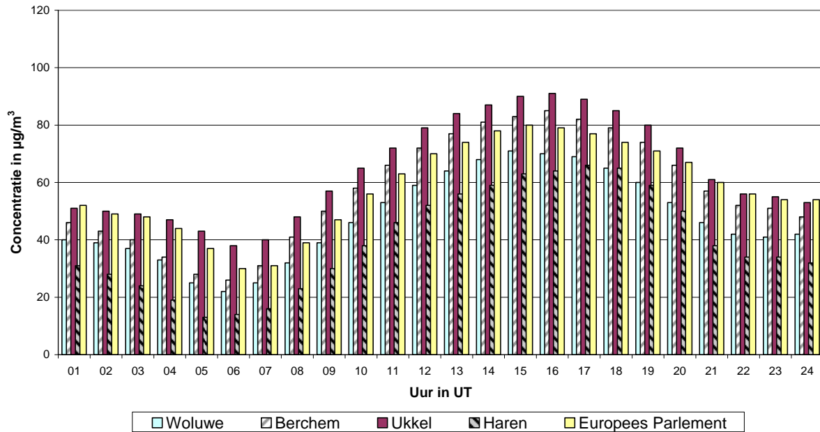
Fig. 8 : Gemiddeld dagverloop van de O 3 -concentratie in de periode mei – augustus 2008
