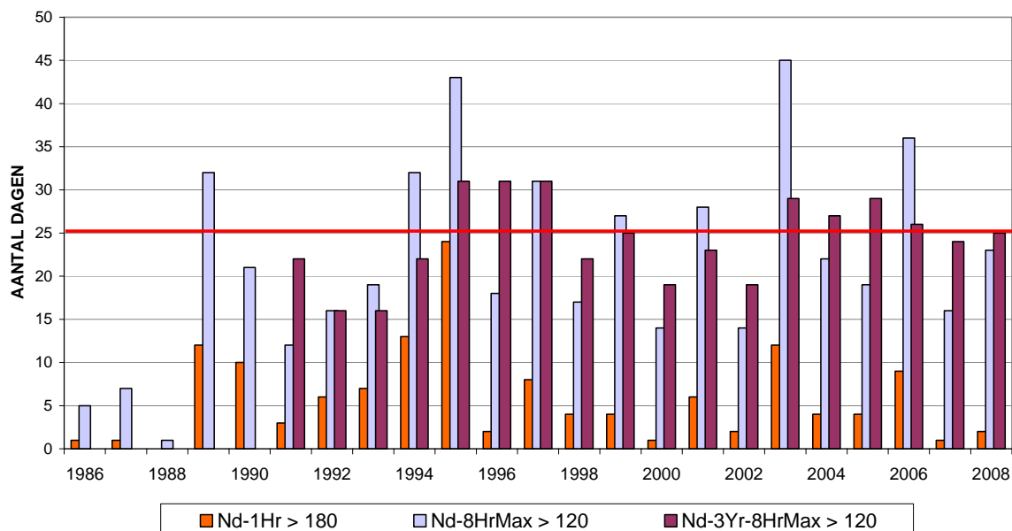
Fig. 21 : Ozon : aantal dagen met overschrijdingen in het Gewest Jaarperioden: 1 januari – 31 december (1986-2007) Voorlopige resultaten voor het jaar 2008 (1 januari – 30 september)
