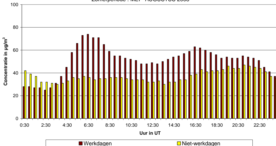
Fig. 54.a : Kroonlaan te Elsene : Gemiddeld dagverloop van de NO 2 -concentratie op werkdagen en niet-werkdagen tijdens de periode mei - augustus 2008
