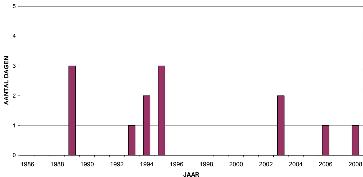
Fig. 18 : Ozon - Evolutie aantal overschrijdingsdagen in het Brussels Hoofdstedelijk Gewest Alarmdrempel: Uurwaarde > 240 \mu\text{g}/\text{m}^3
