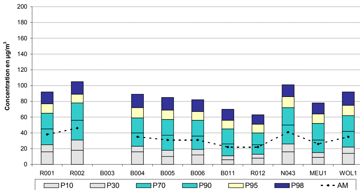
NO 2 - COMPARAISON POSTES de MESURE DISTRIBUTION DES FREQUENCES CUMULEES - VALEURS HORAIRES Période ESTIVALE "AVRIL - SEPTEMBRE 2009"
