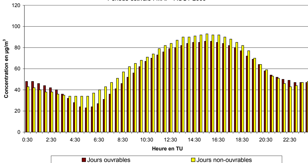
Fig. 47.a : Berchem-Ste-Agathe : Évolution journalière moyenne de la concentration en \text{O}_3 les jours ouvrables et non-ouvrables pendant la période mai - août 2009
