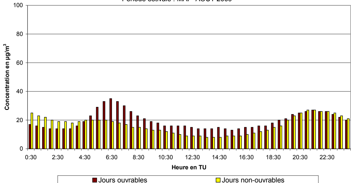
Fig. 46.b : Uccle : Évolution journalière moyenne de la concentration en NO 2 les jours ouvrables et non-ouvrables pendant la période mai - août 2009
