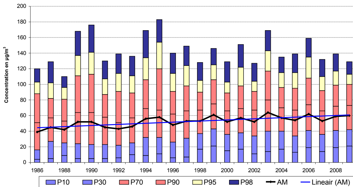
Fig. 70 : Ozone à Uccle – Valeurs horaires –évolution à long terme Périodes estivales 1986 - 2009
