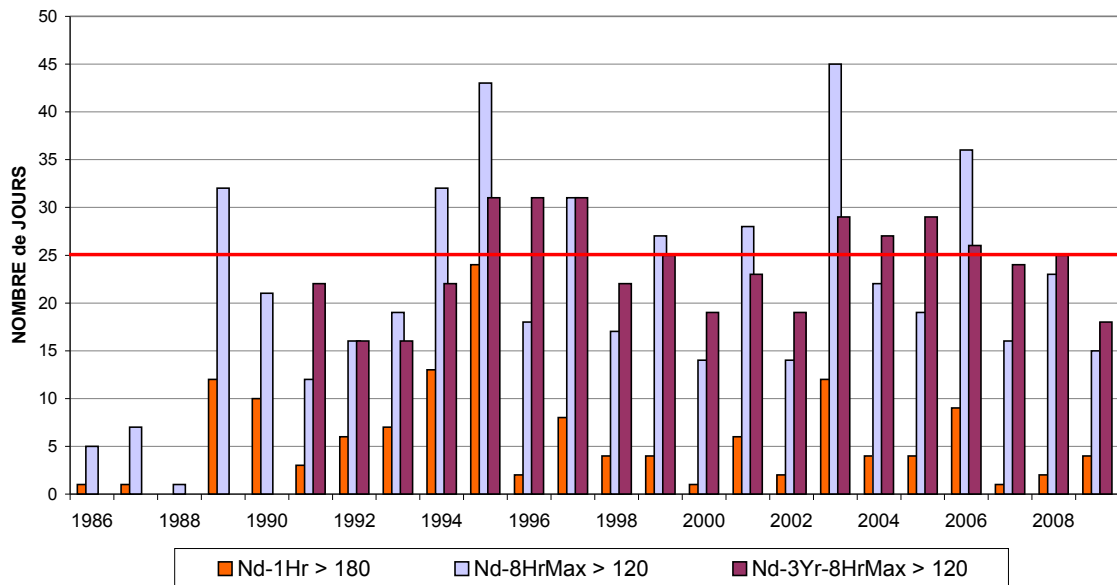
Fig. 21 : Ozone : nombre de jours avec dépassements en Région de Bruxelles-Capitale Périodes annuelles : 1 janvier – 31 décembre (1986 – 2008) Données partielles pour l'année 2009 (1 er janvier – 31 octobre)
