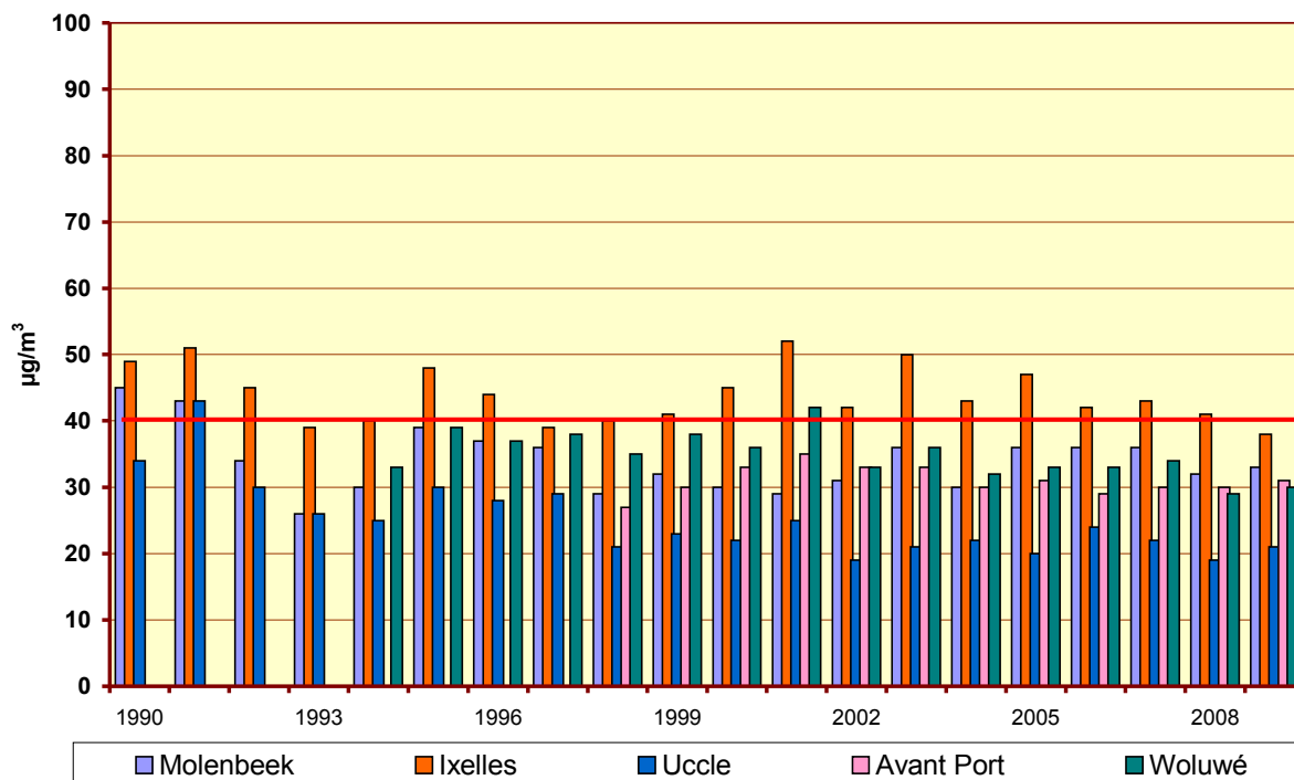
Fig. 27.d : NO 2 – Évolution de la concentration moyenne les 'Dimanches' Périodes annuelles 1990 – 2008 et « Janvier – Octobre 2009 »
