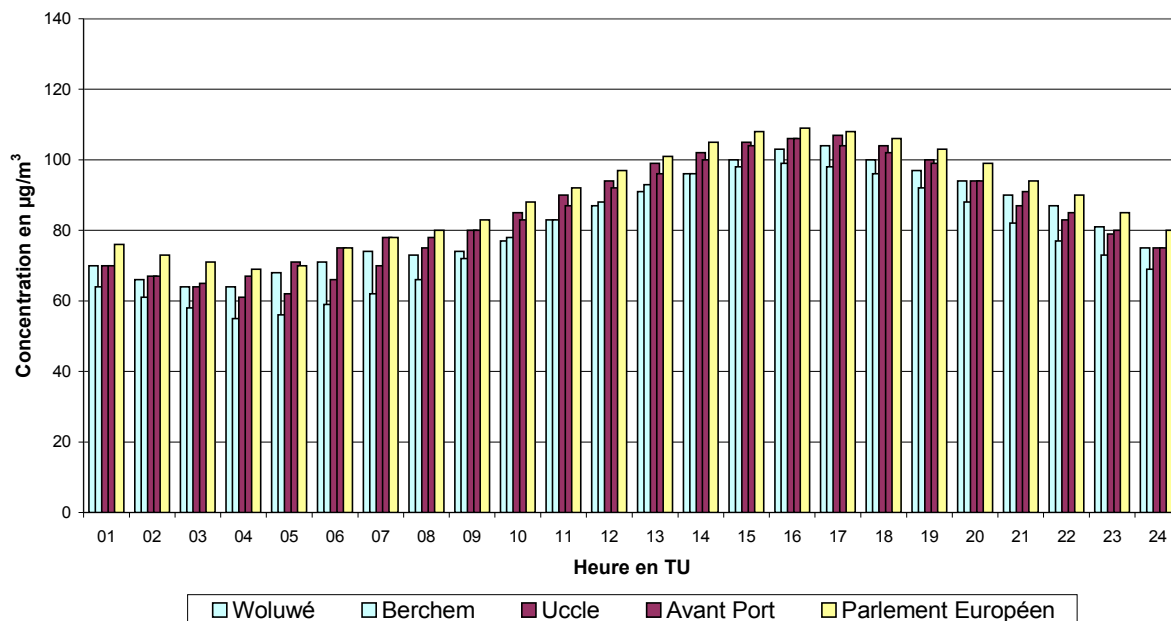
Fig. 10 : Évolution journalière moyenne des concentrations en [O 3 + NO 2 ], exprimées en équivalent O 3 , durant la période mai – août 2009
