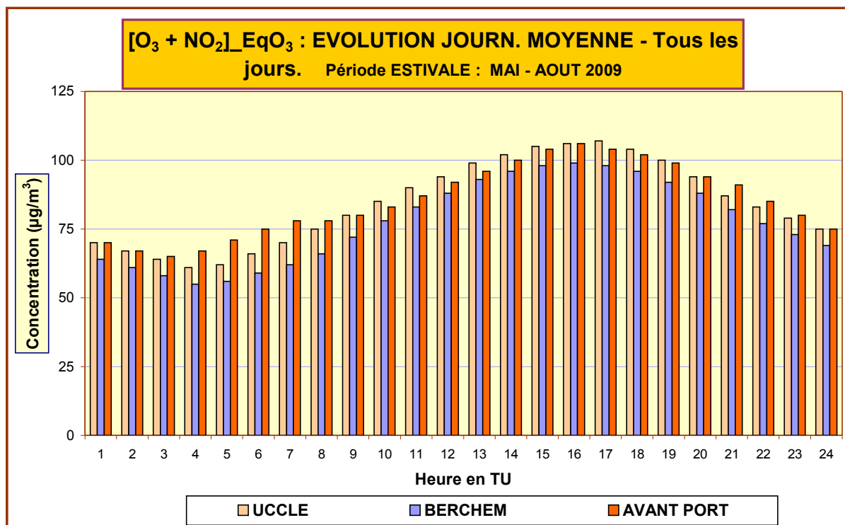
Fig. 67 : [O 3 + NO 2 ] – Évolution journalière moyenne – Comparaison entre 3 postes de mesure Période « mai –août 2009 »
