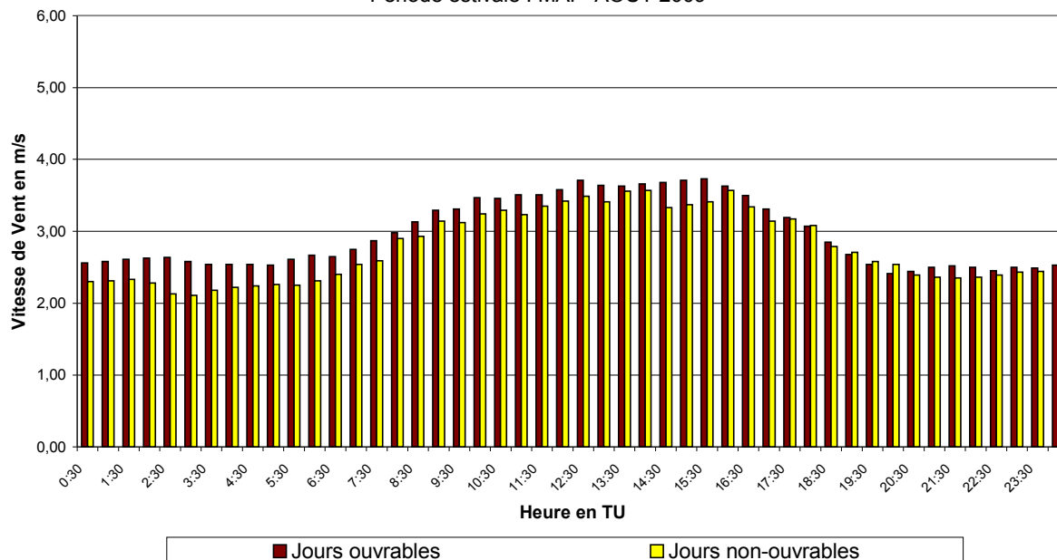
Fig. 55.b : Uccle : Évolution journalière moyenne de la vitesse de vent les jours ouvrables et non-ouvrables pendant la période mai – août 2009
