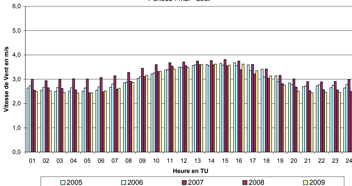
Fig. 38 : Vitesse de vent - évolution journalière moyenne Périodes estivales « mai – août » 2005, 2006, 2007, 2008 et 2009
