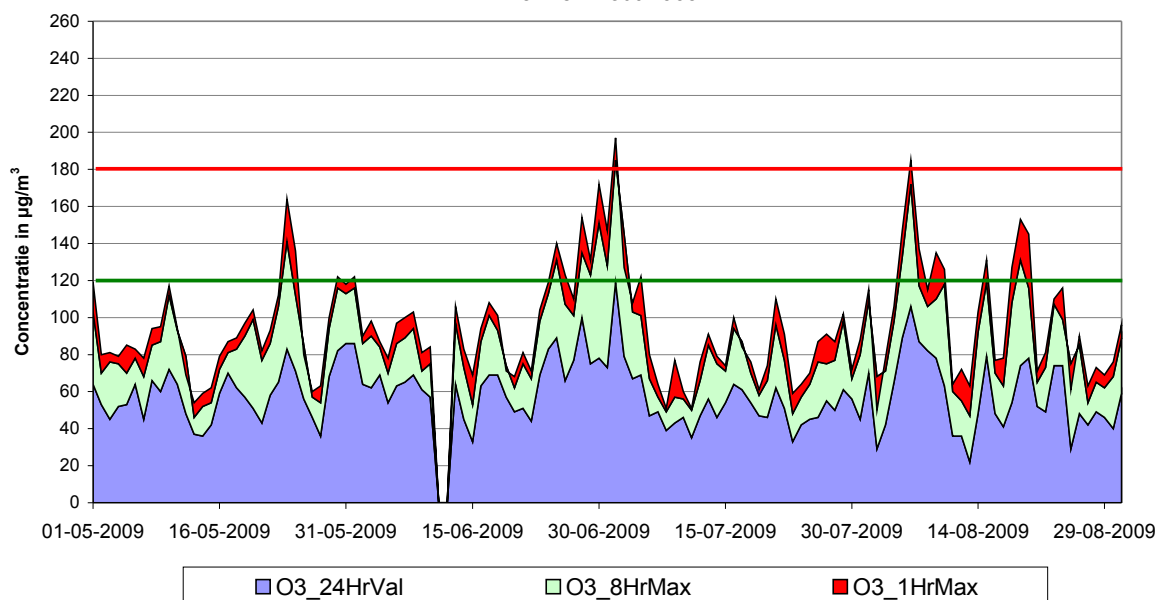
Fig. 22 : Ozone – Évolution Valeur Journalière (24HrVal), valeur maximale sur 8 heures (8HrMax) et valeur maximale horaire (1HrMax). Période : mai – août 2009. Postes de mesure à Uccle et Berchem-Ste-Agathe
