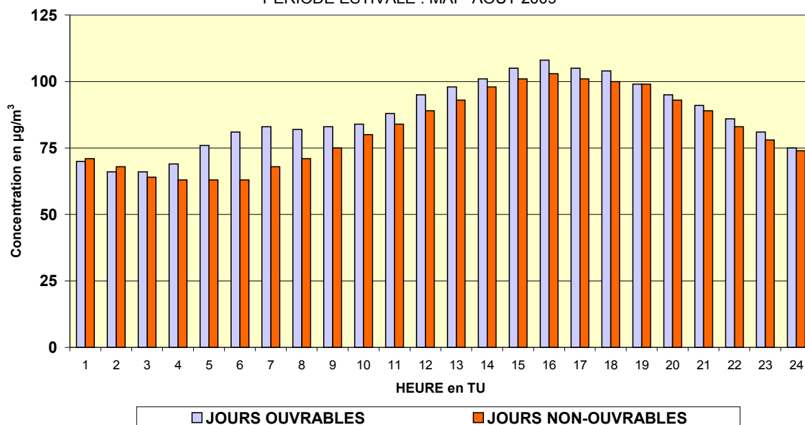
Fig. 69 : [O 3 + NO 2 ] – Évolution journalière moyenne les jours ouvrables et les jours non ouvrables Postes de mesure d'Uccle et de l'Avant Port (trafic) - Période « mai –août 2009 »
