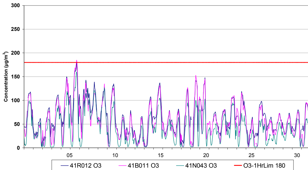
Fig. 6 : Évolution des concentrations horaires en Ozone – Uccle, Berchem et Avant Port – Août 2009
