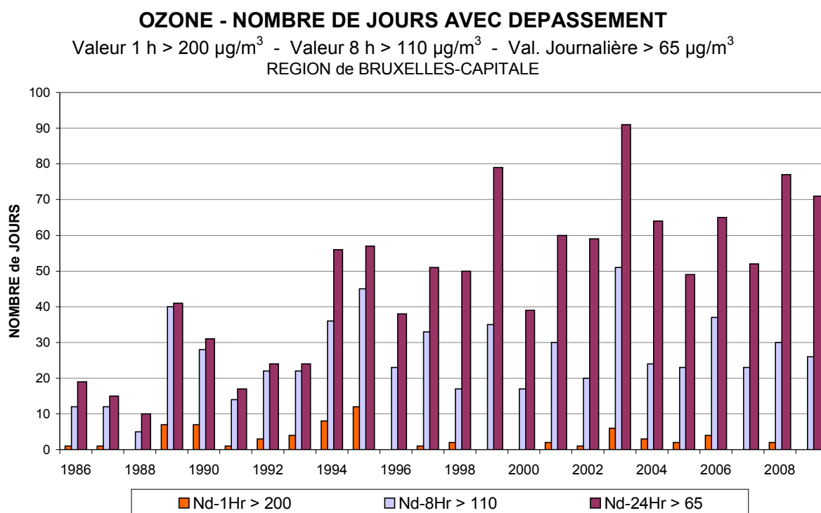
Fig. 25 : Ozone : nombre de jours avec dépassements (directive 92/72/CE) Période : janvier - décembre (1986 à 2008) 2009 : Janvier - Octobre
