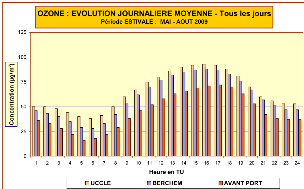
Fig. 65 : Ozone – Évolution journalière moyenne – Comparaison entre 3 postes de mesure Période « mai –août 2009 »
