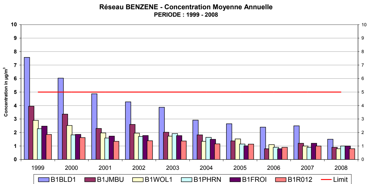
Fig. 30 : Réseau Benzène – Évolution de la concentration moyenne annuelle dans quelques postes de mesure. Période 1999 - 2008
