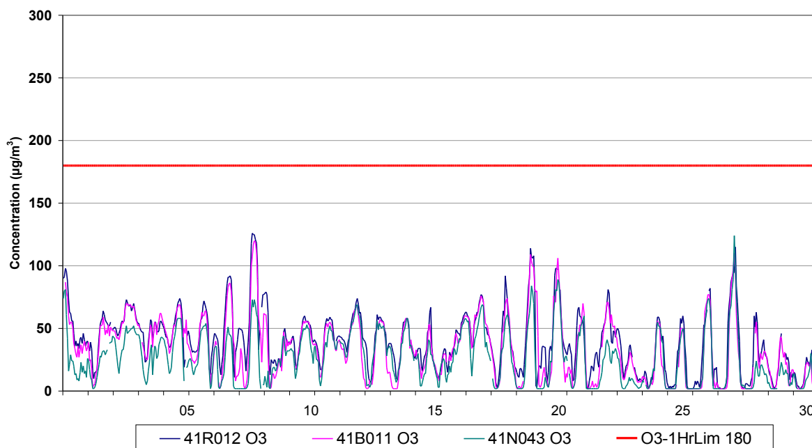
Fig. 7 : Évolution des concentrations horaires en Ozone – Uccle, Berchem et Avant Port – Septembre 2009
