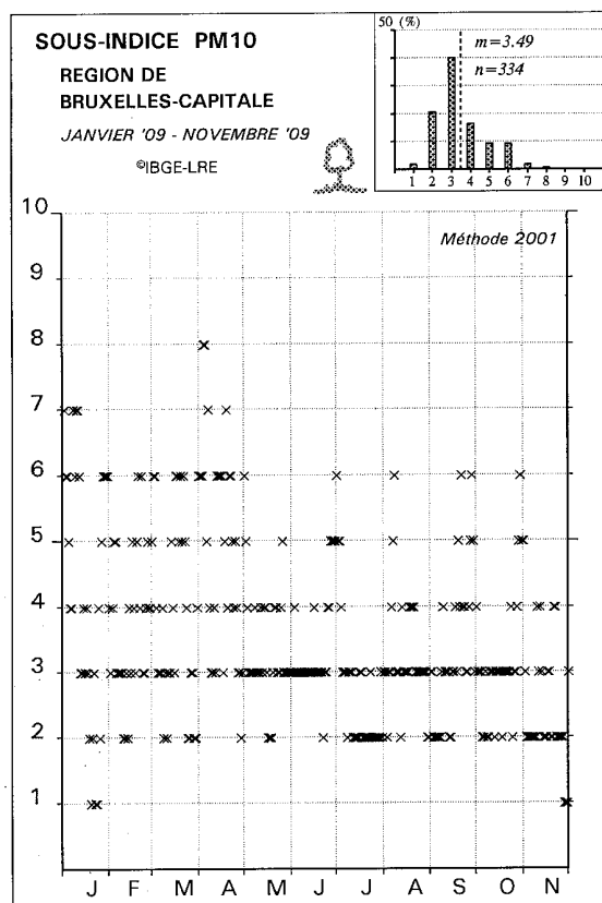
Fig. 60 : Les sous-indices pour NO 2 , O 3 et PM10 - Indice général (2009)
