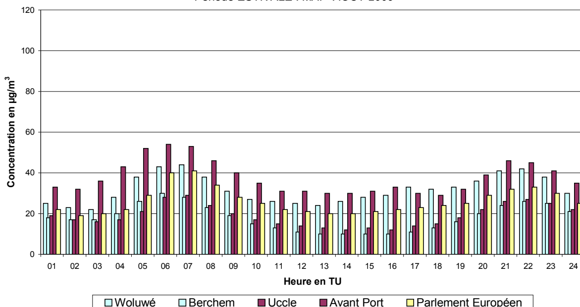
Fig. 9 : Évolution journalière moyenne des concentrations en NO 2 durant la période mai-août 2009
