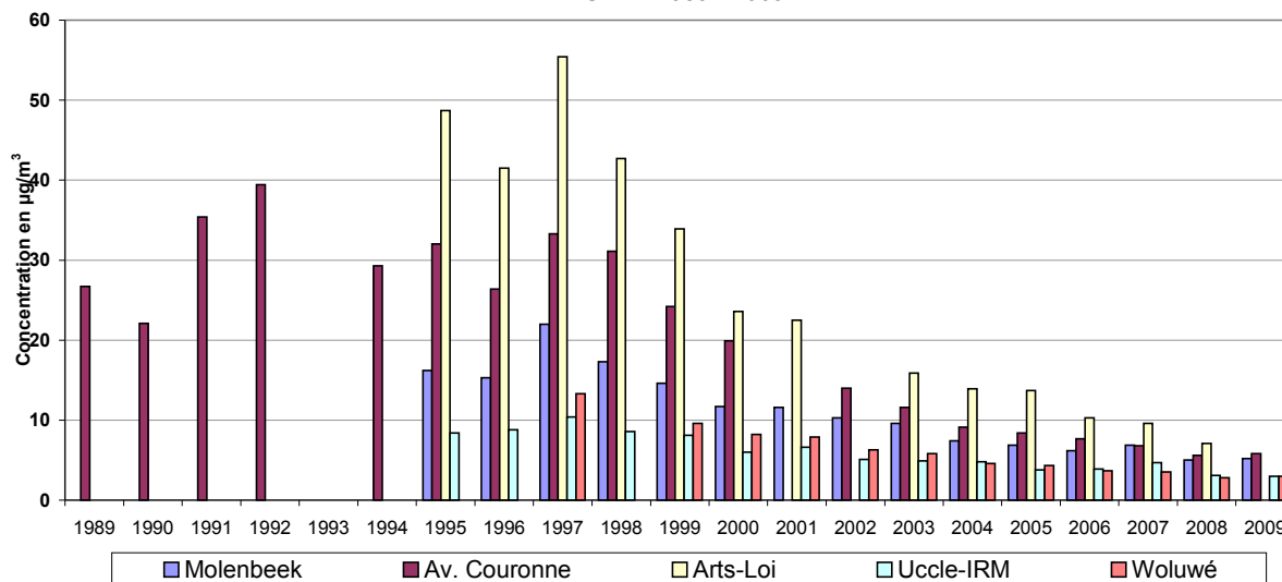
Fig. 29 : Toluène – Évolution de la concentration moyenne annuelle Période : Janvier – Décembre (1989-2008) et 'Janvier – Septembre 2009'
