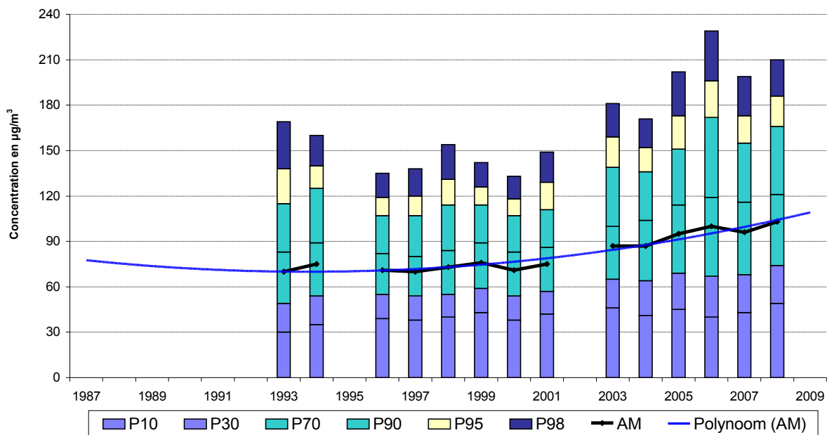
Fig. 41 : Arts-Loi – Évolution de Valeurs Horaires en NO 2 Période estivale « avril – septembre » (1993-2009)
