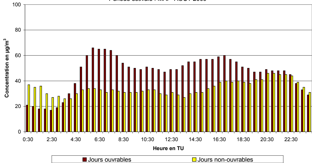
Fig. 54.a : Avenue de la Couronne à Ixelles : Évolution journalière moyenne de la concentration en NO 2 les jours ouvrables et non-ouvrables pendant la période mai - août 2009
