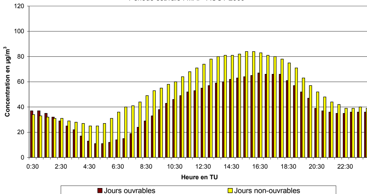
Fig. 49.a : Avant Port : Évolution journalière moyenne de la concentration en O 3 les jours ouvrables et non-ouvrables pendant la période mai - août 2009
