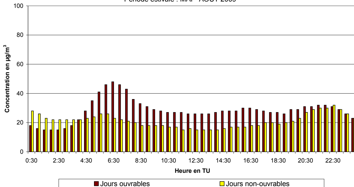
Fig. 53.a : Eastman-Belliard : Évolution journalière moyenne de la concentration en NO 2 les jours ouvrables et non-ouvrables pendant la période mai - août 2009
