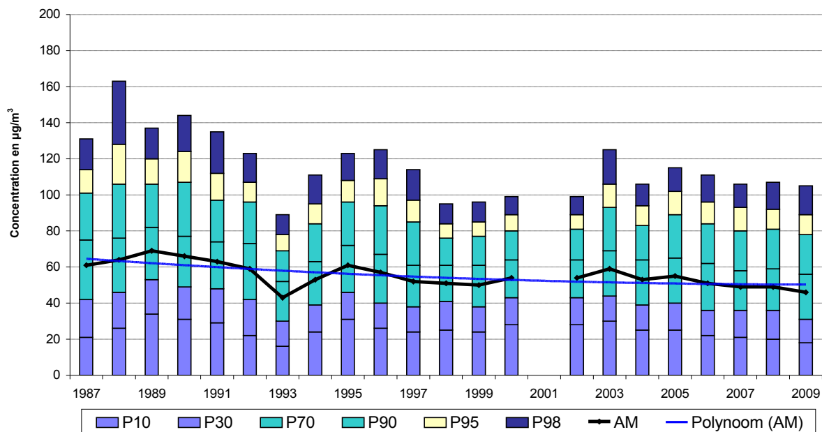
Fig. 40 : Ixelles – Évolution de Valeurs Horaires en NO 2 Période estivale « avril – septembre » (1991-2009)
