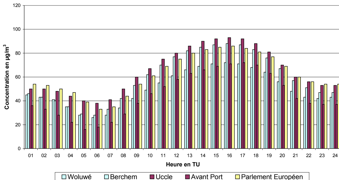
Fig. 8 : Évolution journalière moyenne des concentrations en O 3 durant la période mai-août 2009
