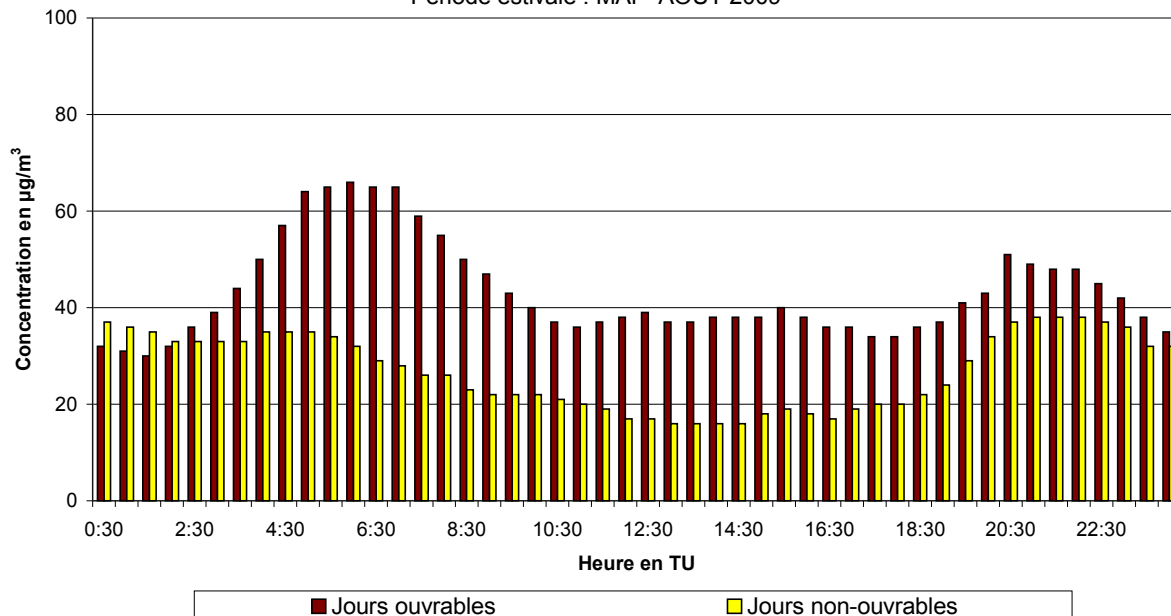
Fig. 49.b : Avant Port : Évolution journalière moyenne de la concentration en NO 2 les jours ouvrables et non-ouvrables pendant la période mai - août 2009
