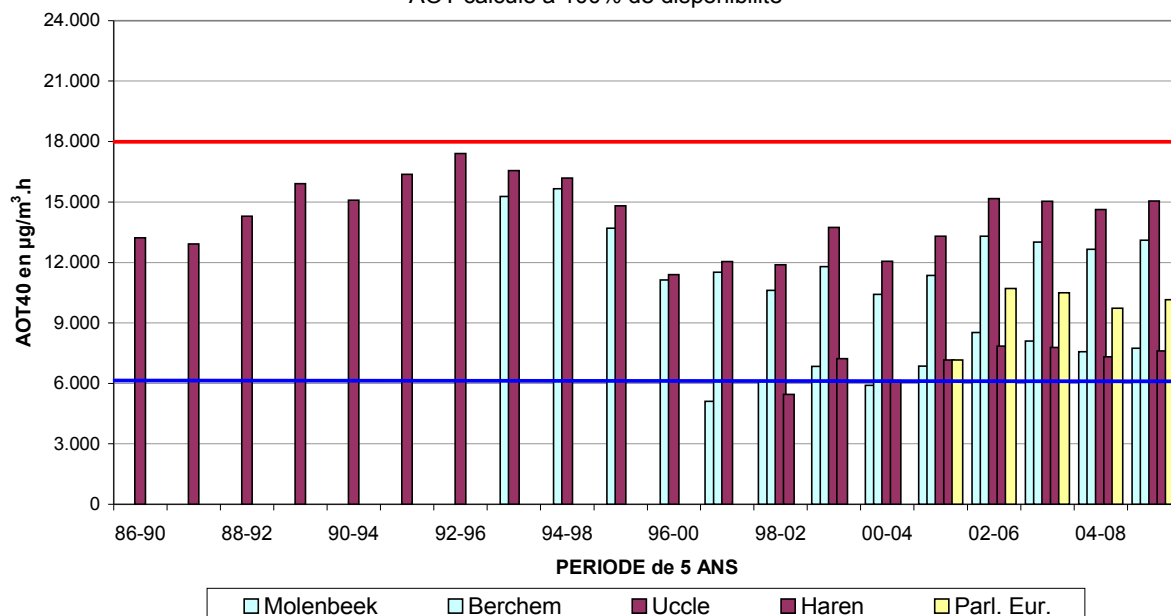
Fig. 15 : Évolution AOT40-MJ dans le temps (1986-2009) AOT40 pour la période Mai – Juillet, 8-20 h d'Europe centrale Résultats par an et moyenné sur 5 ans
