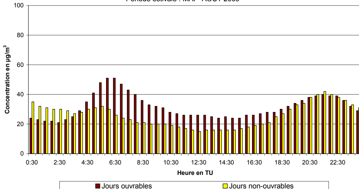
Fig. 52.b : Ste-Catherine : Évolution journalière moyenne de la concentration en NO 2 les jours ouvrables et non-ouvrables pendant la période mai – août 2009
