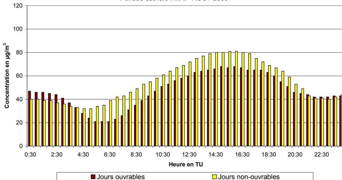
Fig. 50.a : Woluwé-St-Lambert : Évolution journalière moyenne de la concentration en O 3 les jours ouvrables et non-ouvrables pendant la période mai - août 2009
