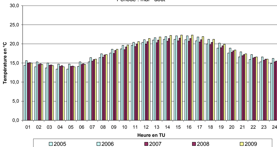
Fig. 37 : Température - évolution journalière moyenne Périodes estivales « mai – août » 2005, 2006, 2007, 2008 et 2009
