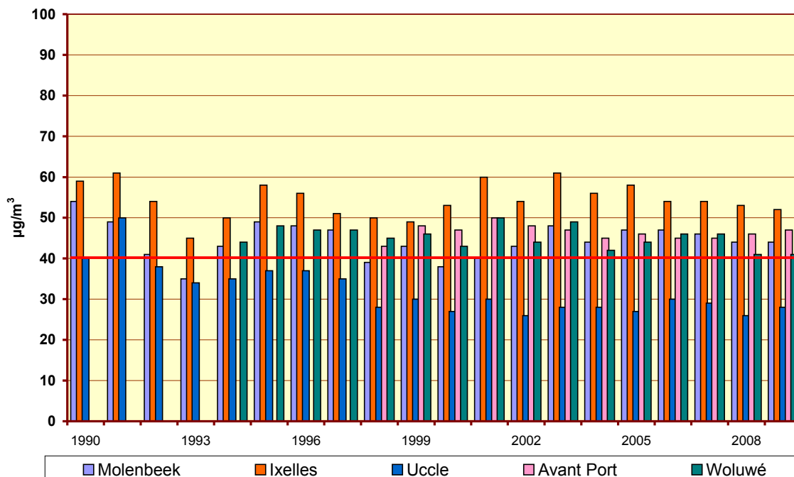
Fig. 27.a : NO 2 – Évolution de la concentration moyenne annuelle ( tous les jours ) Périodes annuelles 1990 – 2008 et « Janvier – Octobre 2009 »
