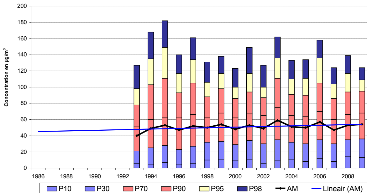
Fig. 34 : Berchem-Ste-Agathe - Évolution des Valeurs Horaires en Ozone (1993-2009) Période estivale « avril – septembre »
