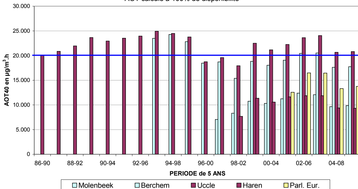
Fig. 16 : Évolution AOT40-AS dans le temps (1986-2009) AOT40 pour la période Avril – Septembre, 8-20 h d'Europe centrale Résultats par an et moyenné sur 5 ans
