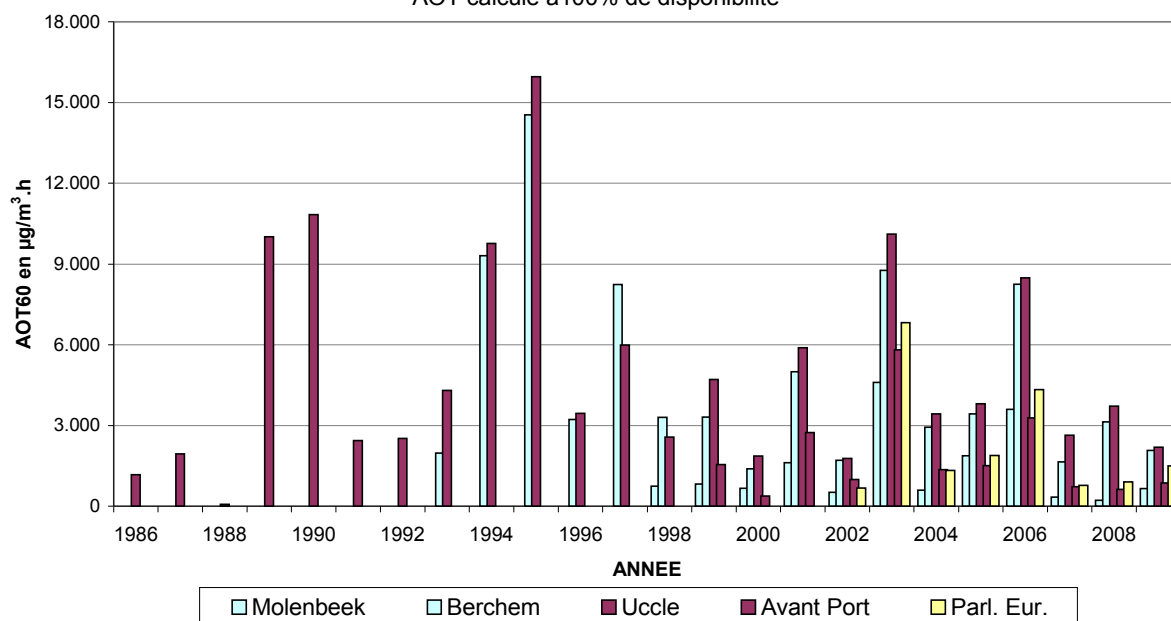
Fig. 24: Évolution AOT60 dans le temps (1986-2009)
