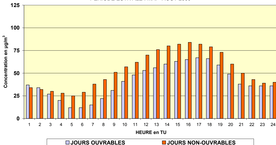
Fig. 68 : Ozone – Évolution journalière moyenne les jours ouvrables et les jours non ouvrables Postes de mesure d'Uccle et de l'Avant Port (trafic) - Période « mai –août 2009 »
