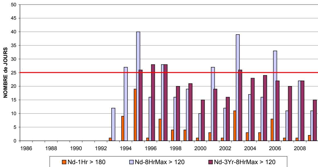
Fig. 20 : Ozone à Berchem : nombre de jours avec dépassements Périodes annuelles : 1 janvier – 31 décembre (1986 – 2008) Données partielles pour l'année 2009 (1 er janvier – 31 octobre)
