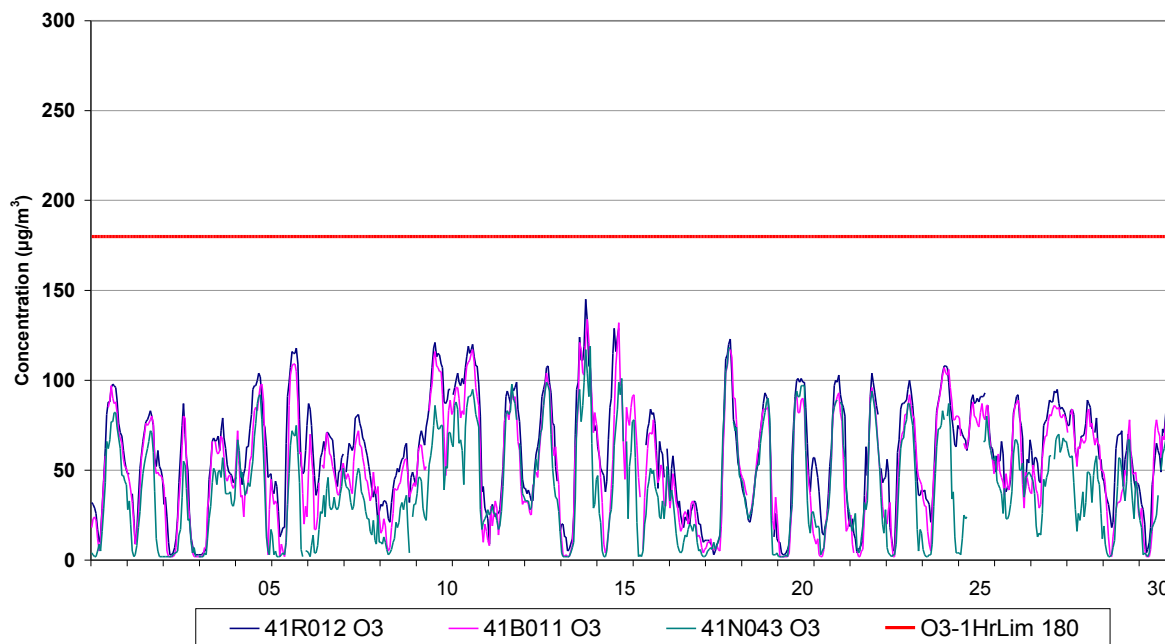
Fig. 2 : Évolution des concentrations horaires en Ozone – Uccle, Berchem et Avant Port – Avril 2009
