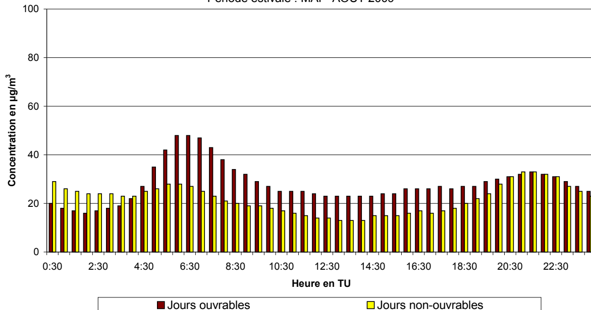
Fig. 51.b : Parlement Européen : Évolution journalière moyenne de la concentration en NO 2 les jours ouvrables et non-ouvrables pendant la période mai – août 2009
