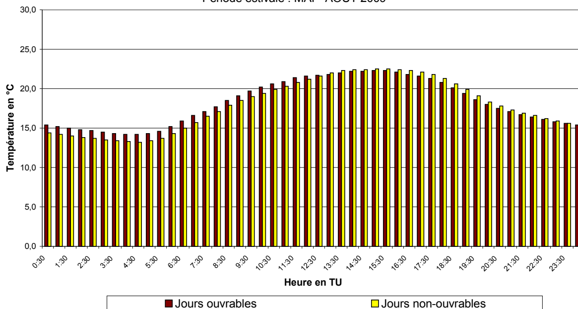
Fig. 55.a : Uccle : Évolution journalière moyenne de la température les jours ouvrables et non-ouvrables pendant la période mai – août 2009
