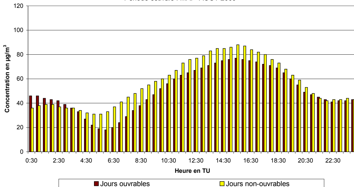
Fig. 52.a : Ste-Catherine : Évolution journalière moyenne de la concentration en O 3 les jours ouvrables et non-ouvrables pendant la période mai - août 2009
