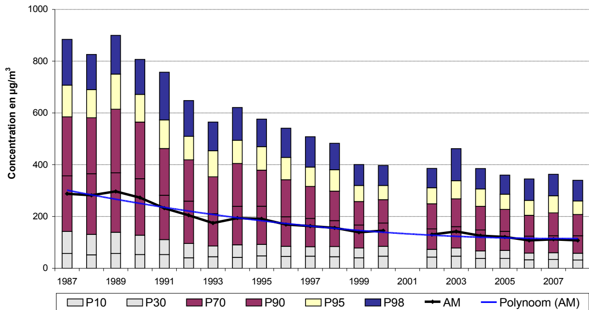
Fig. 72 : NO x à Ixelles – Avenue de la Couronne ( canyon street ) – Valeurs horaires Évolution à long terme - Périodes annuelles 1987 - 2008
