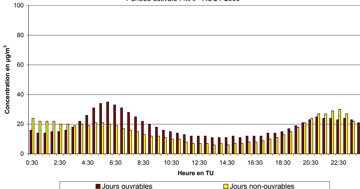
Fig. 47.b : Berchem-Ste-Agathe : Évolution journalière moyenne de la concentration en \text{NO}_2 les jours ouvrables et non-ouvrables pendant le période mai – août 2009
