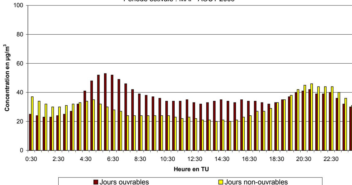
Fig. 48.b : Molenbeek : Évolution journalière moyenne de la concentration en NO 2 les jours ouvrables et non-ouvrables pendant la période mai – août 2009
