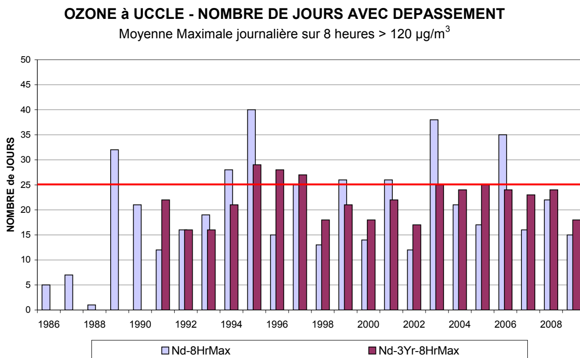
Fig. 12: Ozone – évolution du nombre de jours avec dépassement à Uccle. Valeur cible pour la Santé Publique. Valeur maximale sur 8 heures > 120 µg/m 3 . Période : Janvier – Décembre (1986-2008). [2009] : Janvier - Octobre
