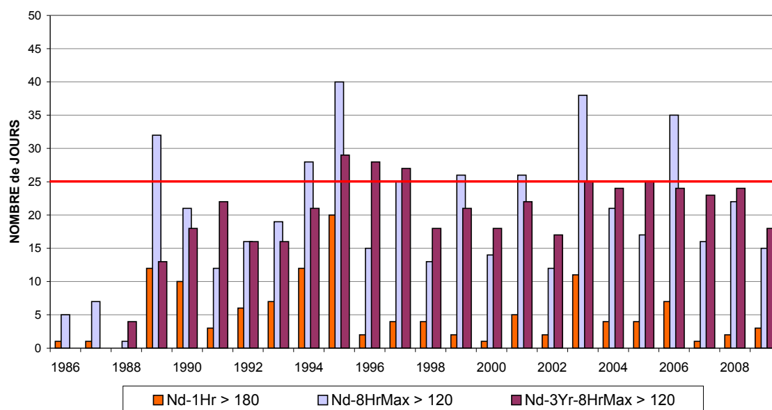
Fig. 19 : Ozone à Uccle : nombre de jours avec dépassements Périodes annuelles : 1 janvier – 31 décembre (1986 – 2008) Données partielles pour l'année 2009 (1 er janvier – 31 octobre)
