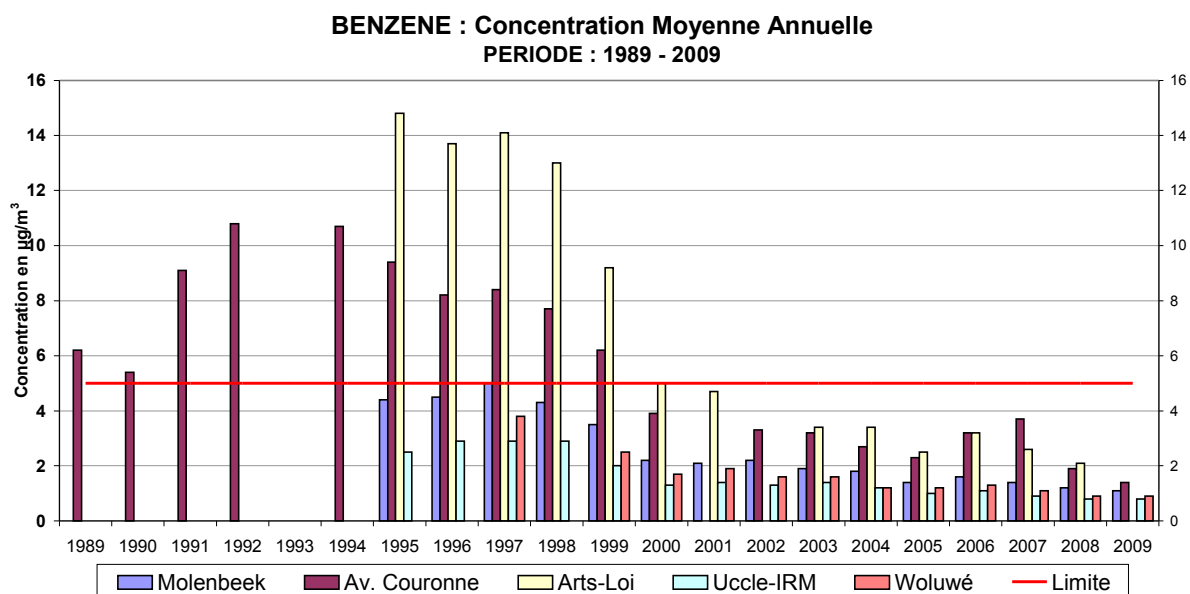
Fig. 28 : Benzène – Évolution de la concentration moyenne annuelle Période : Janvier – Décembre (1989-2008) et 'Janvier – Septembre 2009'
