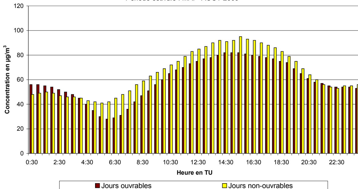
Fig. 51.a : Parlement Européen : Évolution journalière moyenne de la concentration en O 3 les jours ouvrables et non-ouvrables pendant la période mai - août 2009
