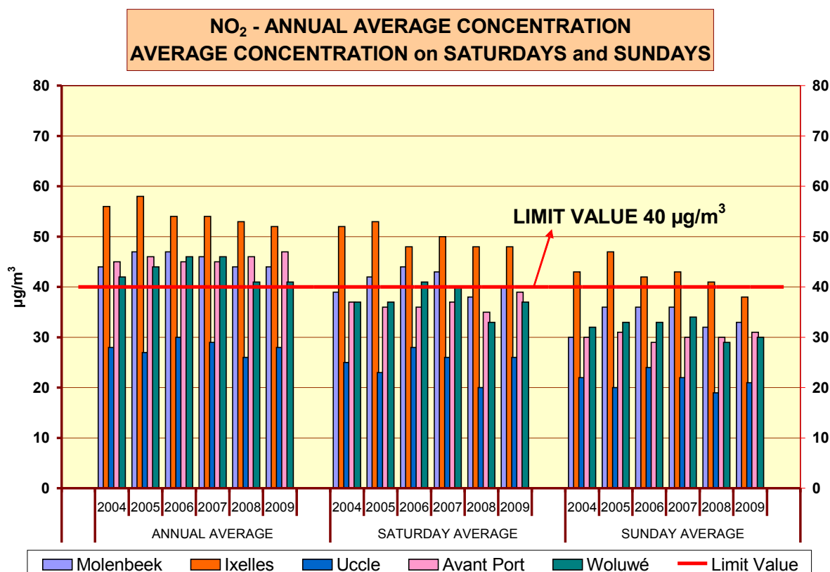
Fig. 26 : NO 2 – Comparaison entre la concentration moyenne annuelle et la concentration moyenne des 'Samedis' et des 'Dimanches' pour une sélection de postes de mesure. Périodes annuelles 2004-2008 et "Janvier – Octobre 2009"
