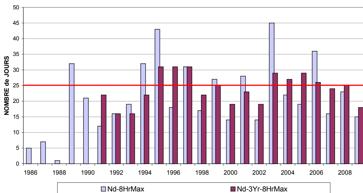
Fig. 14: Ozone – évolution du nombre de jours avec dépassement dans la Région. Valeur cible pour la Santé Publique. Valeur maximale sur 8 heures > 120 µg/m 3 . Période : Janvier – Décembre (1986-2008). [2009] : Janvier - Octobre
