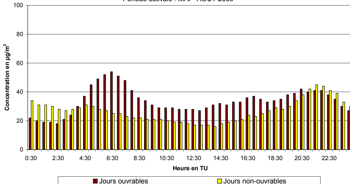
Fig. 50.b : Woluwé-St-Lambert : Évolution journalière moyenne de la concentration en NO 2 les jours ouvrables et non-ouvrables pendant la période mai – août 2009
