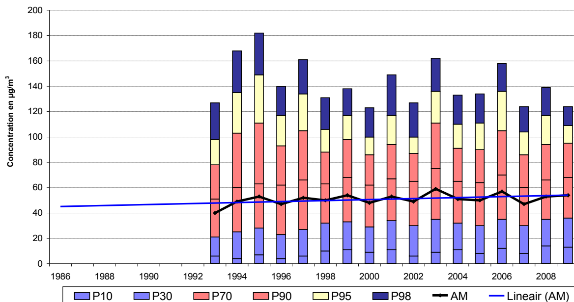
Fig. 71 : Ozone à Berchem-Ste-Agathe – Valeurs horaires –évolution à long terme Périodes estivales 1993 - 2009
