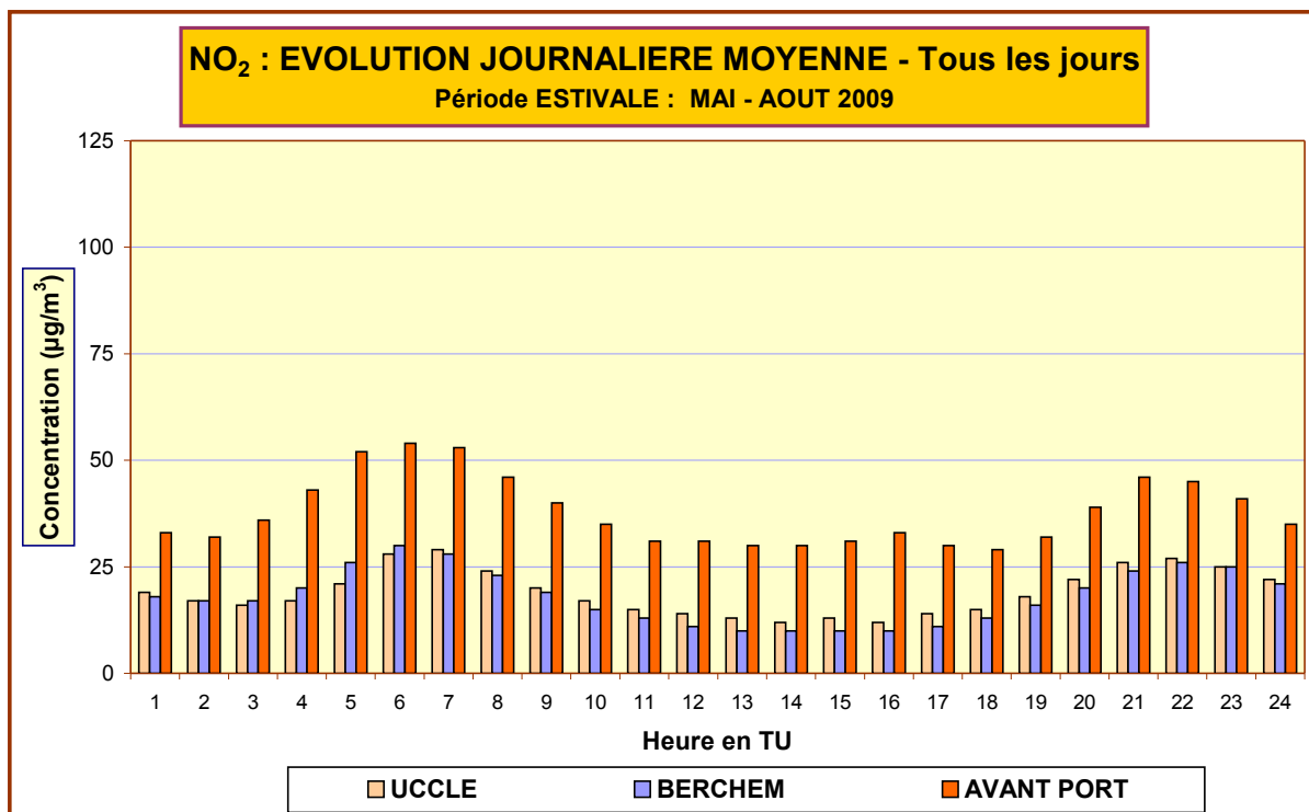
Fig. 66 : NO 2 – Évolution journalière moyenne – Comparaison entre 3 postes de mesure Période « mai –août 2009 »
