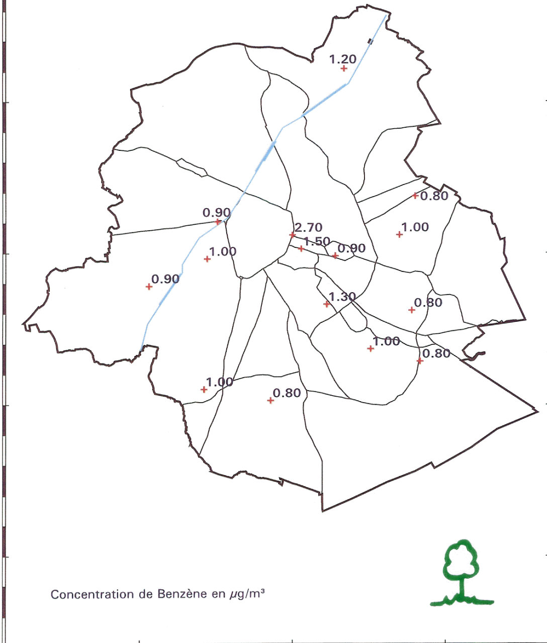
Fig. 31 : Benzène – Distribution spatiale de concentration moyenne annuelle en 2008
