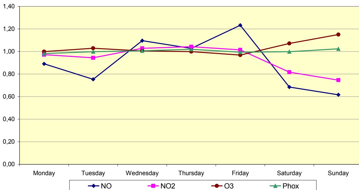
Fig. 59.a : Poste de mesure à Uccle – Profil hebdomadaire moyen des concentrations en NO, NO 2 , O 3 et [NO 2 +O 3 ] sur trois périodes estivales successives : ‘avril – septembre’ 2007, 2008 et 2009
