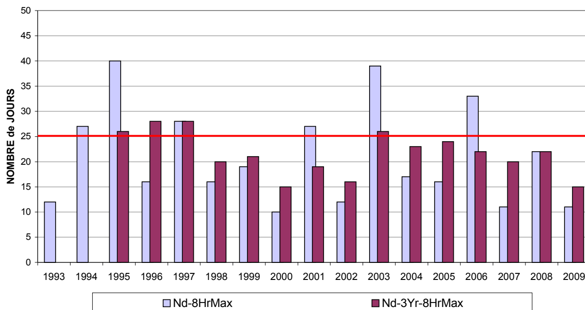
Fig. 13: Ozone – évolution du nombre de jours avec dépassement à Berchem. Valeur cible pour la Santé Publique. Valeur maximale sur 8 heures > 120 µg/m 3 . Période : Janvier – Décembre (1993-2008). [2009] : Janvier - Octobre
