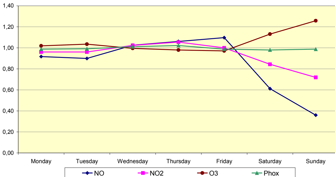
Fig. 59.b : Poste de mesure à Molenbeek – Profil hebdomadaire moyen des concentrations en NO, NO 2 , O 3 et [NO 2 +O 3 ] sur trois périodes estivales successives : ‘avril – septembre’ 2007, 2008 et 2009
