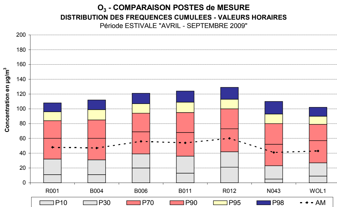
Fig. 32 : Ozone - Distribution de fréquences cumulées - valeurs horaires: avril - septembre 2009
