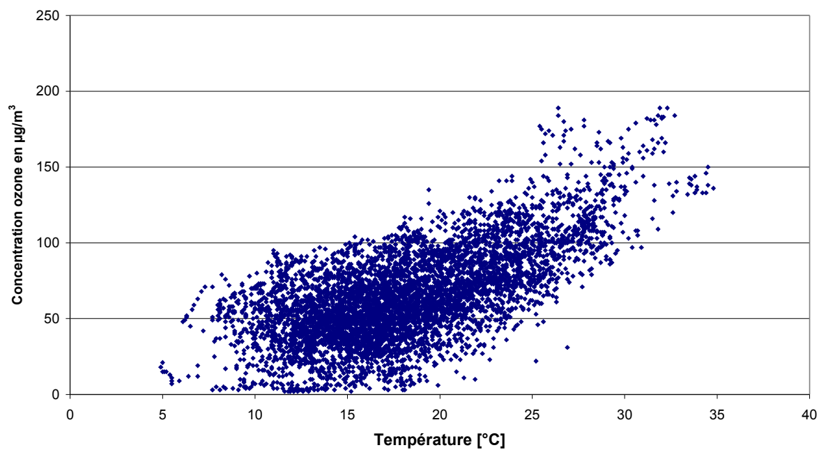
Fig. 42 : Uccle : Concentrations en ozone en fonction de la température (mai - août 2009)
