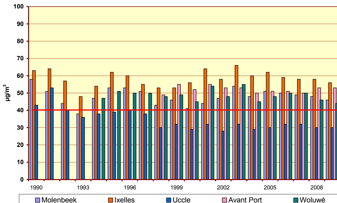
Fig. 27.b : NO 2 – Évolution de la concentration moyenne les ' jours ouvrables ' Périodes annuelles 1990 – 2008 et « Janvier – Octobre 2009 »
