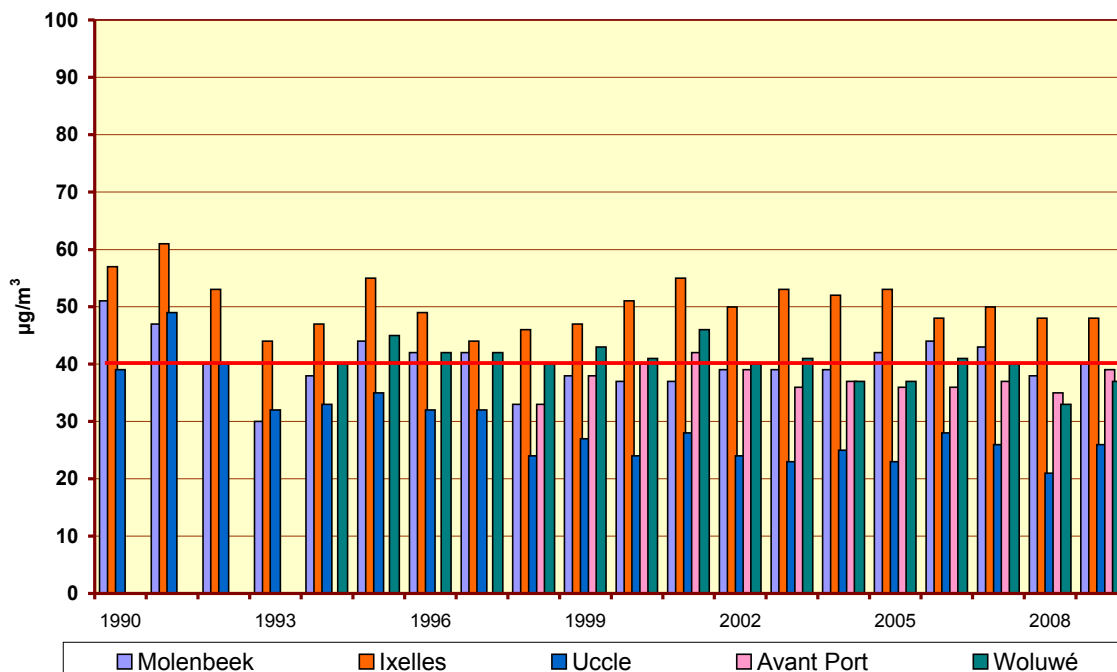
Fig. 27.c : NO 2 – Évolution de la concentration moyenne les 'Samedis' Périodes annuelles 1990 – 2008 et « Janvier – Octobre 2009 »
