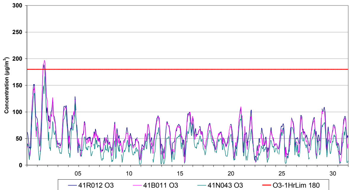
Fig. 5 : Évolution des concentrations horaires en Ozone – Uccle, Berchem et Avant Port – Juillet 2009
