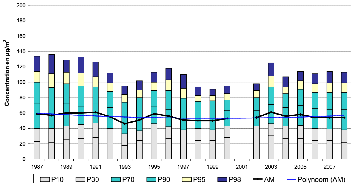
Fig. 73 : NO x à Ixelles – Avenue de la Couronne ( canyon street ) – Valeurs horaires Évolution à long terme - Périodes annuelles 1987 - 2008
