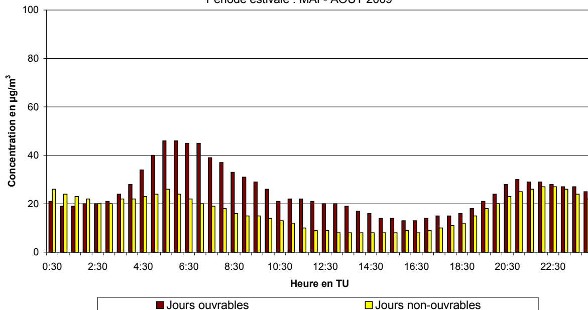
Fig. 53.b : Parc Meudon : Évolution journalière moyenne de la concentration en NO 2 les jours ouvrables et non-ouvrables pendant la période mai - août 2009
