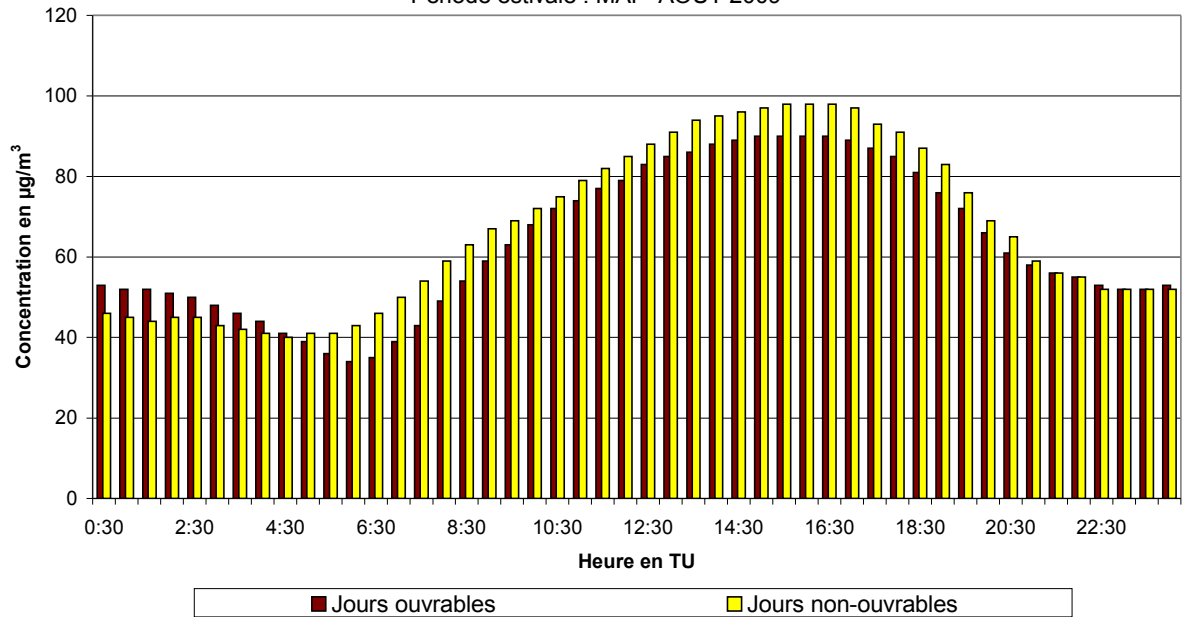
Fig. 46.a : Uccle : Évolution journalière moyenne de la concentration en O 3 les jours ouvrables et non-ouvrables pendant la période mai - août 2009
