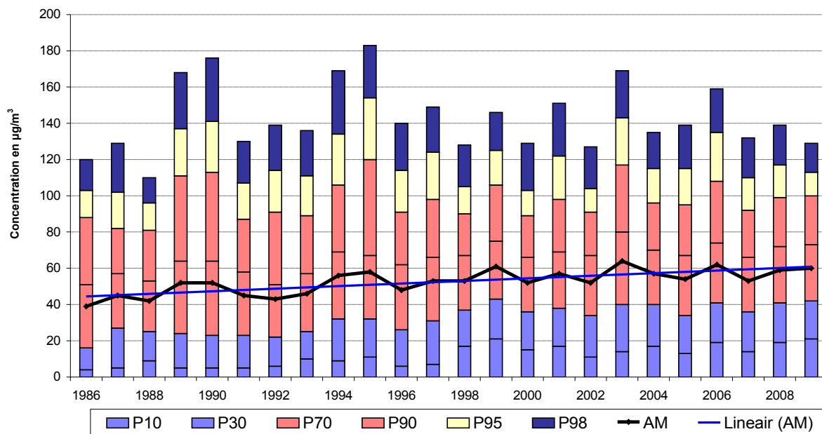
Fig. 33 : Uccle - Évolution des Valeurs Horaires en Ozone (1986-2009) Période estivale « avril – septembre »
