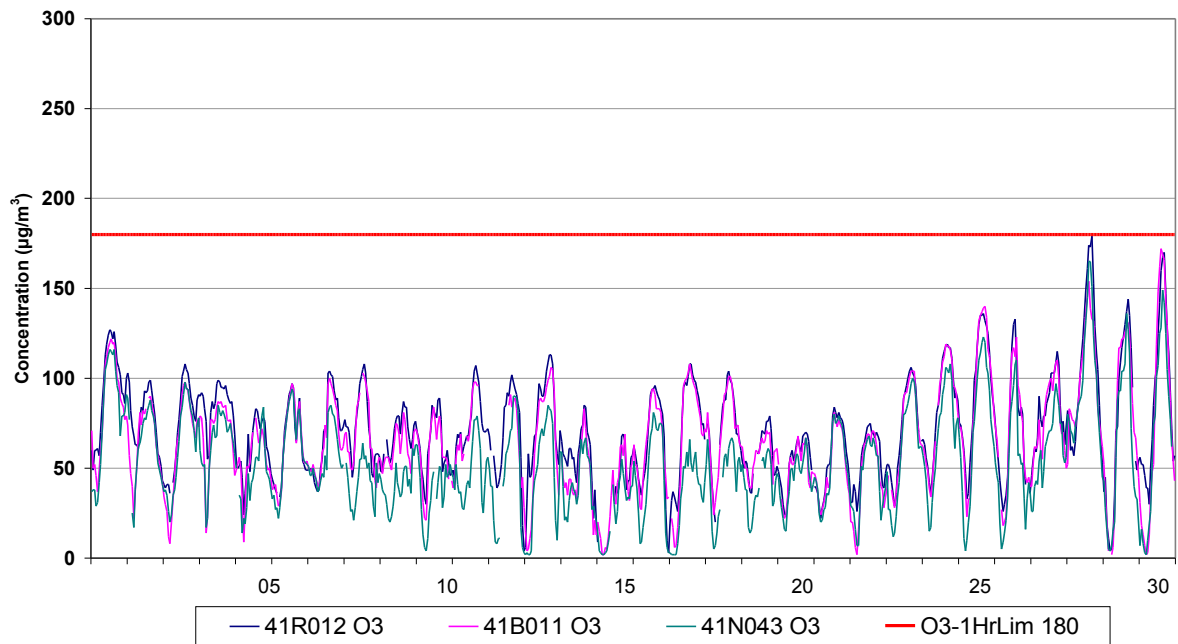
Fig. 4 : Évolution des concentrations horaires en Ozone – Uccle, Berchem et Avant Port – Juin 2009
