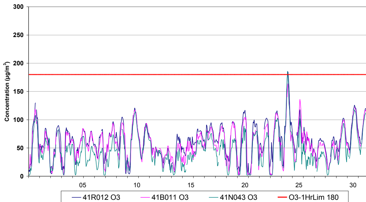
Fig. 3 : Évolution des concentrations horaires en Ozone – Uccle, Berchem et Avant Port – Mai 2009
