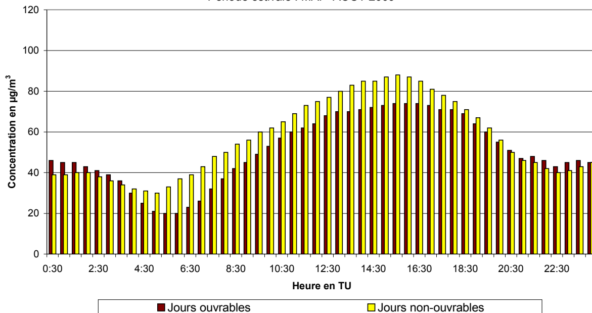
Fig. 48.a : Molenbeek : Évolution journalière moyenne de la concentration en O 3 les jours ouvrables et non-ouvrables pendant la période mai- août 2009
