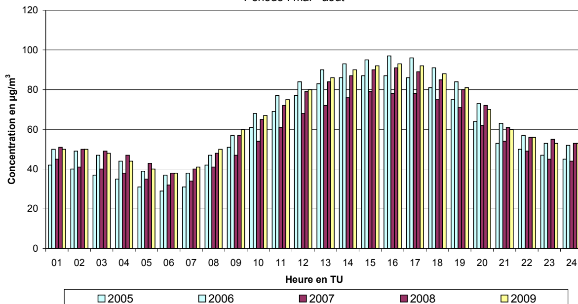
Fig. 35 : Évolution journalière moyenne en ozone à Uccle (R012) Comparaison des niveaux durant les périodes estivales récentes (2005 à 2009)
