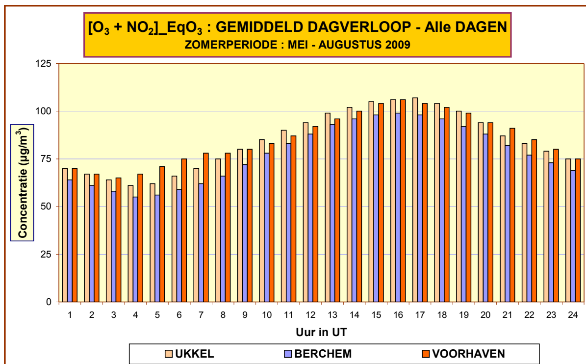
Fig. 67: [O 3 + NO 2 ] – Evolutie Dagverloop – Vergelijking tussen 3 meetposten Periode “mei – augustus 2009”
