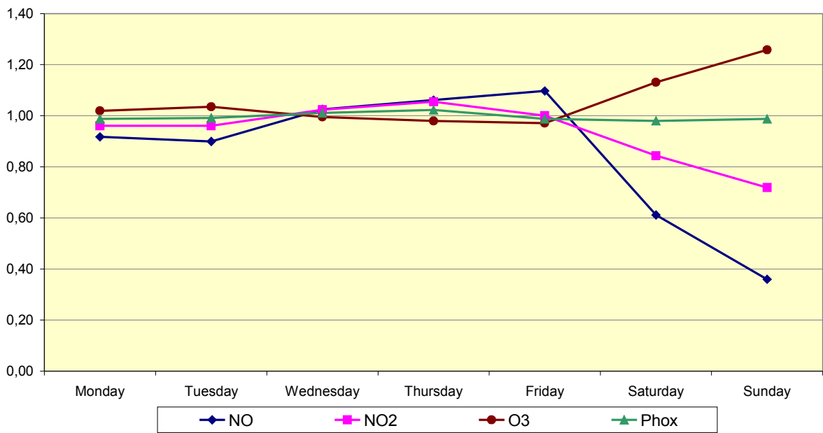
Fig. 59.b : Meetpost te Molenbeek – Gemiddeld weekpatroon voor NO, NO 2 , O 3 en [NO 2 +O 3 ] over drie opeenvolgende zomerperiodes 'april – september' 2007, 2008 en 2009
