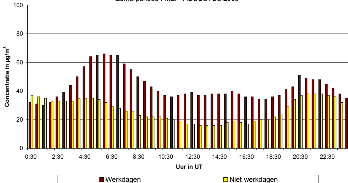
Fig. 49.b : Voorhaven : Gemiddeld dagverloop van de NO 2 -concentratie op werkdagen en niet-werkdagen tijdens de periode mei - augustus 2009
