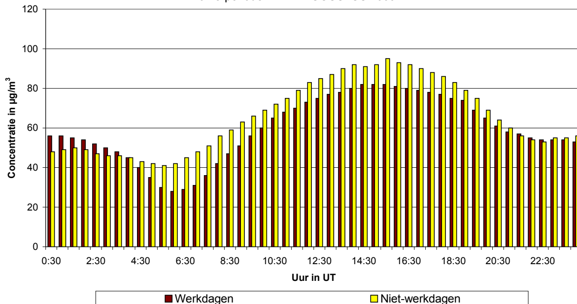
Fig. 51.a : Europees Parlement : Gemiddeld dagverloop van de O 3 -concentratie op werkdagen en niet-werkdagen tijdens de periode mei - augustus 2009
