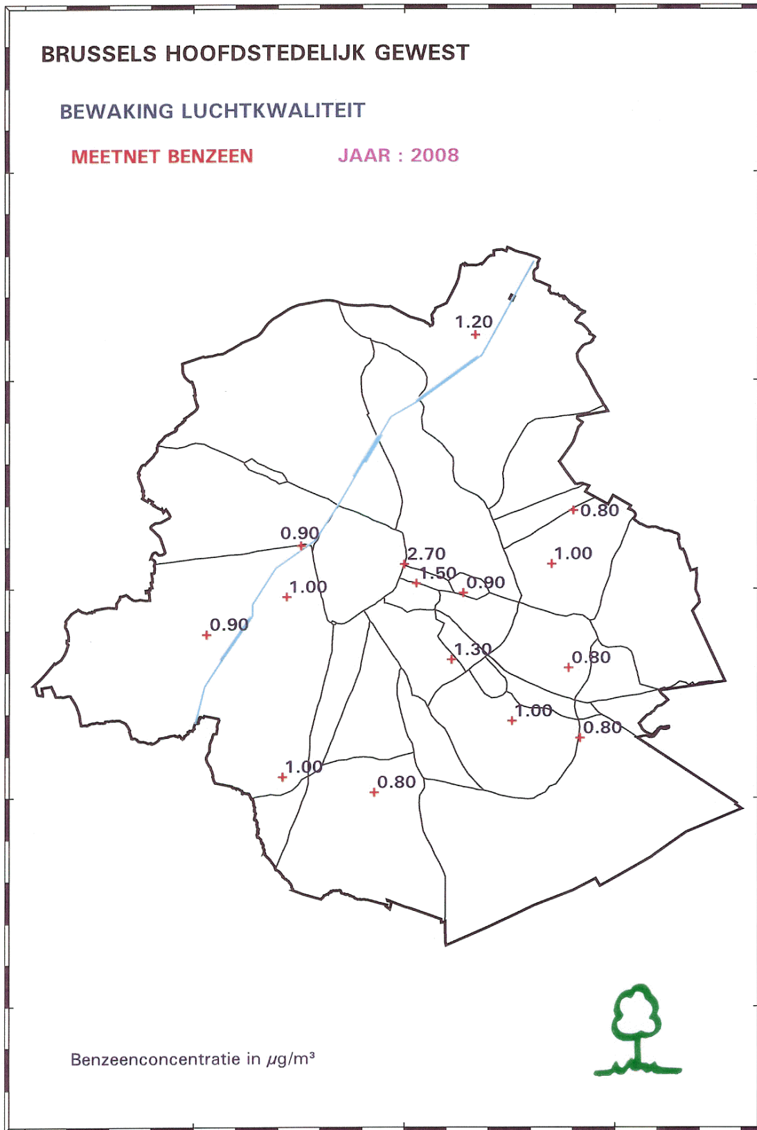
Fig. 31 : Benzeen – Ruimtelijke spreiding jaargemiddelde concentratie in 2008
