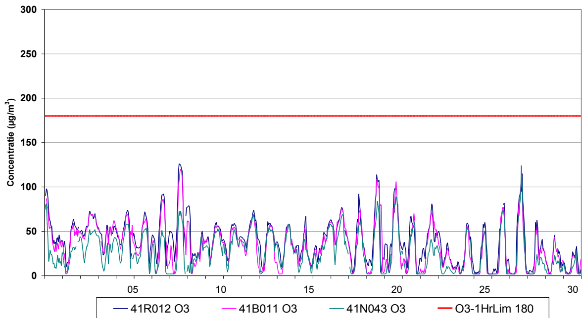
Fig. 7 : Evolutie van de uurwaarden voor ozon – Ukkel, Berchem en Voorhaven – September 2009
