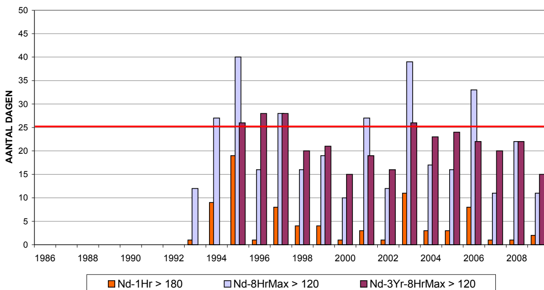
Fig. 20 : Ozon te St.-Ag.-Berchem : aantal dagen met overschrijdingen Jaarperioden: 1 januari – 31 december (1986-2008) Voorlopige resultaten voor het jaar 2009 (1 januari – 31 oktober)
