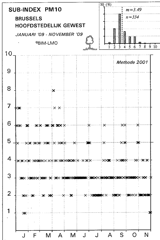
Fig. 60 : Subindexen voor NO 2 , O 3 en PM10 – Index Algemene Luchtkwaliteit (2009)
