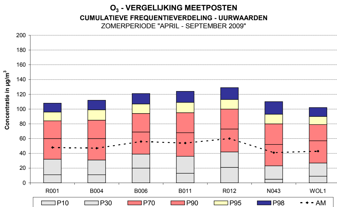
Fig. 32 : Ozon - Cumulatieve frequentieverdeling uurwaarden : april - september 2009
