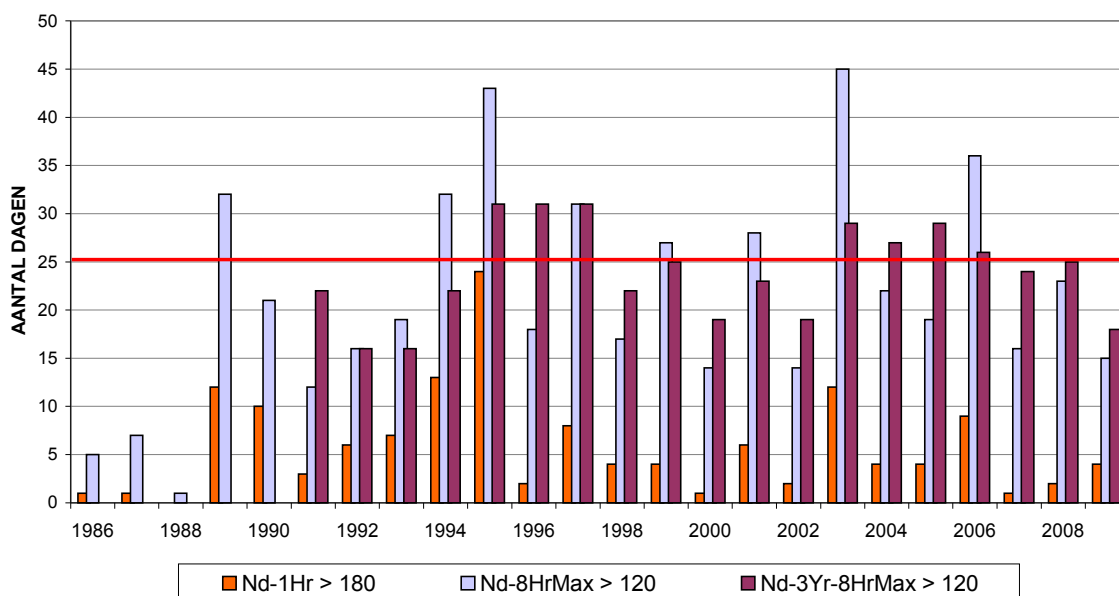
Fig. 21 : Ozon : aantal dagen met overschrijdingen in het Gewest Jaarperioden: 1 januari – 31 december (1986-2008) Voorlopige resultaten voor het jaar 2009 (1 januari – 31 oktober)
