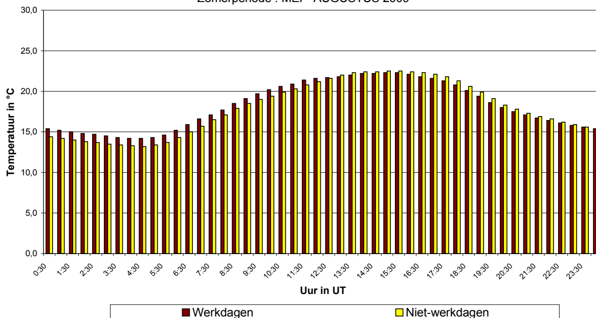
Fig. 55.a : Ukkel : Gemiddeld dagverloop van de temperatuur op werkdagen en niet-werkdagen tijdens de periode mei – augustus 2009
