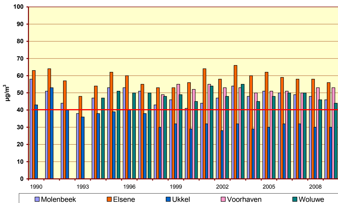
Fig. 27.b : NO 2 - Evolutie gemiddelde concentratie op 'werkdagen' Jaarperiodes 1990-2008 en "Januari – Oktober 2009"
