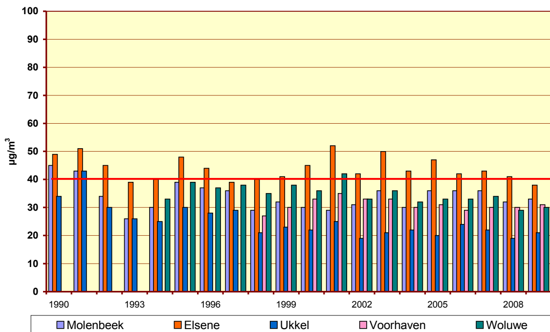
Fig. 27.d : NO 2 - Evolutie gemiddelde concentratie op 'Zondag' Jaarperiodes 1990-2008 en "Januari - Oktober 2009"
