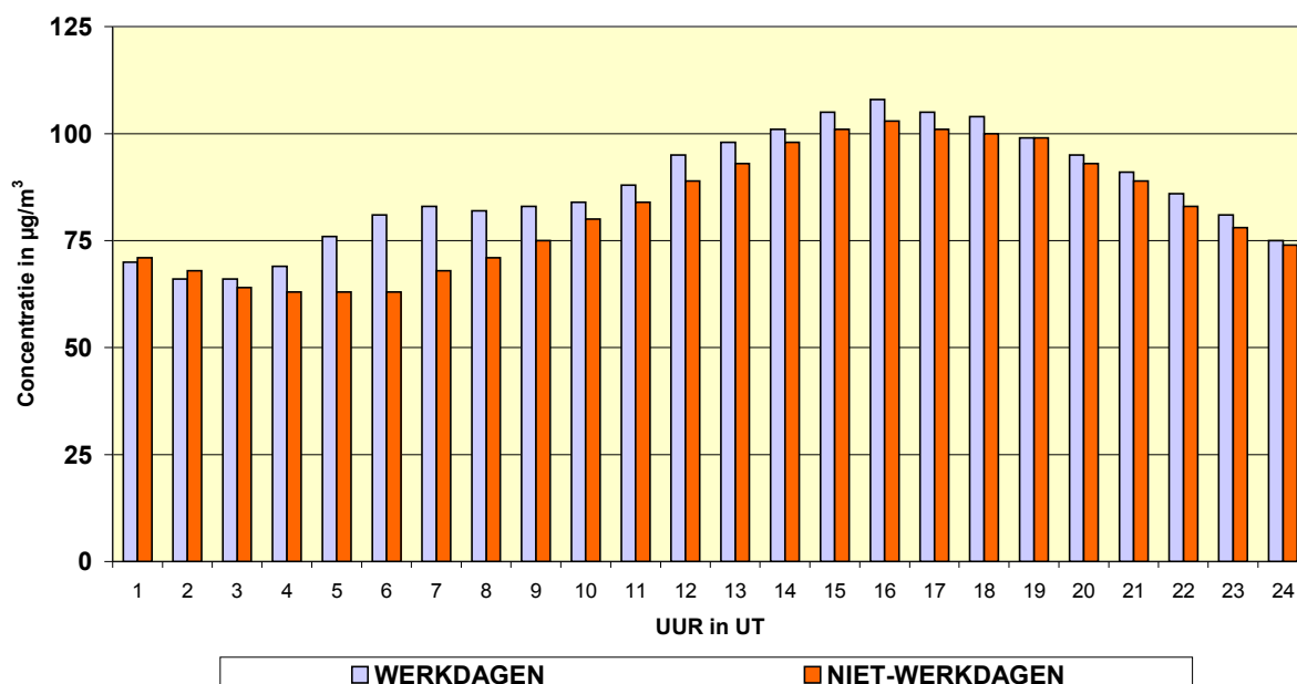
Fig. 69: [O 3 + NO 2 ] – Evolutie Dagverloop voor werkdagen en niet-werkdagen Meetposten Ukkel en Voorhaven - Periode “mei – augustus 2009”
