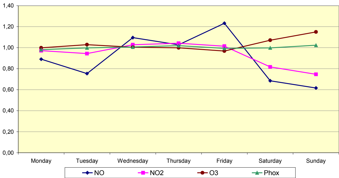
Fig. 59.a : Meetpost te Ukkel – Gemiddeld weekpatroon voor NO, NO 2 , O 3 en [NO 2 +O 3 ] over drie opeenvolgende zomerperiodes 'april – september' 2007, 2008 en 2009
