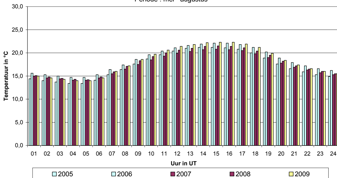
Gemiddeld dagverloop Temperatuur Vergelijking 2005, 2006, 2007, 2008 en 2009 Periode : mei - augustus
