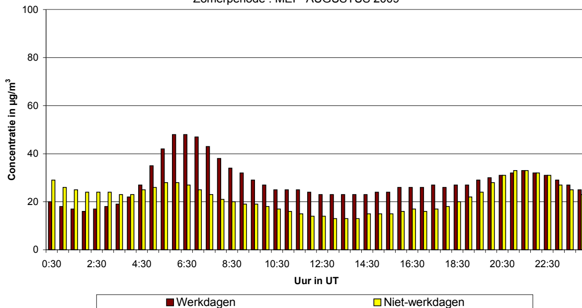
Fig. 51.b : Europees Parlement : Gemiddeld dagverloop van de NO 2 -concentratie op werkdagen en niet-werkdagen tijdens de periode mei - augustus 2009
