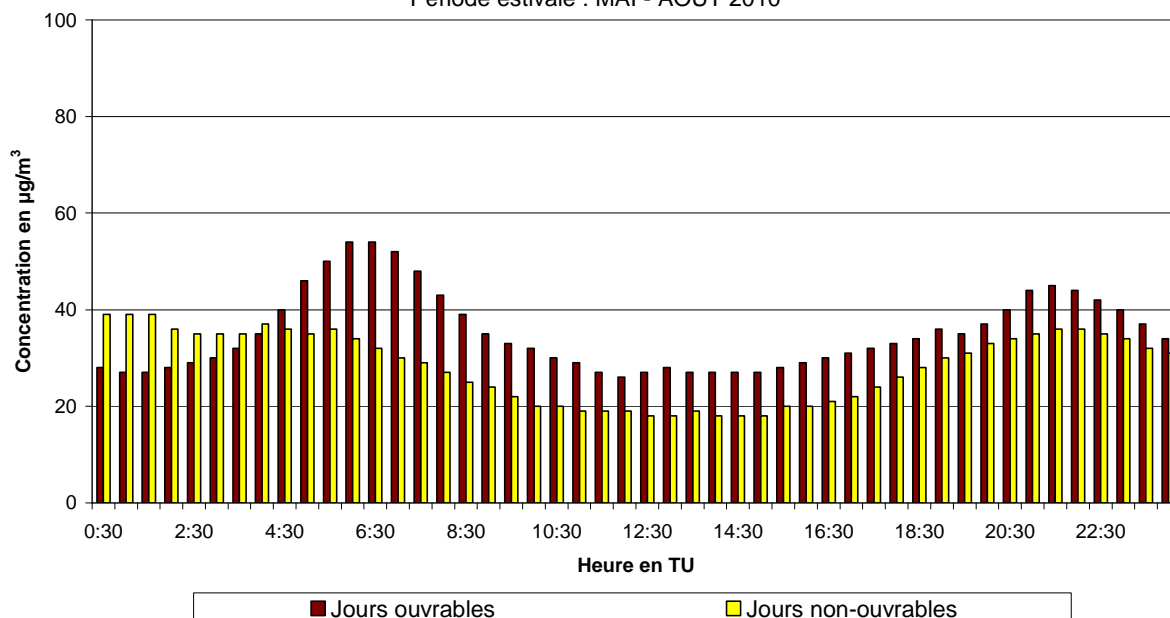
Fig. 52.b : Ste-Catherine : Évolution journalière moyenne de la concentration en NO 2 les jours ouvrables et non-ouvrables pendant la période mai - août 2010
