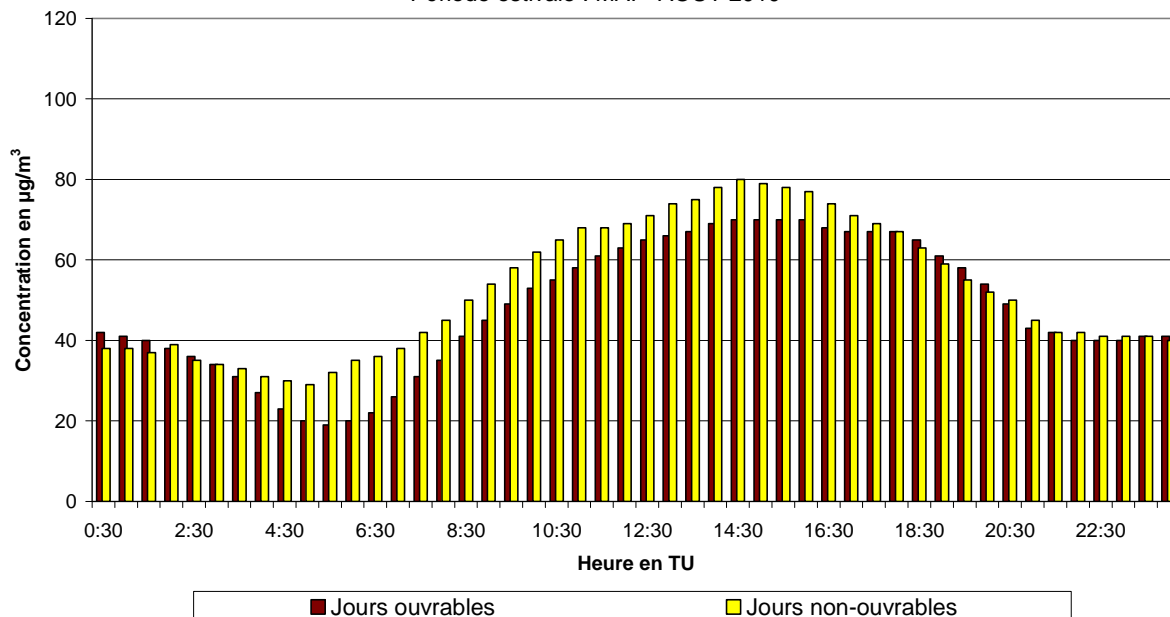
Fig. 48.a : Molenbeek : Évolution journalière moyenne de la concentration en \text{O}_3 les jours ouvrables et non-ouvrables pendant la période mai- août 2010
