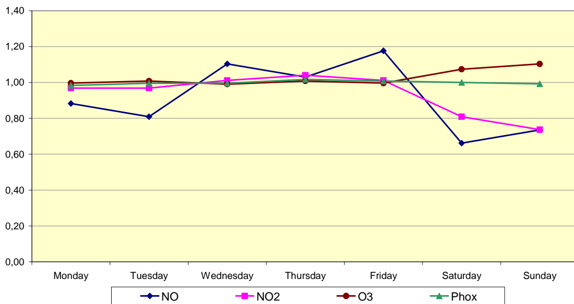
Fig. 59.a : Poste de mesure à Uccle – Profil hebdomadaire moyen des concentrations en NO, NO 2 , O 3 et [NO 2 +O 3 ] sur trois périodes estivales successives : ‘avril – septembre’ 2008, 2009 et 2010
