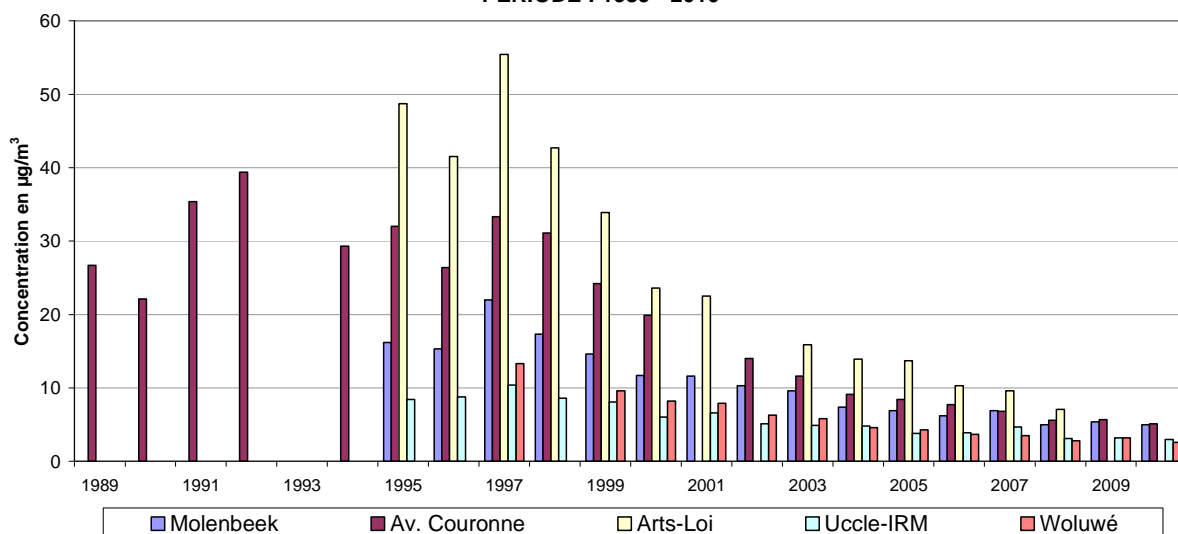
Fig. 29 : Toluène – Évolution de la concentration moyenne annuelle Période : Janvier – Décembre (1989-2009) et 'Janvier – Septembre 2010'
