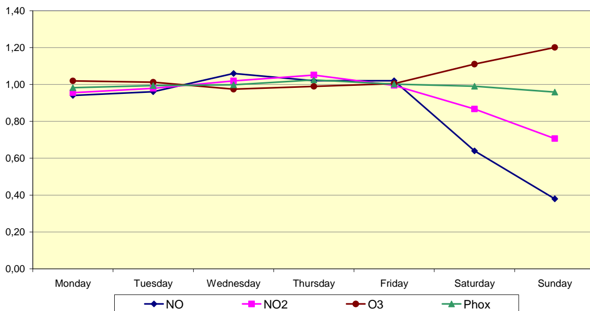
Fig. 59.b : Poste de mesure à Molenbeek – Profil hebdomadaire moyen des concentrations en NO, NO 2 , O 3 et [NO 2 +O 3 ] sur trois périodes estivales successives : ‘avril – septembre’ 2008, 2009 et 2010
