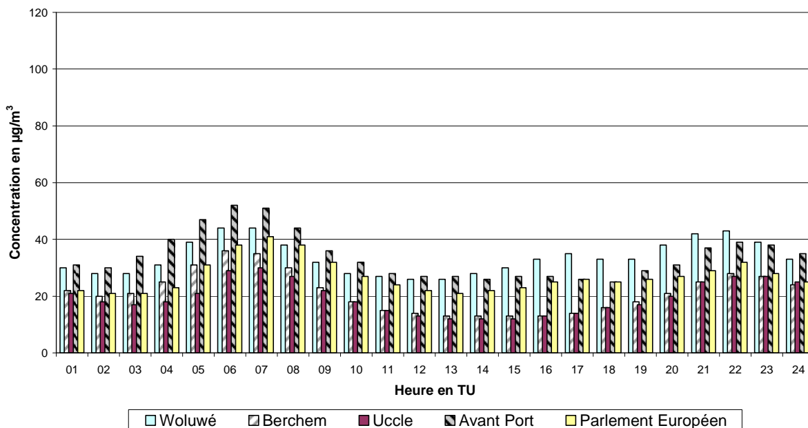
Fig. 9 : Évolution journalière moyenne des concentrations en NO 2 durant la période mai-août 2010
