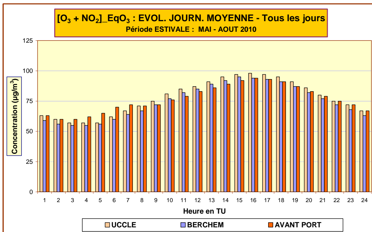
Fig. 67 : [O 3 + NO 2 ] – Évolution journalière moyenne – Comparaison entre 3 postes de mesure Période « mai –août 2010 »
