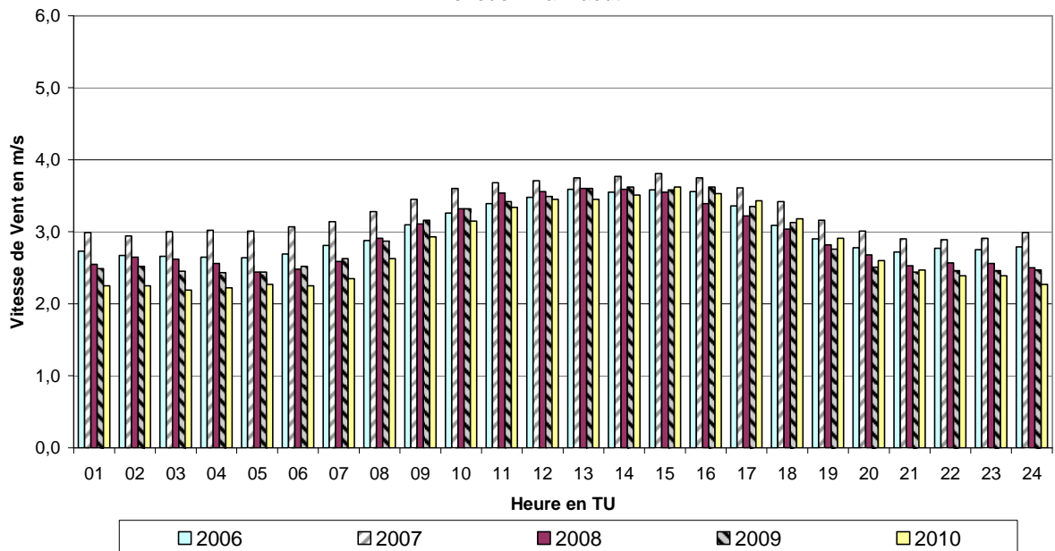
Fig. 38 : Vitesse de vent - évolution journalière moyenne Périodes estivales « mai – août » 2006, 2007, 2008, 2009 et 2010
