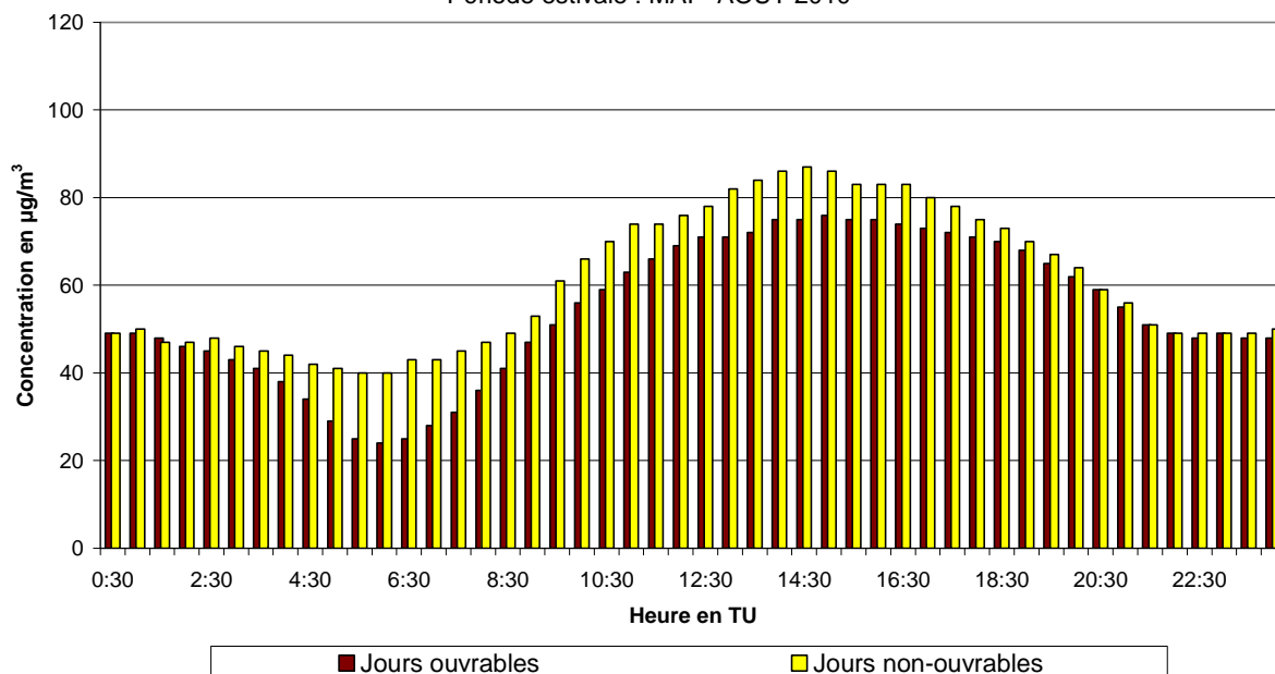
Fig. 51.a : Parlement Européen : Évolution journalière moyenne de la concentration en O 3 les jours ouvrables et non-ouvrables pendant la période mai - août 2010
