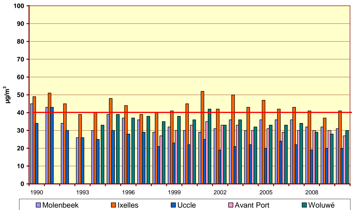
Fig. 27.d : NO 2 – Évolution de la concentration moyenne les 'Dimanches' Périodes annuelles 1990 – 2009 et « Janvier – Septembre 2010 »
