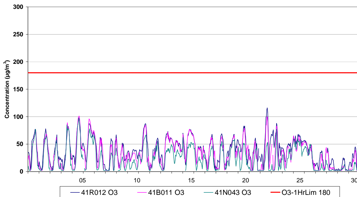
Fig. 7 : Évolution des concentrations horaires en Ozone – Uccle, Berchem et Avant Port – Septembre 2010
