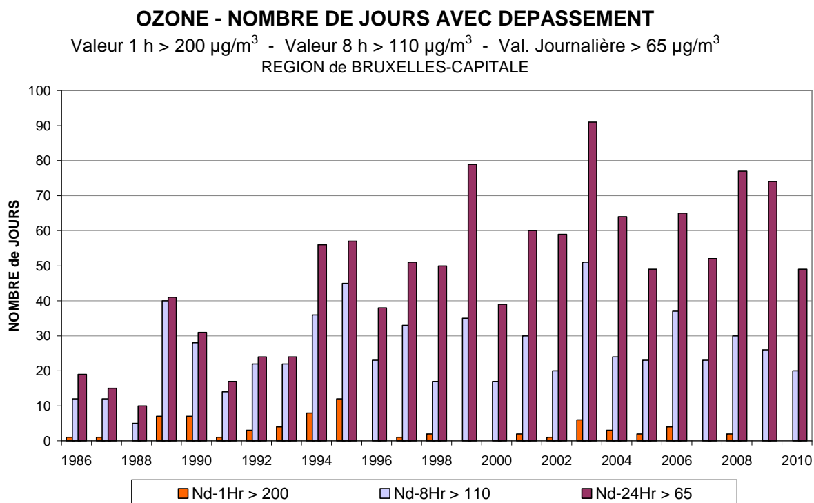
Fig. 25 : Ozone : nombre de jours avec dépassements (directive 92/72/CE) Période : janvier - décembre (1986 à 2009) 2010 : Janvier - Septembre
