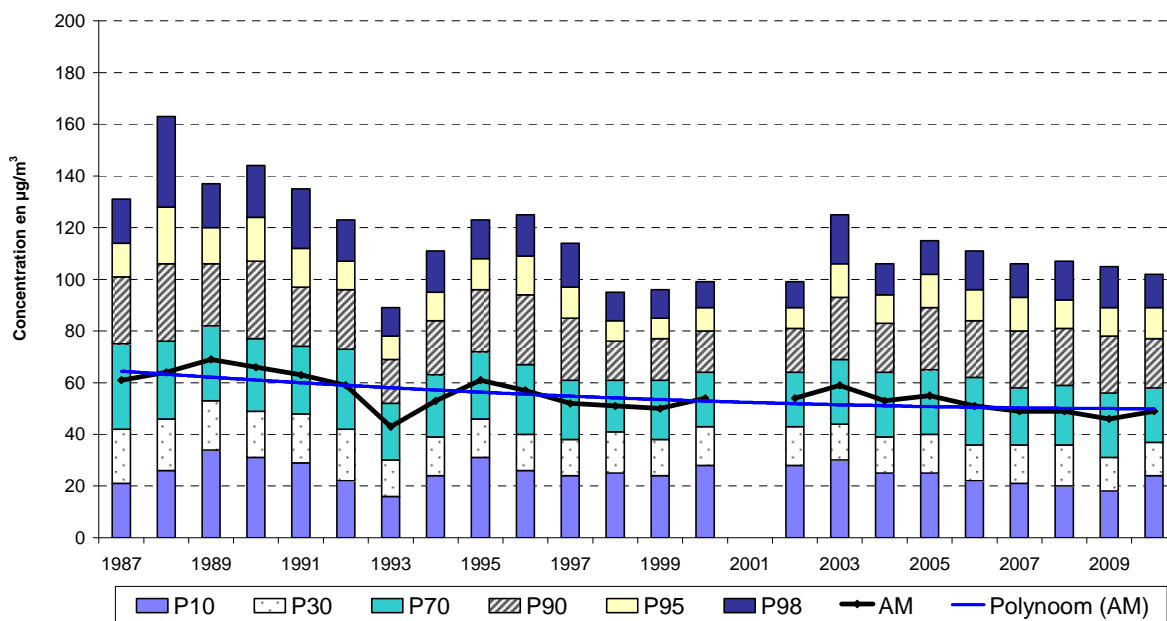
Fig. 40 : Ixelles – Évolution de Valeurs Horaires en NO 2 Période estivale « avril – septembre » (1987-2010)
