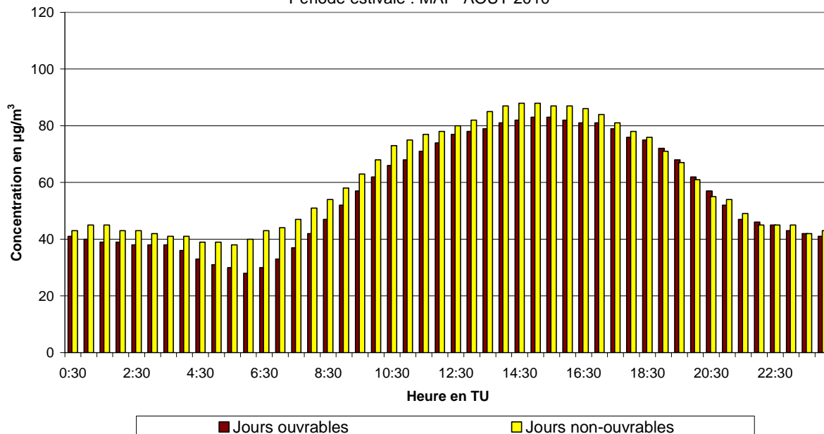
Fig. 46.a : Uccle : Évolution journalière moyenne de la concentration en O 3 les jours ouvrables et non-ouvrables pendant la période mai - août 2010
