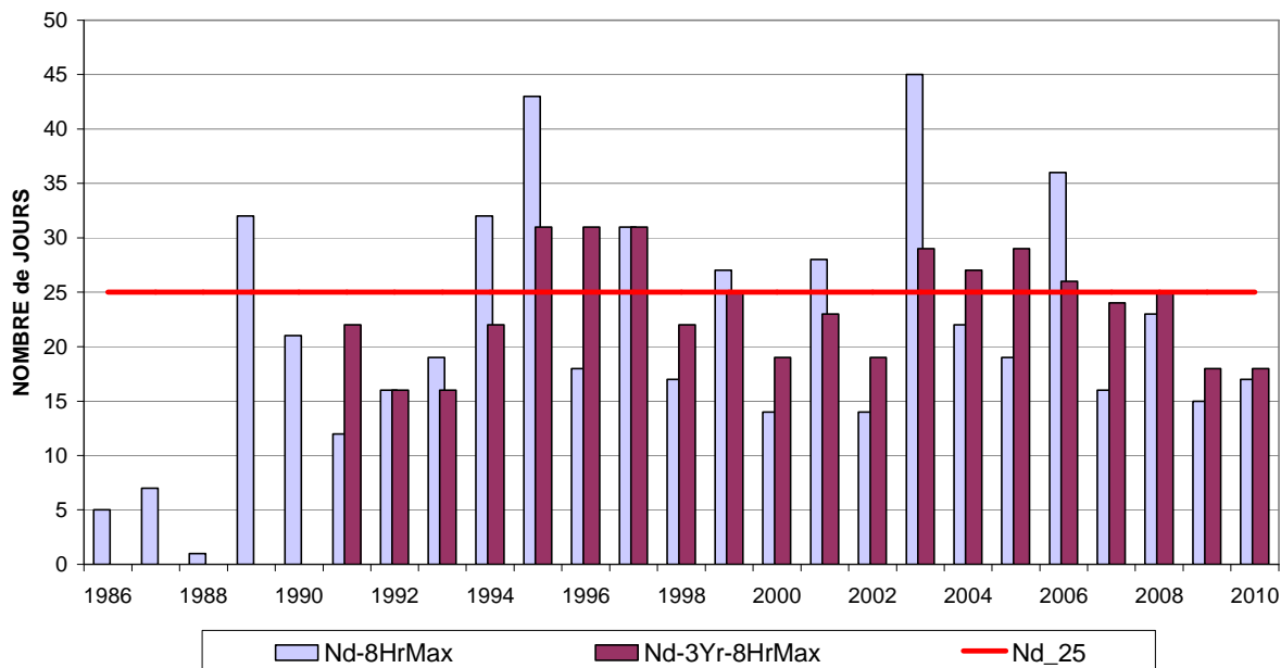
Fig. 14: Ozone – évolution du nombre de jours avec dépassement dans la Région. Valeur cible pour la Santé Publique. Valeur maximale sur 8 heures > 120 µg/m 3 . Période : Janvier – Décembre (1986-2009). [2010] : Janvier - Septembre
