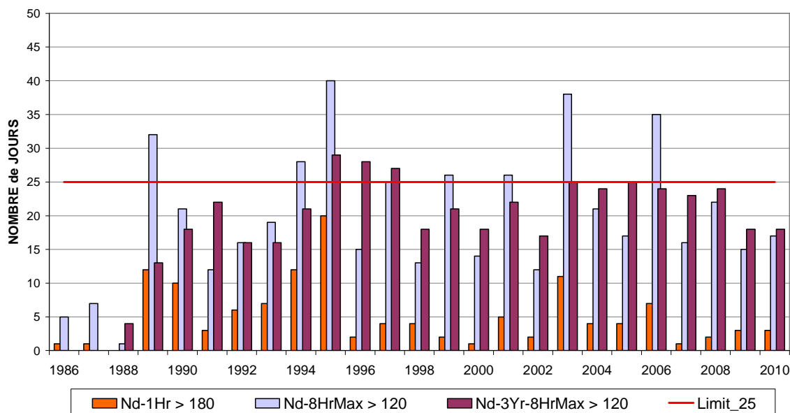
Fig. 19 : Ozone à Uccle : nombre de jours avec dépassements Périodes annuelles : 1 janvier – 31 décembre (1986 – 2009) Données partielles pour l'année 2010 (1 er janvier – 30 septembre)
