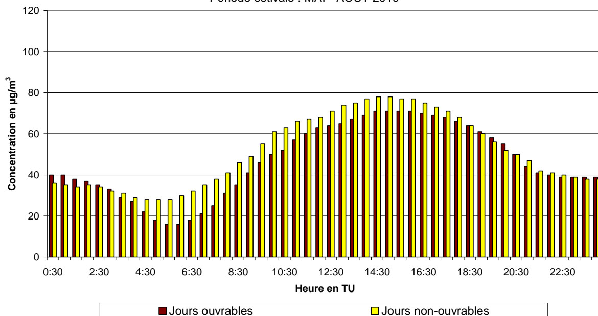
Fig. 52.a : Ste-Catherine : Évolution journalière moyenne de la concentration en O 3 les jours ouvrables et non-ouvrables pendant la période mai - août 2010
