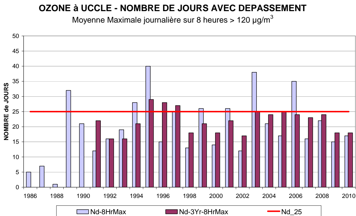
Fig. 12: Ozone – évolution du nombre de jours avec dépassement à Uccle. Valeur cible pour la Santé Publique. Valeur maximale sur 8 heures > 120 µg/m 3 . Période : Janvier – Décembre (1986-2009). [2010] : Janvier - Septembre
