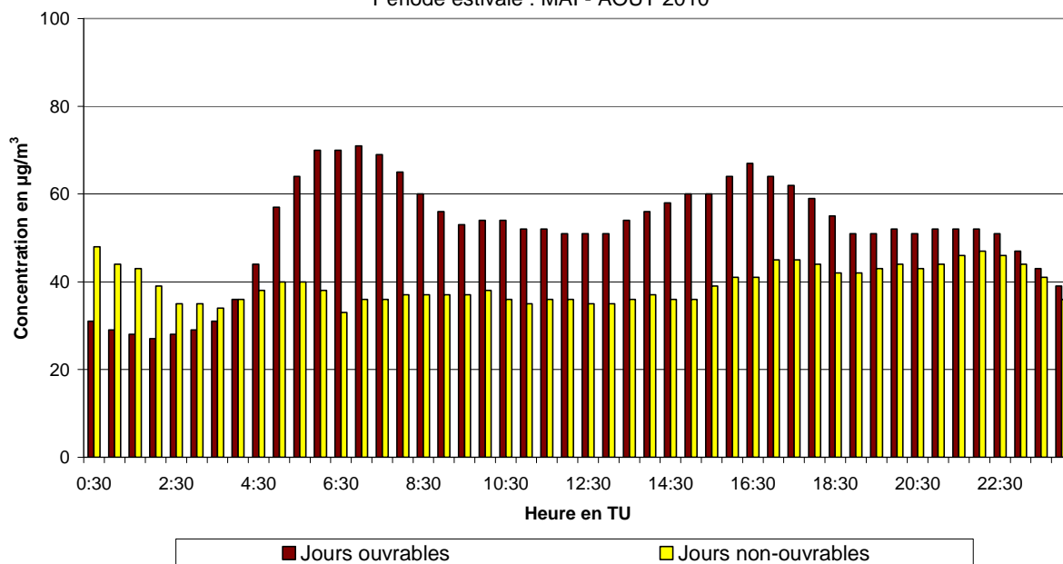
Fig. 54.a : Avenue de la Couronne à Ixelles : Évolution journalière moyenne de la concentration en NO 2 les jours ouvrables et non-ouvrables pendant la période mai - août 2010
