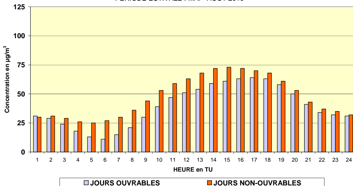
Fig. 68 : Ozone – Évolution journalière moyenne les jours ouvrables et les jours non ouvrables Postes de mesure d’Uccle et de l’Avant Port (trafic) - Période « mai –août 2010 »
