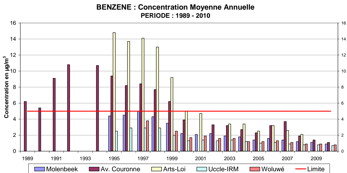
Fig. 28 : Benzène – Évolution de la concentration moyenne annuelle Période : Janvier – Décembre (1989-2009) et 'Janvier – Septembre 2010'
