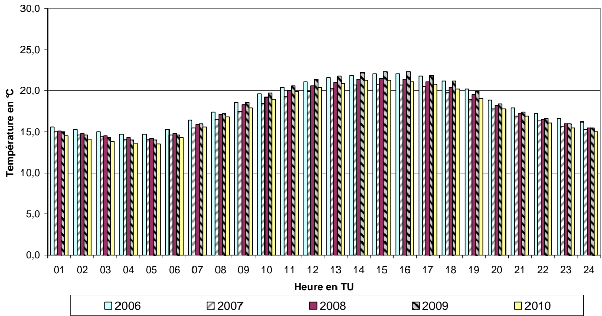
Fig. 37 : Température - évolution journalière moyenne Périodes estivales « mai – août » 2006, 2007, 2008, 2009 et 2010
