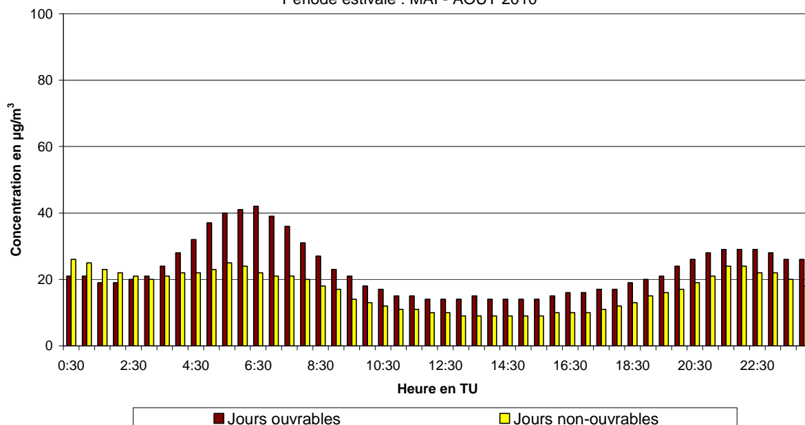
Fig. 47.b : Berchem-Ste-Agathe : Évolution journalière moyenne de la concentration en NO_2 les jours ouvrables et non-ouvrables pendant le période mai – août 2010
