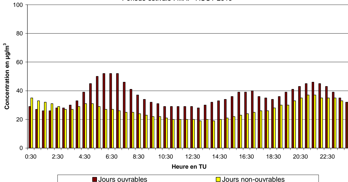
Fig. 50.b : Woluwé-St-Lambert : Évolution journalière moyenne de la concentration en NO 2 les jours ouvrables et non-ouvrables pendant la période mai - août 2010
