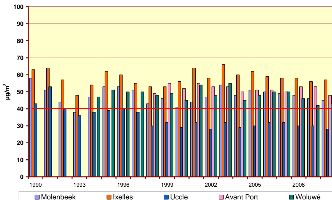
Fig. 27.b : NO 2 – Évolution de la concentration moyenne les ' jours ouvrables ' Périodes annuelles 1990 – 2009 et « Janvier –Septembre 2010 »
