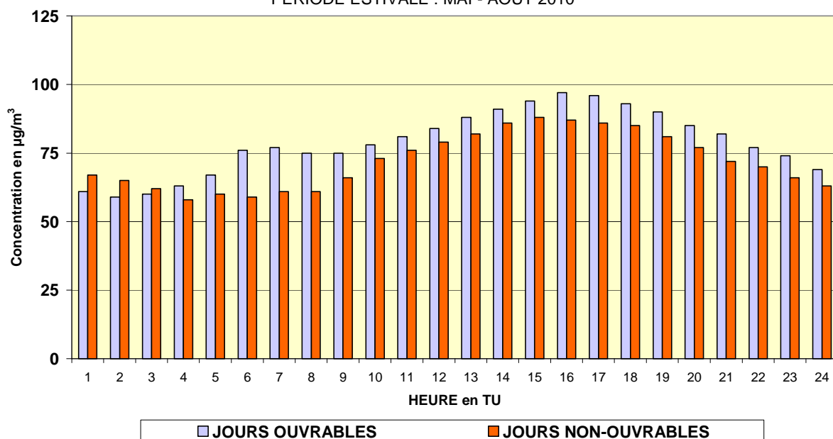
Fig. 69 : [O 3 + NO 2 ] – Évolution journalière moyenne les jours ouvrables et les jours non ouvrables Postes de mesure d'Uccle et de l'Avant Port (trafic) - Période « mai –août 2010 »
