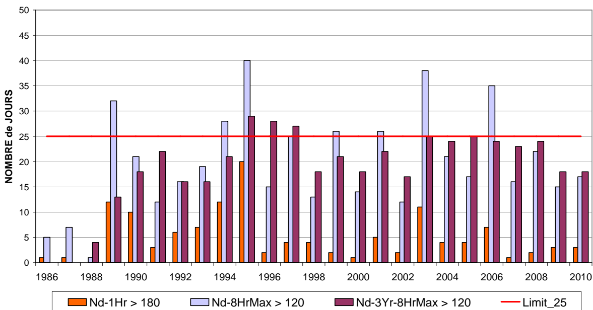
Fig. 62 : Ozone – nombre de jours avec dépassements à Uccle Nombre de jours avec des valeurs horaires supérieures à 180 \mu\text{g}/\text{m}^3 et des valeurs maximales sur 8 heures supérieures à 120 \mu\text{g}/\text{m}^3 (par an et moyenné sur 3 ans)
