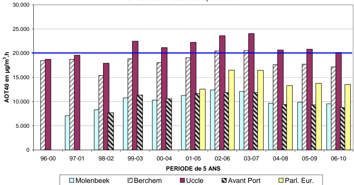
Fig. 16 : Évolution AOT40-AS dans le temps (1996-2010) AOT40 pour la période Avril – Septembre, 8-20 h d'Europe centrale Résultats par an et moyenné sur 5 ans
