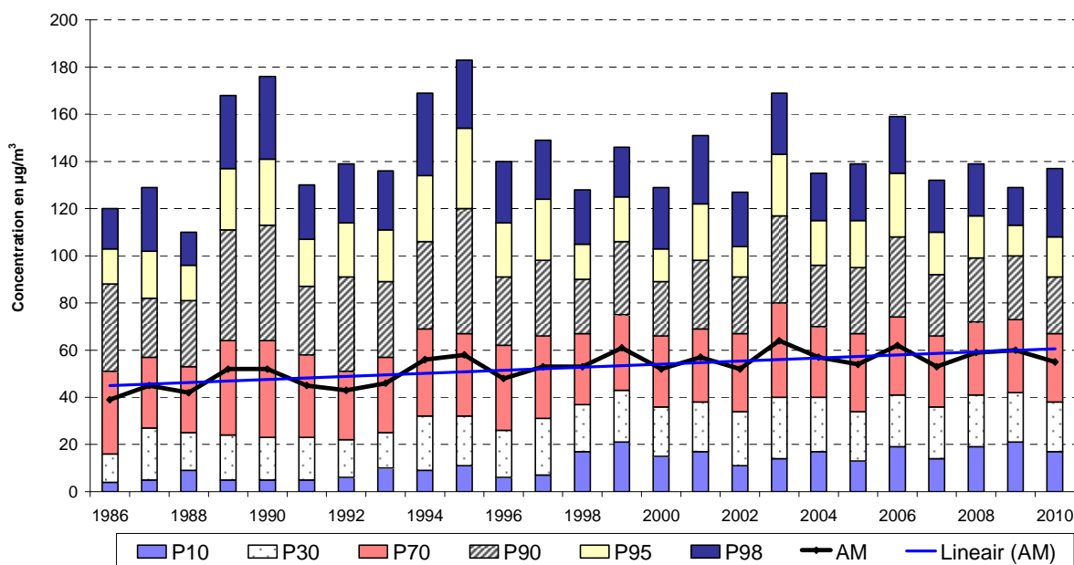
Fig. 33 : Uccle - Évolution des Valeurs Horaires en Ozone (1986-2010) Période estivale « avril – septembre »
