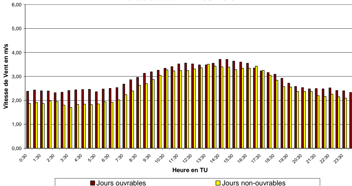
Fig. 55.b : Uccle : Évolution journalière moyenne de la vitesse de vent les jours ouvrables et non-ouvrables pendant la période mai – août 2010
