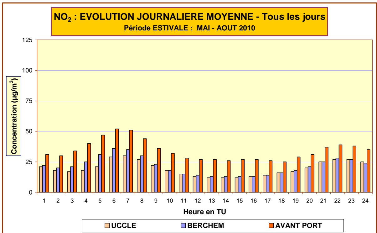
Fig. 66 : NO 2 – Évolution journalière moyenne – Comparaison entre 3 postes de mesure Période « mai –août 2010 »
