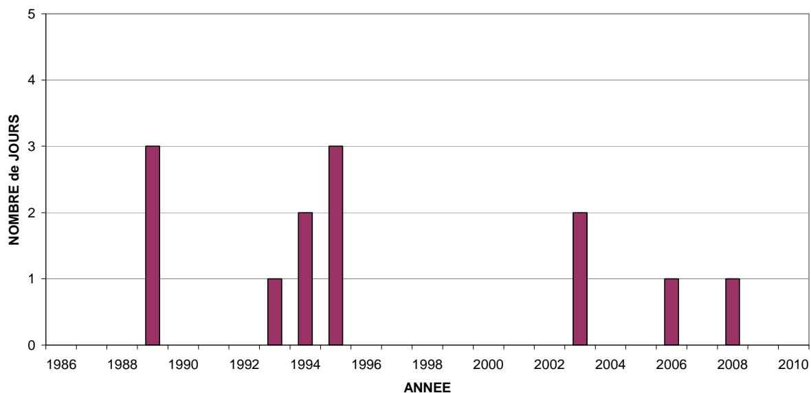
Fig. 18 : Ozone – Évolution du nombre de jours avec dépassement en Région de Bruxelles-Capitale
