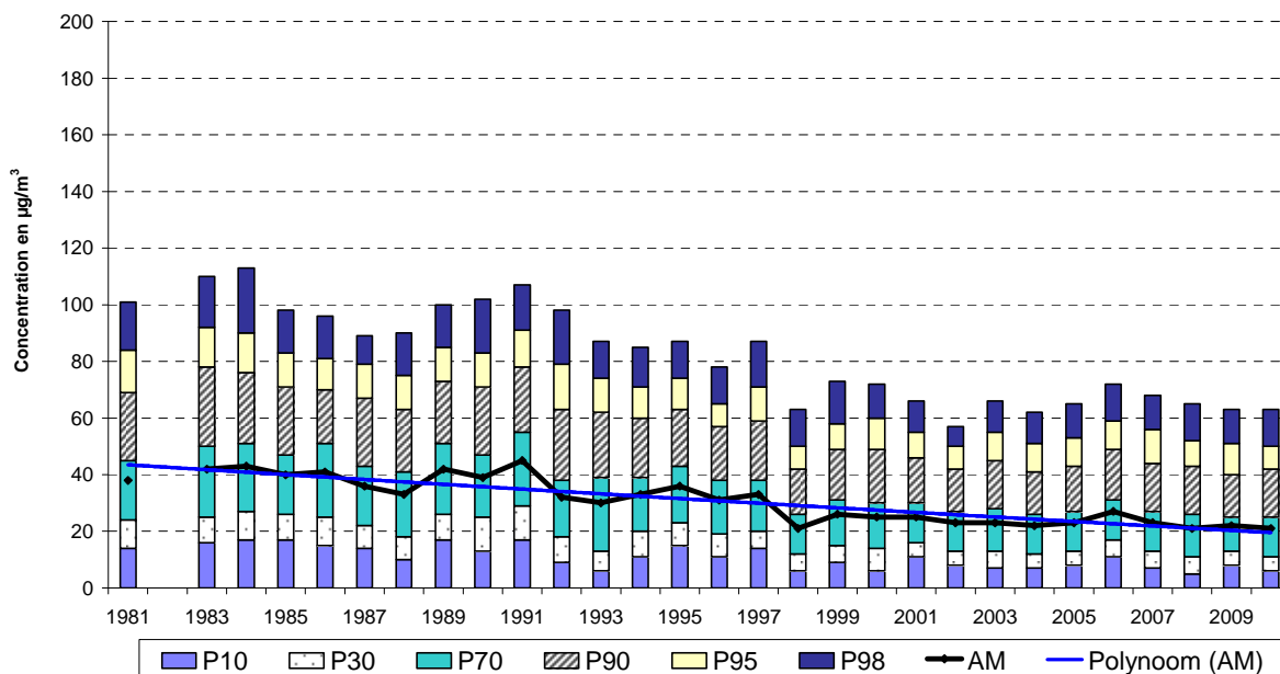
Fig. 41 : Arts-Loi – Évolution de Valeurs Horaires en NO 2 Période estivale « avril – septembre » (1981-2010)
