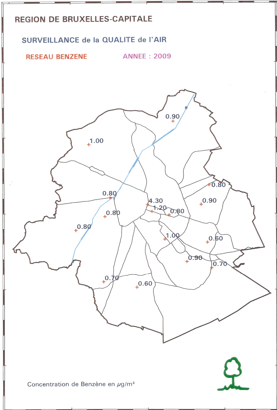
Fig. 31 : Benzène – Distribution spatiale de concentration moyenne annuelle en 2009
