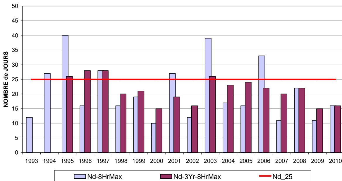
Fig. 13: Ozone – évolution du nombre de jours avec dépassement à Berchem. Valeur cible pour la Santé Publique. Valeur maximale sur 8 heures > 120 µg/m 3 . Période : Janvier – Décembre (1993-2009). [2010] : Janvier - Septembre
