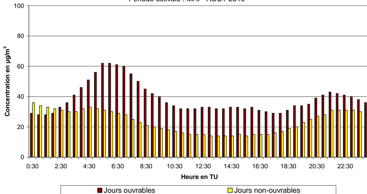
Fig. 49.b : Avant Port : Évolution journalière moyenne de la concentration en NO 2 les jours ouvrables et non-ouvrables pendant la période mai – août 2010
