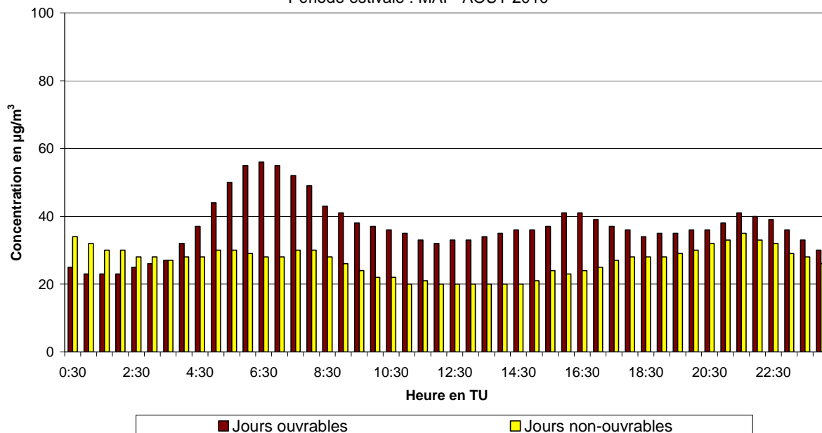
Fig. 53.a : Eastman-Belliard : Évolution journalière moyenne de la concentration en NO 2 les jours ouvrables et non-ouvrables pendant la période mai - août 2010
