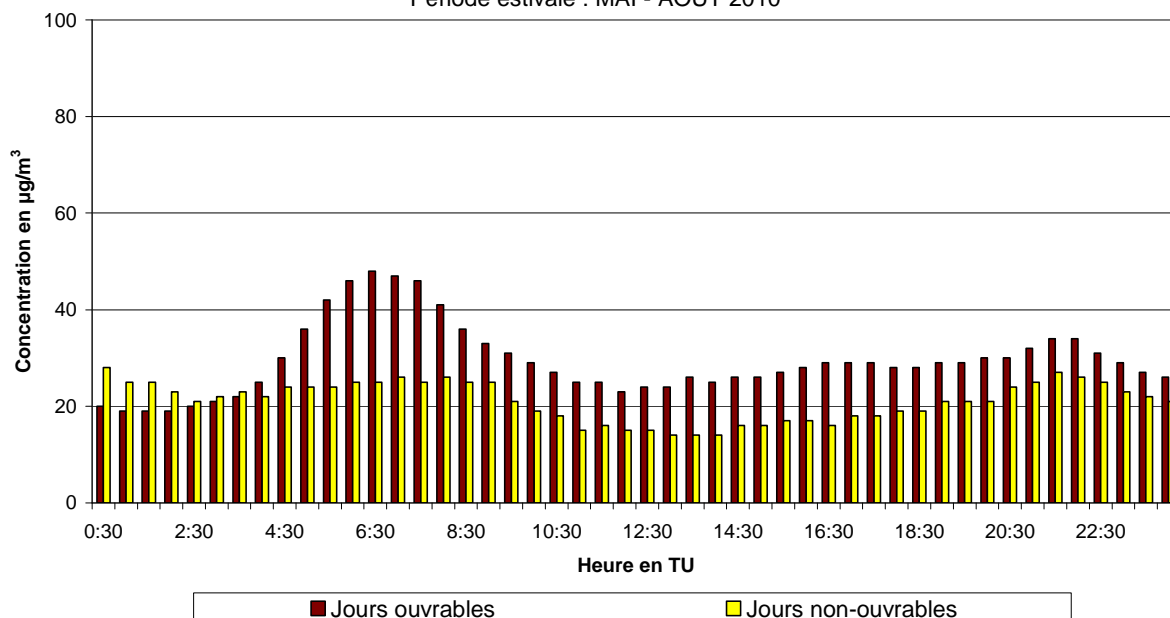
Fig. 51.b : Parlement Européen : Évolution journalière moyenne de la concentration en NO 2 les jours ouvrables et non-ouvrables pendant la période mai – août 2010
