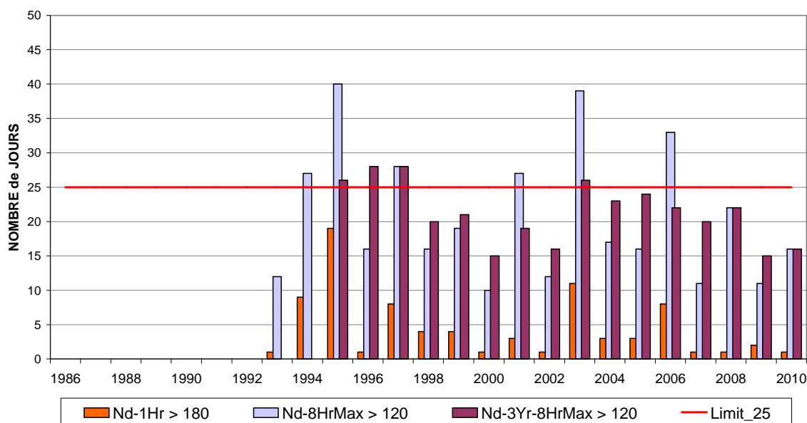
Fig. 20 : Ozone à Berchem : nombre de jours avec dépassements Périodes annuelles : 1 janvier – 31 décembre (1986 – 2009) Données partielles pour l'année 2010 (1 er janvier – 30 septembre)
