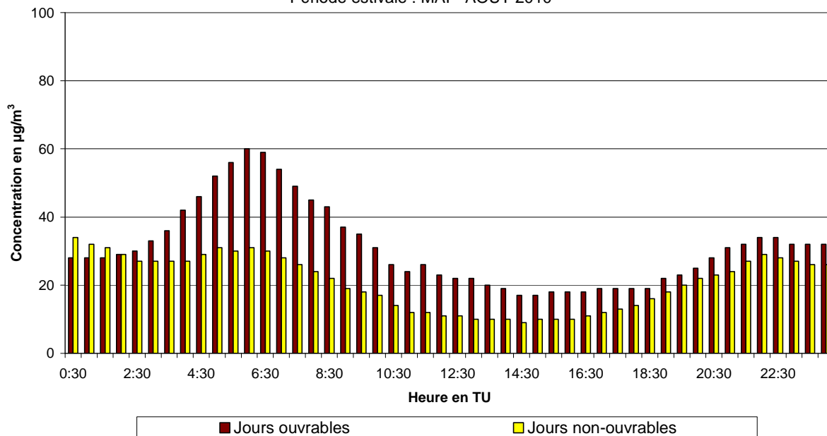
Fig. 53.b : Parc Meudon : Évolution journalière moyenne de la concentration en NO 2 les jours ouvrables et non-ouvrables pendant la période mai – août 2010
