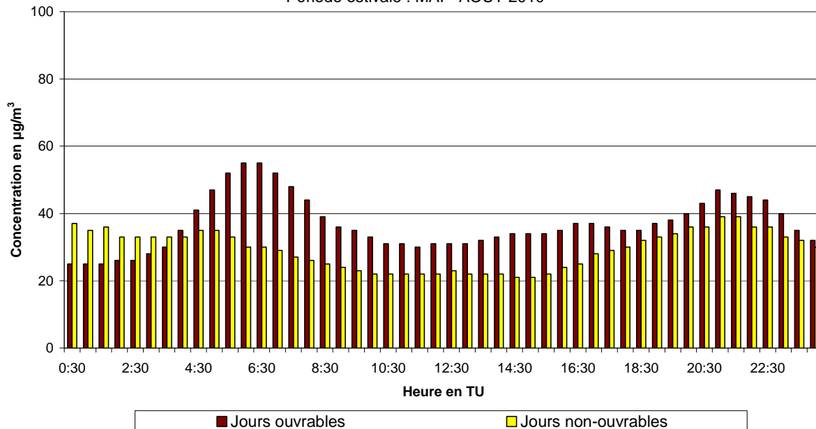
Fig. 48.b : Molenbeek : Évolution journalière moyenne de la concentration en \text{NO}_2 les jours ouvrables et non-ouvrables pendant la période mai – août 2010
