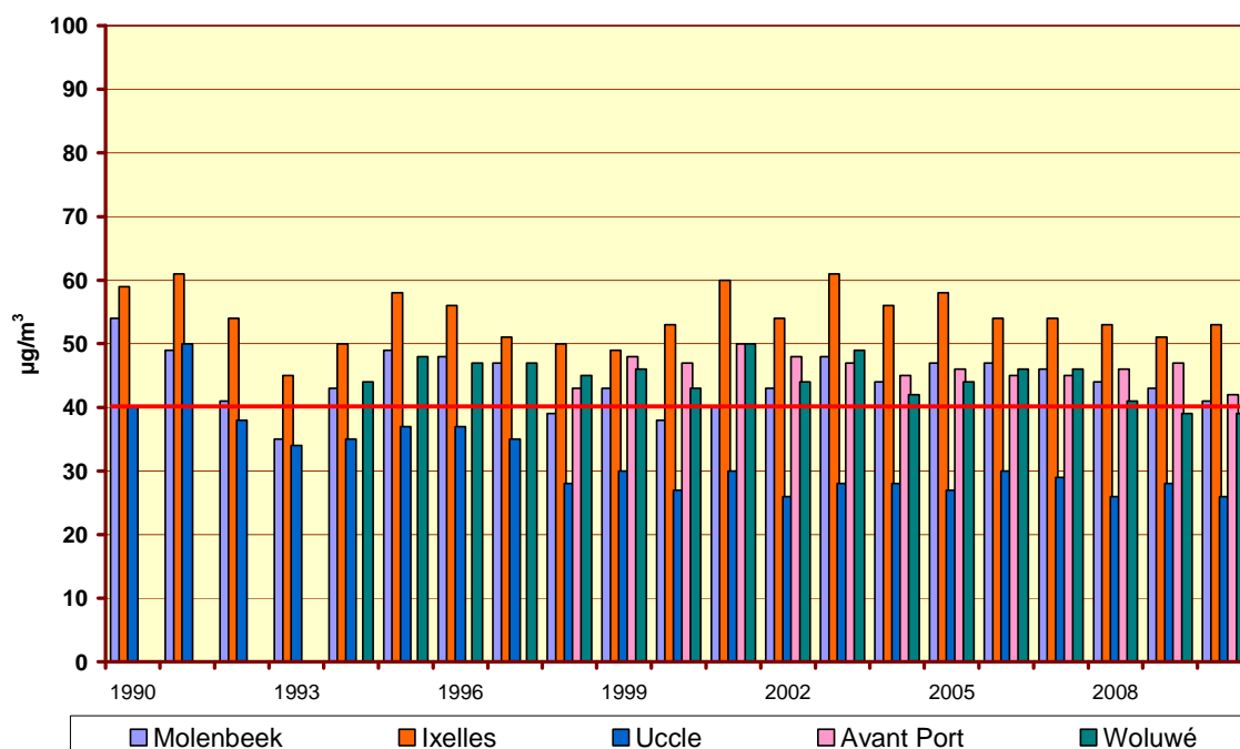
Fig. 27.a : NO 2 – Évolution de la concentration moyenne annuelle ( tous les jours ) Périodes annuelles 1990 – 2009 et « Janvier –Septembre 2010 »
