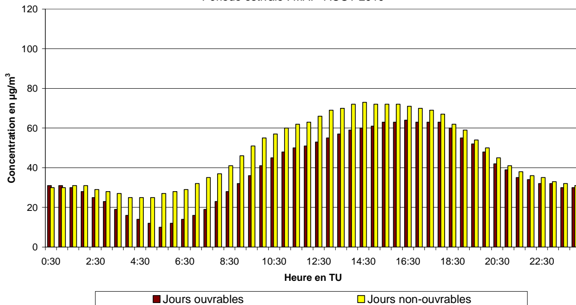
Fig. 49.a : Avant Port : Évolution journalière moyenne de la concentration en O 3 les jours ouvrables et non-ouvrables pendant la période mai - août 2010
