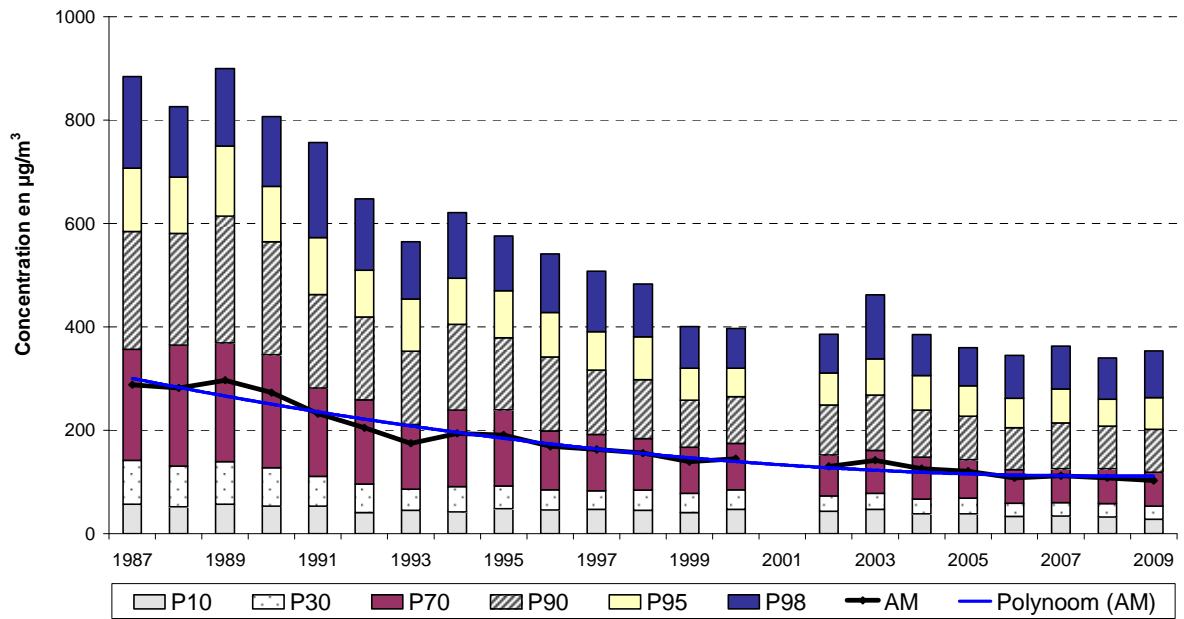
Fig. 72 : NO x à Ixelles – Avenue de la Couronne ( canyon street ) – Valeurs horaires Évolution à long terme - Périodes annuelles 1987 - 2009
