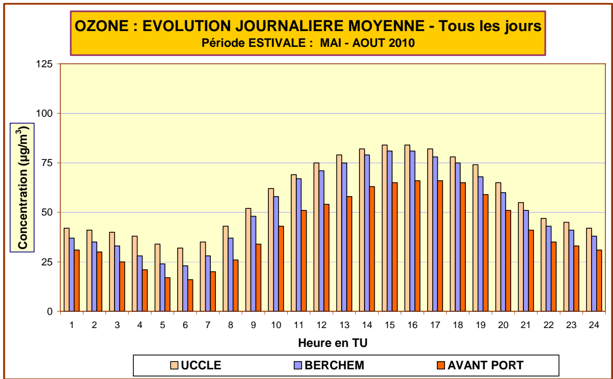
Fig. 65 : Ozone – Évolution journalière moyenne – Comparaison entre 3 postes de mesure Période « mai –août 2010 »
