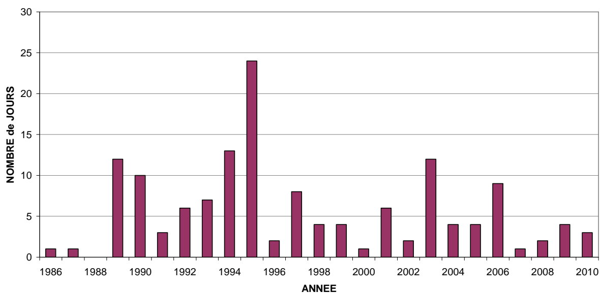
Fig. 17 : Ozone – Évolution du nombre de jours avec dépassement en Région de Bruxelles-Capitale
