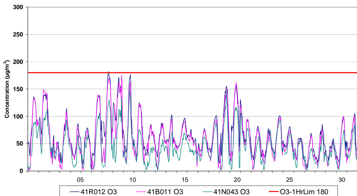
Fig. 5 : Évolution des concentrations horaires en Ozone – Uccle, Berchem et Avant Port – Juillet 2010
