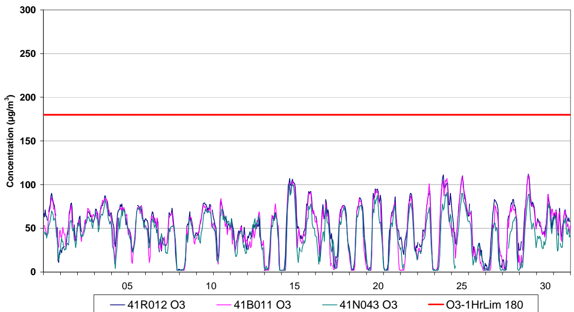
Fig. 3 : Évolution des concentrations horaires en Ozone – Uccle, Berchem et Avant Port – Mai 2010
