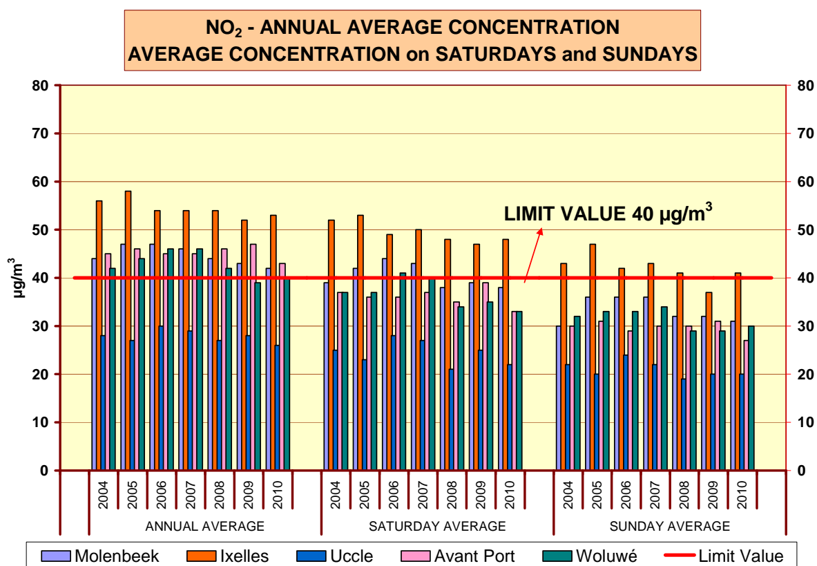
Fig. 26 : NO 2 – Comparaison entre la concentration moyenne annuelle et la concentration moyenne des 'Samedis' et des 'Dimanches' pour une sélection de postes de mesure. Périodes annuelles 2004-2009 et "Janvier – Septembre 2010"
