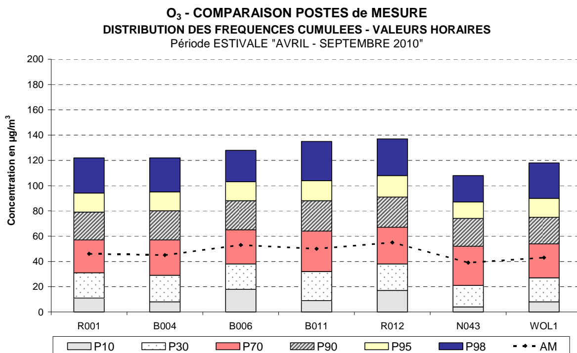
Fig. 32 : Ozone - Distribution de fréquences cumulées - valeurs horaires: avril - septembre 2010
