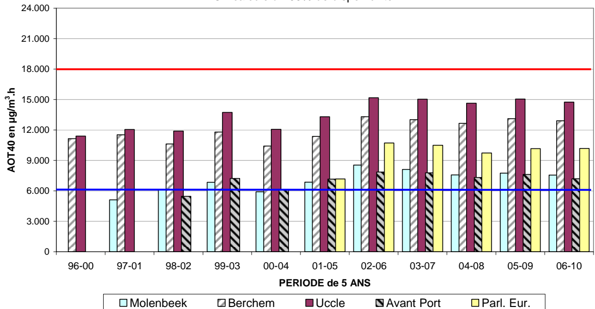
Fig. 15 : Évolution AOT40-MJ dans le temps (1996-2010) AOT40 pour la période Mai – Juillet, 8-20 h d'Europe centrale Résultats par an et moyenné sur 5 ans
