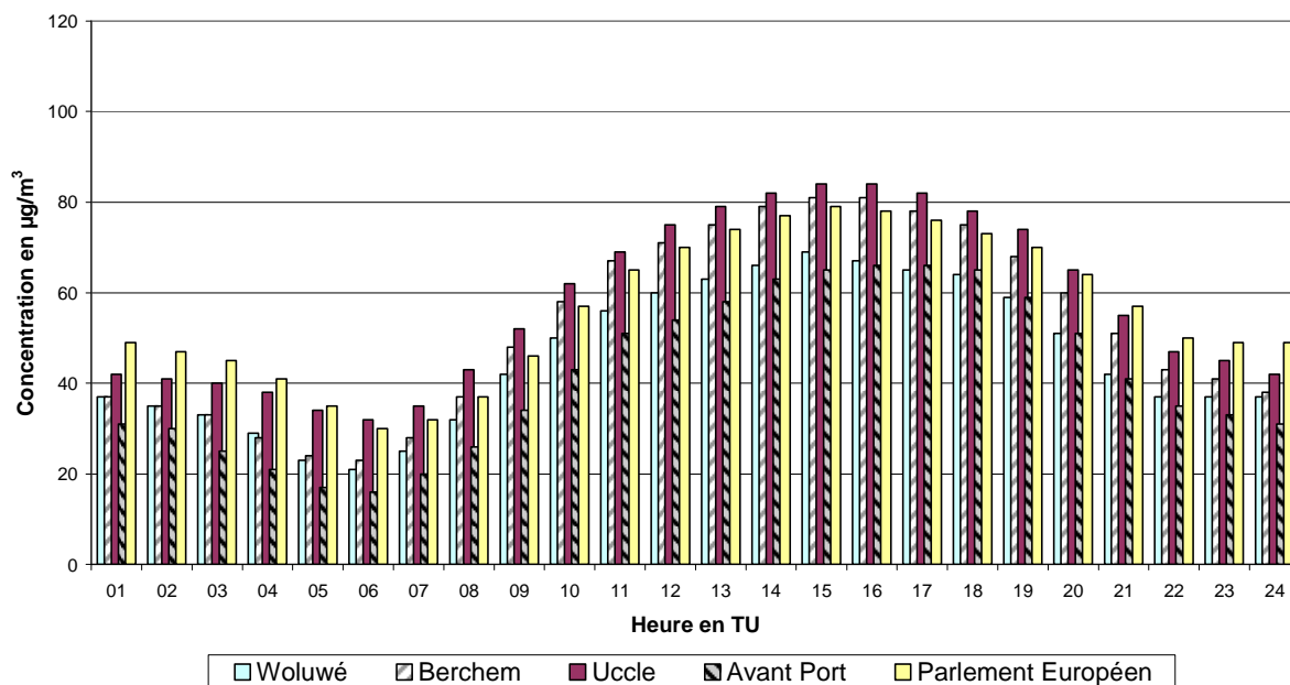
Fig. 8 : Évolution journalière moyenne des concentrations en O 3 durant la période mai-août 2010
