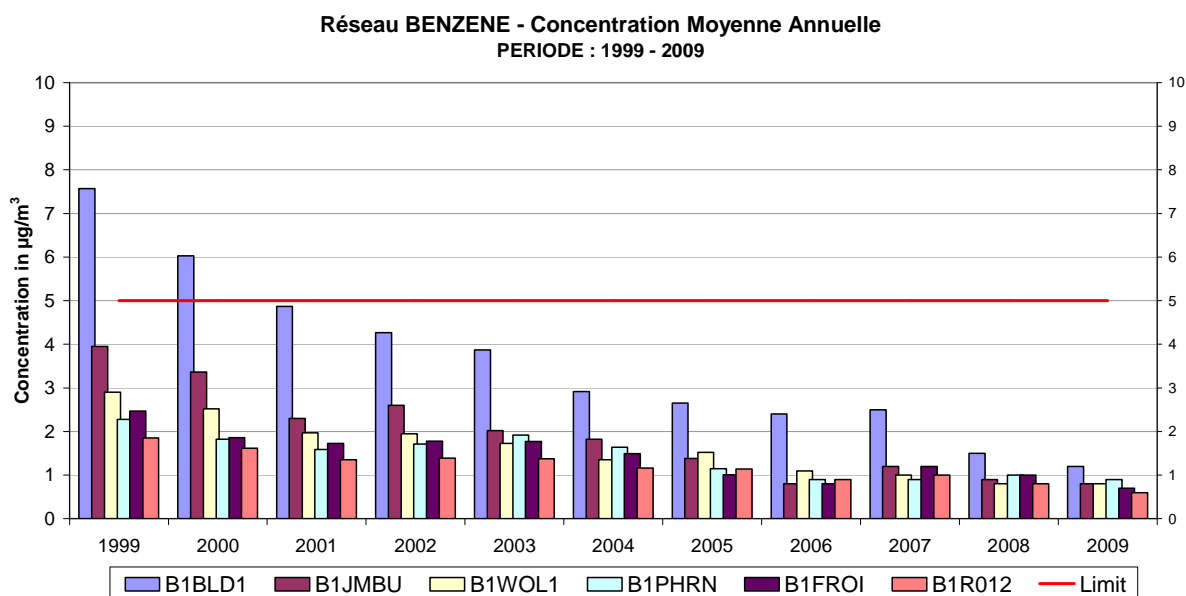
Fig. 30 : Réseau Benzène – Évolution de la concentration moyenne annuelle dans quelques postes de mesure. Période 1999 - 2009
