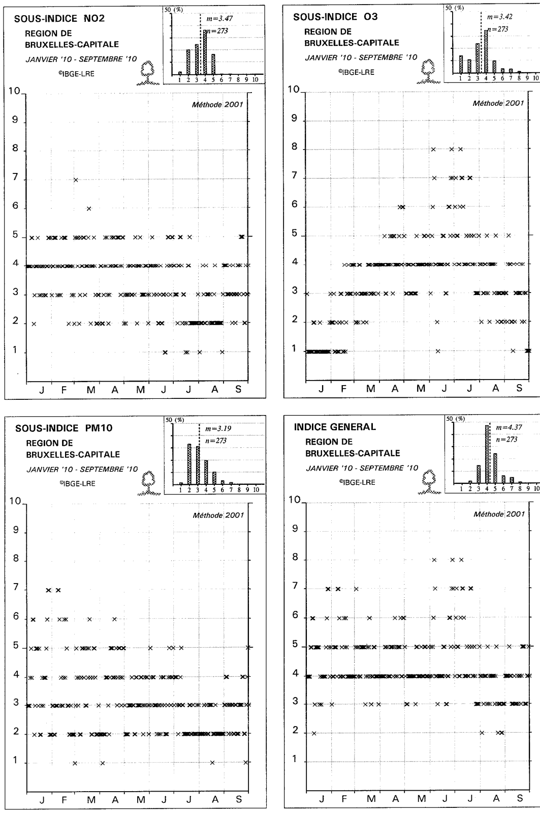
Fig. 60 : Les sous-indices pour NO 2 , O 3 et PM 10 - Indice général Janvier – Septembre 2010
