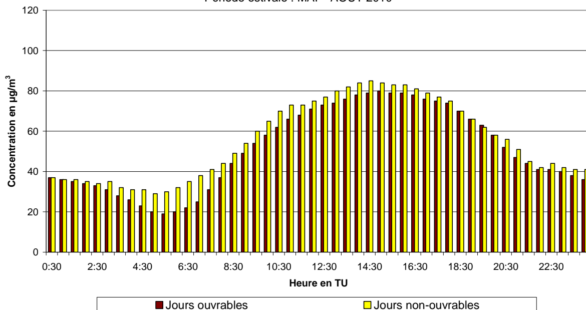
Fig. 47.a : Berchem-Ste-Agathe : Évolution journalière moyenne de la concentration en O_3 les jours ouvrables et non-ouvrables pendant la période mai - août 2010
