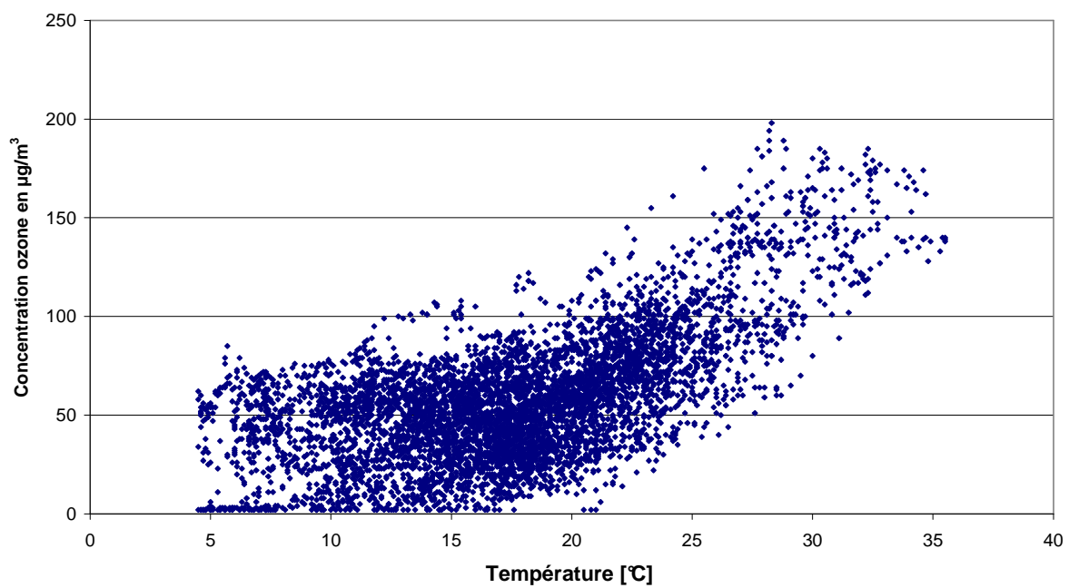
Fig. 42 : Uccle : Concentrations en ozone en fonction de la température (mai - août 2010)
