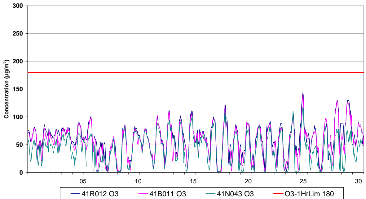
Fig. 2 : Évolution des concentrations horaires en Ozone – Uccle, Berchem et Avant Port – Avril 2010
