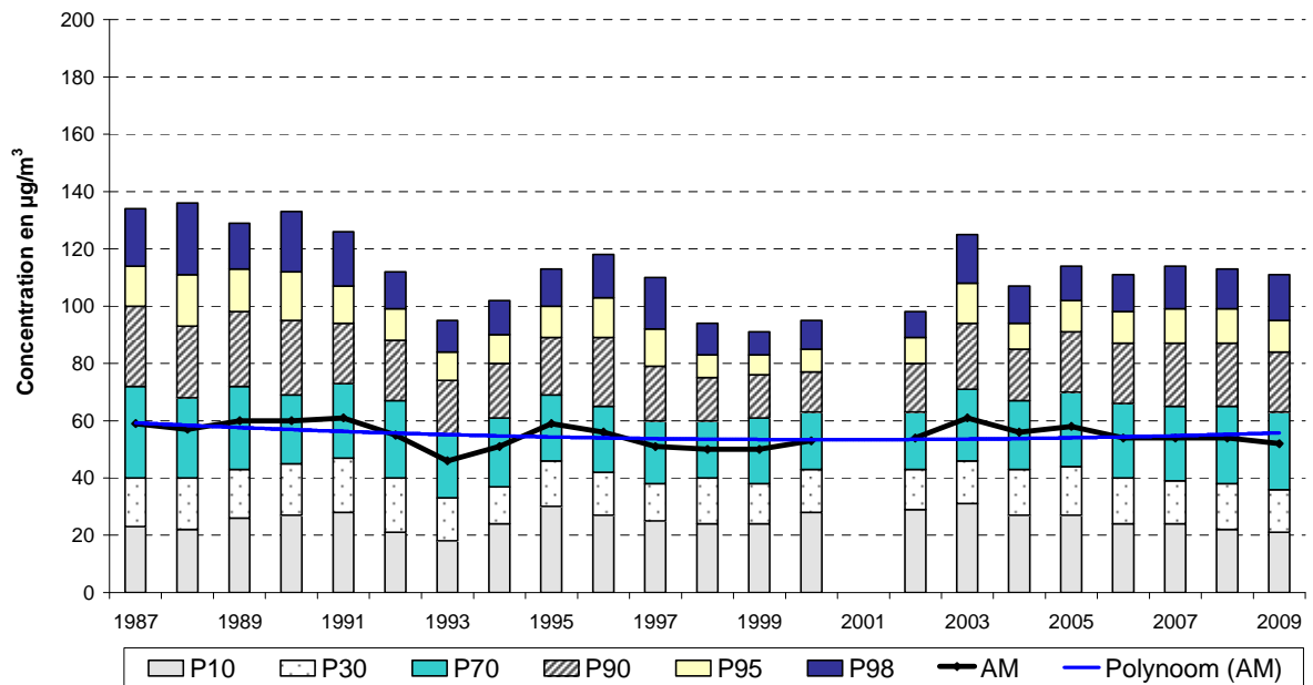
Fig. 73 : NO x à Ixelles – Avenue de la Couronne ( canyon street ) – Valeurs horaires Évolution à long terme - Périodes annuelles 1987 - 2009
