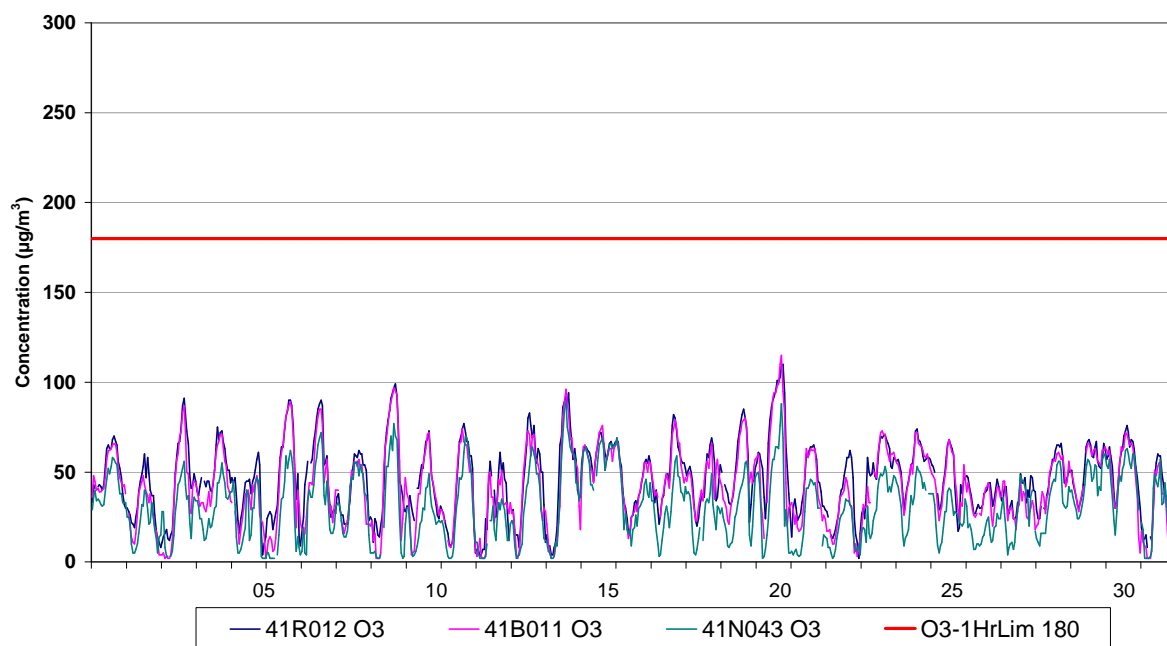
Fig. 6 : Évolution des concentrations horaires en Ozone – Uccle, Berchem et Avant Port – Août 2010
