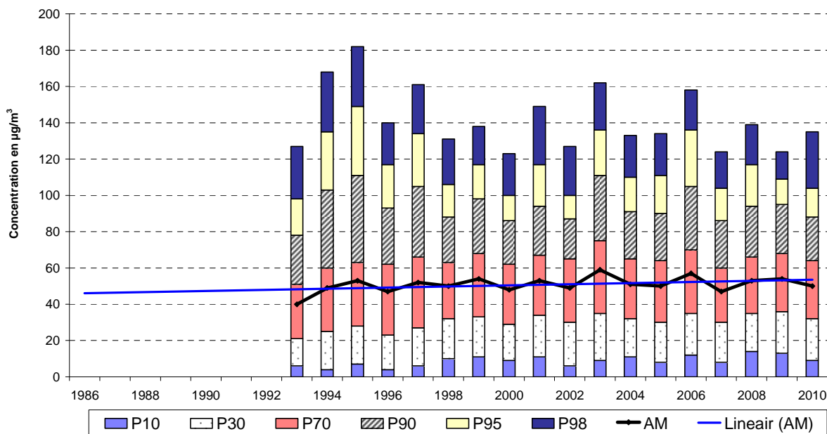
Fig. 34 : Berchem-Ste-Agathe - Évolution des Valeurs Horaires en Ozone (1993-2010) Période estivale « avril – septembre »
