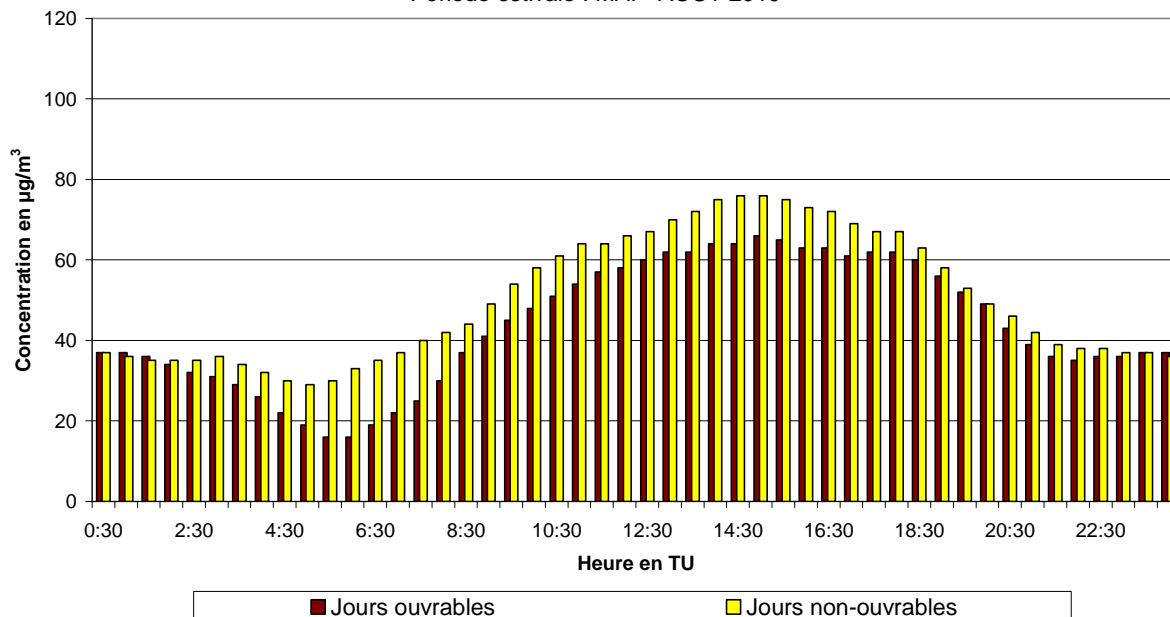
Fig. 50.a : Woluwé-St-Lambert : Évolution journalière moyenne de la concentration en O 3 les jours ouvrables et non-ouvrables pendant la période mai - août 2010
