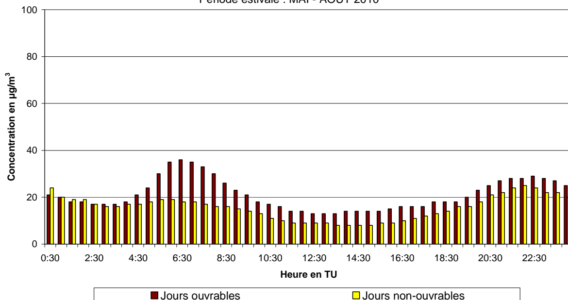
Fig. 46.b : Uccle : Évolution journalière moyenne de la concentration en NO 2 les jours ouvrables et non-ouvrables pendant la période mai - août 2010
