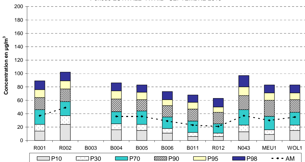
Fig.39 : NO 2 - Distribution de fréquences cumulées - valeurs horaires: avril - septembre 2010
