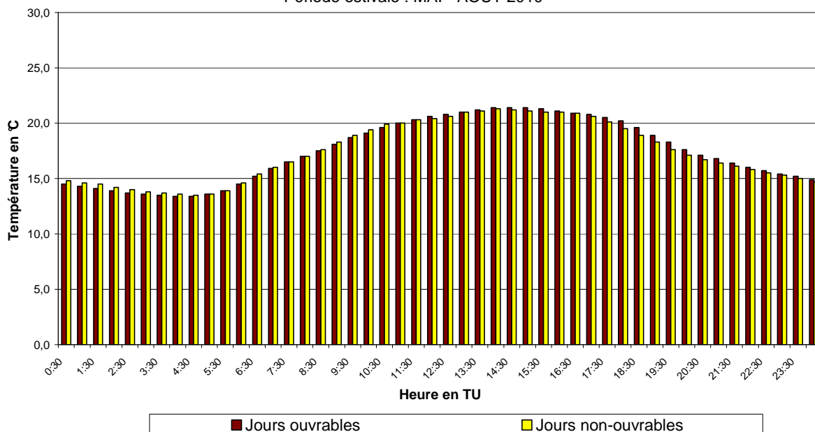
Fig. 55.a : Uccle : Évolution journalière moyenne de la température les jours ouvrables et non-ouvrables pendant la période mai – août 2010
