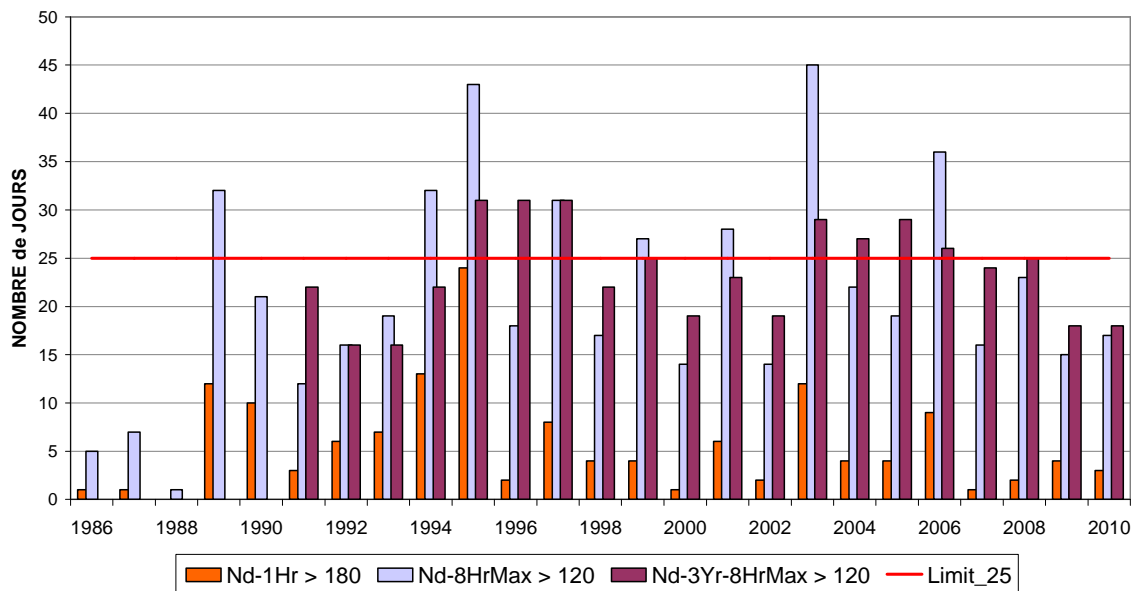
Fig. 21 : Ozone : nombre de jours avec dépassements en Région de Bruxelles-Capitale Périodes annuelles : 1 janvier – 31 décembre (1986 – 2009) Données partielles pour l'année 2010 (1 er janvier – 30 septembre)
