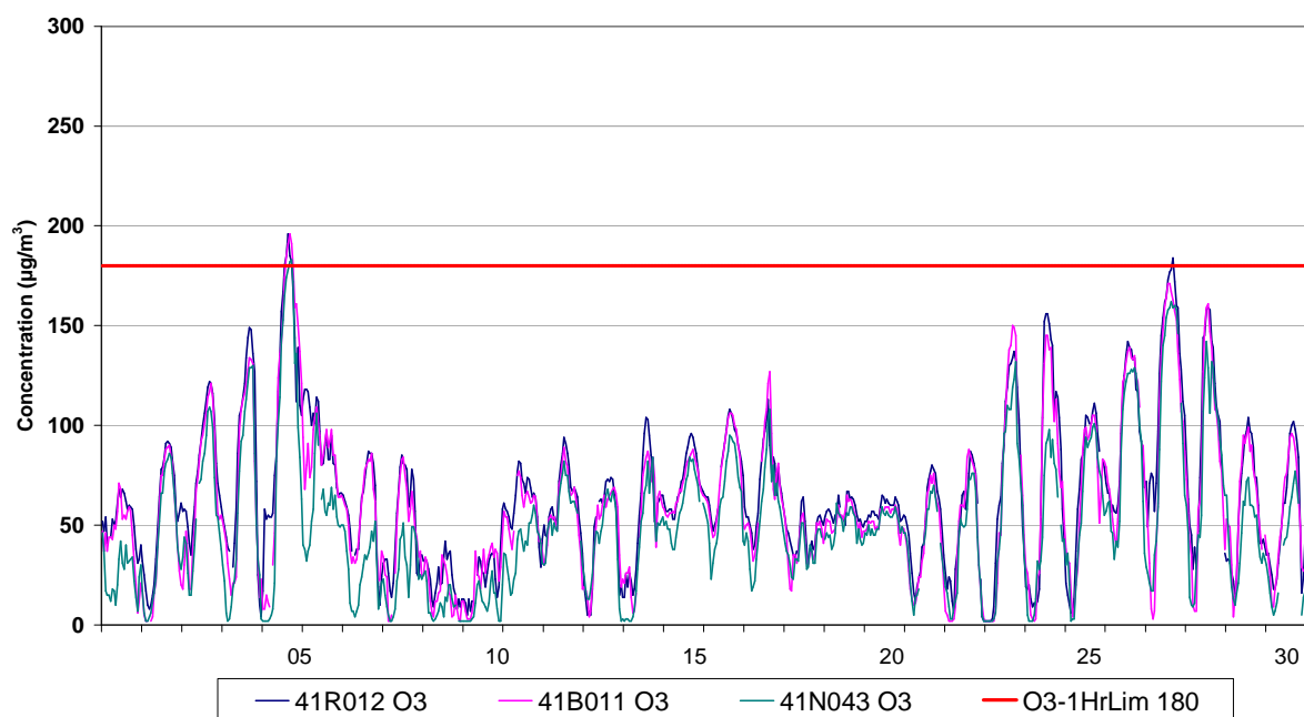
Fig. 4 : Évolution des concentrations horaires en Ozone – Uccle, Berchem et Avant Port – Juin 2010
