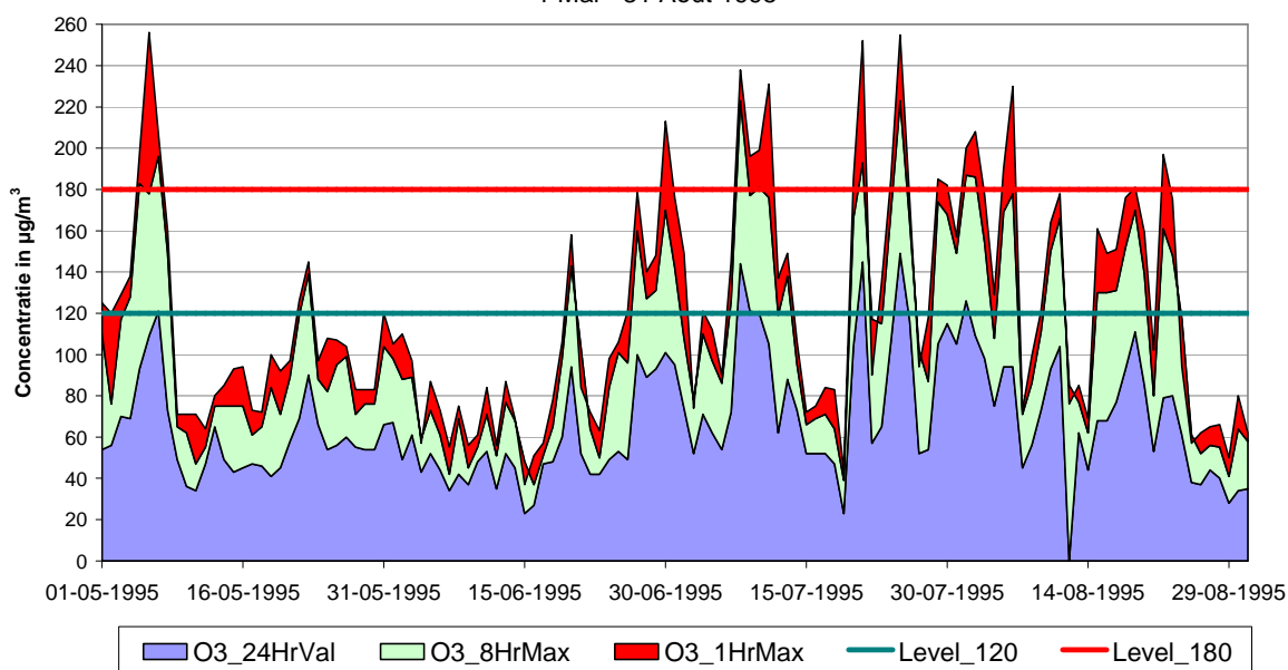
Fig. 23 : Ozone à Uccle – Évolution Valeur Journalière (24HrVal), valeur maximale sur 8 heures (8HrMax) et valeur maximale horaire (1HrMax). Comparaison des périodes estivales de 2003 et 1995.
