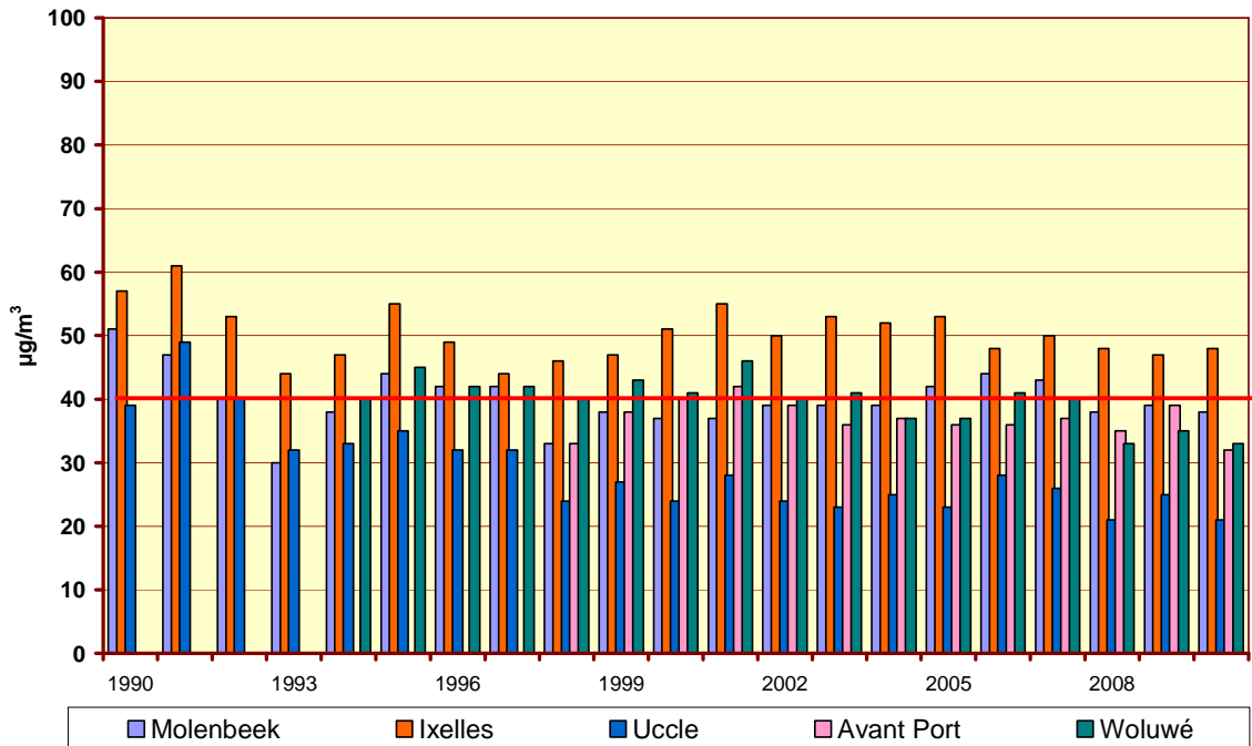
Fig. 27.c : NO 2 – Évolution de la concentration moyenne les 'Samedis' Périodes annuelles 1990 – 2009 et « Janvier – Septembre 2010 »
