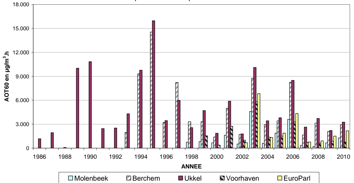
Fig. 24: Évolution AOT60 dans le temps (1986-2010) Période: JANVIER - DÉCEMBRE (1986-2009) 2010 : Janvier - Septembre
