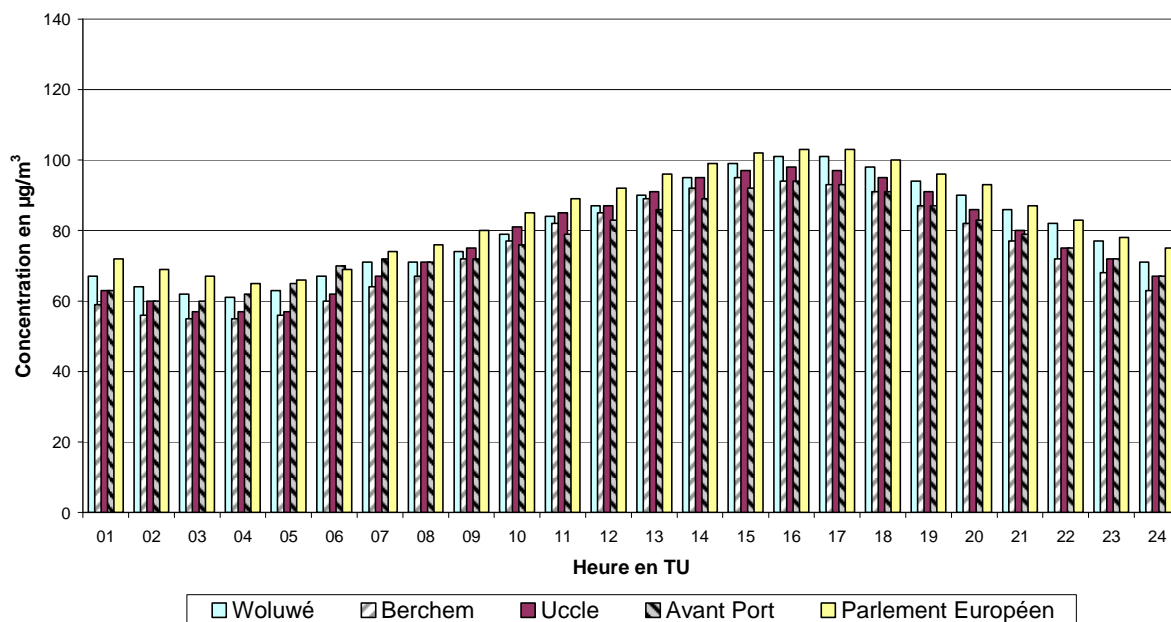
Fig. 10 : Évolution journalière moyenne des concentrations en [O 3 + NO 2 ], exprimées en équivalent O 3 , durant la période mai – août 2010
