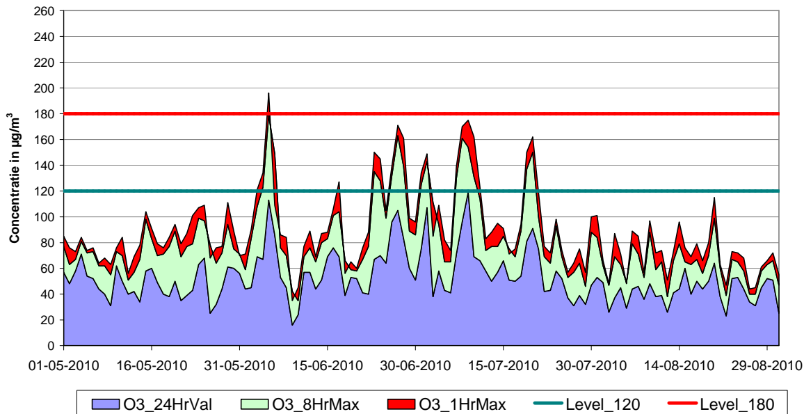
Fig. 22 : Ozone – Évolution Valeur Journalière (24HrVal), valeur maximale sur 8 heures (8HrMax) et valeur maximale horaire (1HrMax). Période : mai – août 2010. Postes de mesure à Uccle et Berchem-Ste-Agathe
