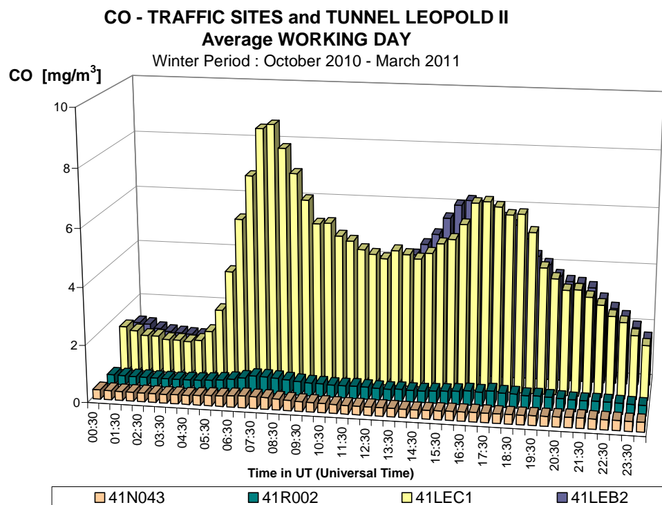
Fig. 33 : CO-dagverloop voor een gemiddelde werkdag tijdens de winter 2010-2011 Meetposten verkeer in de omgevingslucht – Voorhaven (N043) en Kroonlaan (R002) Meetposten in de tunnel Leopold II – LEC1 (centrum) en LEC2 (basiliek)
