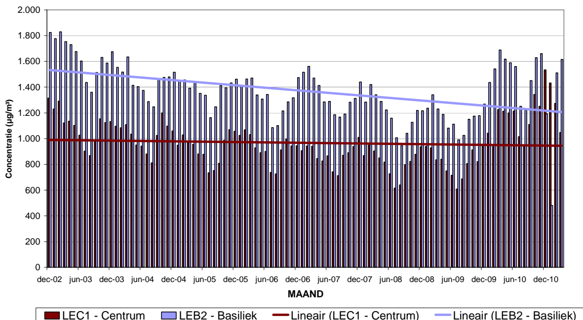
Fig. 9 : NO 2 en NO - Evolutie maandgemiddelde concentratie in beide meetposten van de Leopold II tunnel. Periode "December 2002 – Maart 2011"
