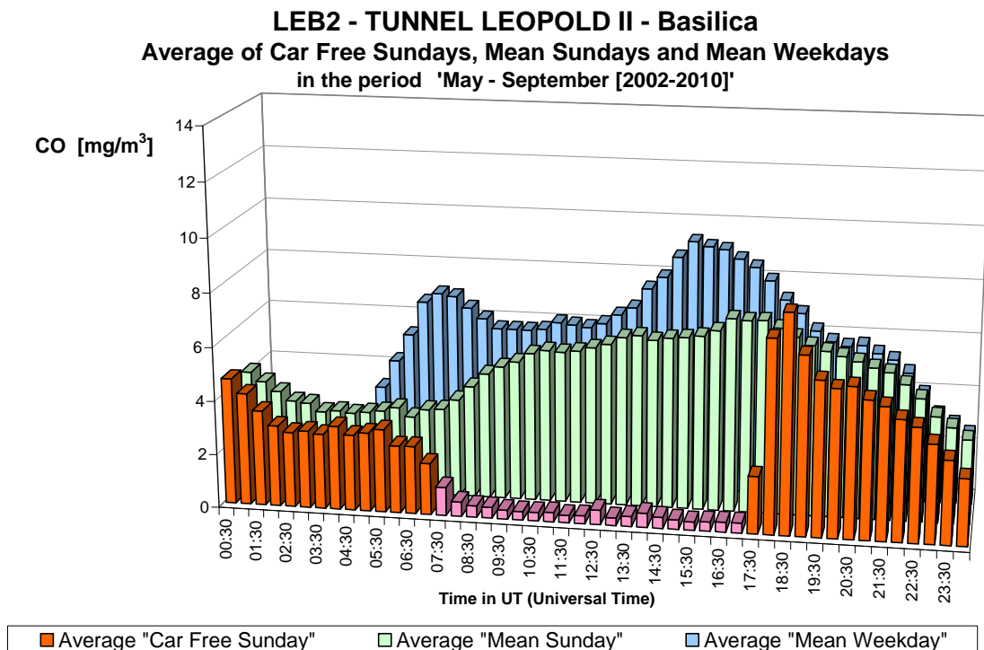
Fig. 32.b : CO in de Leopold II tunnel, richting Basiliek – Gemiddelde Dagprofiel van de negen autoluwe zondagen en van alle zondagen en werkdagen in de periodes 'mei – september 2002-2010'
