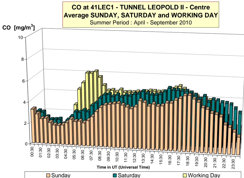
Fig. 19 : CO-dagverloop in de meetpost 41LEC1 (richting centrum) Vergelijking voor een gemiddelde zondag, zaterdag en werkdag Winterperiode 2010-2011 en zomerperiode 2010
