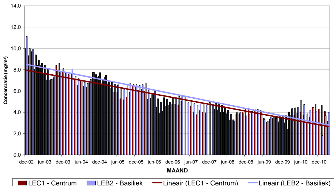
Fig. 10 : NO x en CO - Evolutie maandgemiddelde concentratie in beide meetposten van de Leopold II tunnel. Periode "December 2002 – Maart 2011"
