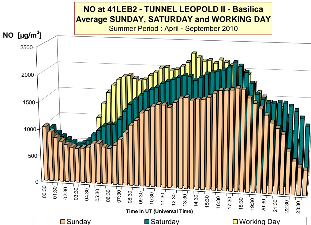
Fig. 18 : NO-dagverloop in de meetpost 41LEB2 (richting basiliek) Vergelijking voor een gemiddelde zondag, zaterdag en werkdag Winterperiode 2010-2011 en zomerperiode 2010
