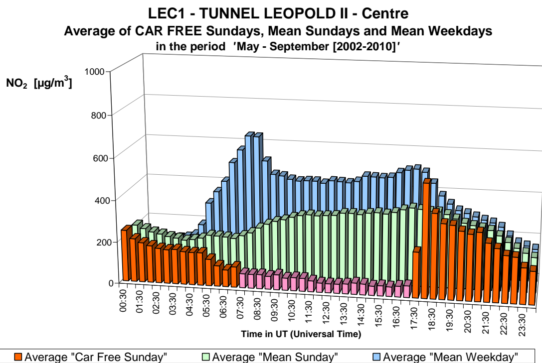
Fig. 27.b : NO 2 in de Leopold II tunnel, richting Centrum – Gemiddelde Dagprofiel van de negen autoluwe zondagen en van alle zondagen en werkdagen in de periodes ‘mei – september 2002-2010’
