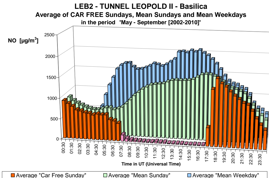
Fig. 30.b : NO in de Leopold II tunnel, richting Basiliek – Gemiddelde Dagprofiel van de negen autoluwe zondagen en van alle zondagen en werkdagen in de periodes 'mei – september 2002-2010'
