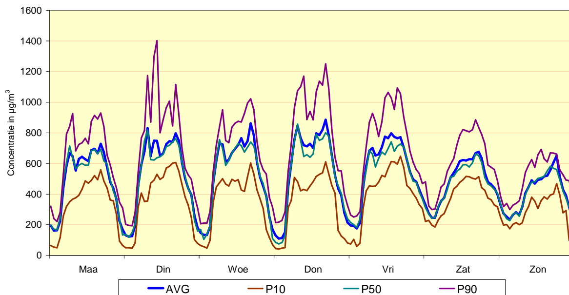
Fig. 21 : Meetpost 41LEC1 (centrum) - Gemiddeld weekverloop voor NO 2 Vergelijking winterperiode 2010 - 2011 en zomerperiode 2010
