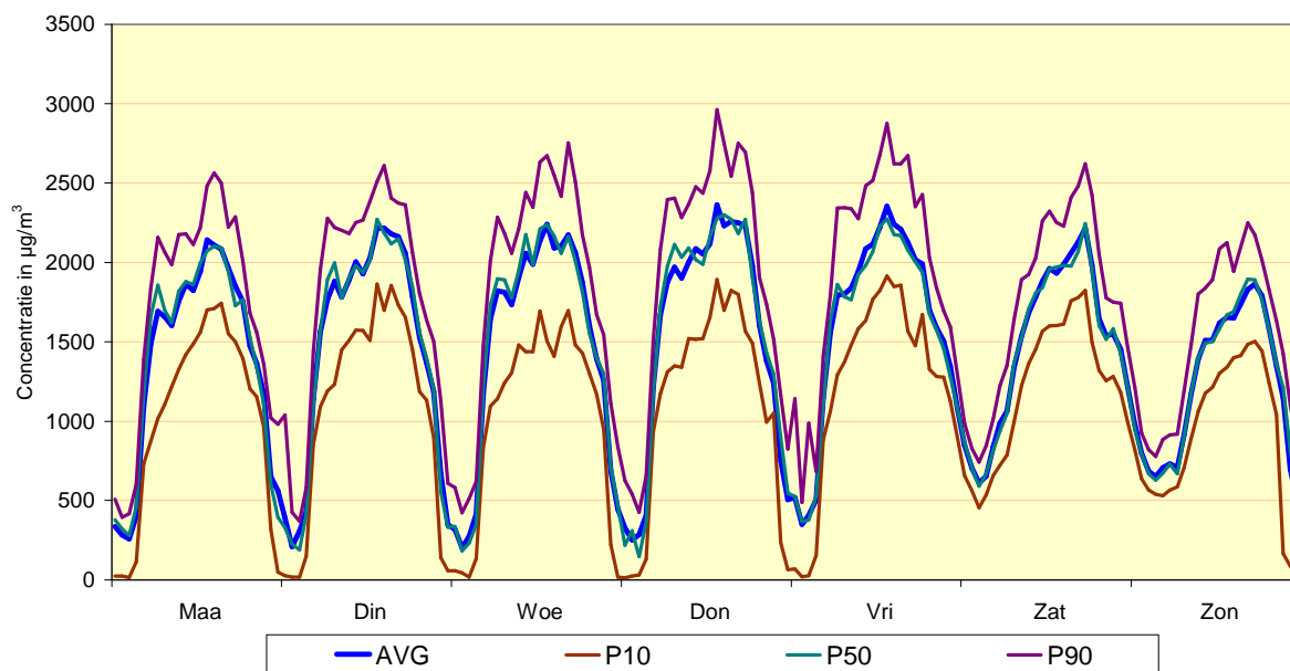
Fig. 26 : Meetpost 41LEB2 (basiliek) - Gemiddeld weekverloop voor NO Vergelijking winterperiode 2010 - 2011 en zomerperiode 2010
