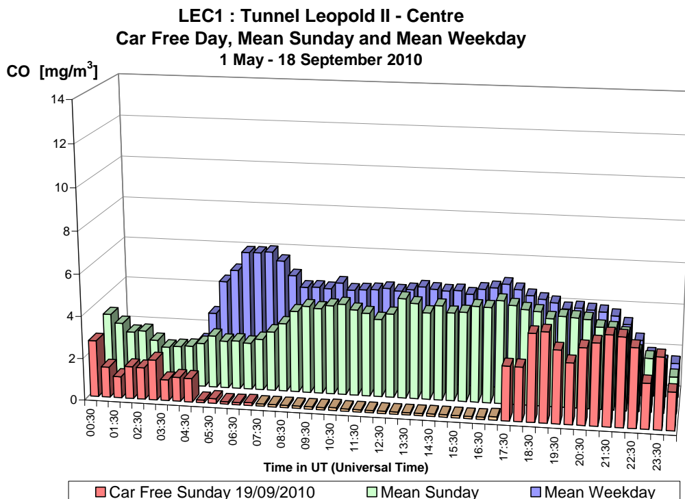
Fig. 31.a : CO in de Leopold II tunnel, richting Centrum – Dagprofiel autoluwe zondag 19-09-2010, gemiddelde zondag en gemiddelde werkdag in de periode ‘mei – september 2010’
