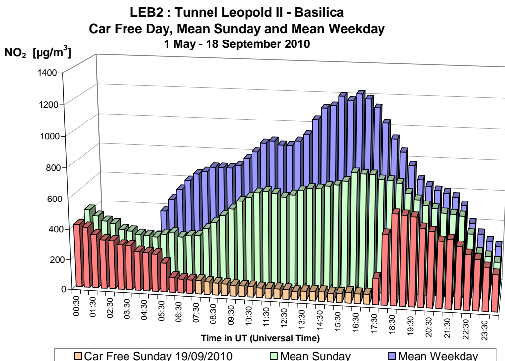
Fig. 28.a : NO 2 in de Leopold II tunnel, richting Basiliek – Dagprofiel autoluwe zondag 19-09-2010, gemiddelde zondag en een gemiddelde werkdag in de periode ‘mei – september 2010’
