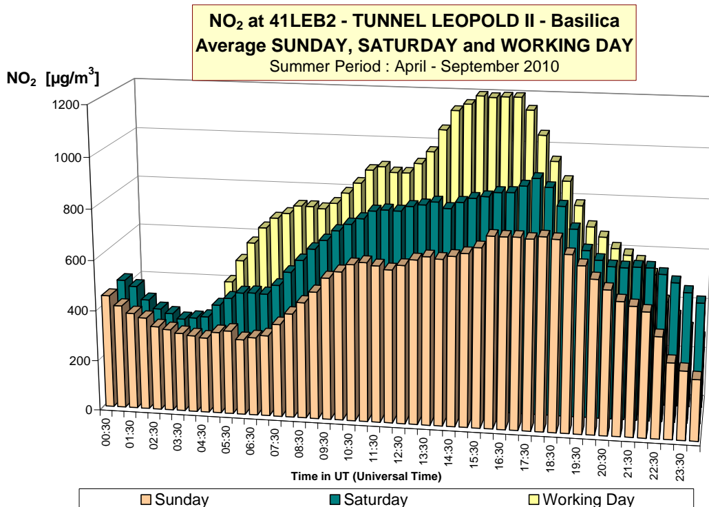
Fig. 16 : NO 2 -dagverloop in de meetpost 41LEB2 (richting basiliek) Vergelijking voor een gemiddelde zondag, zaterdag en werkdag Winterperiode 2010-2011 en zomerperiode 2010
