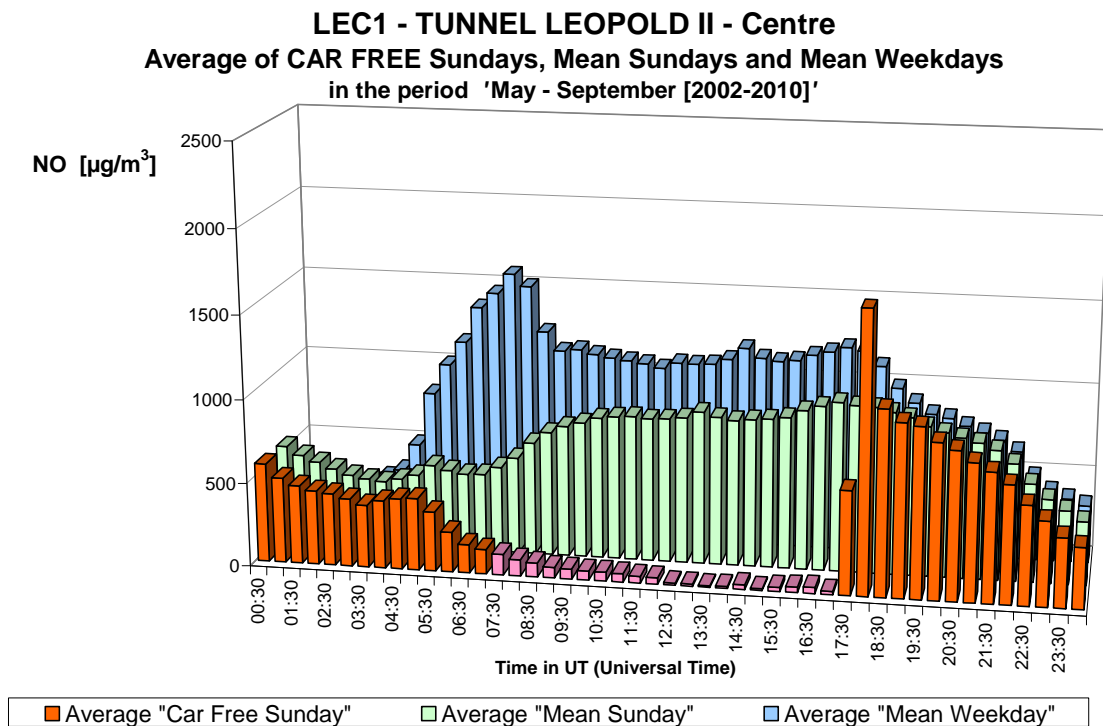
Fig. 29.b : NO in de Leopold II tunnel, richting Centrum – Gemiddelde Dagprofiel van de negen autoluwe zondagen en van alle zondagen en werkdagen in de periodes ‘mei – september 2002-2010’
