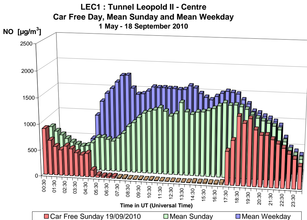
Fig. 29.a : NO in de Leopold II tunnel, richting Centrum – Dagprofiel autoluwe zondag 19-09-2010, gemiddelde zondag en gemiddelde werkdag in de periode ‘mei – september 2010’
