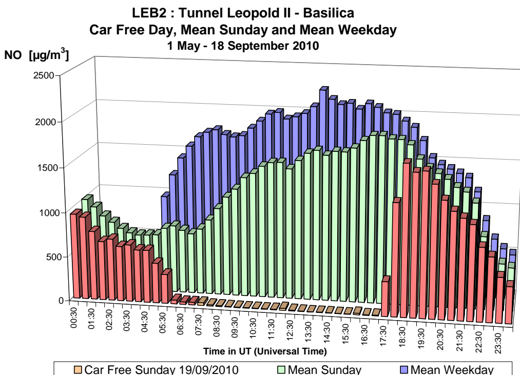
Fig. 30.a : NO in de Leopold II tunnel, richting Basiliek – Dagprofiel autoluwe zondag 19-09-2010, gemiddelde zondag en een gemiddelde werkdag in de periode 'mei – september 2010'
