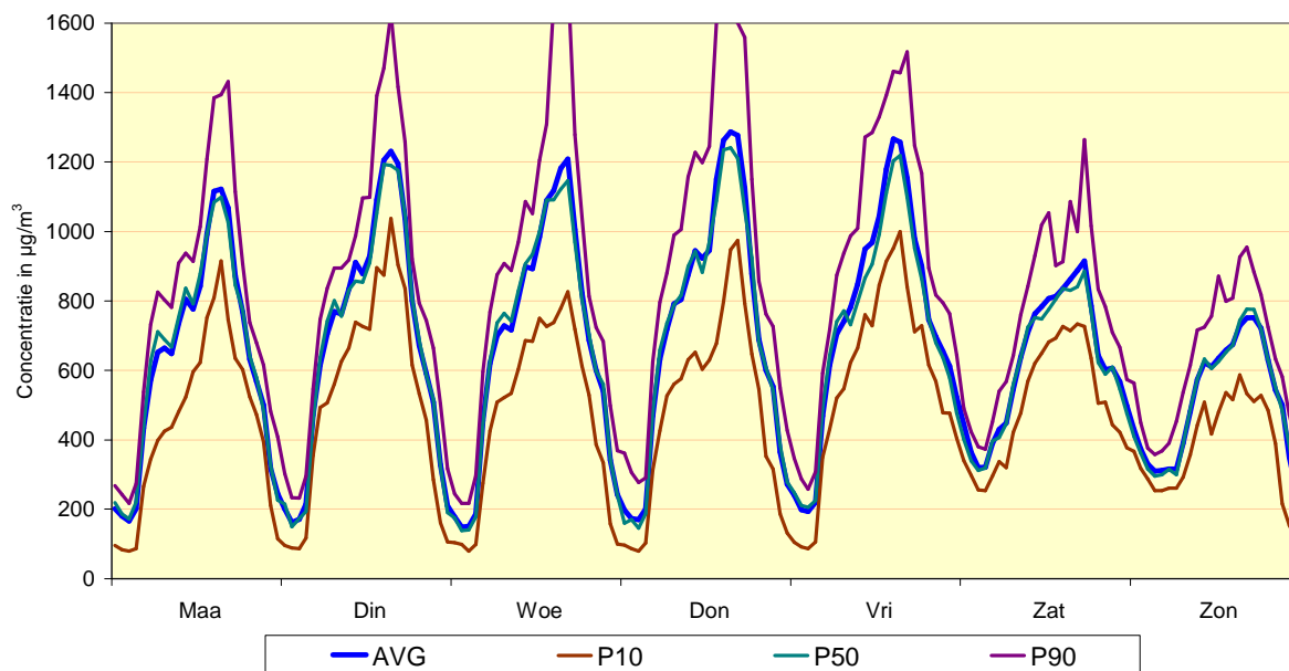
Fig. 22 : Meetpost 41LEB2 (basiliek) - Gemiddeld weekverloop voor NO 2 Vergelijking winterperiode 2010 - 2011 en zomerperiode 2010
