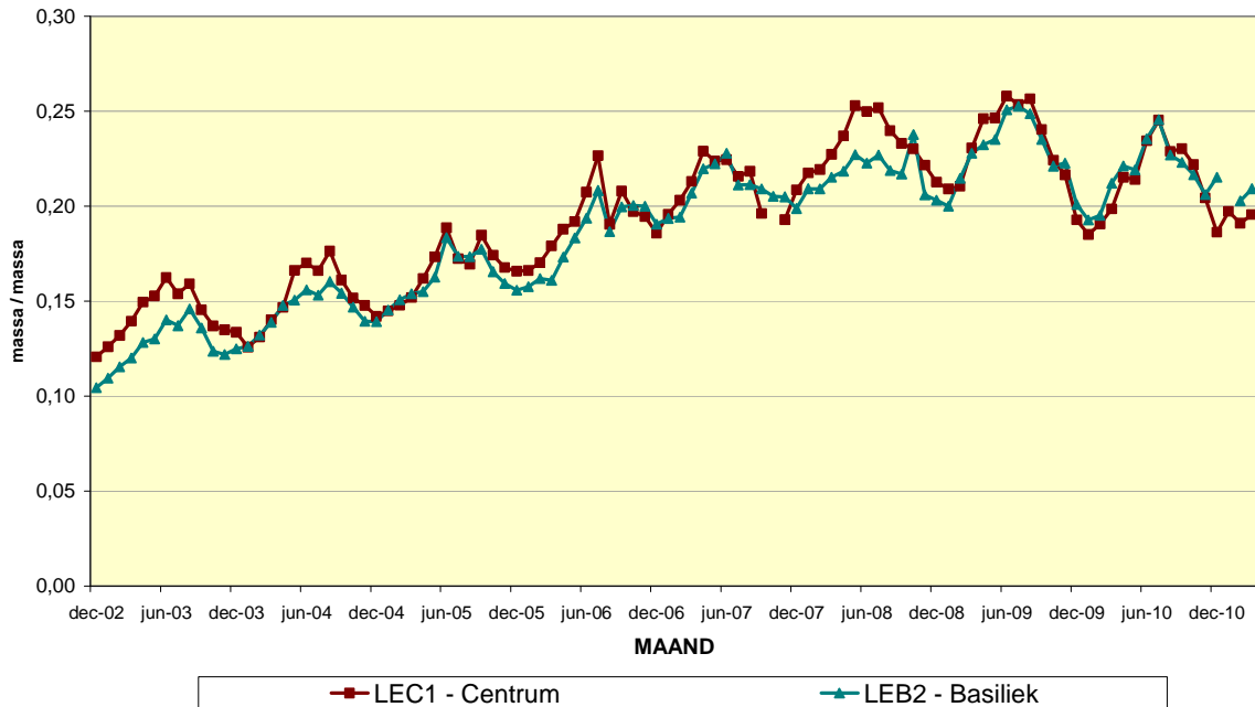
Fig. 11 : Evolutie van de verhouding NO 2 /NO x in beide meetposten van de Leopold II tunnel. Periode "December 2002 – Maart 2011"
