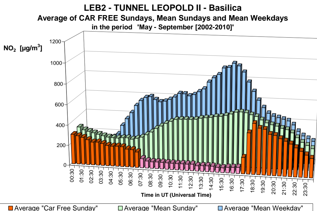
Fig. 28.b : NO 2 in de Leopold II tunnel, richting Basiliek – Gemiddelde Dagprofiel van de negen autoluwe zondagen en van alle zondagen en werkdagen in de periodes ‘mei – september 2002-2010’
