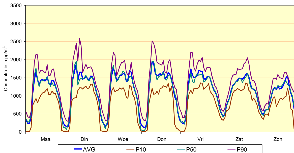
Fig. 25 : Meetpost 41LEC1 (centrum) - Gemiddeld weekverloop voor NO Vergelijking winterperiode 2010 - 2011 en zomerperiode 2010
