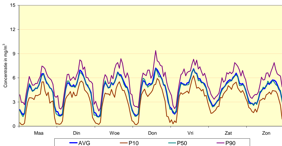
Fig. 24 : Meetpost 41LEB2 (basiliek) - Gemiddeld weekverloop voor CO Vergelijking winterperiode 2010 - 2011 en zomerperiode 2010
