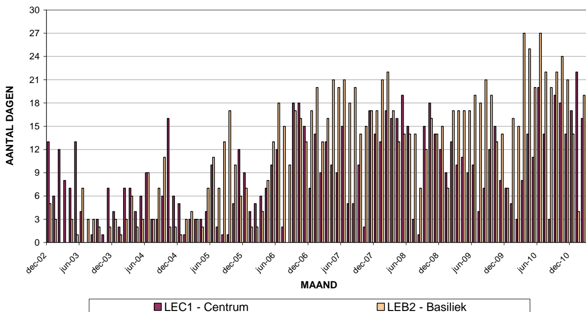
Fig. 12 : NO 2 – 20-Minutsgemiddelden > 1.000 µg/m 3 . Totaal aantal overschrijdingen per maand en aantal dagen per maand met overschrijding (december 2002 – maart 2011)
