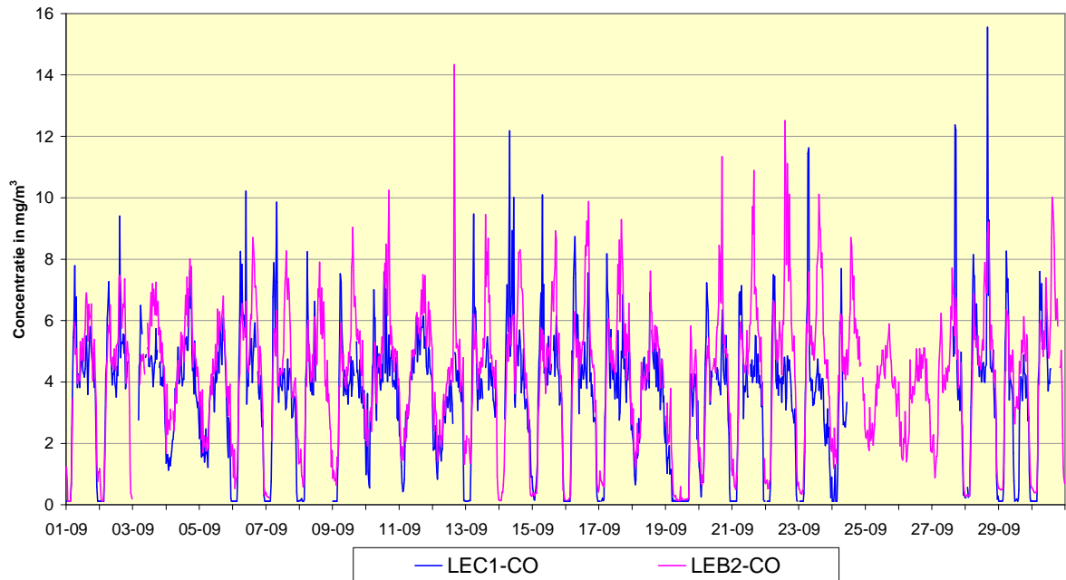
Fig. 3: CO - Evolutie van de uurwaarden en de halfuurwaarden tijdens de maand september 2010 Meetplaats 41LEC1, richting Centrum - Meetplaats 41LEB2, richting Basiliek
