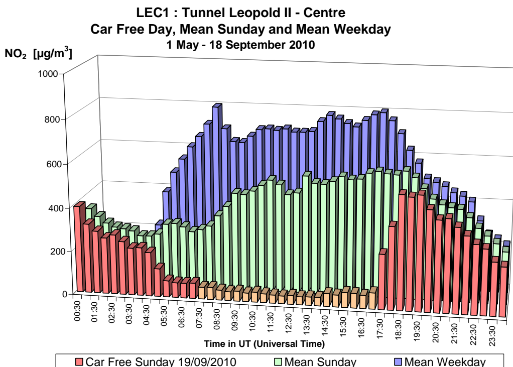
Fig. 27.a : NO 2 in de Leopold II tunnel, richting Centrum – Dagprofiel autoluwe zondag 19-09-2010, gemiddelde zondag en gemiddelde werkdag in de periode ‘mei – september 2010’
