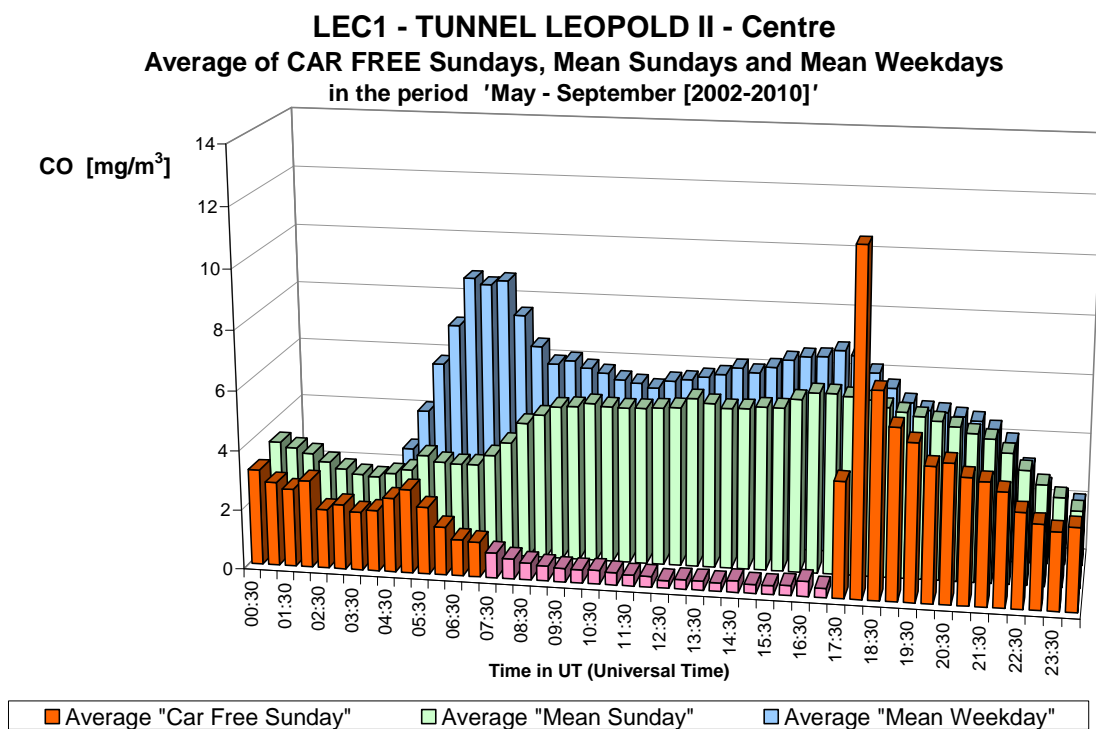
Fig. 31.b : CO in de Leopold II tunnel, richting Centrum – Gemiddelde Dagprofiel van de negen autoluwe zondagen en van alle zondagen en werkdagen in de periodes ‘mei – september 2002-2010’
