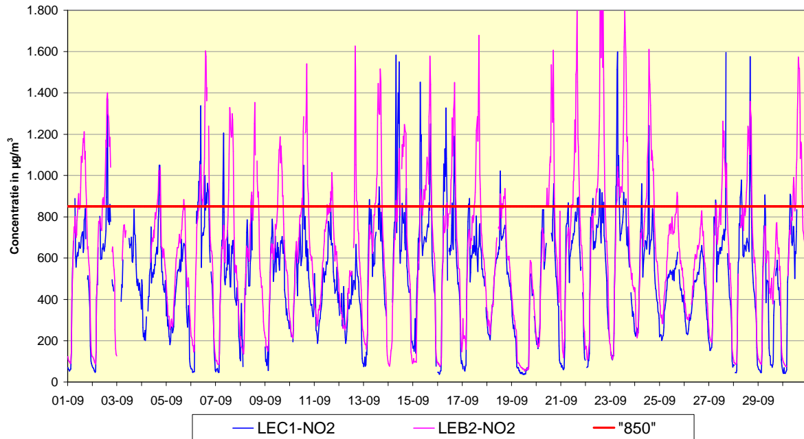
Fig. 1: NO 2 - Evolutie van de uurwaarden en de halfuurwaarden tijdens de maand september 2010 Meetplaats 41LEC1, richting Centrum - Meetplaats 41LEB2, richting Basiliek
