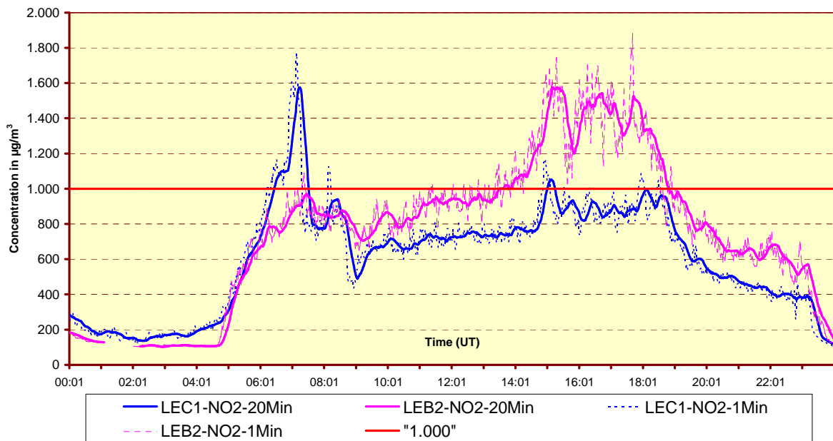
Fig. 4: NO 2 - evolutie minuutwaarden en voortschrijdend 20-minuutsgemiddelde in beide meetposten van de Leopold II tunnel Donderdag 7 oktober 2010 en maandag 22 november 2010
