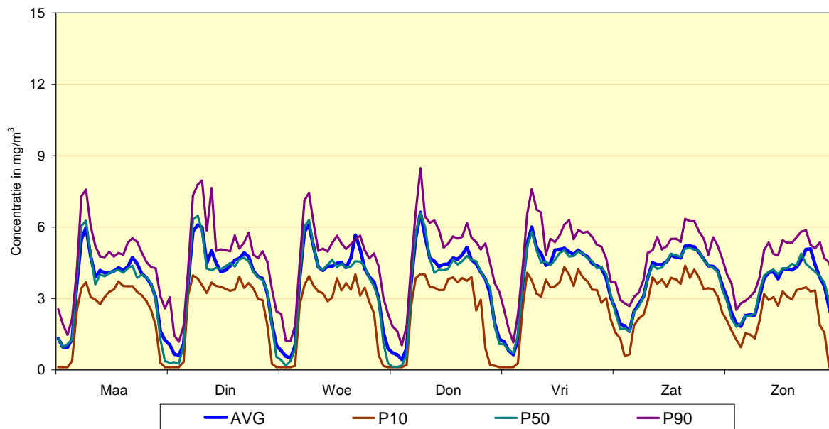
Fig. 23 : Meetpost 41LEC1 (centrum) - Gemiddeld weekverloop voor CO Vergelijking winterperiode 2010 - 2011 en zomerperiode 2010
