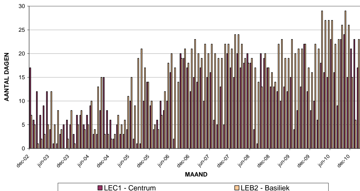
Fig. 13 : NO 2 – Halfuurswaarden > 850 µg/m 3 . Totaal aantal overschrijdingen per maand en aantal dagen per maand met overschrijding (december 2002 – maart 2011)
