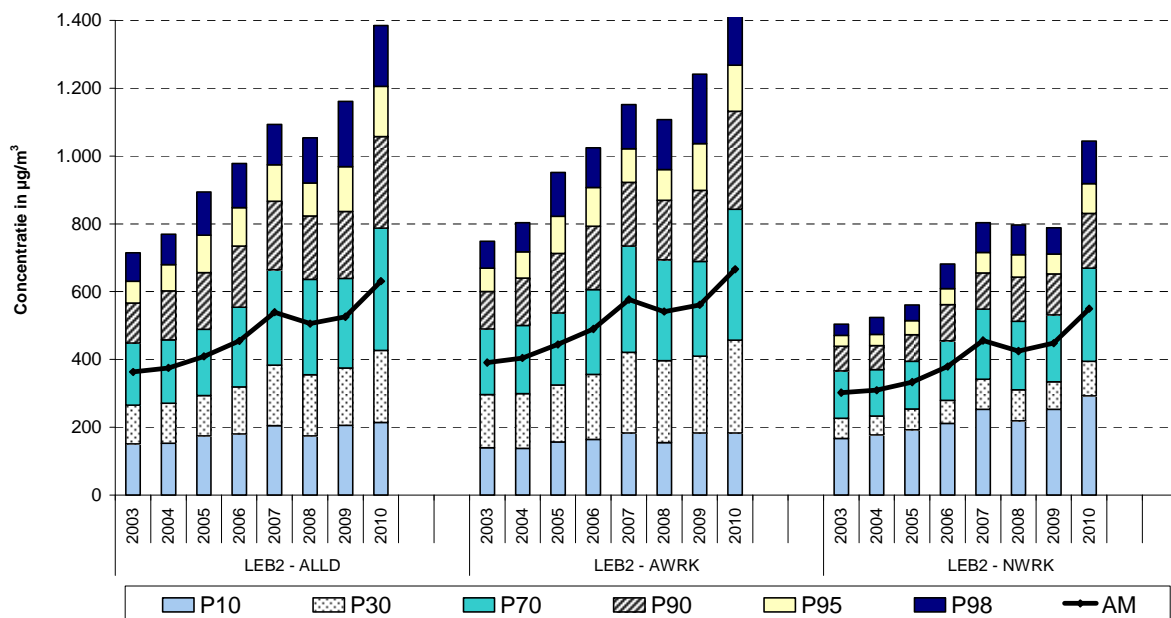
Fig. 5 : NO 2 - Cumulatieve Frequentieverdeling Uurwaarden in beide meetposten van de Leopold II tunnel. Selectie alle dagen , alle werkdagen en alle niet-werkdagen Jaarperiodes 2003 t/m 2010
