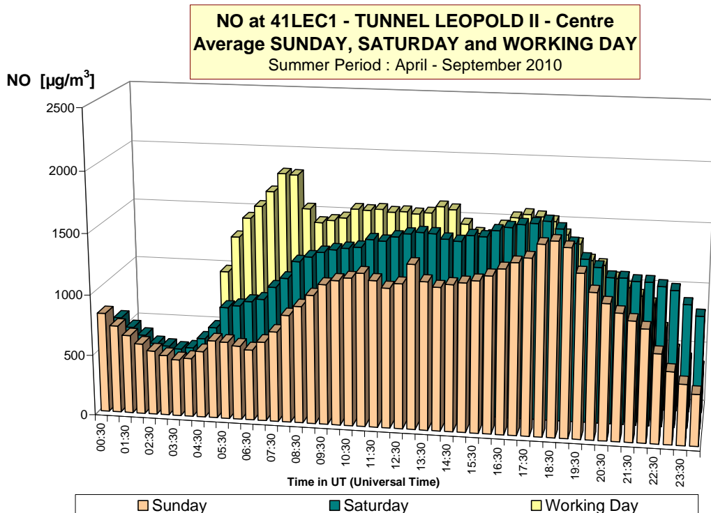
Fig. 17 : NO-dagverloop in de meetpost 41LEC1 (richting centrum) Vergelijking voor een gemiddelde zondag, zaterdag en werkdag Winterperiode 2010-2011 en zomerperiode 2010
