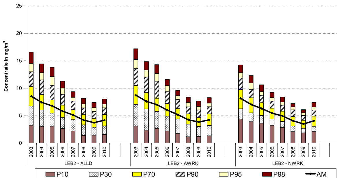
Fig. 6 : CO - Cumulatieve Frequentieverdeling Uurwaarden in beide meetposten van de Leopold II tunnel. Selectie alle dagen , alle werkdagen en alle niet-werkdagen Jaarperiodes 2003 t/m 2010
