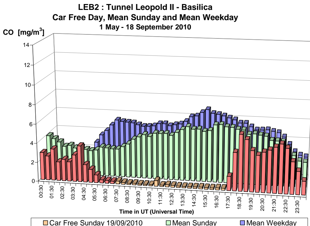
Fig. 32.a : CO in de Leopold II tunnel, richting Basiliek – Dagprofiel autoluwe zondag 19-09-2010, gemiddelde zondag en een gemiddelde werkdag in de periode 'mei – september 2010'
