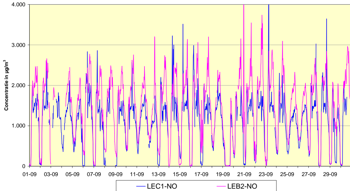
Fig. 2: NO - Evolutie van de uurwaarden en de halfuurwaarden tijdens de maand september 2010 Meetplaats 41LEC1, richting Centrum - Meetplaats 41LEB2, richting Basiliek
