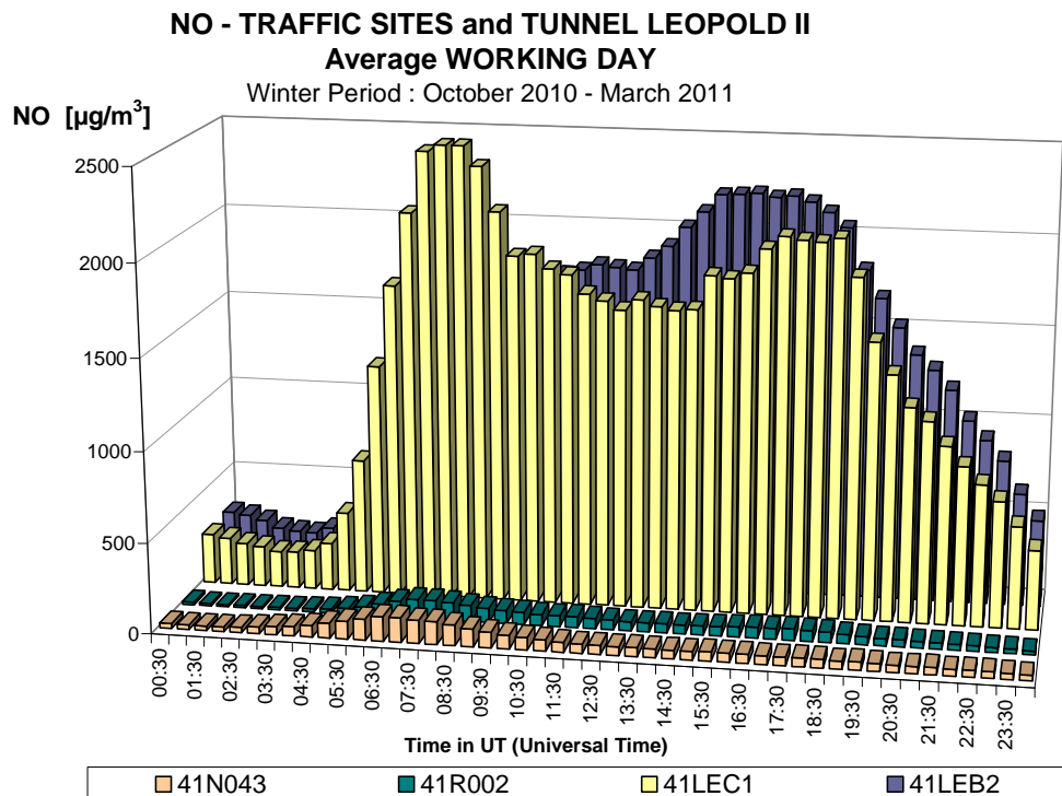
Fig. 34 : Dagverloop NO 2 en NO voor een gemiddelde werkdag tijdens de winter 2010-2011 Meetposten verkeer in de omgevingslucht – Voorhaven (N043) en Kroonlaan (R002) Meetposten in de tunnel Leopold II – LEC1 (centrum) en LEC2 (basiliek)
