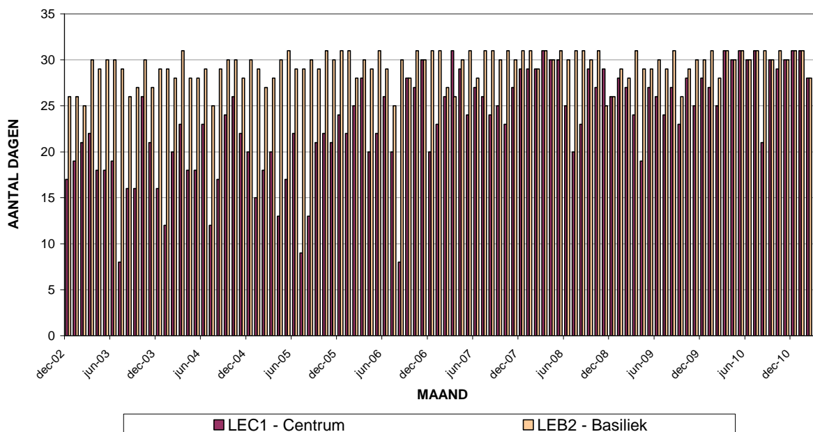
Fig. 14 : NO 2 -Uurwaarden > 400 µg/m 3 . Totaal aantal overschrijdingen per maand en aantal dagen per maand met overschrijding (december 2002 – maart 2011)
