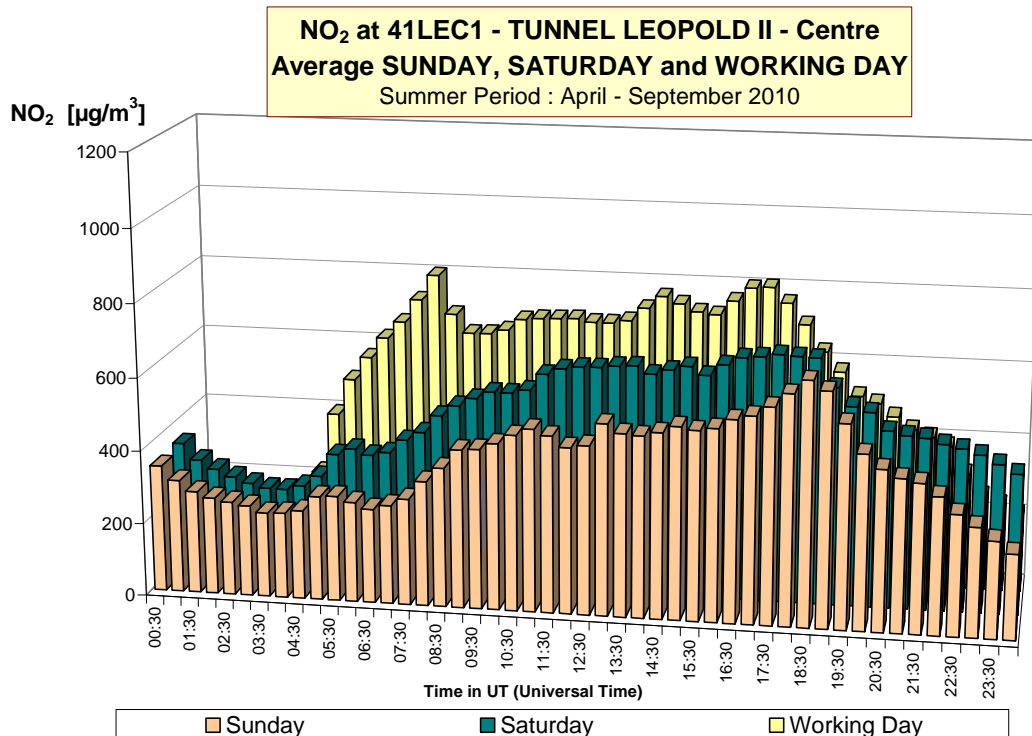
Fig. 15 : NO 2 -dagverloop in de meetpost 41LEC1 (richting centrum) Vergelijking voor een gemiddelde zondag, zaterdag en werkdag Winterperiode 2010-2011 en zomerperiode 2010
