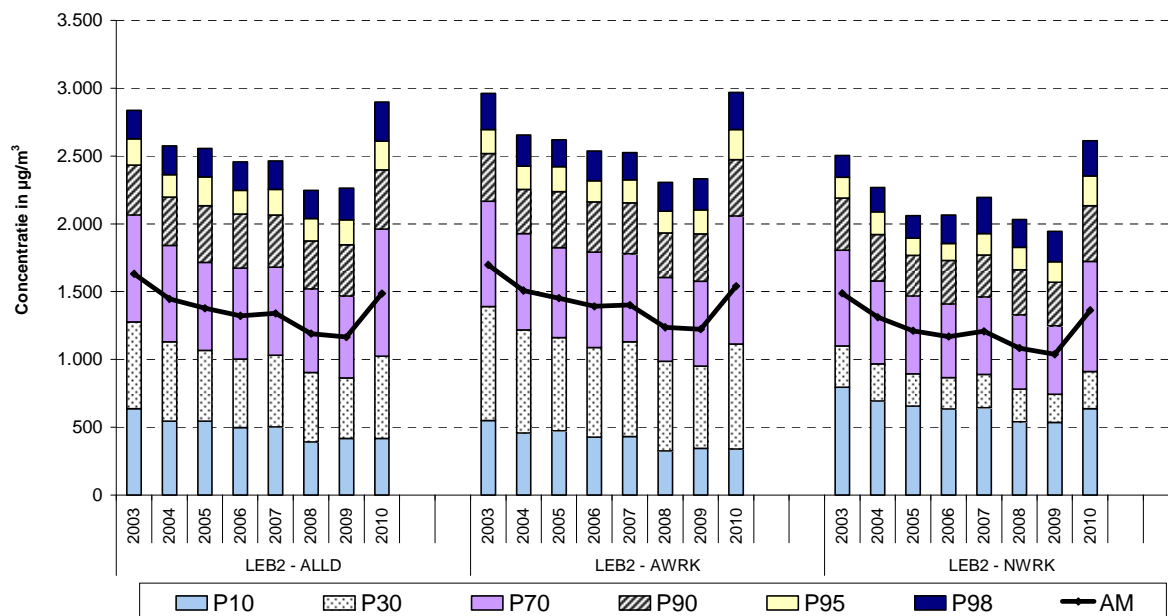
Fig. 7 : NO - Cumulatieve Frequentieverdeling Uurwaarden in beide meetposten van de Leopold II tunnel. Selectie alle dagen , alle werkdagen en alle niet-werkdagen Jaarperiodes 2003 t/m 2010
