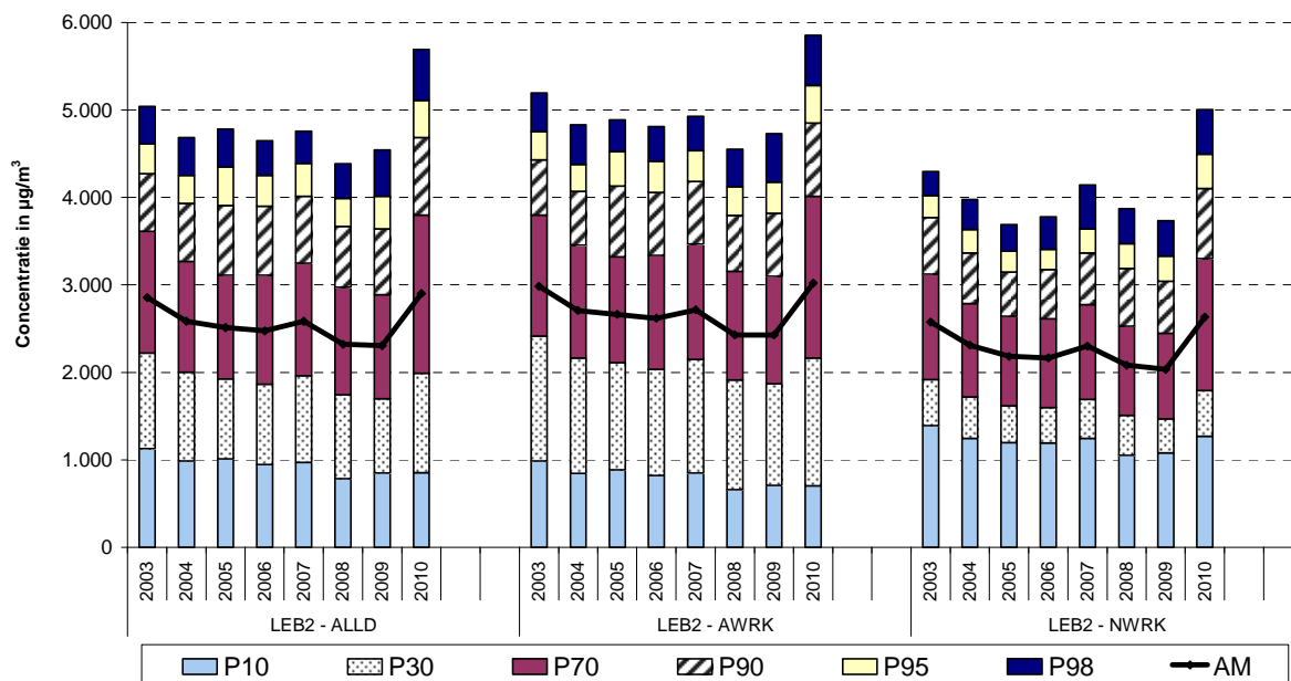
Fig. 8 : NO x - Cumulatieve Frequentieverdeling Uurwaarden in beide meetposten van de Leopold II tunnel. Selectie alle dagen , alle werkdagen en alle niet-werkdagen Jaarperiodes 2003 t/m 2010
