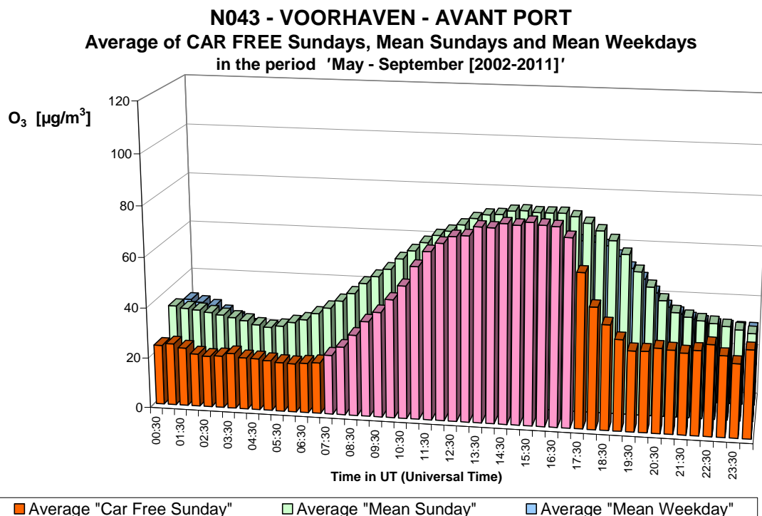
Fig. 21.b : O 3 in de Voorhaven – Gemiddelde Dagprofiel van de tien autoluwe zondagen en van alle zondagen en werkdagen in de periodes “mei – september 2002-2011”.
