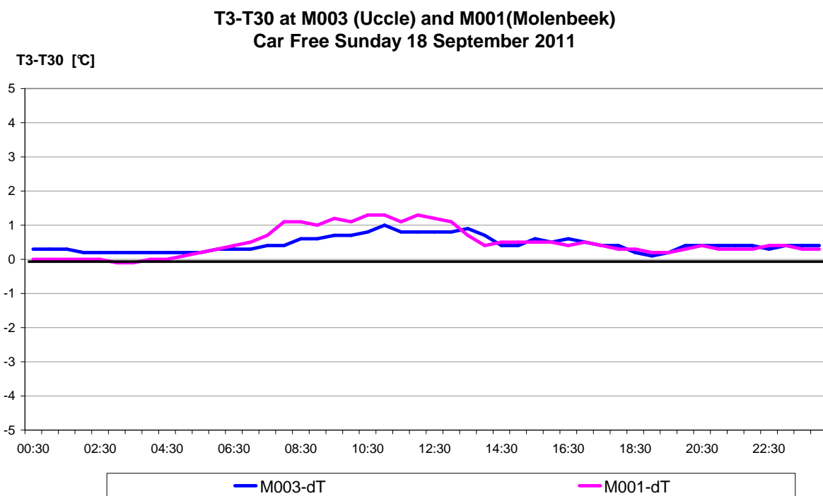
Fig. 9.a : Autoluwe zondag 18-09-2011: Temperatuurverschil tussen 3 en 30 m hoogte [ dT = T_3 - T_{30} ] Een negatieve waarde betekent een temperatuursinversie in de onderste luchtlaag, tegen de grond.
