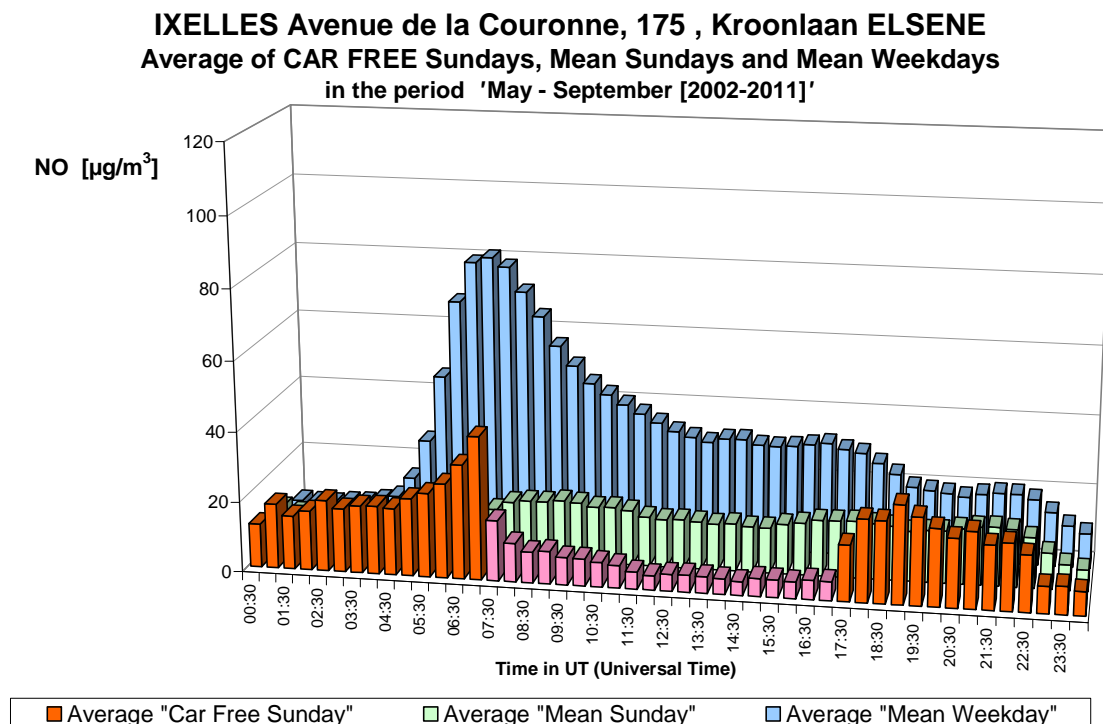
Fig. 10.b : NO in de Kroonlaan te Elsene – Gemiddelde Dagprofiel van de tien autoluwe zondagen en van alle zondagen en werkdagen in de periodes “mei – september 2002-2011”.
