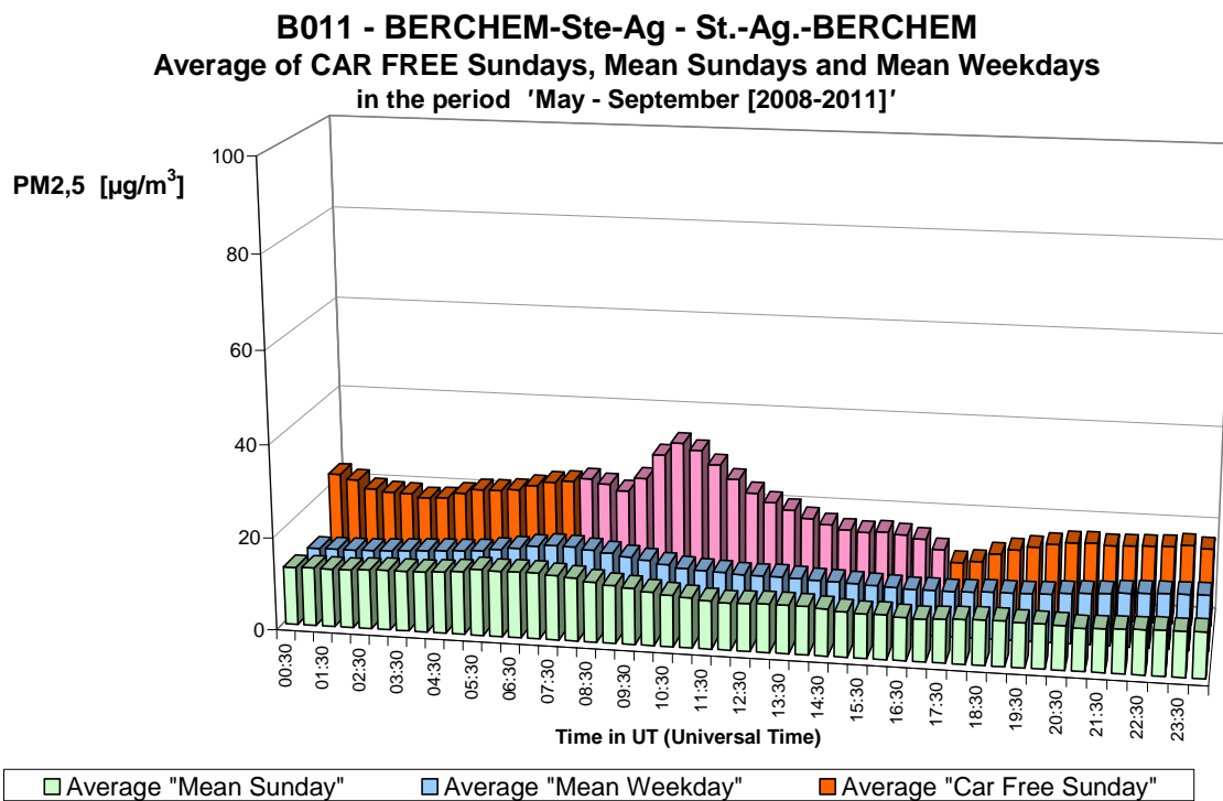
Fig. 37.b : PM2,5 te Berchem – Gemiddelde Dagprofiel van alle zondagen, van alle werkdagen en van de vier autoluwe zondagen in de periodes “mei – september 2008-2011”.
