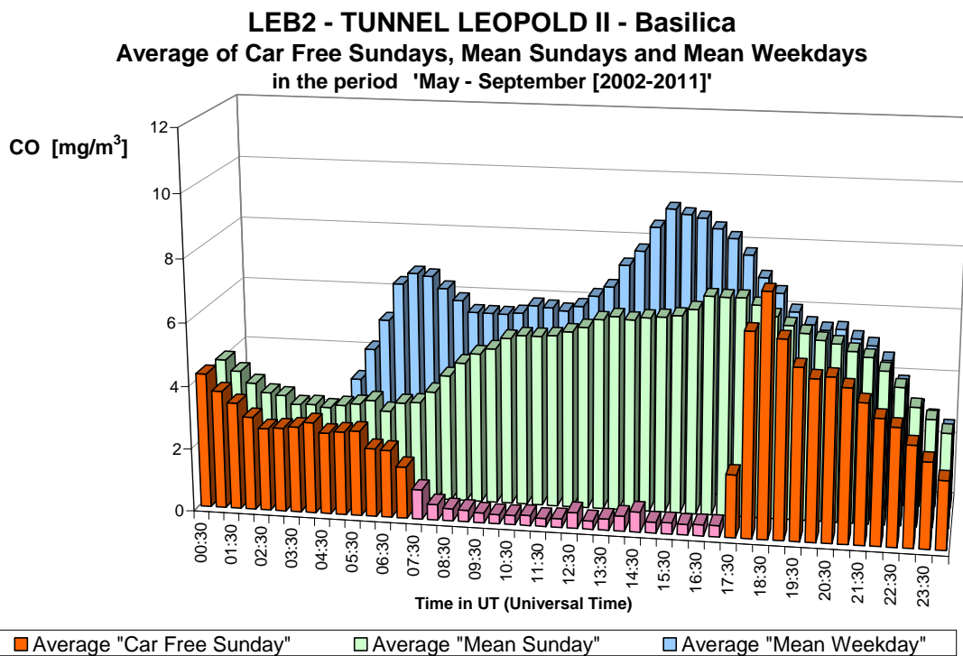
Fig. 8.b : CO in de Leopold II tunnel, richting Basiliek – Gemiddelde Dagprofiel van de tien autoluwe zondagen en van alle zondagen en werkdagen in de periodes “mei – september 2002-2011”.
