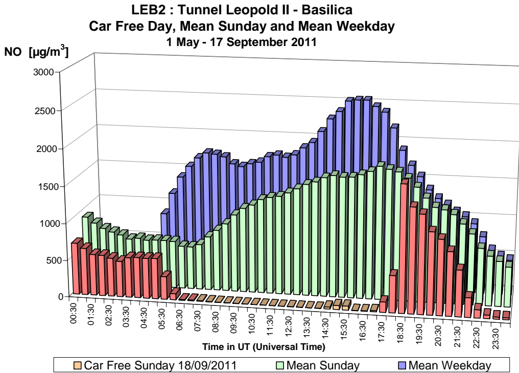
Fig. 5.a : NO in de Leopold II tunnel, richting Basiliek – Dagprofiel autoluwe zondag 18-09-2011, gemiddelde zondag en gemiddelde werkdag in de periode “mei – september 2011”.
