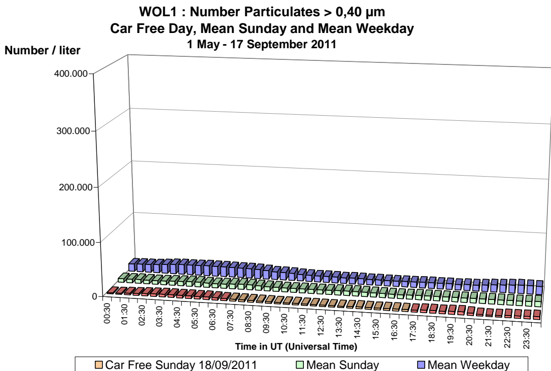
Fig. 46 : St.-Lambr.-Woluwe – Aantal Deeltjes > 0,40 µm – Dagprofiel van de autoluwe zondag van 18-09-2011 en van een gemiddelde zondag en een gemiddelde werkdag (mei – september 2011)
