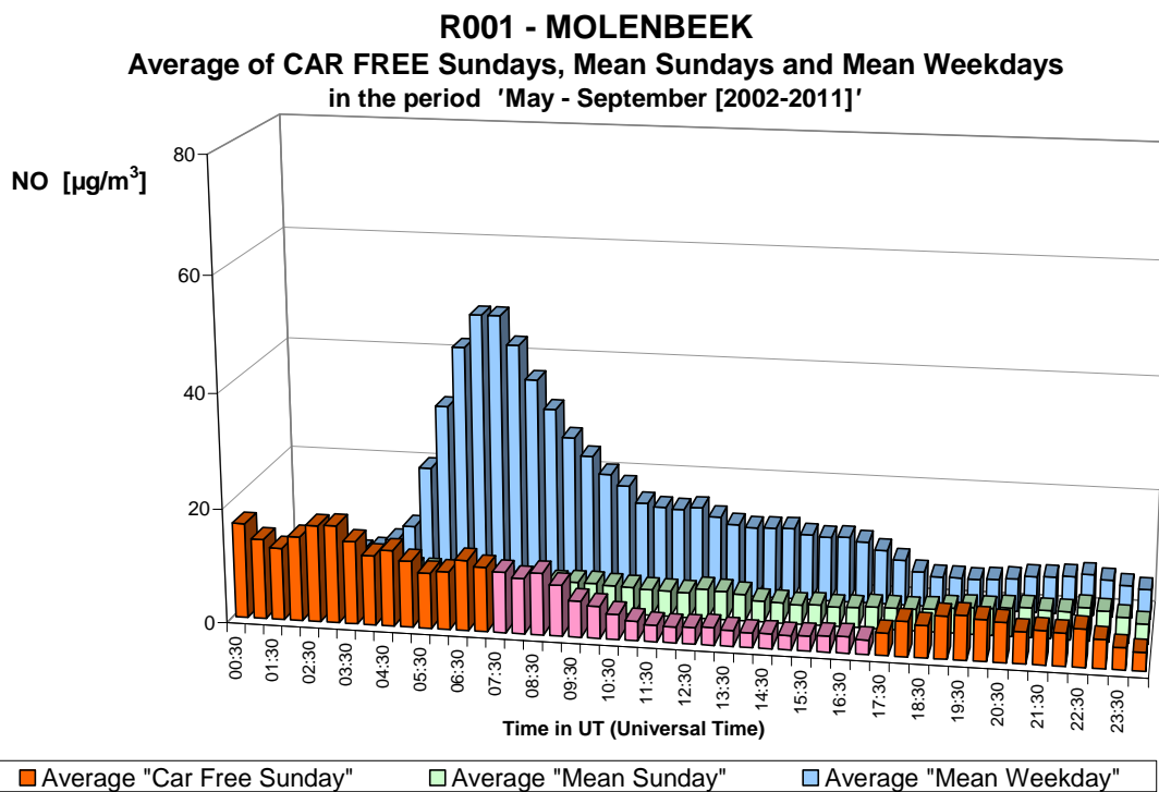
Fig. 12.b : NO te Molenbeek – Gemiddelde Dagprofiel van de tien autoluwe zondagen en van alle zondagen en werkdagen in de periodes “mei – september 2002-2011”.
