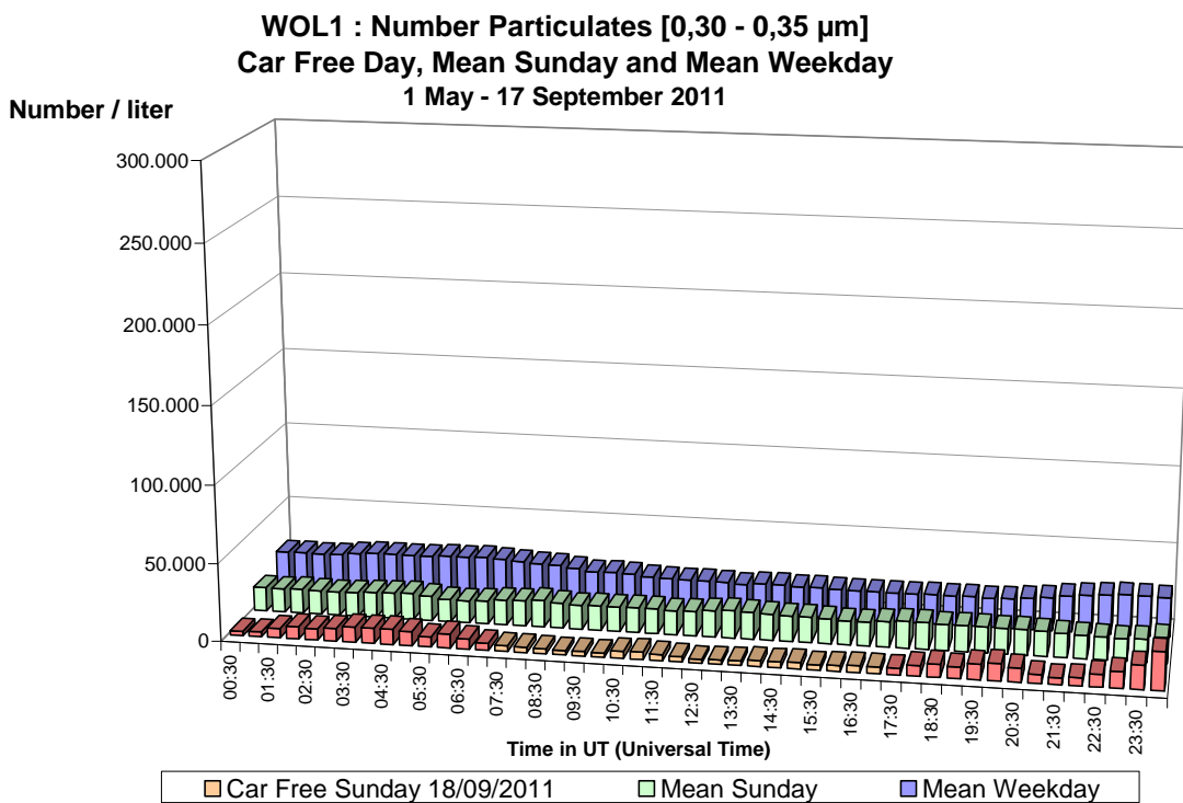
Fig. 53 : St.-Lambr.-Woluwe – Aantal Deeltjes tussen 0,30 en 0,35 µm – Dagprofiel van de autoluwe zondag van 18-09-2011 en van een gemiddelde zondag en werkdag (mei – september 2011)
