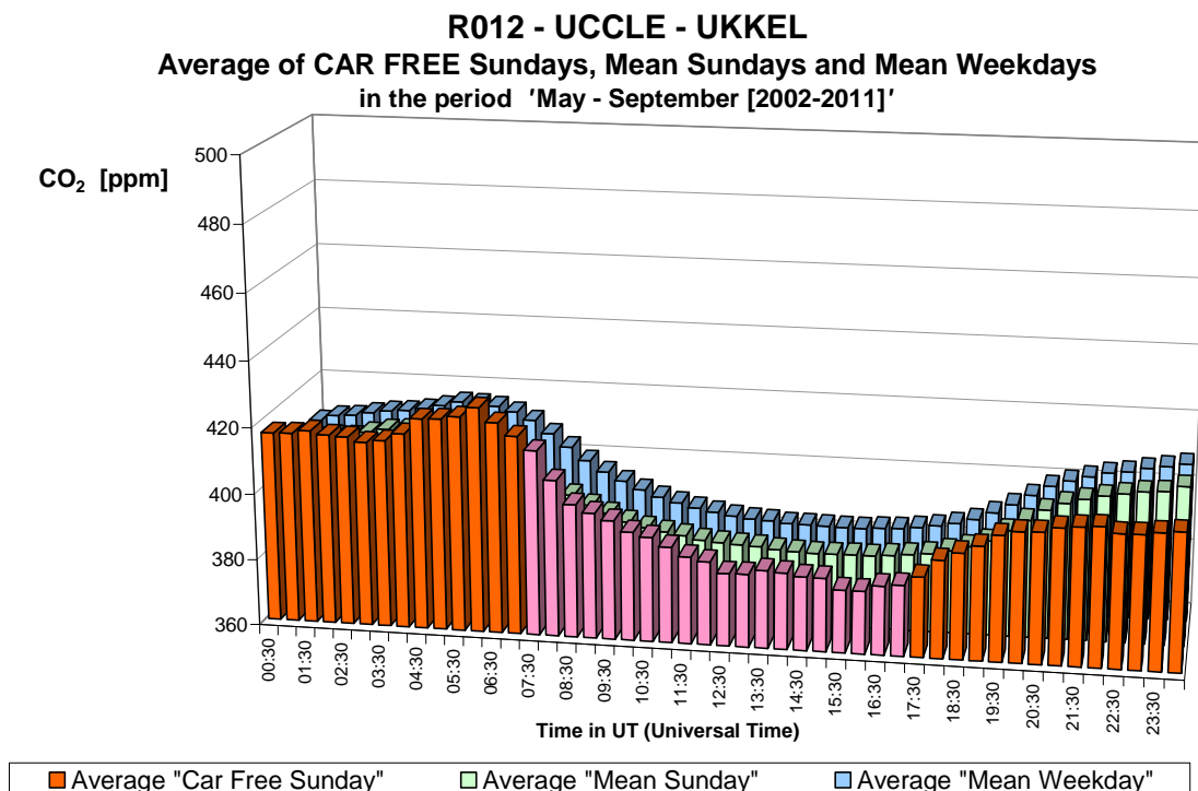
Fig. 29.b : CO 2 te Ukkel – Gemiddelde Dagprofiel van de tien autoluwe zondagen en van alle zondagen en werkdagen in de periodes “mei – september 2002-2011”.
