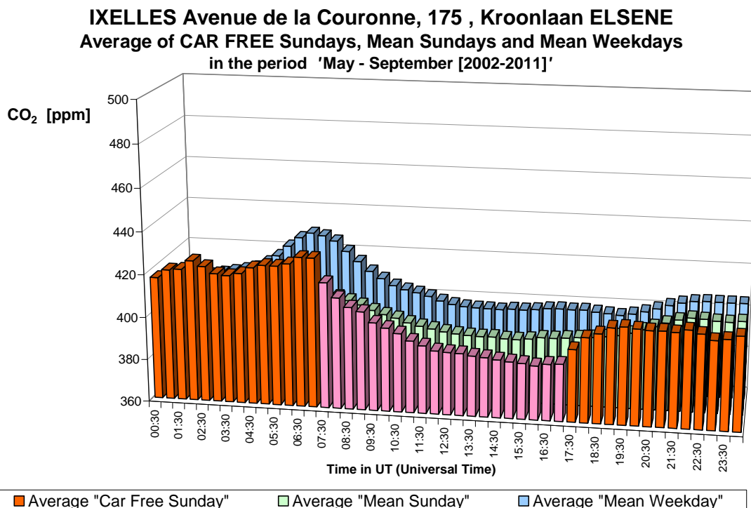
Fig. 27.b : CO 2 in de Kroonlaan te Elsene – Gemiddelde Dagprofiel van de tien autoluwe zondagen en van alle zondagen en werkdagen in de periodes “mei – september 2002-2011”.
