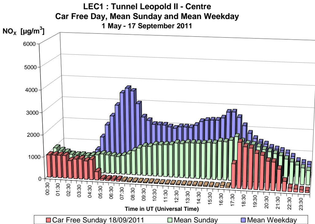
Fig. 3.a : NO x in de Leopold II tunnel, richting Centrum – Dagprofiel autoluwe zondag 18-09-2011, gemiddelde zondag en gemiddelde werkdag in de periode “mei – september 2011”.
