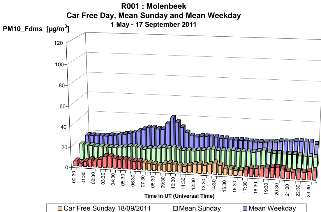
Fig. 30.a : PM10 te Molenbeek – Dagprofiel van de autoluwe zondag 18-09-2011, van een gemiddelde zondag en een gemiddelde werkdag in de periode “mei – september 2011”.
