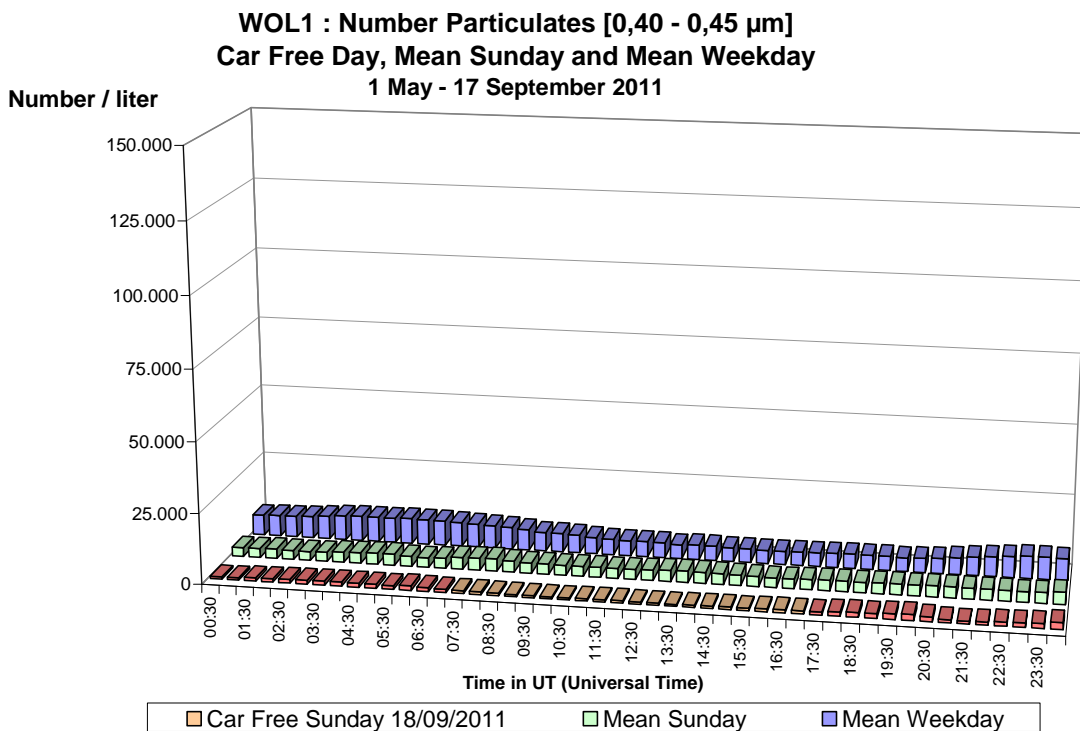
Fig. 54 : St.-Lambr.-Woluwe – Aantal Deeltjes tussen 0,40 en 0,45 µm – Dagprofiel van de autoluwe zondag van 18-09-2011 en van een gemiddelde zondag en werkdag (mei – september 2011)
