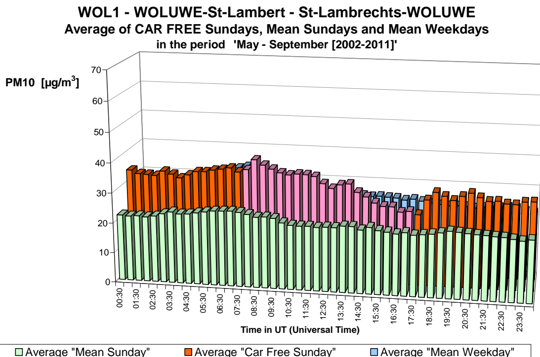
Fig. 35.b : PM10 te St.-Lambr.-Woluwe – Gemiddelde Dagprofiel van alle zondagen, van de tien autoluwe zondagen en van alle werkdagen in de periodes “mei – september 2002-2011”.
