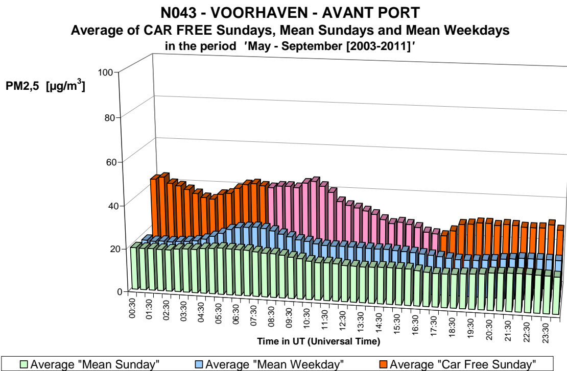
Fig. 39.b : PM2,5 in de Voorhaven – Gemiddelde Dagprofiel van alle zondagen, van alle werkdagen en van de negen autoluwe zondagen in de periodes “mei – september 2003-2011”.
