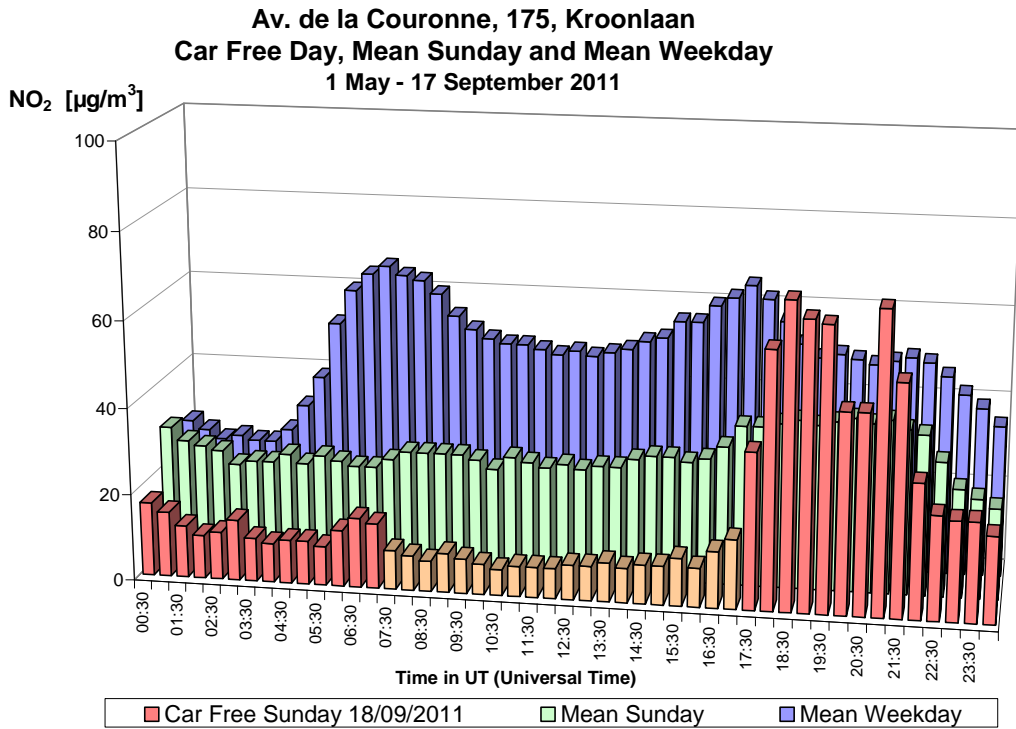
Fig. 11.a : NO 2 in de Kroonlaan te Elsene – Dagprofiel autoluwe zondag 18-09-2011, gemiddelde zondag en gemiddelde werkdag in de periode “mei – september 2011”.
