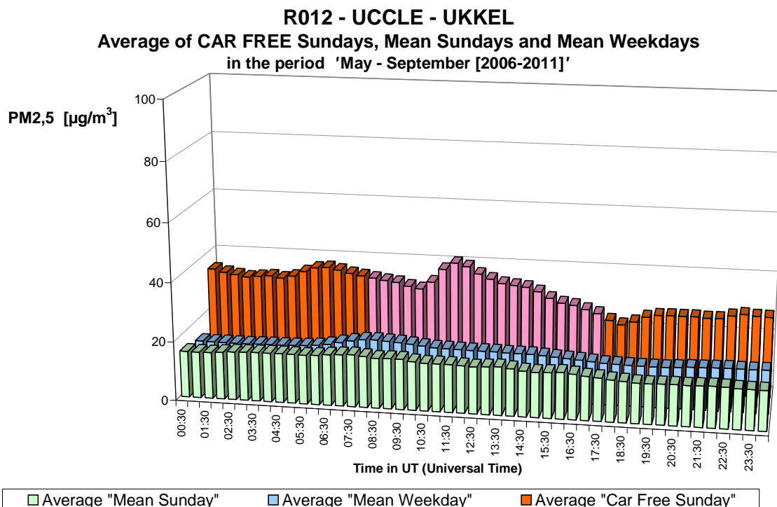
Fig. 38.b : PM 2,5 te Ukkel – Gemiddelde Dagprofiel van alle zondagen, van alle werkdagen en van de zes autoluwe zondagen in de periodes “mei – september 2006-2011”.
