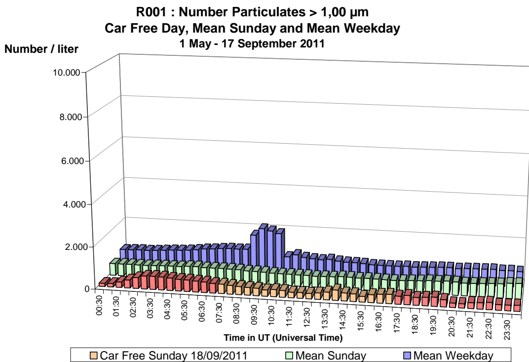
Fig. 63 Molenbeek – Aantal Deeltjes > 1,00 \mu\text{m} – Dagprofiel van de autoluwe zondag van 18-09-2011 en van een gemiddelde zondag en een gemiddelde werkdag (mei – september 2011)
