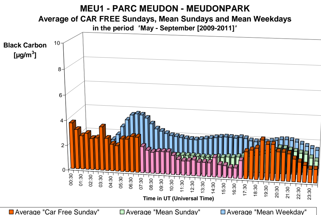
Fig. 43.b : Black Carbon te Woluwe – Gemiddelde Dagprofiel van de drie autoluwe zondagen en van alle zondagen en alle werkdagen in de periodes “mei – september 2009-2011”.
