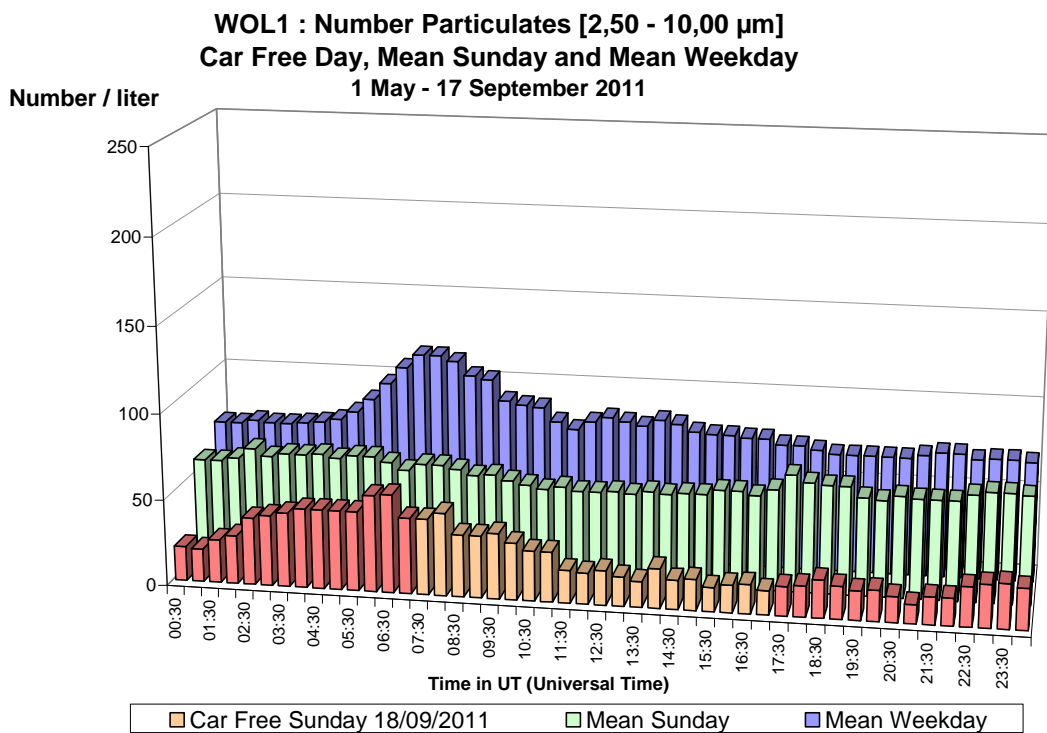
Fig. 57 : St.-Lambr.-Woluwe – Aantal Deeltjes tussen 2,50 en 10 µm – Dagprofiel van de autoluwe zondag van 18-09-2011 en van een gemiddelde zondag en werkdag (mei – september 2011).
