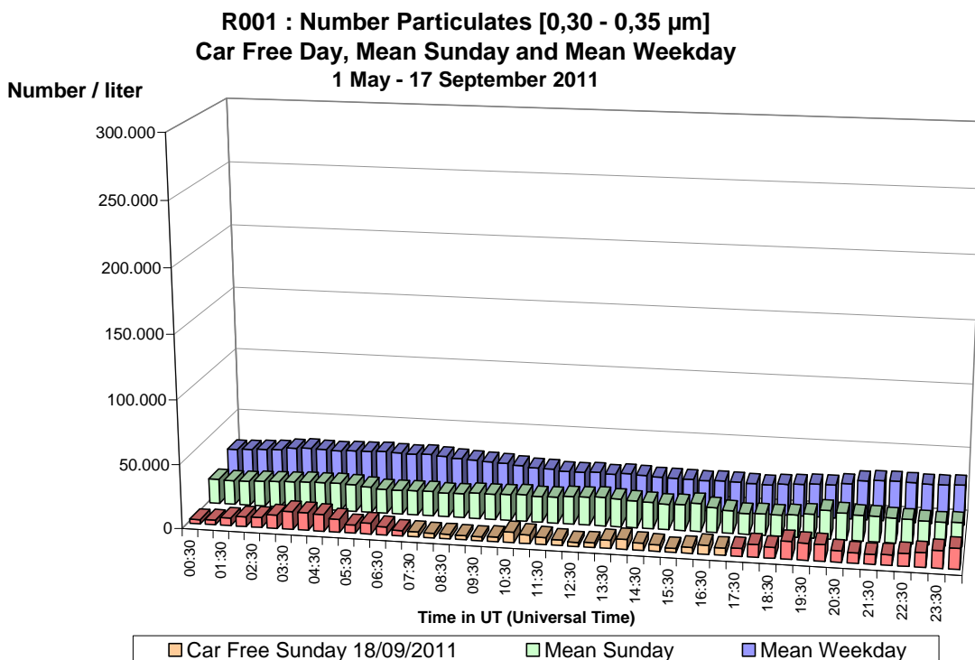
Fig. 67 Molenbeek – Aantal Deeltjes tussen 0,30 en 0,35 \mu\text{m} – Dagprofiel van de autoluwe zondag van 18-09-2011 en van een gemiddelde zondag en werkdag (mei – september 2011)
