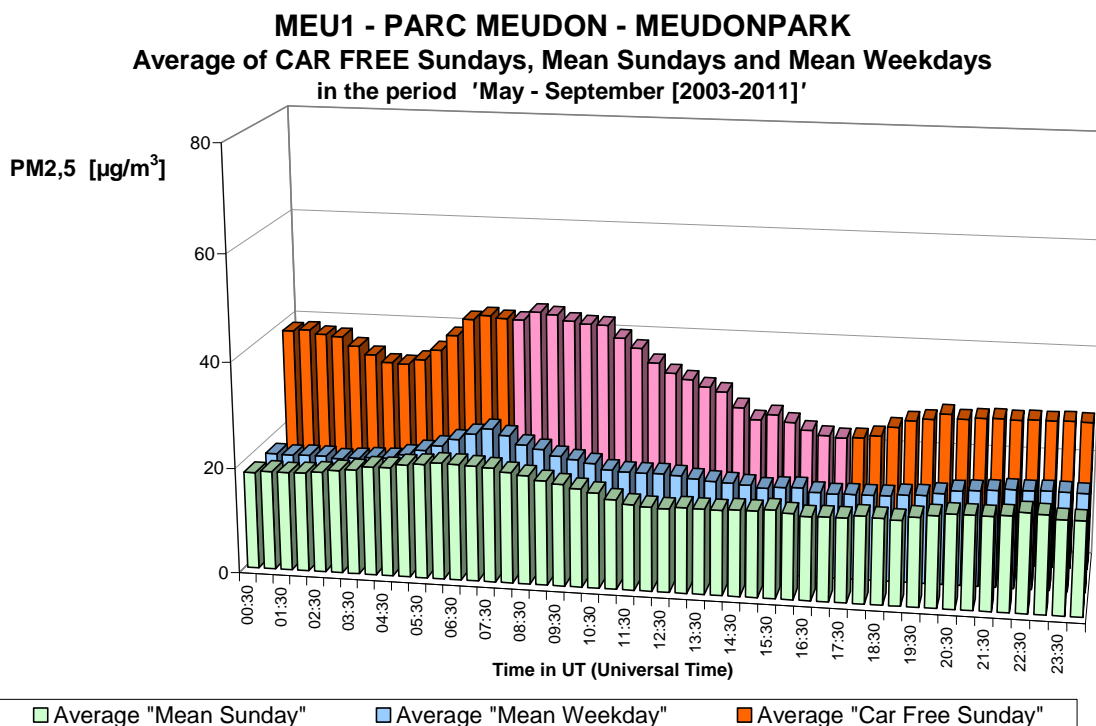
Fig. 40.b : PM2,5 in het Meudonpark – Gemiddelde Dagprofiel van alle zondagen, van alle werkdagen en van de negen autoluwe zondagen in de periodes “mei – september 2003-2011”.
