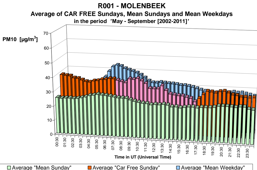
Fig. 30.b : PM10 te Molenbeek – Gemiddelde Dagprofiel van alle zondagen, van de tien autoluwe zondagen en van alle werkdagen in de periodes “mei – september 2002-2011”.
