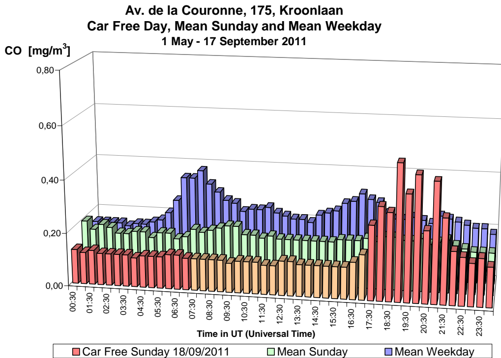
Fig. 24.a : CO in de Kroonlaan te Elsene – Dagprofiel autoluwe zondag 18-09-2011, gemiddelde zondag en gemiddelde werkdag in de periode “mei – september 2011”.
