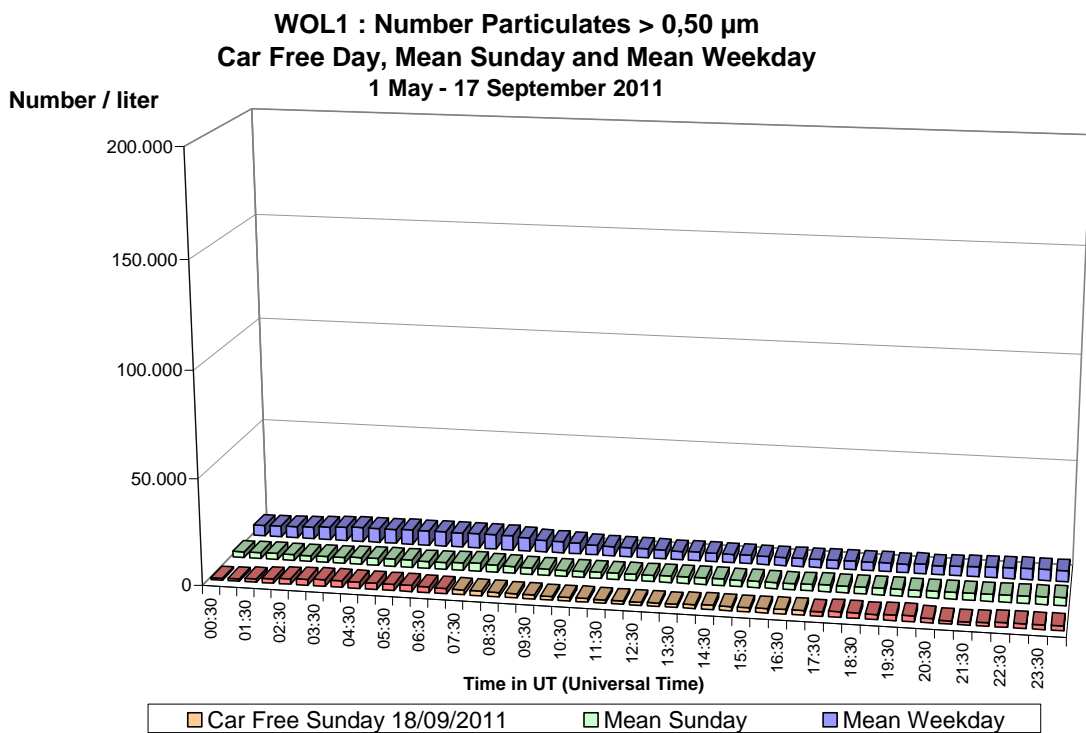
Fig. 47 : St.-Lambr.-Woluwe – Aantal Deeltjes > 0,50 µm – Dagprofiel van de autoluwe zondag van 18-09-2011 en van een gemiddelde zondag en een gemiddelde werkdag (mei – september 2011)
