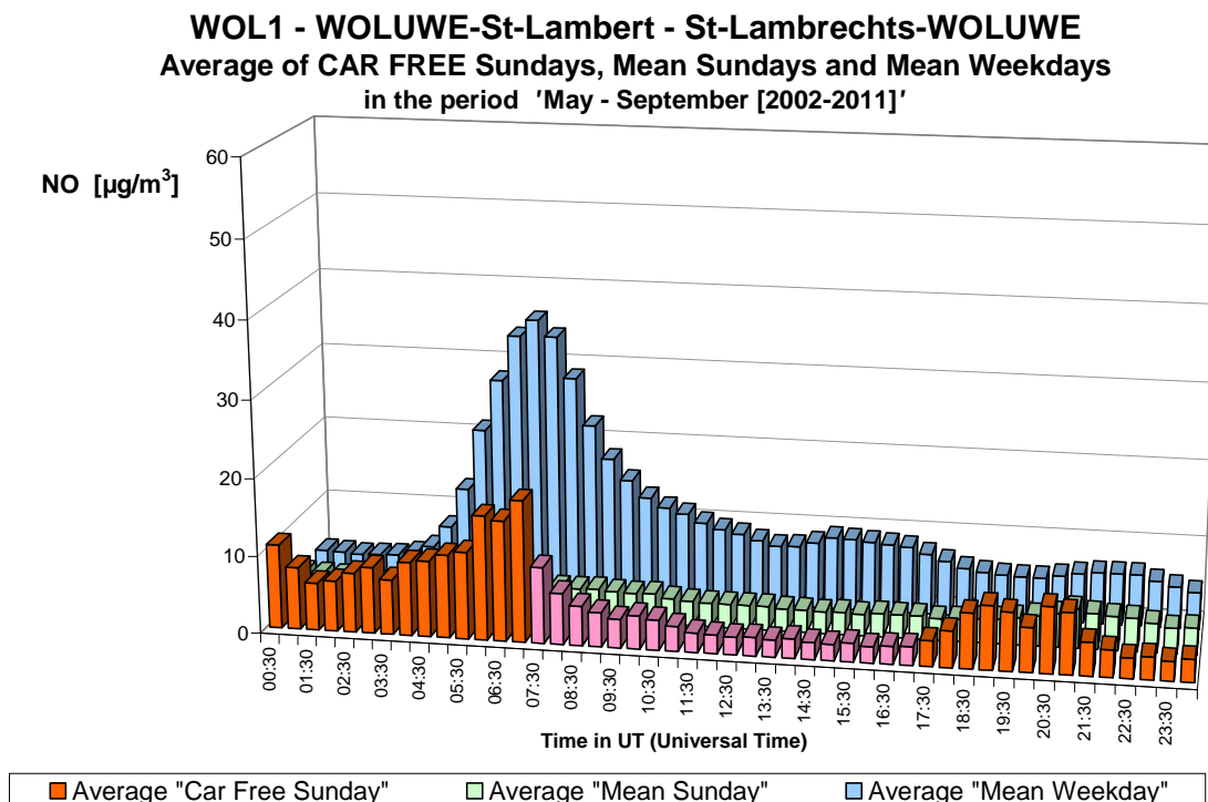
Fig. 16.b : NO te St.-Lambr.-Woluwe – Gemiddelde Dagprofiel van de tien autoluwe zondagen en van alle zondagen en werkdagen in de periodes “mei – september 2002-2011”.
