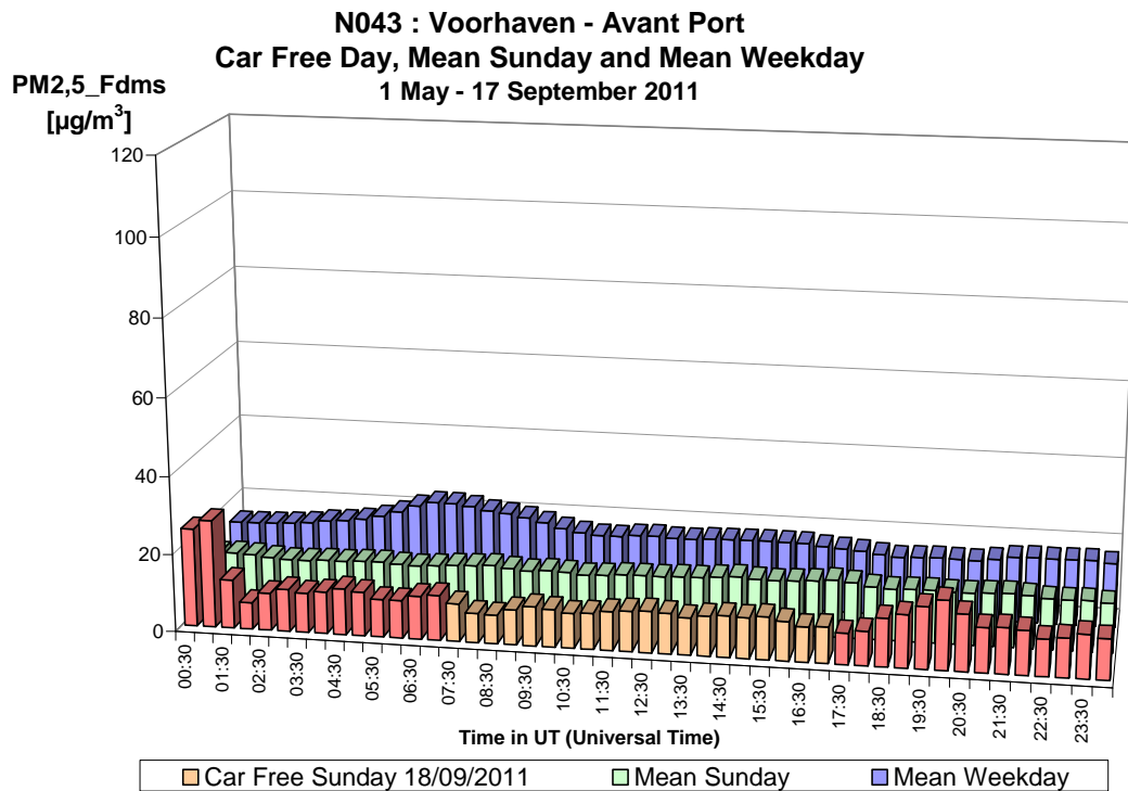
Fig. 39.a : PM2,5 in de Voorhaven – Dagprofiel van de autoluwe zondag 18-09-2011, van een gemiddelde zondag en een gemiddelde werkdag in de periode “mei – september 2011”.
