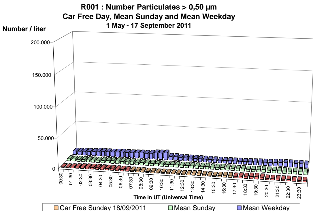
Fig. 61 : Molenbeek – Aantal Deeltjes > 0,50 µm – Dagprofiel van de autoluwe zondag van 18-09-2011 en van een gemiddelde zondag en een gemiddelde werkdag (mei – september 2011)
