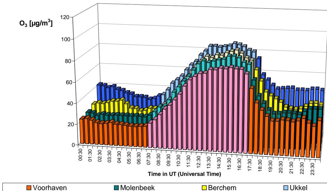
Fig. 23.a: Gemiddelde over tien autoluwe zondagen – Dagprofiel voor O 3 Situatie in 4 verschillende meetposten: Voorhaven, Molenbeek, Berchem en Ukkel
