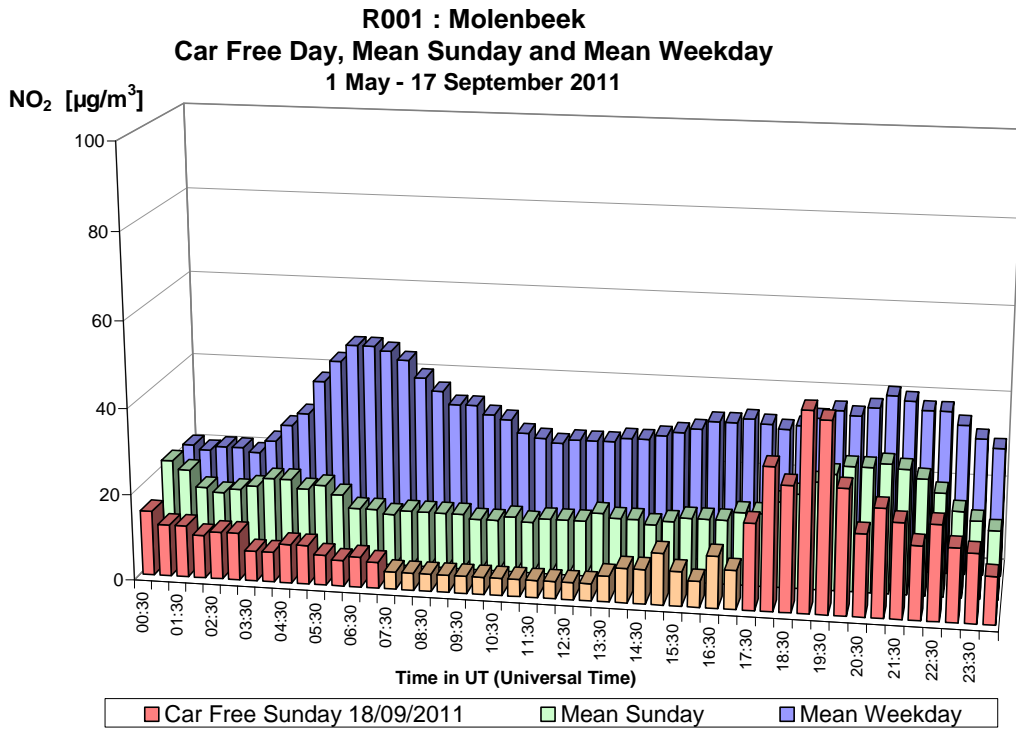
Fig. 13.a : NO 2 te Molenbeek – Dagprofiel autoluwe zondag 18-09-2011, gemiddelde zondag en gemiddelde werkdag in de periode “mei – september 2011”.
