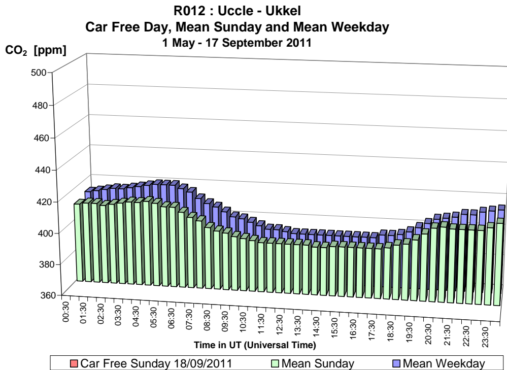
Fig. 29.a : CO 2 te Ukkel – Dagprofiel autoluwe zondag 18-09-2011, gemiddelde zondag en gemiddelde werkdag in de periode “mei – september 2011”.
