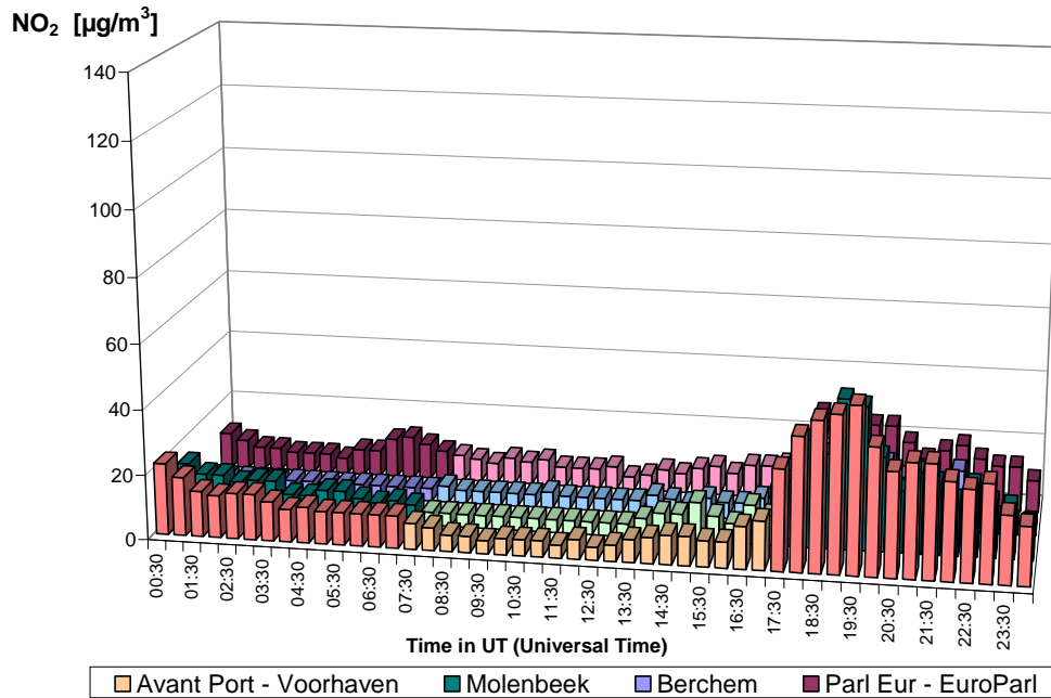
Fig. 22.b: Autoluwe zondag 18 september 2011 – Complementair dagprofiel voor NO 2 Situatie in 4 verschillende meetposten: Voorhaven, Molenbeek, Berchem en Ukkel
