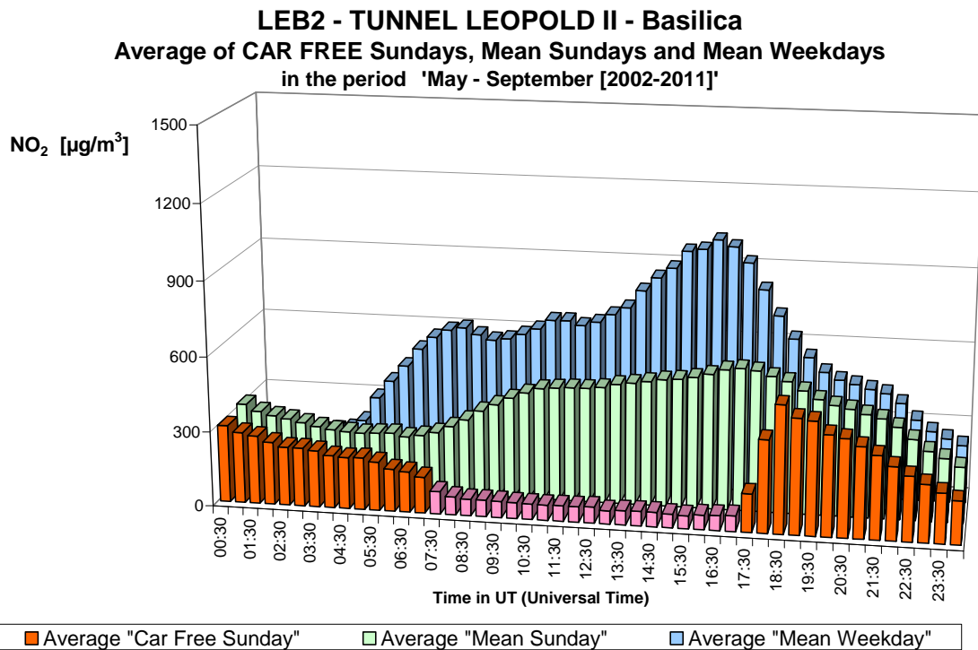
Fig. 6.b : NO 2 in de Leopold II tunnel, richting Basiliek – Gemiddelde Dagprofiel van de tien autoluwe zondagen en van alle zondagen en werkdagen in de periodes “mei – september 2002-2011”.
