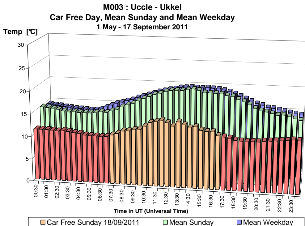
Fig. 9.b : Temperatuur – Dagprofiel autoluwe zondag 18-09-2011, gemiddelde zondag en gemiddelde werkdag in de periode “mei – september 2011”.
