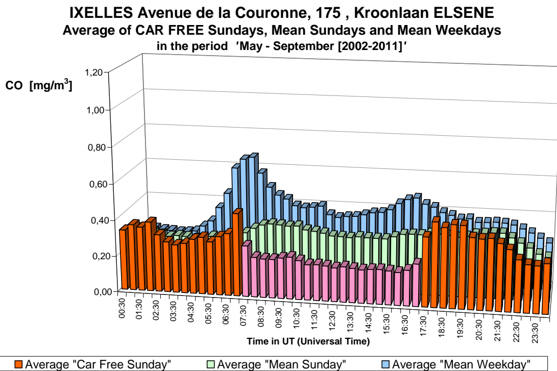
Fig. 24.b : CO in de Kroonlaan te Elsene – Gemiddelde Dagprofiel van de tien autoluwe zondagen en van alle zondagen en werkdagen in de periodes “mei – september 2002-2011”.
