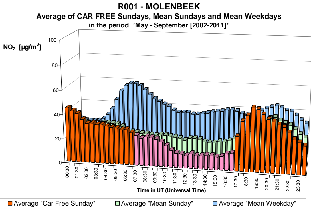
Fig. 13.b : NO 2 te Molenbeek – Gemiddelde Dagprofiel van de tien autoluwe zondagen en van alle zondagen en de werkdagen in de periodes “mei – september 2002-2011”.
