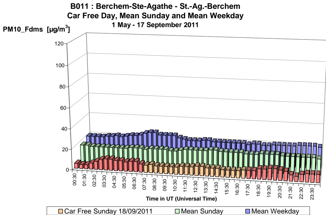
Fig. 31.a : PM10 te St.-Ag.-Berchem – Dagprofiel van de autoluwe zondag 18-09-2011, van een gemiddelde zondag en een gemiddelde werkdag in de periode “mei – september 2011”.
