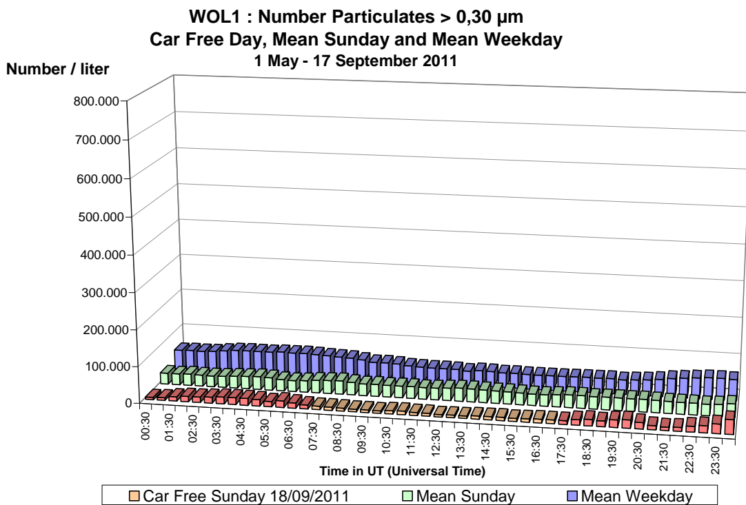
Fig. 45 : St.-Lambr.-Woluwe – Aantal Deeltjes > 0,30 µm – Dagprofiel van de autoluwe zondag van 18-09-2011 en van een gemiddelde zondag en een gemiddelde werkdag (mei – september 2011)
