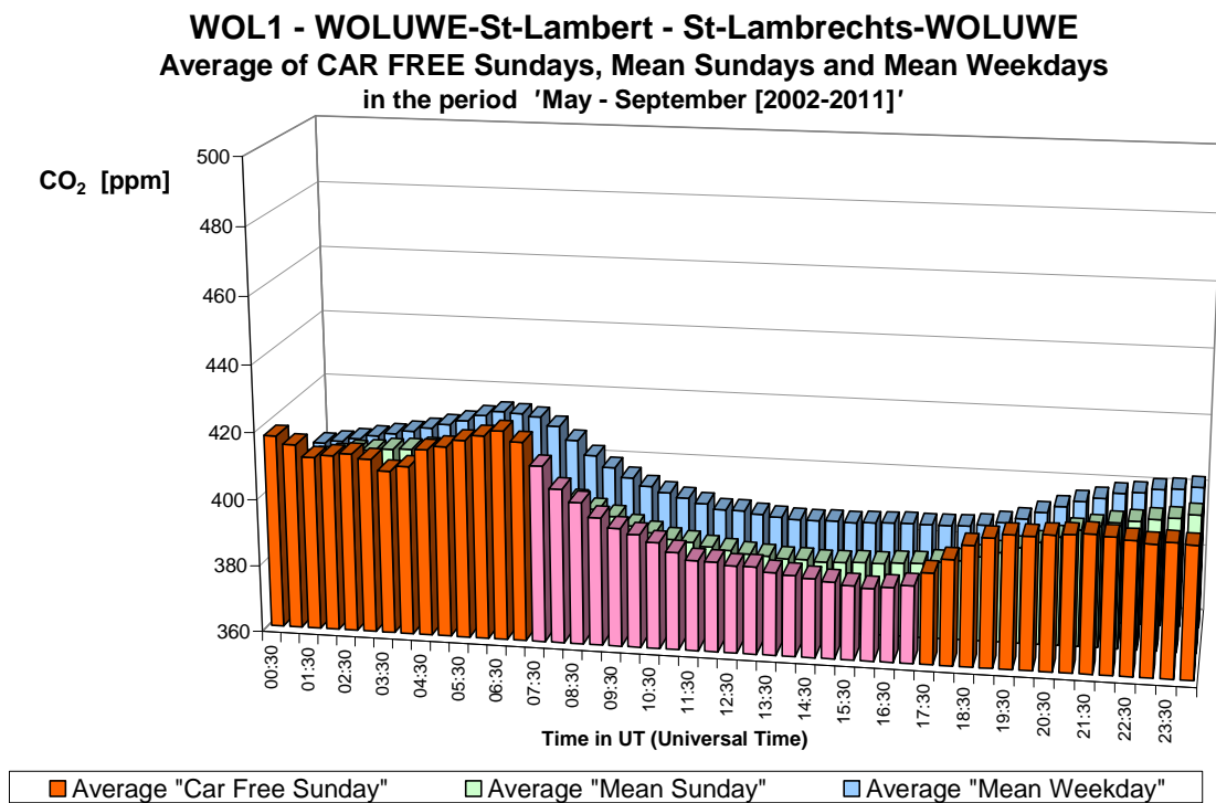
Fig. 28.b : CO 2 te St.-Lambr.-Woluwe – Gemiddelde Dagprofiel van de tien autoluwe zondagen en van alle zondagen en werkdagen in de periodes “mei – september 2002-2011”.
