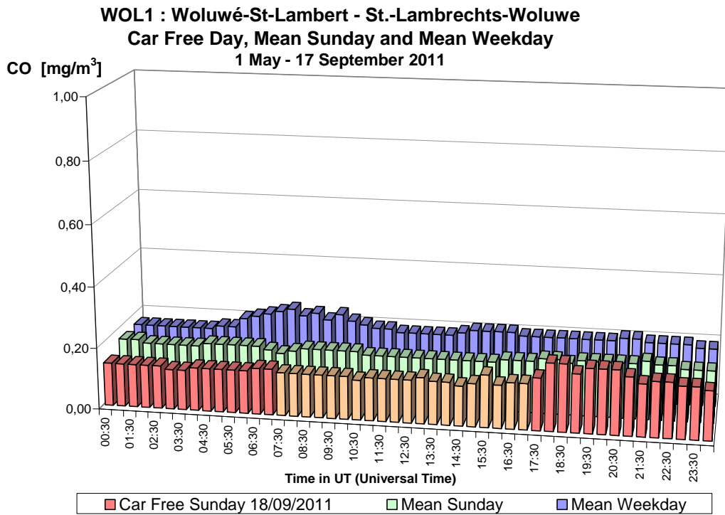
Fig. 26.a : CO te St.-Lambr.-Woluwe – Dagprofiel autoluwe zondag 18-09-2011, gemiddelde zondag en gemiddelde werkdag in de periode “mei – september 2011”.
