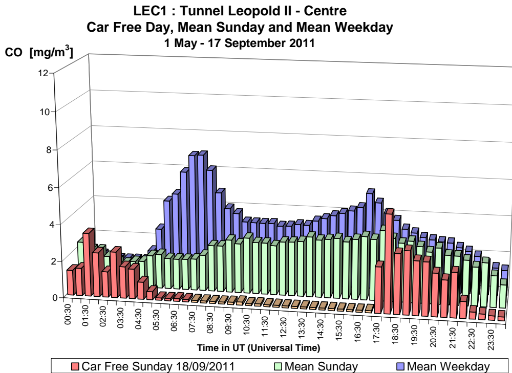
Fig. 4.a : CO in de Leopold II tunnel, richting Centrum – Dagprofiel autoluwe zondag 18-09-2011, gemiddelde zondag en gemiddelde werkdag in de periode “mei – september 2011”.
