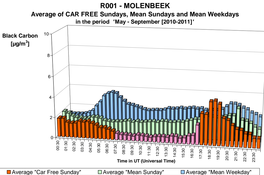
Fig. 41.b : Black Carbon te Molenbeek – Gemiddelde Dagprofiel van de twee autoluwe zondagen en van alle zondagen en alle werkdagen in de periodes “mei – september 2010-2011”.
