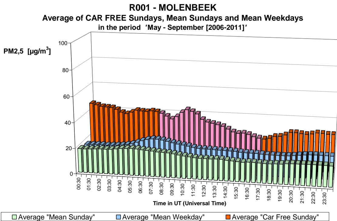
Fig. 36.b : PM2,5 te Molenbeek – Gemiddelde Dagprofiel van alle zondagen, van alle werkdagen en van de zes autoluwe zondagen in de periodes “mei – september 2006-2011”.
