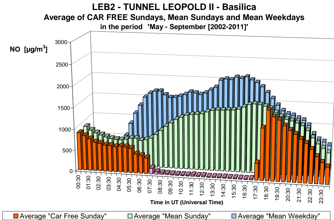
Fig. 5.b : NO in de Leopold II tunnel, richting Basiliek – Gemiddelde Dagprofiel van de tien autoluwe zondagen en van alle zondagen en werkdagen in de periodes “mei – september 2002-2011”.
