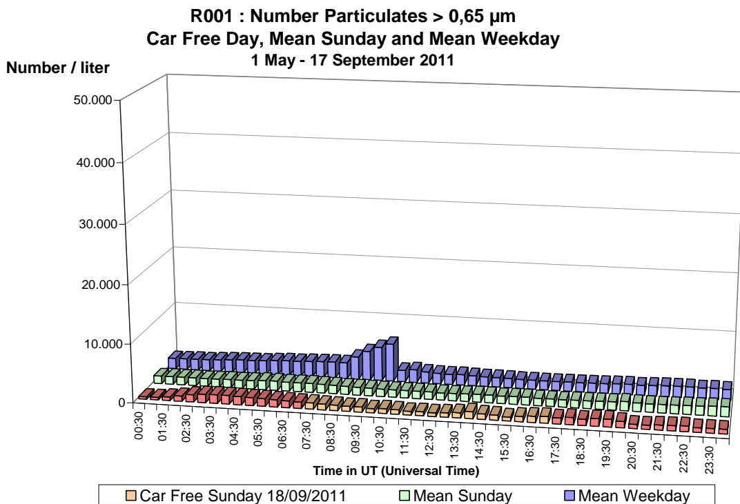
Fig. 62 Molenbeek – Aantal Deeltjes > 0,65 \mu\text{m} – Dagprofiel van de autoluwe zondag van 18-09-2011 en van een gemiddelde zondag en een gemiddelde werkdag (mei – september 2011)
