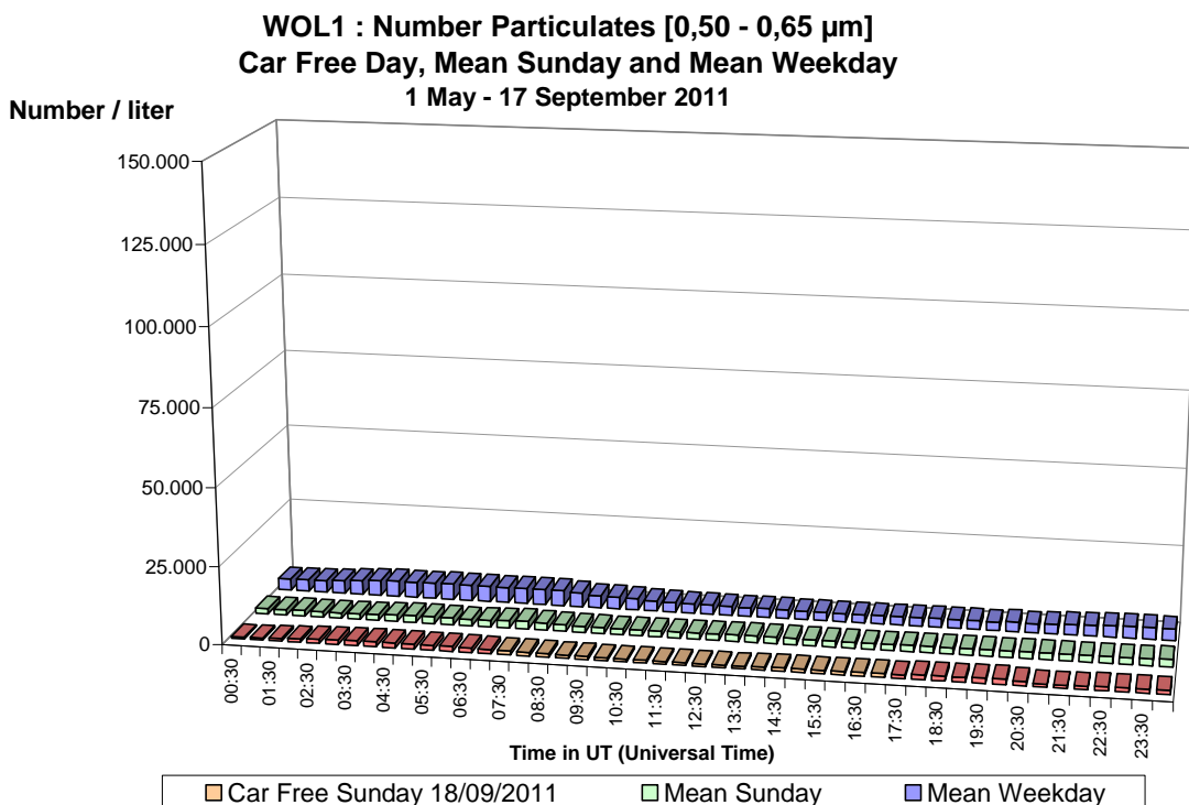
Fig. 55 : St.-Lambr.-Woluwe – Aantal Deeltjes tussen 0,50 en 0,65 µm – Dagprofiel van de autoluwe zondag van 18-09-2011 en van een gemiddelde zondag en werkdag (mei – september 2011)
