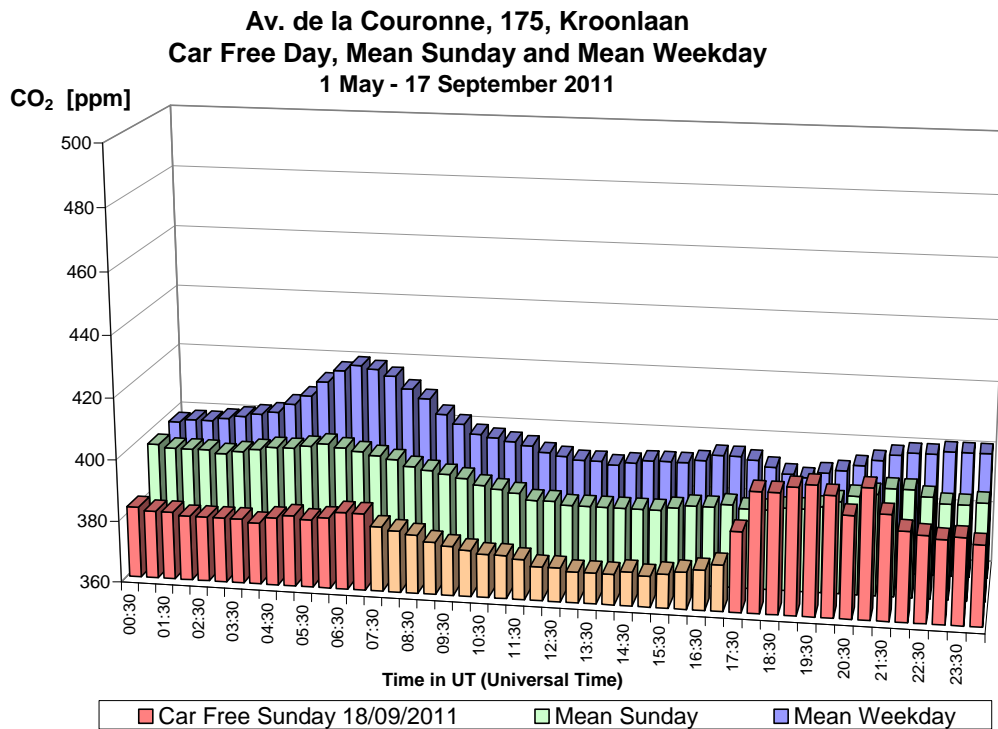
Fig. 27.a : CO 2 in de Kroonlaan te Elsene – Dagprofiel autoluwe zondag 18-09-2011, gemiddelde zondag en gemiddelde werkdag in de periode “mei – september 2011”.
