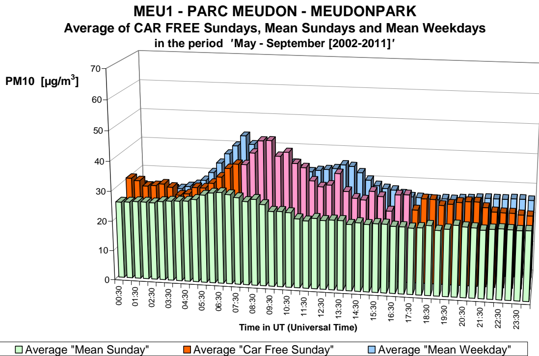
Fig. 34.b : PM10 in het Meudonpark – Gemiddelde Dagprofiel van alle zondagen, van de tien autoluwe zondagen en van alle werkdagen in de periodes “mei – september 2002-2011”.
