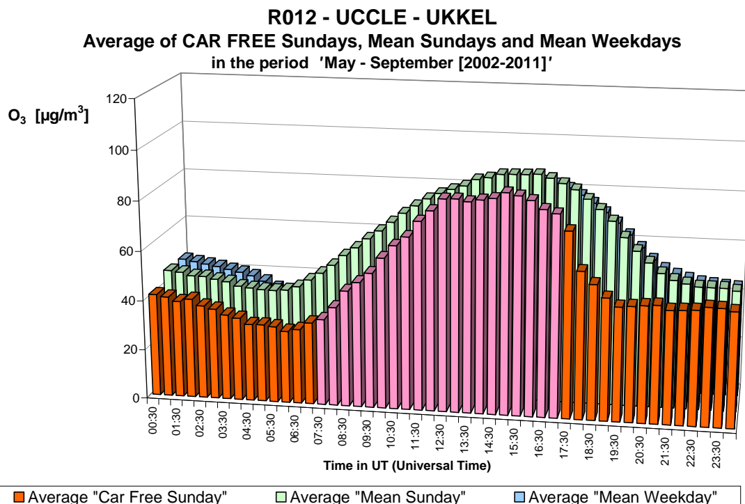
Fig. 19.b : O 3 te Ukkel – Gemiddelde Dagprofiel van de tien autoluwe zondagen en van alle zondagen en werkdagen in de periodes “mei – september 2002-2011”.
