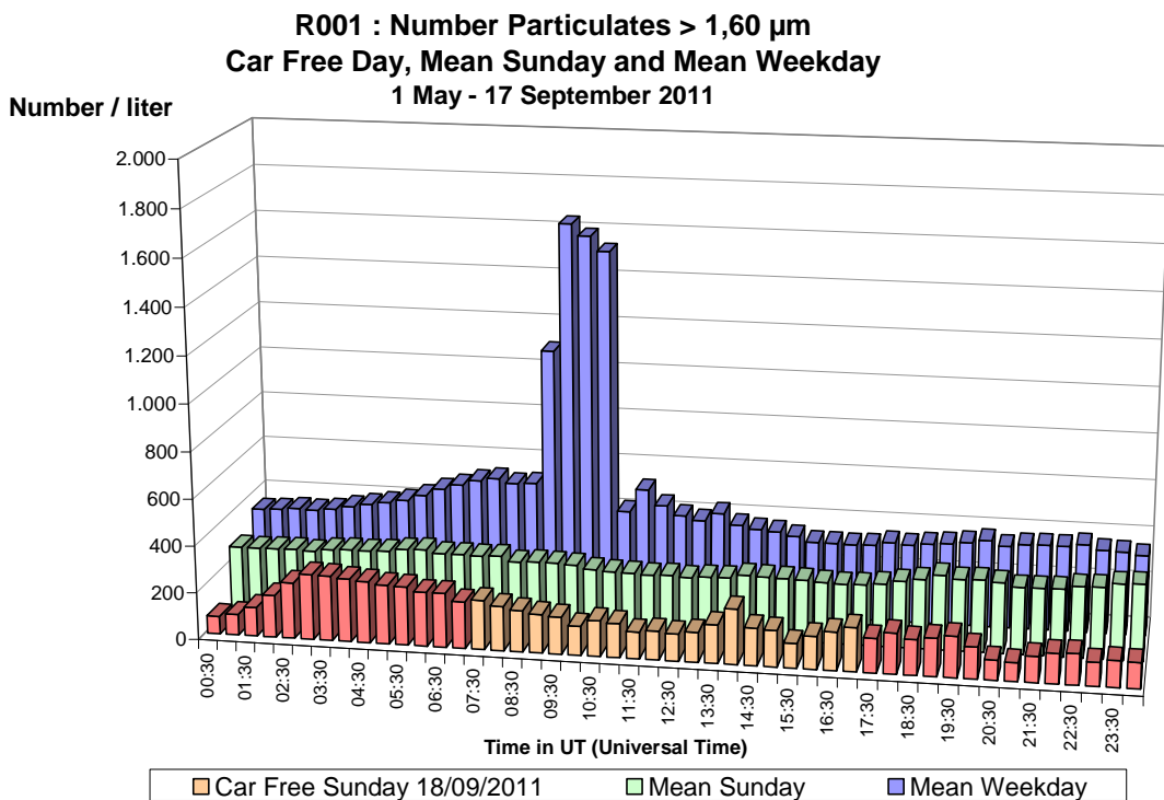
Fig. 64 Molenbeek – Aantal Deeltjes > 1,60 \mu\text{m} – Dagprofiel van de autoluwe zondag van 18-09-2011 en van een gemiddelde zondag en werkdag (mei – september 2011).
