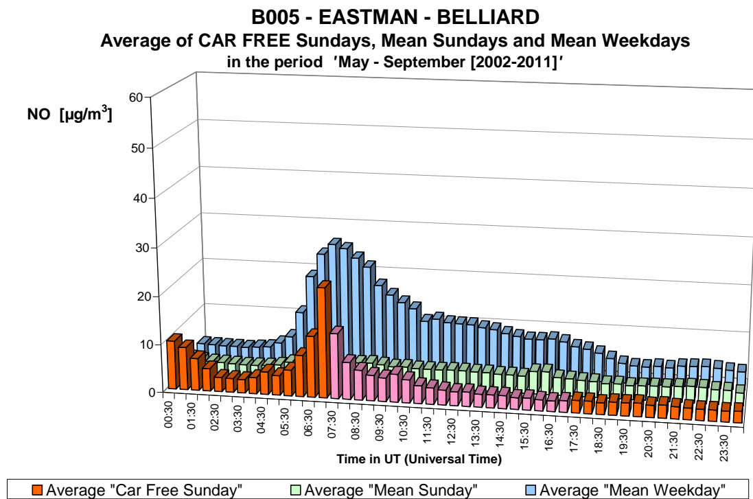
Fig. 14.b : NO in de meetpost Eastman-Belliard – Gemiddelde Dagprofiel van de tien autoluwe zondagen en van alle zondagen en werkdagen in de periodes “mei – september 2002-2011”.
