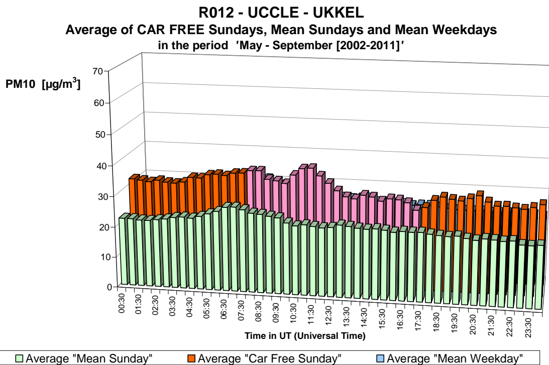
Fig. 32.b : PM10 te Ukkel – Gemiddelde Dagprofiel van alle zondagen, van de tien autoluwe zondagen en van alle werkdagen in de periodes “mei – september 2002-2011”.
