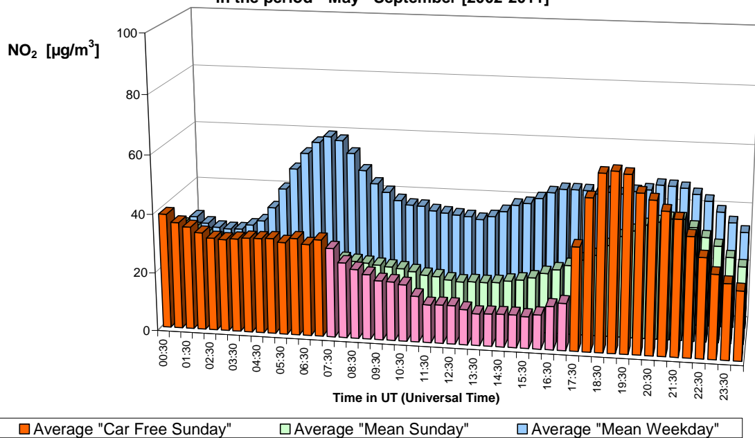
Fig. 17.b : NO 2 te St.-Lambr.-Woluwe – Gemiddelde Dagprofiel van de tien autoluwe zondagen en van alle zondagen en werkdagen in de periodes “mei – september 2002-2011”.
