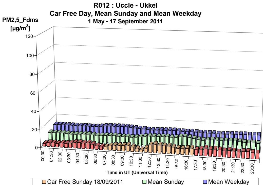
Fig. 38.a : PM 2,5 te Ukkel – Dagprofiel van de autoluwe zondag 18-09-2011, van een gemiddelde zondag en een gemiddelde werkdag in de periode “mei – september 2011”.
