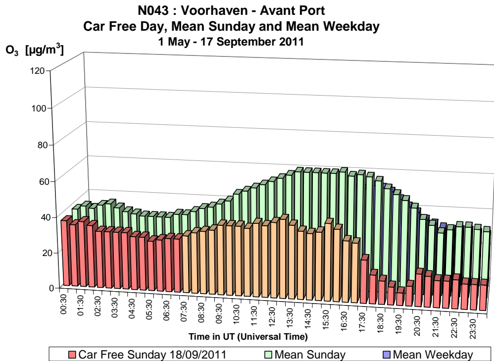
Fig. 21.a : O 3 in de Voorhaven – Dagprofiel autoluwe zondag 18-09-2011, gemiddelde zondag en gemiddelde werkdag in de periode “mei – september 2011”.
