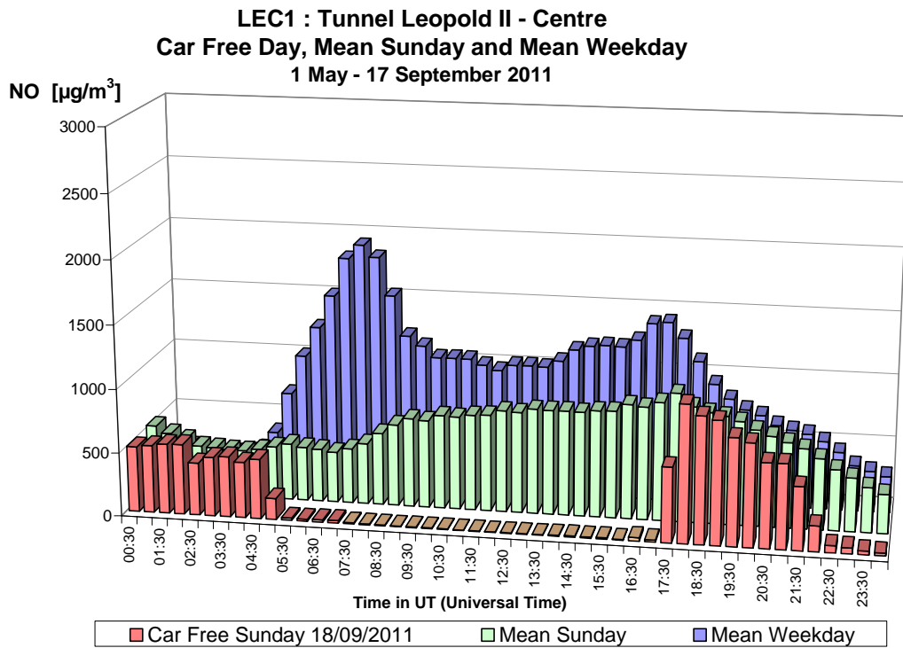
Fig. 1.a : NO in de Leopold II tunnel, richting Centrum – Dagprofiel autoluwe zondag 18-09-2011, gemiddelde zondag en gemiddelde werkdag in de periode “mei – september 2011”.
