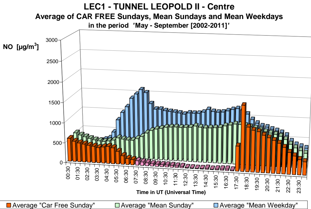
Fig. 1.b : NO in de Leopold II tunnel, richting Centrum – Gemiddelde Dagprofiel van de tien autoluwe zondagen en van alle zondagen en werkdagen in de periodes “mei – september 2002-2011”.
