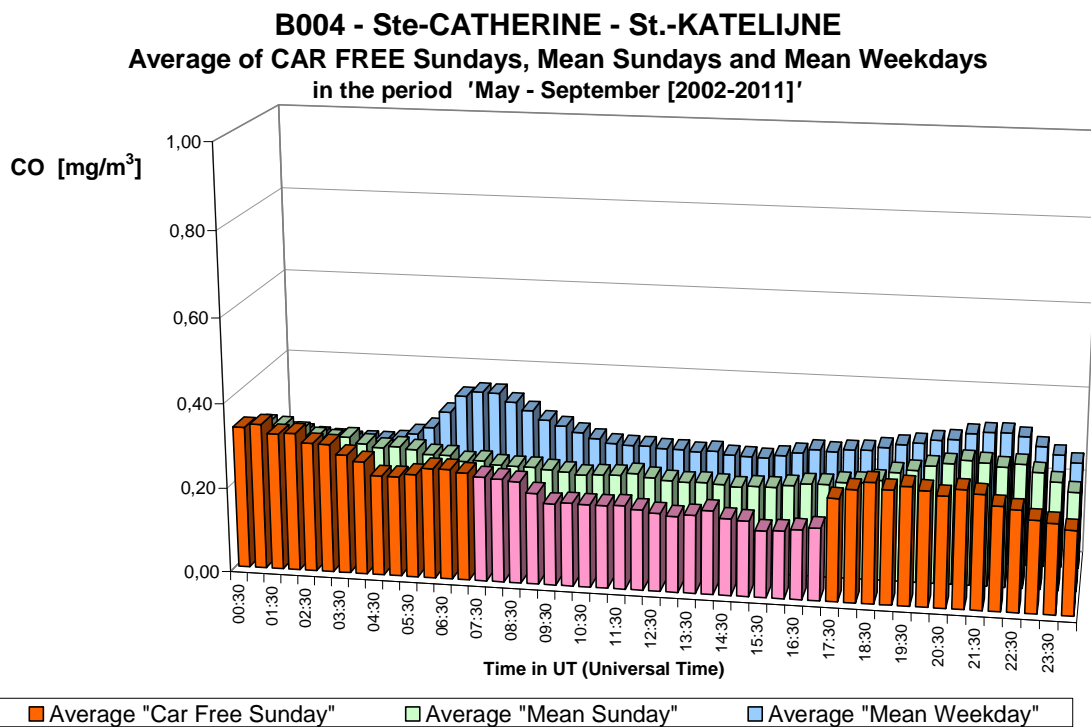
Fig. 25.b : CO in de meetpost St.-Katelijne – Gemiddelde Dagprofiel van de tien autoluwe zondagen en van alle zondagen en werkdagen in de periodes “mei – september 2002-2011”.
