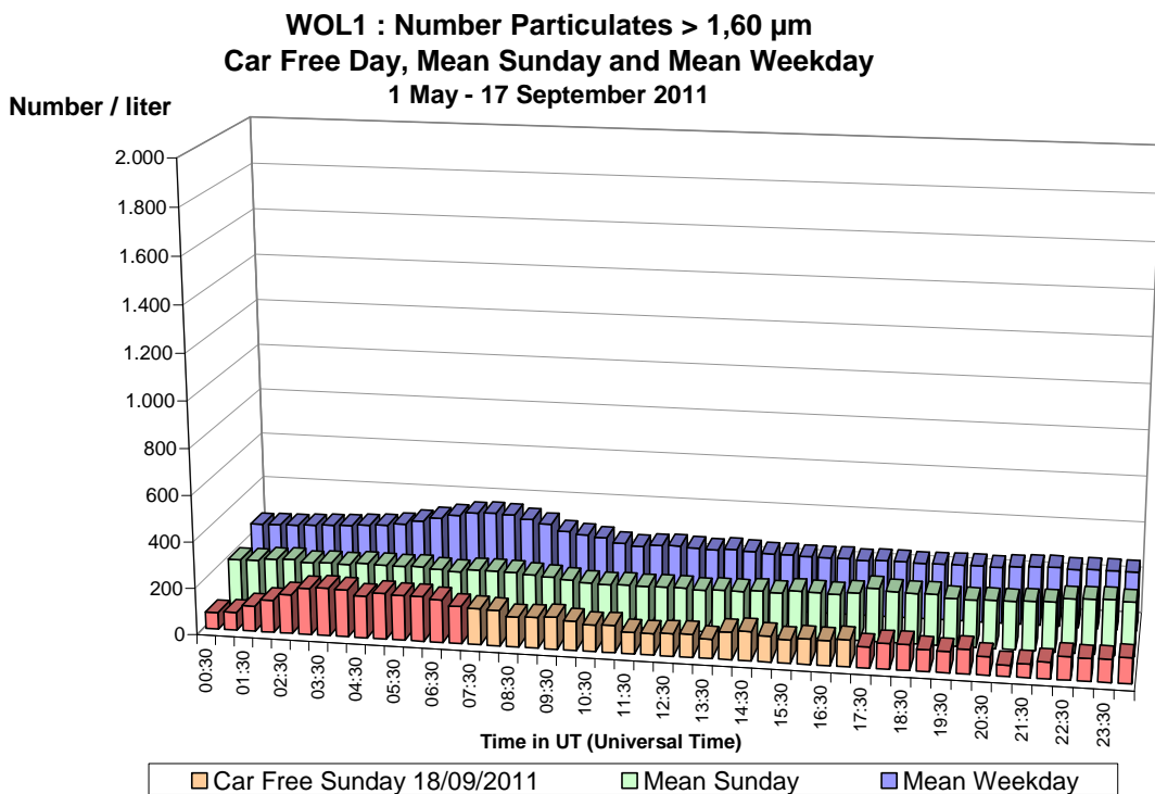
Fig. 50 : St.-Lambr.-Woluwe – Aantal Deeltjes > 1,60 µm – Dagprofiel van de autoluwe zondag van 18-09-2011 en van een gemiddelde zondag en werkdag (mei – september 2011).
