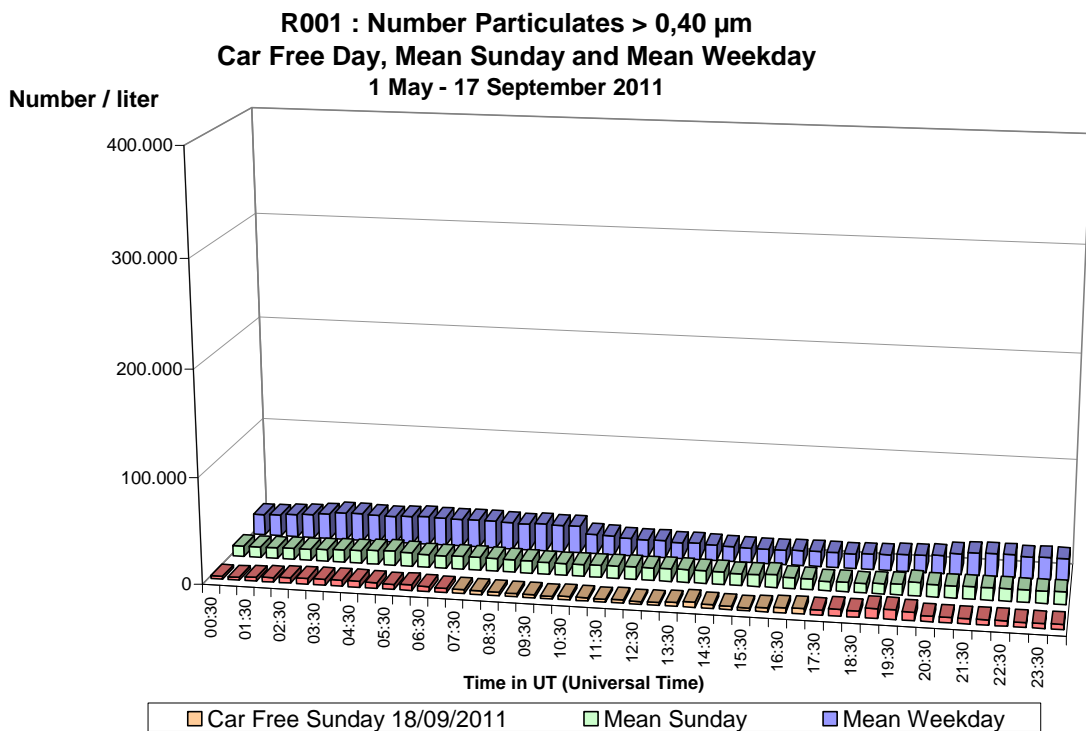
Fig. 60 : Molenbeek – Aantal Deeltjes > 0,40 µm – Dagprofiel van de autoluwe zondag van 18-09-2011 en van een gemiddelde zondag en een gemiddelde werkdag (mei – september 2011)
