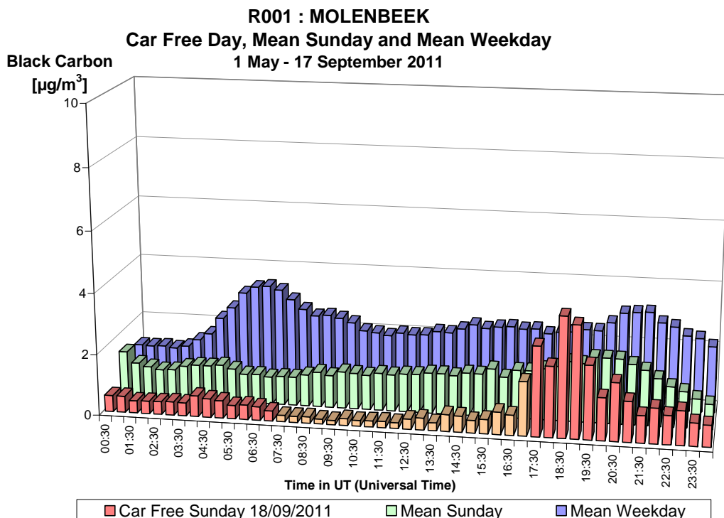
Fig. 41.a : Black Carbon te Molenbeek – Dagprofiel van de autoluwe zondag 18-09-2011, een gemiddelde zondag en een gemiddelde werkdag in de periode “juli – september 2011”
