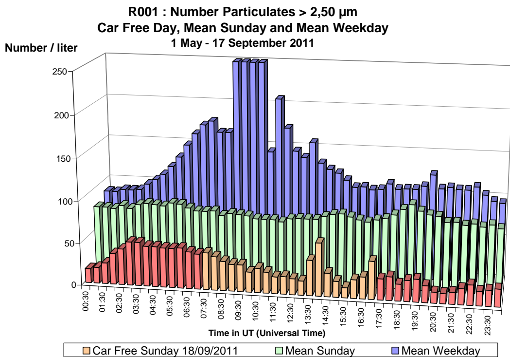
Fig. 65 Molenbeek – Aantal Deeltjes > 2,50 \mu\text{m} – Dagprofiel van de autoluwe zondag van 18-09-2011 en van een gemiddelde zondag en werkdag (mei – september 2011).
