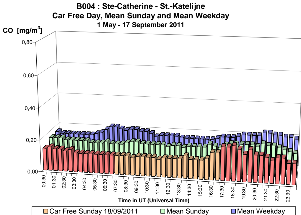
Fig. 25.a : CO in de meetpost St.-Katelijne – Dagprofiel autoluwe zondag 18-09-2011, gemiddelde zondag en gemiddelde werkdag in de periode “mei – september 2011”.
