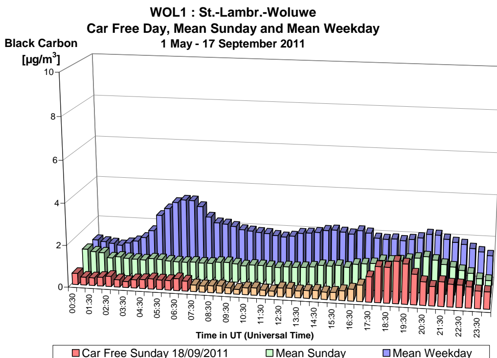
Fig. 43.a : Black Carbon te Woluwe – Dagprofiel van de autoluwe zondag 18-09-2011, een gemiddelde zondag en een gemiddelde werkdag in de periode “juli – september 2011”
