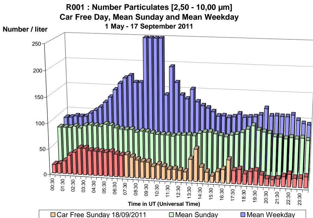
Fig. 71 Molenbeek – Aantal Deeltjes tussen 2,50 en 10 \mu\text{m} – Dagprofiel van de autoluwe zondag van 18-09-2011 en van een gemiddelde zondag en werkdag (mei – september 2011).
