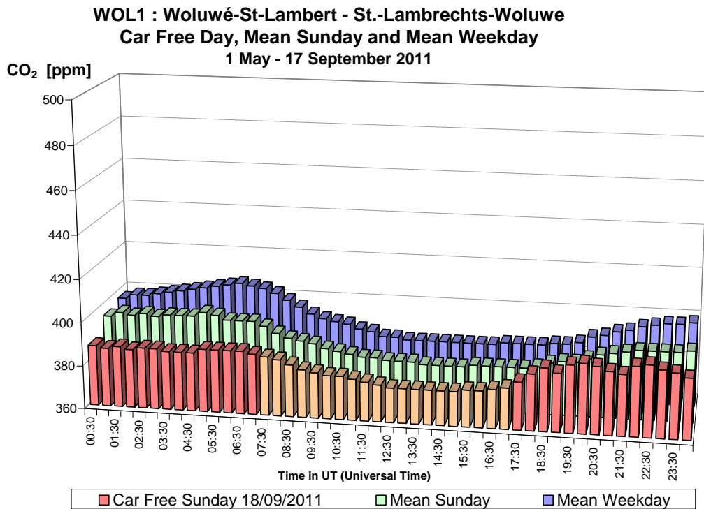
Fig. 28.a : CO 2 te St.-Lambr.-Woluwe – Dagprofiel autoluwe zondag 18-09-2011, gemiddelde zondag en gemiddelde werkdag in de periode “mei – september 2011”.
