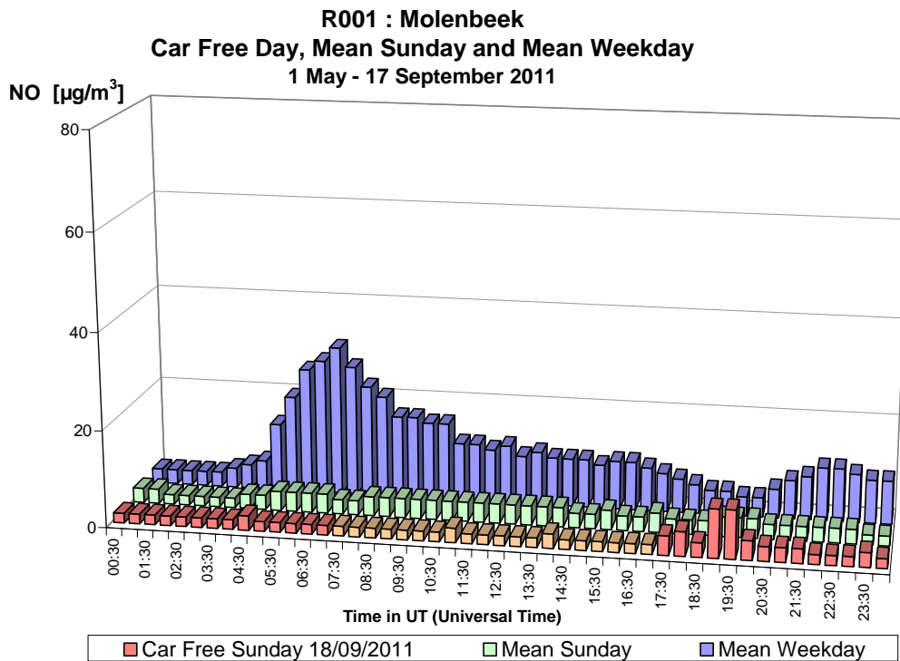
Fig. 12.a : NO te Molenbeek – Dagprofiel autoluwe zondag 18-09-2011, gemiddelde zondag en gemiddelde werkdag in de periode “mei – september 2011”.
