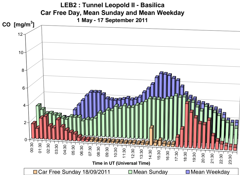
Fig. 8.a : CO in de Leopold II tunnel, richting Basiliek – Dagprofiel autoluwe zondag 18-09-2011, gemiddelde zondag en gemiddelde werkdag in de periode “mei – september 2011”.
