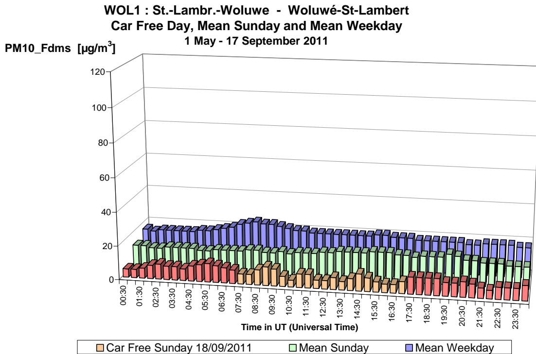
Fig. 35.a : PM10 te St.-Lambr.-Woluwe – Dagprofiel van de autoluwe zondag 18-09-2011, van een gemiddelde zondag en een gemiddelde werkdag in de periode “mei – september 2011”.
