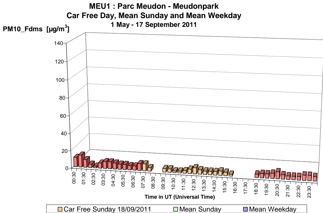
Fig. 34.a : PM10 in het Meudonpark – Dagprofiel van de autoluwe zondag 18-09-2011, van een gemiddelde zondag en een gemiddelde werkdag in de periode “mei – september 2011”.
