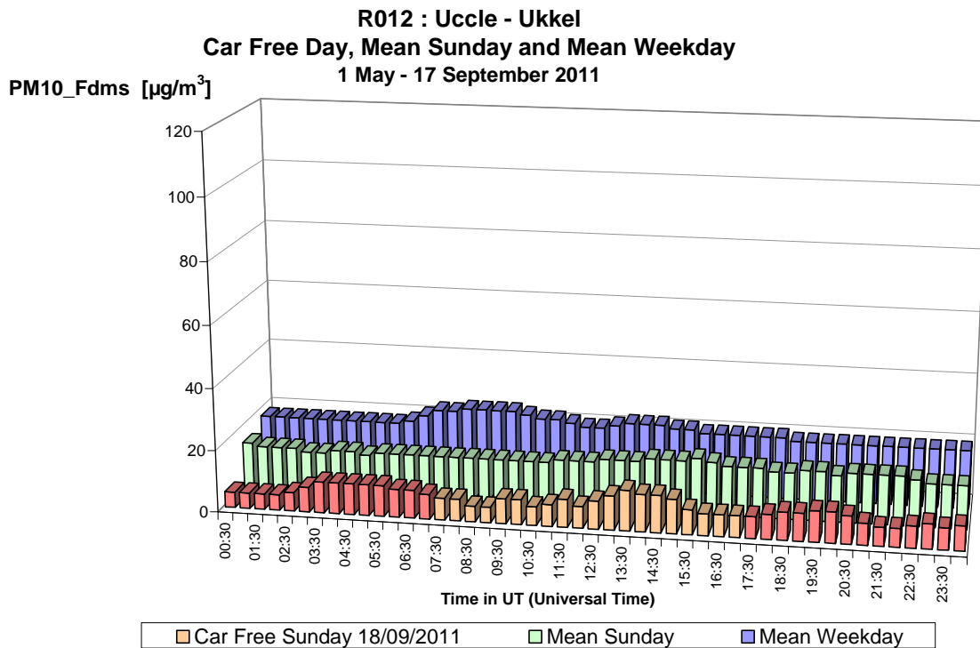
Fig. 32.a : PM10 te Ukkel – Dagprofiel van de autoluwe zondag 18-09-2011, van een gemiddelde zondag en een gemiddelde werkdag in de periode “mei – september 2011”.
