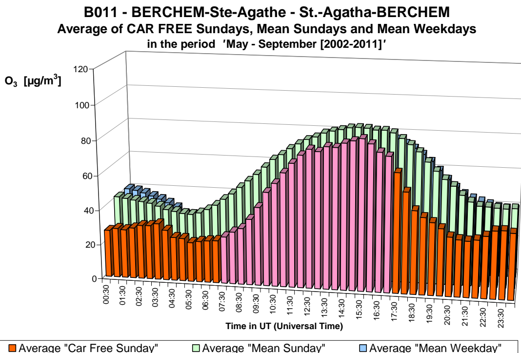
Fig. 20.b : O 3 te St.-Ag.-Berchem – Gemiddelde Dagprofiel van de tien autoluwe zondagen en van alle zondagen en werkdagen in de periodes “mei – september 2002-2011”.
