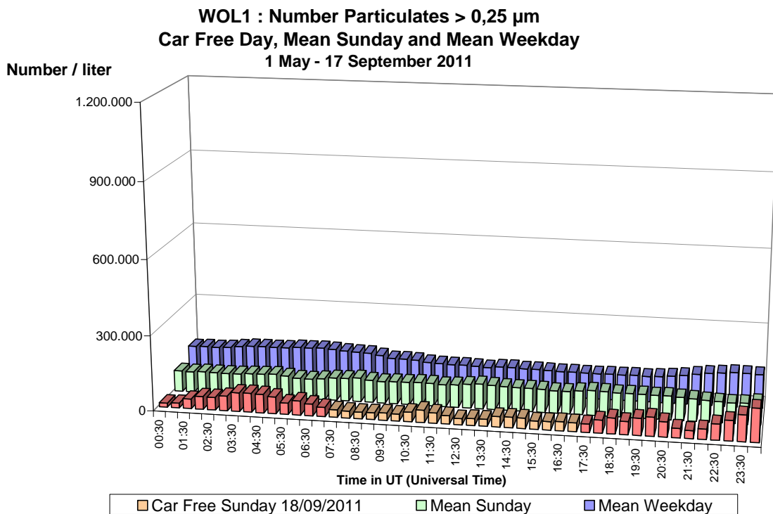
Fig. 44 : St.-Lambr.-Woluwe – Aantal Deeltjes > 0,25 µm – Dagprofiel van de autoluwe zondag van 18-09-2011 en van een gemiddelde zondag en een gemiddelde werkdag (mei – september 2011)
