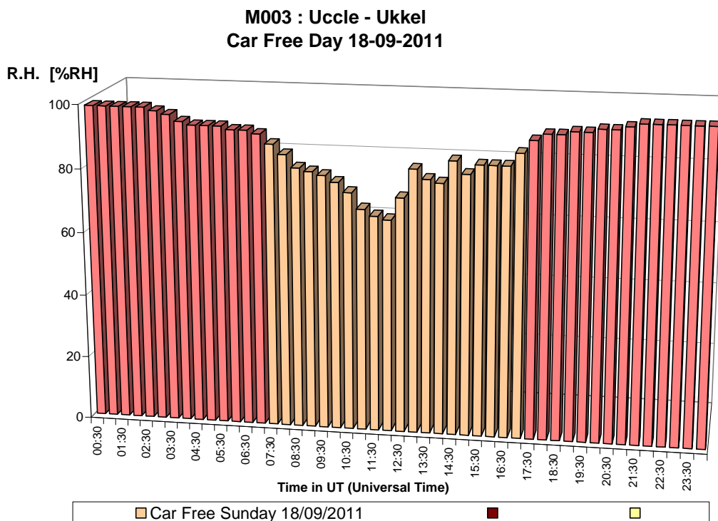
Fig. 9.c : Relatieve Vochtigheid – Dagprofiel autoluwe zondag 18-09-2011.
