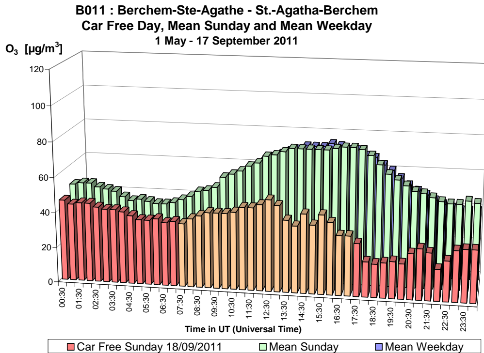
Fig. 20.a : O 3 te St.-Ag.-Berchem – Dagprofiel autoluwe zondag 18-09-2011, gemiddelde zondag en gemiddelde werkdag in de periode “mei – september 2011”.
