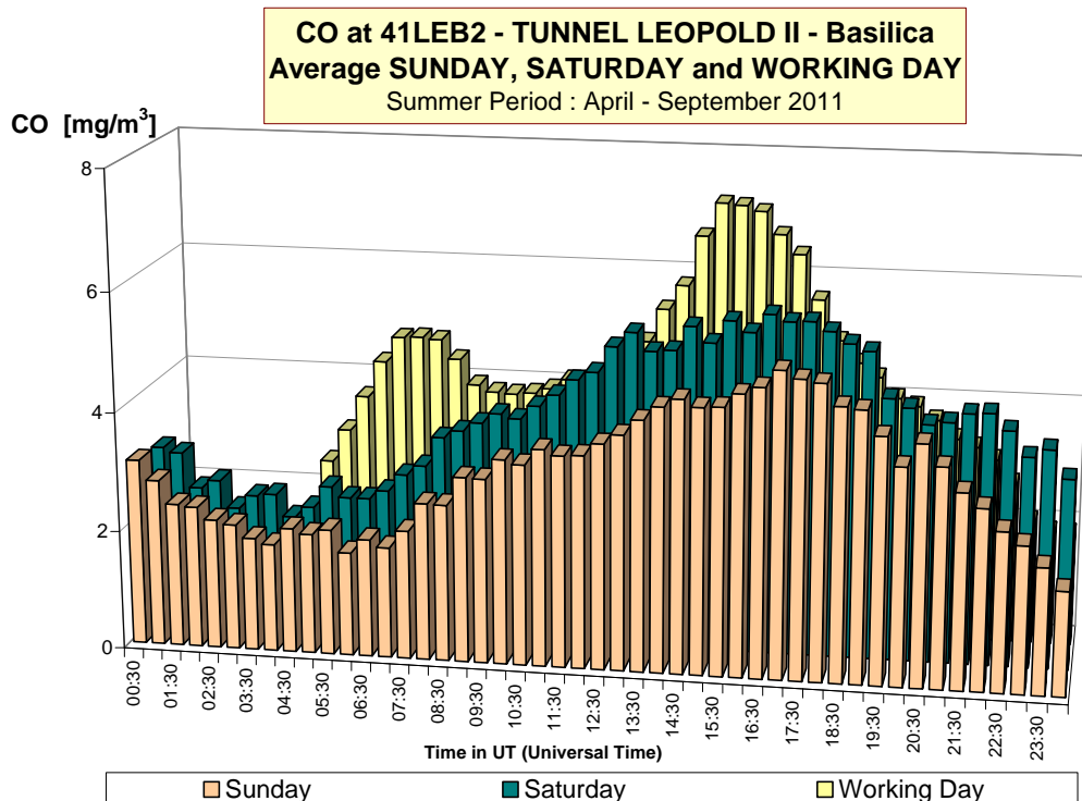
Fig. 20 : CO – évolution journalière moyenne au poste de mesure 41LEB2 (basilique) Comparaison entre un dimanche, un samedi et un jour ouvrable moyen Période hivernale 2011-2012 et période estivale 2011
