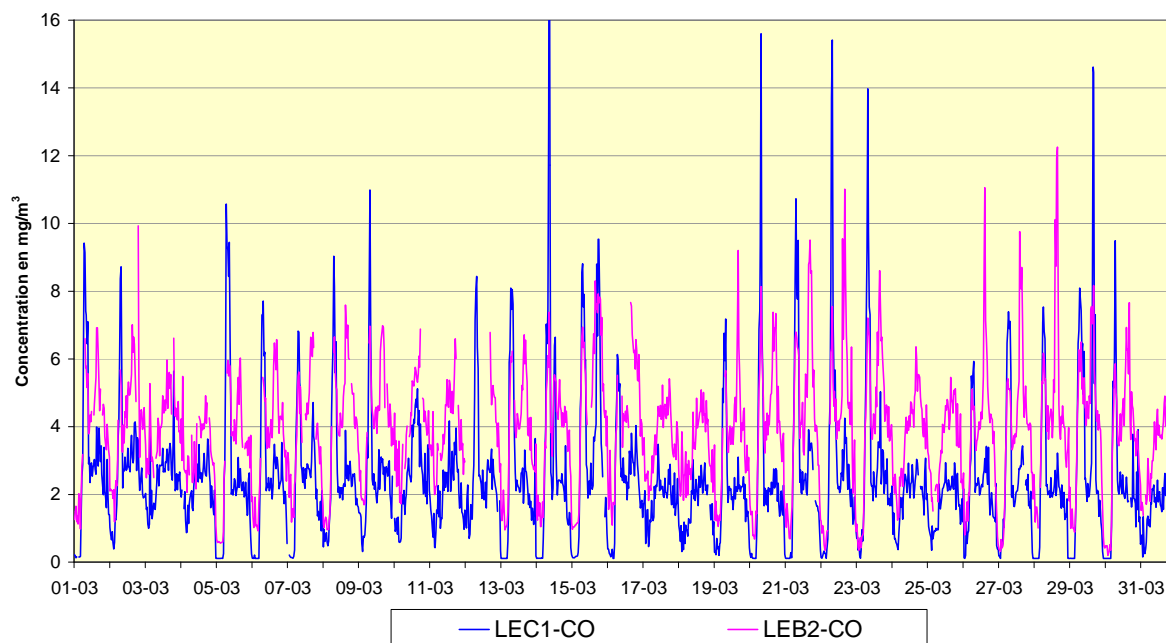
Fig. 3: CO - Évolution des valeurs horaires et semi horaires en mars 2012 Poste de mesure 41LEC1, direction Centre – Poste de mesure 41LEB2, direction Basilique
