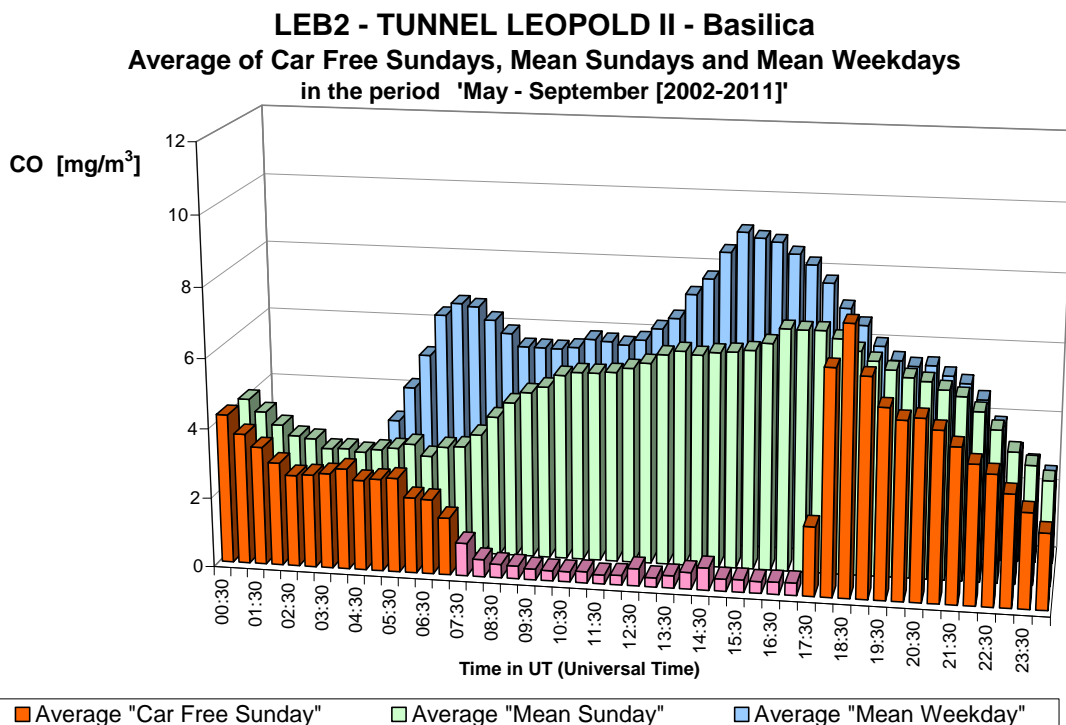
Fig. 32.b : CO dans le tunnel Léopold II, direction Basilique – Profil journalier sur les dix dimanches sans voiture et sur tous les dimanches et jours ouvrables des périodes 'mai – septembre 2002-2011'.
