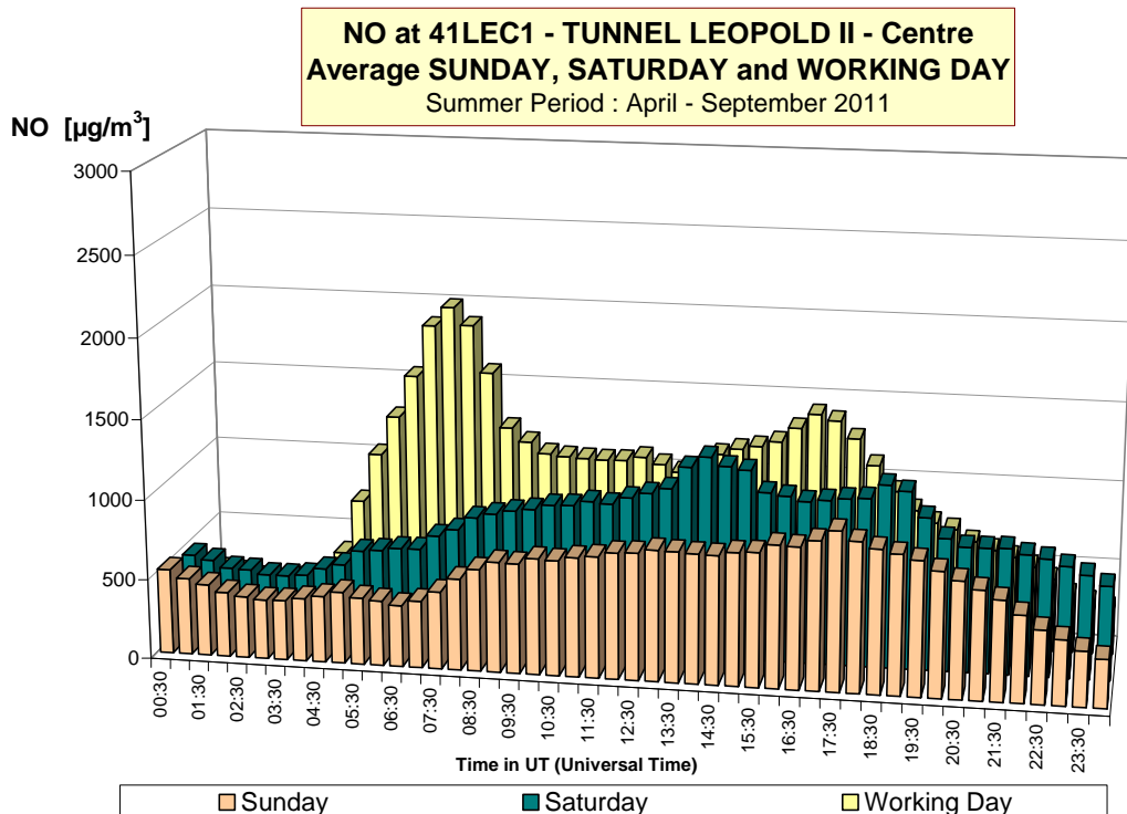
Fig. 17 : NO – évolution journalière moyenne au poste de mesure 41LEC1 (centre) Comparaison entre un dimanche, un samedi et un jour ouvrable moyen Période hivernale 2011-2012 et période estivale 2011
