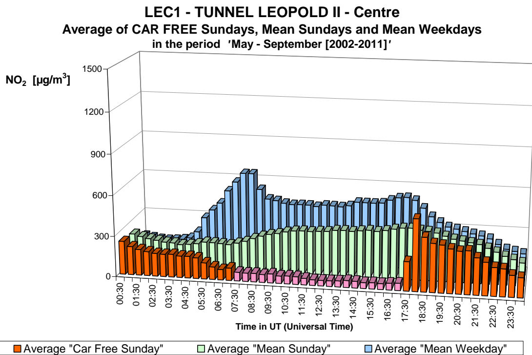
Fig. 27.b : NO 2 dans le tunnel Léopold II, direction Centre – Profil journalier sur les dix dimanches sans voiture et sur tous les dimanches et jours ouvrables des périodes 'mai – septembre 2002-2011'.
