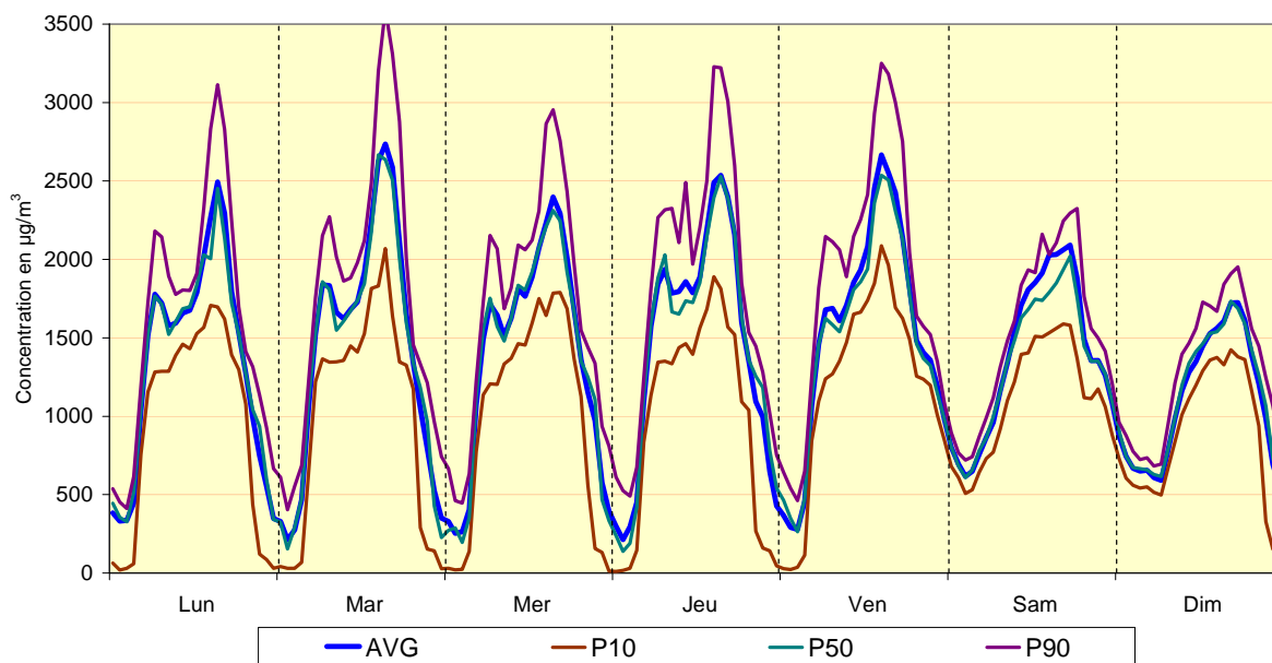
Fig. 26 : Poste de Mesure 41LEB2 (basilique) – Évolution hebdomadaire moyenne pour le NO Période hivernale 2011 - 2012 et période estivale 2011
