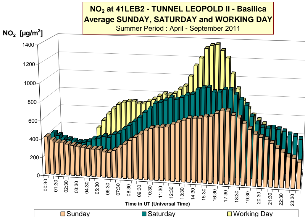
Fig. 16 : NO 2 – évolution journalière moyenne au poste de mesure 41LEB2 (basilique) Comparaison entre un dimanche, un samedi et un jour ouvrable moyen Période hivernale 2011-2012 et période estivale 2011
