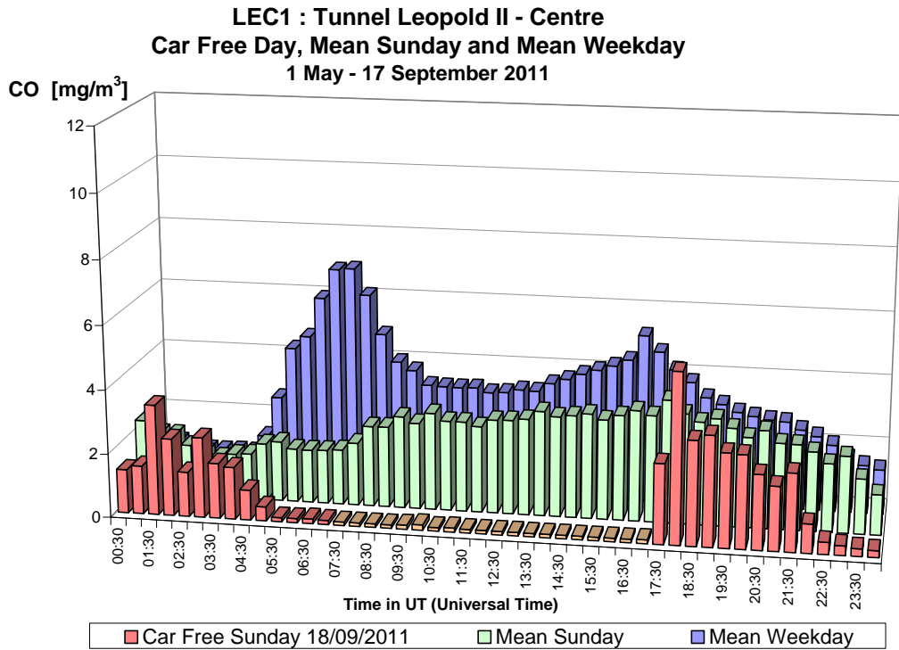
Fig. 31.a : CO dans le tunnel Léopold II, direction Centre – Profil journalier du dimanche sans voiture 18-09-2011, d'un dimanche moyen et d'un jour ouvrable moyen de la période 'mai – septembre 2011'.
