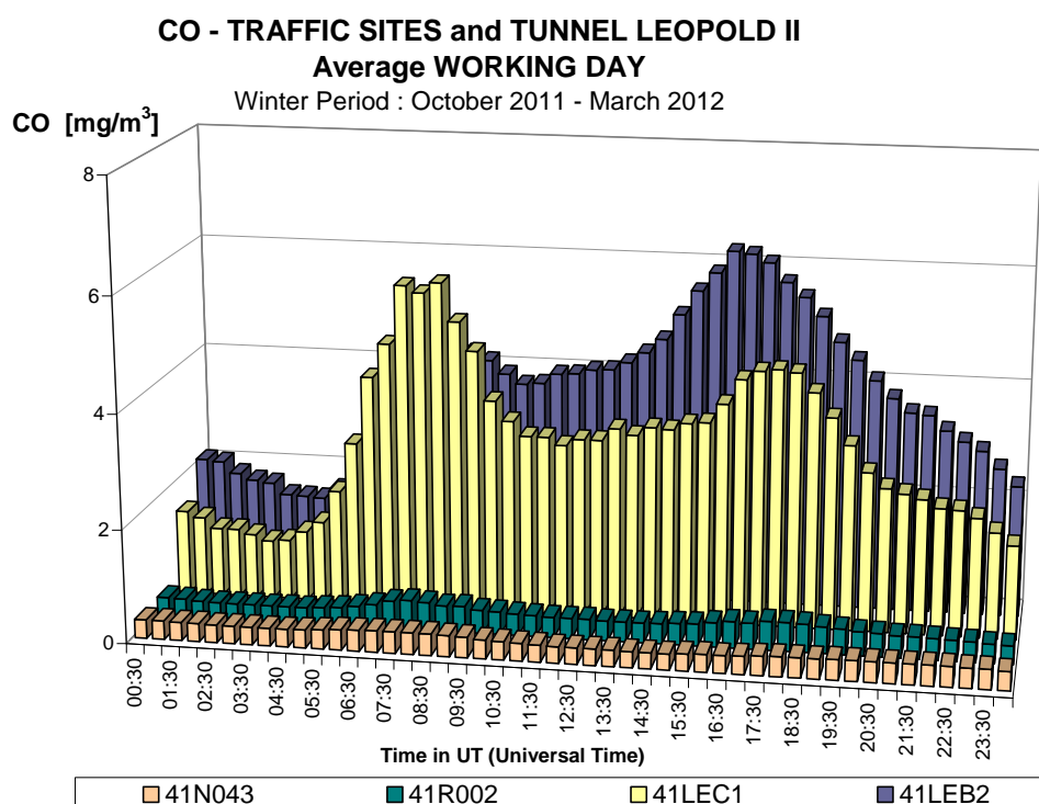
Fig. 33 : CO - Évolution journalière moyenne d'un jour ouvrable moyen ( hiver 2011-2012 ) Postes de mesure trafic à l'air ambiant – Avant Port (N043) et Av. de la Couronne (R002) Postes de mesure du Tunnel Léopold II – LEC1 (Centre) et LEB2 (Basilique)
