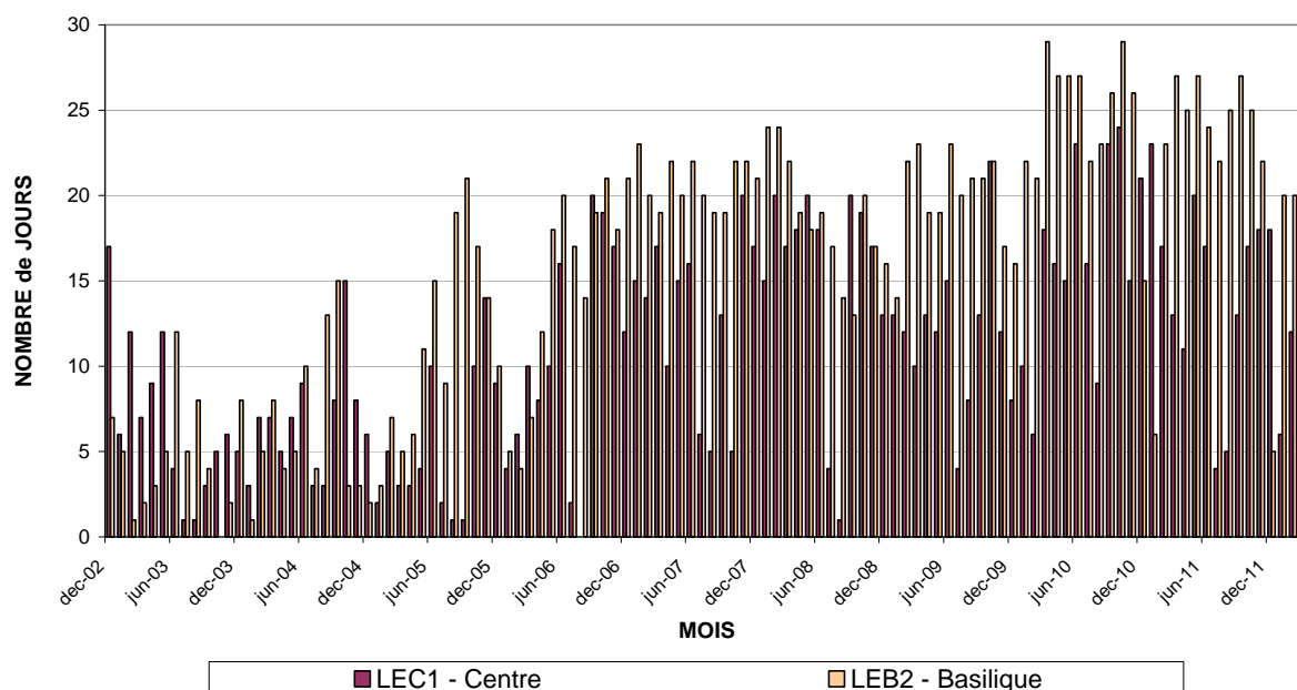
Fig. 13 : NO 2 – Valeurs Semi horaires > 850 µg/m 3 . Nombre de dépassements par mois et nombre de jours par mois avec dépassements (décembre 2002 – mars 2012)
