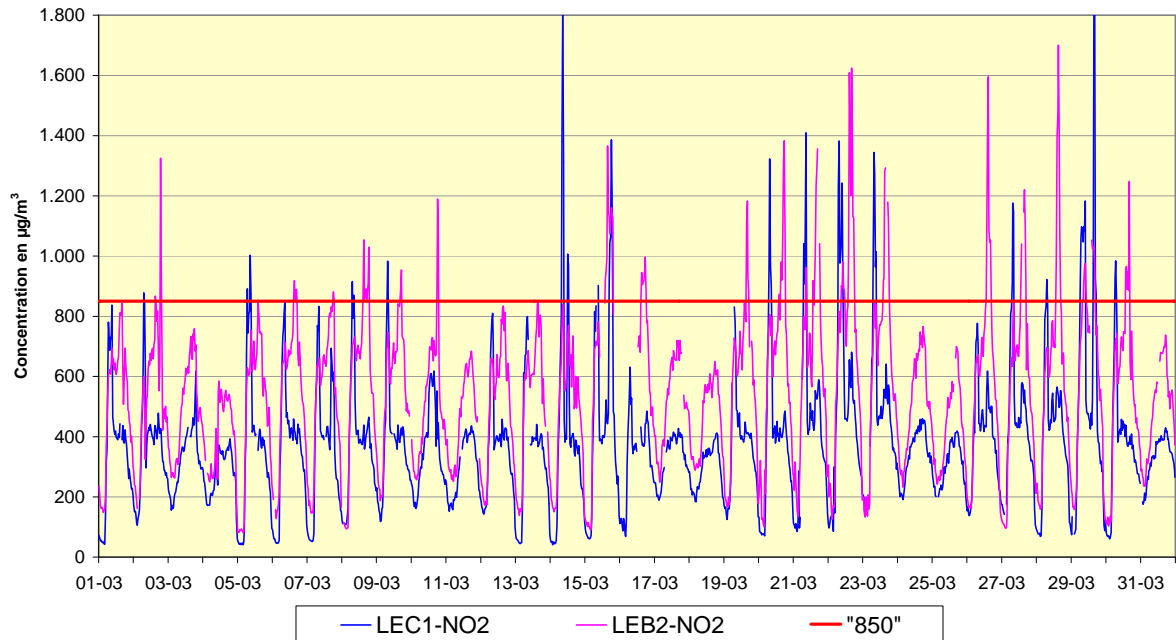
Fig. 1: NO 2 - Évolution des valeurs horaires et semi horaires en mars 2012 Poste de mesure 41LEC1, direction Centre – Poste de mesure 41LEB2, direction Basilique
