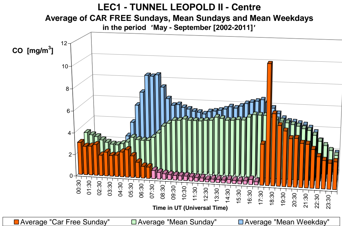
Fig. 31.b : CO dans le tunnel Léopold II, direction Centre – Profil journalier sur les dix dimanches sans voiture et sur tous les dimanches et jours ouvrables des périodes 'mai – septembre 2002-2011'.
