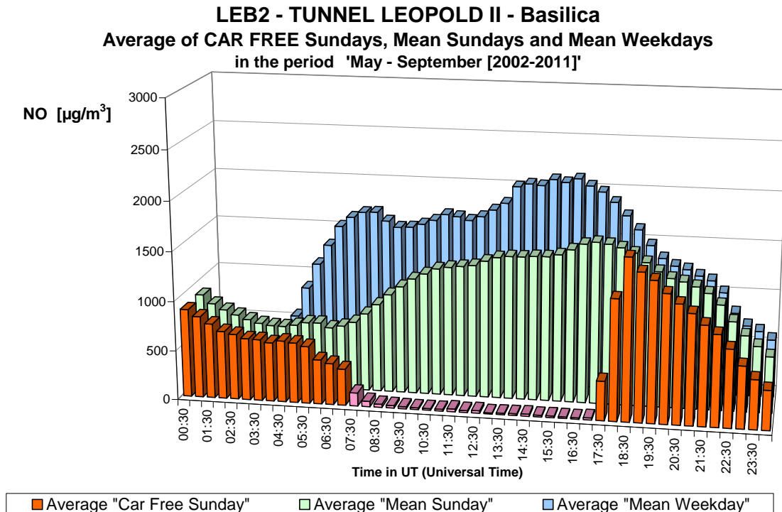
Fig. 30.b : NO dans le tunnel Léopold II, direction Basilique – Profil journalier sur les dix dimanches sans voiture et sur tous les dimanches et jours ouvrables des périodes 'mai – septembre 2002-2011'.
