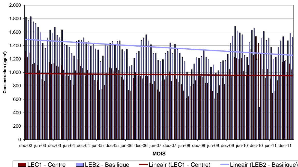
Fig. 9 : NO 2 et NO – Évolution des concentrations moyennes mensuelles dans les deux postes de mesure du tunnel Léopold II. Période – « Décembre 2002 – Mars 2012 »
