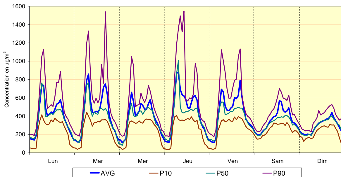
Fig. 21 : Poste de Mesure 41LEC1 (centre) – Évolution hebdomadaire moyenne pour le NO 2 Période hivernale 2011 - 2012 et période estivale 2011
