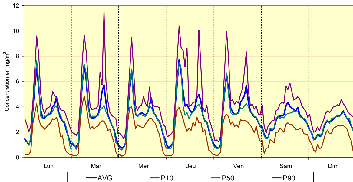
Fig. 23 : Poste de Mesure 41LEC1 (centre) – Évolution hebdomadaire moyenne pour le CO Période hivernale 2011 - 2012 et période estivale 2011
