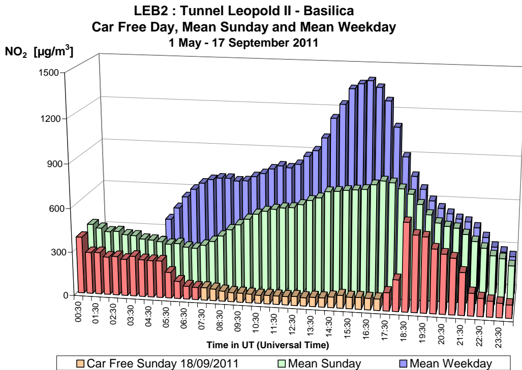
Fig. 28.a : NO 2 dans le tunnel Léopold II, direction Basilique – Profil journalier du dimanche sans voiture, d'un dimanche moyen et d'un jour ouvrable moyen de la période 'mai – septembre 2011'.
