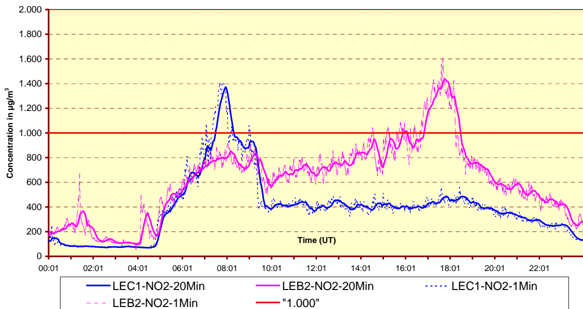
Fig. 4: NO 2 – évolution des valeurs minutes et de la moyenne glissante sur 20 minutes dans les deux postes de mesure du tunnel Léopold II Mardi 14 février 2012 et mardi 20 mars 2012
