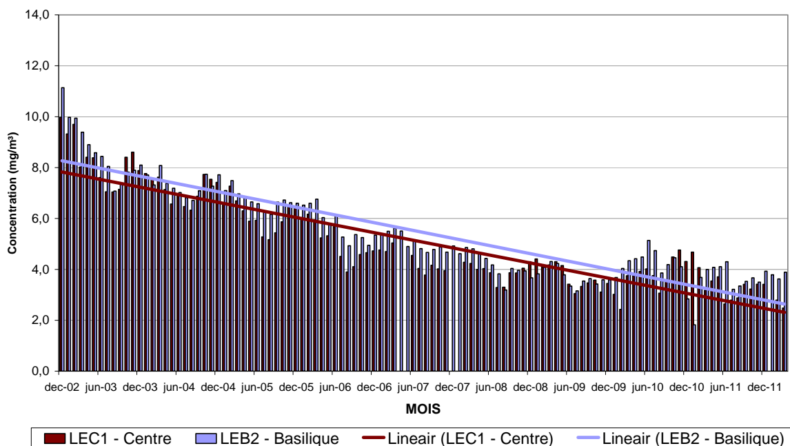
Fig. 10 : NO x et CO – Évolution des concentrations moyennes mensuelles dans les deux postes de mesure du tunnel Léopold II. Période – « Décembre 2002 – Mars 2012 »
