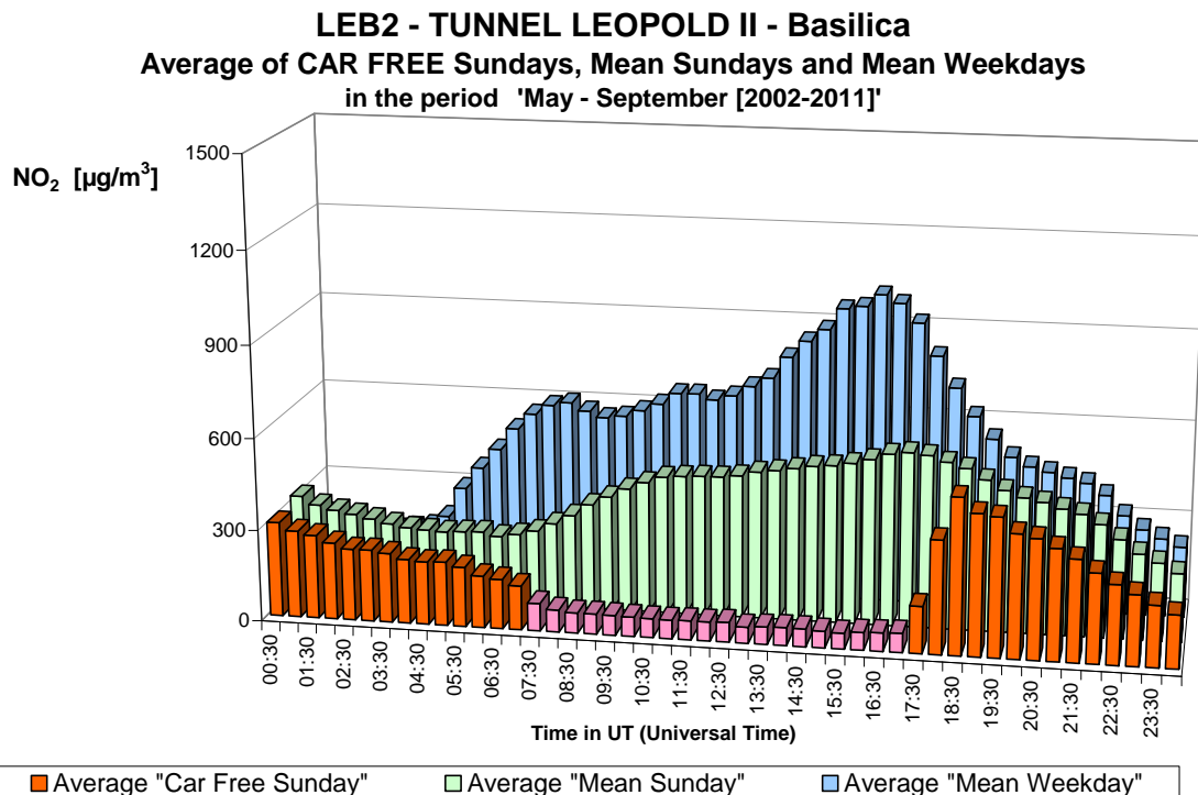
Fig. 28.b : NO 2 dans le tunnel Léopold II, direction Basilique – Profil journalier sur les dix dimanches sans voiture et sur tous les dimanches et jours ouvrables des périodes 'mai – septembre 2002-2011'.
