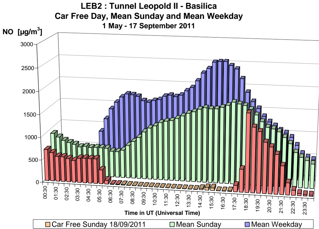
Fig. 30.a : NO dans le tunnel Léopold II, direction Basilique – Profil journalier du dimanche sans voiture, d'un dimanche moyen et d'un jour ouvrable moyen de la période 'mai – septembre 2011'.
