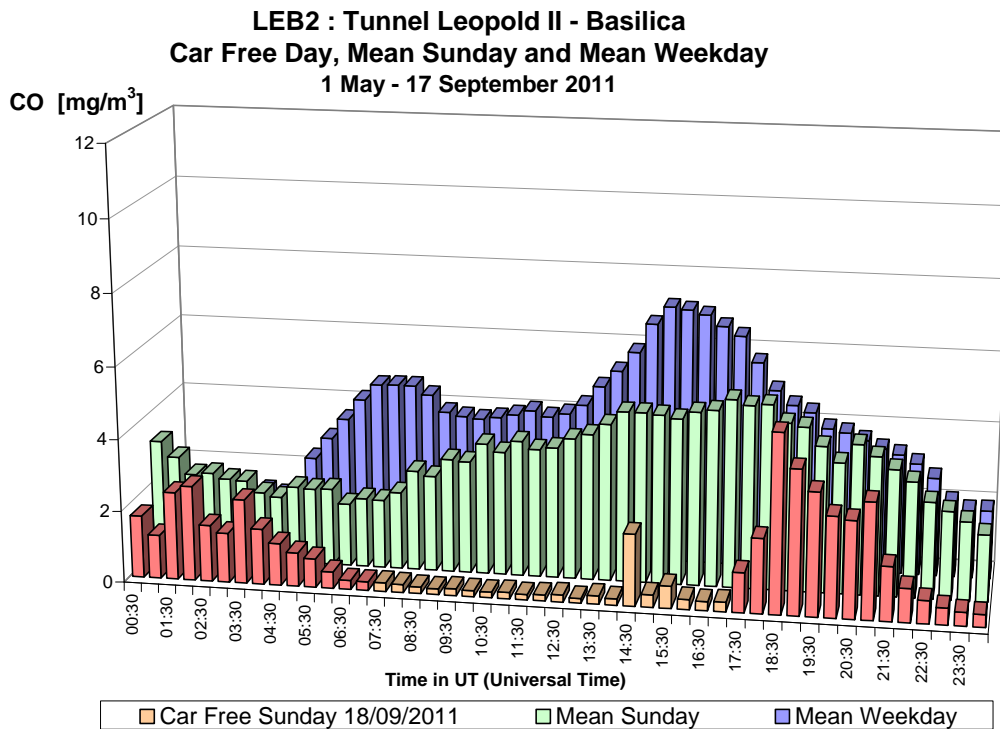
Fig. 32.a : CO dans le tunnel Léopold II, direction Basilique – Profil journalier du dimanche sans voiture, d'un dimanche moyen et d'un jour ouvrable moyen de la période 'mai – septembre 2011'.
