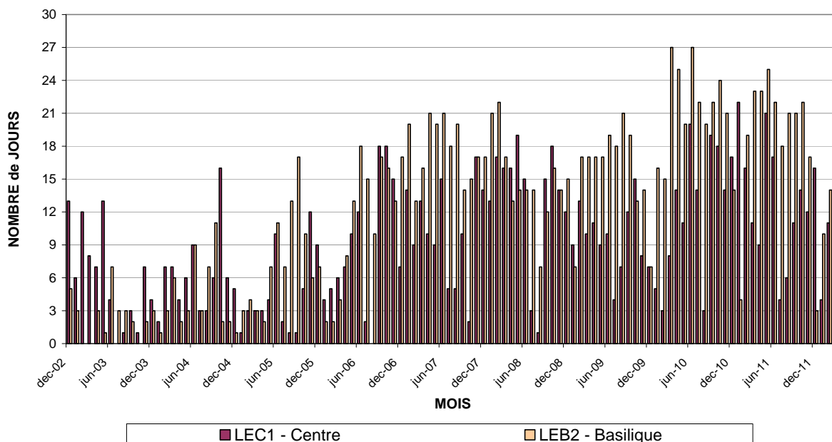
Fig. 12 : NO 2 –Moyennes glissantes sur 20 minutes > 1.000 µg/m 3 . Nombre de dépassements par mois et nombre de jours par mois avec dépassements (décembre 2002 – mars 2012)
