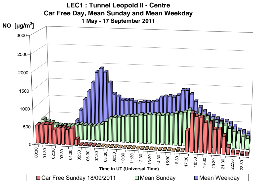
Fig. 29.a : NO dans le tunnel Léopold II, direction Centre – Profil journalier du dimanche sans voiture 18-09-2011, d'un dimanche moyen et d'un jour ouvrable moyen de la période 'mai – septembre 2011'.
