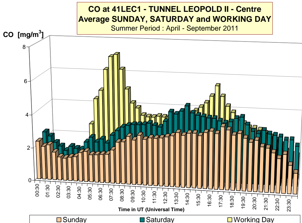
Fig. 19 : CO – évolution journalière moyenne au poste de mesure 41LEC1 (centre) Comparaison entre un dimanche, un samedi et un jour ouvrable moyen Période hivernale 2011-2012 et période estivale 2011
