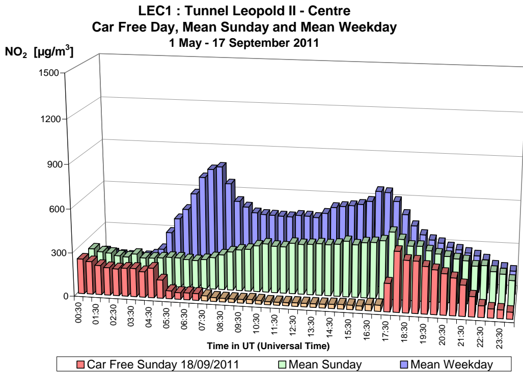
Fig. 27.a : NO 2 dans le tunnel Léopold II, direction Centre – Profil journalier du dimanche sans voiture 18-09-2011, d'un dimanche moyen et d'un jour ouvrable moyen de la période 'mai – septembre 2011'.
