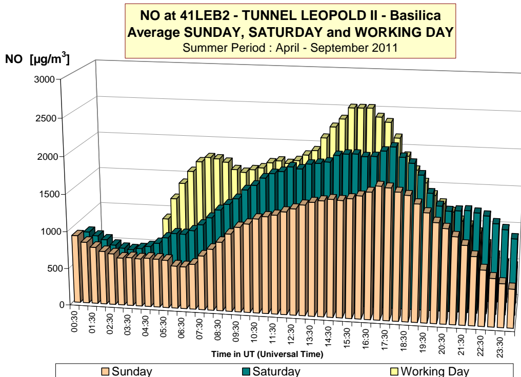
Fig. 18 : NO – évolution journalière moyenne au poste de mesure 41LEB2 (basilique) Comparaison entre un dimanche, un samedi et un jour ouvrable moyen Période hivernale 2011-2012 et période estivale 2011
