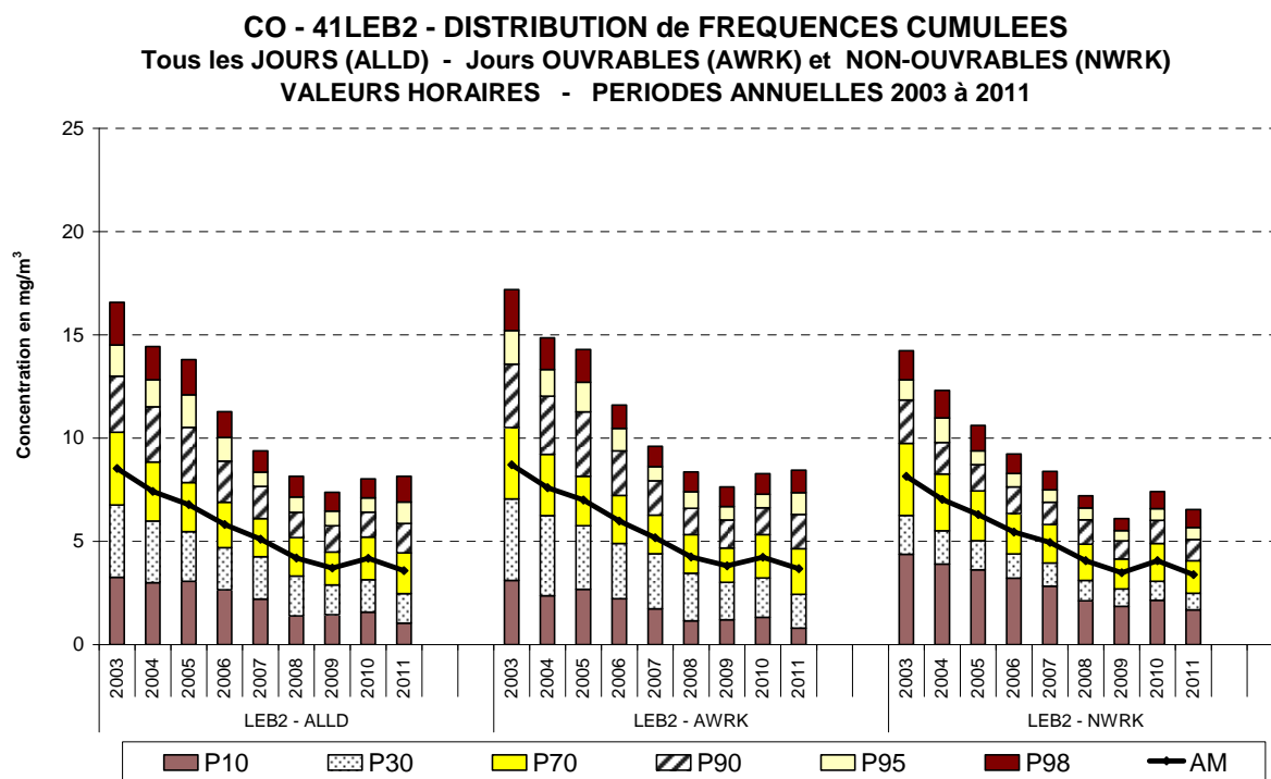
Fig. 6 : CO - Distribution de Fréquences Cumulées des Valeurs Horaïres dans les deux postes de mesure du tunnel Léopold II. Sélection tous les jours , les jours ouvrables et non ouvrables . Périodes annuelles de 2003 à 2011
