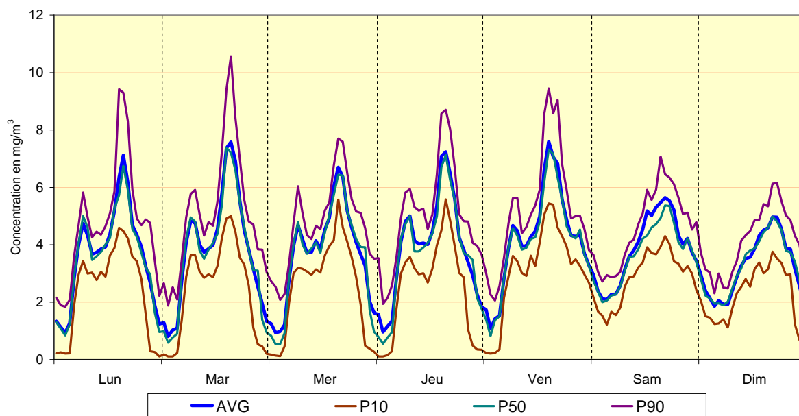
Fig. 24 : Poste de Mesure 41LEB2 (basilique) – Évolution hebdomadaire moyenne pour le CO Période hivernale 2011 - 2012 et période estivale 2011
