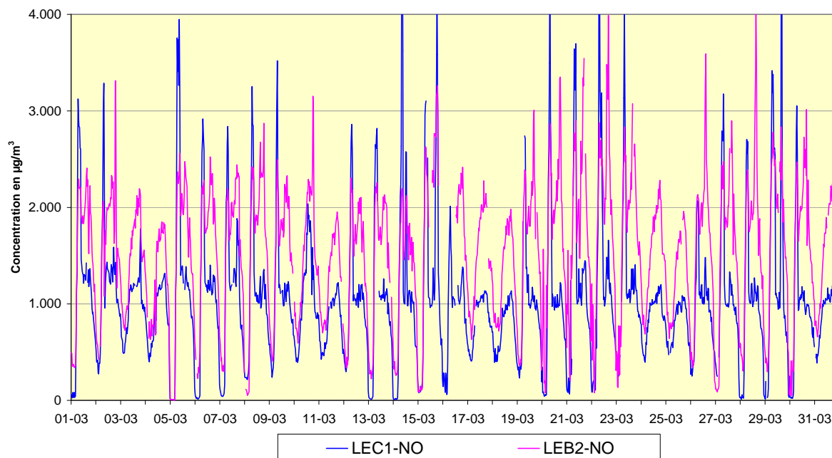
Fig. 2: NO - Évolution des valeurs horaires et semi horaires en mars 2012 Poste de mesure 41LEC1, direction Centre – Poste de mesure 41LEB2, direction Basilique
