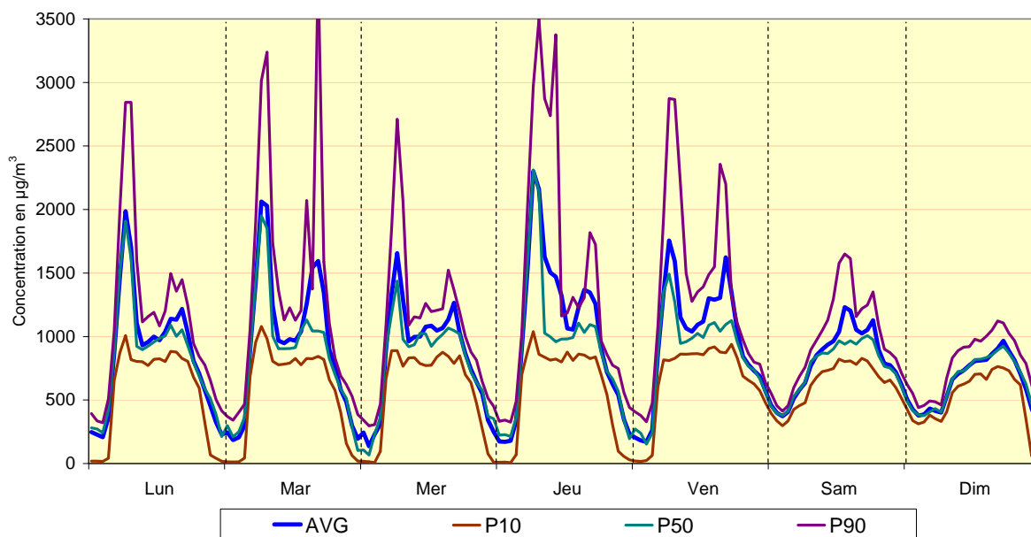
Fig. 25 : Poste de Mesure 41LEC1 (centre) – Évolution hebdomadaire moyenne pour le NO Période hivernale 2011 - 2012 et période estivale 2011
