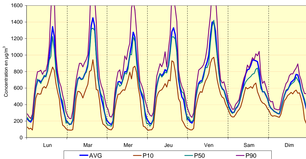
Fig. 22 : Poste de Mesure 41LEB2 (basilique) – Évolution hebdomadaire moyenne pour le NO 2 Période hivernale 2011 - 2012 et période estivale 2011
