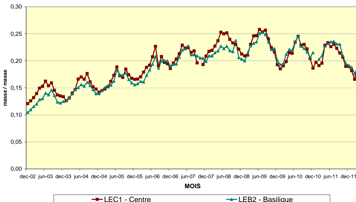
Fig. 11 : Évolution du rapport NO 2 /NO x dans les deux postes de mesure du tunnel Léopold II. Période – « Décembre 2002 – Mars 2012 »
