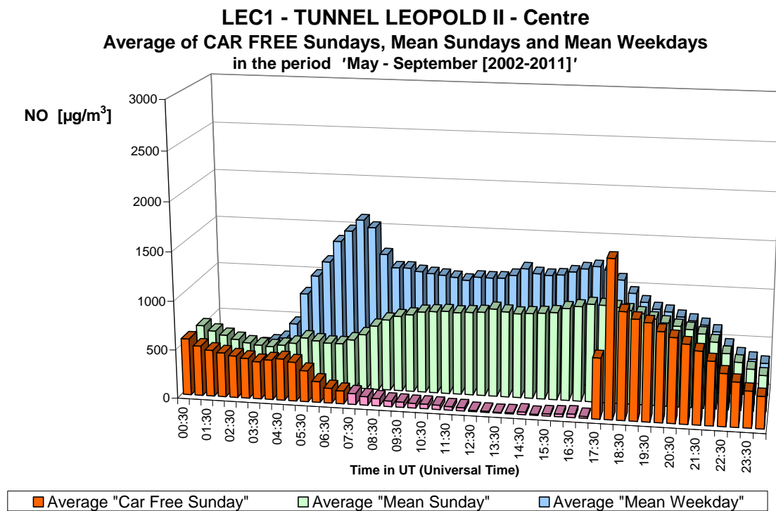
Fig. 29.b : NO dans le tunnel Léopold II, direction Centre – Profil journalier sur les dix dimanches sans voiture et sur tous les dimanches et jours ouvrables des périodes 'mai – septembre 2002-2011'.
