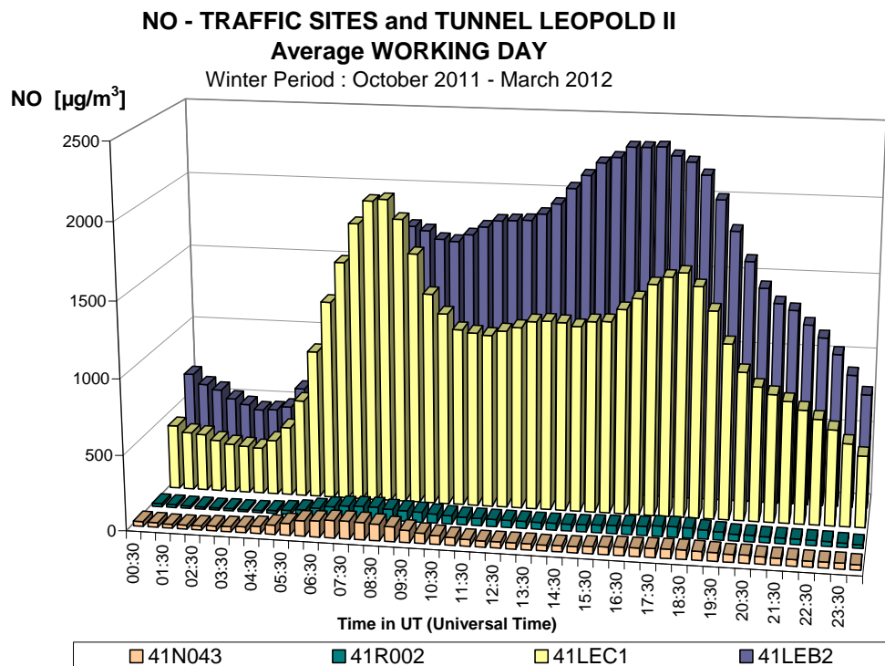
Fig. 34 : NO 2 et NO - Évolution journalière moyenne d'un jour ouvrable moyen ( hiver 2011-2012 ) Postes de mesure trafic à l'air ambiant – Avant Port (N043) et Av. de la Couronne (R002) Postes de mesure du Tunnel Léopold II – LEC1 (Centre) et LEB2 (Basilique)
