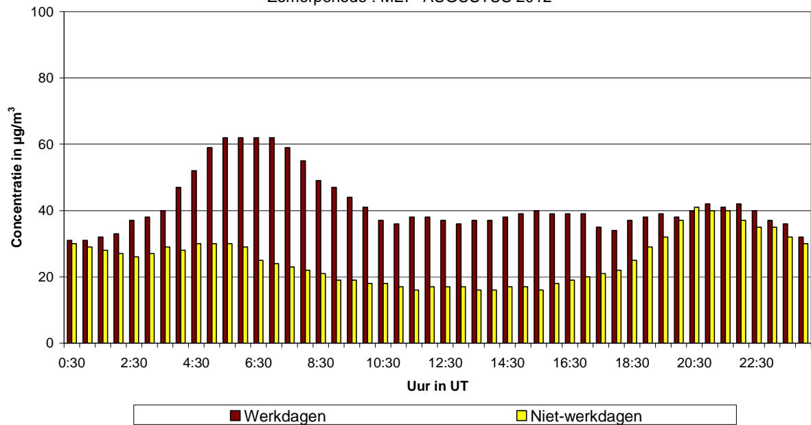
Fig. 49.b : Voorhaven : Gemiddeld dagverloop van de NO 2 -concentratie op werkdagen en niet-werkdagen tijdens de periode mei - augustus 2012
