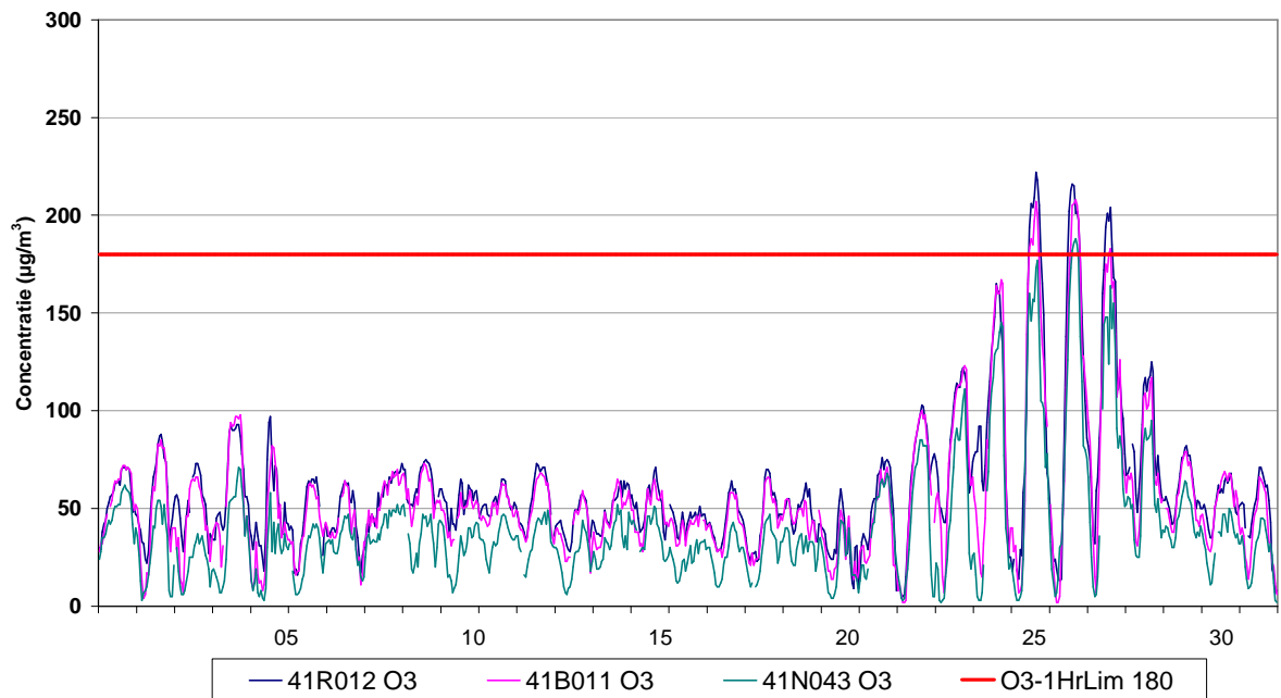
Fig. 5 : Evolutie van de uurwaarden voor ozon – Ukkel, Berchem en Voorhaven – Juli 2012
