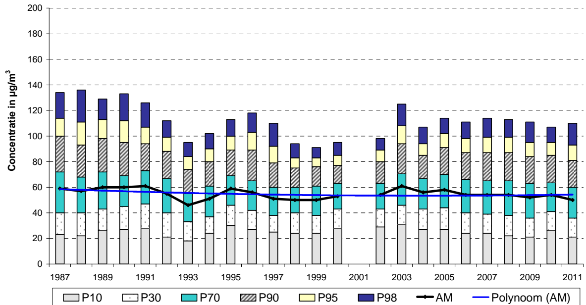
Fig. 73: NO 2 – Kroonlaan te Elsene ( canyon street ) - Uurgemiddelde concentratie Evolutie over langere termijn - Jaarperiodes 1987 – 2011
