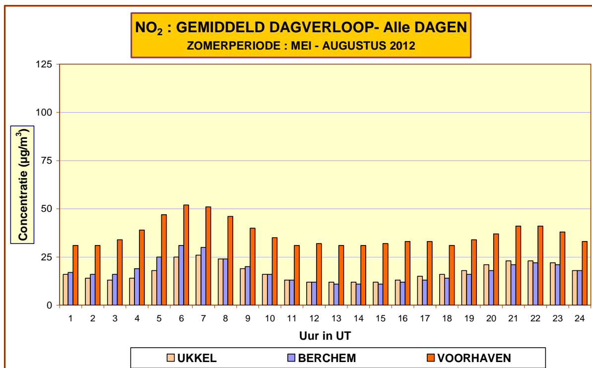
Fig. 66: NO 2 – Evolutie Dagverloop – Vergelijking tussen 3 meetposten Periode “mei –augustus 2012”
