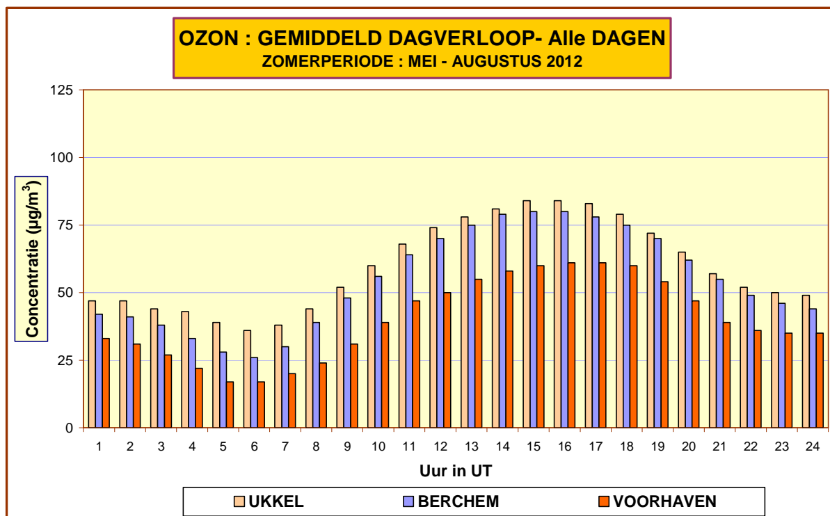
Fig. 65: Ozon – Evolutie Dagverloop – Vergelijking tussen 3 meetposten Periode “mei –augustus 2012”
