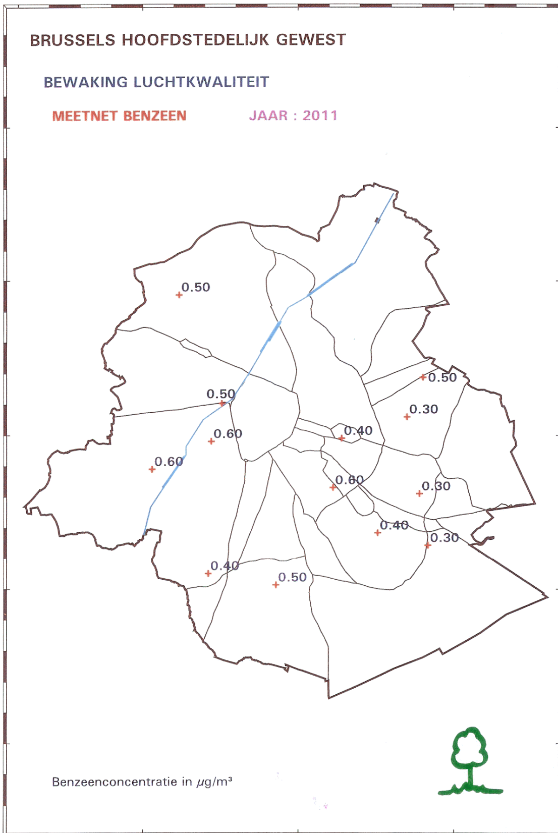
Fig. 31 : Benzeen – Ruimtelijke spreiding jaargemiddelde concentratie in 2011
