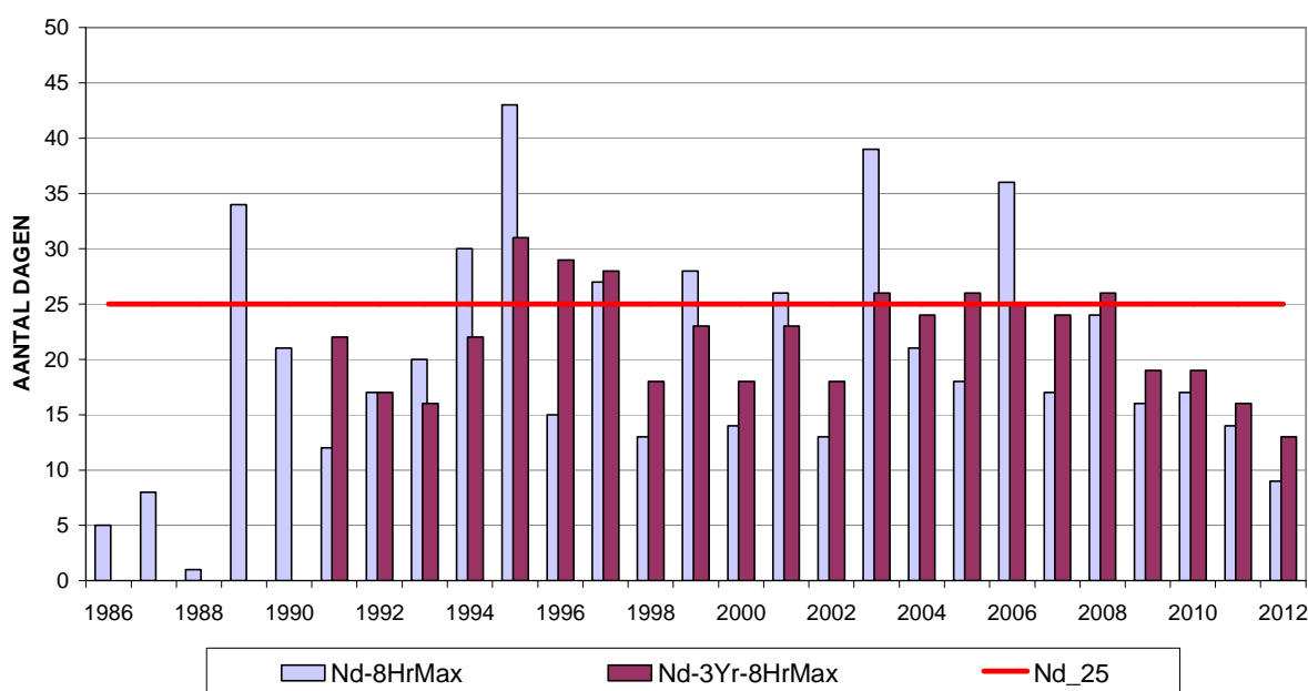
Fig. 12 : Ozon - Evolutie aantal overschrijdingsdagen in de meetpost te Ukkel Streefwaarde voor de gezondheid: Maximale 8-uurwaarde > 120 µg/m 3 Periode : Januari – December (1986-2011). [2012]: Januari – September
