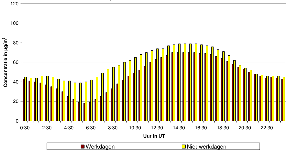
Fig. 52.a : St.-Katelijne : Gemiddeld dagverloop van de O 3 -concentratie op werkdagen en niet-werkdagen tijdens de periode mei - augustus 2012
