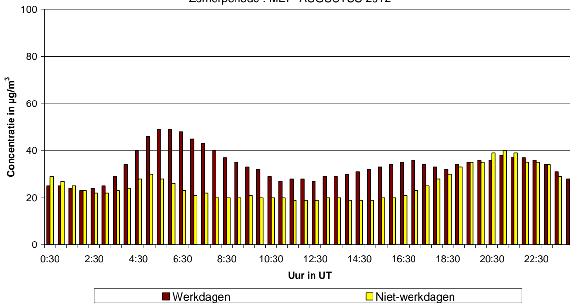
Fig. 48.b : Molenbeek : Gemiddeld dagverloop van de NO 2 -concentratie op werkdagen en niet-werkdagen tijdens de periode mei – augustus 2012
