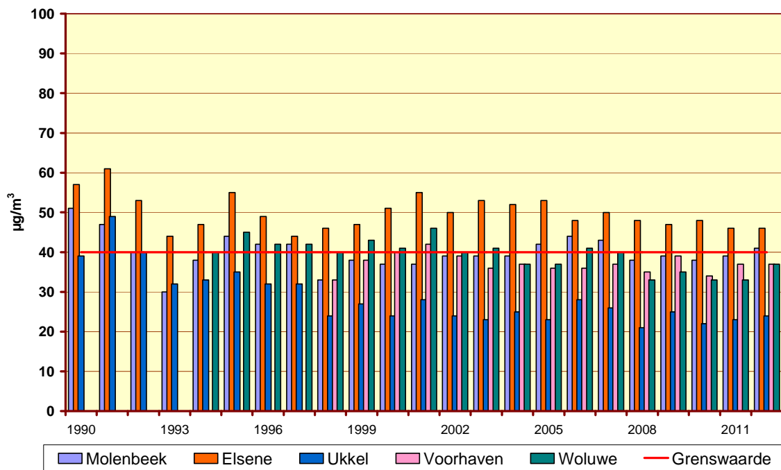
Fig. 27.c : NO 2 - Evolutie gemiddelde concentratie op 'Zaterdag' Jaarperiodes 1990-2011 en "Oktober 2011 - September 2012"
