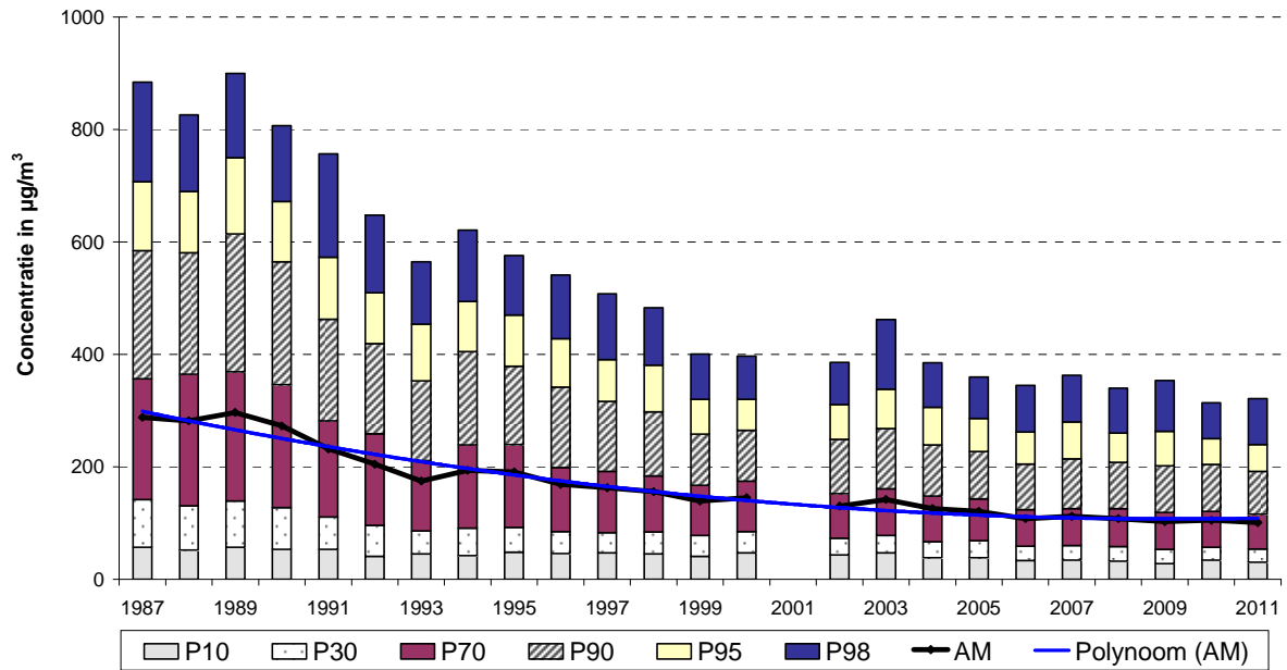
Fig. 72: NO x – Kroonlaan te Elsene ( canyon street ) - Uurgemiddelde concentratie Evolutie over langere termijn - Jaarperiodes 1987 – 2011
