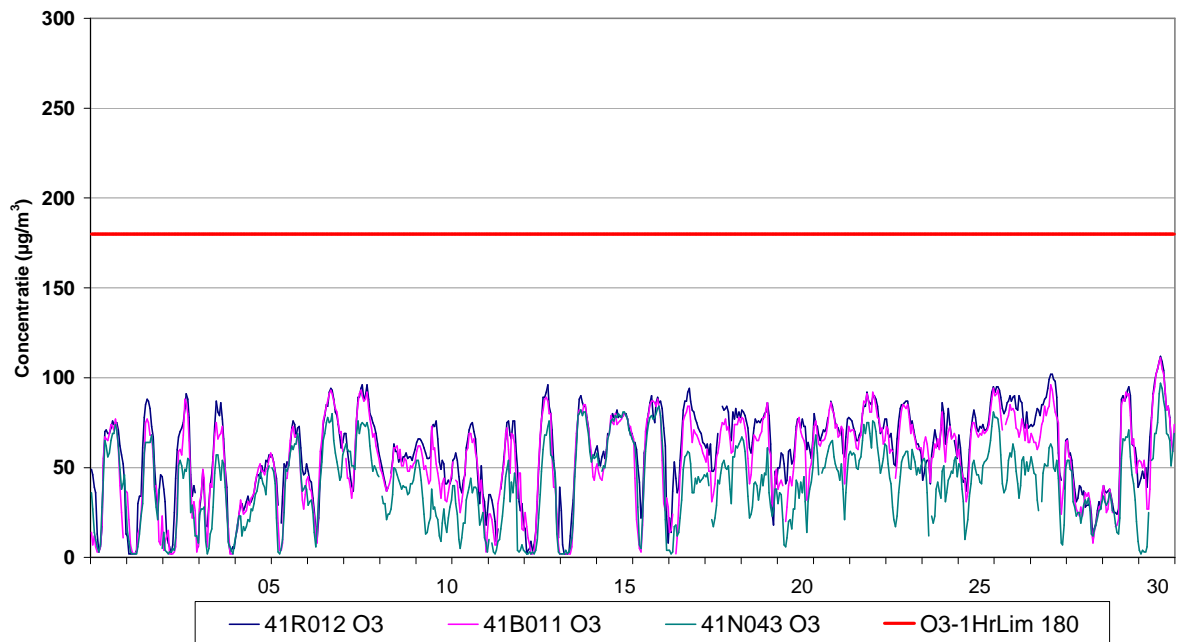
Fig. 2 : Evolutie van de uurwaarden voor ozon – Ukkel, Berchem en Voorhaven – April 2012
