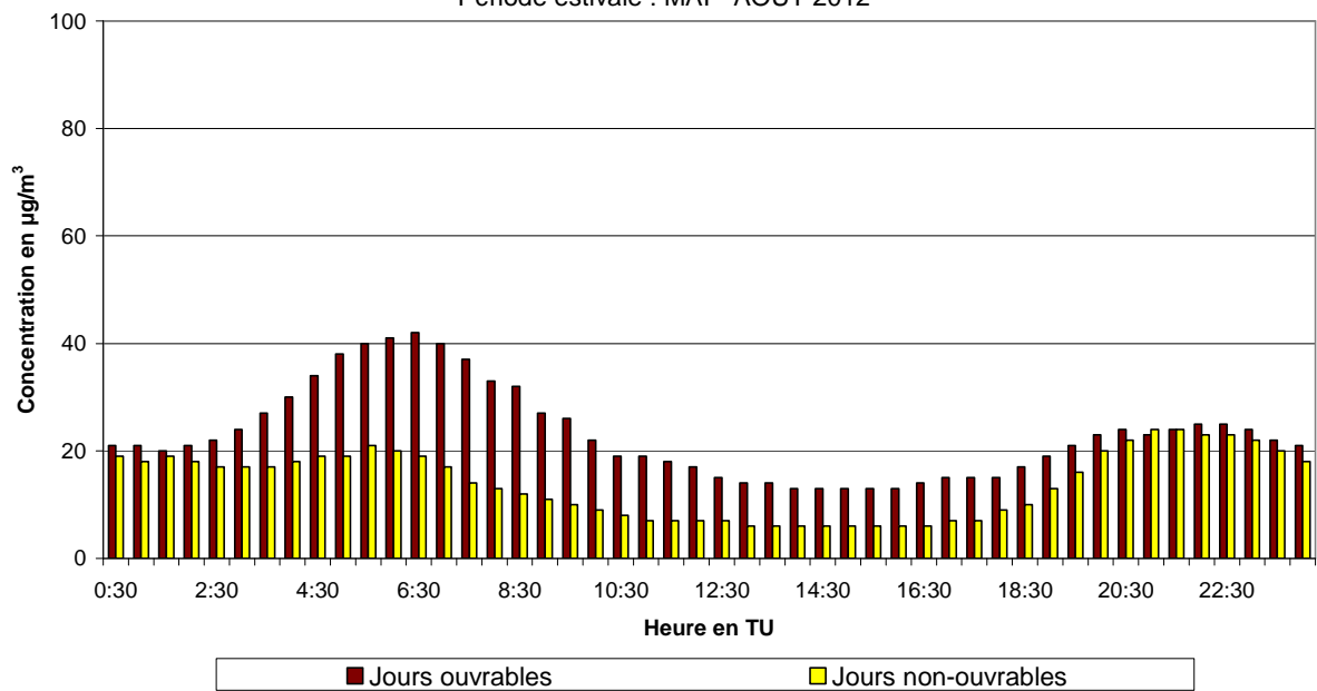
Fig. 53.b : Meudon Park : Gemiddeld dagverloop van de NO 2 -concentratie op werkdagen en niet-werkdagen tijdens de periode mei - augustus 2012
