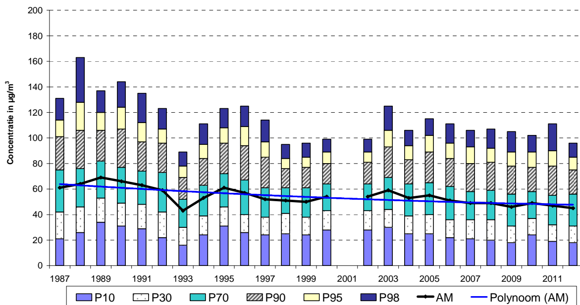
Fig. 40 : Elsene – Evolutie NO 2 -uurwaarden (1987-2012) Zomerperiode "april – september"
