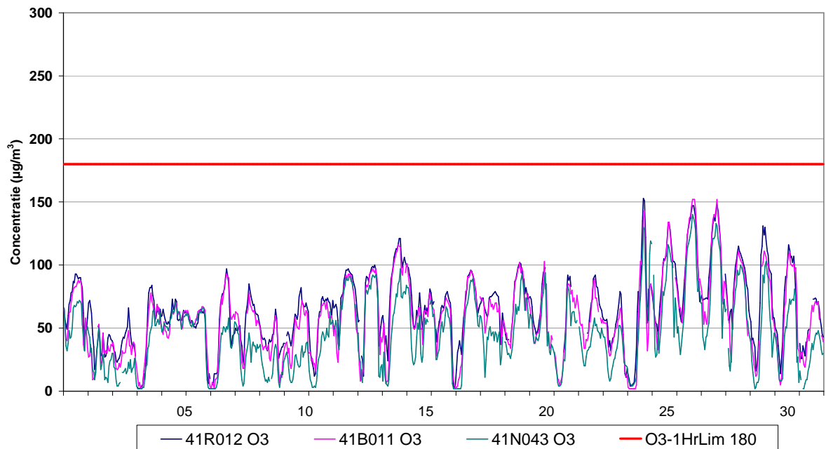
Fig. 3 : Evolutie van de uurwaarden voor ozon – Ukkel, Berchem en Voorhaven – Mei 2012
