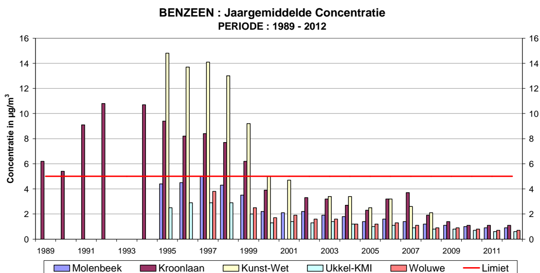
Fig. 28 : Benzeen - Evolutie jaargemiddelde concentratie Periode : Januari – December (1989-2011) en 'Oktober 2011 – September 2012'
