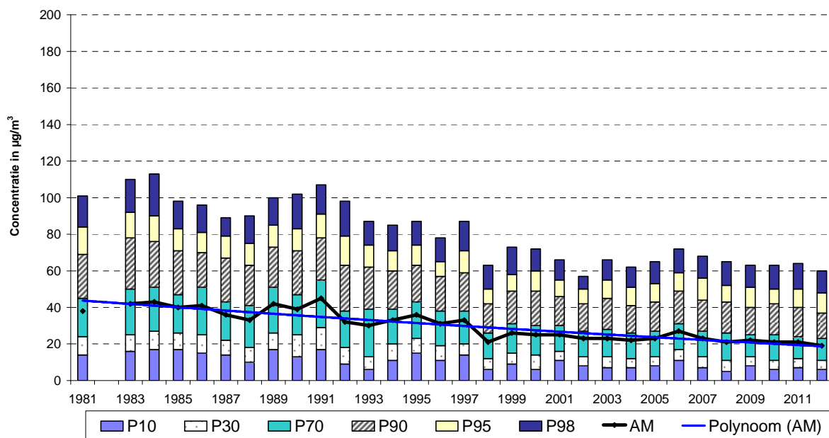
Fig. 41 : Ukkel – Evolutie NO 2 -uurwaarden (1981-2012) Zomerperiode "april – september"
