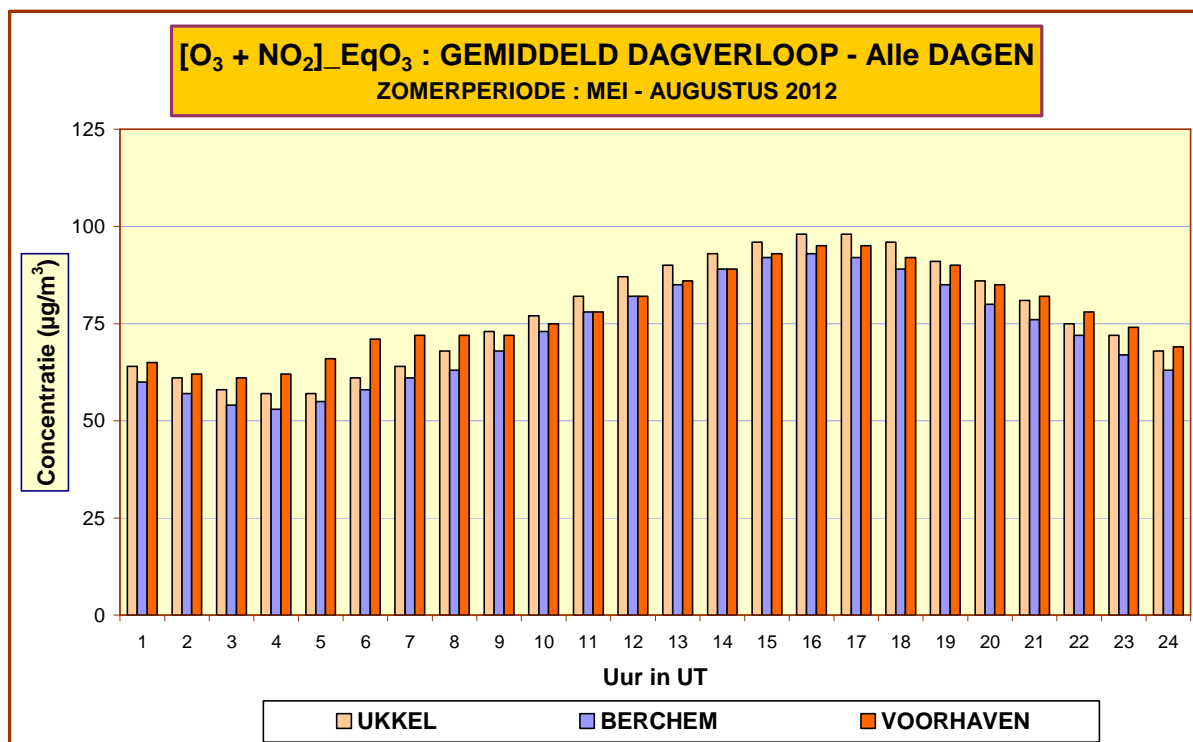
Fig. 67: [O 3 + NO 2 ] – Evolutie Dagverloop – Vergelijking tussen 3 meetposten Periode “mei – augustus 2012”
