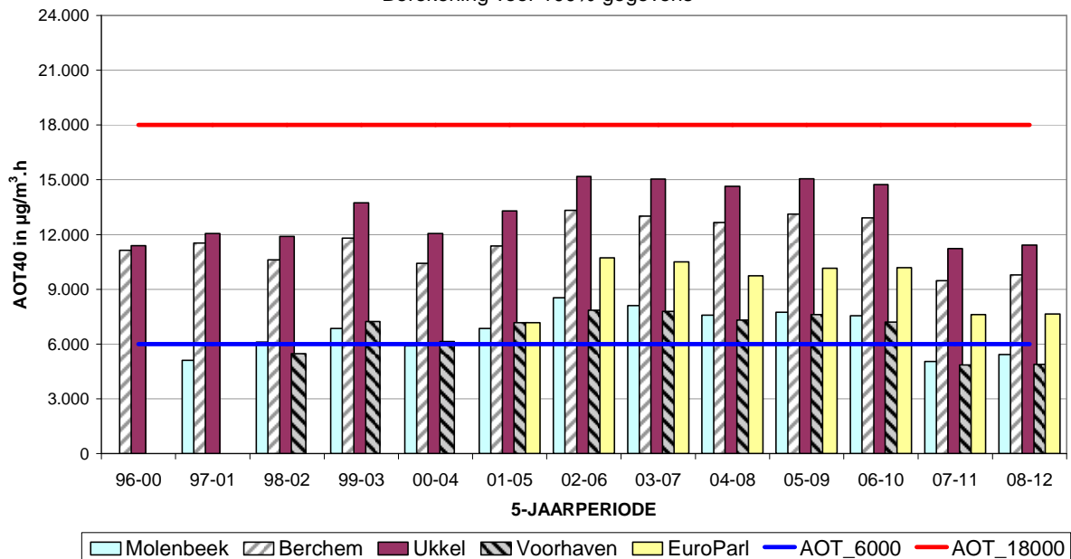
Fig. 15: Evolutie AOT40-MJ in de tijd (1996-2012) AOT40 over de periode Mei – Juli, 8-20 h MET - Midden-Europese tijd Resultaten per jaar en gemiddeld over 5 jaar
