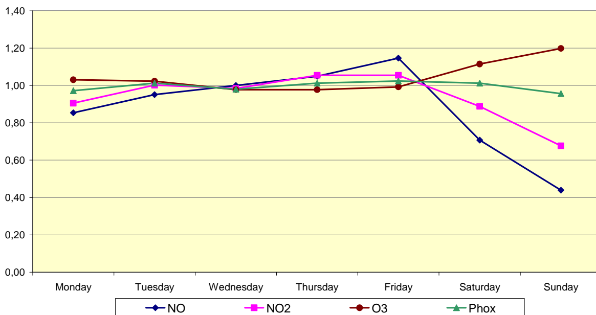
Fig. 59.b : Meetpost te Molenbeek – Gemiddeld weekpatroon voor NO, NO 2 , O 3 en [NO 2 +O 3 ] over drie opeenvolgende zomerperiodes 'april – september' 2010, 2011 en 2012
