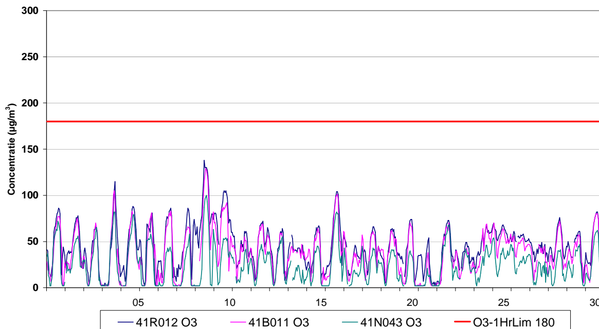
Fig. 7 : Evolutie van de uurwaarden voor ozon – Ukkel, Berchem en Voorhaven – September 2012
