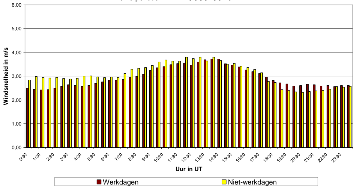
Fig. 55.b : Ukkel : Gemiddeld dagverloop van de windsnelheid op werkdagen en niet-werkdagen tijdens de periode mei – augustus 2012
