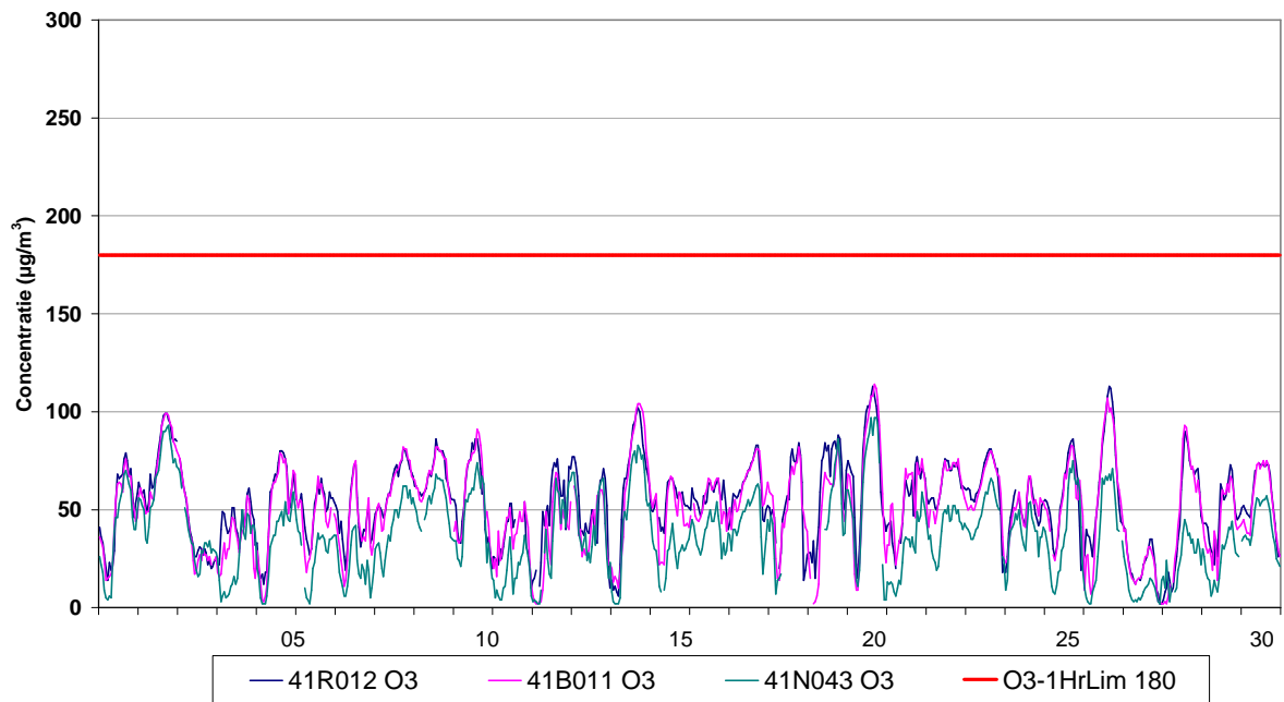
Fig. 4 : Evolutie van de uurwaarden voor ozon – Ukkel, Berchem en Voorhaven – Juni 2012
