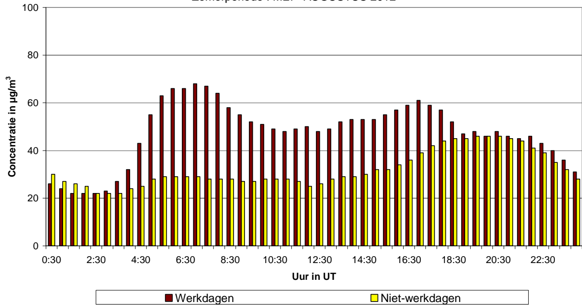
Fig. 54.a : Kroonlaan te Elsene : Gemiddeld dagverloop van de NO 2 -concentratie op werkdagen en niet-werkdagen tijdens de periode mei - augustus 2012
