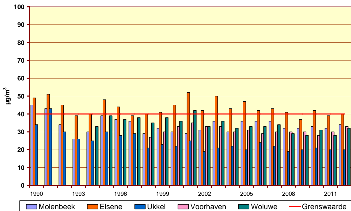
Fig. 27.d : NO 2 - Evolutie gemiddelde concentratie op 'Zondag' Jaarperiodes 1990-2011 en "Oktober 2011 - September 2012"
