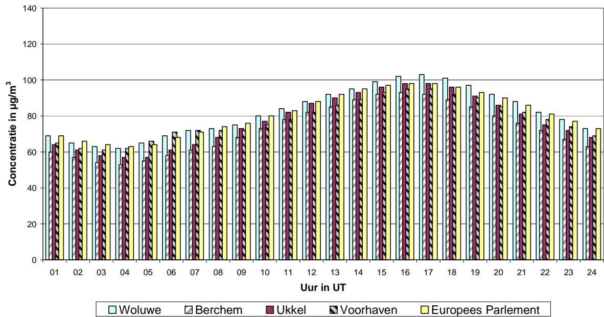
Fig. 10 : Gemiddeld dagverloop voor de som van de gasvormige oxidantia [O 3 + NO 2 ], uitgedrukt als equivalente massaconcentratie ozon, tijdens de periode mei – augustus 2012
