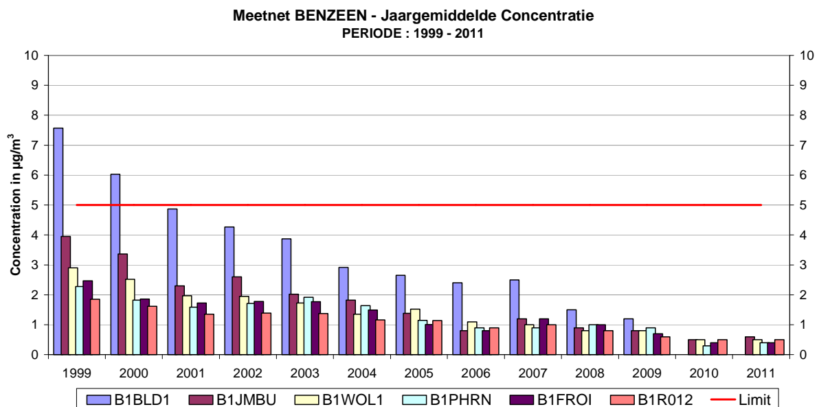
Fig. 30 : Benzeen – Evolutie jaargemiddelde concentratie in een aantal meetpunten van het benzeenmeetnet – Periode : 1999 - 2011
