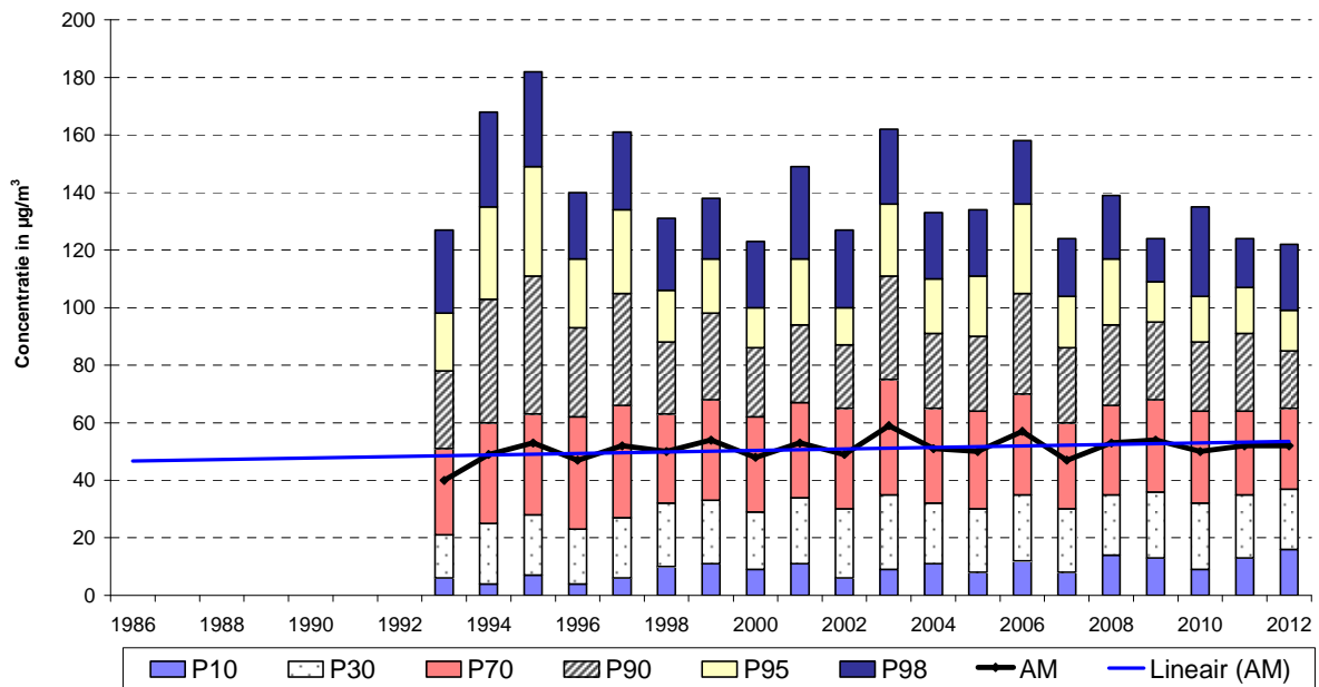
Fig. 71: Ozon te St.-Ag.-Berchem – Uurgemiddelde concentratie – evolutie over langere termijn Zomerperiodes 1993 - 2012
