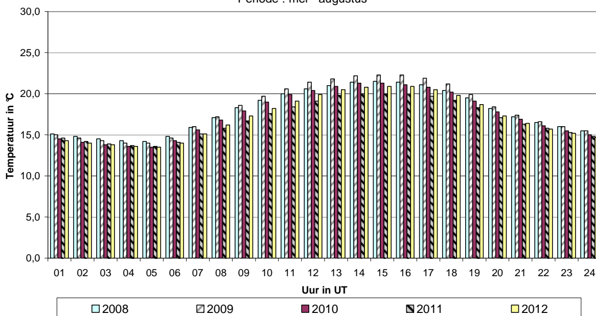
Gemiddeld dagverloop Temperatuur Vergelijking 2008, 2009, 2010, 2011 en 2012 Periode : mei - augustus
