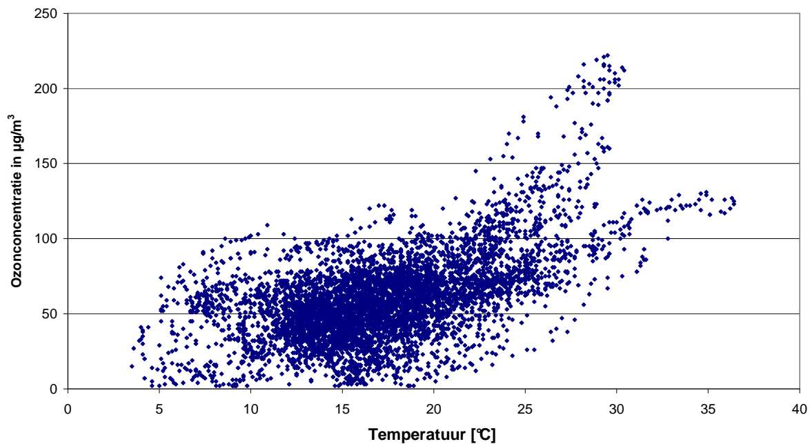
Fig. 42 : Ukkel : Ozonconcentraties versus temperatuur (mei - augustus 2012)
