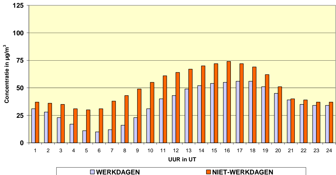
Fig. 68: Ozon – Evolutie Dagverloop voor werkdagen en niet-werkdagen Meetposten Ukkel en Voorhaven - Periode “mei – augustus 2012”
