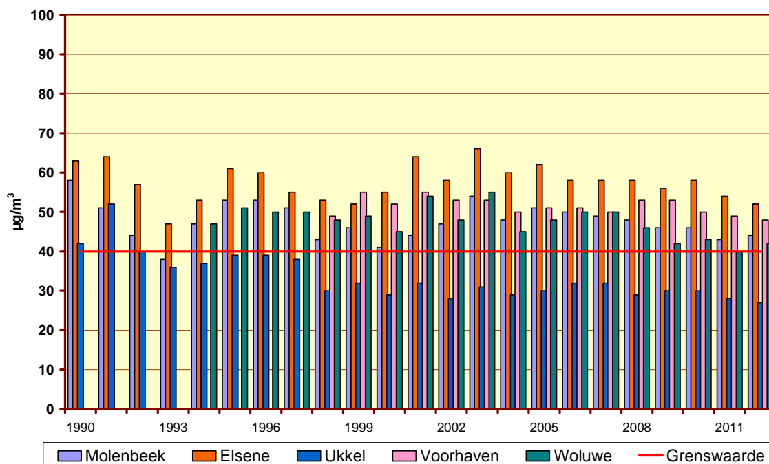
Fig. 27.b : NO 2 - Evolutie gemiddelde concentratie op 'werkdagen' Jaarperiodes 1990-2011 en "Oktober 2011 – September 2012"
