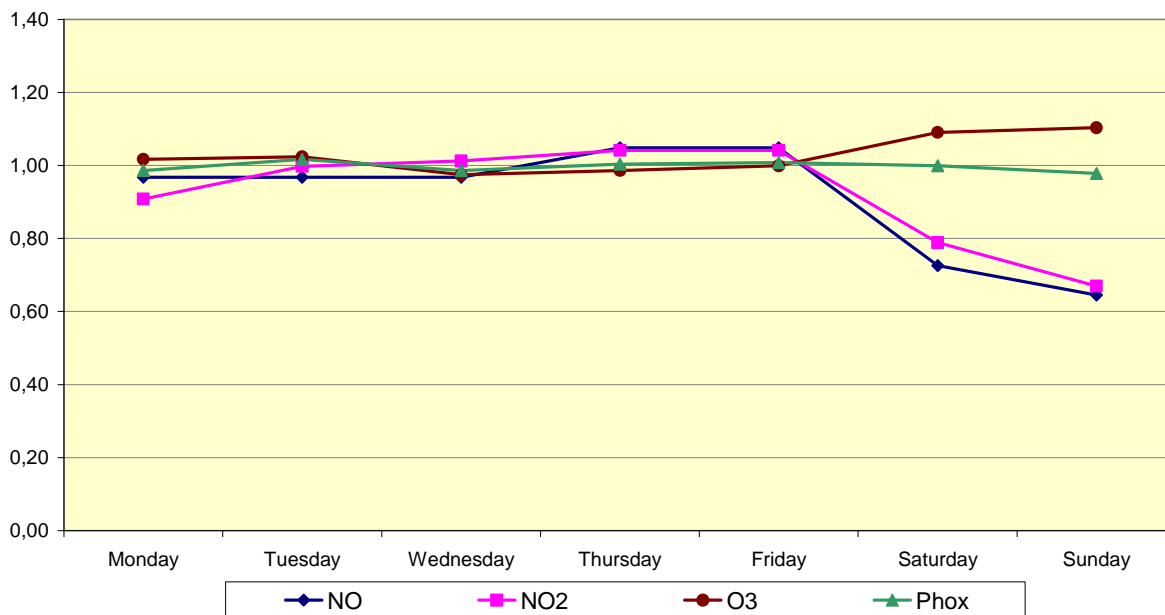
Fig. 59.a : Meetpost te Ukkel – Gemiddeld weekpatroon voor NO, NO 2 , O 3 en [NO 2 +O 3 ] over drie opeenvolgende zomerperiodes 'april – september' 2010, 2011 en 2012
