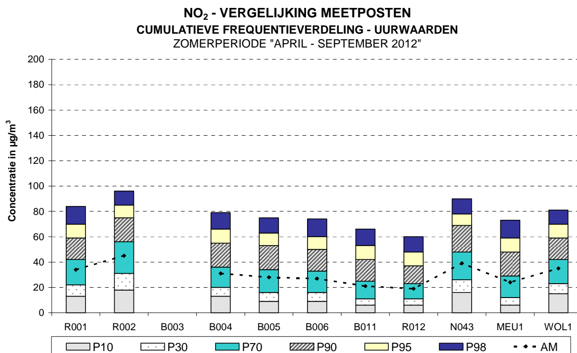
Fig. 39 : NO 2 - Cumulatieve frequentieverdeling uurwaarden: april - september 2012
