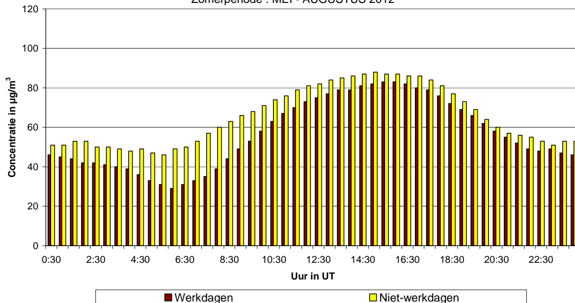
Fig. 46.a : Ukkel : Gemiddeld dagverloop van de O 3 -concentratie op werkdagen en niet-werkdagen tijdens de periode mei - augustus 2012
