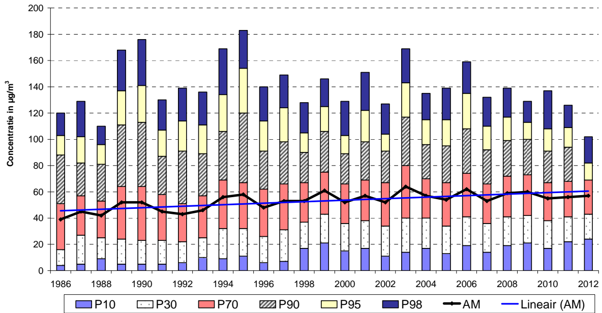
Fig. 70: Ozon te Ukkel – Uurgemiddelde concentratie – evolutie over langere termijn Zomerperiodes 1986 - 2012
