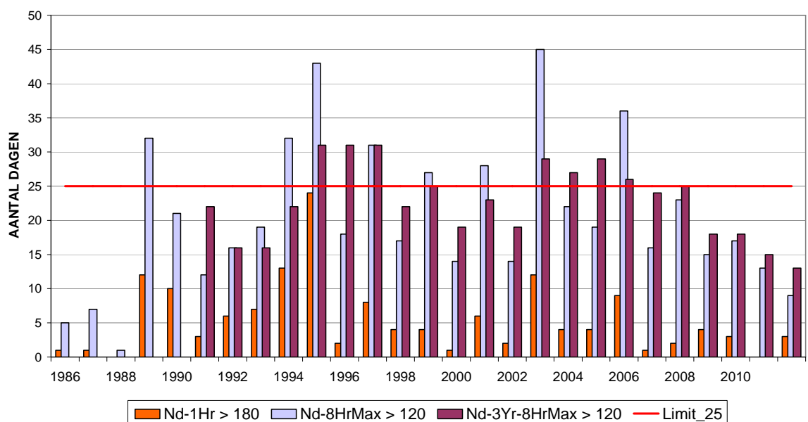
Fig. 21 : Ozon : aantal dagen met overschrijdingen in het Gewest Jaarperioden: 1 januari – 31 december (1986-2011) Voorlopige resultaten voor het jaar 2012 (1 januari – 30 september)
