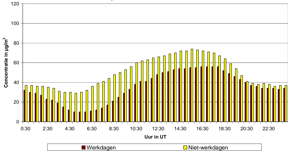
Fig. 49.a : Voorhaven : Gemiddeld dagverloop van de O 3 -concentratie op werkdagen en niet-werkdagen tijdens de periode mei - augustus 2012
