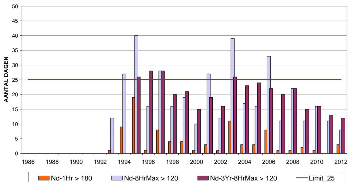
Fig. 20 : Ozon te St.-Ag.-Berchem : aantal dagen met overschrijdingen Jaarperioden: 1 januari – 31 december (1986-2011) Voorlopige resultaten voor het jaar 2012 (1 januari – 30 september)
