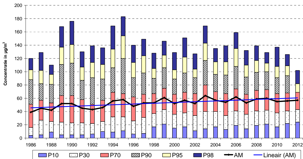
Fig. 33 : Evolutive O 3 -uurwaarden te Ukkel (1986-2012) Zomerperiode "april – september"
