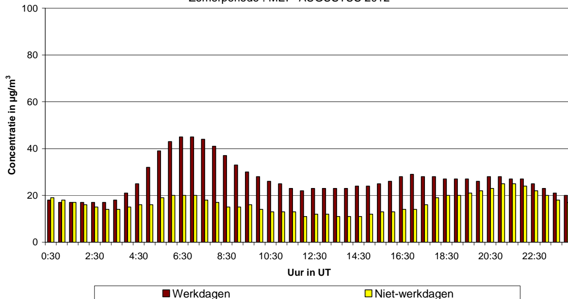
Fig. 51.b : Europees Parlement : Gemiddeld dagverloop van de NO 2 -concentratie op werkdagen en niet-werkdagen tijdens de periode mei – augustus 2012
