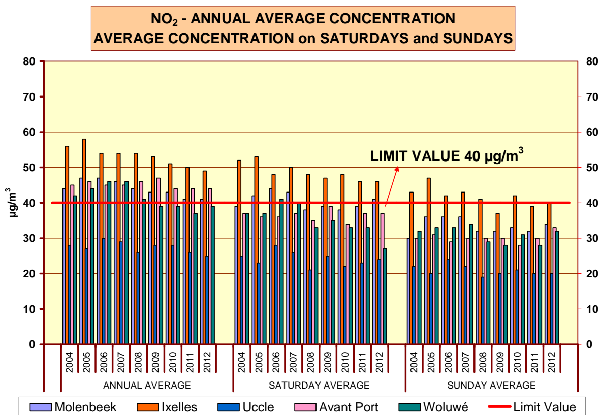
Fig. 26 : NO 2 – Vergelijking jaargemiddelde concentratie met de gemiddelde concentratie op 'Zaterdag' en 'Zondagen' voor een selectie van meetposten. Jaarperiodes 2004-2011 en "Oktober 2011 – September 2012"
