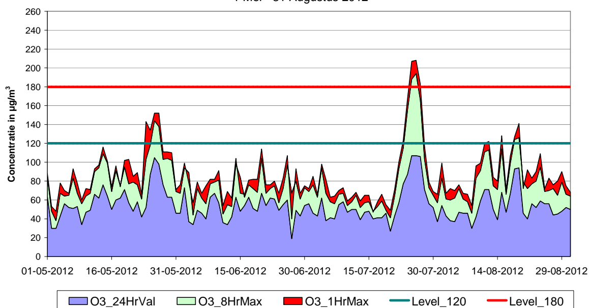
Fig. 22 : Ozon - Evolutie Dagwaarde (24HrVal), maximale 8-uurwaarde (8HrMax) en maximale uurwaarde (1HMax). Periode : mei - augustus 2012 Meetposten te Ukkel en St.-Agatha-Berchem
