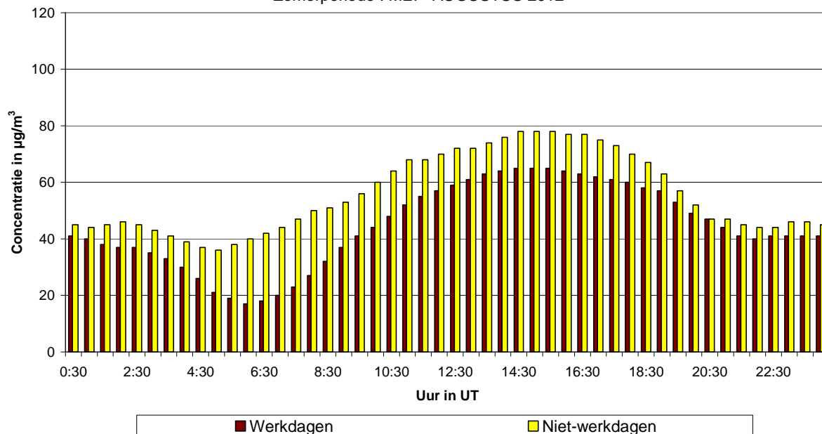
Fig. 50.a : St.-Lambr.-Woluwe : Gemiddeld dagverloop van de O 3 -concentratie op werkdagen en niet-werkdagen tijdens de periode mei - augustus 2012
