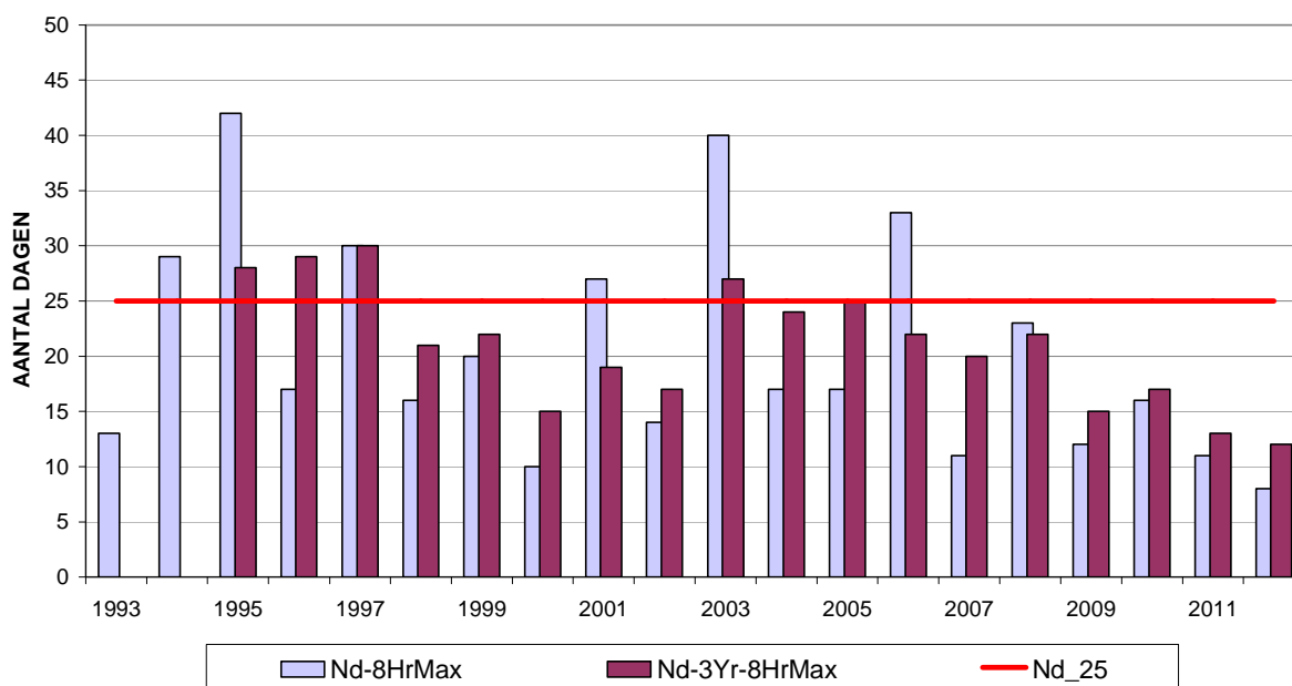
Fig. 13 : Ozon - Evolutie aantal overschrijdingsdagen in de meetpost te Berchem Streefwaarde voor de gezondheid: Maximale 8-uurwaarde > 120 µg/m 3 Periode : Januari – December (1993-2011). [2012]: Januari – September
