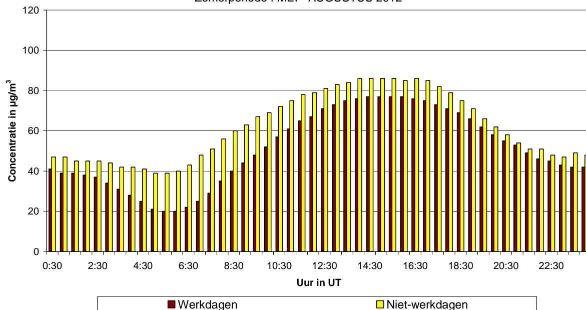
Fig. 47.a : St.-Agatha-Berchem : Gemiddeld dagverloop van de O 3 -concentratie op werkdagen en niet-werkdagen tijdens de periode mei - augustus 2012
