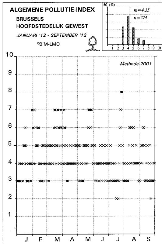
Fig. 60 : Subindexen voor NO 2 , O 3 en PM10 – Index Algemene Luchtkwaliteit Januari – September 2012
