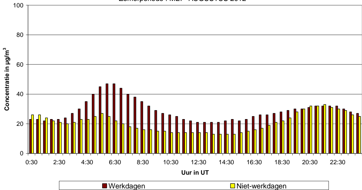
Fig. 52.b : St.-Katelijne : Gemiddeld dagverloop van de NO 2 -concentratie op werkdagen en niet-werkdagen tijdens de periode mei – augustus 2012
