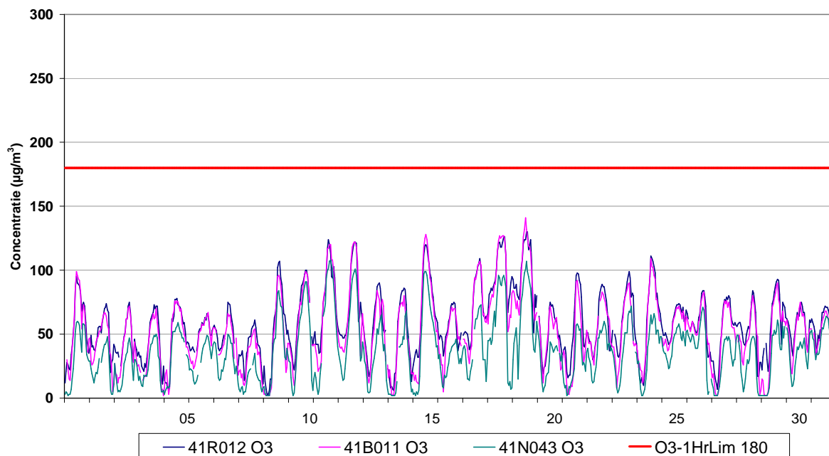
Fig. 6 : Evolutie van de uurwaarden voor ozon – Ukkel, Berchem en Voorhaven – Augustus 2012
