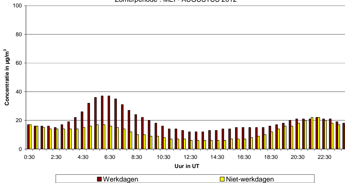
Fig. 47.b : St.-Agatha-Berchem : Gemiddeld dagverloop van de NO 2 -concentratie op werkdagen en niet-werkdagen tijdens de periode mei – augustus 2012
