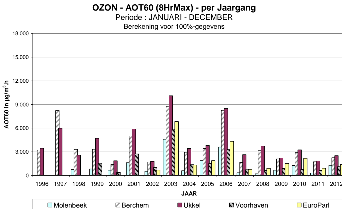
Fig. 24: Evolutie AOT60 in de tijd (1996-2012) Periode: JANUARI – DECEMBER (1996 – 2011) 2012 : Januari - September
