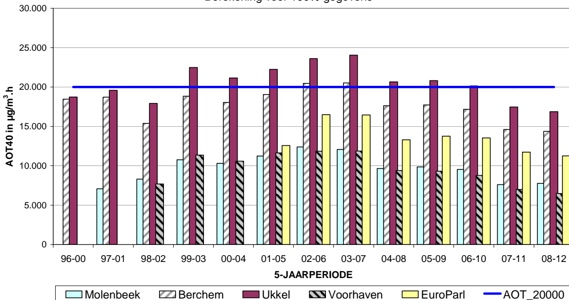
Fig. 16: Evolutie AOT40-AS in de tijd (1996-2012) AOT over de periode April – September, 8-20 h MET - Midden-Europese tijd Resultaten per jaar en gemiddeld over 5 jaar Berekende AOT-waarden (100%-beschikbaarheid gegevens)
