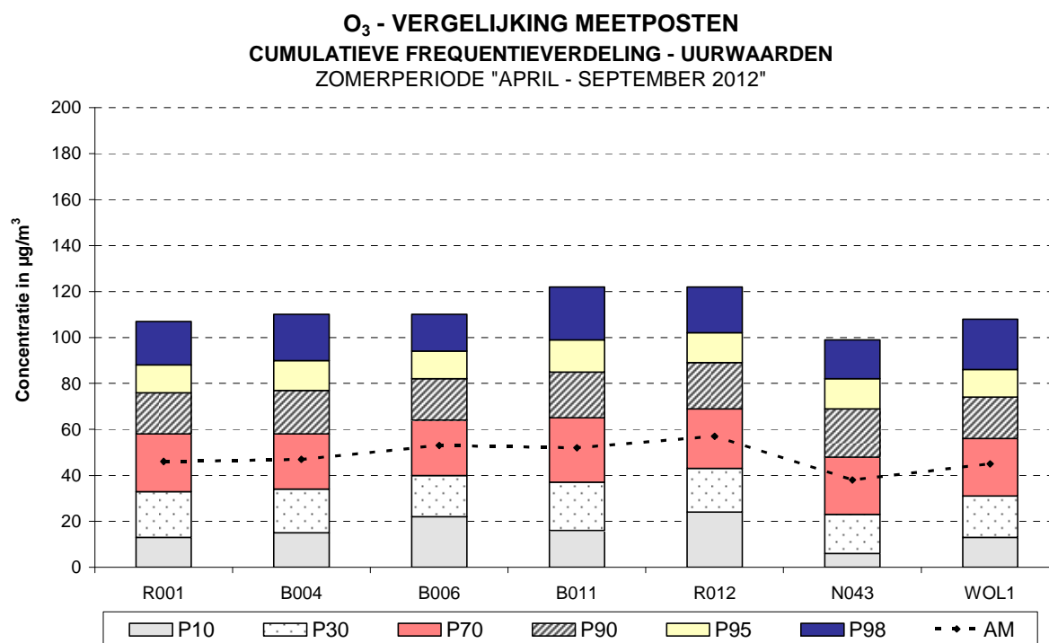
Fig. 32 : Ozon - Cumulatieve frequentieverdeling uurwaarden : april - september 2012
