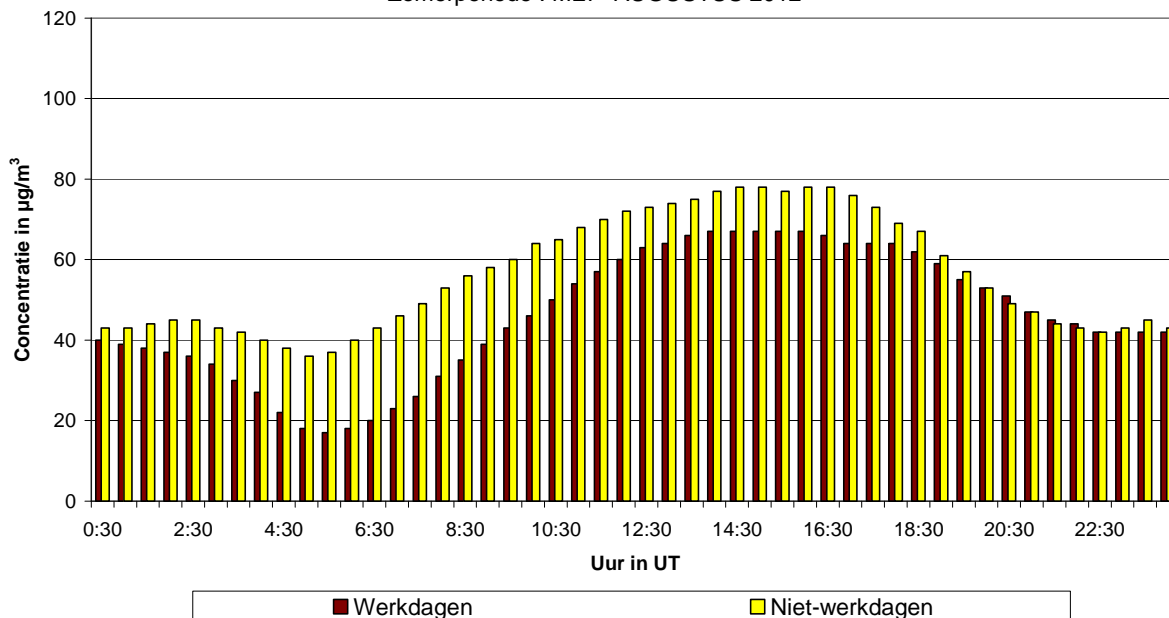
Fig. 48.a : Molenbeek : Gemiddeld dagverloop van de O 3 -concentratie op werkdagen en niet-werkdagen tijdens de periode mei - augustus 2012
