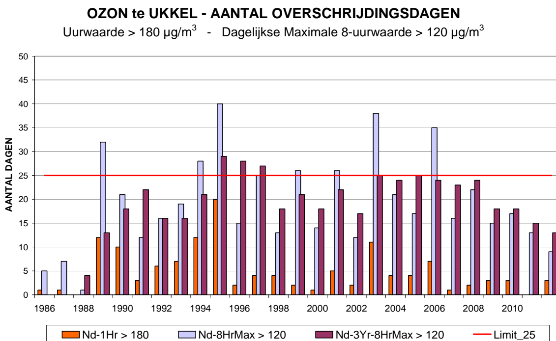
Fig. 19 : Ozon te Ukkel : aantal dagen met overschrijdingen Jaarperioden: 1 januari – 31 december (1986-2011) Voorlopige resultaten voor het jaar 2012 (1 januari – 30 september)
