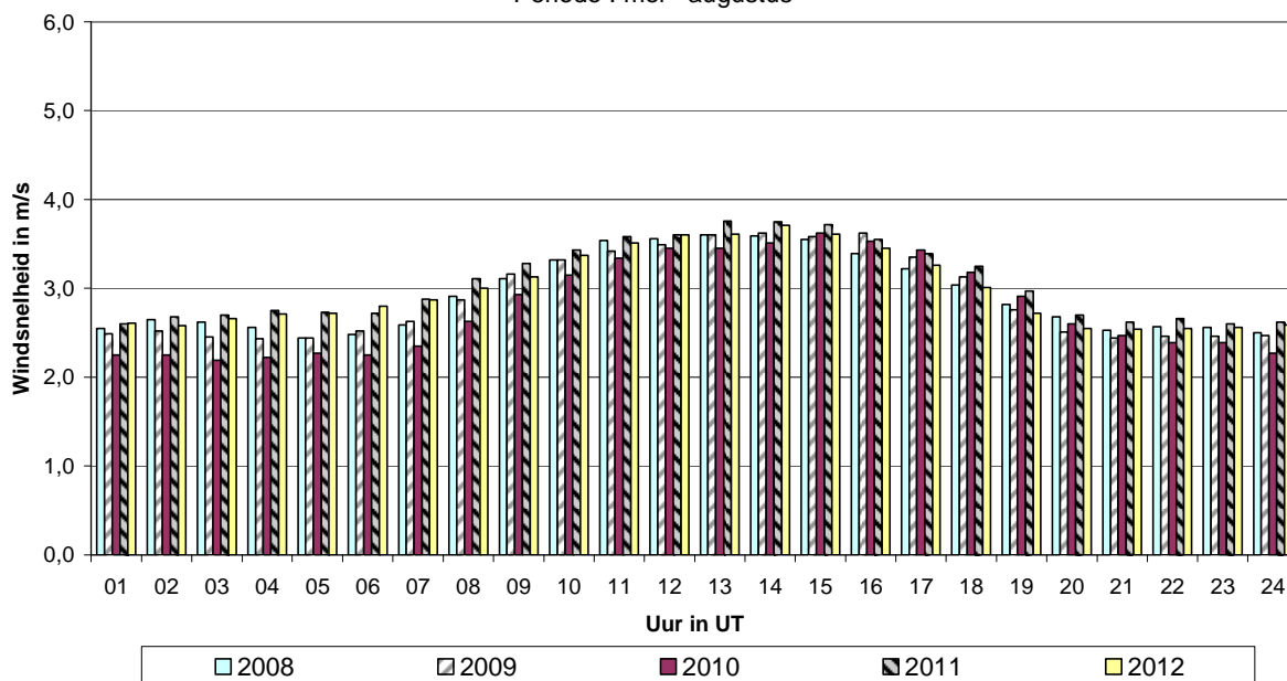
Gemiddeld dagverloop Windsnelheid Vergelijking 2008, 2009, 2010, 2011 en 2012 Periode : mei - augustus
