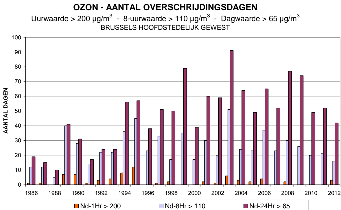
Fig. 25 : Ozon : aantal dagen met overschrijdingen (richtlijn 92/72/EG) Periode : januari - december (1986 t/m 2011) 2012 : Januari – September
