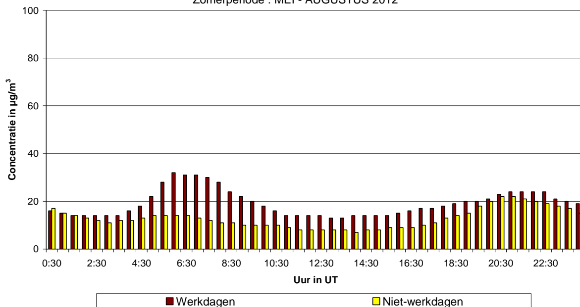
Fig. 46.b : Ukkel : Gemiddeld dagverloop van de NO 2 -concentratie op werkdagen en niet-werkdagen tijdens de periode mei – augustus 2012
