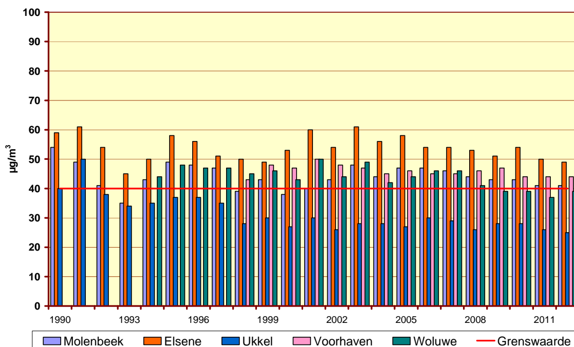
Fig. 27.a : NO 2 - Evolutie jaargemiddelde concentratie Jaarperiodes 1990-2011 en "Oktober 2011 – September 2012"
