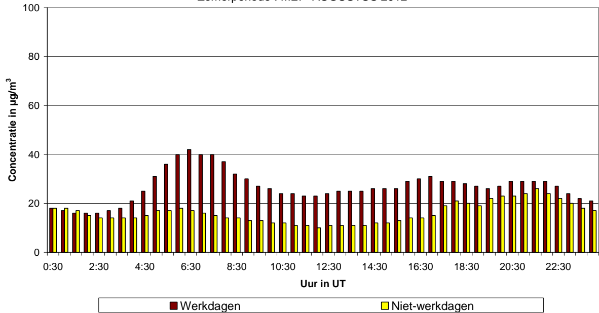
Fig. 53.a : Eastman-Belliard : Gemiddeld dagverloop van de NO 2 -concentratie op werkdagen en niet-werkdagen tijdens de periode mei - augustus 2012
