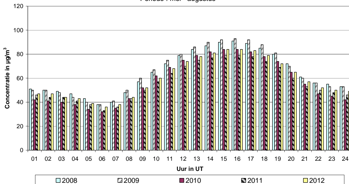
Fig. 35 : Gemiddeld dagverloop O 3 -concentratie te Ukkel (R012) Evolutie tijdens recente zomerperiodes (2008-2012)
