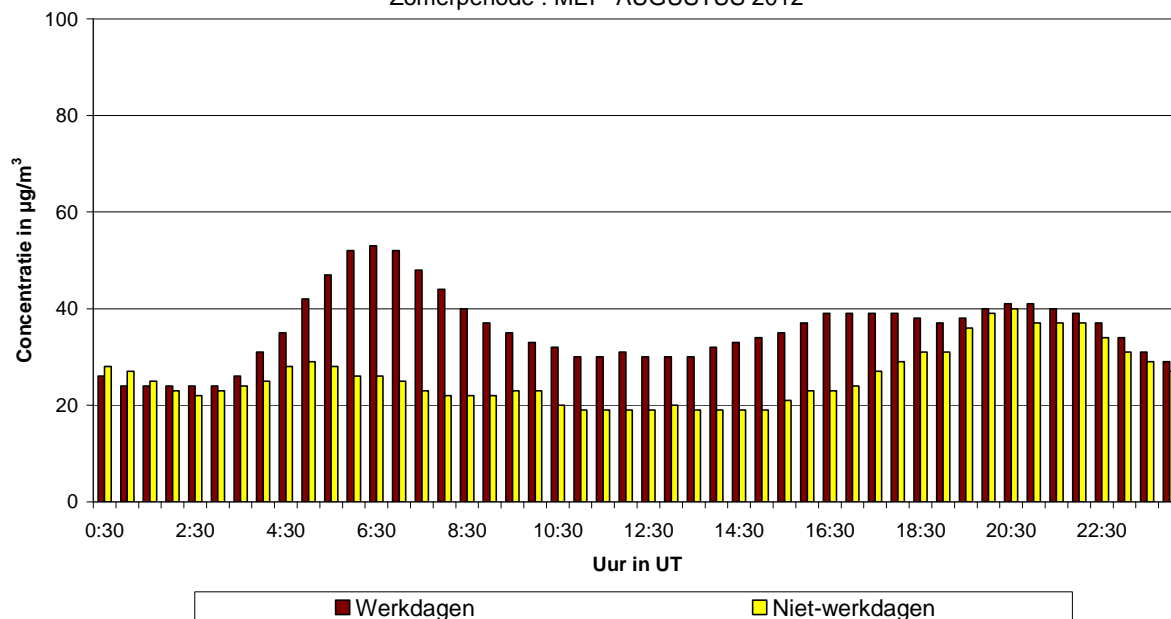
Fig. 50.b : St.-Lambr.-Woluwe : Gemiddeld dagverloop van de NO 2 -concentratie op werkdagen en niet-werkdagen tijdens de periode mei – augustus 2012
