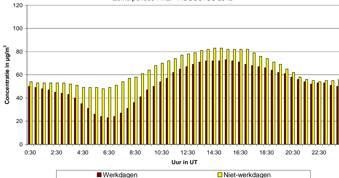
Fig. 51.a : Europees Parlement : Gemiddeld dagverloop van de O 3 -concentratie op werkdagen en niet-werkdagen tijdens de periode mei - augustus 2012
