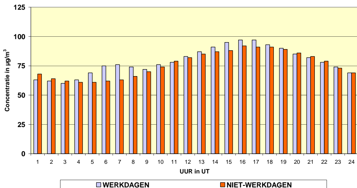
Fig. 69: [O 3 + NO 2 ] – Evolutie Dagverloop voor werkdagen en niet-werkdagen Meetposten Ukkel en Voorhaven - Periode “mei – augustus 2012”
