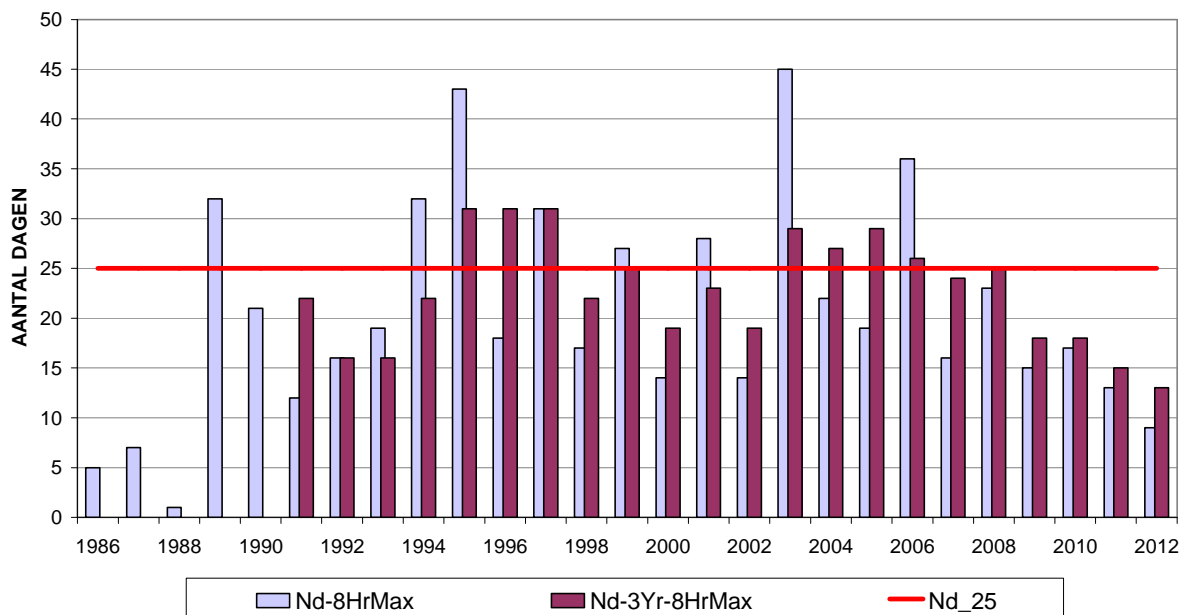
Fig. 14 : Ozon - Evolutie aantal overschrijdingsdagen in het Brussels Hoofdstedelijk Gewest Streefwaarde voor de gezondheid: Maximale 8-uurwaarde > 120 µg/m 3 Periode : Januari – December (1986-2011). [2012]: Januari – September
