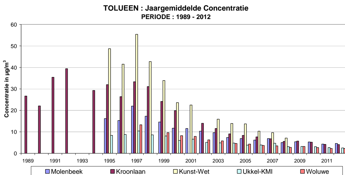
Fig. 29 : Tolueen - Evolutive jaargemiddelde concentratie Periode : Januari – December (1989-2011) en 'Oktober 2011 – September 2012'
