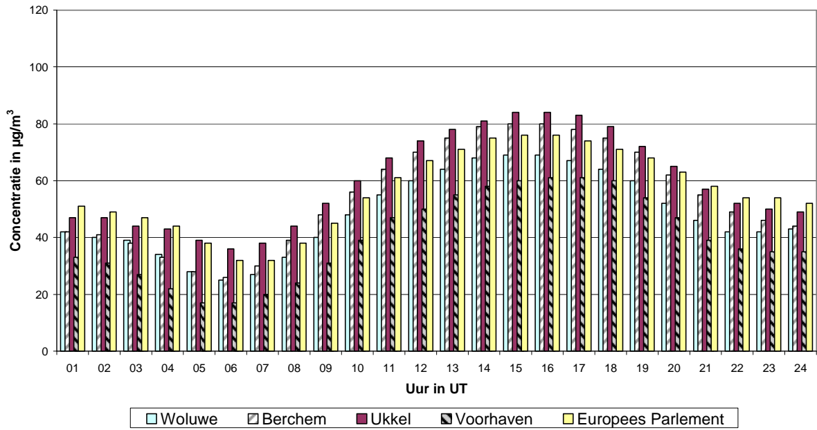
Fig. 8 : Gemiddeld dagverloop van de O 3 -concentratie in de periode mei – augustus 2012
