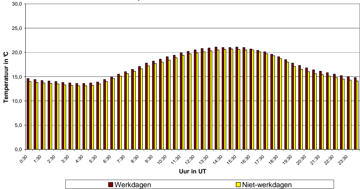
Fig. 55.a : Ukkel : Gemiddeld dagverloop van de temperatuur op werkdagen en niet-werkdagen tijdens de periode mei – augustus 2012
