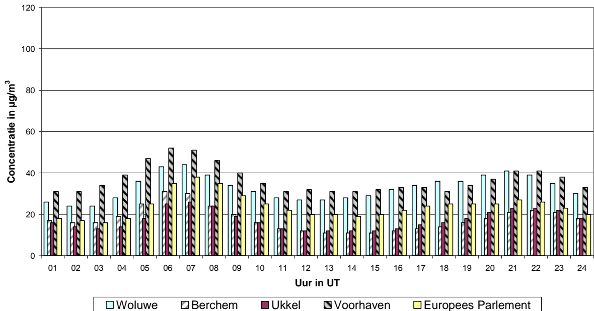
Fig. 9 : Gemiddeld dagverloop van de NO 2 -concentratie in de periode mei – augustus 2012
