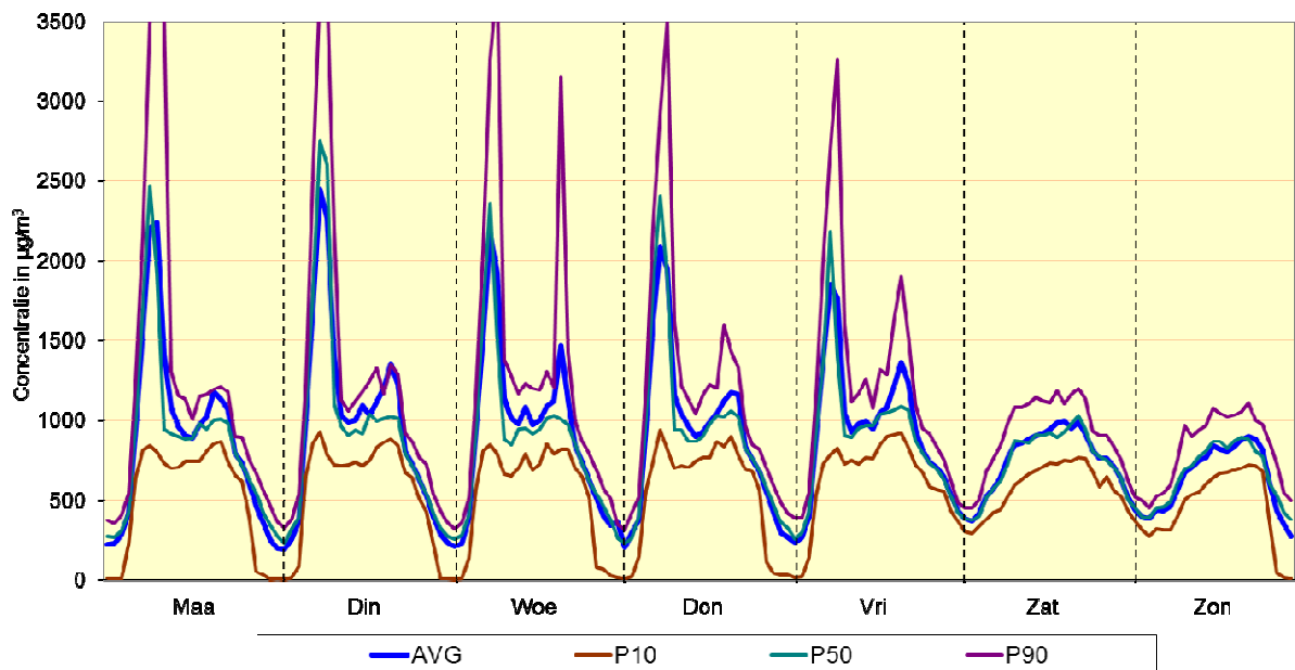
Fig. 25 : Meetpost 41LEC1 (centrum) - Gemiddeld weekverloop voor NO Vergelijking winterperiode 2012 - 2013 en zomerperiode 2013
