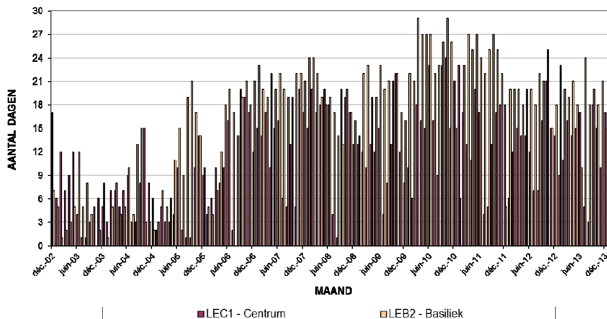
Fig. 13 : NO 2 – Halfuurswaarden > 850 µg/m 3 . Totaal aantal overschrijdingen per maand en aantal dagen per maand met overschrijding (december 2002 – december 2013)
