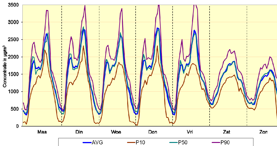
Fig. 26 : Meetpost 41LEB2 (basiliek) - Gemiddeld weekverloop voor NO Vergelijking winterperiode 2012 - 2013 en zomerperiode 2013
