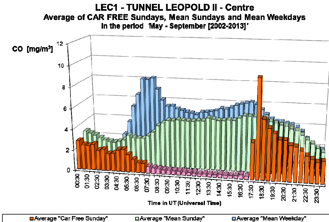
Fig. 31.b : CO in de Leopold II tunnel, richting Centrum – Gemiddelde Dagprofiel van de twaalf autoluwe zondagen en van alle zondagen en werkdagen in de periodes ‘mei – september 2002-2013’
