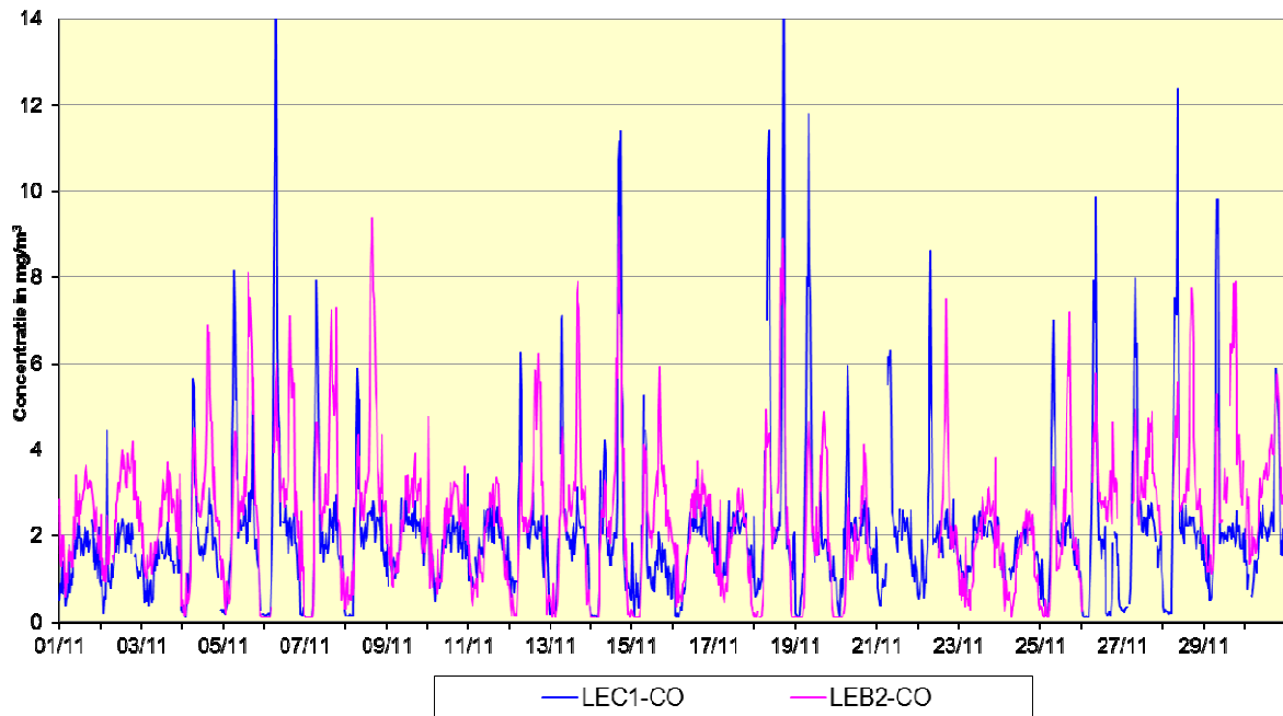
Fig. 3: CO - Evolutie van de uurwaarden en de halfuurwaarden tijdens de maand november 2013 Meetplaats 41LEC1, richting Centrum - Meetplaats 41LEB2, richting Basiliek
