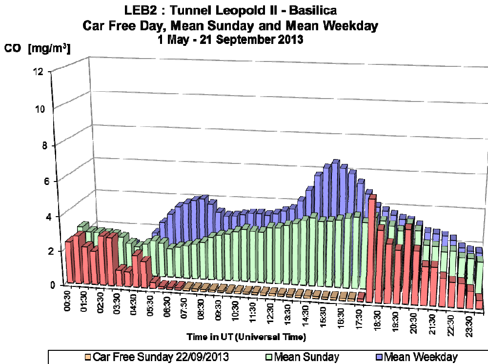
Fig. 32.a : CO in de Leopold II tunnel, richting Basiliek – Dagprofiel autoluwte zondag 22-09-2013, gemiddelde zondag en een gemiddelde werkdag in de periode 'mei – september 2013'
