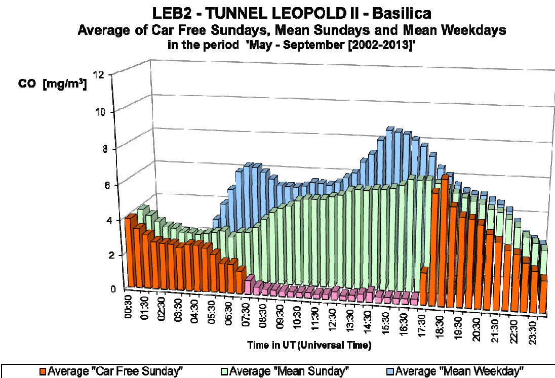
Fig. 32.b : CO in de Leopold II tunnel, richting Basiliek – Gemiddelde Dagprofiel van de twaalf autoluwte zondagen en van alle zondagen en werkdagen in de periodes 'mei – september 2002-2013'
