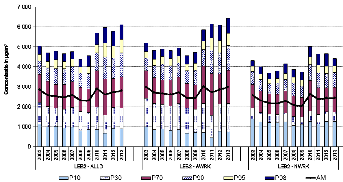
Fig. 8 : NO x - Cumulatieve Frequentieverdeling Jurwaarden in beide meetposten van de Leopold II tunnel. Selectie alle dagen , alle werkdagen en alle niet-werkdagen Jaarperiodes 2003 t/m 2013
