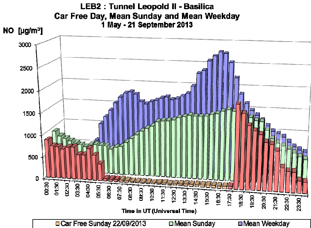
Fig. 30.a : NO in de Leopold II tunnel, richting Basiliek – Dagprofiel autoluwe zondag 22-09-2013, gemiddelde zondag en een gemiddelde werkdag in de periode ‘mei – september 2013’
