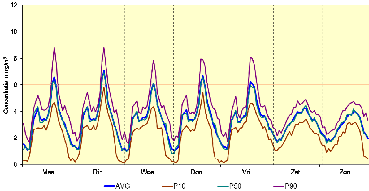
Fig. 24 : Meetpost 41LEB2 (basiliek) - Gemiddeld weekverloop voor CO Vergelijking winterperiode 2012 - 2013 en zomerperiode 2013
