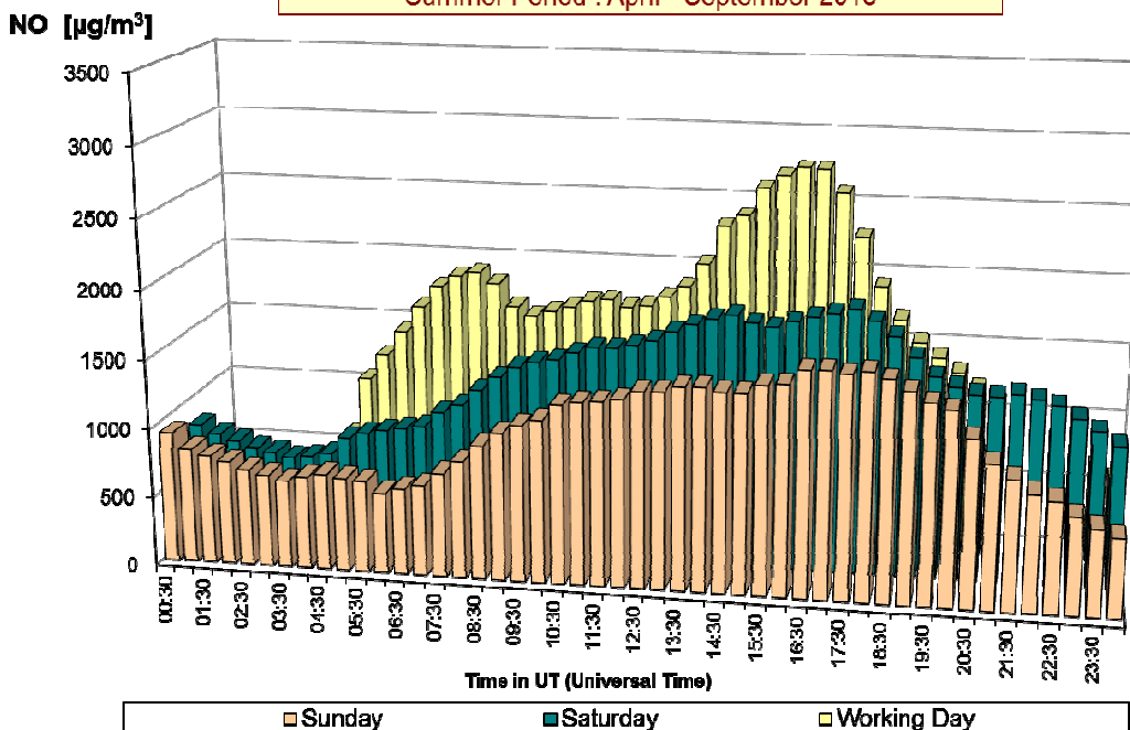
Fig. 18 : NO-dagverloop in de meetpost 41LEB2 (richting basiliek) Vergelijking voor een gemiddelde zondag, zaterdag en werkdag Winterperiode 2012-2013 en zomerperiode 2013
