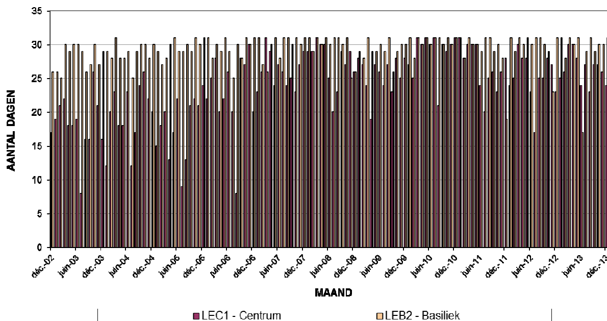
Fig. 14 : NO 2 -Uurwaarden > 400 µg/m 3 . Totaal aantal overschrijdingen per maand en aantal dagen per maand met overschrijding (december 2002 – december 2013)
