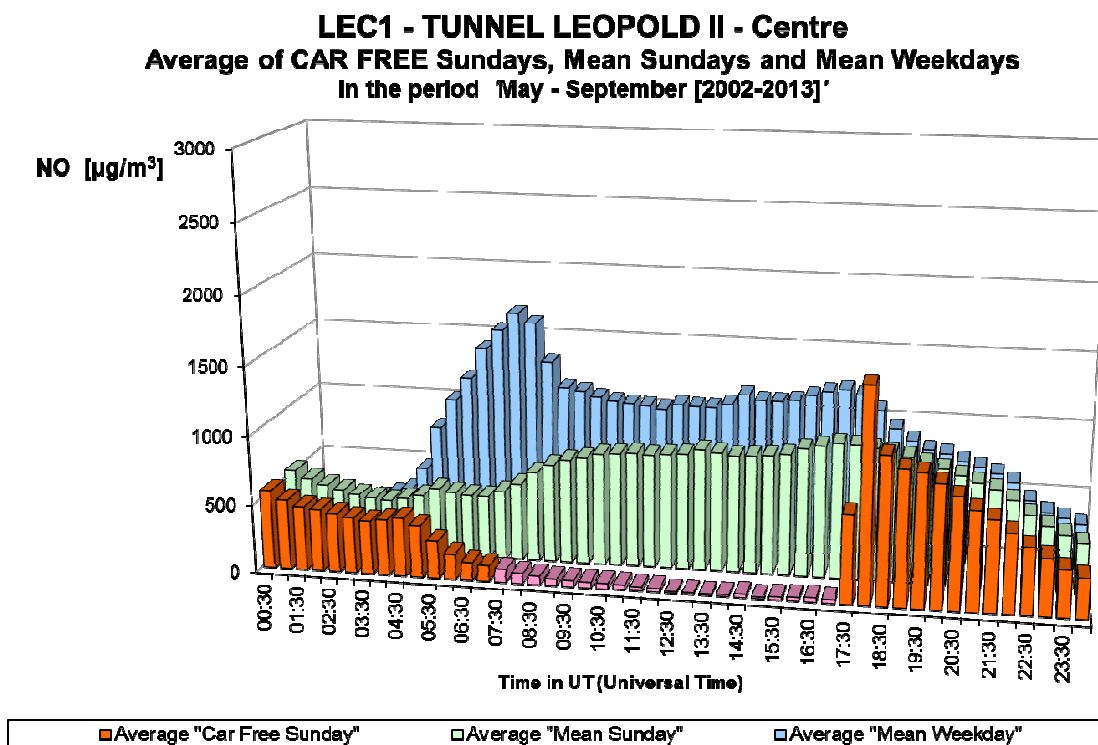
Fig. 29.b : NO in de Leopold II tunnel, richting Centrum – Gemiddelde Dagprofiel van de twaalf autoluwe zondagen en van alle zondagen en werkdagen in de periodes ‘mei – september 2002-2013’
