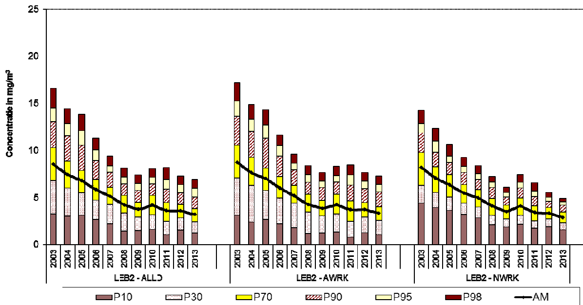
Fig. 6 : CO - Cumulatieve Frequentieverdeling Jurwaarden in beide meetposten van de Leopold II tunnel. Selectie alle dagen , alle werkdagen en alle niet-werkdagen Jaarperiodes 2003 t/m 2013
