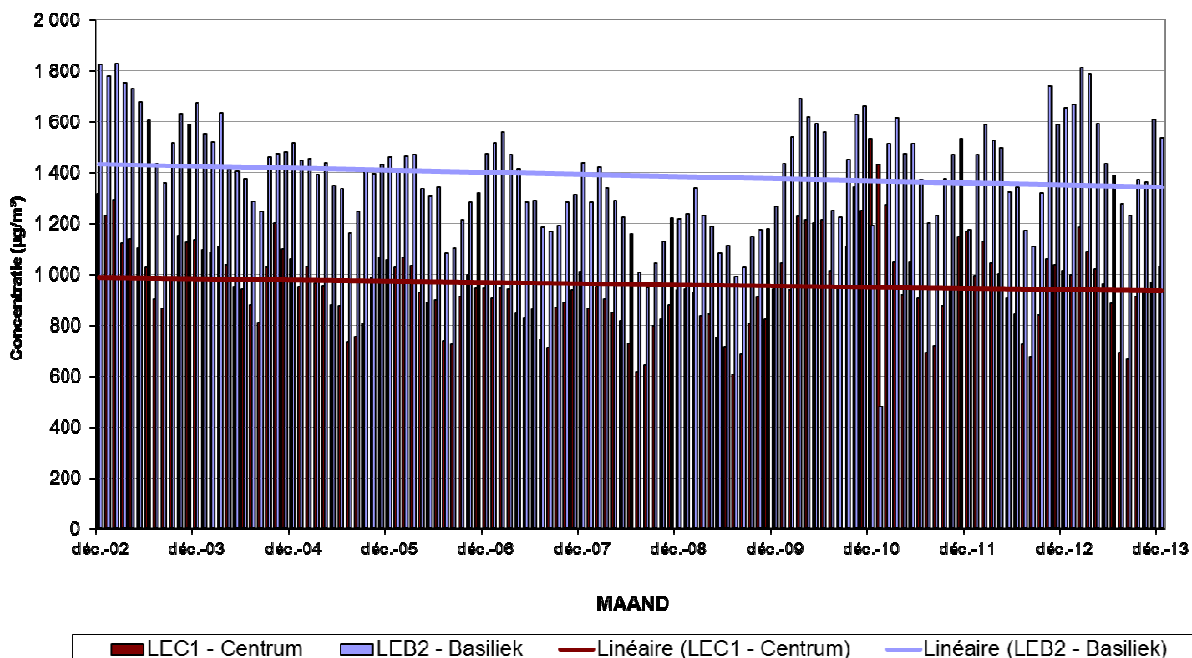
Fig. 9 : NO 2 en NO - Evolutie maandgemiddelde concentratie in beide meetposten van de Leopold II tunnel. Periode "December 2002 – December 2013"
