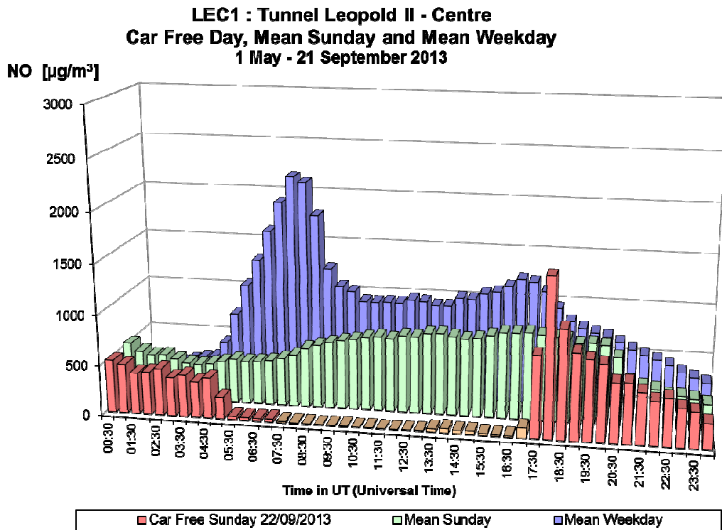
Fig. 29.a : NO in de Leopold II tunnel, richting Centrum – Dagprofiel autoluwe zondag 22-09-2013, gemiddelde zondag en gemiddelde werkdag in de periode ‘mei – september 2013’
