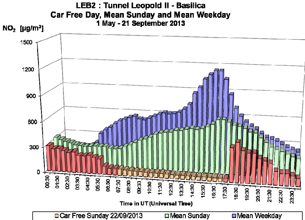
Fig. 28.a : NO 2 in de Leopold II tunnel, richting Basiliek – Dagprofiel autoluwe zondag 22-09-2013, gemiddelde zondag en een gemiddelde werkdag in de periode ‘mei – september 2013’
