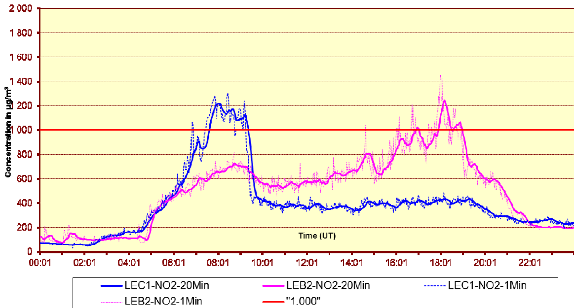
Fig. 4: NO 2 - evolutie minuutwaarden en voortschrijdend 20-minuutsgemiddelde in beide meetposten van de Leopold II tunnel Dinsdag 01 oktober 2013 en dinsdag 19 november 2013
