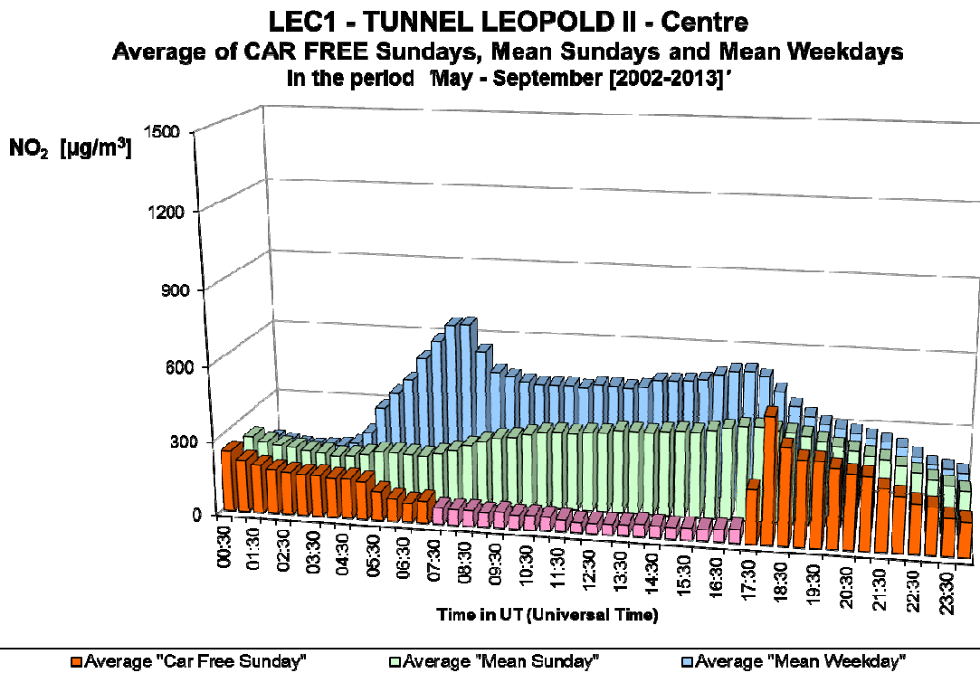
Fig. 27.b : NO 2 in de Leopold II tunnel, richting Centrum – Gemiddelde Dagprofiel van de twaalf autoluwe zondagen en van alle zondagen en werkdagen in de periodes ‘mei – september 2002-2013’
