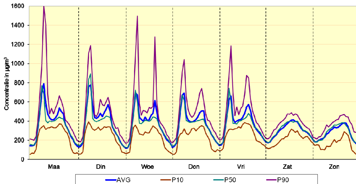
Fig. 21 : Meetpost 41LEC1 (centrum) - Gemiddeld weekverloop voor NO 2 Vergelijking winterperiode 2012 - 2013 en zomerperiode 2013
