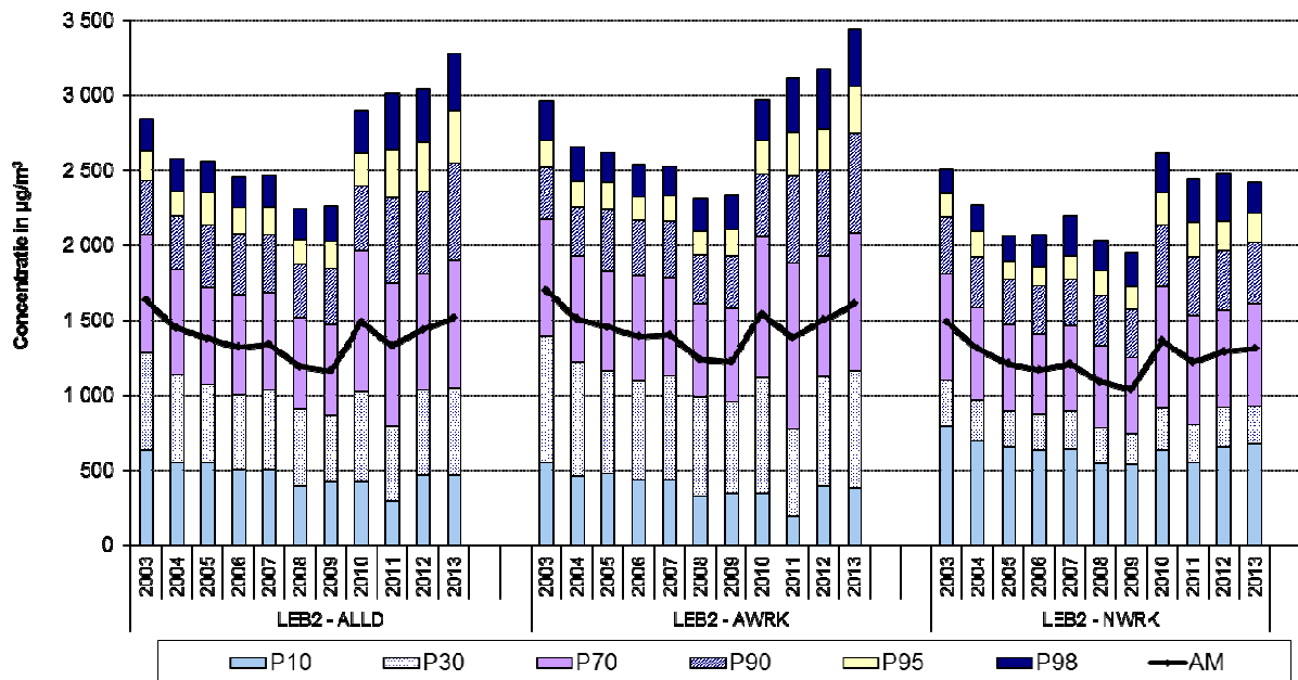
Fig. 7 : NO - Cumulatieve Frequentieverdeling Jurwaarden in beide meetposten van de Leopold II tunnel. Selectie alle dagen , alle werkdagen en alle niet-werkdagen Jaarperiodes 2003 t/m 2013
