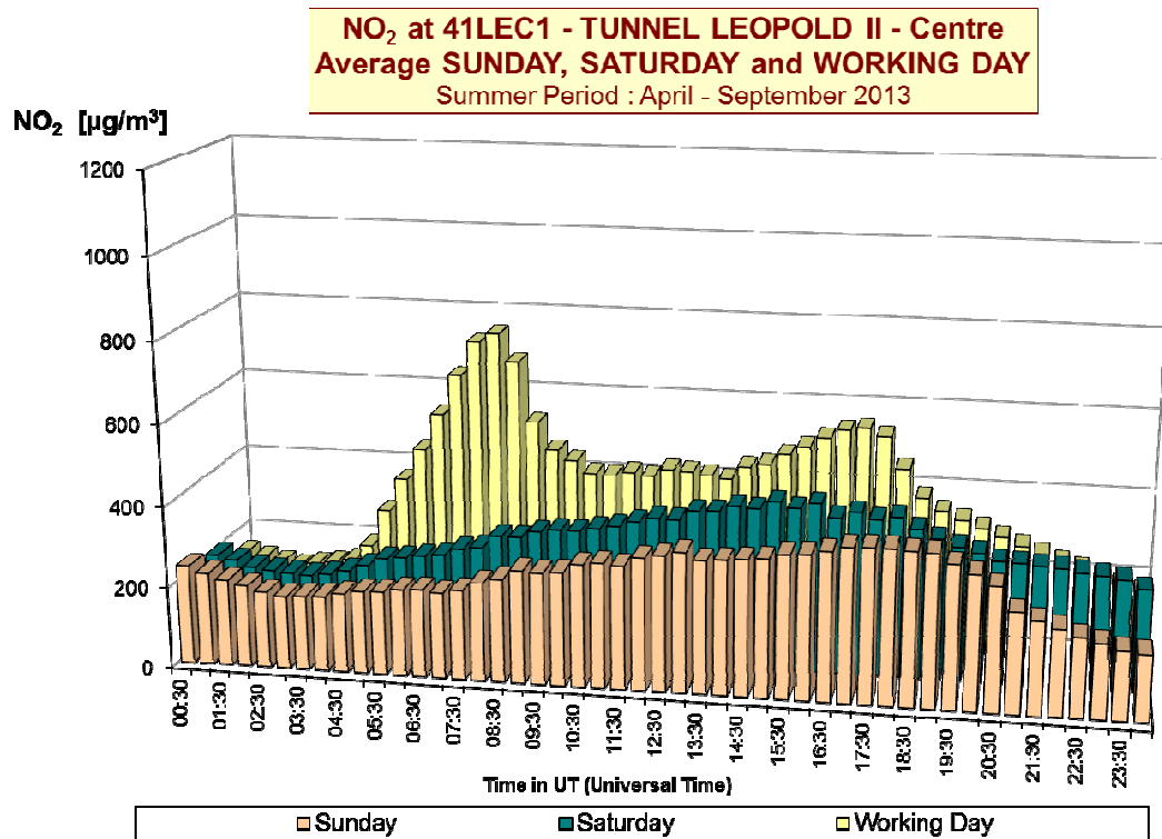
Fig. 15 : NO 2 -dagverloop in de meetpost 41LEC1 (richting centrum) Vergelijking voor een gemiddelde zondag, zaterdag en werkdag Winterperiode 2012-2013 en zomerperiode 2013
