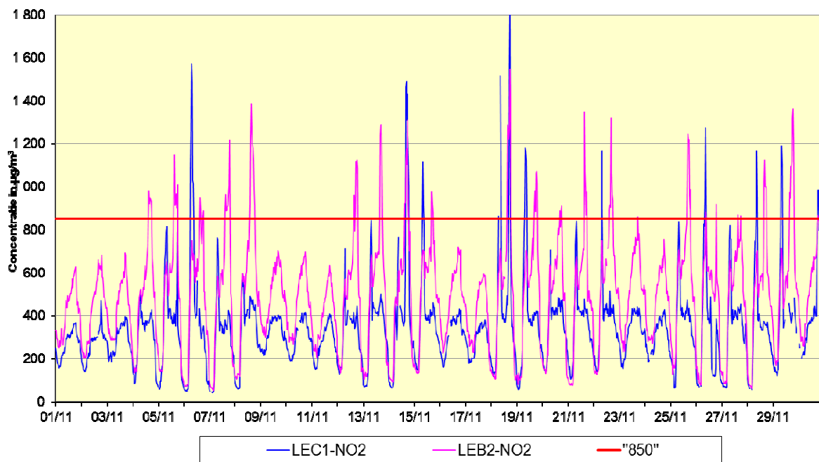
Fig. 1: NO 2 - Evolutie van de uurwaarden en de halfuurwaarden tijdens de maand november 2013 Meetplaats 41LEC1, richting Centrum - Meetplaats 41LEB2, richting Basiliek
