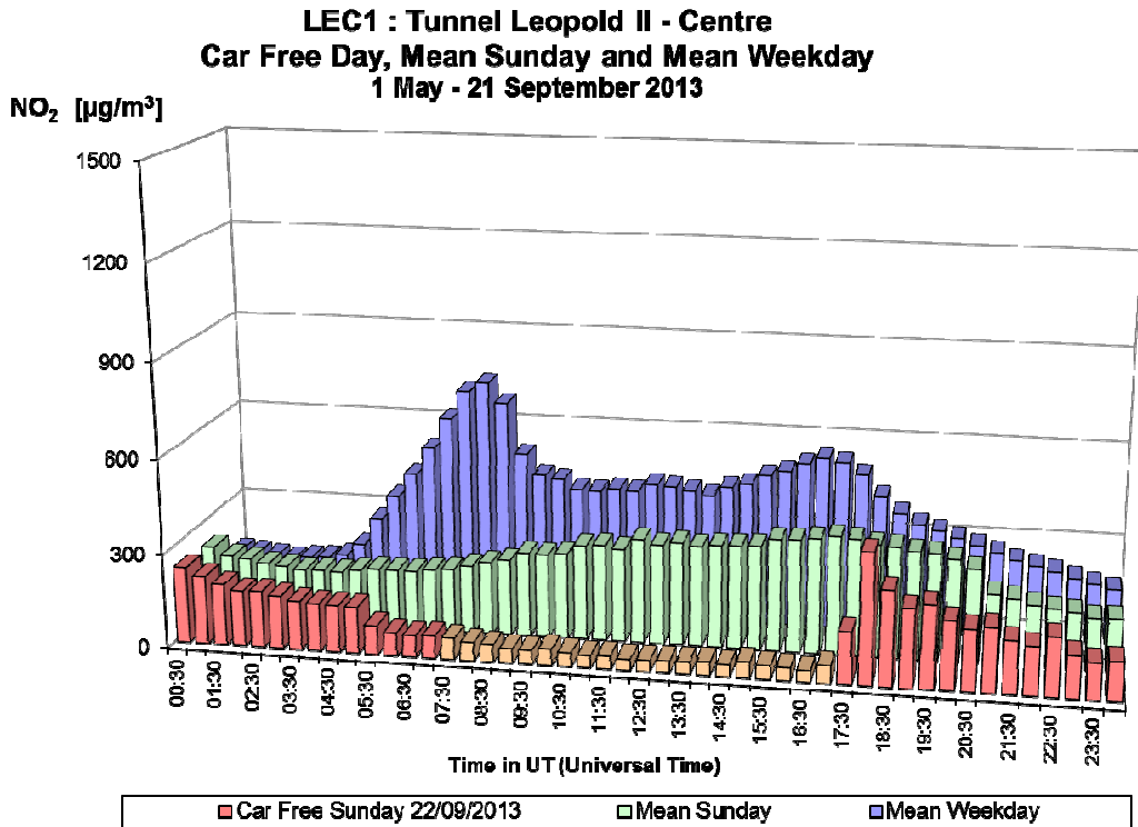
Fig. 27.a : NO 2 in de Leopold II tunnel, richting Centrum – Dagprofiel autoluwe zondag 22-09-2013, gemiddelde zondag en gemiddelde werkdag in de periode ‘mei – september 2013’
