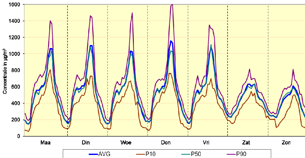
Fig. 22 : Meetpost 41LEB2 (basiliek) - Gemiddeld weekverloop voor NO 2 Vergelijking winterperiode 2012 - 2013 en zomerperiode 2013
