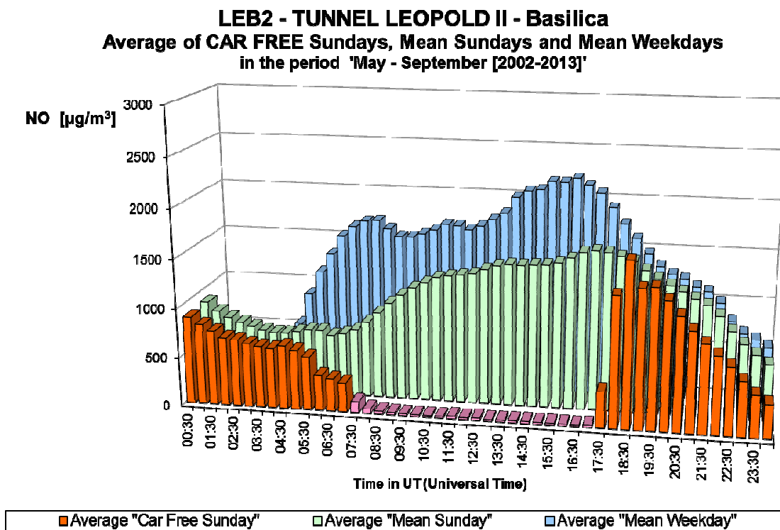
Fig. 30.b : NO in de Leopold II tunnel, richting Basiliek – Gemiddelde Dagprofiel van de twaalf autoluwe zondagen en van alle zondagen en werkdagen in de periodes ‘mei – september 2002-2013’
