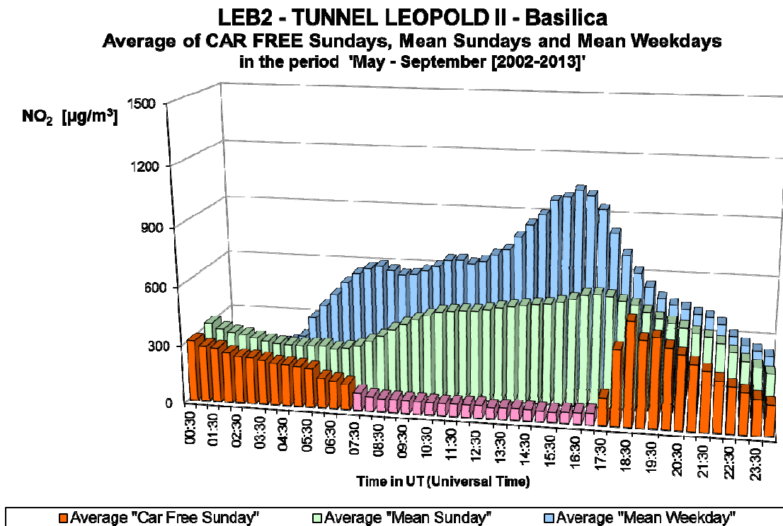
Fig. 28.b : NO 2 in de Leopold II tunnel, richting Basiliek – Gemiddelde Dagprofiel van de twaalf autoluwe zondagen en van alle zondagen en werkdagen in de periodes ‘mei – september 2002-2013’
