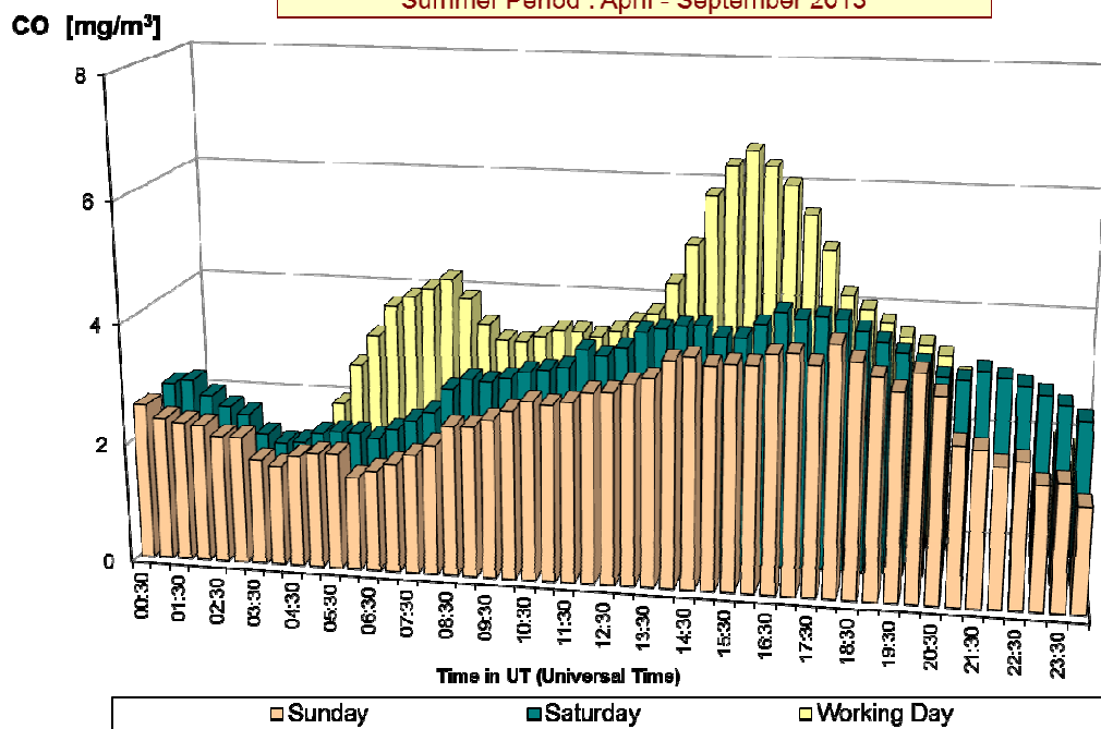
Fig. 20 : CO-dagverloop in de meetpost 41LEB2 (richting basiliek) Vergelijking voor een gemiddelde zondag, zaterdag en werkdag Winterperiode 2012-2013 en zomerperiode 2013
