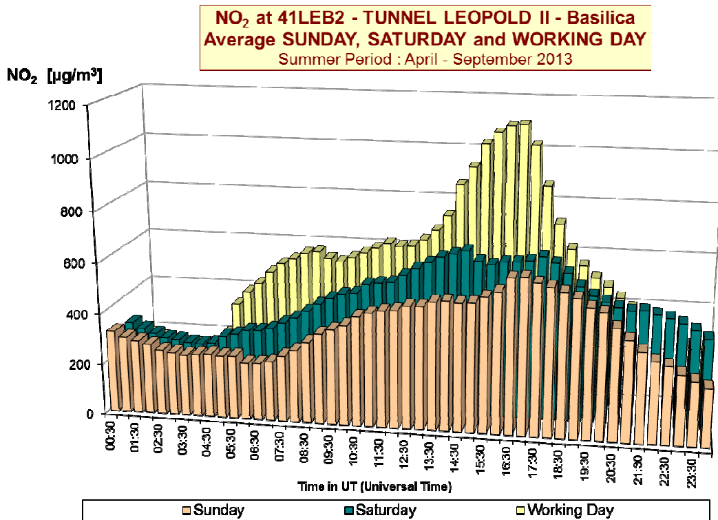
Fig. 16 : NO 2 -dagverloop in de meetpost 41LEB2 (richting basiliek) Vergelijking voor een gemiddelde zondag, zaterdag en werkdag Winterperiode 2012-2013 en zomerperiode 2013
