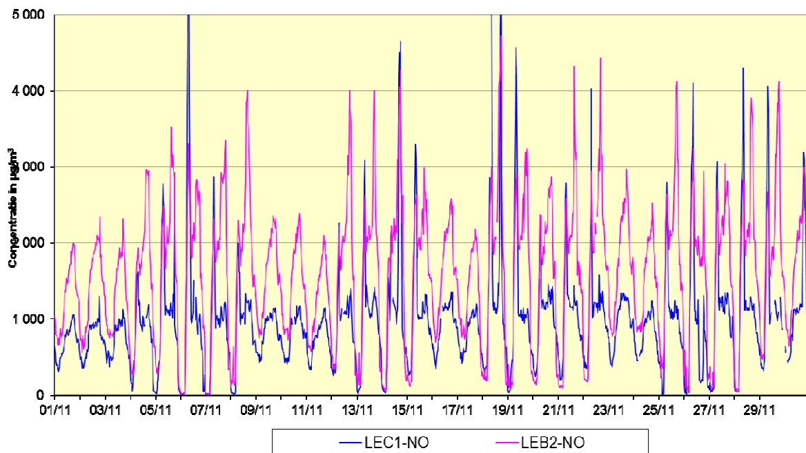
Fig. 2: NO - Evolutie van de uurwaarden en de halfuurswaarden tijdens de maand november 2013 Meetplaats 41LEC1, richting Centrum - Meetplaats 41LEB2, richting Basiliek
