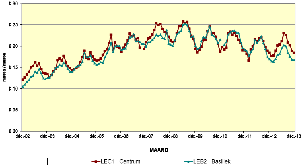
Fig. 11 : Evolutie van de verhouding NO 2 /NO x in beide meetposten van de Leopold II tunnel. Periode "December 2002 – December 2013"
