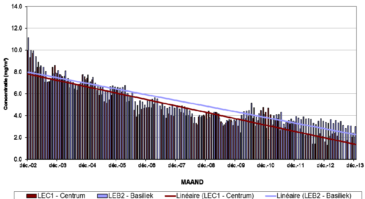
Fig. 10 : NO x en CO - Evolutive maandgemiddelde concentratie in beide meetposten van de Leopold II tunnel. Periode "December 2002 – December 2013"
